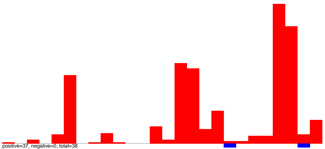
AeAeg_Aag2smallRNA_DENV1_rep2.24_35.rep
