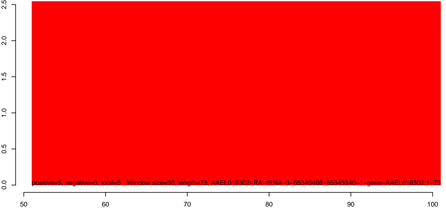
AeAeg_Aag2smallIRNA_DENV1_rep2.rep
