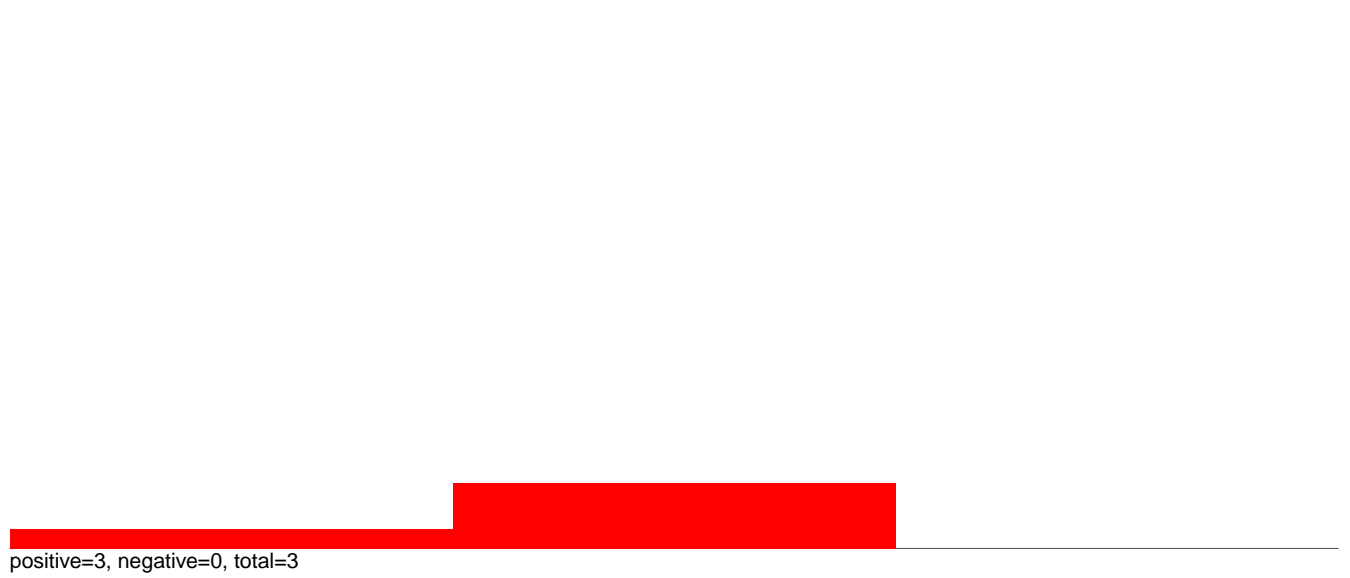
AeAeg_Aag2smallIRNA_DENV1_rep2.rep
