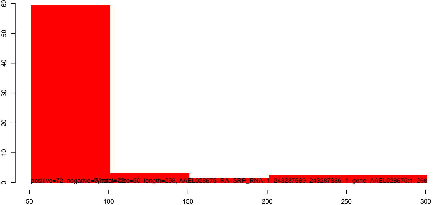
AeAeg_Aag2smallRNA_DENV1_rep2.rep
