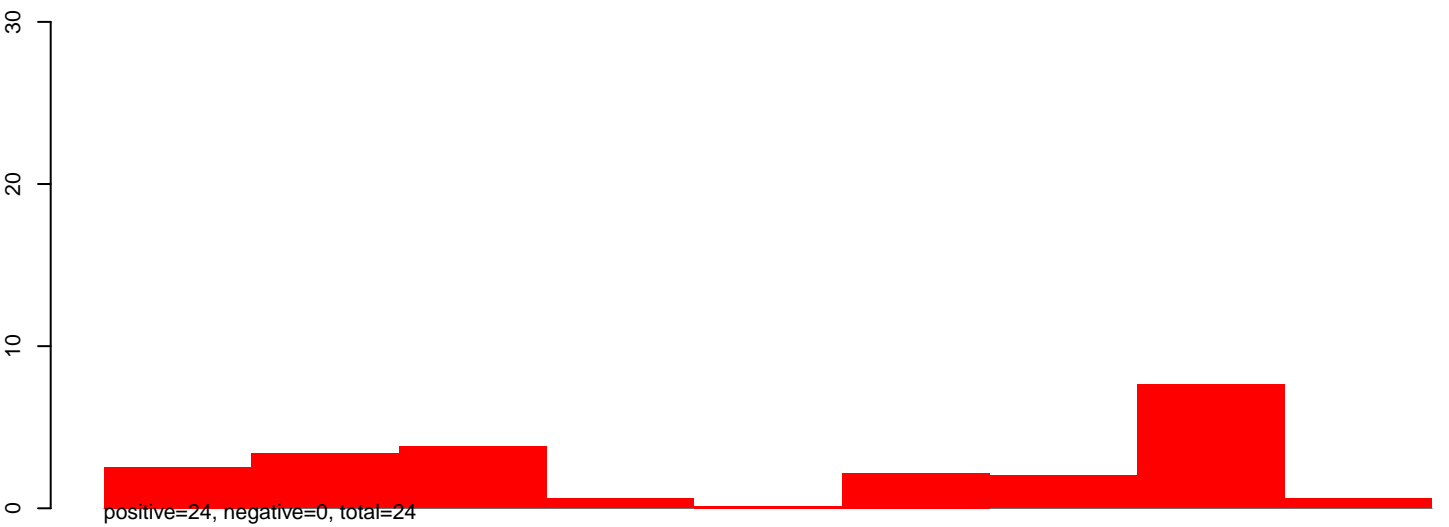
AeAeg_Aag2smallIRNA_DENV1_rep2.rep
