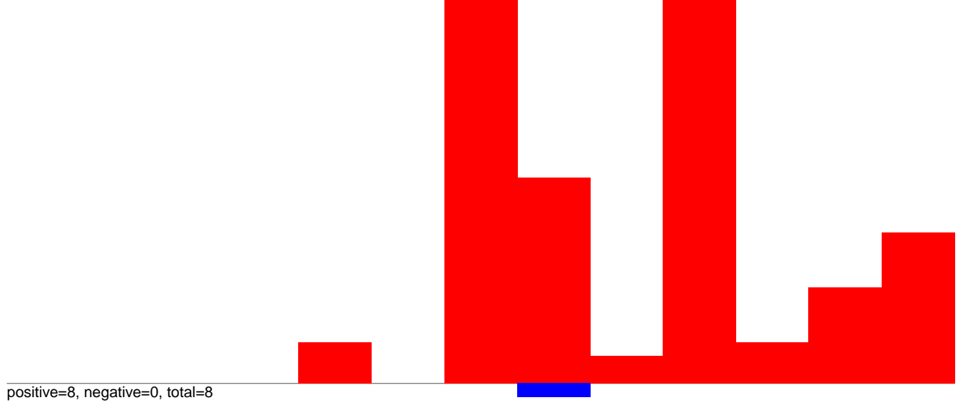
AeAeg_Aag2smallRNA_DENV1_rep2.24_35.rep
