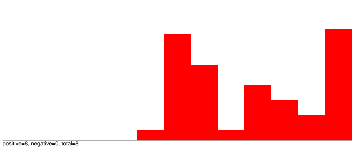
AeAeg_Aag2smallRNA_DENV1_rep2.rep
