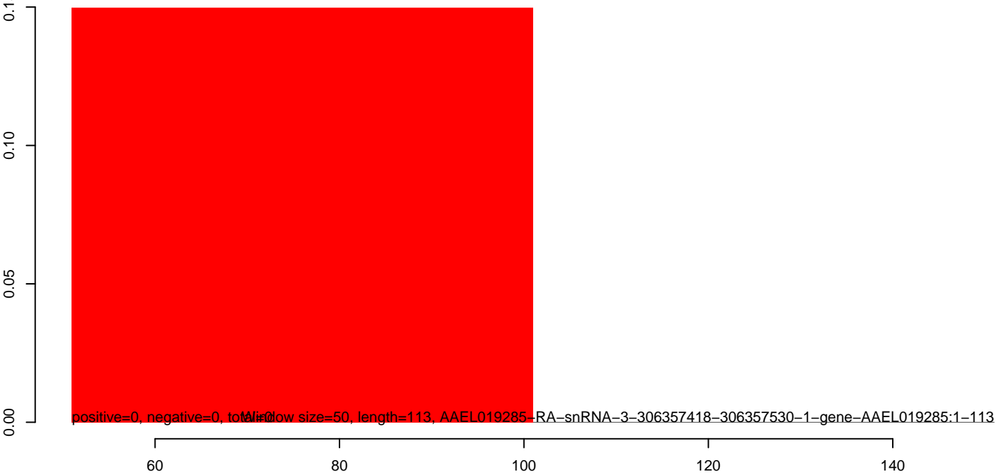
AeAeg_Aag2smallRNA_DENV1_rep2.rep
