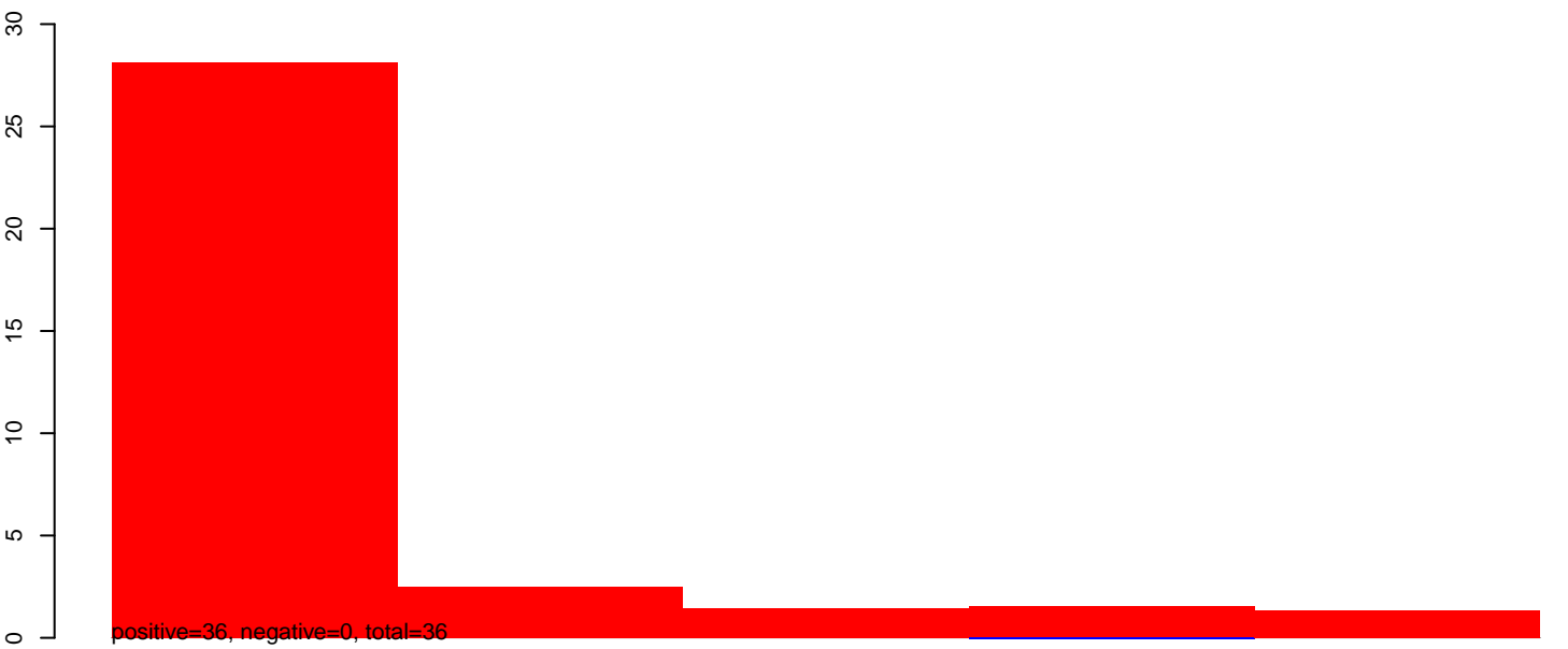
AeAeg_Aag2smallRNA_DENV1_rep2.24_35.rep
