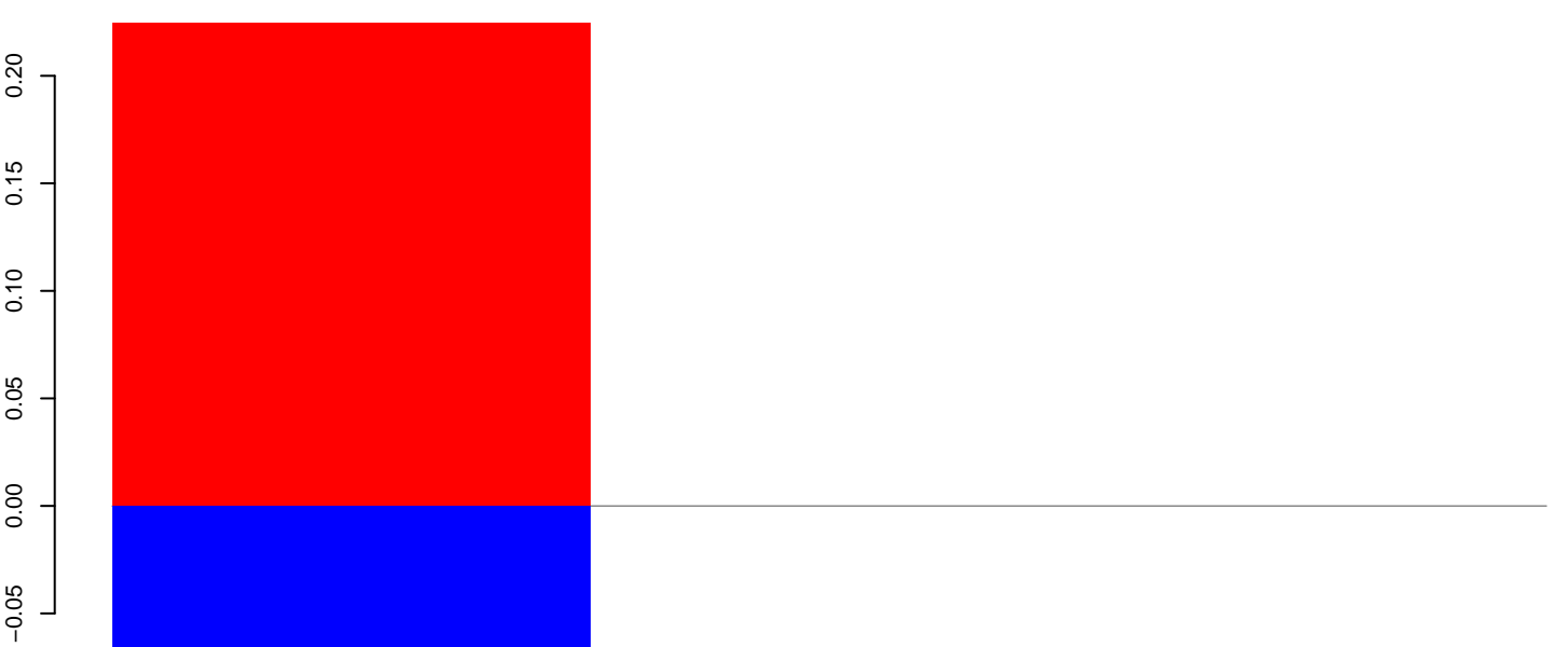
AeAeg_Aag2smallIRNA_DENV1_rep2.rep
