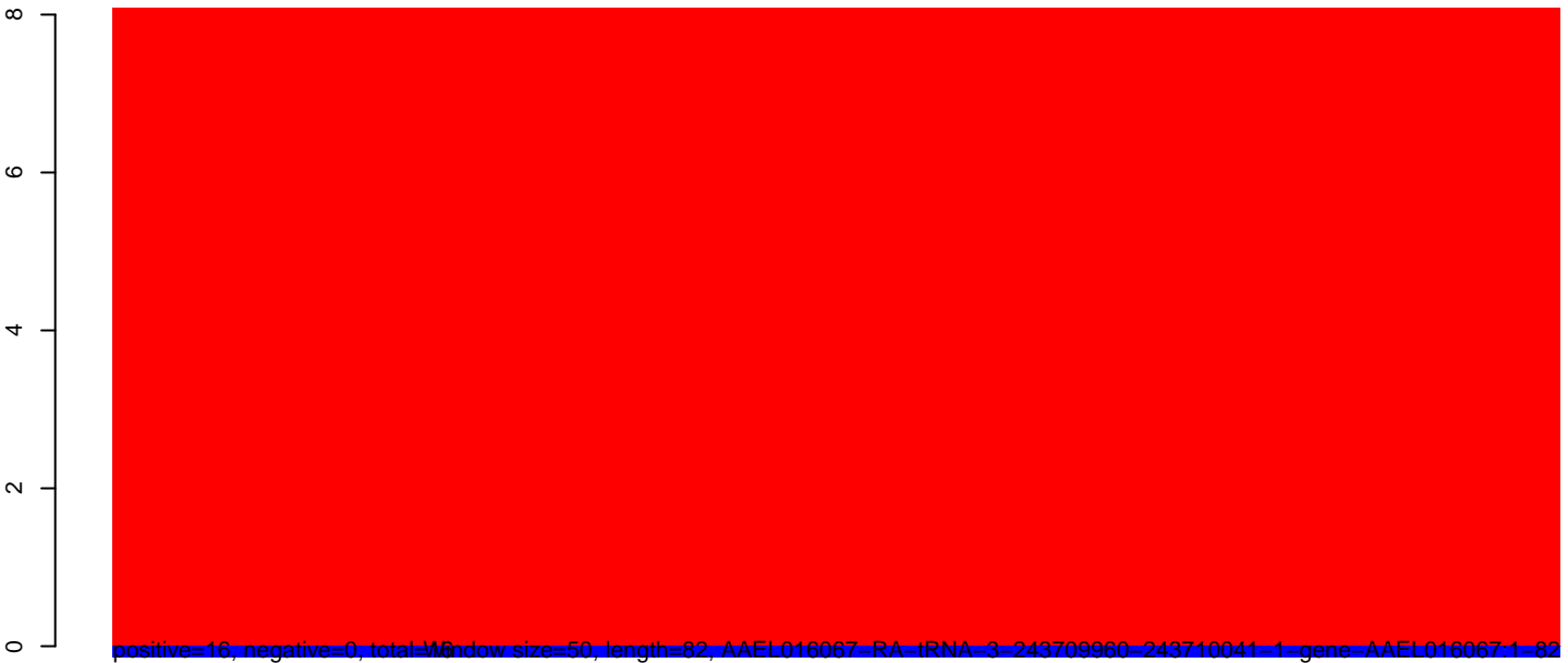
AeAeg_Aag2smallIRNA_DENV1_rep2.rep
