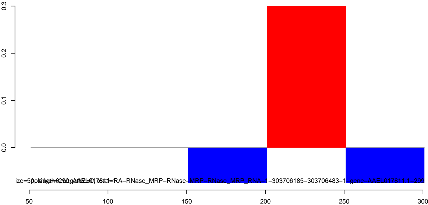
AeAeg_Aag2smallRNA_DENV1_rep2.rep
