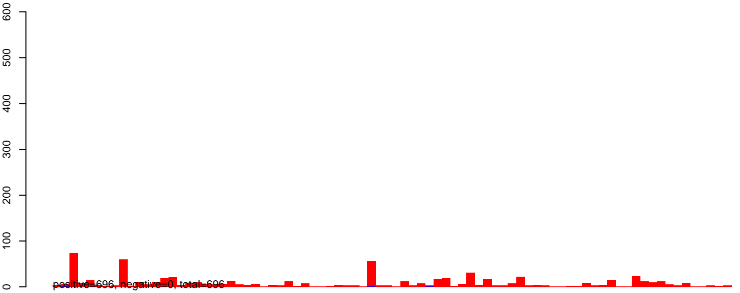
AeAeg_Aag2smallIRNA_DENV1_rep2.rep
