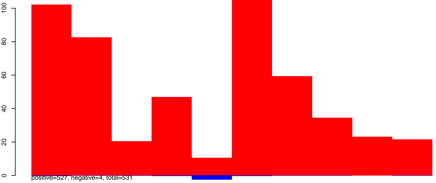
AeAeg_Aag2smallRNA_DENV1_rep2.24_35.rep
