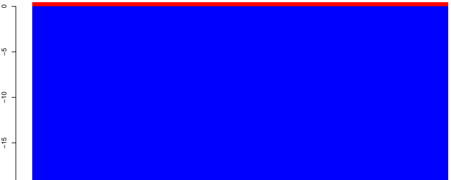
AeAeg_Aag2smallIRNA_DENV1_rep2.rep
