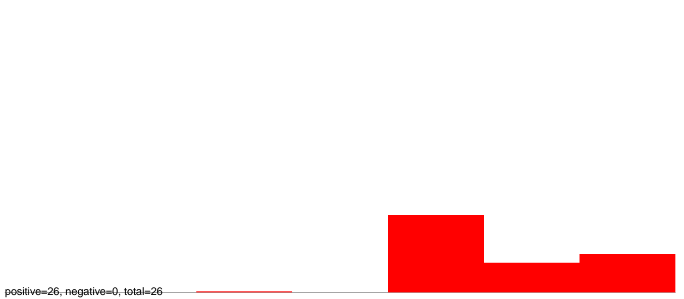
AeAeg_Aag2smallIRNA_DENV1_rep2.rep
