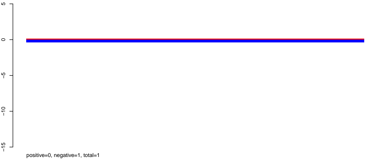
AeAeg_Aag2smallIRNA_DENV1_rep2.rep
