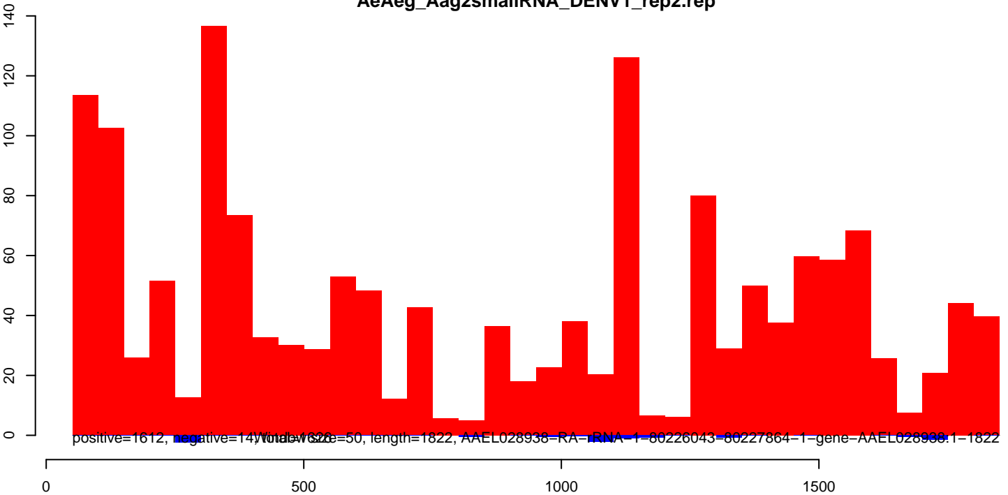
AeAeg_Aag2smallIRNA_DENV1_rep2.rep
