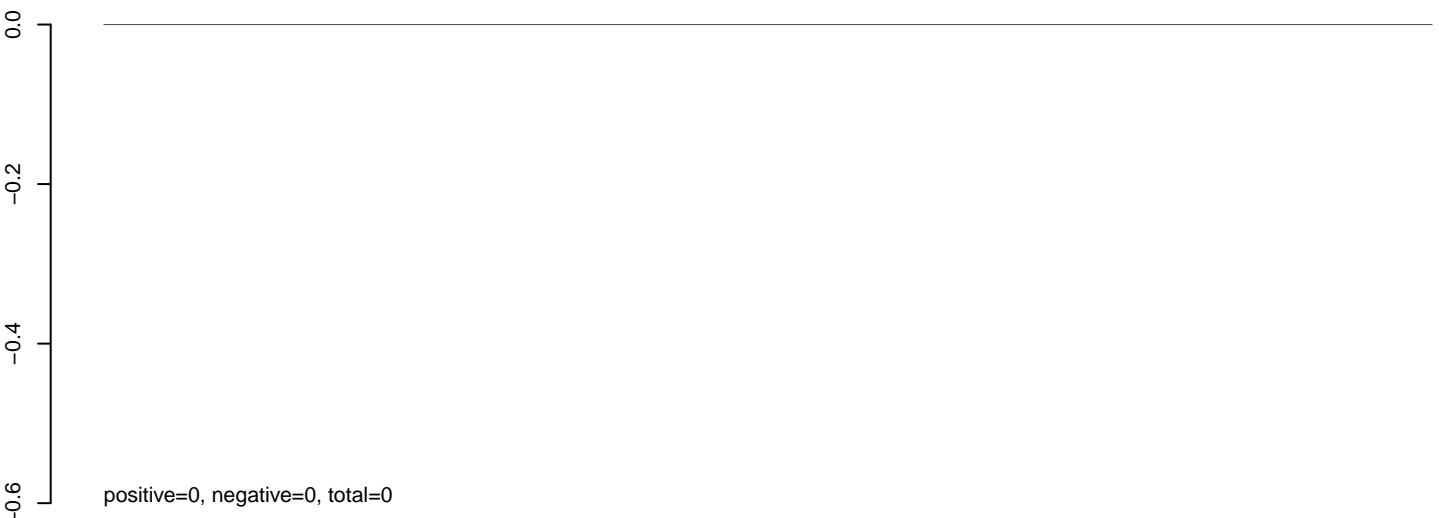
AeAeg_Aag2smallIRNA_DENV1_rep2.rep
