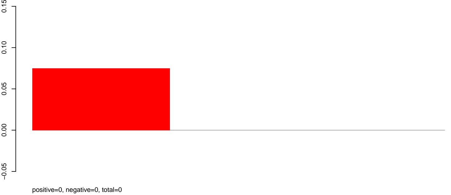
AeAeg_Aag2smallIRNA_DENV1_rep2.rep
