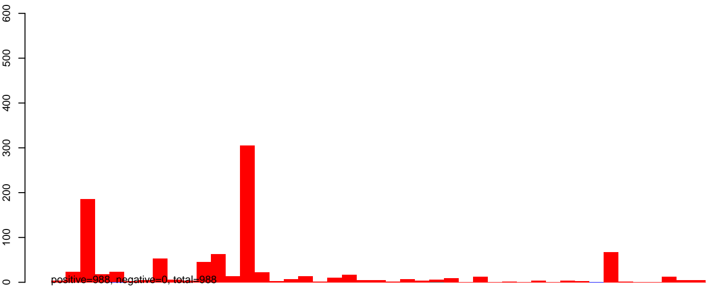
AeAeg_Aag2smallRNA_DENV2K0048_rep2.rep
