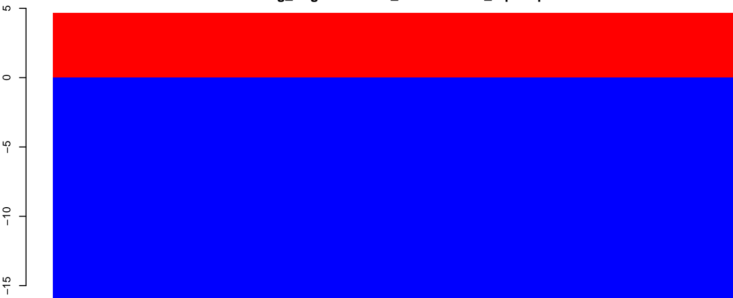
AeAeg_Aag2smallRNA_DENV2K0048_rep2.rep
