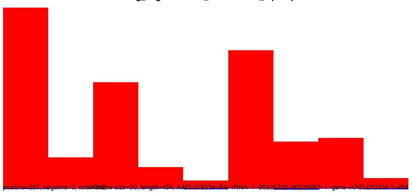
AeAeg_Aag2smallIRNA_DENV2K0048_rep2.rep
