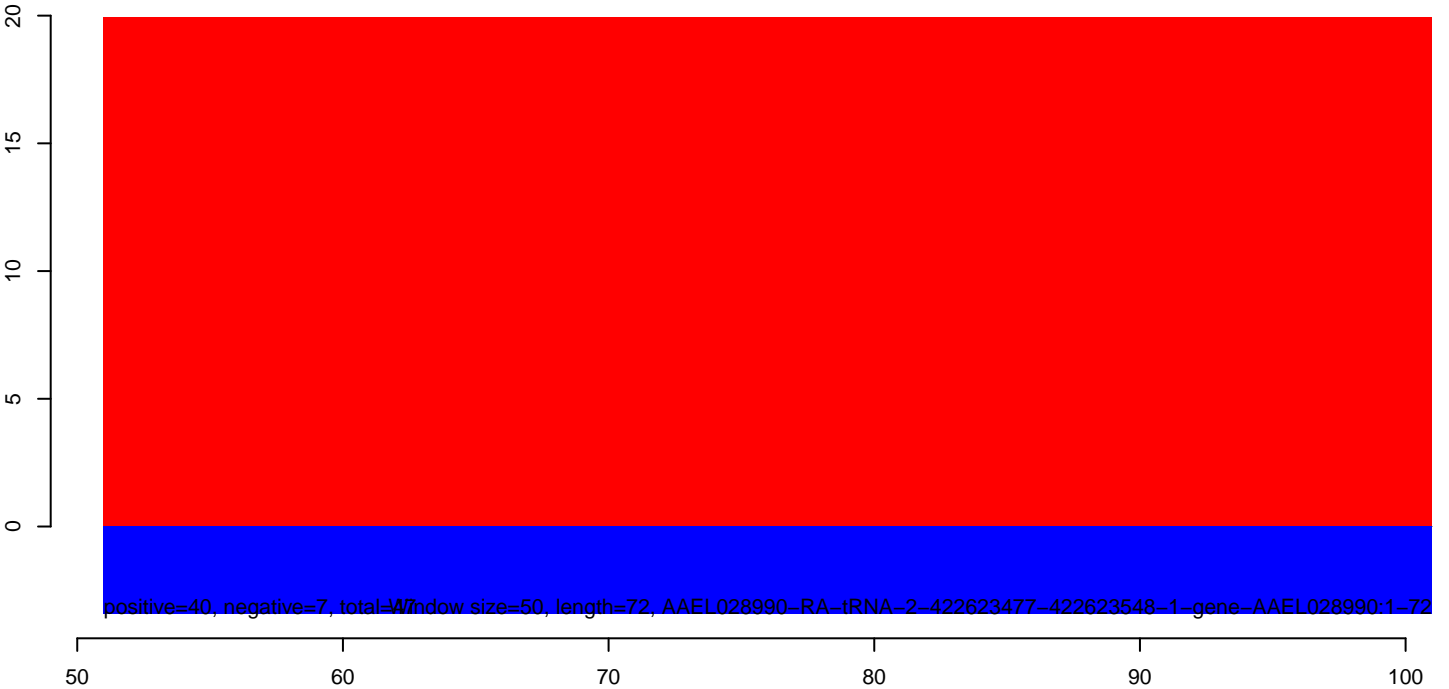
AeAeg_Aag2smallIRNA_DENV2K0048_rep2.rep
