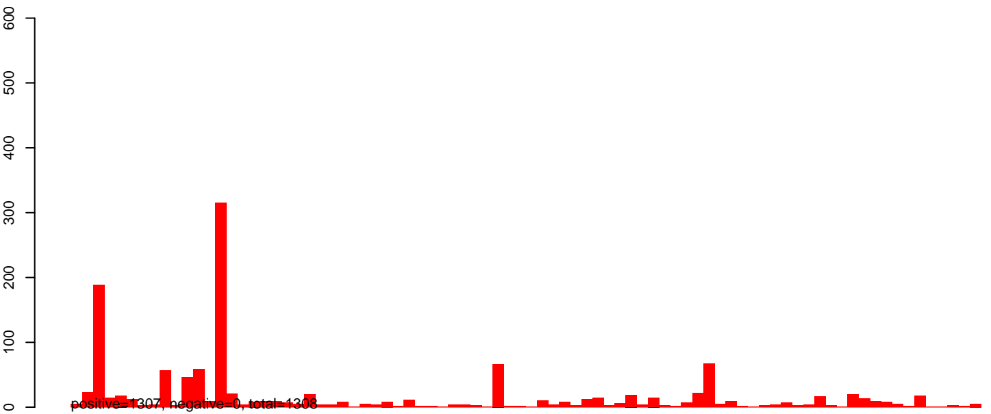
AeAeg_Aag2smallRNA_DENV2K0048_rep2.rep
