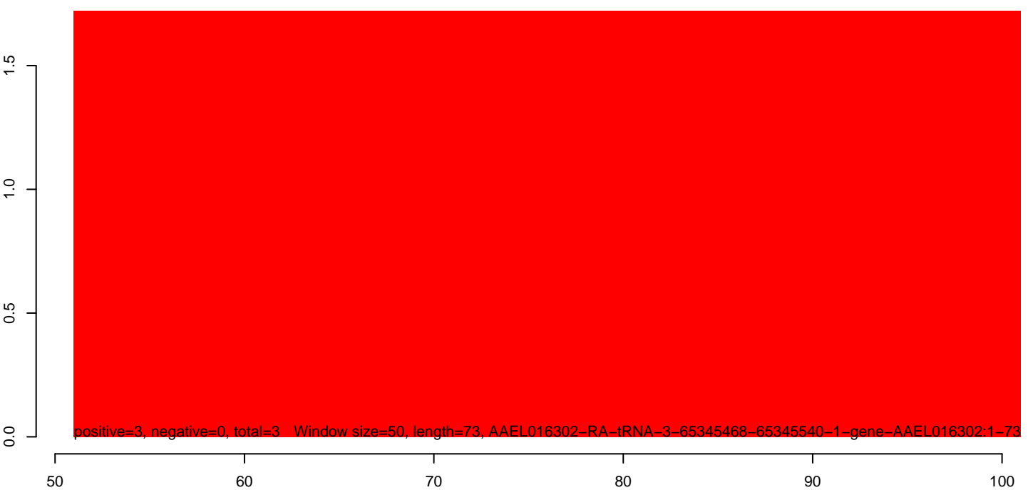
AeAeg_Aag2smallRNA_DENV2K0048_rep2.rep
