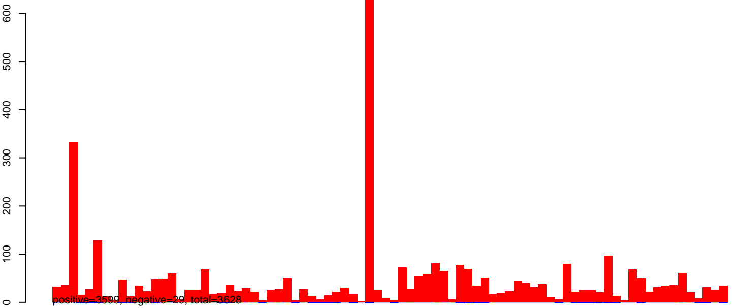
AeAeg_Aag2smallRNA_DENV2K0048_rep2.24_35.rep
