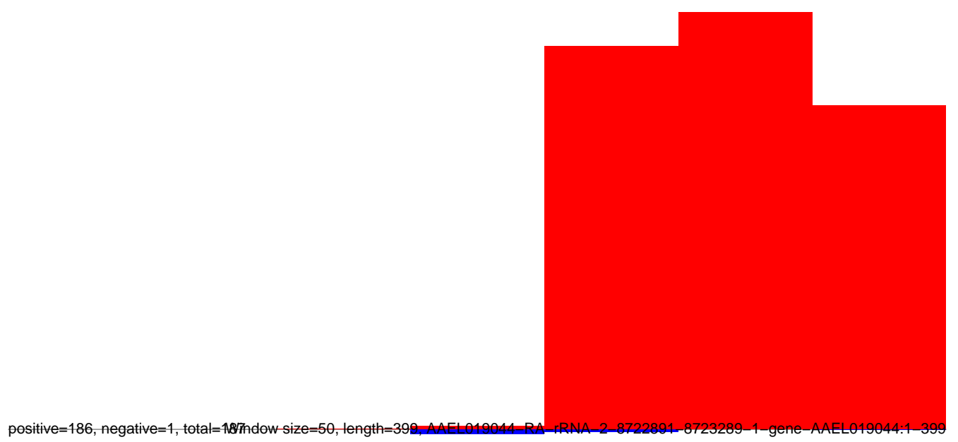
AeAeg_Aag2smallRNA_DENV2K0048_rep2.rep
