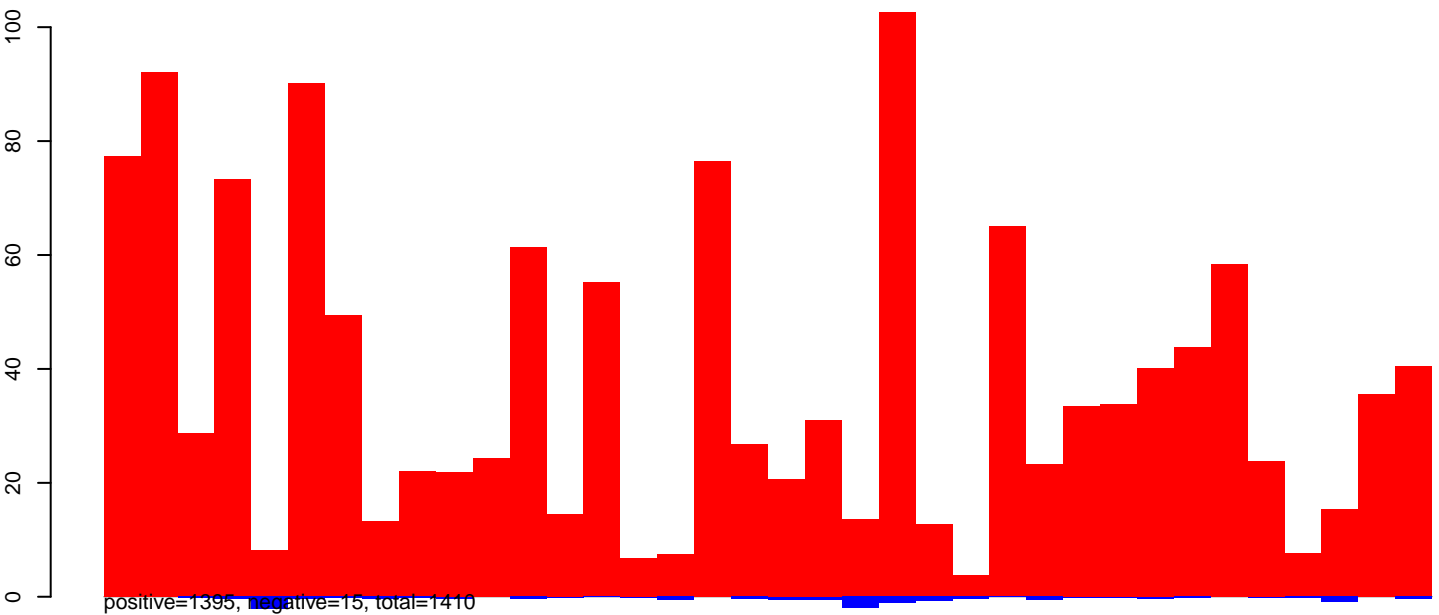
AeAeg_Aag2smallIRNA_DENV2K0048_rep2.24_35.rep
