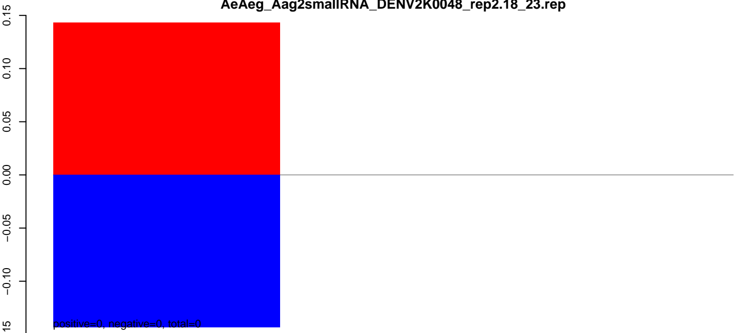
AeAeg_Aag2smallRNA_DENV2K0048_rep2.24_35.rep
