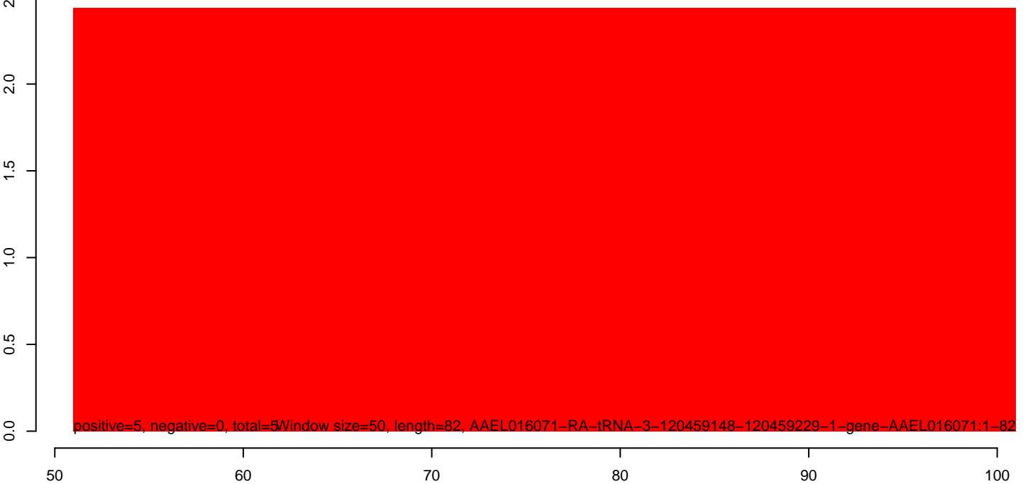
AeAeg_Aag2smallRNA_DENV2K0048_rep2.rep
