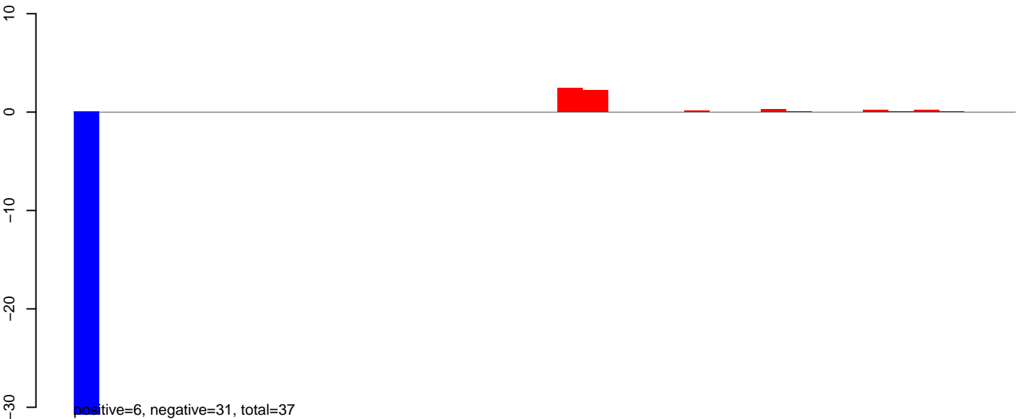
AeAeg_Aag2smallRNA_DENV2K0048_rep2.24_35.rep
