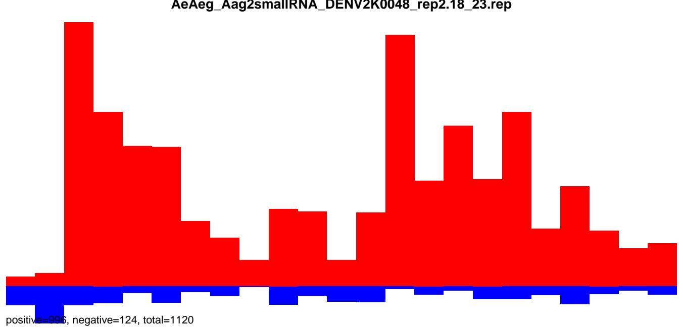
AeAeg_Aag2smallRNA_DENV2K0048_rep2.24_35.rep
