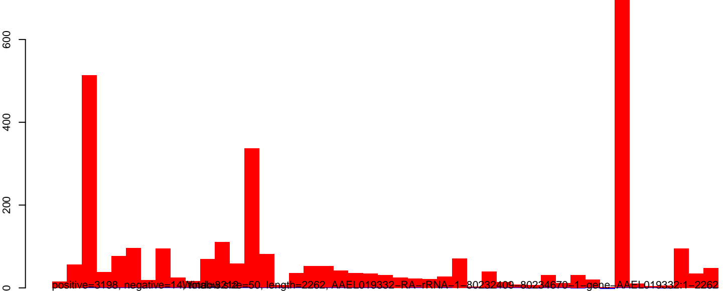
AeAeg_Aag2smallRNA_DENV2K0048_rep2.rep
