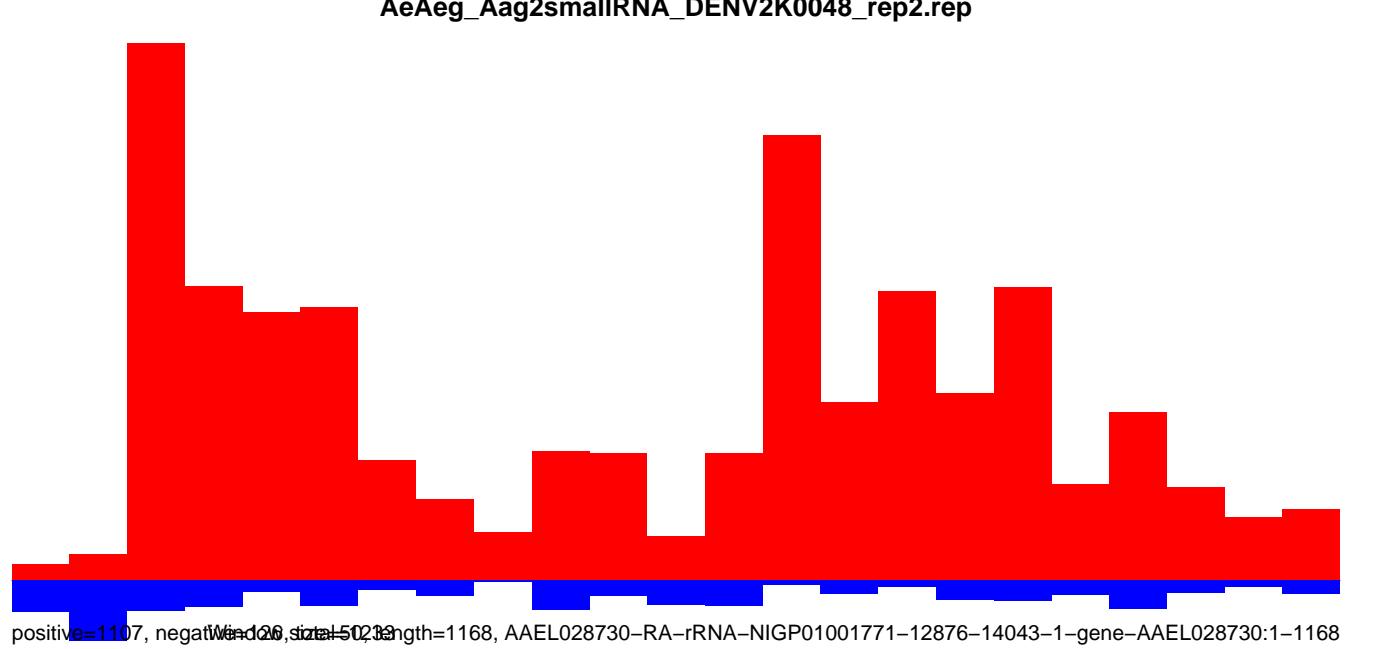
AeAeg_Aag2smallRNA_DENV2K0048_rep2.rep
