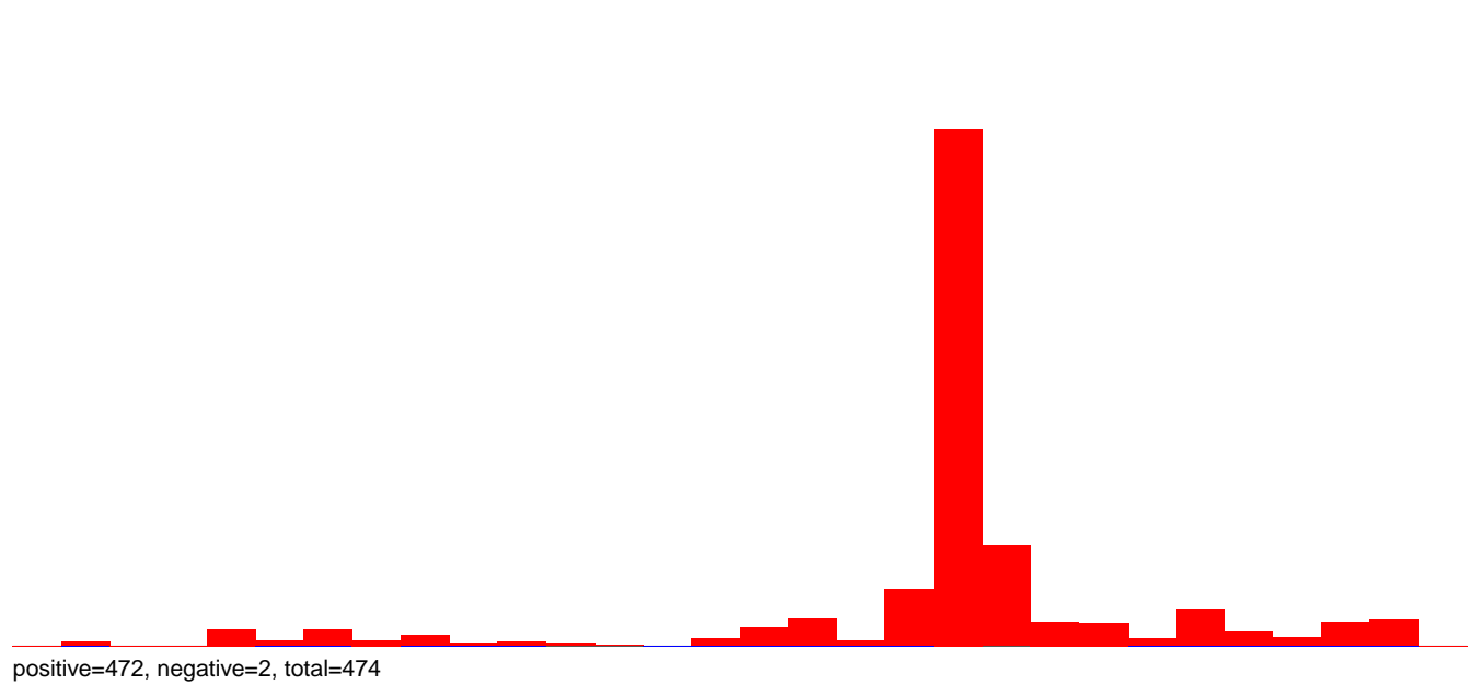
AeAeg_Aag2smallIRNA_DENV2K0048_rep2.rep
