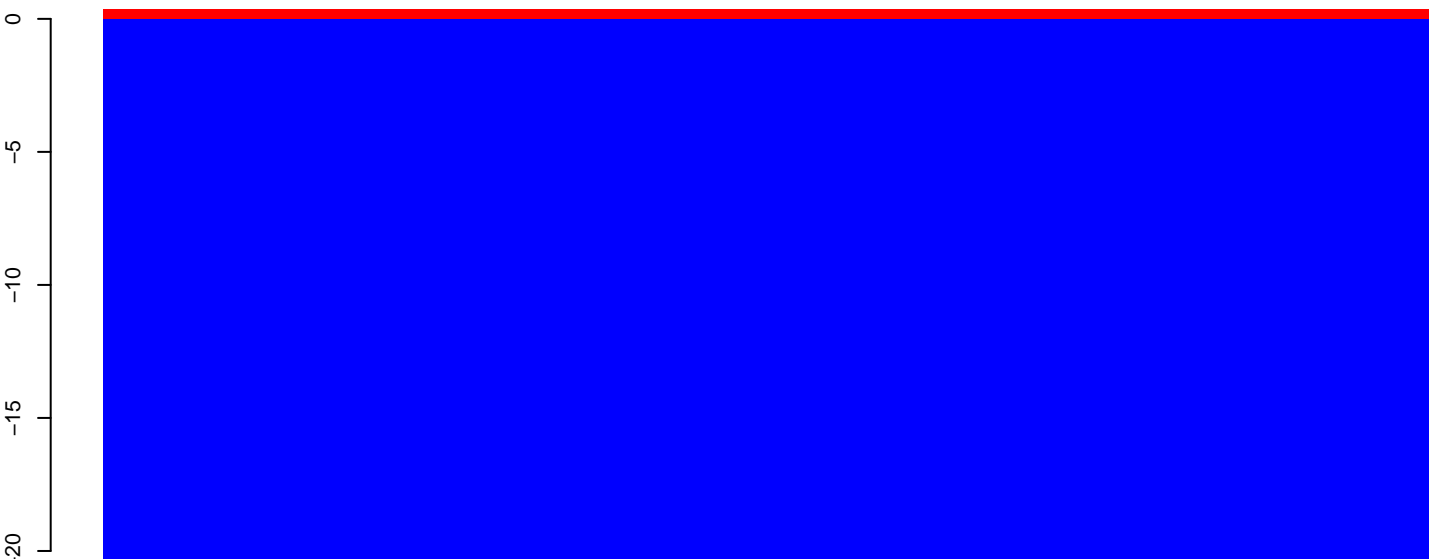
AeAeg_Aag2smallRNA_DENV2K0048_rep2.rep
