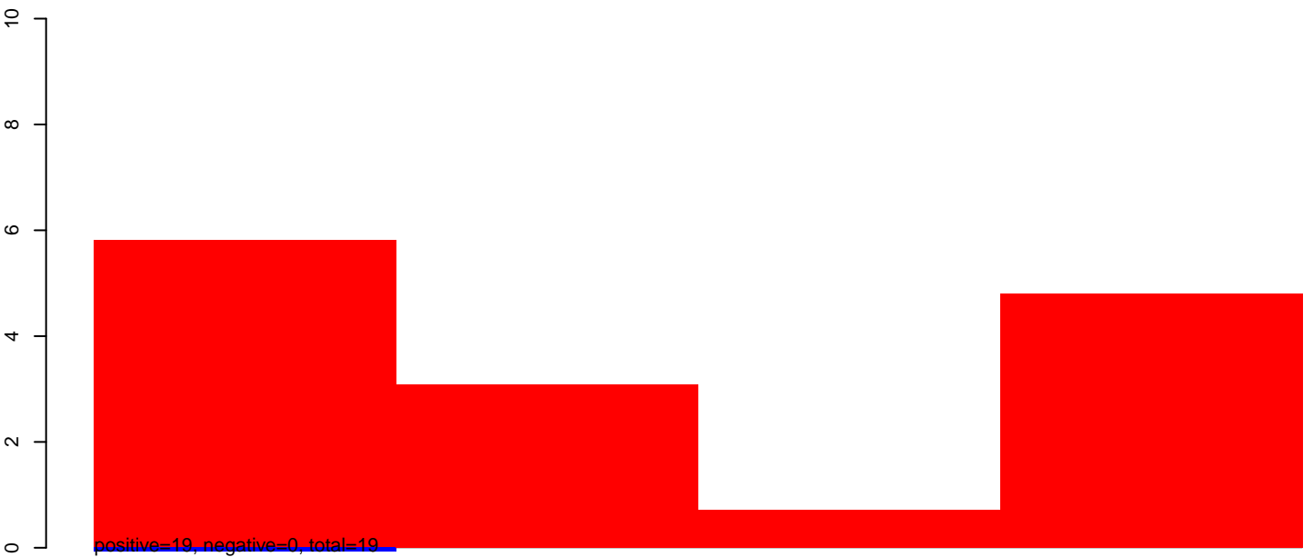
AeAeg_Aag2smallRNA_DENV2K0048_rep2.24_35.rep
