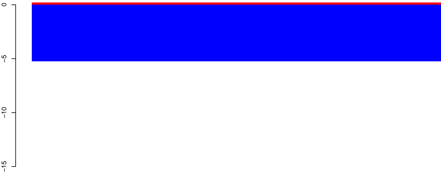
AeAeg_Aag2smallRNA_DENV2K0048_rep2.18_23.rep
