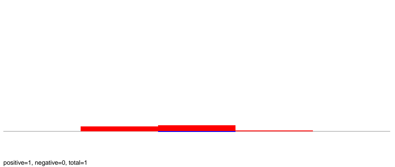
AeAeg_Aag2smallRNA_DENV2K0048_rep2.rep
