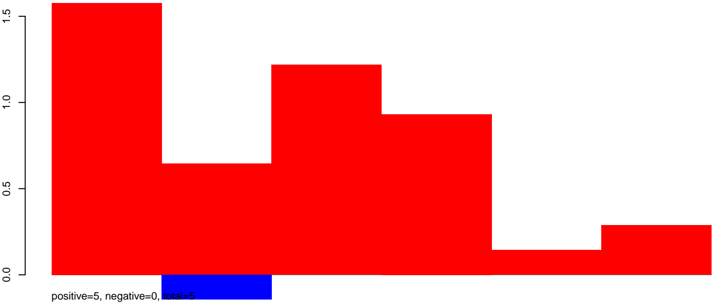
AeAeg_Aag2smallRNA_DENV2K0048_rep2.24_35.rep
