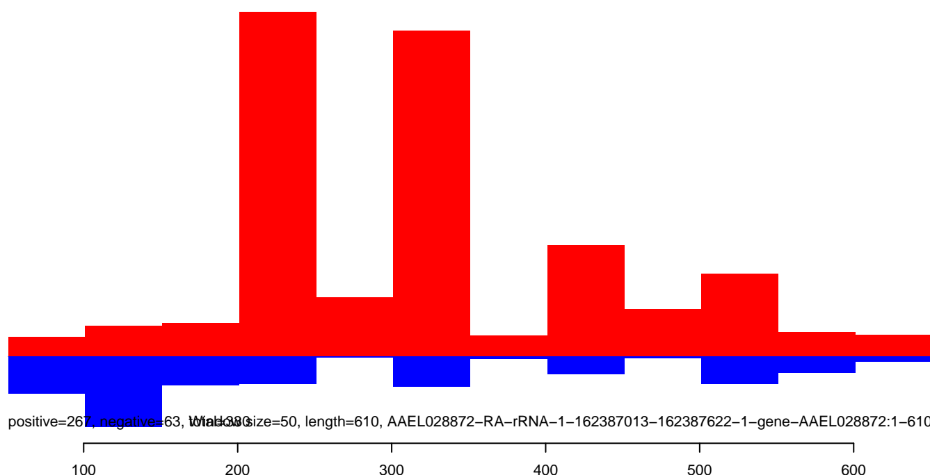
AeAeg_Aag2smallRNA_DENV2K0048_rep2.rep
