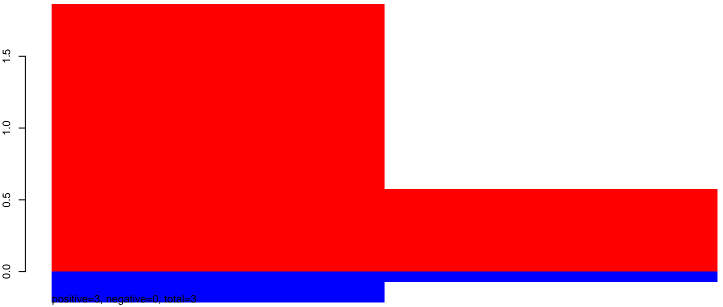
AeAeg_Aag2smallRNA_DENV2K0048_rep2.24_35.rep
