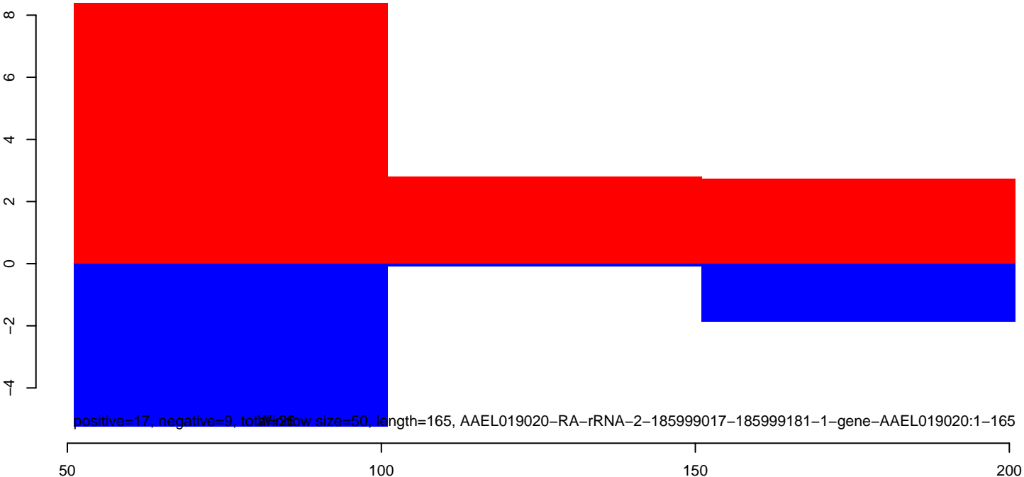
AeAeg_Aag2smallRNA_DENV2K0048_rep2.rep
