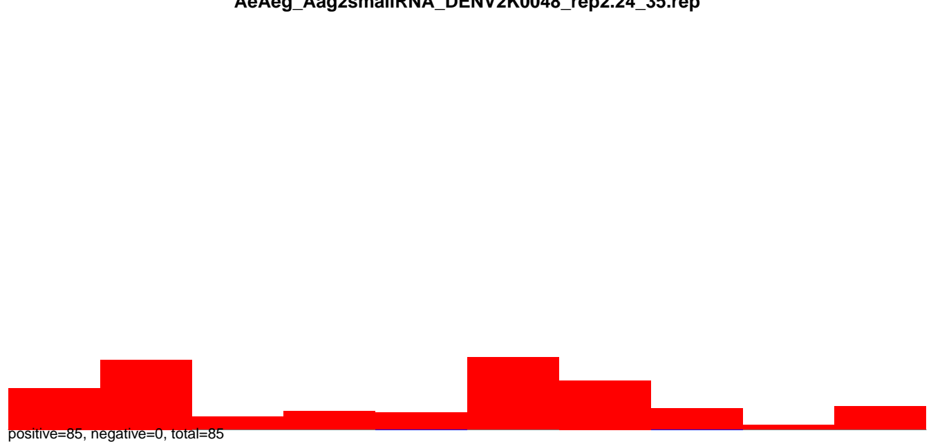
AeAeg_Aag2smallIRNA_DENV2K0048_rep2.rep
