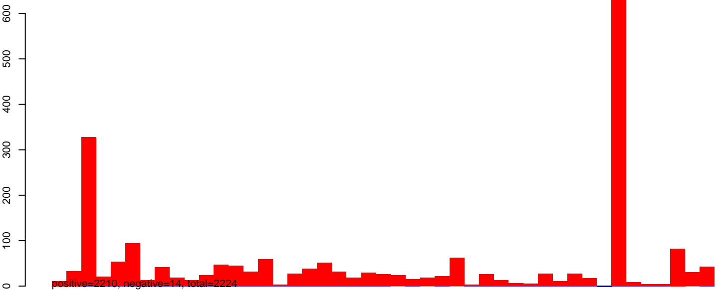
AeAeg_Aag2smallRNA_DENV2K0048_rep2.24_35.rep
