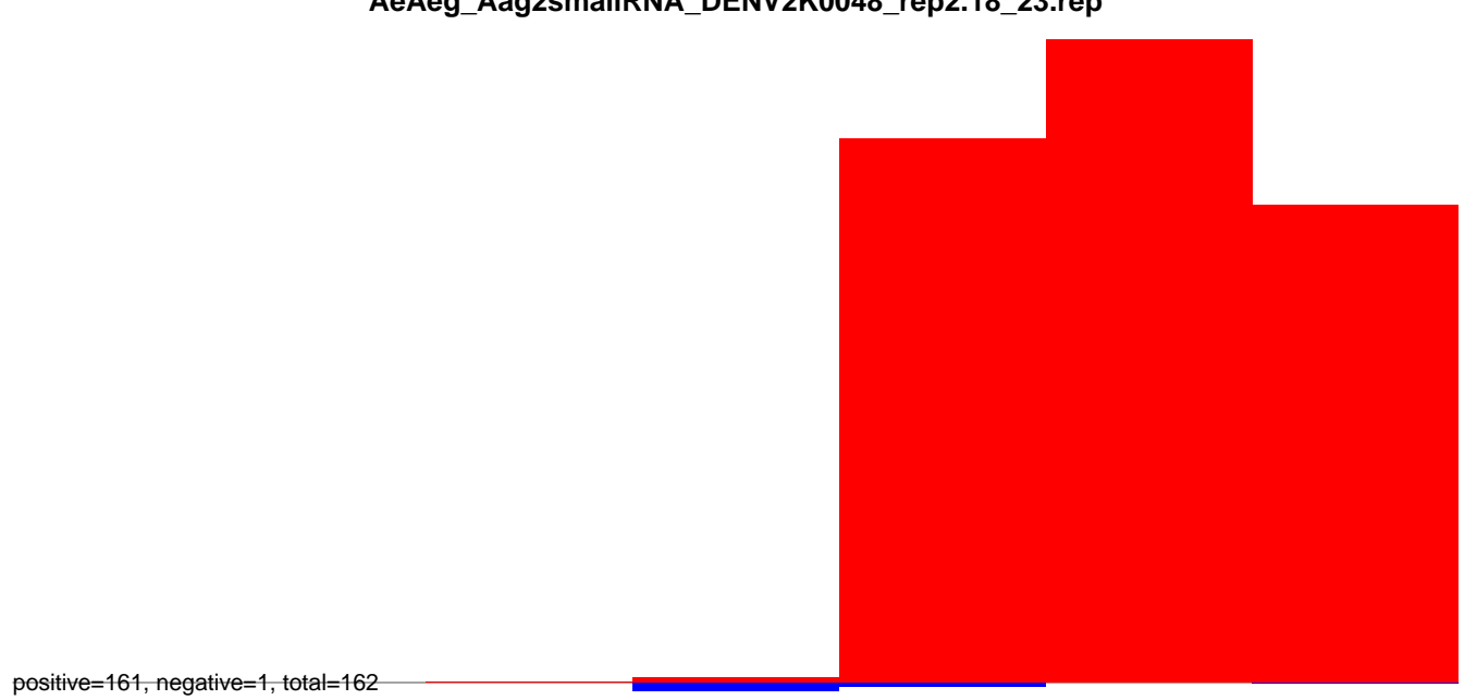
AeAeg_Aag2smallRNA_DENV2K0048_rep2.24_35.rep
