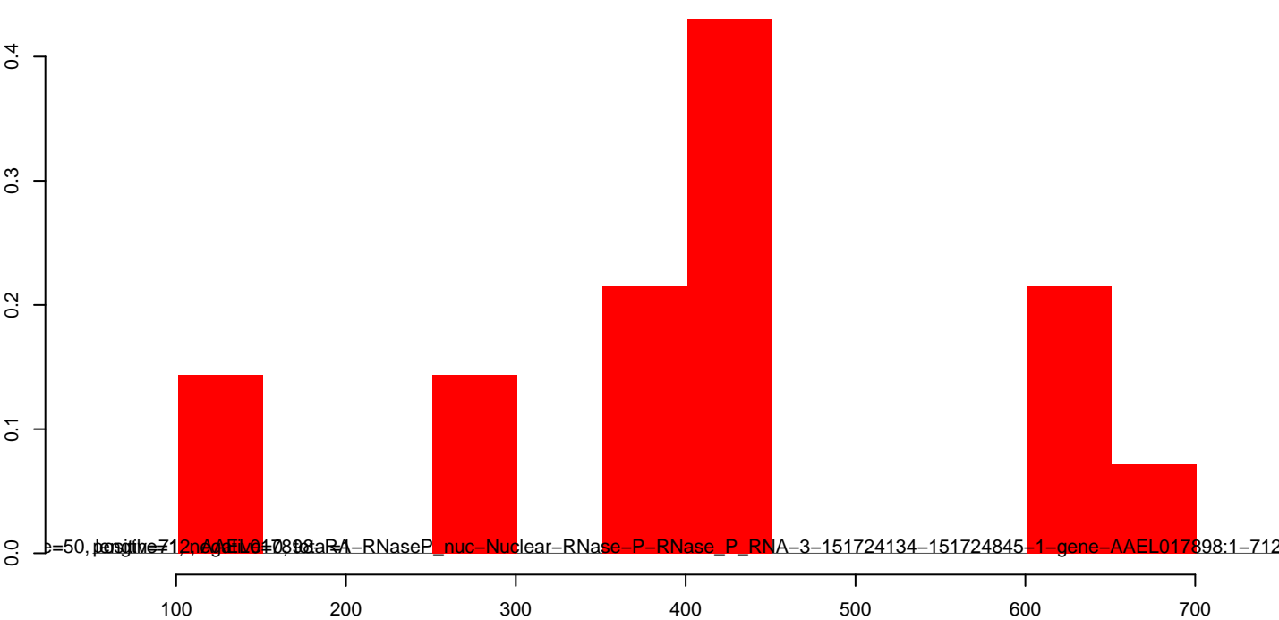
AeAeg_Aag2smallRNA_DENV2K0048_rep2.rep
