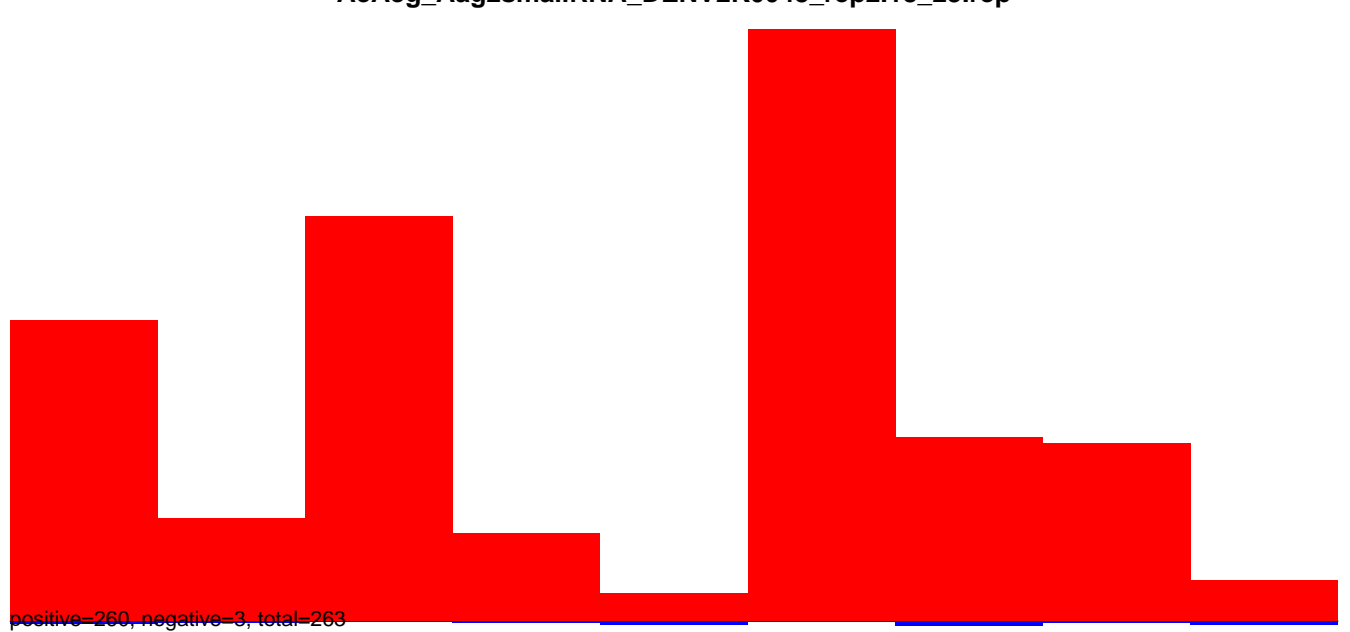
AeAeg_Aag2smallIRNA_DENV2K0048_rep2.24_35.rep
