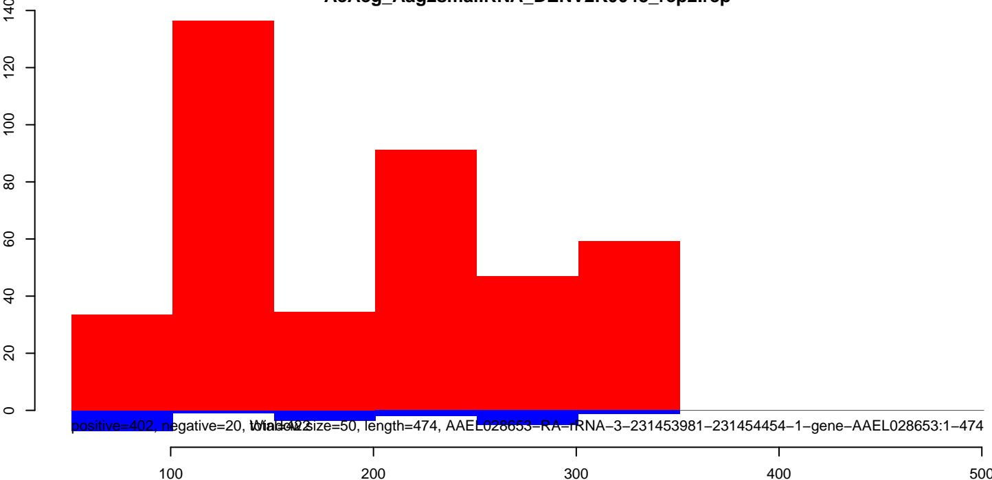
AeAeg_Aag2smallRNA_DENV2K0048_rep2.rep
