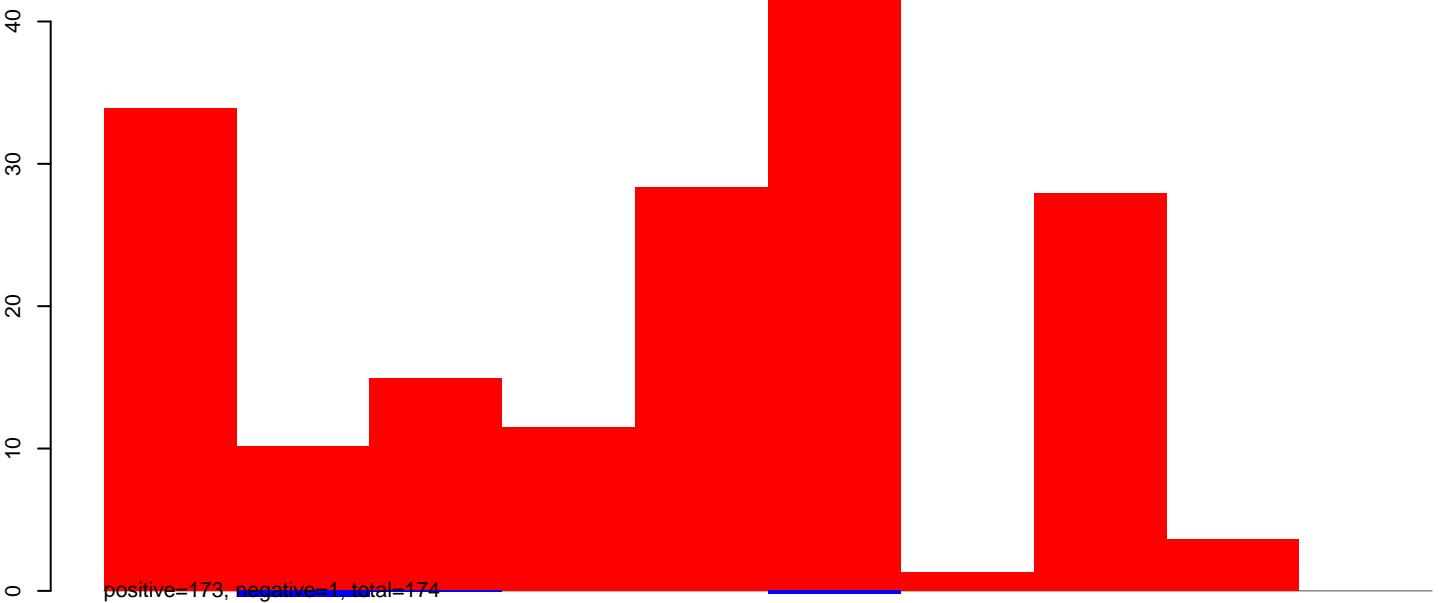
AeAeg_Aag2smallRNA_DENV2K0048_rep2.24_35.rep
