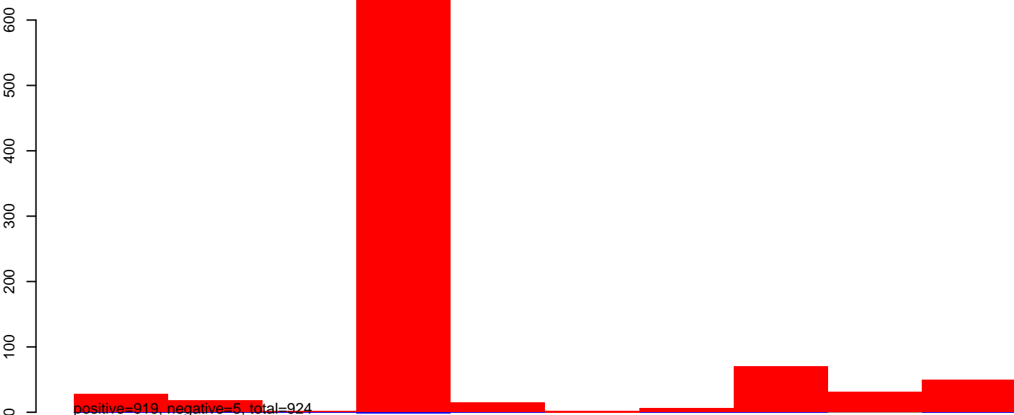
AeAeg_Aag2smallRNA_DENV2K0048_rep2.24_35.rep
