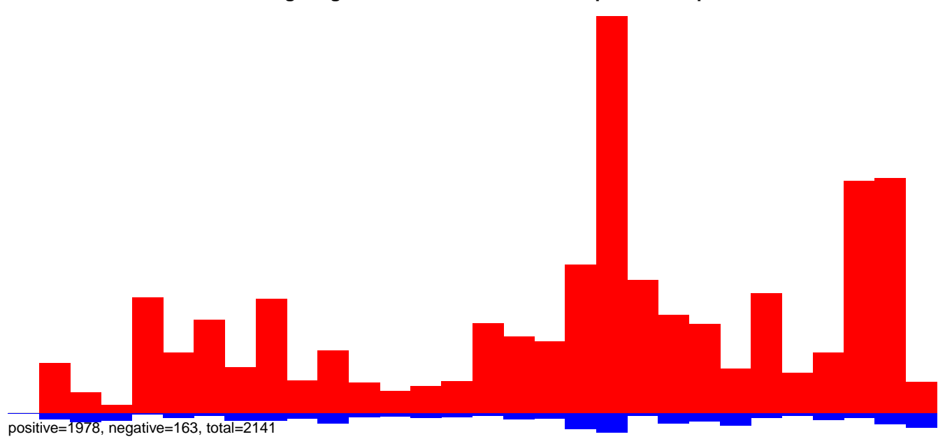
AeAeg_Aag2smallIRNA_DENV2K0048_rep2.24_35.rep
