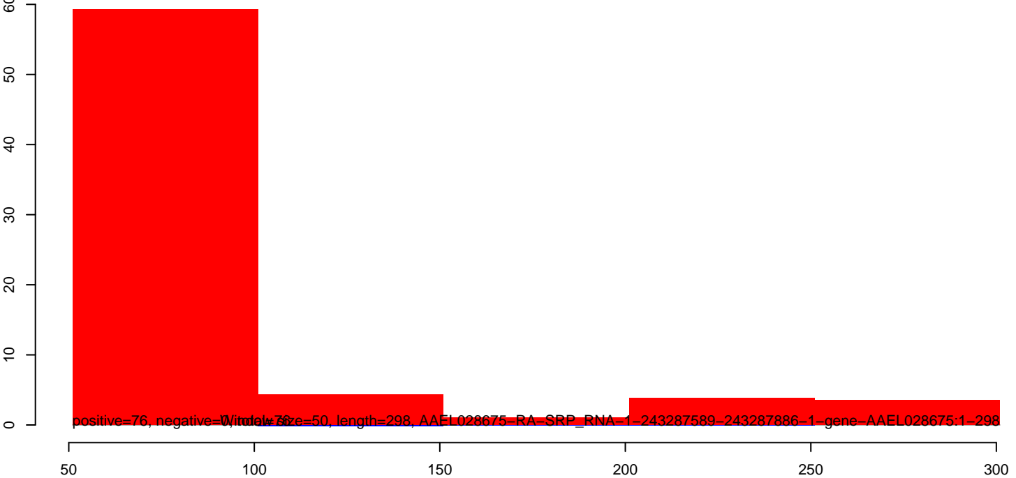
AeAeg_Aag2smallRNA_DENV2K0048_rep2.rep
