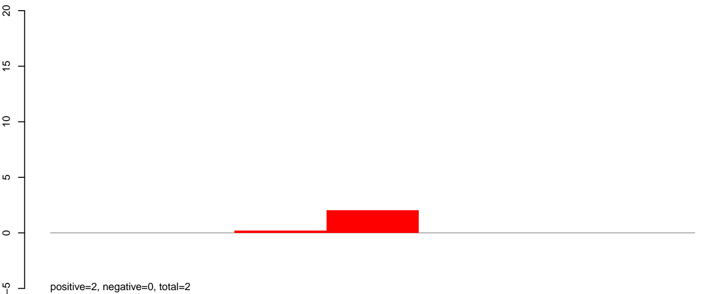
AeAeg_Aag2smallRNA_DENV2K0048_rep2.rep
