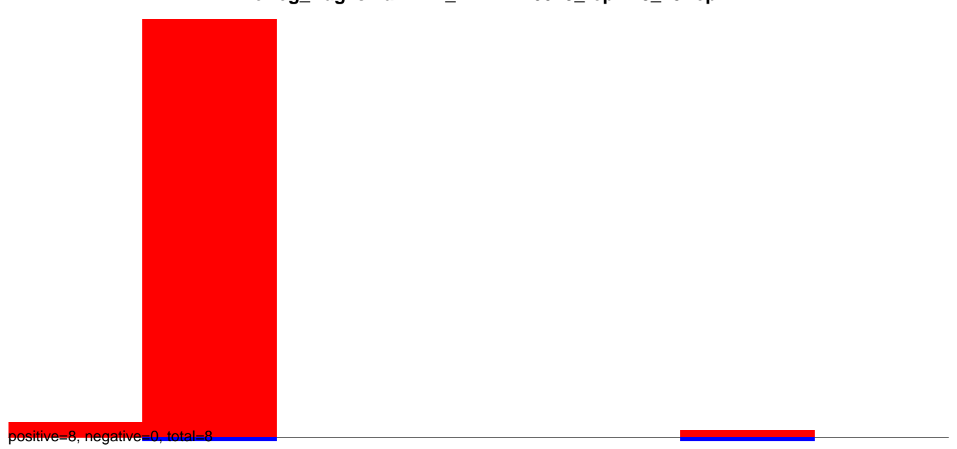
AeAeg_Aag2smallRNA_DENV2K0048_rep2.24_35.rep
