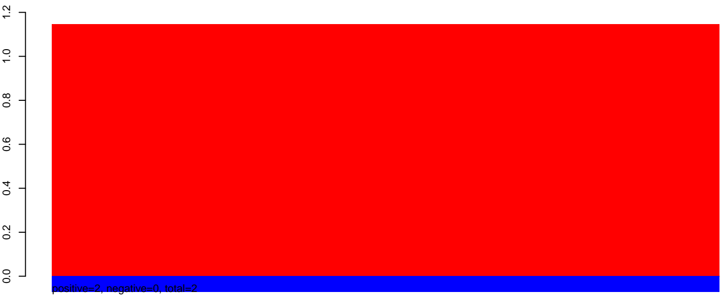
AeAeg_Aag2smallIRNA_DENV2K0048_rep2.24_35.rep
