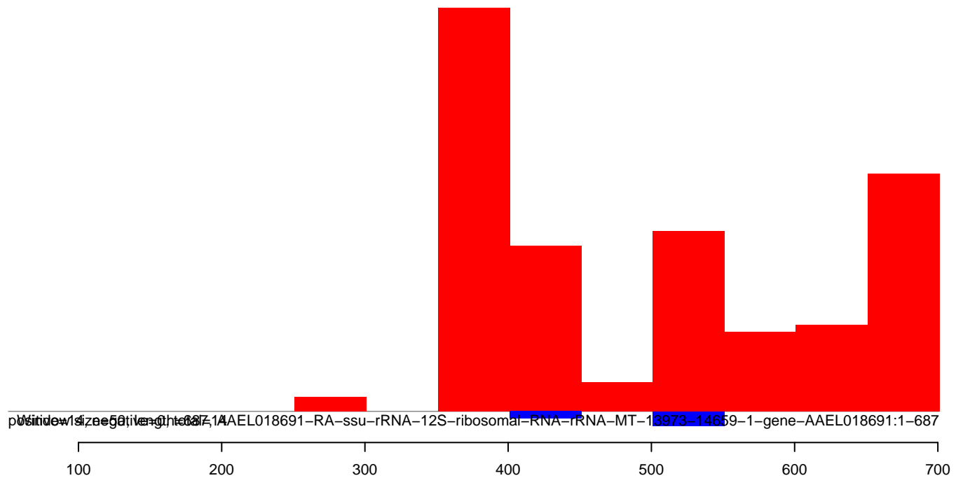
AeAeg_Aag2smallRNA_DENV2K0048_rep2.rep
