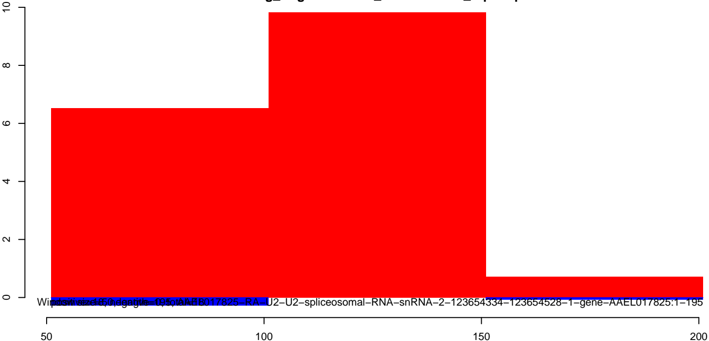
AeAeg_Aag2smallRNA_DENV2K0048_rep2.rep
