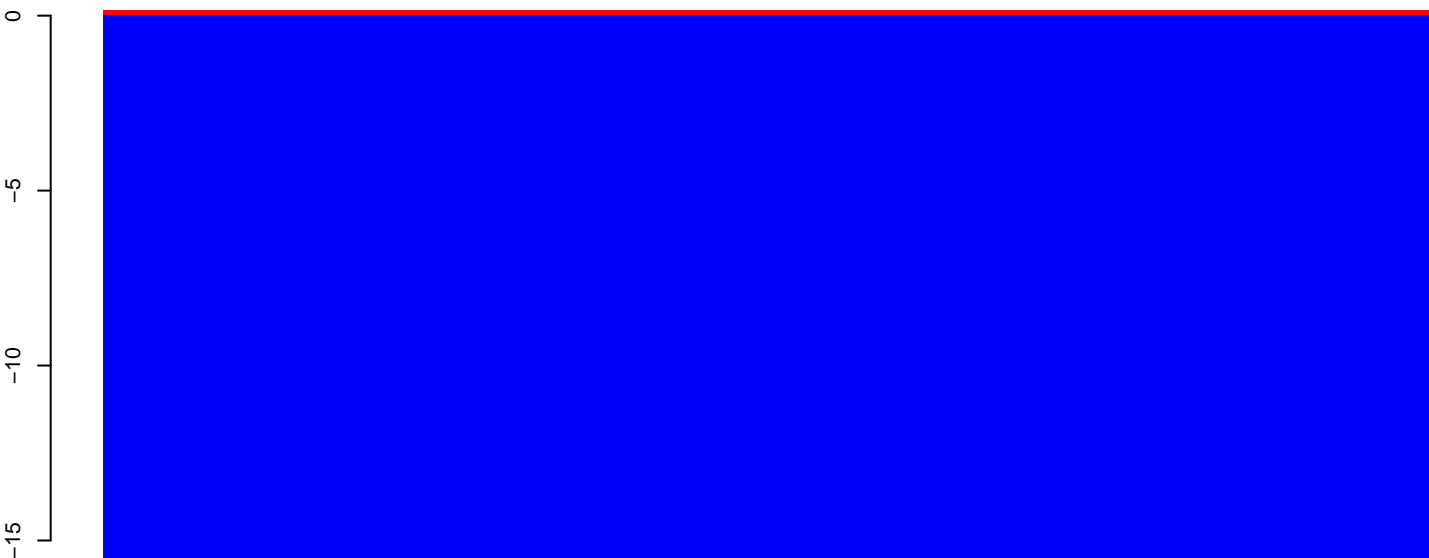
AeAeg_Aag2smallRNA_DENV2K0048_rep2.24_35.rep
