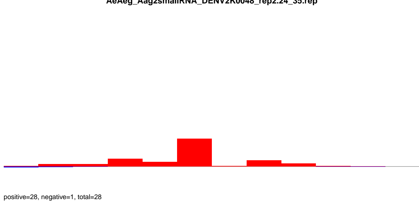
AeAeg_Aag2smallRNA_DENV2K0048_rep2.rep
