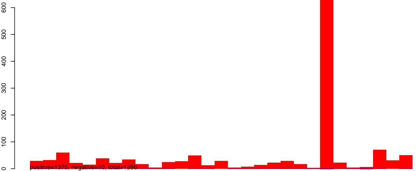
AeAeg_Aag2smallIRNA_DENV2K0048_rep2.24_35.rep
