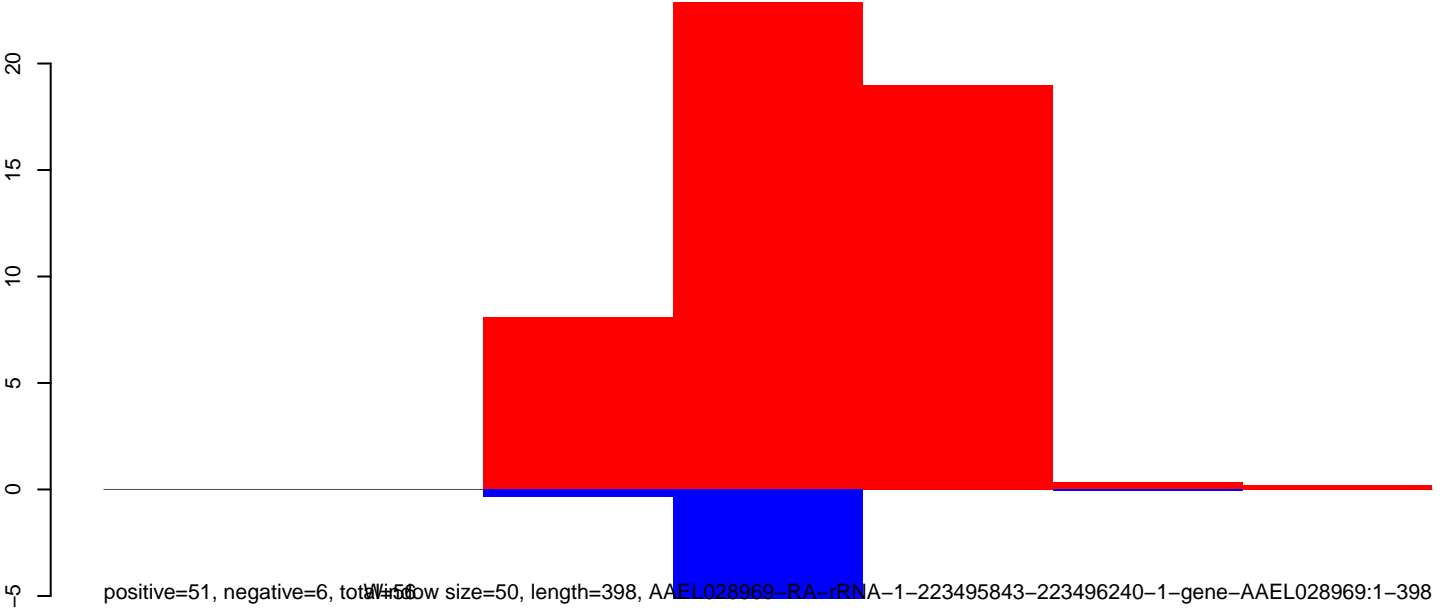
AeAeg_Aag2smallRNA_DENV2K0048_rep2.rep
