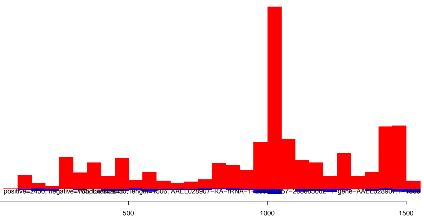
AeAeg_Aag2smallIRNA_DENV2K0048_rep2.rep
