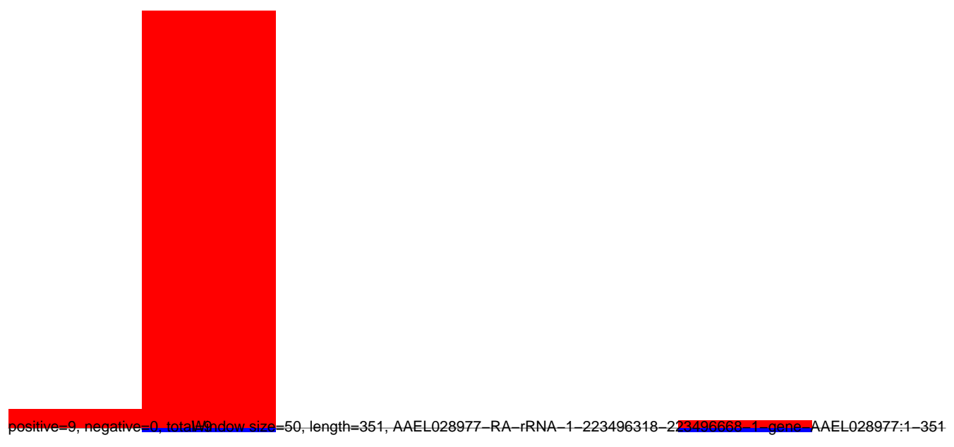
AeAeg_Aag2smallRNA_DENV2K0048_rep2.rep
