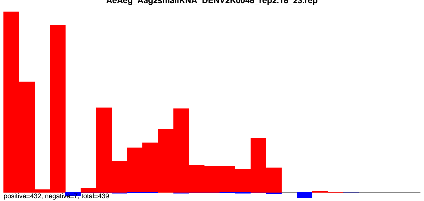
AeAeg_Aag2smallRNA_DENV2K0048_rep2.24_35.rep
