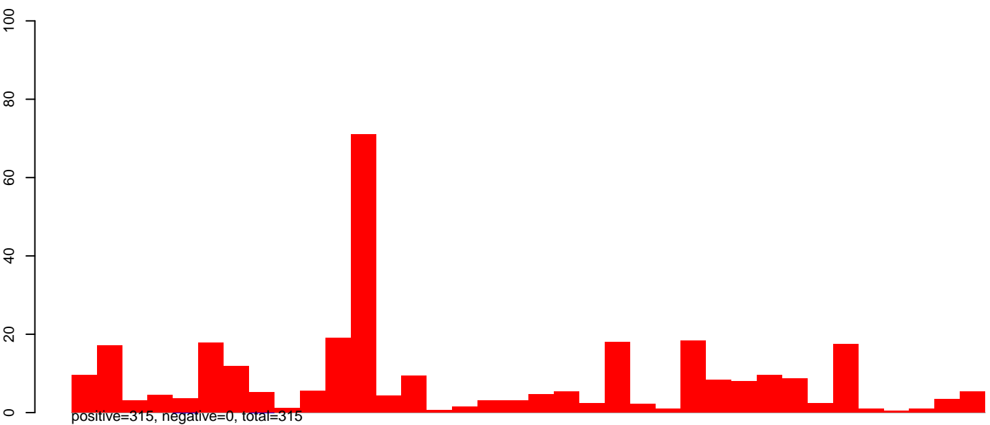
AeAeg_Aag2smallIRNA_DENV2K0048_rep2.rep
