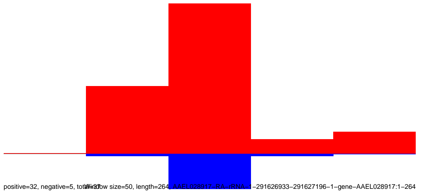
AeAeg_Aag2smallRNA_DENV2K0048_rep2.rep
