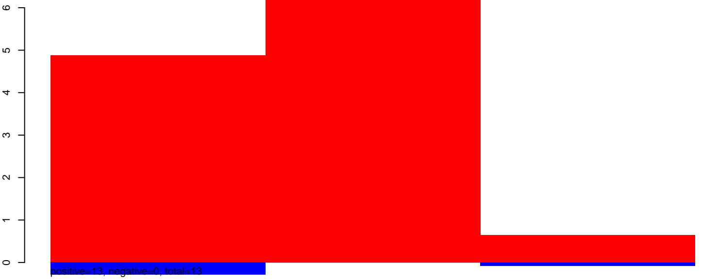
AeAeg_Aag2smallRNA_DENV2K0048_rep2.24_35.rep
