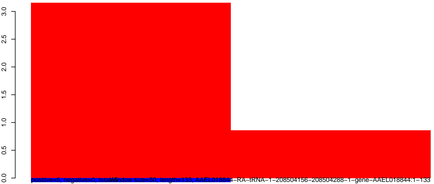
AeAeg_Aag2smallIRNA_DENV2K0048_rep2.rep
