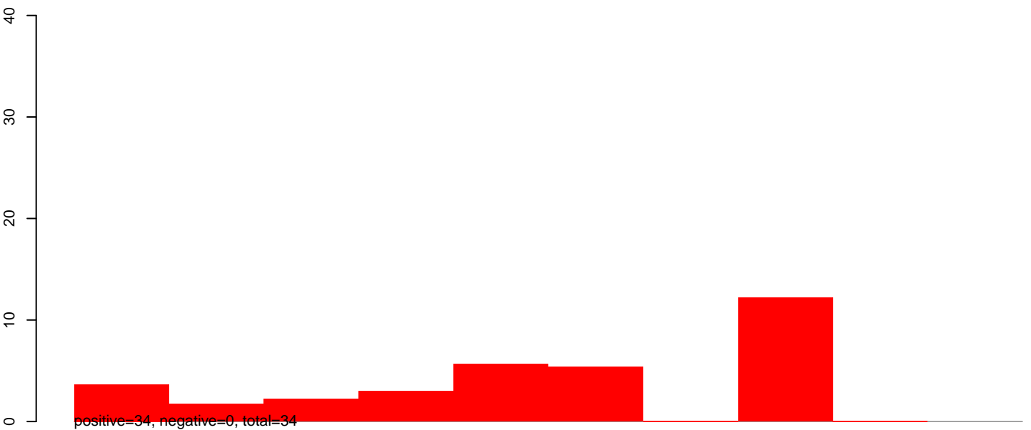
AeAeg_Aag2smallRNA_DENV2K0048_rep2.rep
