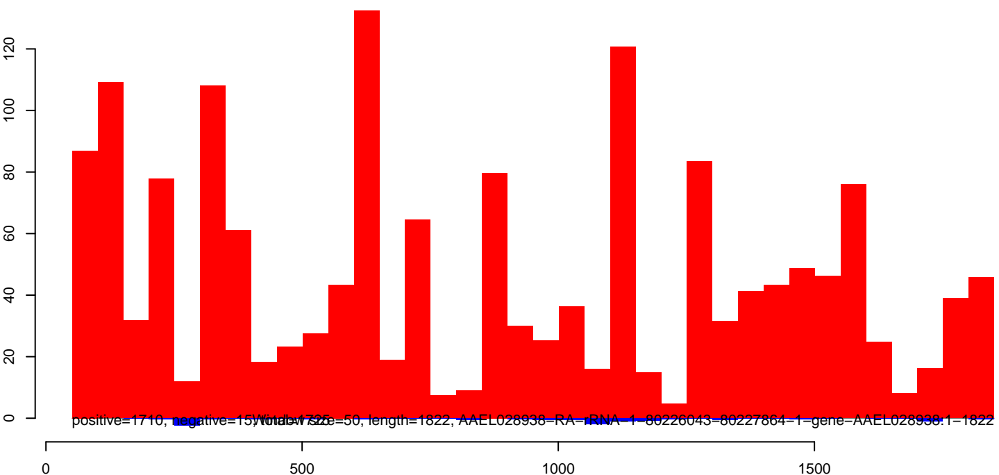
AeAeg_Aag2smallIRNA_DENV2K0048_rep2.rep
