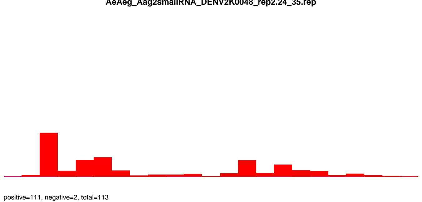
AeAeg_Aag2smallRNA_DENV2K0048_rep2.rep
