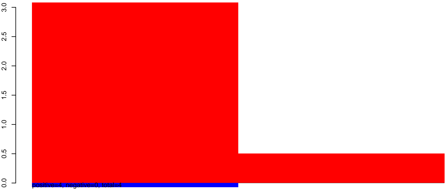
AeAeg_Aag2smallIRNA_DENV2K0048_rep2.24_35.rep
