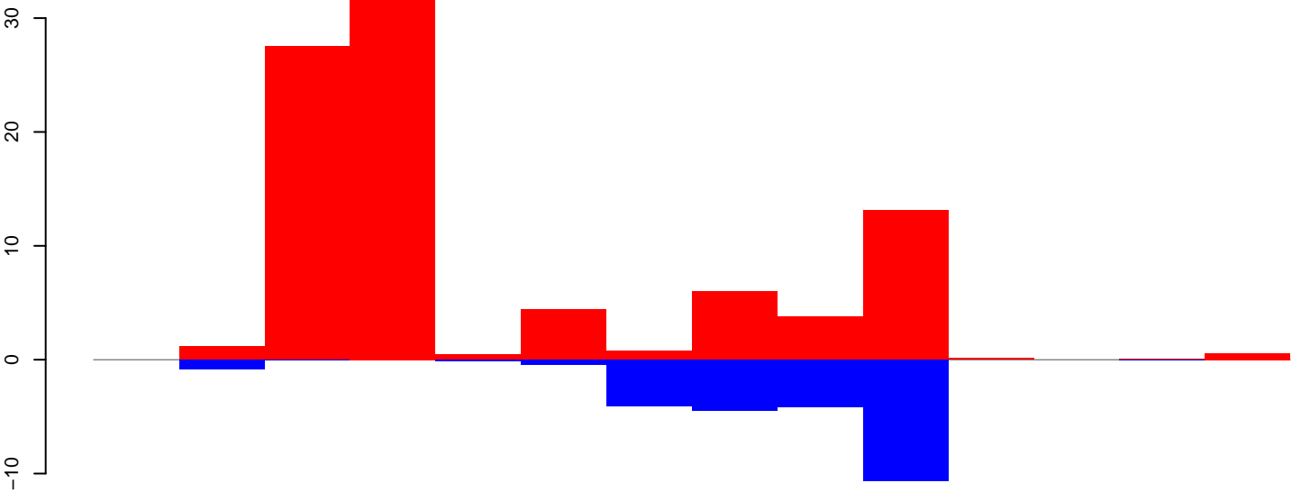
AeAeg_Aag2smallRNA_DENV2K0048_rep2.24_35.rep
