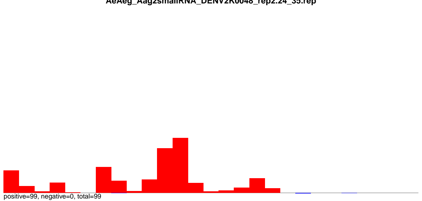
AeAeg_Aag2smallRNA_DENV2K0048_rep2.rep
