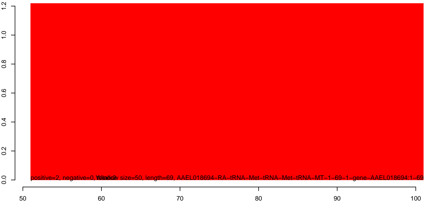
AeAeg_Aag2smallIRNA_DENV2K0048_rep2.rep
