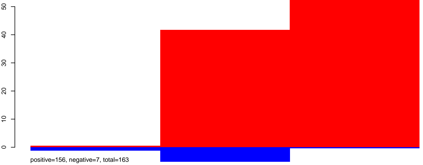
AeAeg_Aag2smallRNA_DENV2K0048_rep2.24_35.rep
