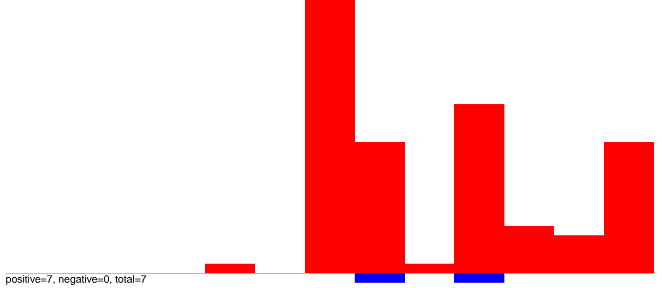
AeAeg_Aag2smallRNA_DENV2K0048_rep2.24_35.rep
