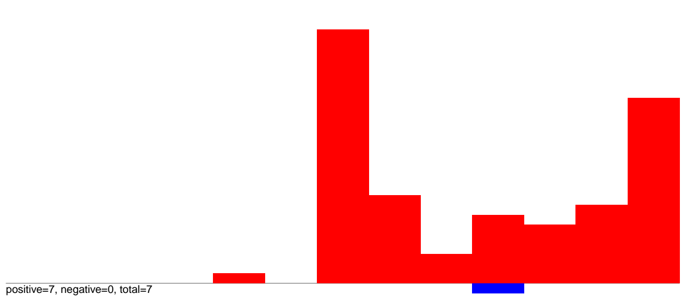
AeAeg_Aag2smallRNA_DENV2K0048_rep2.rep
