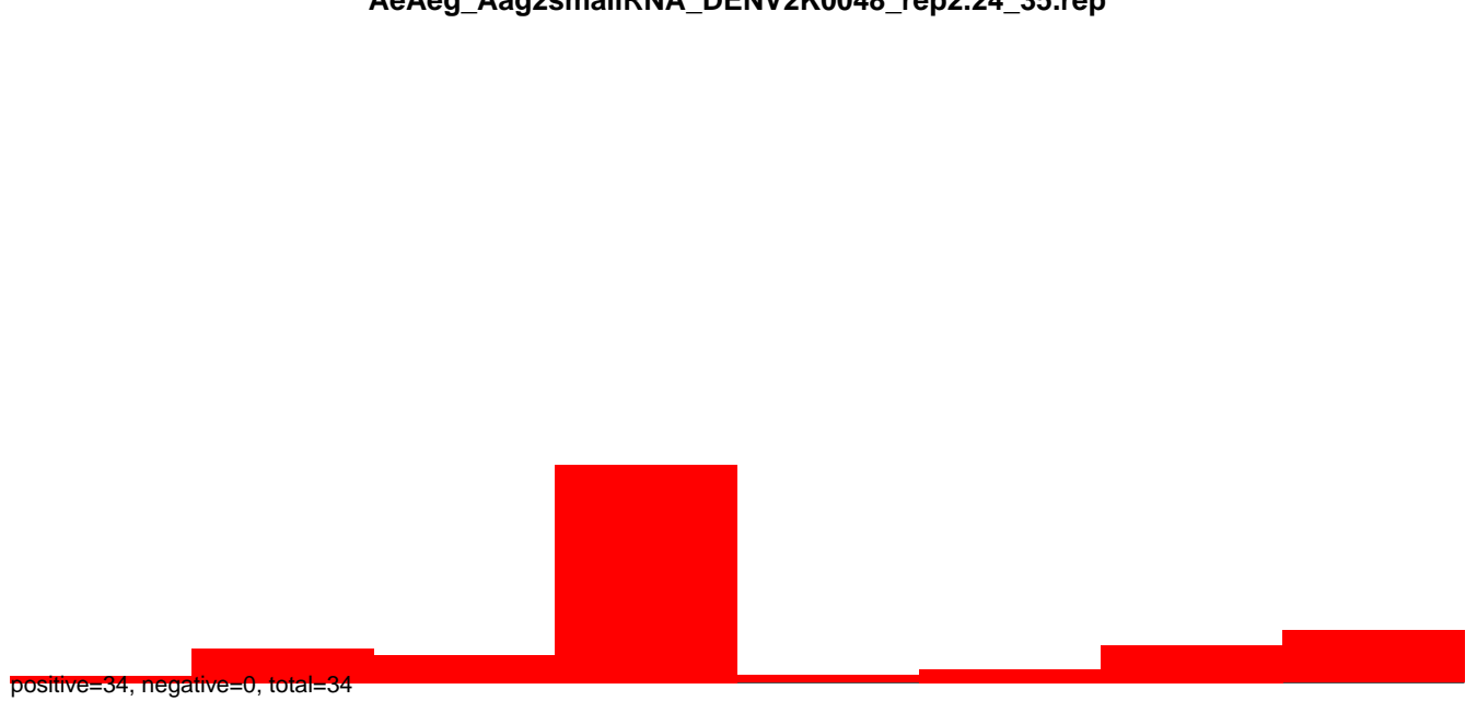
AeAeg_Aag2smallRNA_DENV2K0048_rep2.rep
