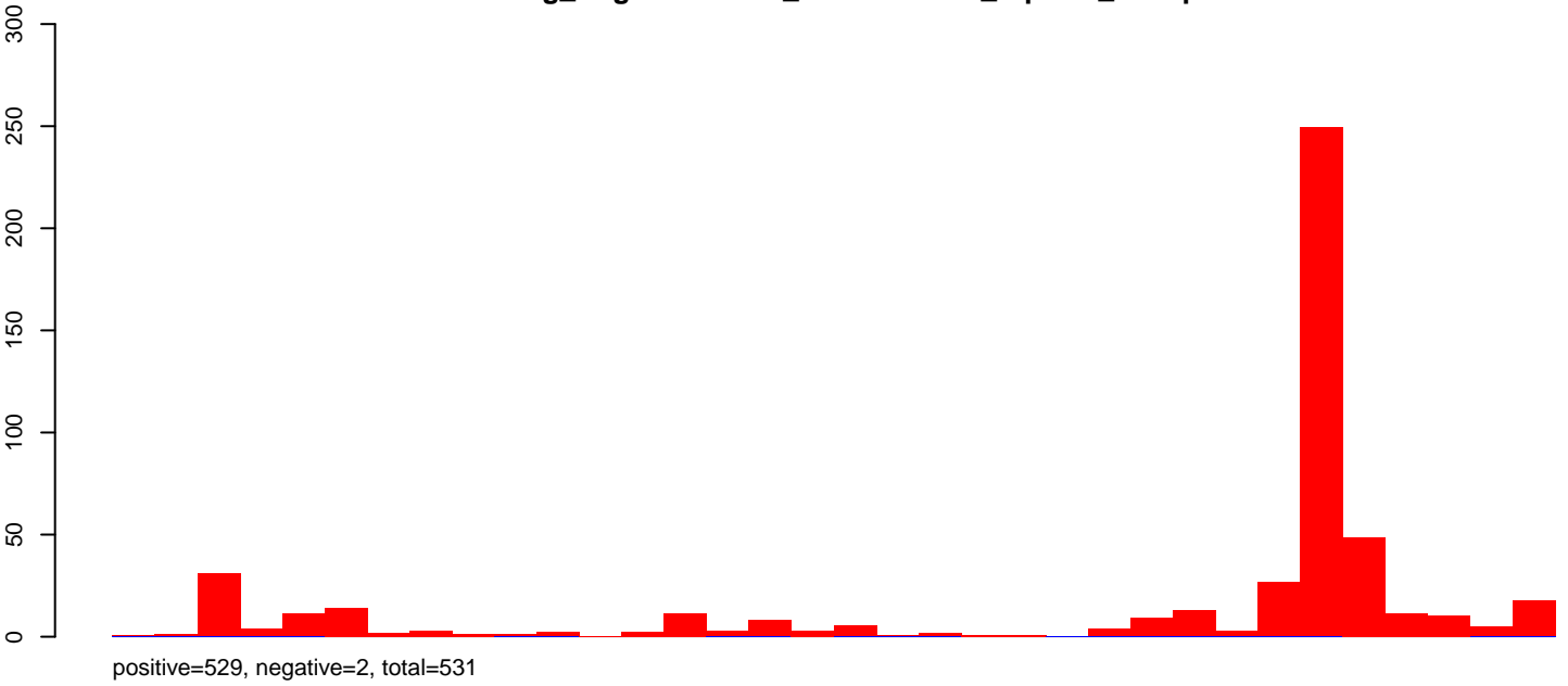
AeAeg_Aag2smallRNA_DENV2K0048_rep2.rep
