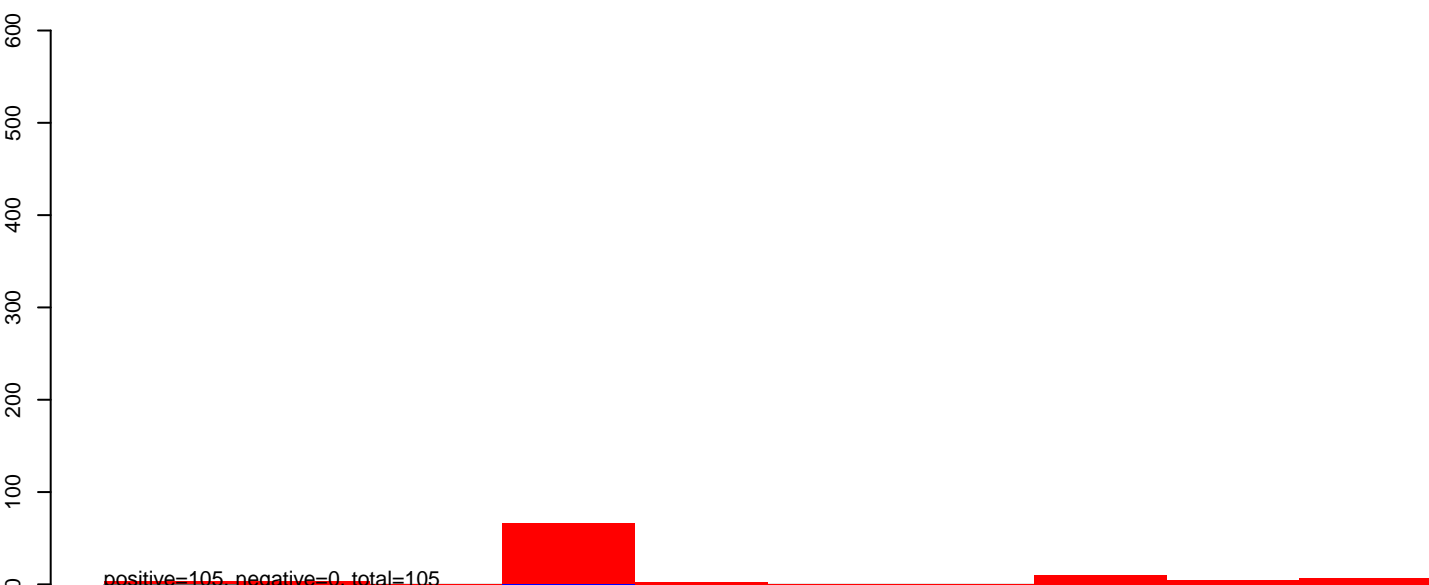
AeAeg_Aag2smallRNA_DENV2K0048_rep2.rep
