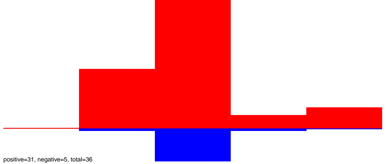
AeAeg_Aag2smallRNA_DENV2K0048_rep2.24_35.rep
