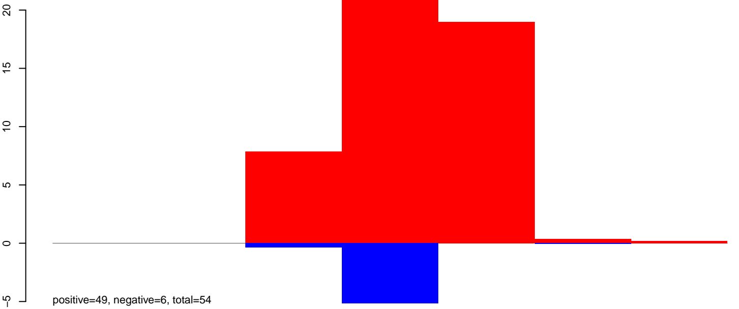
AeAeg_Aag2smallRNA_DENV2K0048_rep2.24_35.rep
