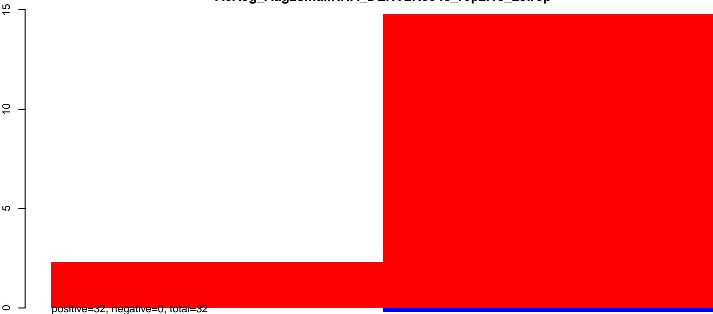
AeAeg_Aag2smallIRNA_DENV2K0048_rep2.24_35.rep
