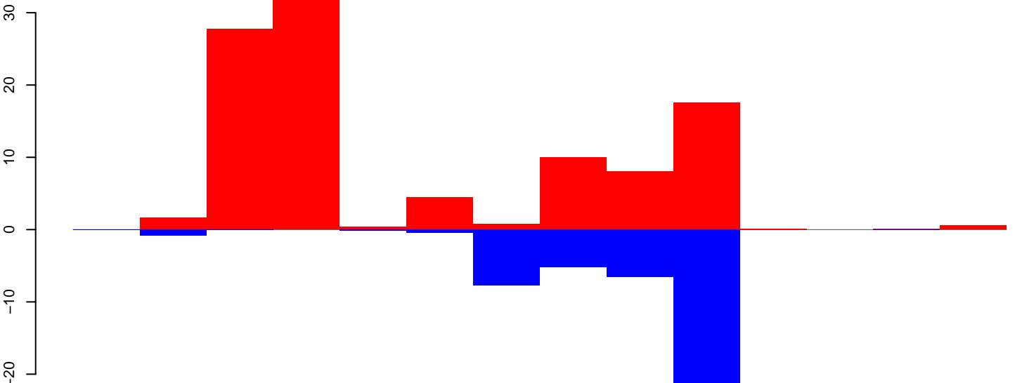
AeAeg_Aag2smallRNA_DENV2K0048_rep2.rep
