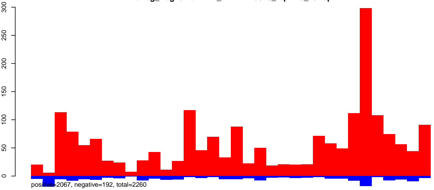
AeAeg_Aag2smallRNA_DENV2K0048_rep2.24_35.rep
