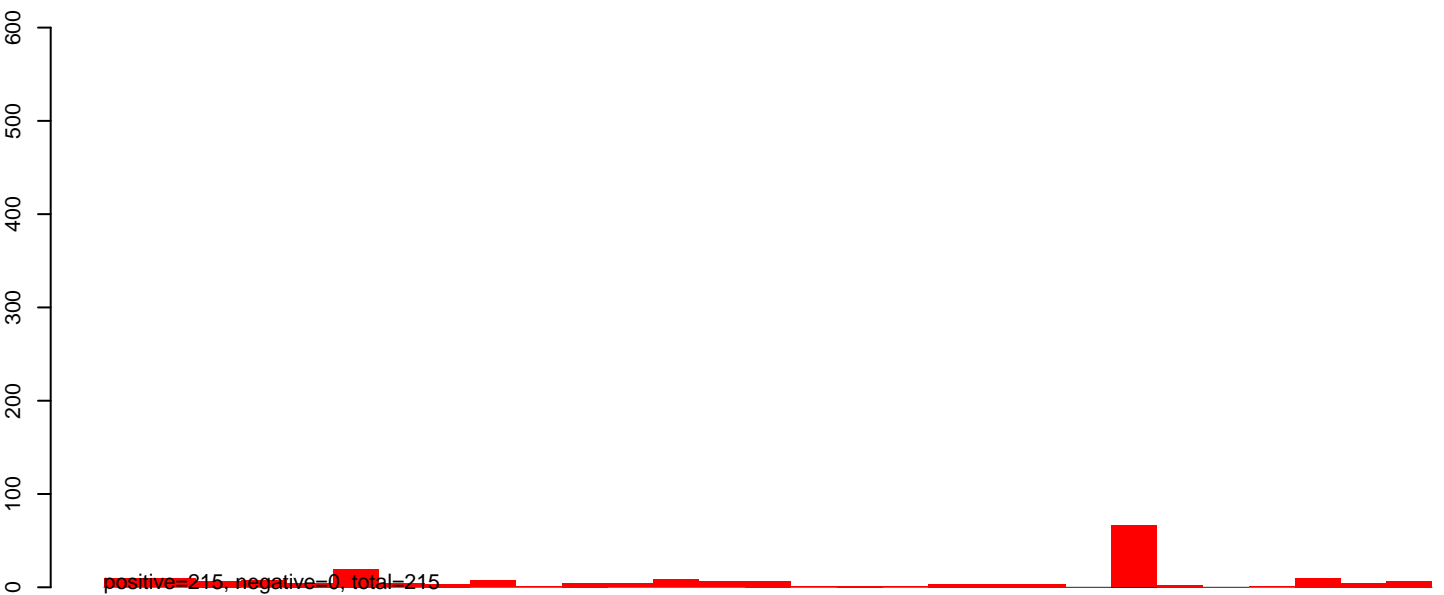
AeAeg_Aag2smallIRNA_DENV2K0048_rep2.rep
