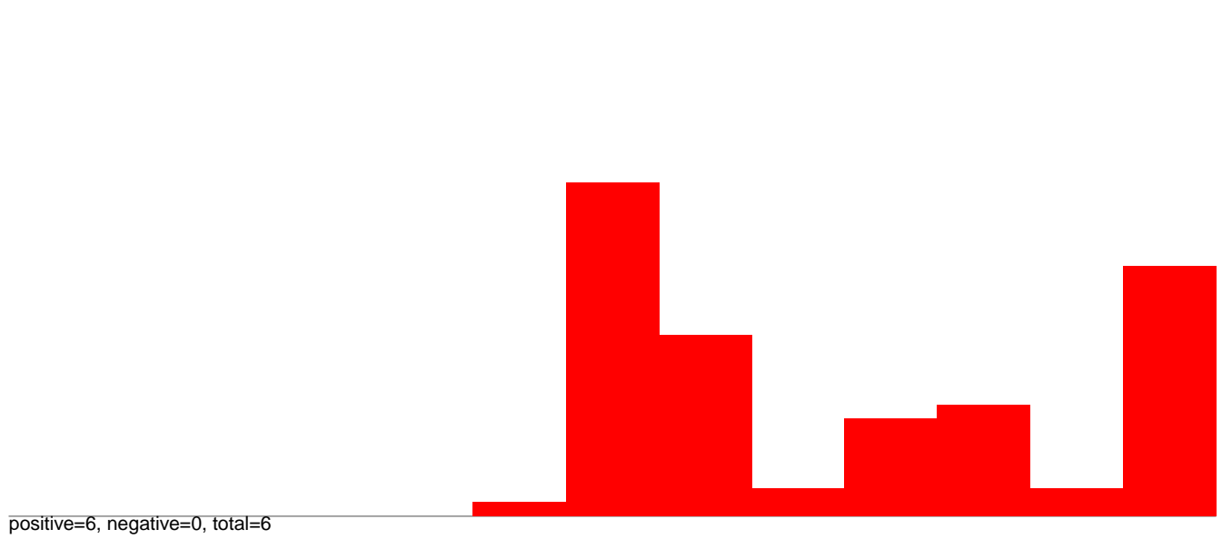
AeAeg_Aag2smallRNA_DENV2NGC_rep2.rep
