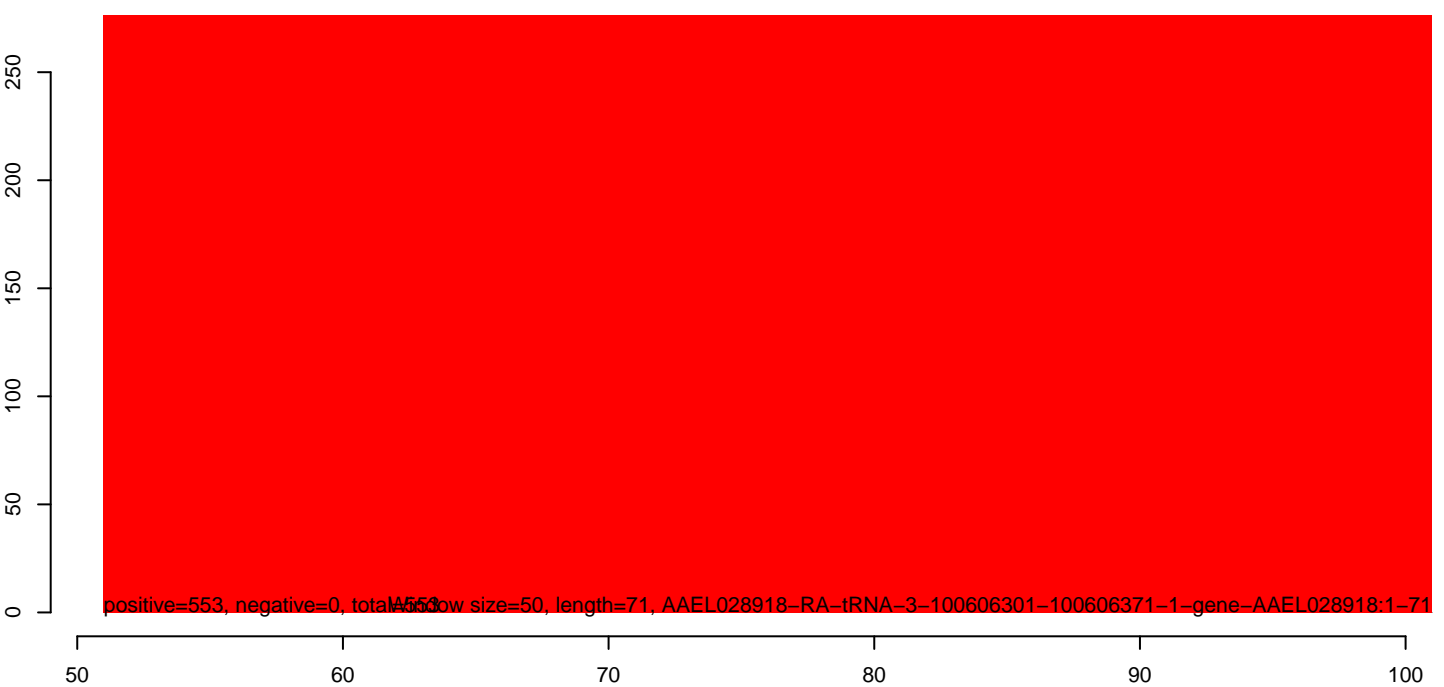
AeAeg_Aag2smallRNA_DENV2NGC_rep2.rep
