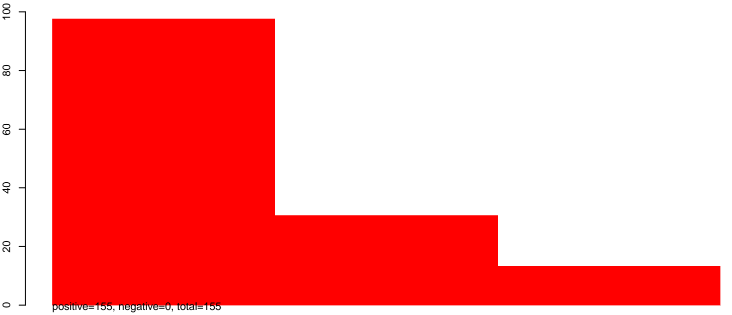
AeAeg_Aag2smallRNA_DENV2NGC_rep2.rep
