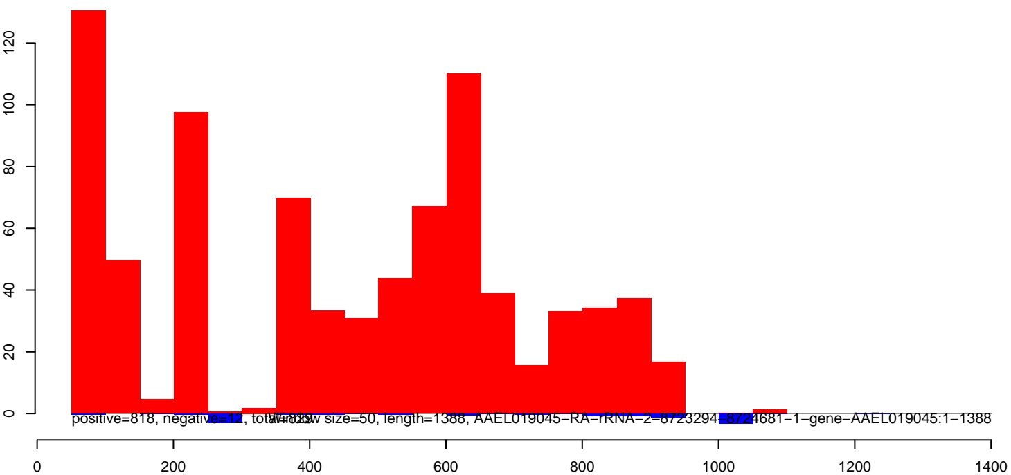
AeAeg_Aag2smallRNA_DENV2NGC_rep2.rep
