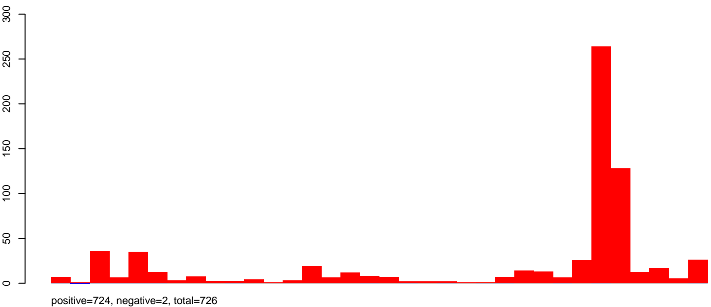
AeAeg_Aag2smallRNA_DENV2NGC_rep2.rep
