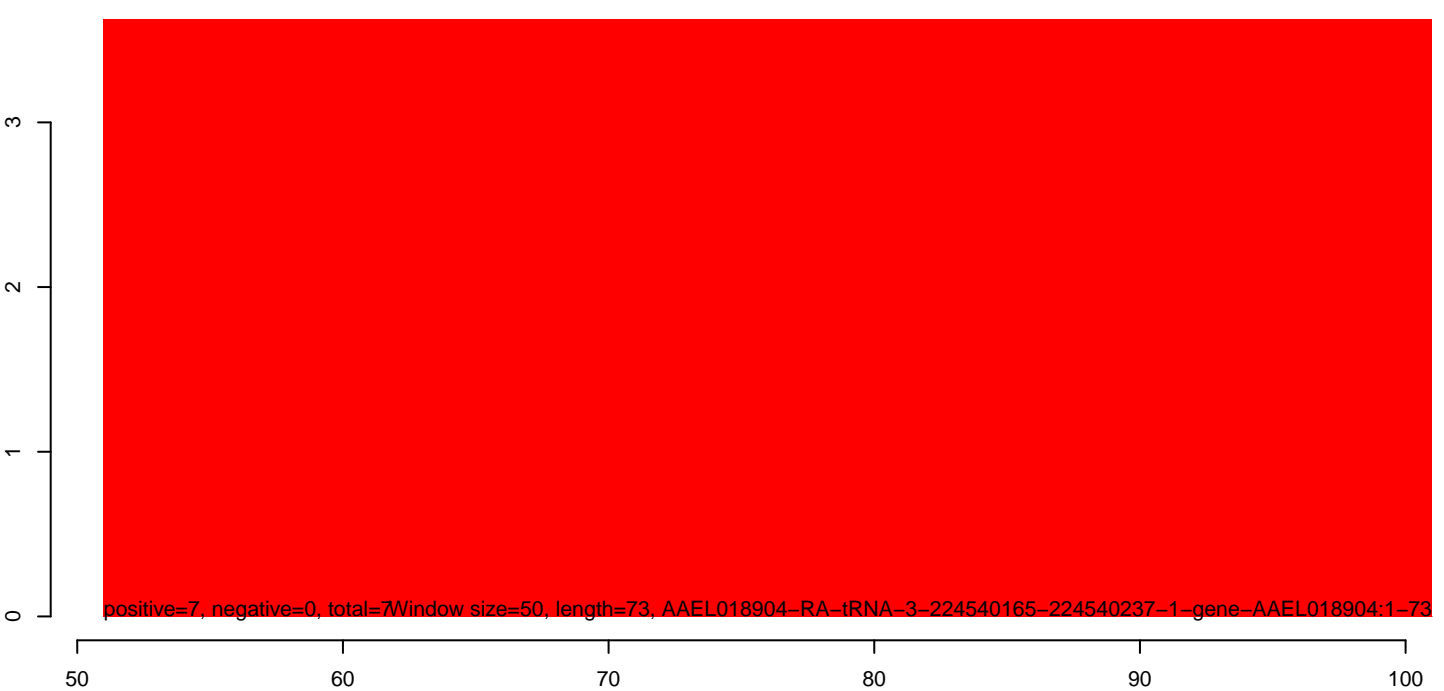
AeAeg_Aag2smallRNA_DENV2NGC_rep2.rep
