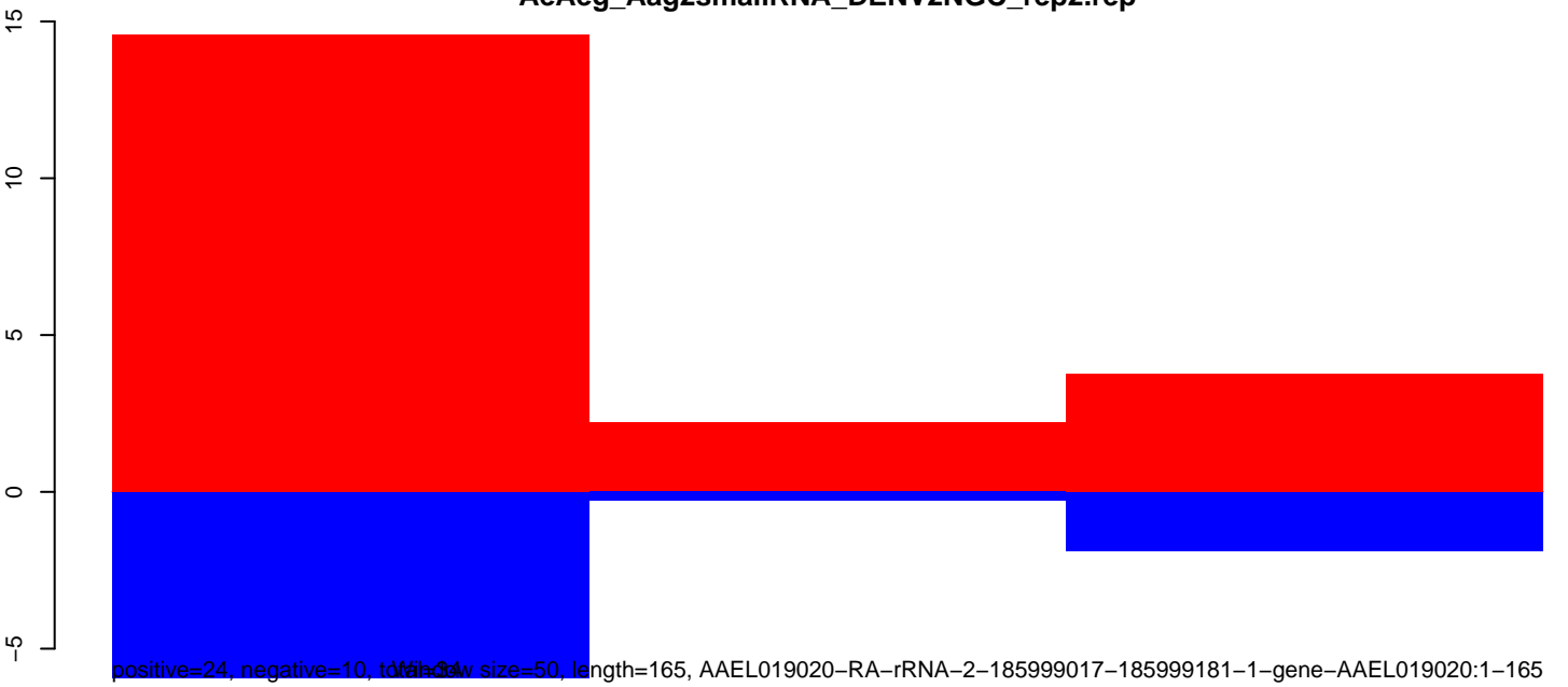
AeAeg_Aag2smallRNA_DENV2NGC_rep2.rep
