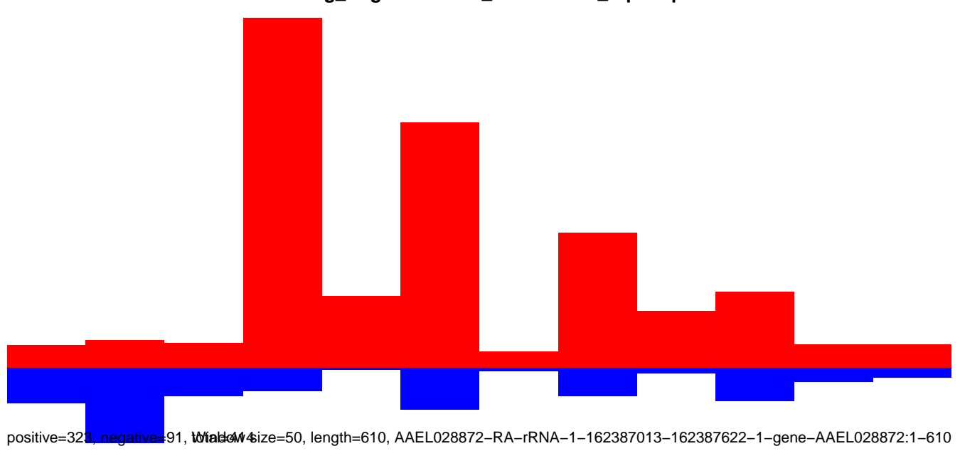
AeAeg_Aag2smallRNA_DENV2NGC_rep2.rep
