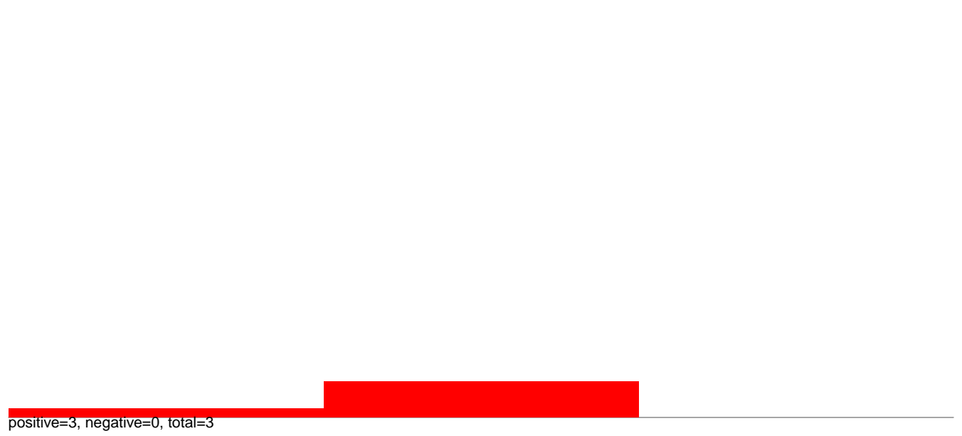
AeAeg_Aag2smallRNA_DENV2NGC_rep2.rep
