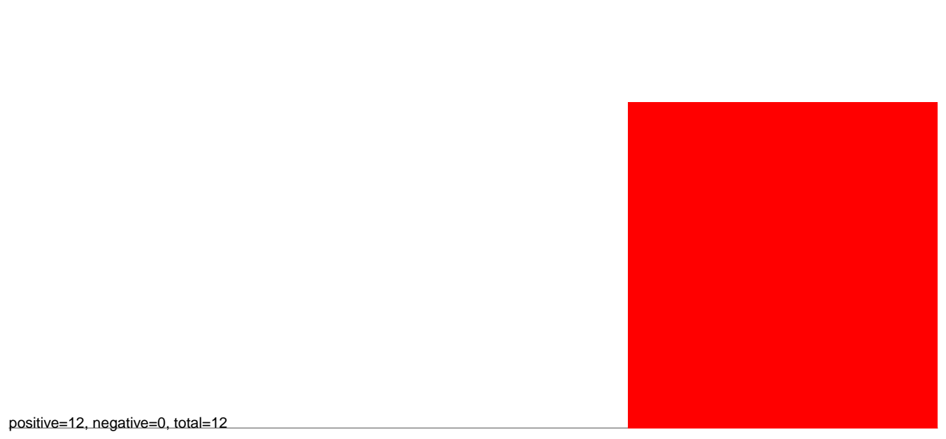
AeAeg_Aag2smallRNA_DENV2NGC_rep2.rep
