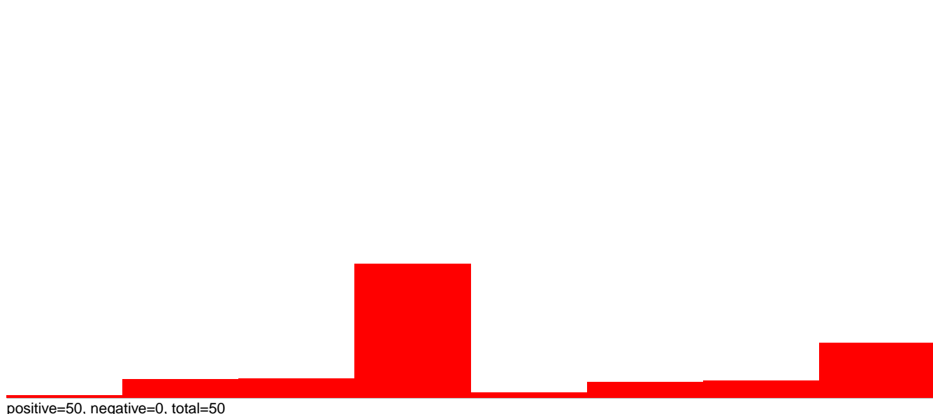
AeAeg_Aag2smallRNA_DENV2NGC_rep2.rep
