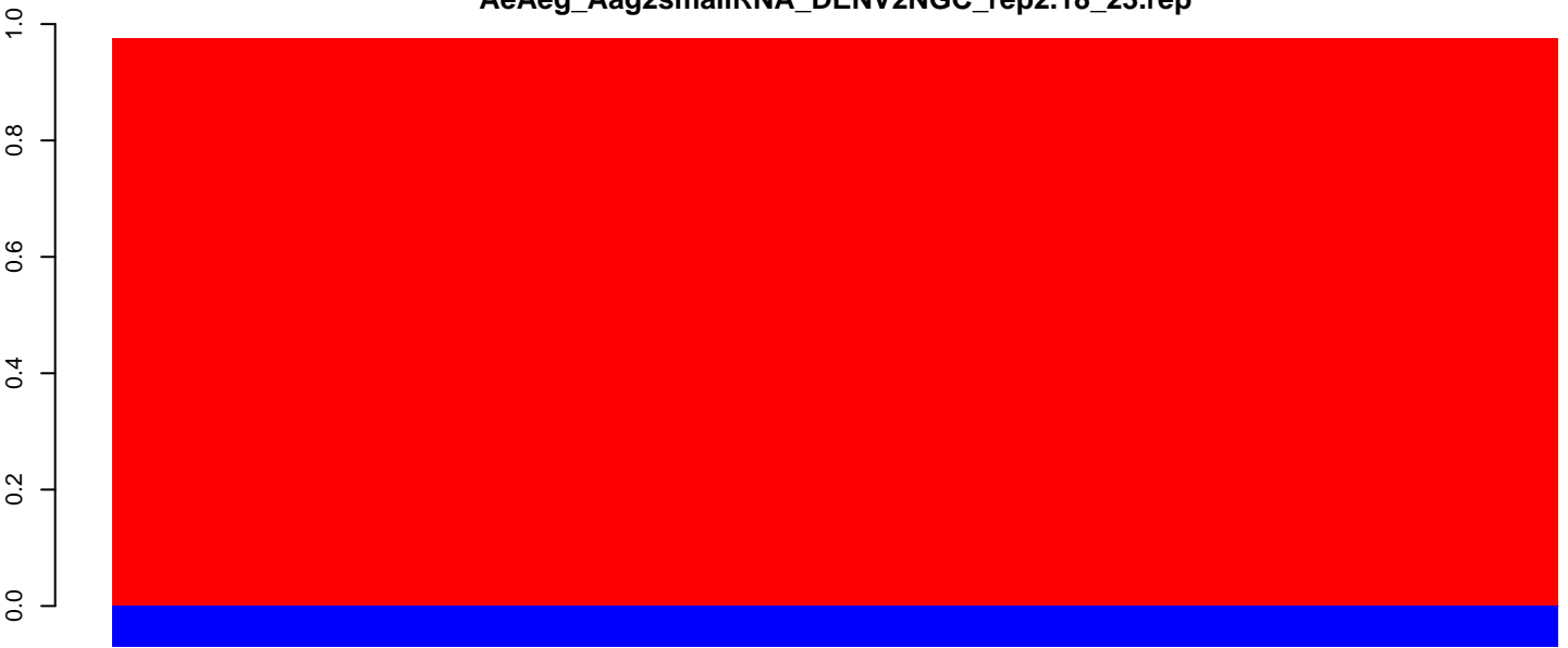
AeAeg_Aag2smallRNA_DENV2NGC_rep2.18_23.rep
