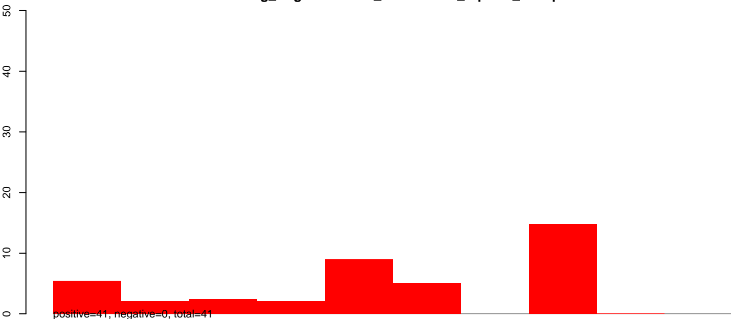
AeAeg_Aag2smallRNA_DENV2NGC_rep2.rep
