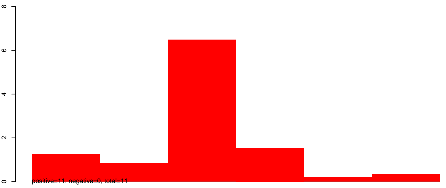
AeAeg_Aag2smallRNA_DENV2NGC_rep2.rep
