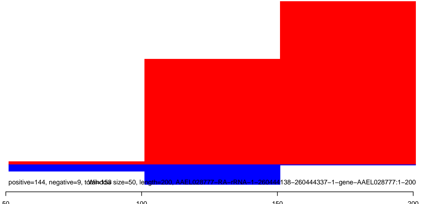
AeAeg_Aag2smallRNA_DENV2NGC_rep2.rep
