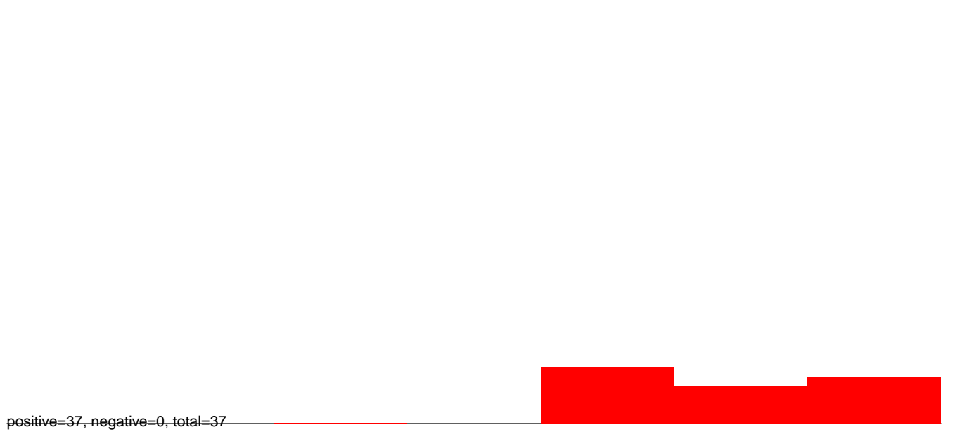
AeAeg_Aag2smallRNA_DENV2NGC_rep2.rep
