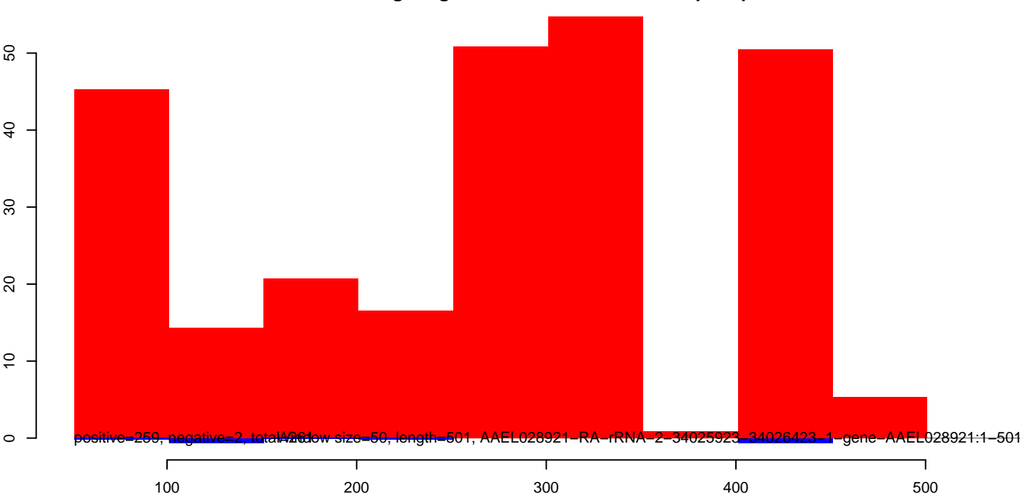
AeAeg_Aag2smallRNA_DENV2NGC_rep2.rep
