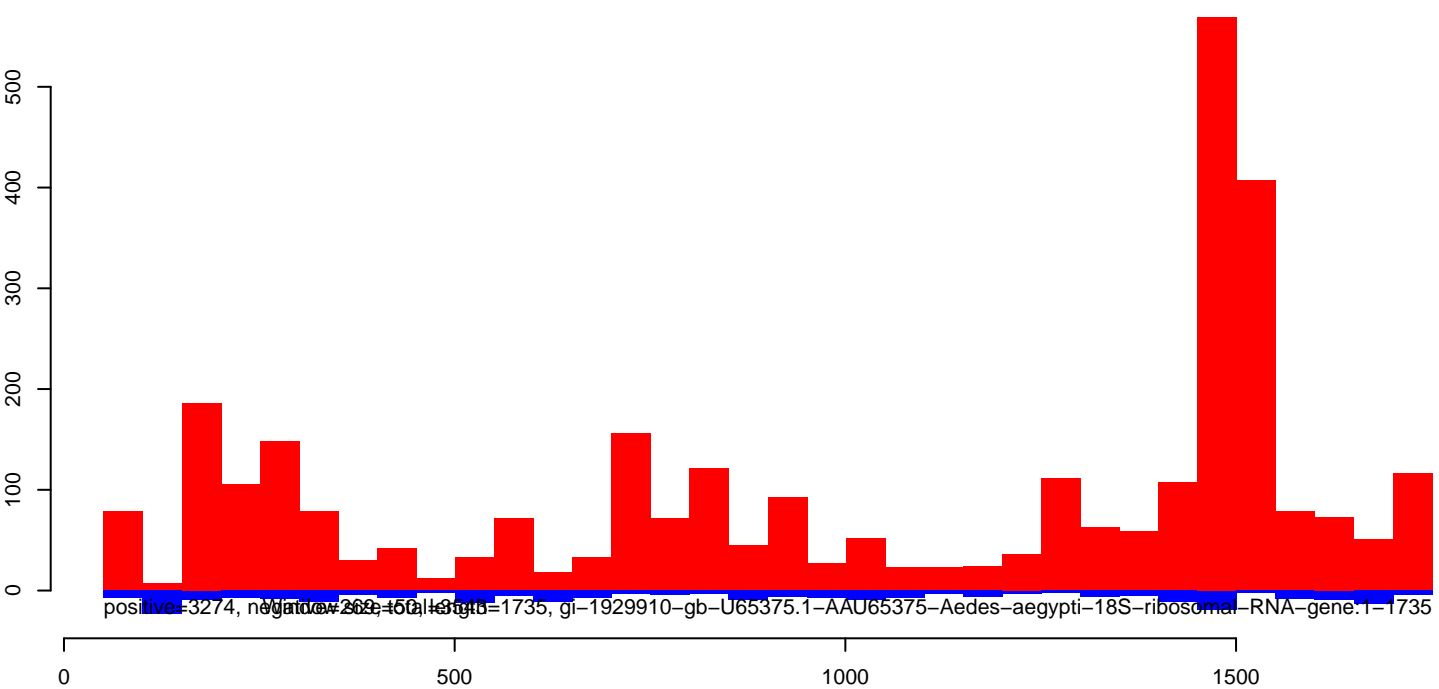
AeAeg_Aag2smallRNA_DENV2NGC_rep2.rep
