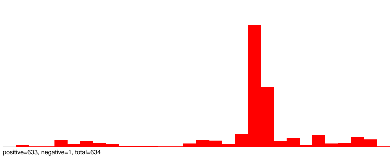
AeAeg_Aag2smallRNA_DENV2NGC_rep2.rep
