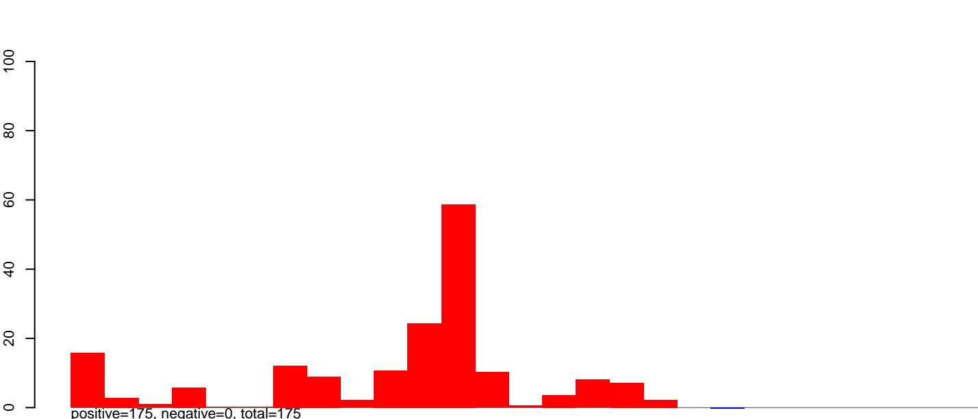
AeAeg_Aag2smallRNA_DENV2NGC_rep2.rep
