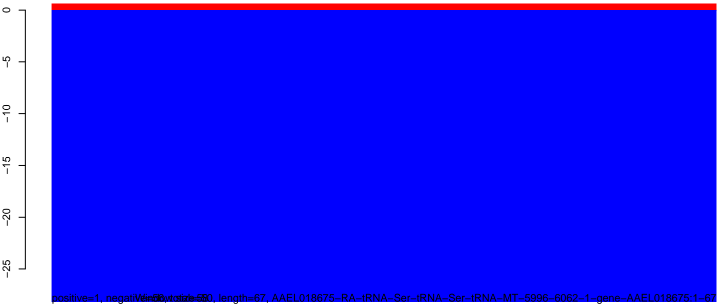
AeAeg_Aag2smallRNA_DENV2NGC_rep2.rep
