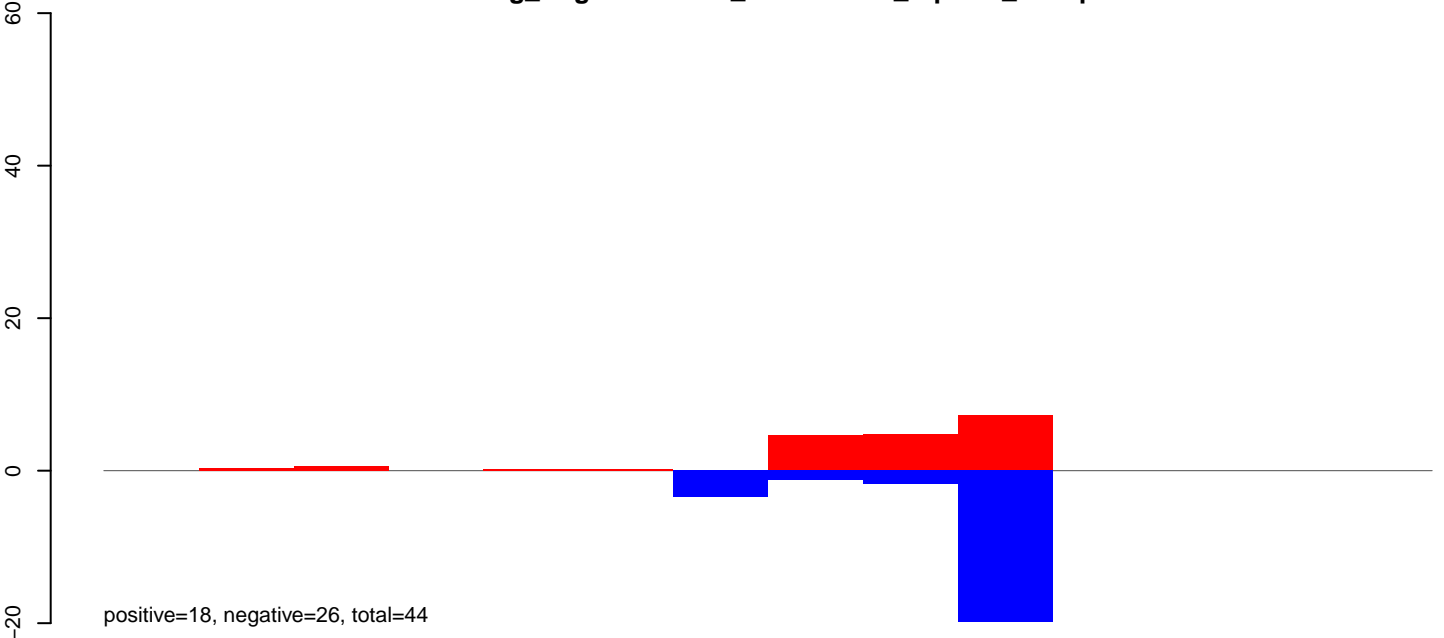
AeAeg_Aag2smallRNA_DENV2NGC_rep2.rep
