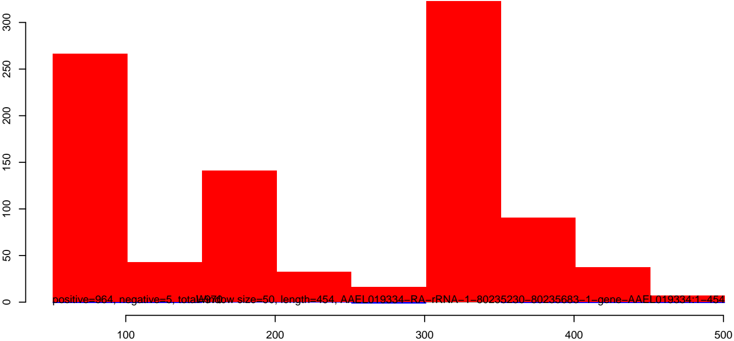
AeAeg_Aag2smallRNA_DENV2NGC_rep2.rep
