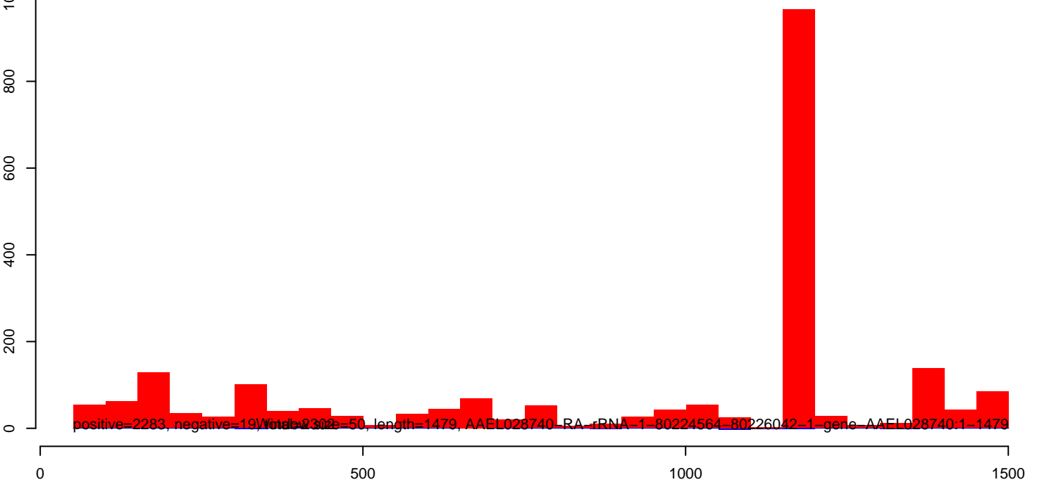
AeAeg_Aag2smallRNA_DENV2NGC_rep2.rep
