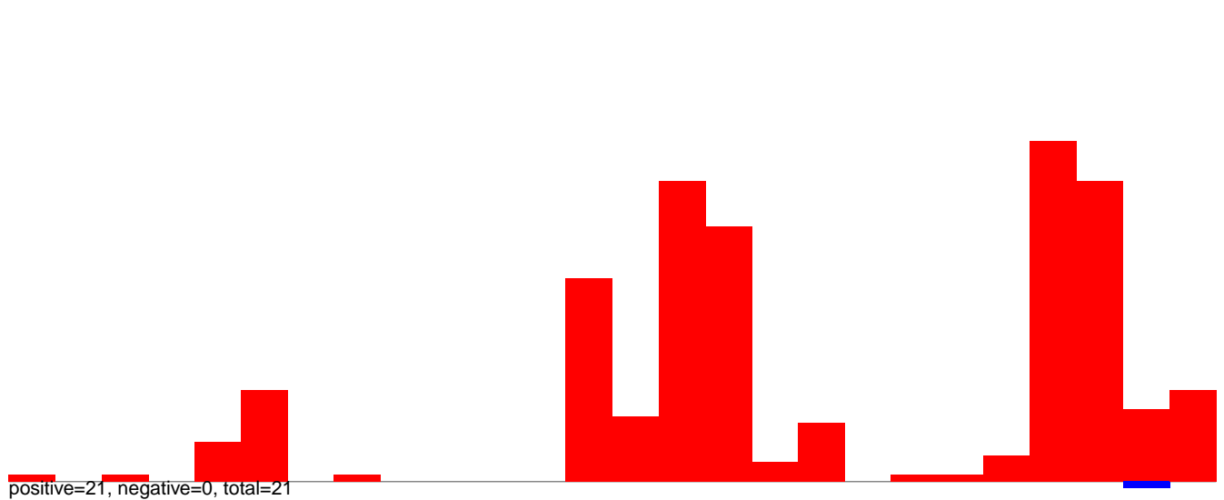
AeAeg_Aag2smallRNA_DENV2NGC_rep2.rep
