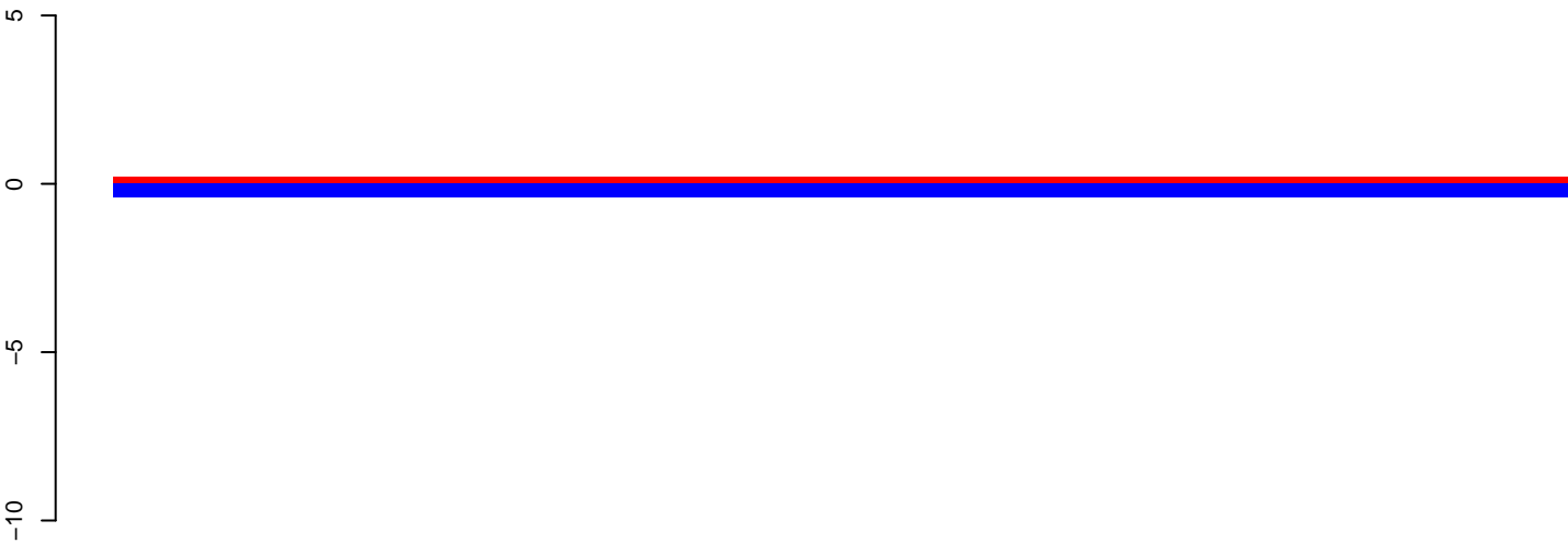
AeAeg_Aag2smallRNA_DENV2NGC_rep2.rep
