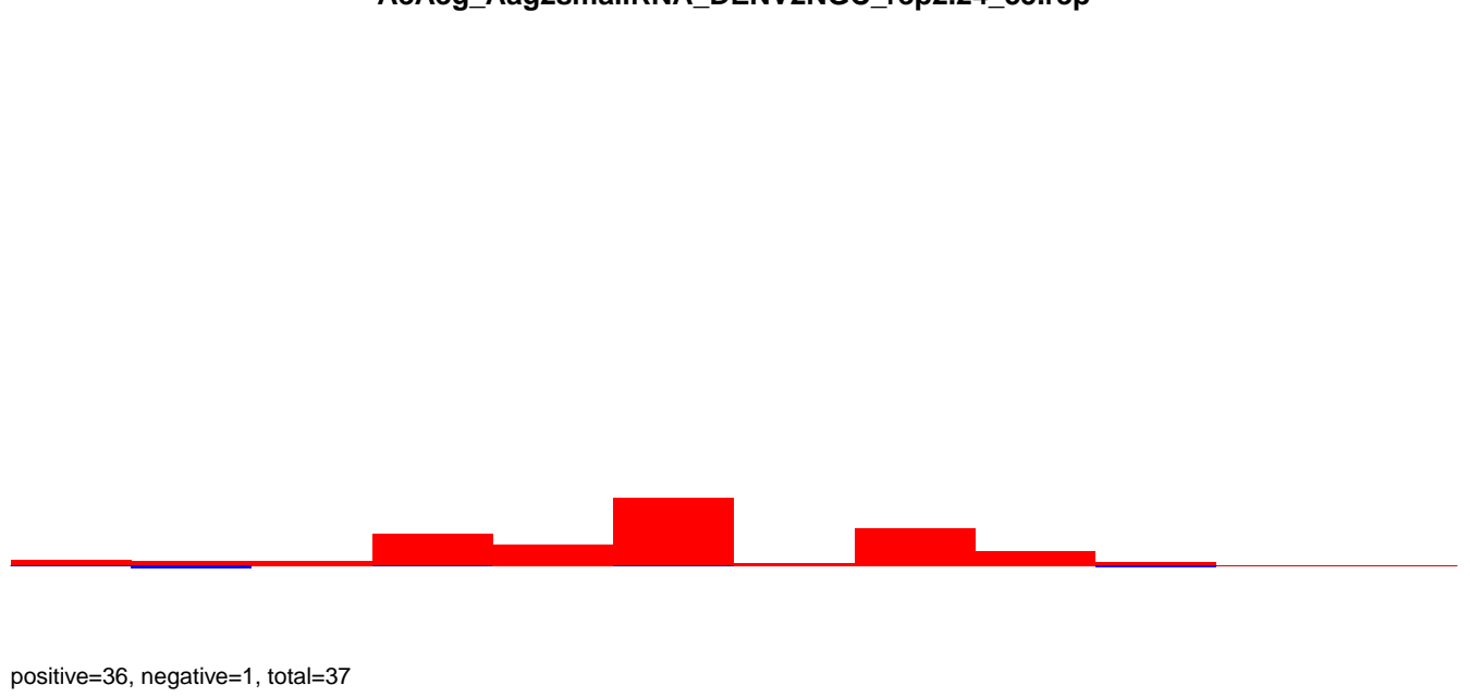
AeAeg_Aag2smallRNA_DENV2NGC_rep2.rep
