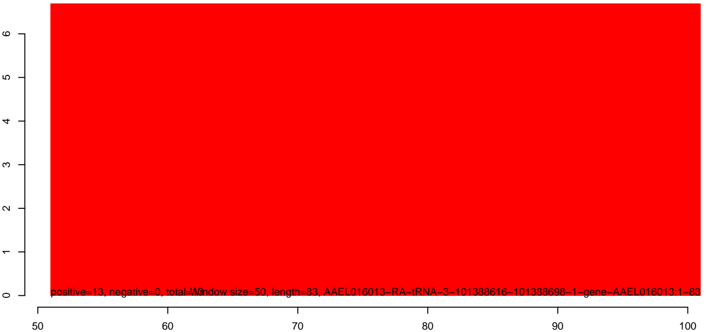
AeAeg_Aag2smallRNA_DENV2NGC_rep2.rep
