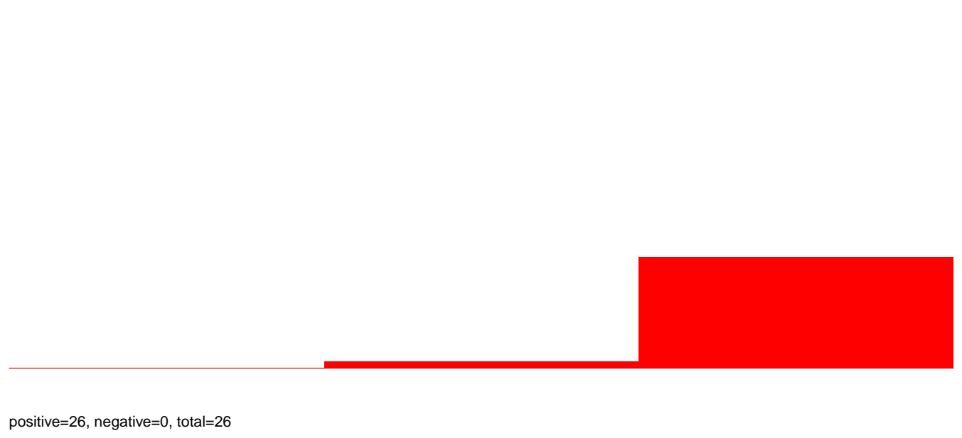
AeAeg_Aag2smallRNA_DENV2NGC_rep2.rep
