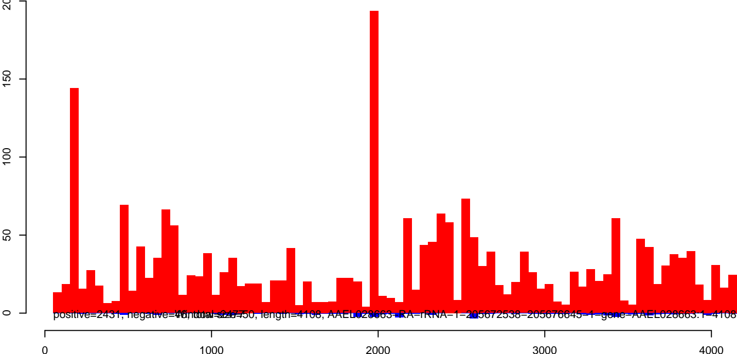
AeAeg_Aag2smallRNA_ZikaOW_rep1.rep
