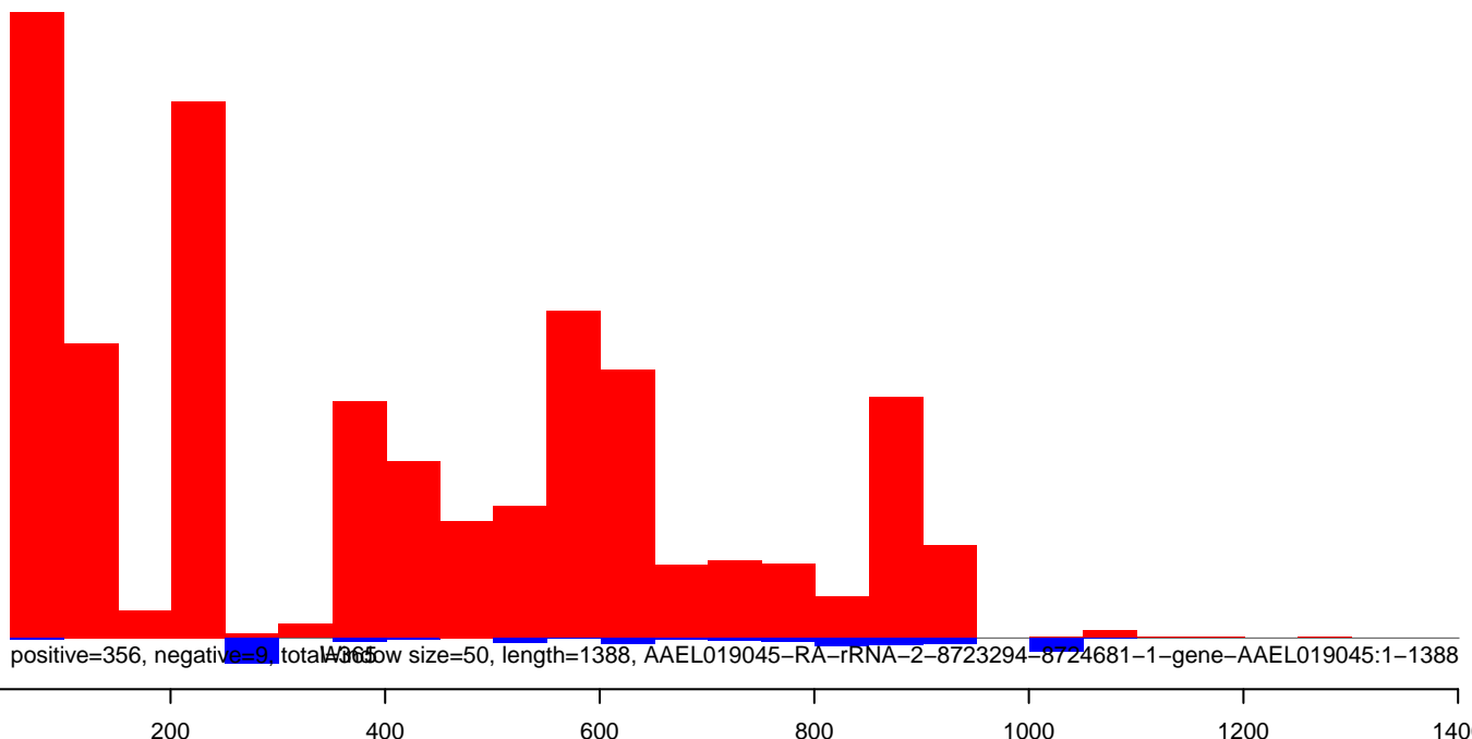
AeAeg_Aag2smallRNA_ZikaOW_rep1.rep
