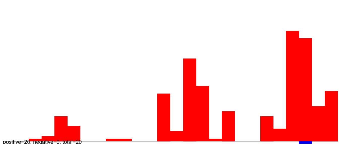
AeAeg_Aag2smallRNA_ZikaOW_rep1.rep
