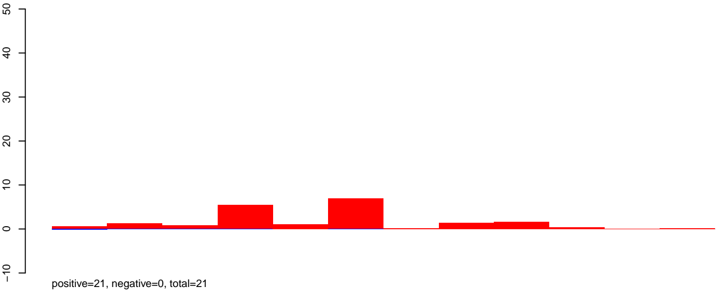
AeAeg_Aag2smallRNA_ZikaOW_rep1.rep
