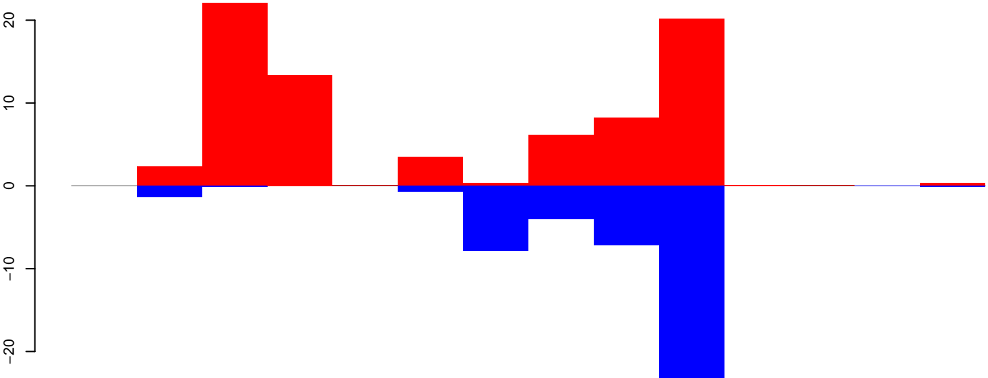
AeAeg_Aag2smallRNA_ZikaOW_rep1.rep
