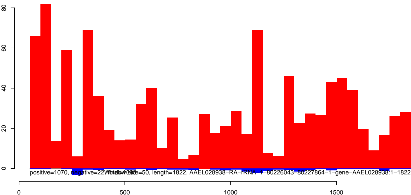
AeAeg_Aag2smallRNA_ZikaOW_rep1.rep
