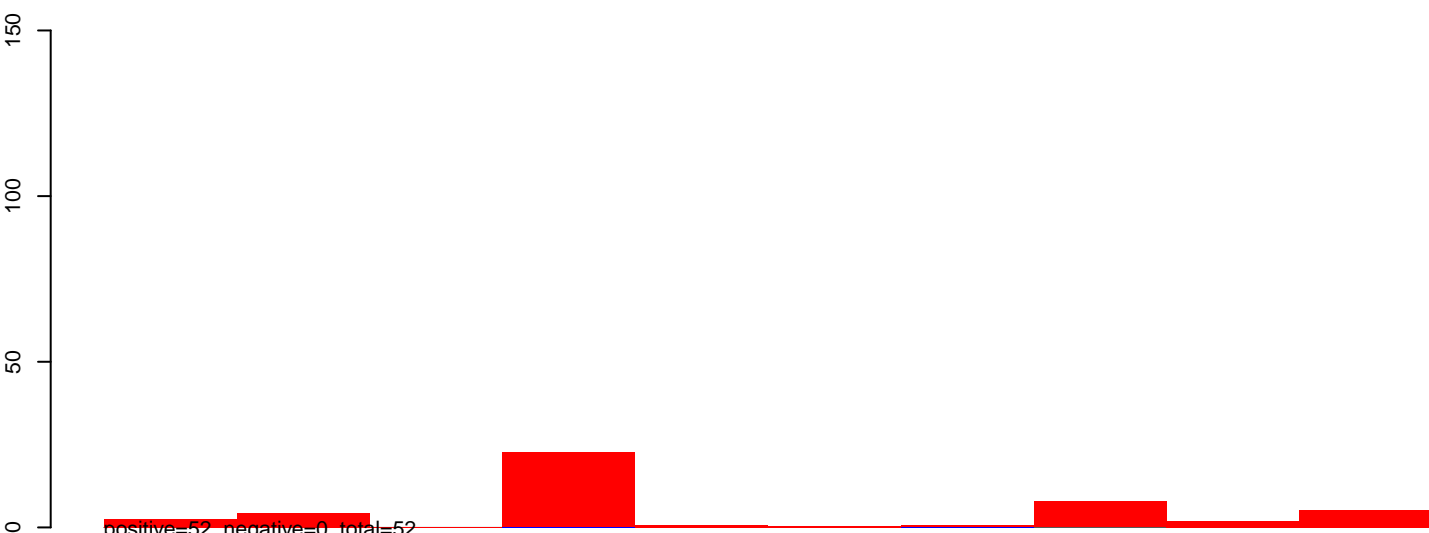
AeAeg_Aag2smallRNA_ZikaOW_rep1.rep
