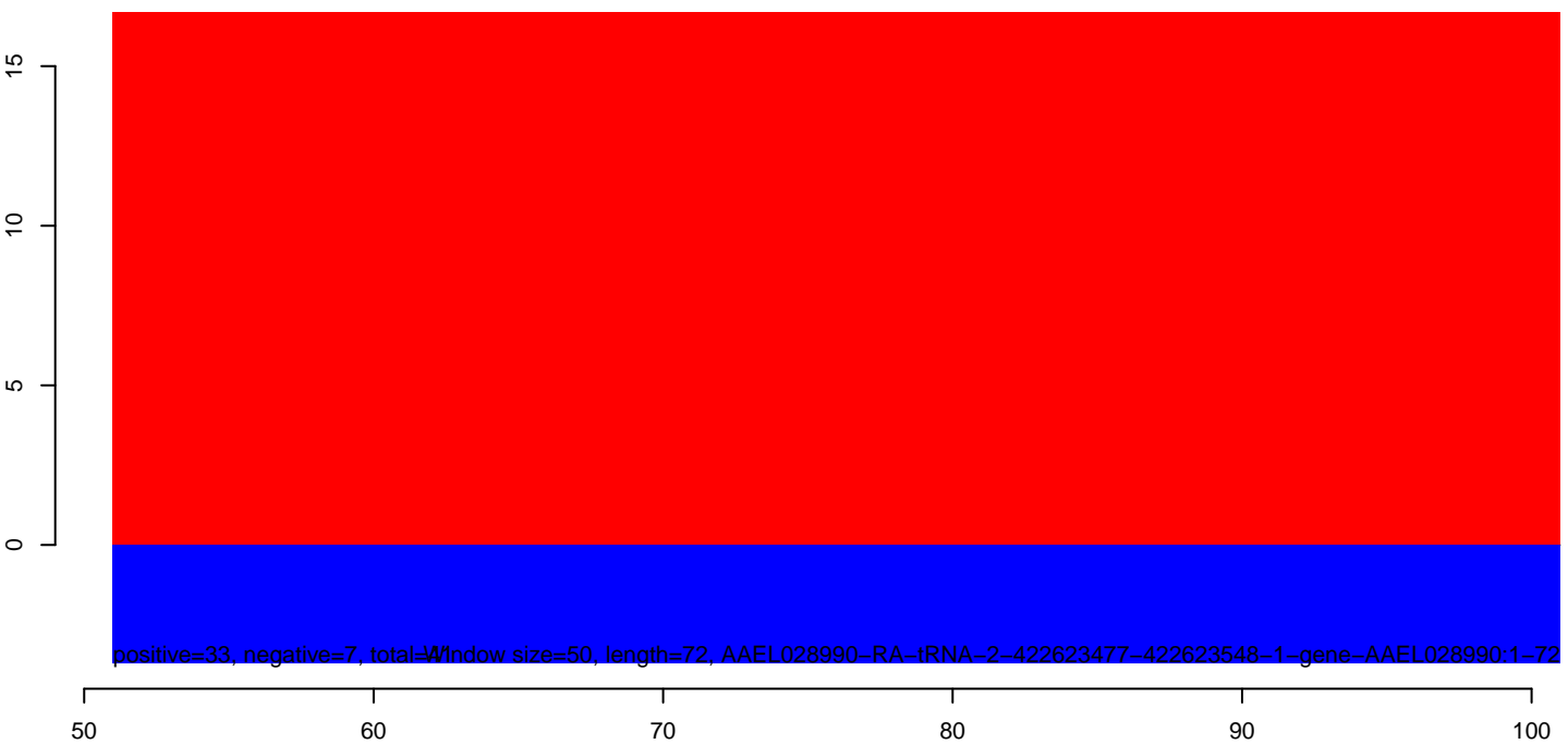
AeAeg_Aag2smallRNA_ZikaOW_rep1.rep
