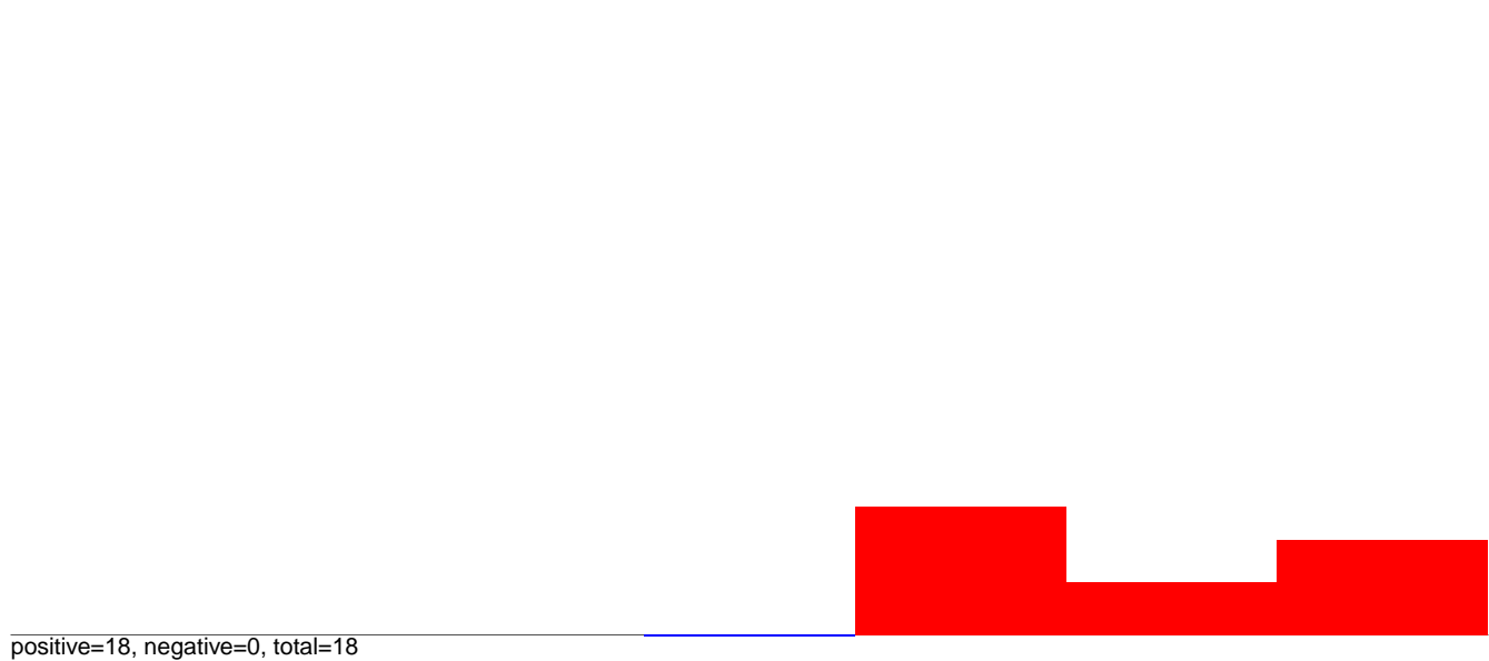
AeAeg_Aag2smallRNA_ZikaOW_rep1.rep
