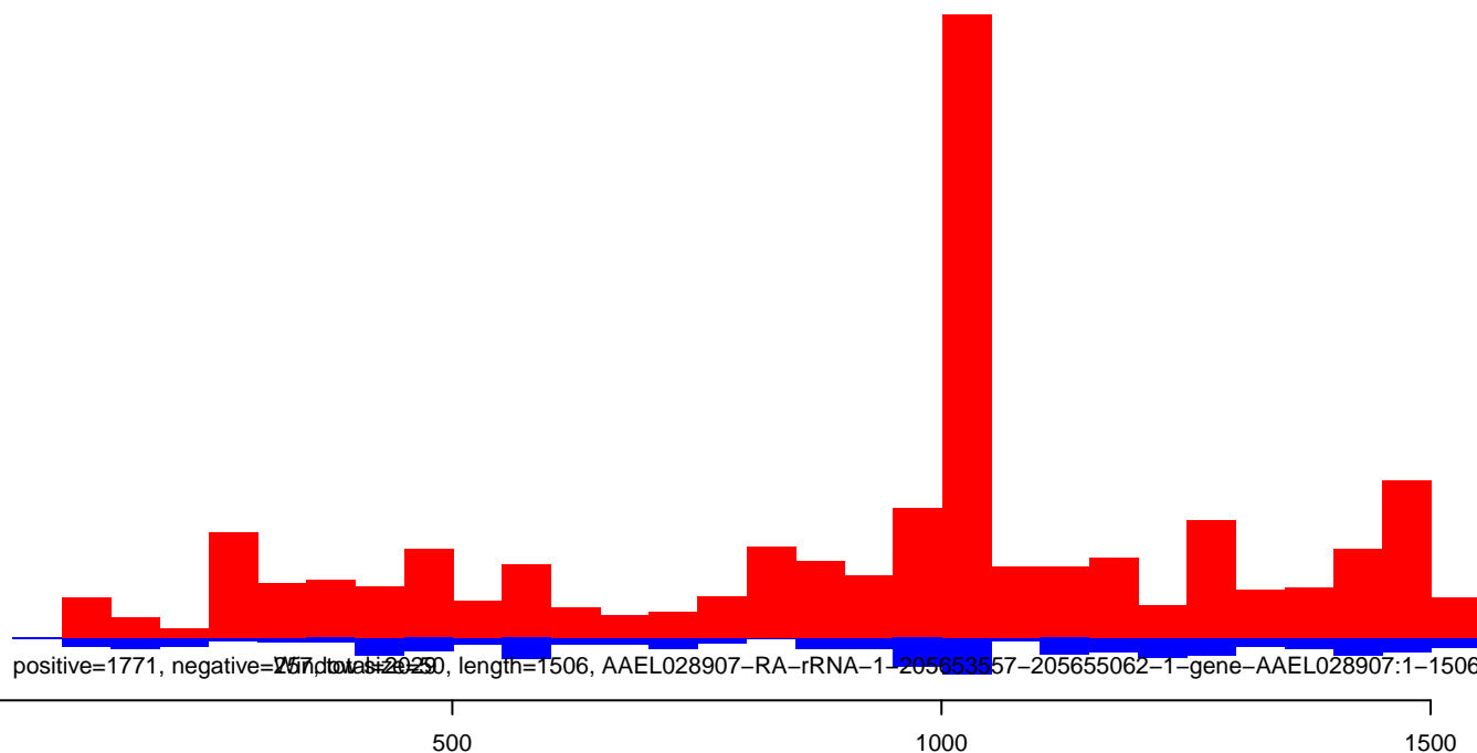
AeAeg_Aag2smallRNA_ZikaOW_rep1.rep
