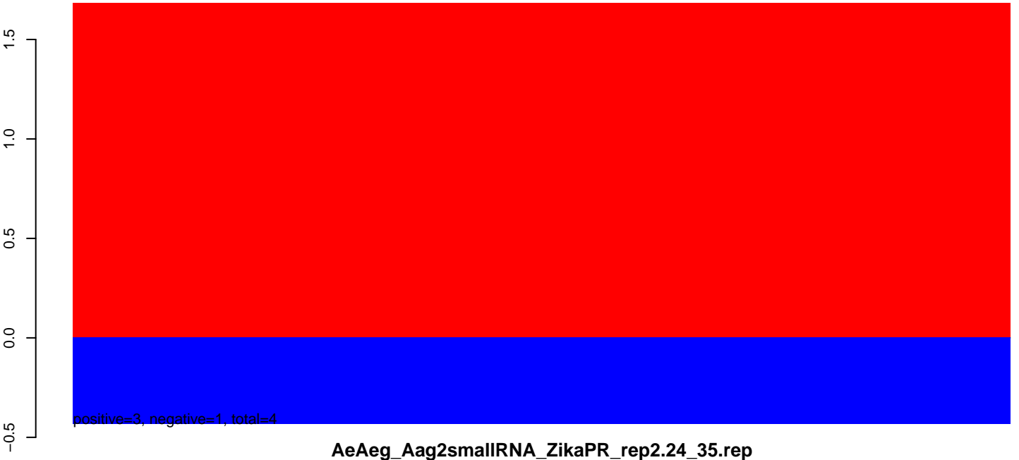
AeAeg_Aag2smallRNA_ZikaPR_rep2.18_23.rep
