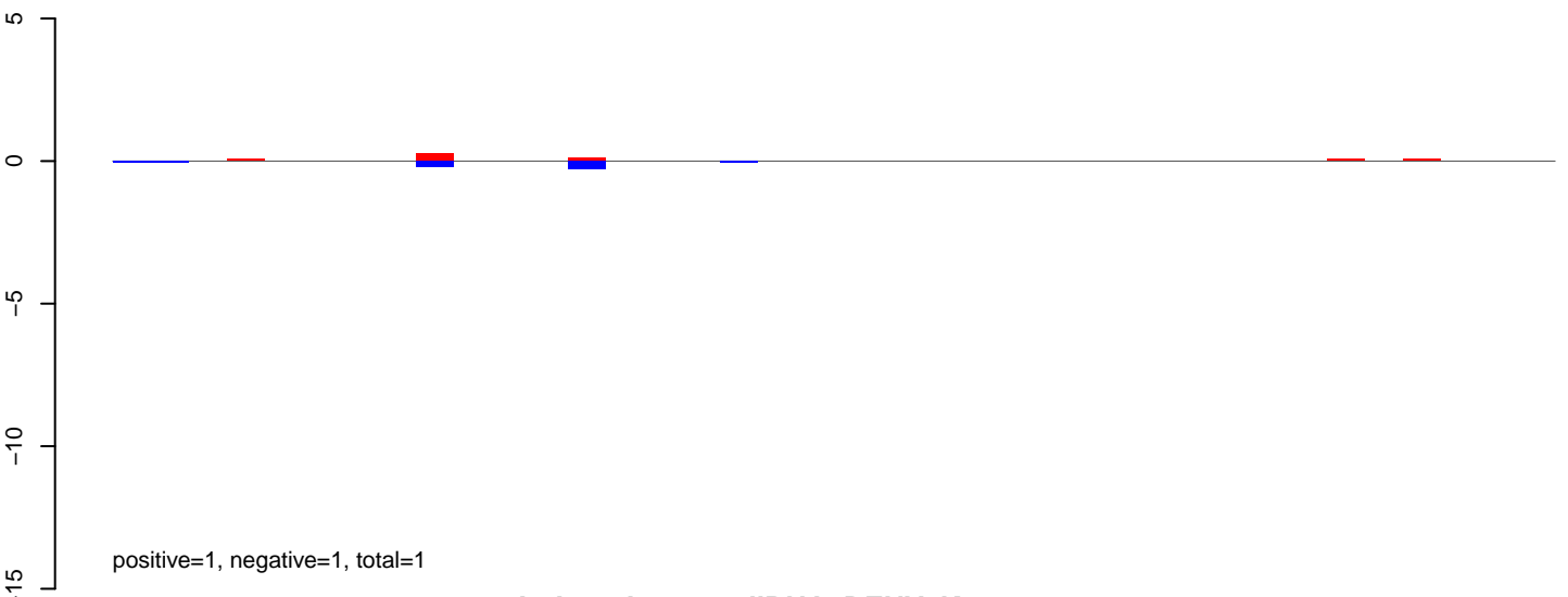
AeAeg_Aag2smallRNA_DENV2K0048_rep2.rep
