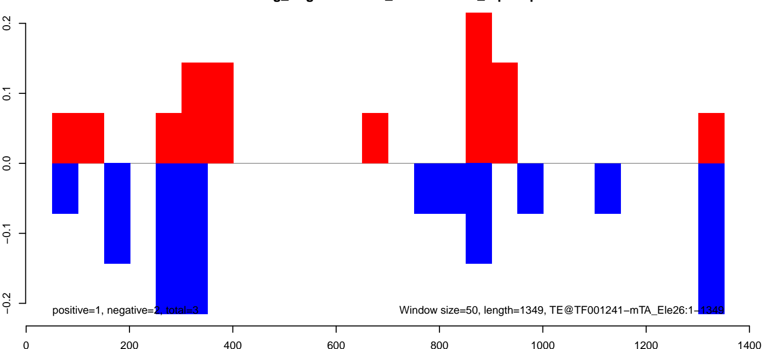
AeAeg_Aag2smallIRNA_DENV2K0048_rep2.rep
