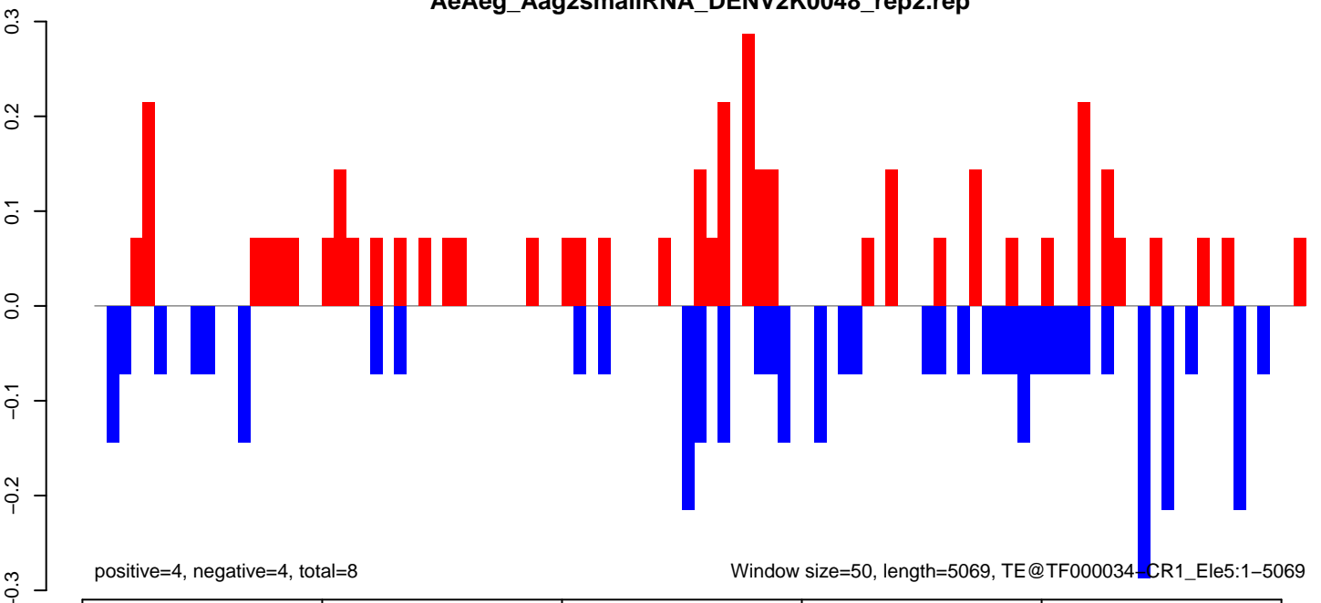
AeAeg_Aag2smallRNA_DENV2K0048_rep2.rep
