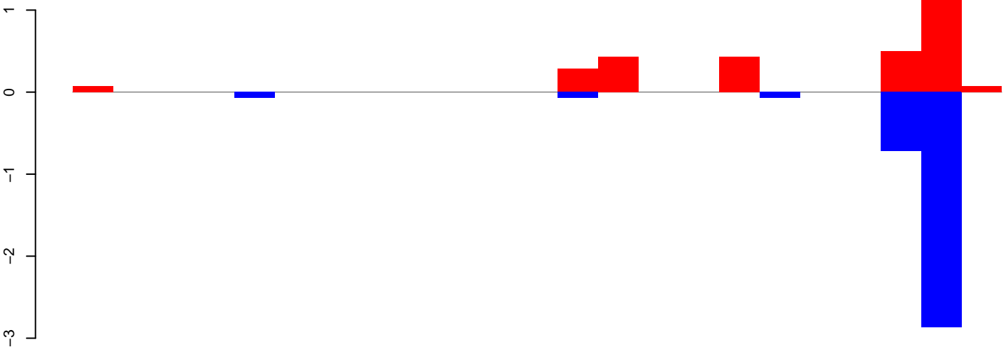
AeAeg_Aag2smallRNA_DENV2K0048_rep2.18_23.rep
