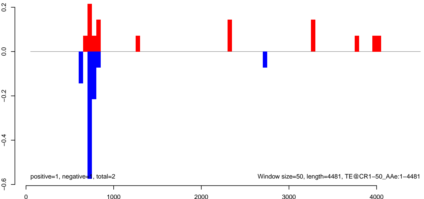
AeAeg_Aag2smallIRNA_DENV2K0048_rep2.rep
