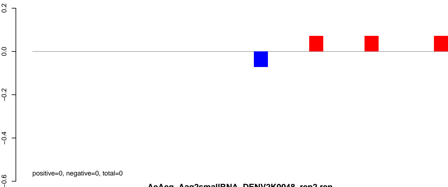
AeAeg_Aag2smallRNA_DENV2K0048_rep2.rep
