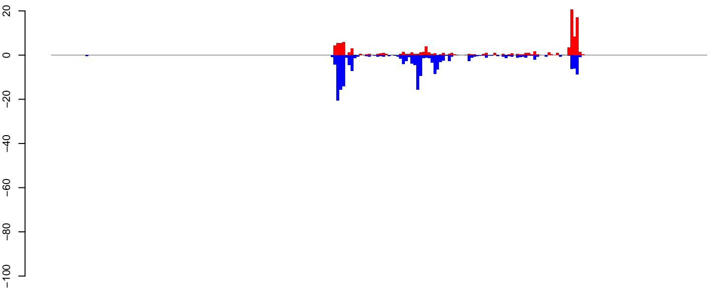
AeAeg_Aag2smallRNA_DENV2K0048_rep2.18_23.rep
