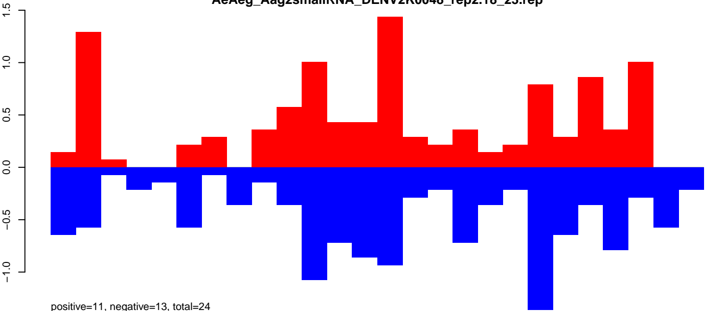
AeAeg_Aag2smallIRNA_DENV2K0048_rep2.24_35.rep
