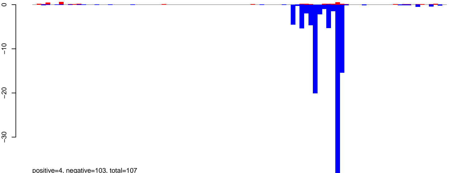
AeAeg_Aag2smallRNA_DENV2K0048_rep2.rep
