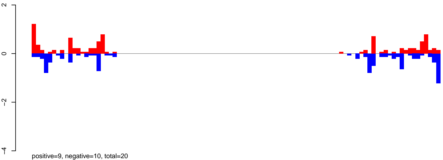
AeAeg_Aag2smallRNA_DENV2K0048_rep2.24_35.rep
