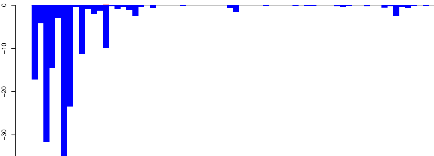
AeAeg_Aag2smallRNA_DENV2K0048_rep2.rep
