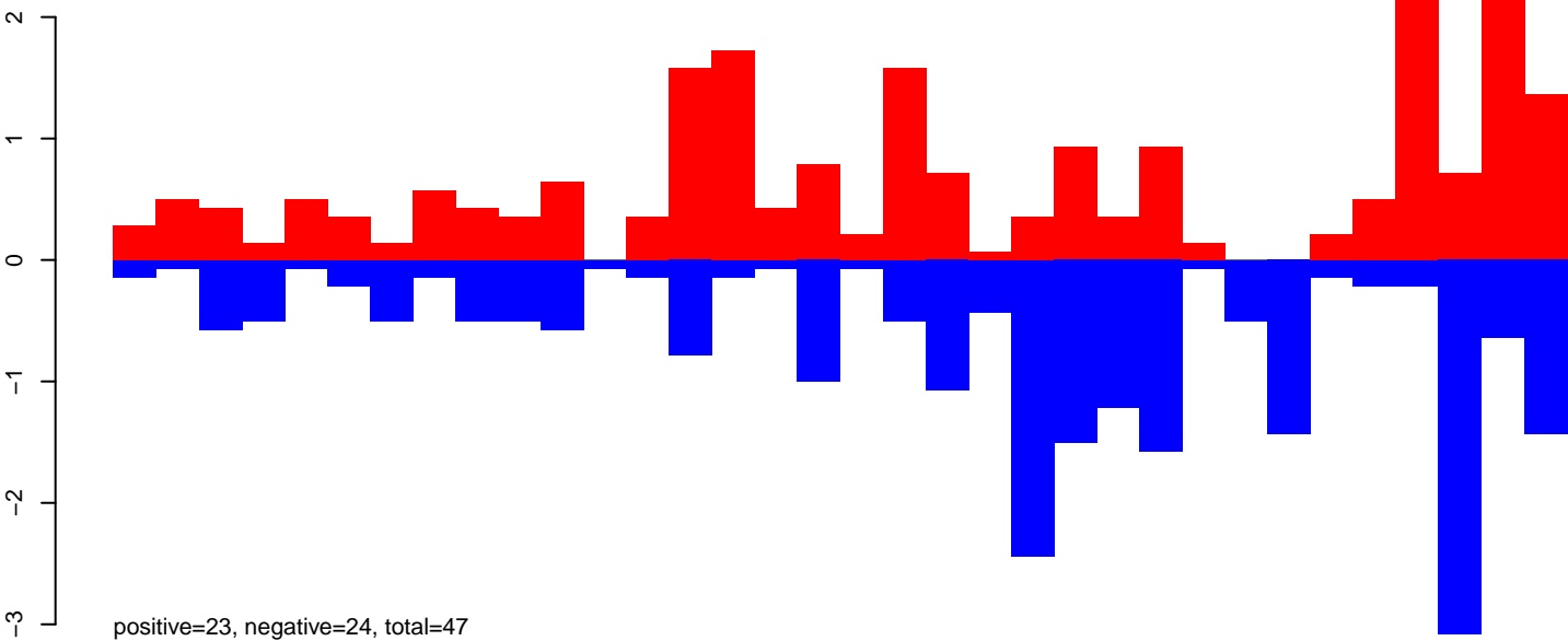
AeAeg_Aag2smallRNA_DENV2K0048_rep2.24_35.rep
