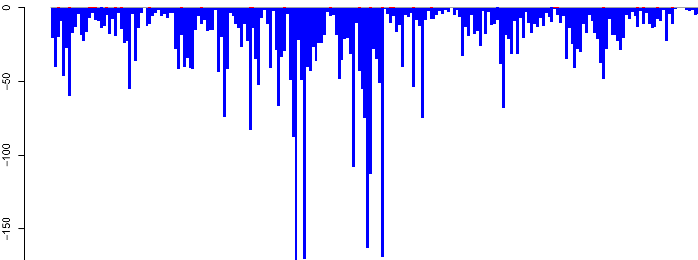
AeAeg_Aag2smallRNA_DENV2K0048_rep2.rep
