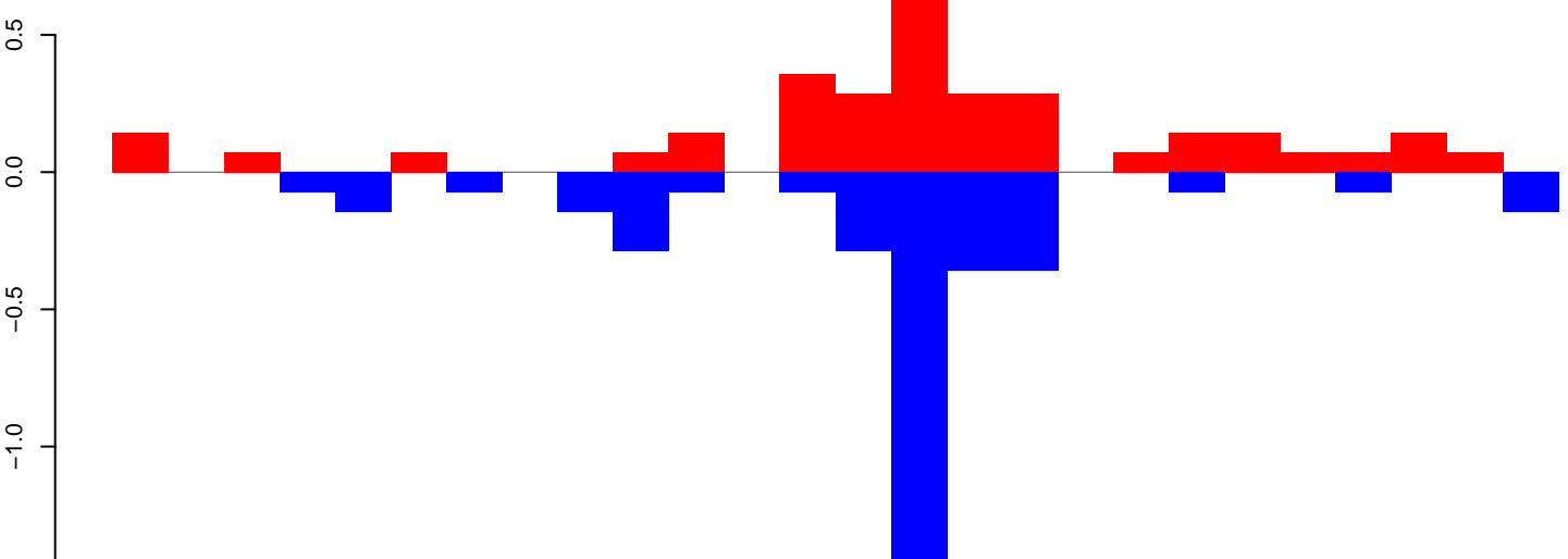
AeAeg_Aag2smallRNA_DENV2K0048_rep2.rep
