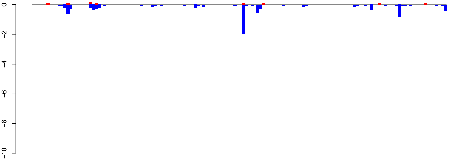
AeAeg_Aag2smallRNA_DENV2K0048_rep2.24_35.rep
