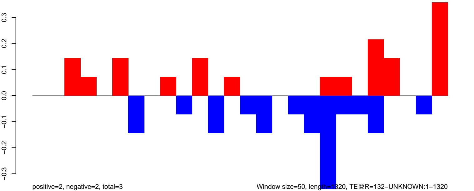
AeAeg_Aag2smallRNA_DENV2K0048_rep2.rep
