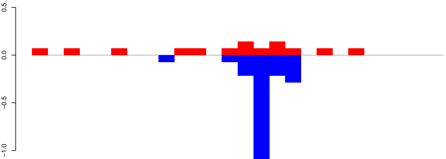
AeAeg_Aag2smallRNA_DENV2K0048_rep2.24_35.rep
