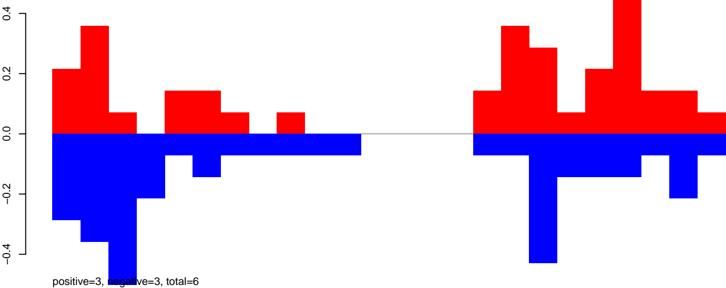
AeAeg_Aag2smallIRNA_DENV2K0048_rep2.24_35.rep
