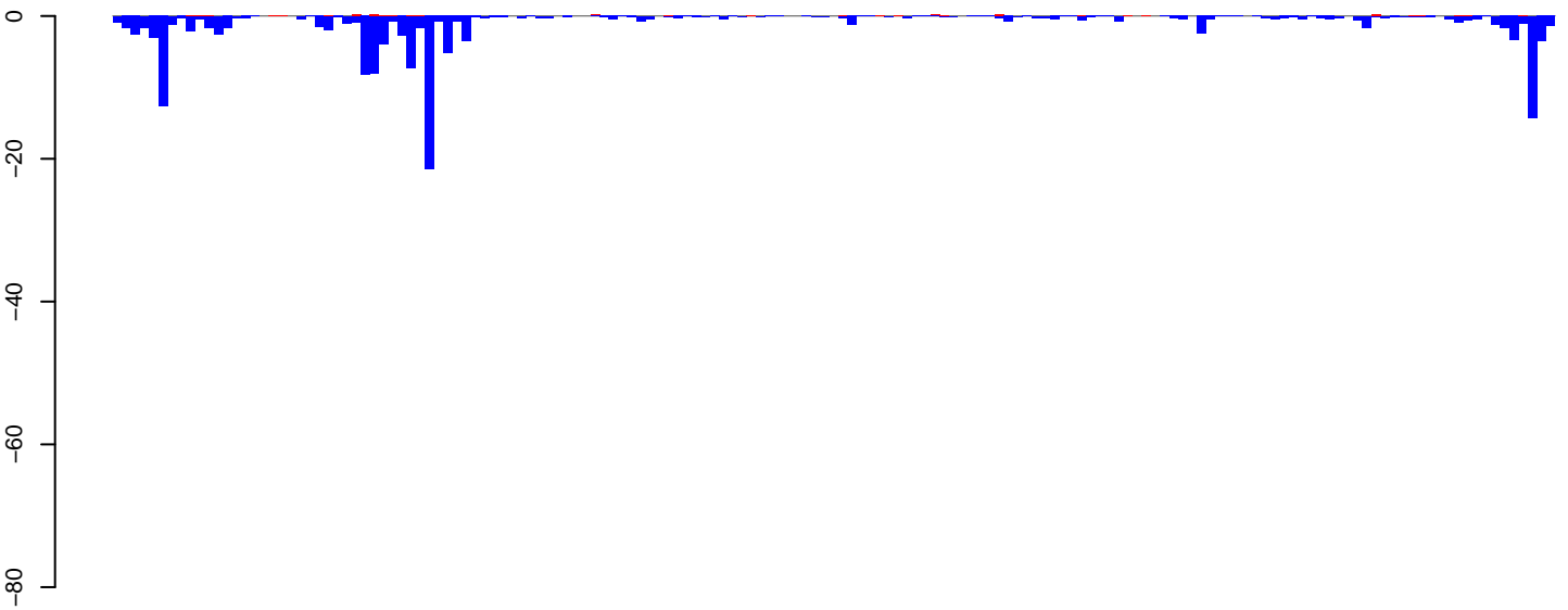
AeAeg_Aag2smallRNA_DENV2K0048_rep2.18_23.rep
