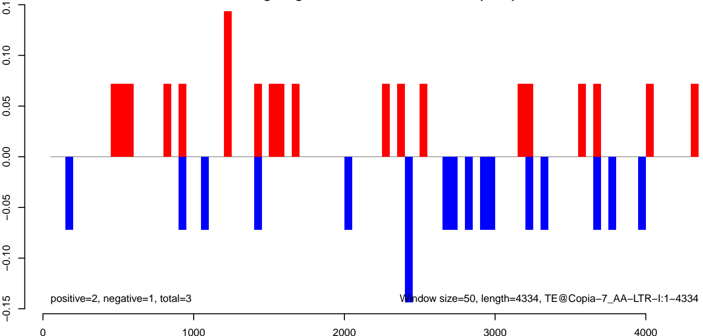
AeAeg_Aag2smallIRNA_DENV2K0048_rep2.rep
