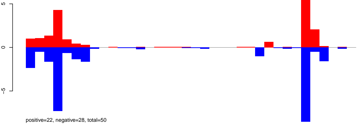
AeAeg_Aag2smallRNA_DENV2K0048_rep2.24_35.rep
