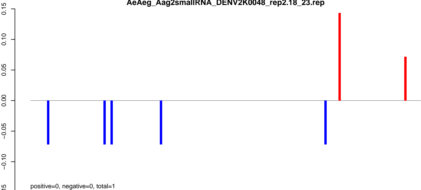
AeAeg_Aag2smallIRNA_DENV2K0048_rep2.24_35.rep
