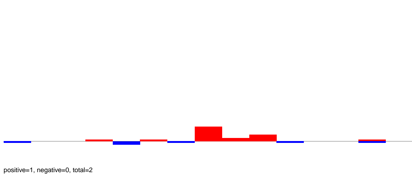
AeAeg_Aag2smallRNA_DENV2K0048_rep2.rep
