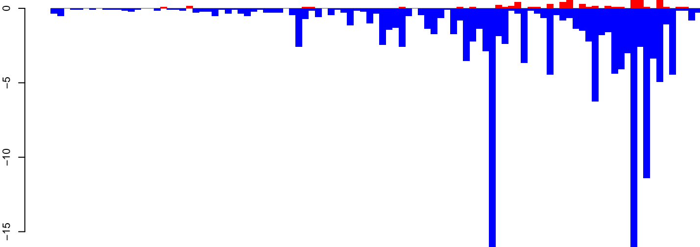
AeAeg_Aag2smallRNA_DENV2K0048_rep2.rep
