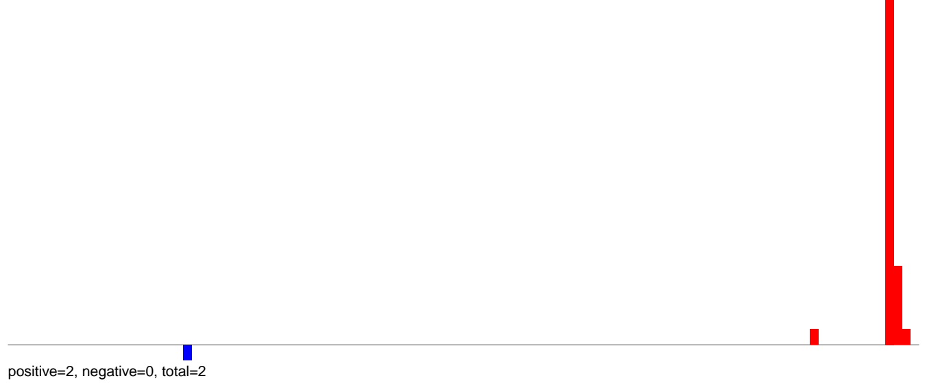
AeAeg_Aag2smallRNA_DENV2K0048_rep2.rep
