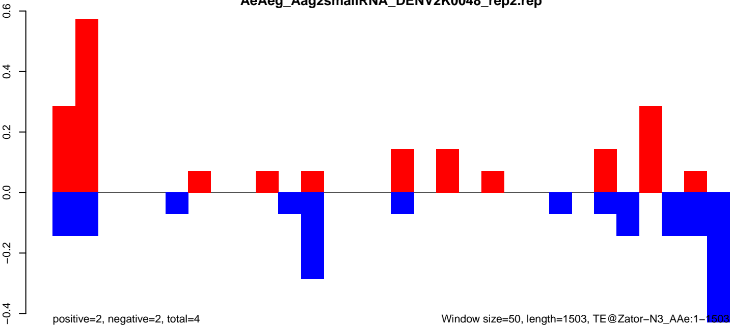
AeAeg_Aag2smallRNA_DENV2K0048_rep2.rep
