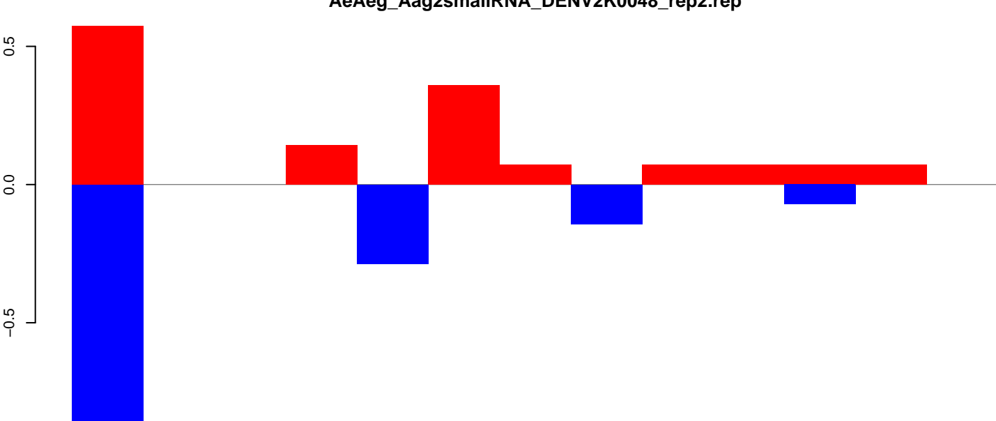
AeAeg_Aag2smallRNA_DENV2K0048_rep2.rep
