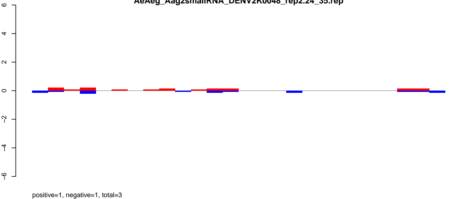
AeAeg_Aag2smallRNA_DENV2K0048_rep2.rep
