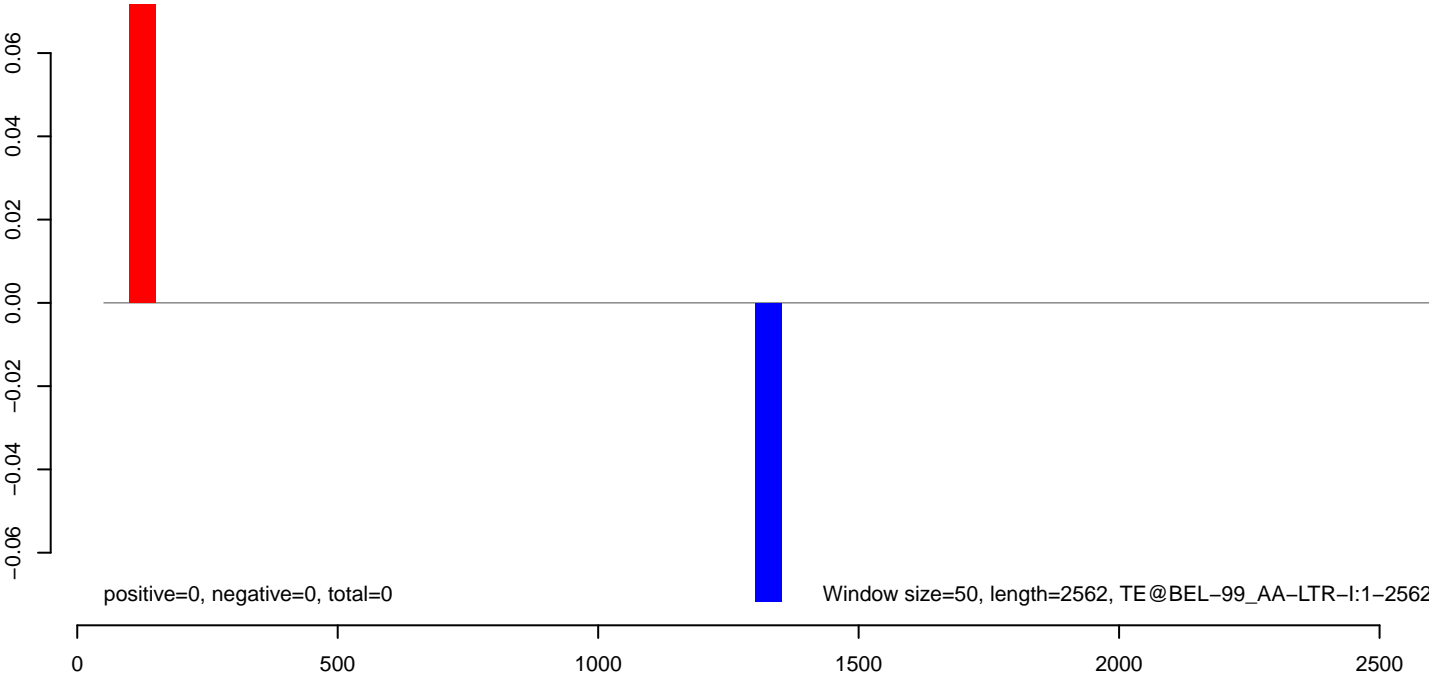
AeAeg_Aag2smallRNA_DENV2K0048_rep2.rep
