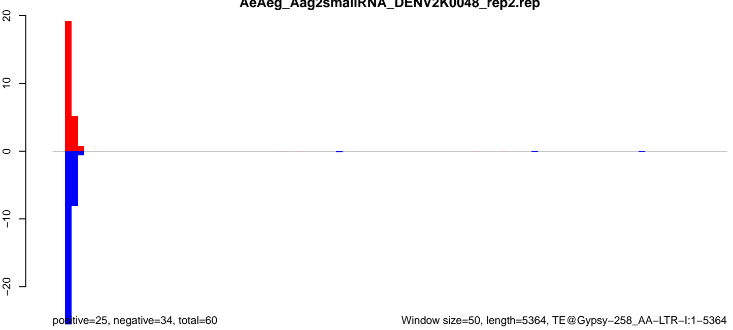
AeAeg_Aag2smallRNA_DENV2K0048_rep2.rep
