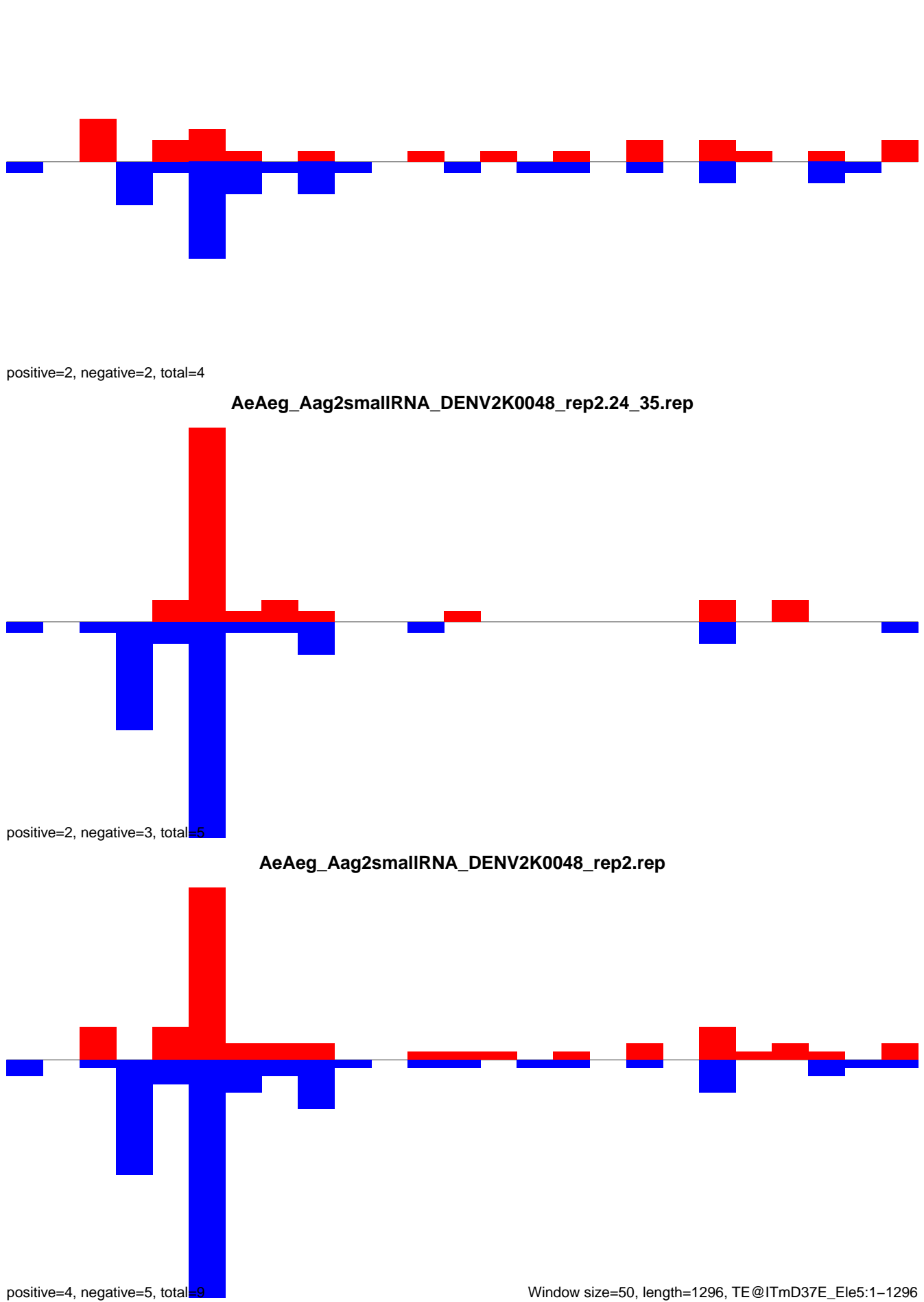
AeAeg_Aag2smallRNA_DENV2K0048_rep2.18_23.rep
