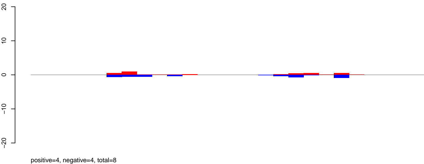
AeAeg_Aag2smallIRNA_DENV2K0048_rep2.rep
