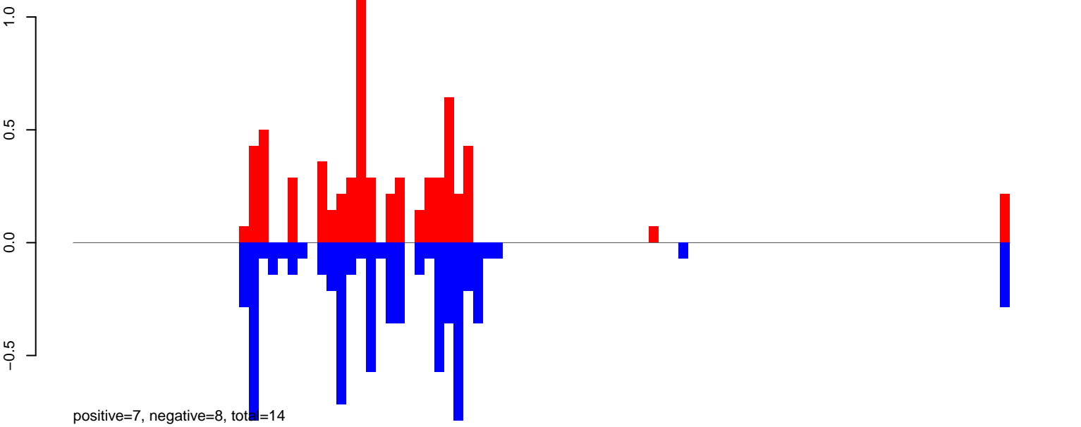
AeAeg_Aag2smallRNA_DENV2K0048_rep2.24_35.rep
