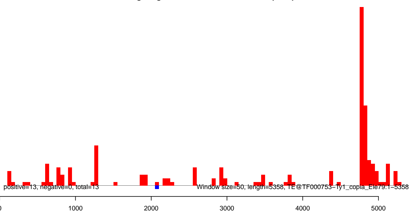
AeAeg_Aag2smallRNA_DENV2K0048_rep2.rep
