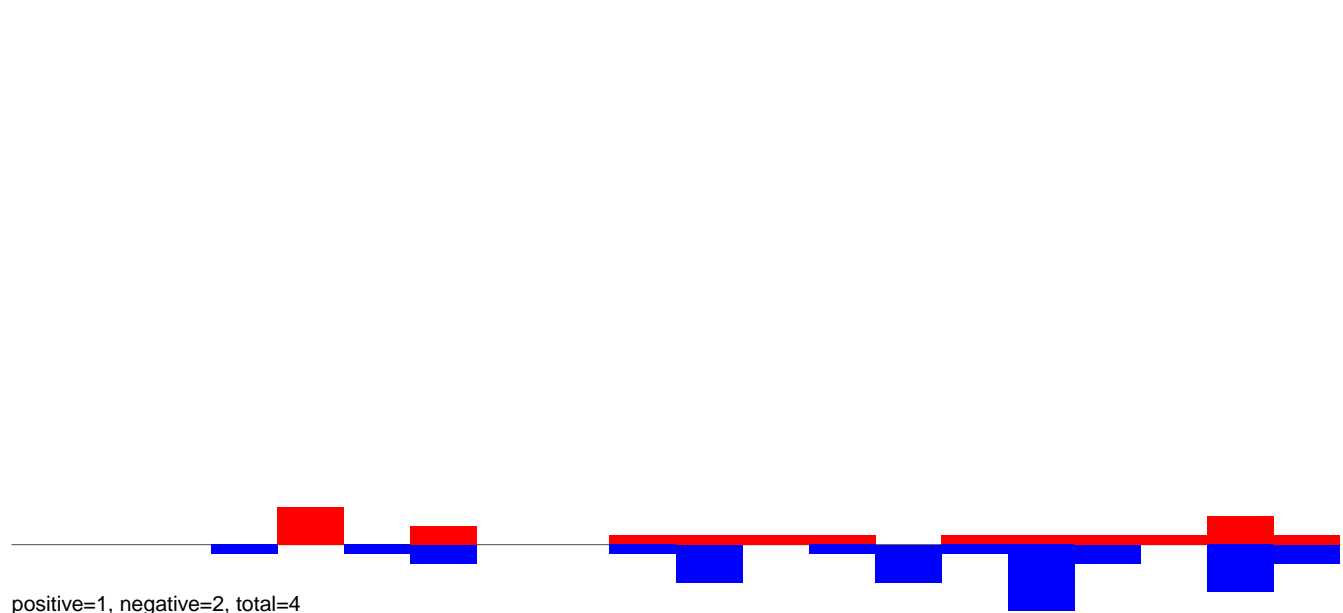
AeAeg_Aag2smallRNA_DENV2K0048_rep2.24_35.rep
