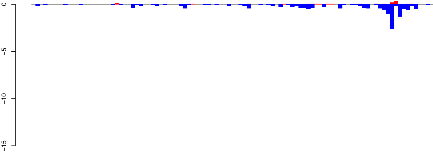
AeAeg_Aag2smallRNA_DENV2K0048_rep2.18_23.rep
