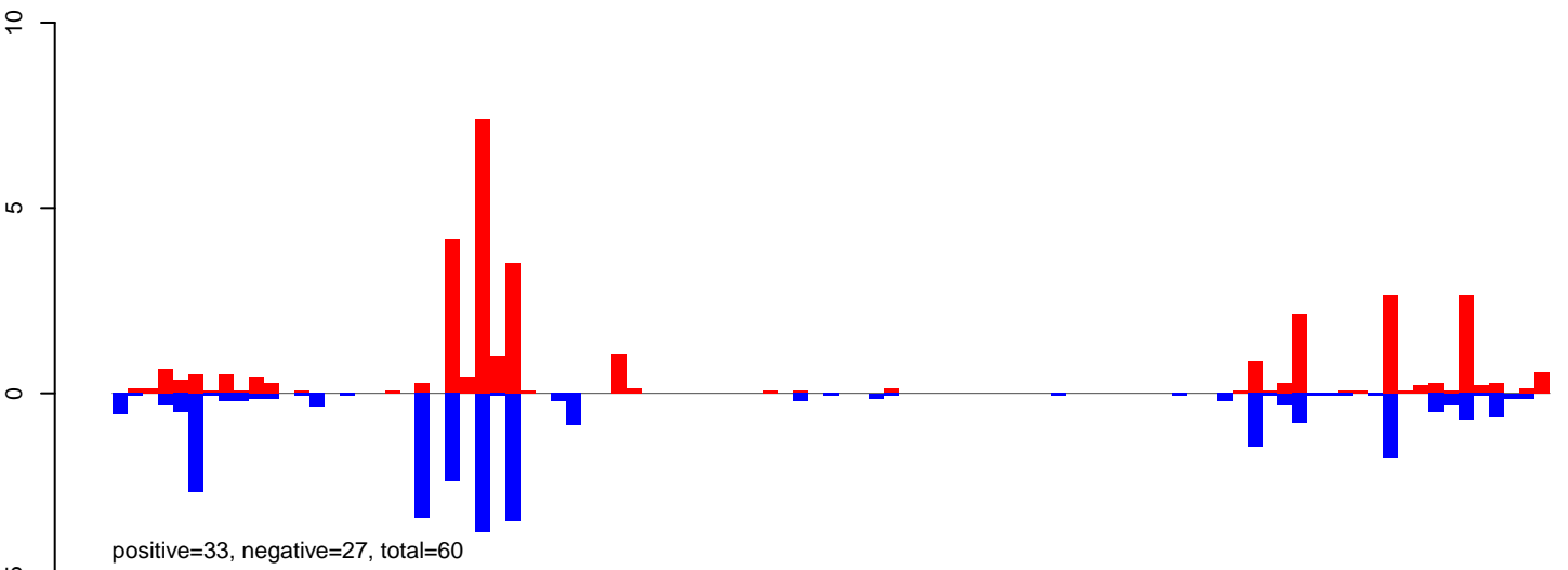
AeAeg_Aag2smallRNA_DENV2K0048_rep2.24_35.rep
