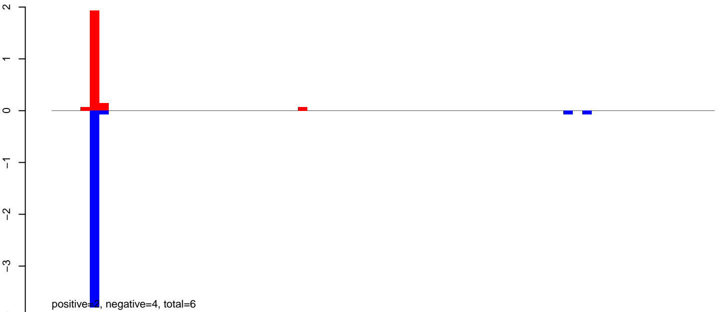
AeAeg_Aag2smallRNA_DENV2K0048_rep2.24_35.rep
