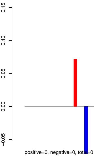
AeAeg_Aag2smallRNA_DENV2K0048_rep2.18_23.rep
