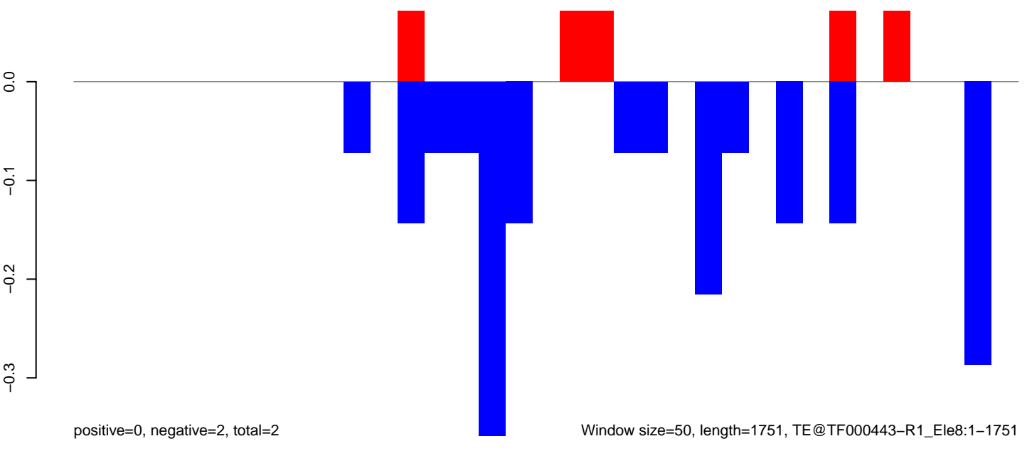
AeAeg_Aag2smallRNA_DENV2K0048_rep2.rep
