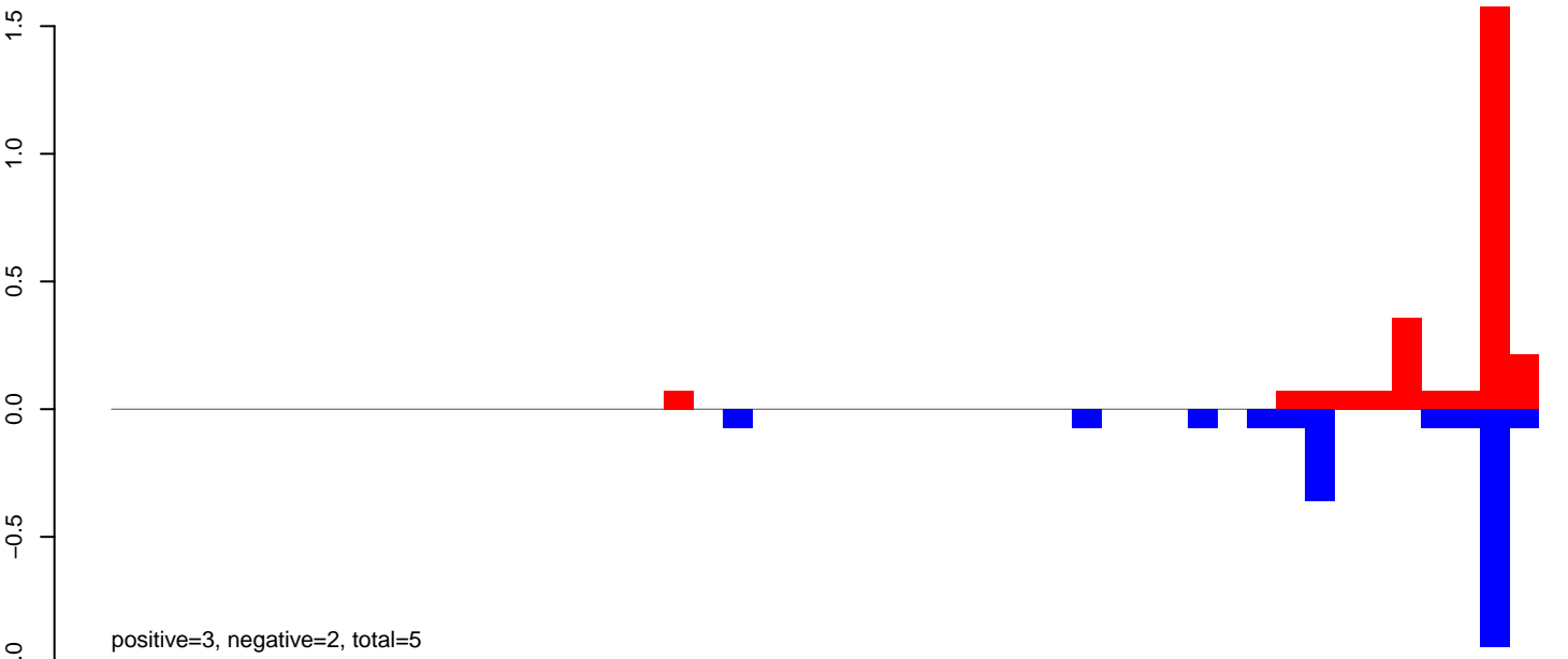
AeAeg_Aag2smallRNA_DENV2K0048_rep2.24_35.rep
