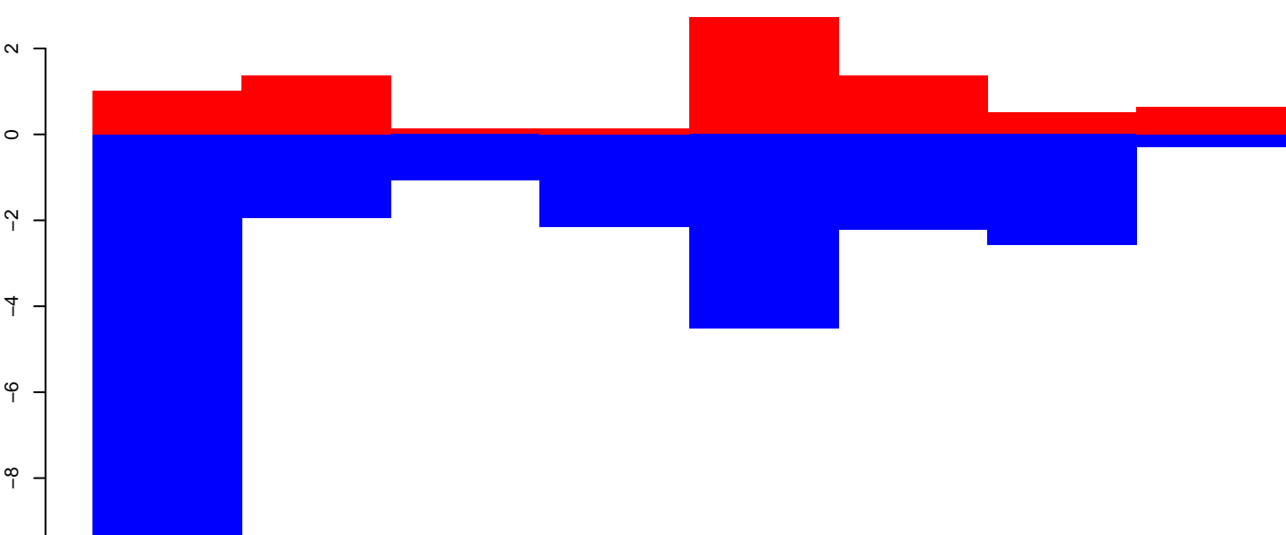
AeAeg_Aag2smallRNA_DENV2K0048_rep2.rep
