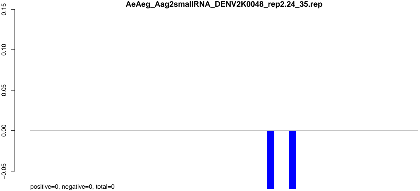
AeAeg_Aag2smallRNA_DENV2K0048_rep2.rep
