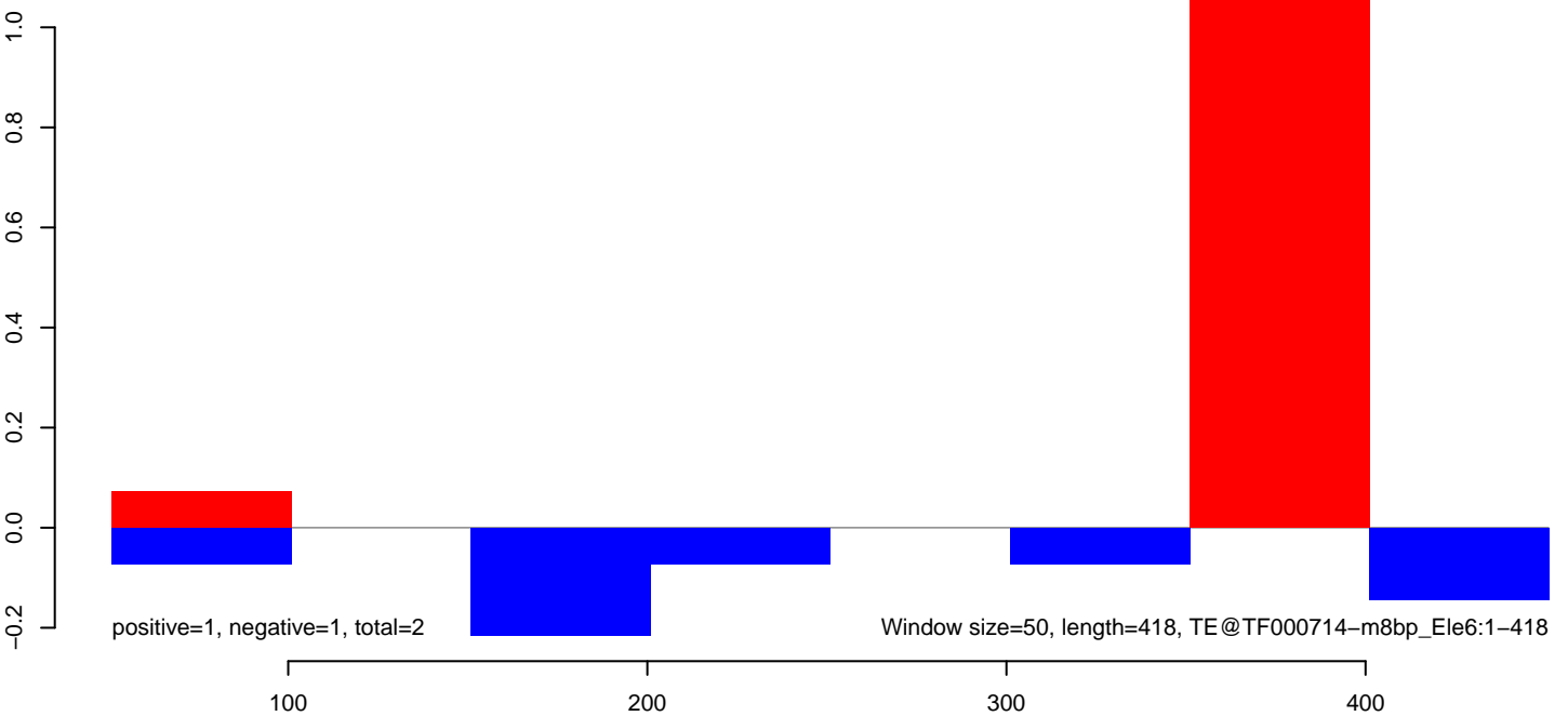
AeAeg_Aag2smallRNA_DENV2K0048_rep2.rep
