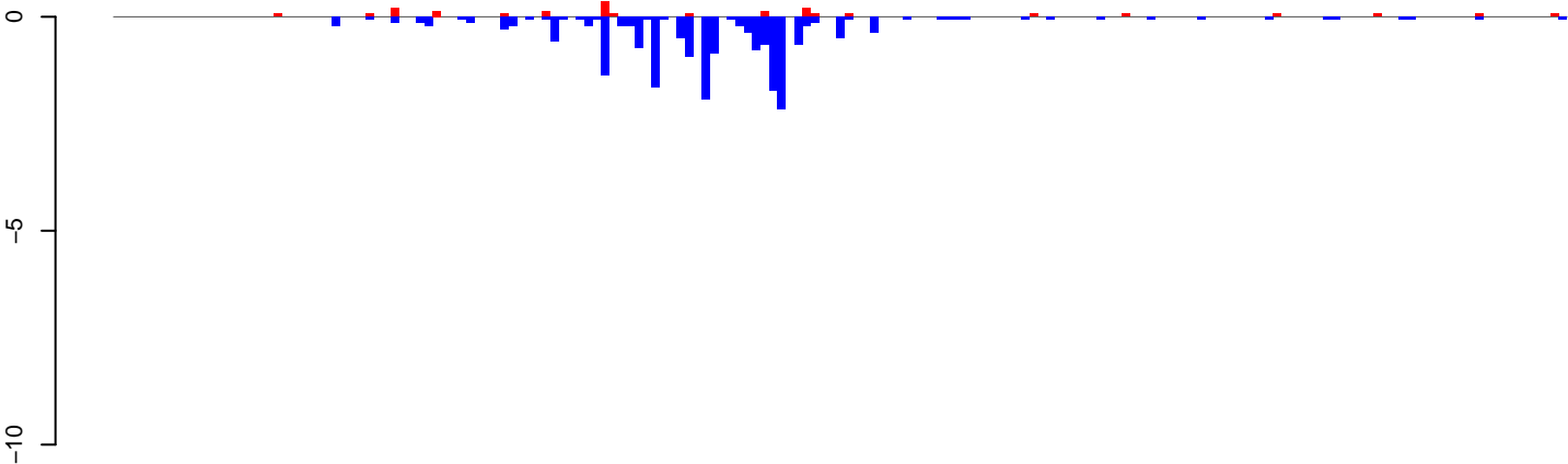
AeAeg_Aag2smallRNA_DENV2K0048_rep2.18_23.rep
