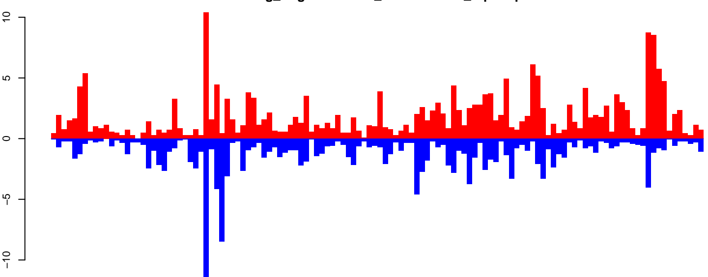
AeAeg_Aag2smallRNA_DENV2K0048_rep2.rep
