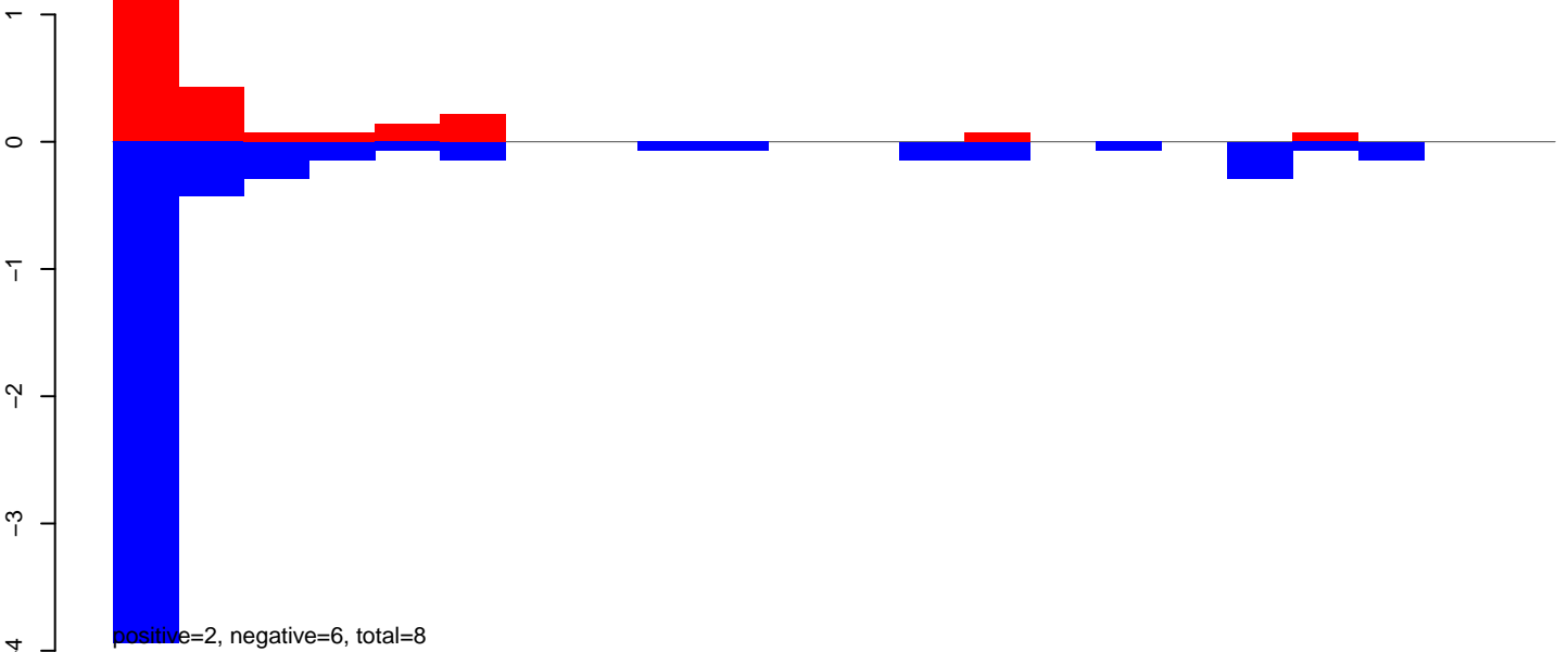
AeAeg_Aag2smallIRNA_DENV2K0048_rep2.rep
