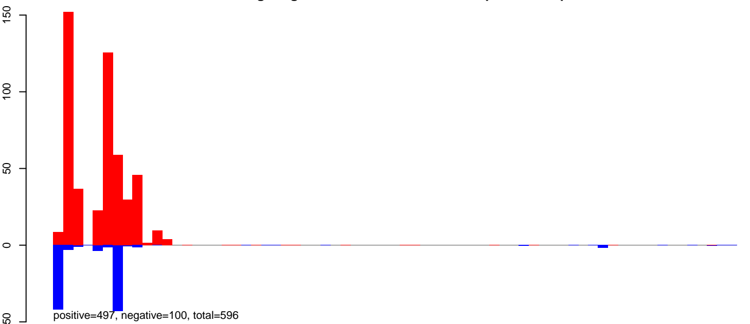
AeAeg_Aag2smallRNA_DENV2K0048_rep2.rep
