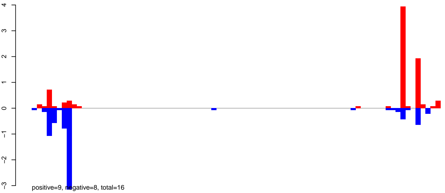
AeAeg_Aag2smallIRNA_DENV2K0048_rep2.24_35.rep
