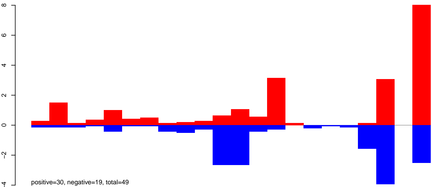
AeAeg_Aag2smallIRNA_DENV2K0048_rep2.24_35.rep
