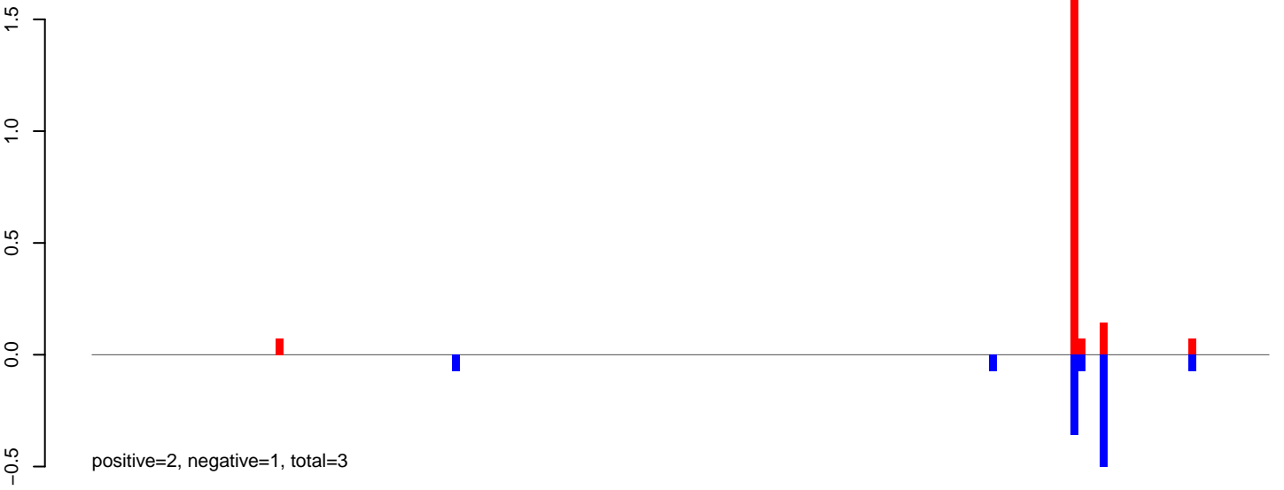
AeAeg_Aag2smallRNA_DENV2K0048_rep2.24_35.rep
