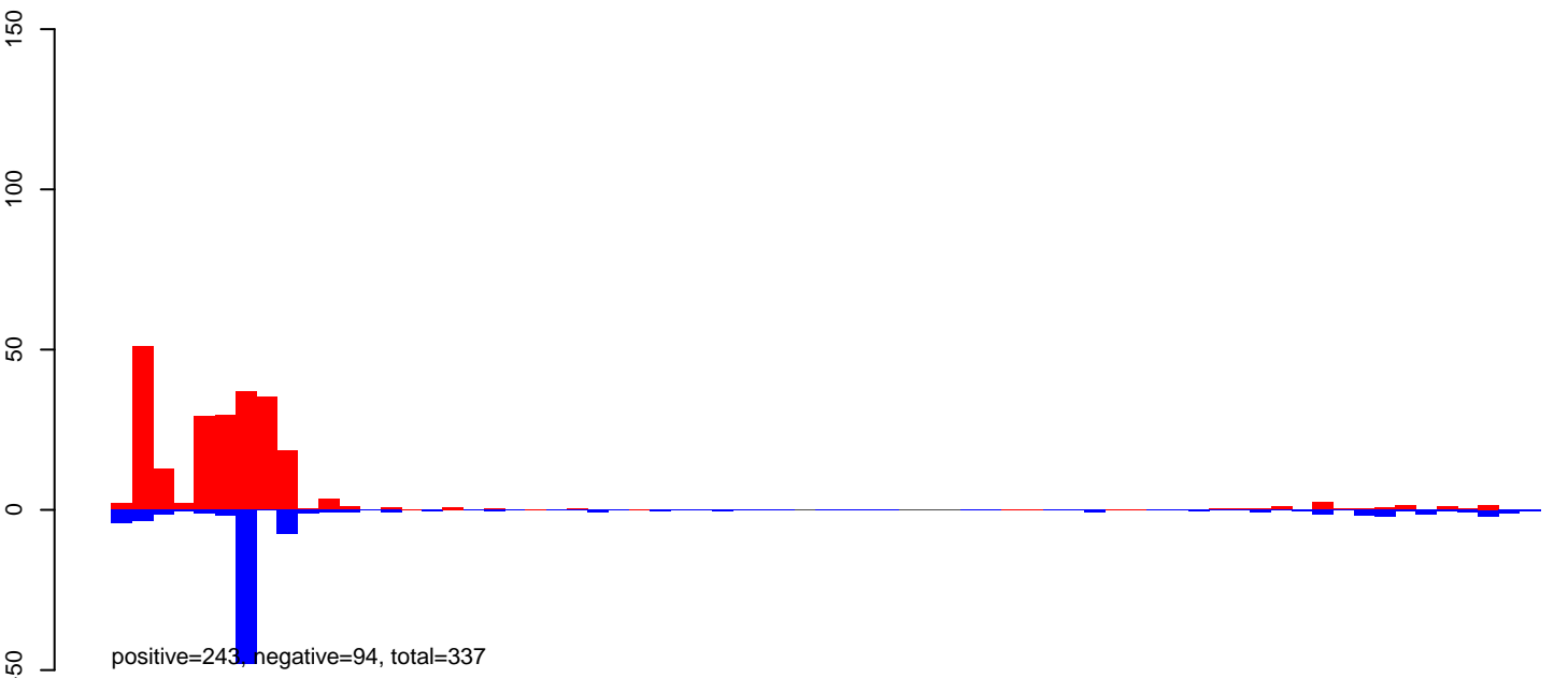
AeAeg_Aag2smallRNA_DENV2K0048_rep2.24_35.rep
