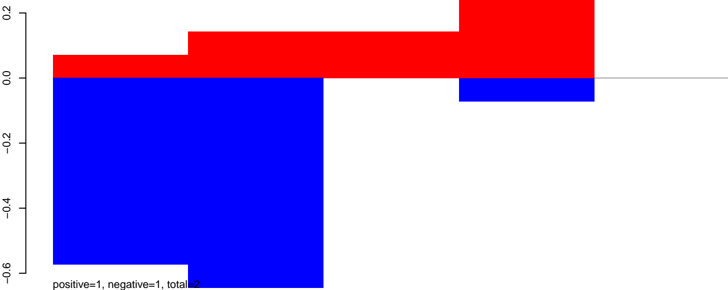
AeAeg_Aag2smallIRNA_DENV2K0048_rep2.24_35.rep
