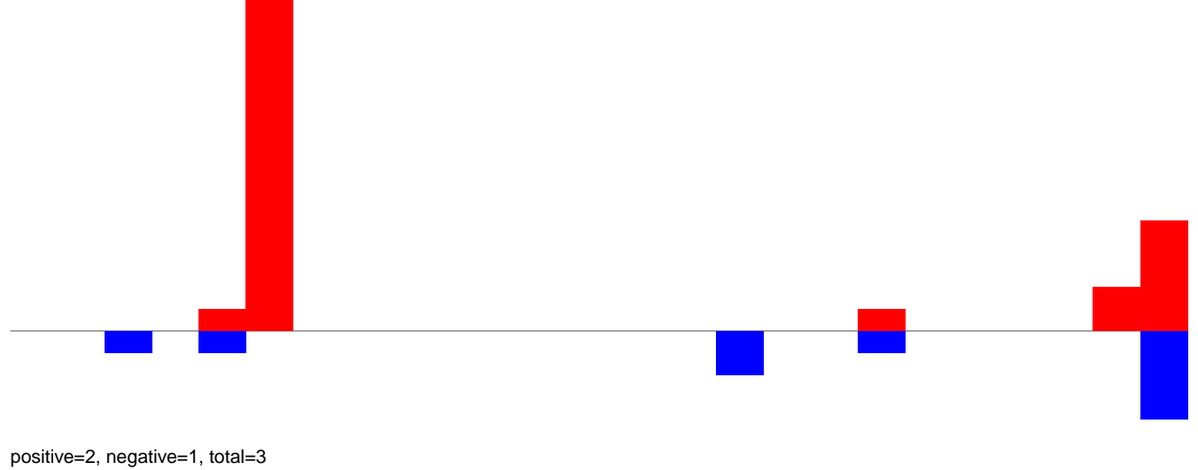
AeAeg_Aag2smallRNA_DENV2K0048_rep2.rep
