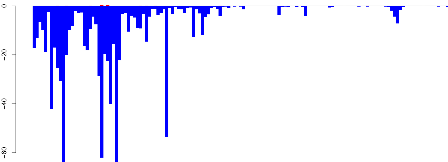
AeAeg_Aag2smallRNA_DENV2K0048_rep2.rep
