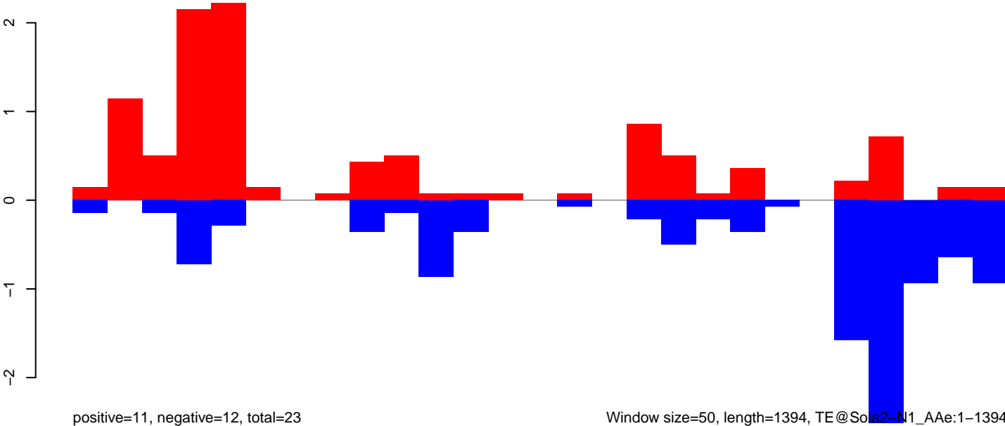
AeAeg_Aag2smallIRNA_DENV2K0048_rep2.rep
