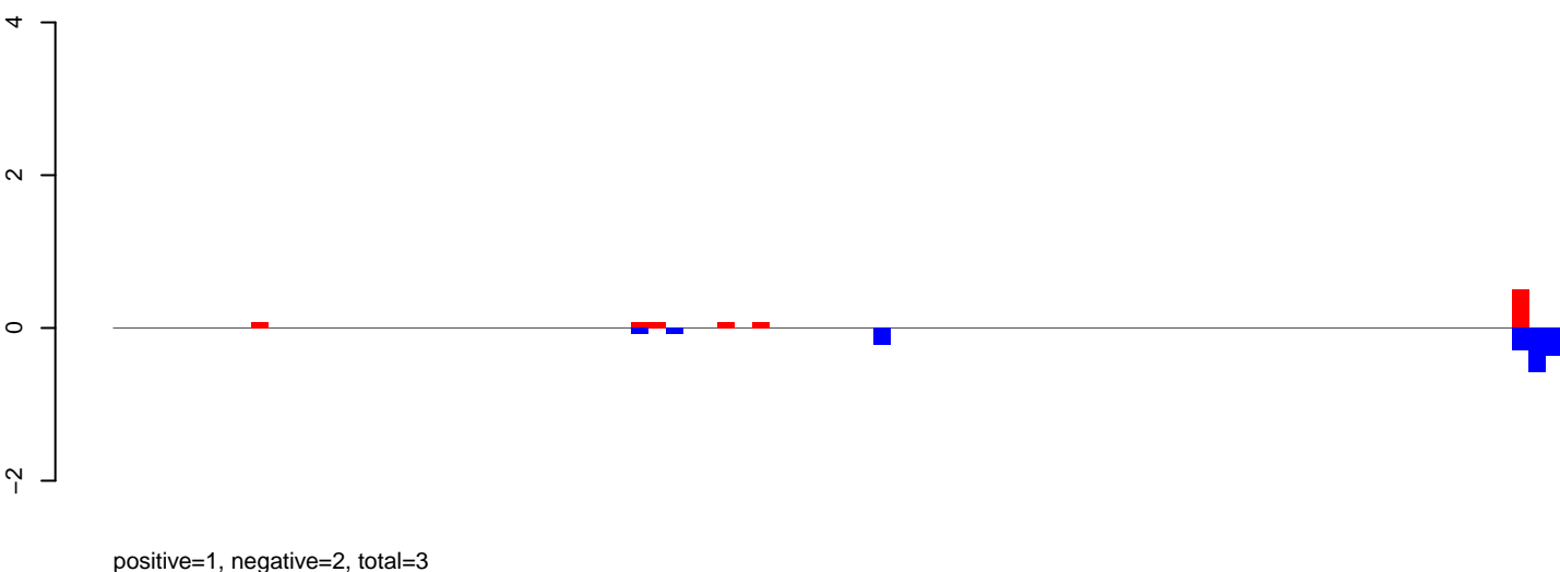
AeAeg_Aag2smallRNA_DENV2K0048_rep2.rep
