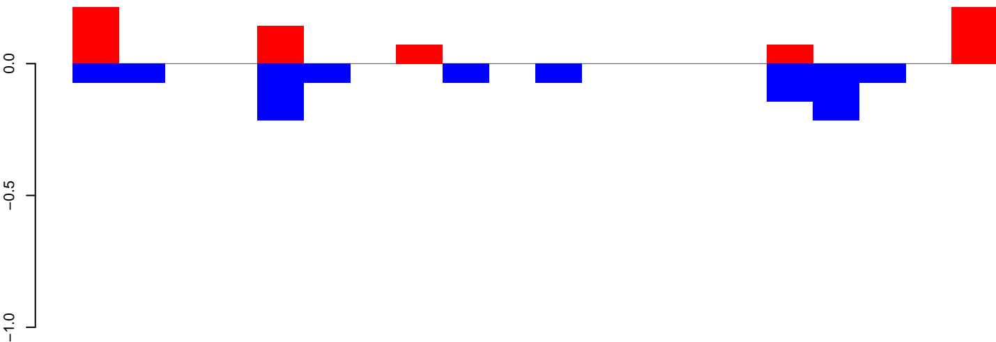
AeAeg_Aag2smallRNA_DENV2K0048_rep2.18_23.rep
