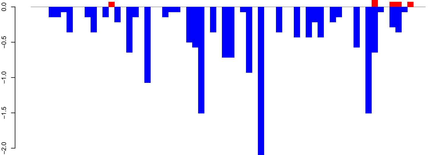
AeAeg_Aag2smallRNA_DENV2K0048_rep2.24_35.rep
