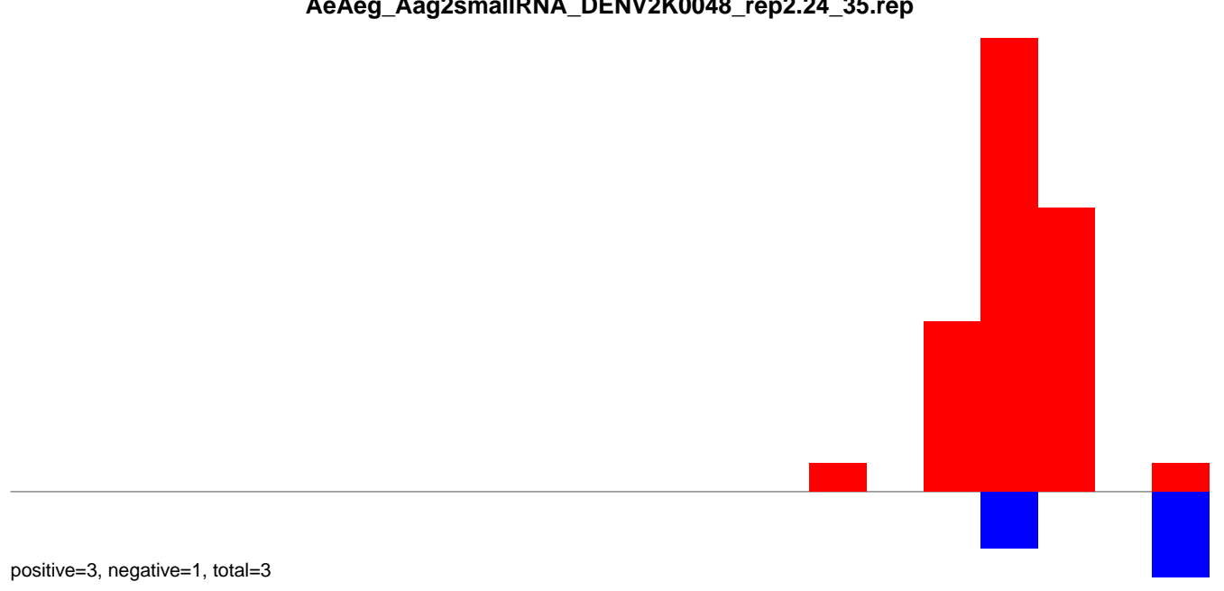
AeAeg_Aag2smallRNA_DENV2K0048_rep2.rep
