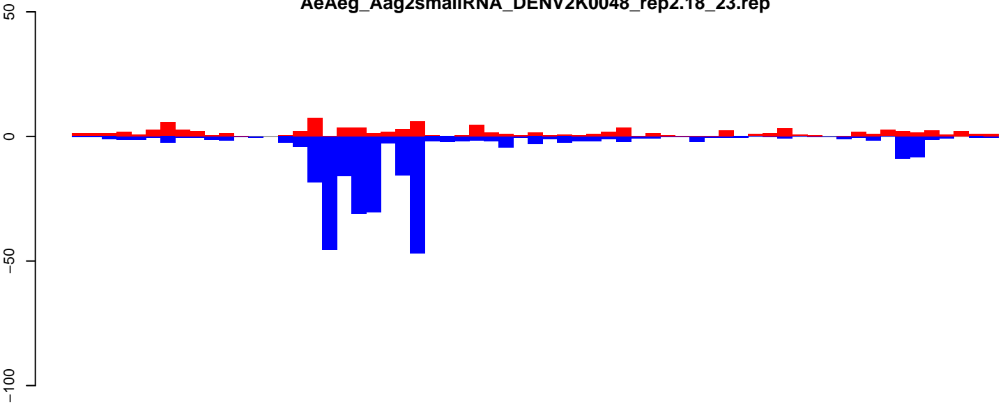
AeAeg_Aag2smallRNA_DENV2K0048_rep2.18_23.rep
