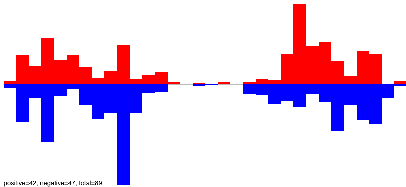
AeAeg_Aag2smallIRNA_DENV2K0048_rep2.24_35.rep
