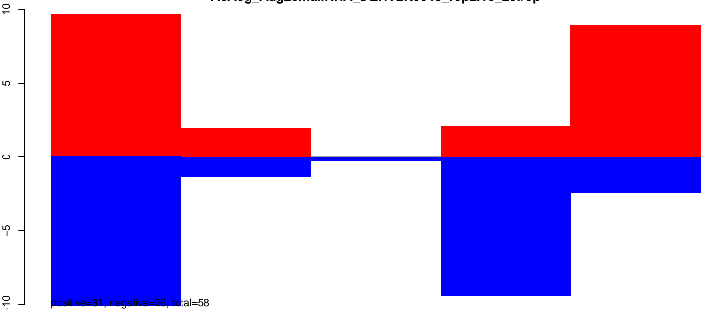
AeAeg_Aag2smallRNA_DENV2K0048_rep2.24_35.rep
