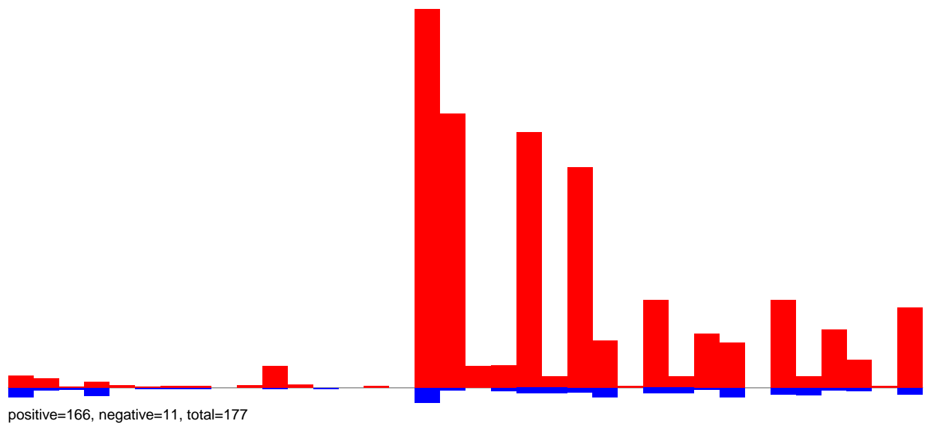
AeAeg_Aag2smallRNA_DENV2K0048_rep2.rep
