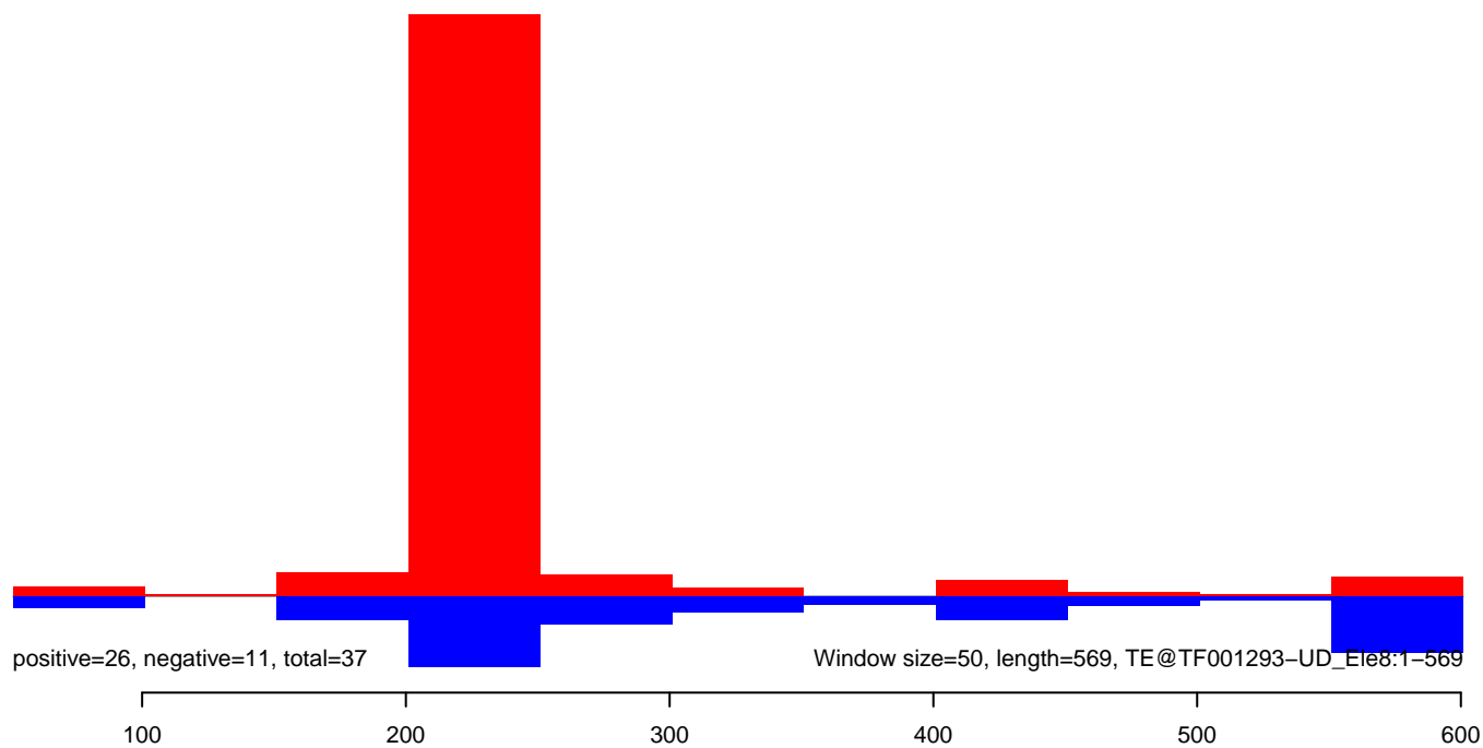
AeAeg_Aag2smallRNA_DENV2K0048_rep2.rep
