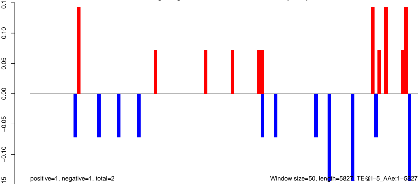
AeAeg_Aag2smallRNA_DENV2K0048_rep2.rep
