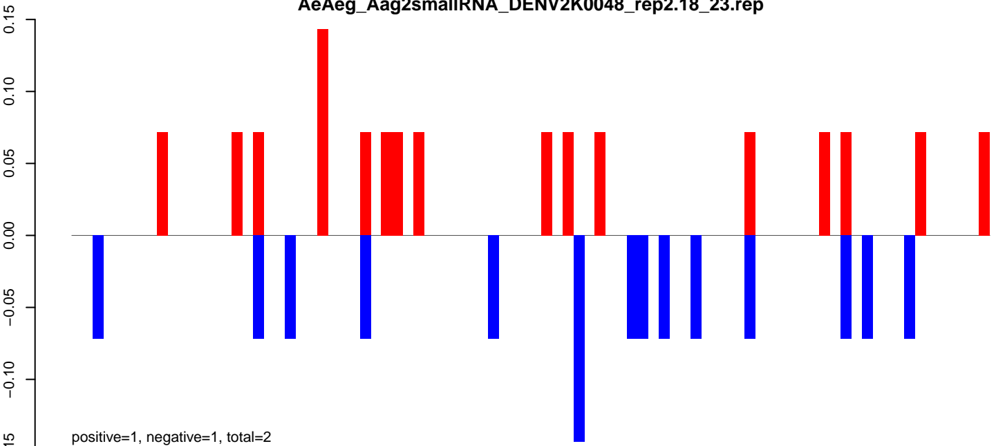
AeAeg_Aag2smallIRNA_DENV2K0048_rep2.24_35.rep
