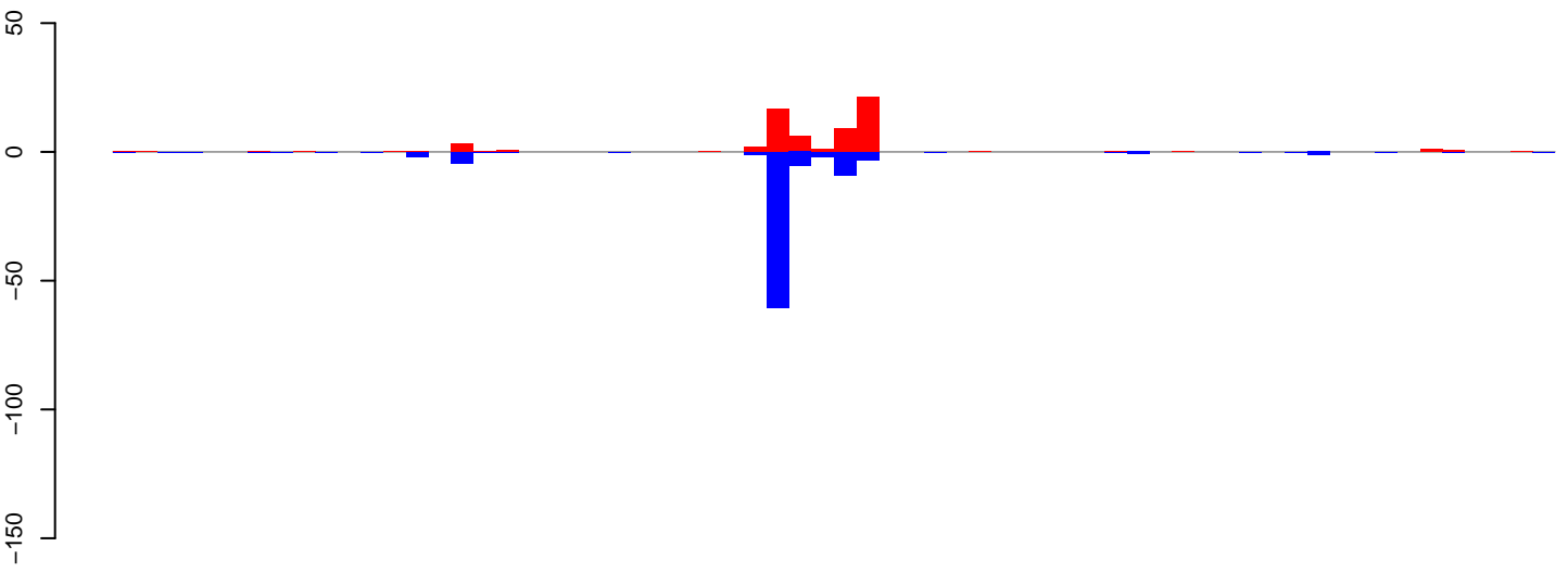
AeAeg_Aag2smallRNA_DENV2K0048_rep2.24_35.rep
