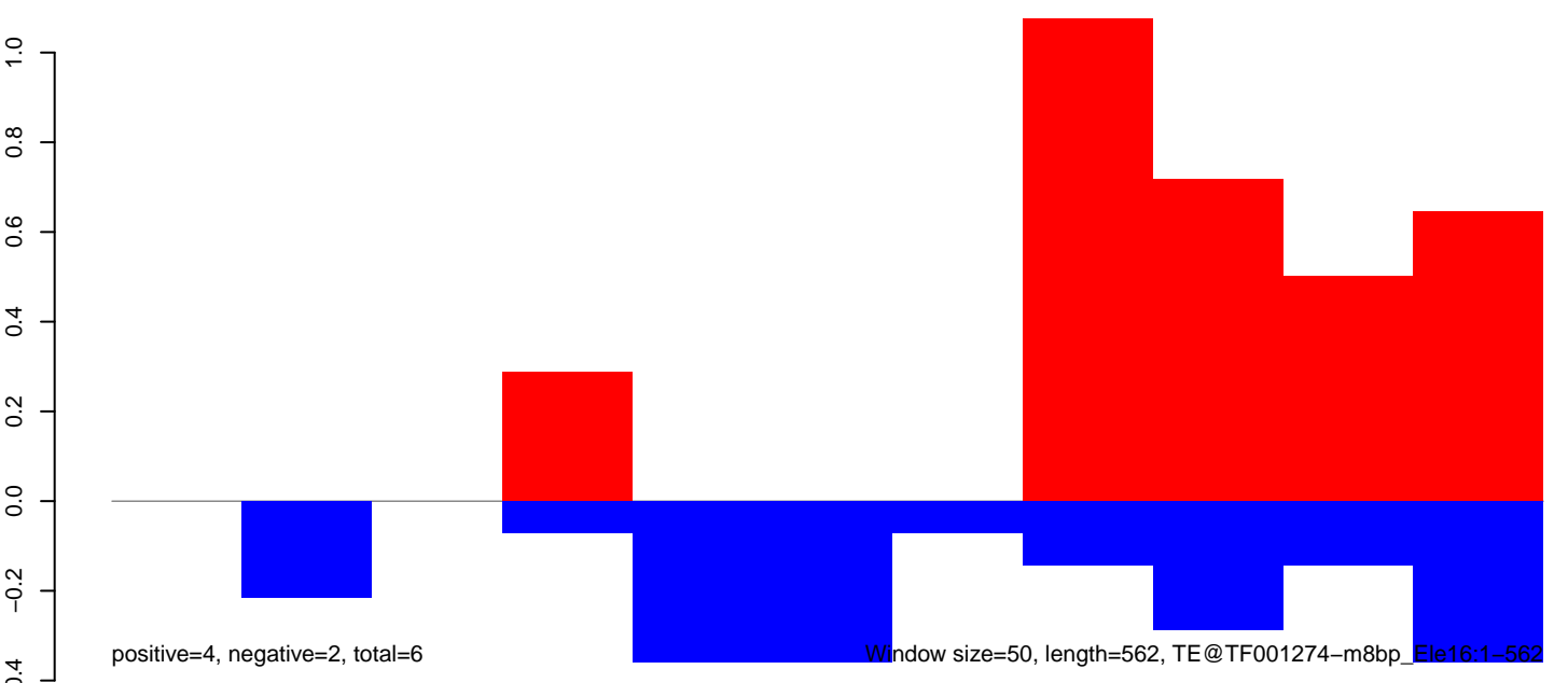
AeAeg_Aag2smallRNA_DENV2K0048_rep2.rep
