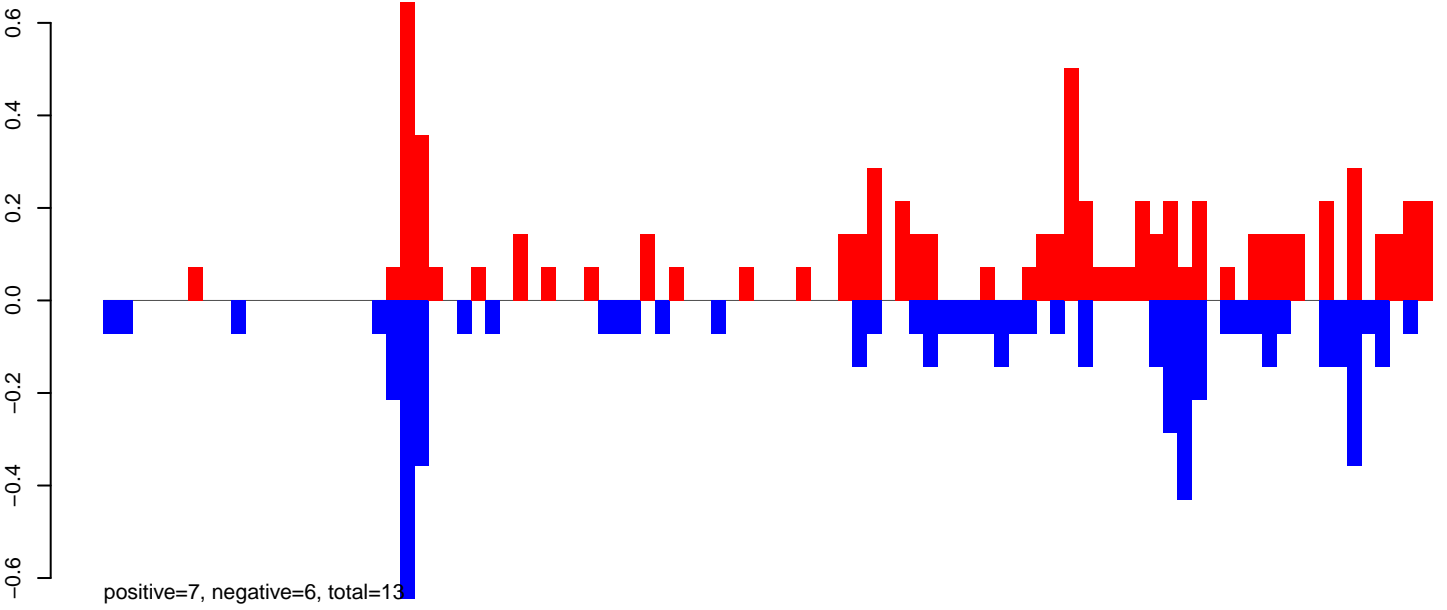
AeAeg_Aag2smallRNA_DENV2K0048_rep2.24_35.rep
