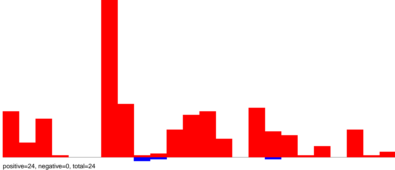
AeAeg_Aag2smallRNA_DENV2K0048_rep2.rep
