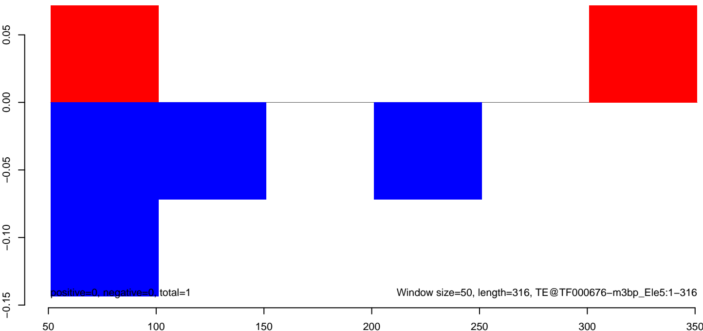
AeAeg_Aag2smallRNA_DENV2K0048_rep2.rep
