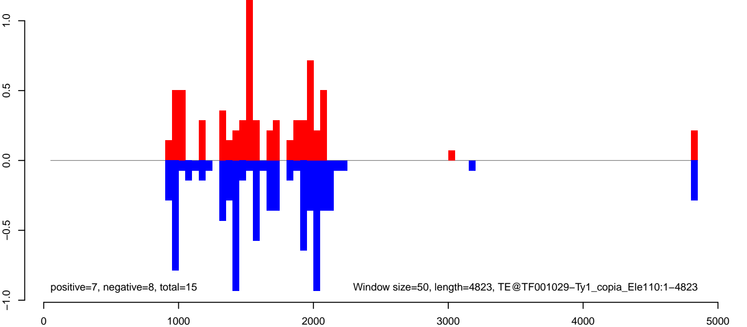
AeAeg_Aag2smallRNA_DENV2K0048_rep2.rep
