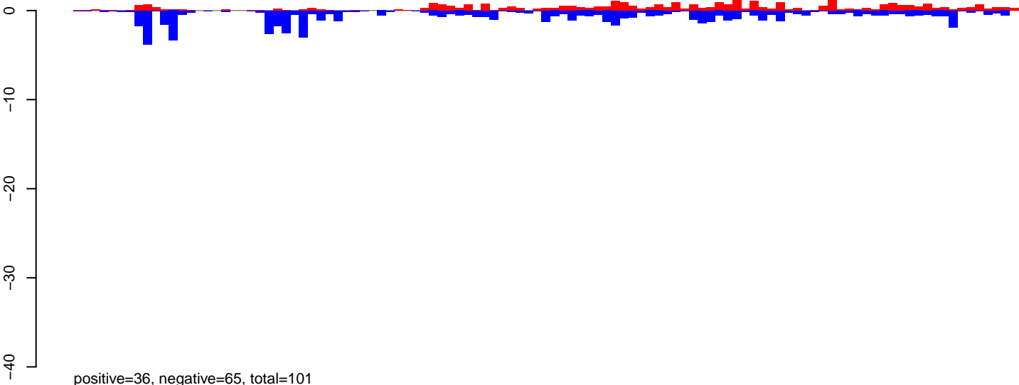
AeAeg_Aag2smallRNA_DENV2K0048_rep2.24_35.rep
