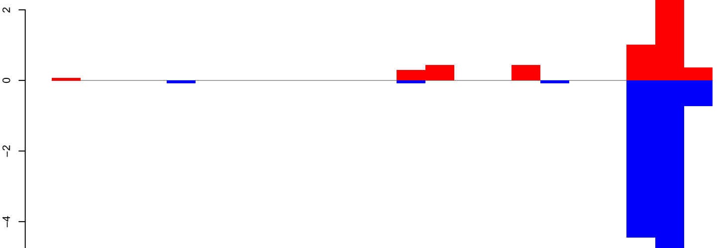
AeAeg_Aag2smallRNA_DENV2K0048_rep2.rep
