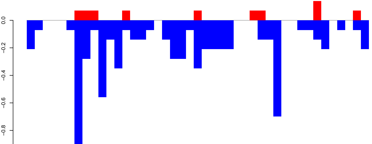
AeAeg_Aag2smallRNA_DENV2NGC_rep2.rep
