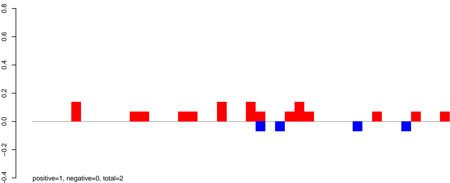
AeAeg_Aag2smallRNA_DENV2NGC_rep2.rep
