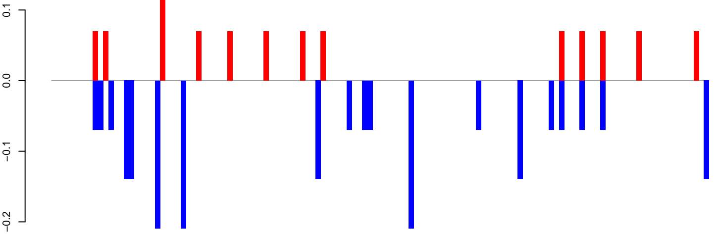
AeAeg_Aag2smallRNA_DENV2NGC_rep2.18_23.rep
