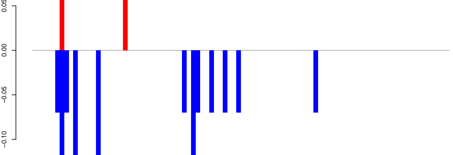
AeAeg_Aag2smallRNA_DENV2NGC_rep2.rep
