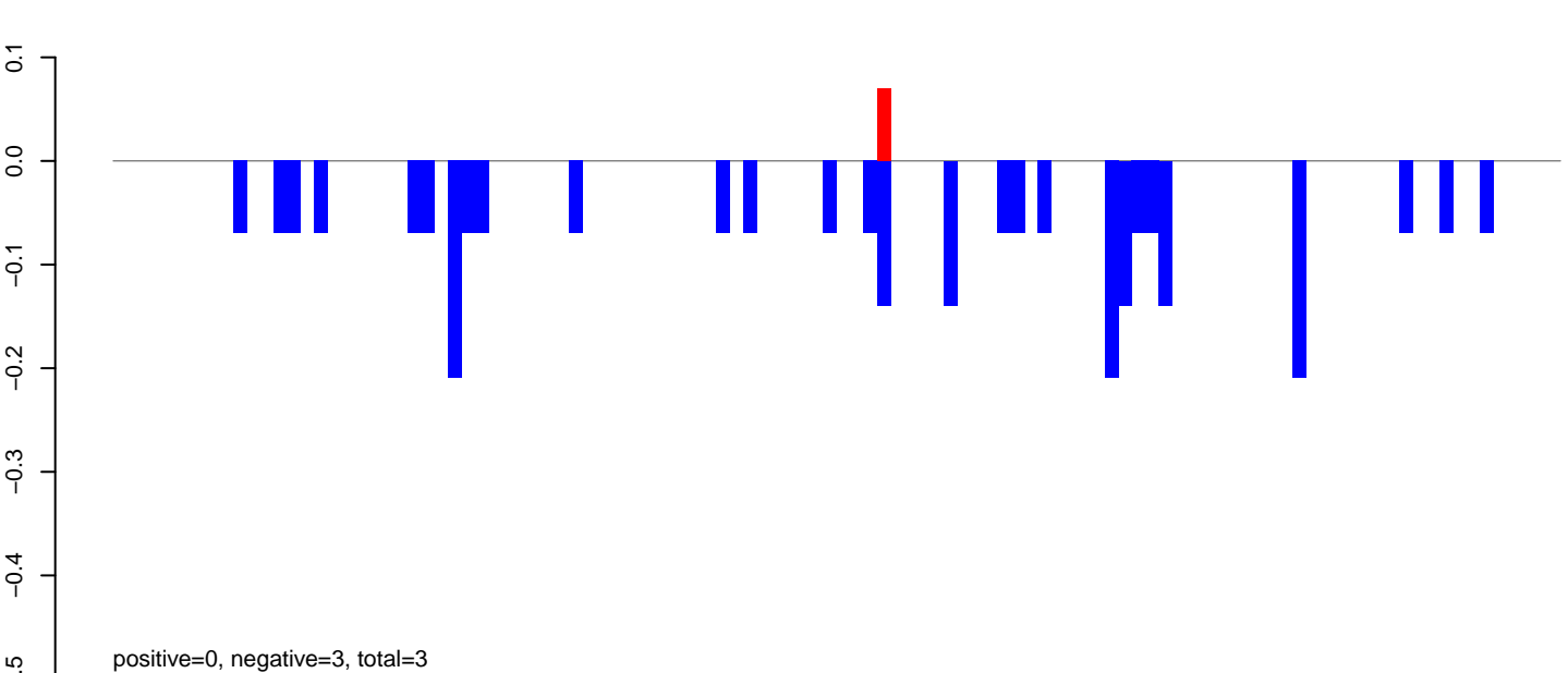
AeAeg_Aag2smallRNA_DENV2NGC_rep2.rep
