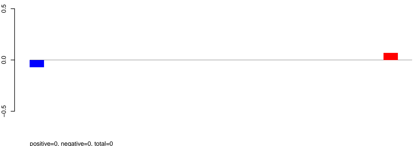
AeAeg_Aag2smallRNA_DENV2NGC_rep2.rep
