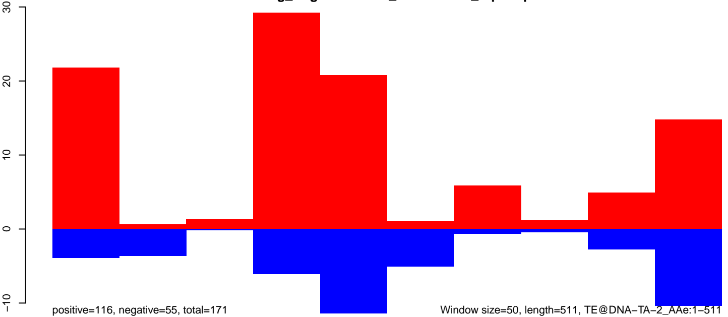
AeAeg_Aag2smallRNA_DENV2NGC_rep2.rep
