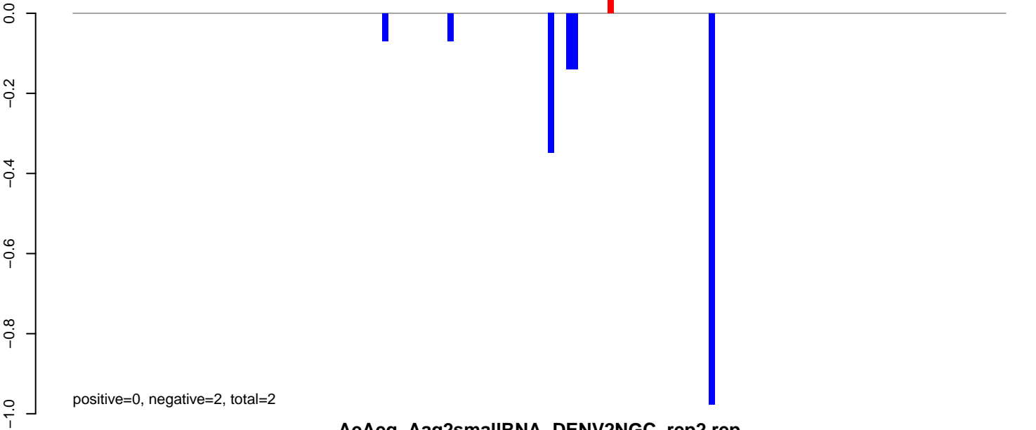
AeAeg_Aag2smallRNA_DENV2NGC_rep2.rep
