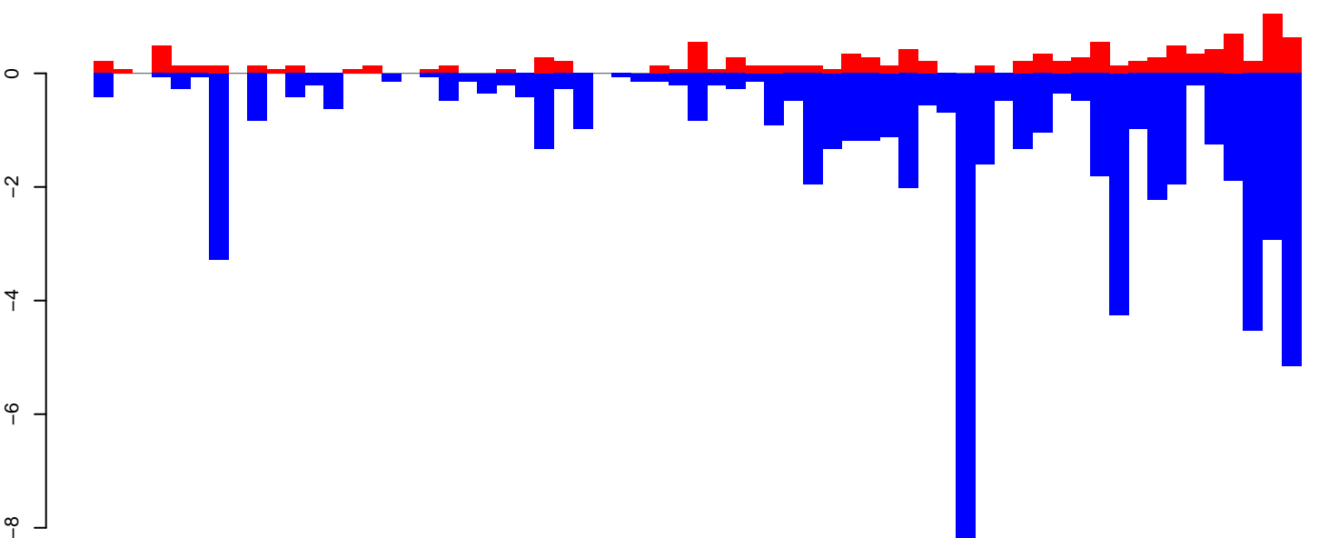
AeAeg_Aag2smallRNA_DENV2NGC_rep2.rep
