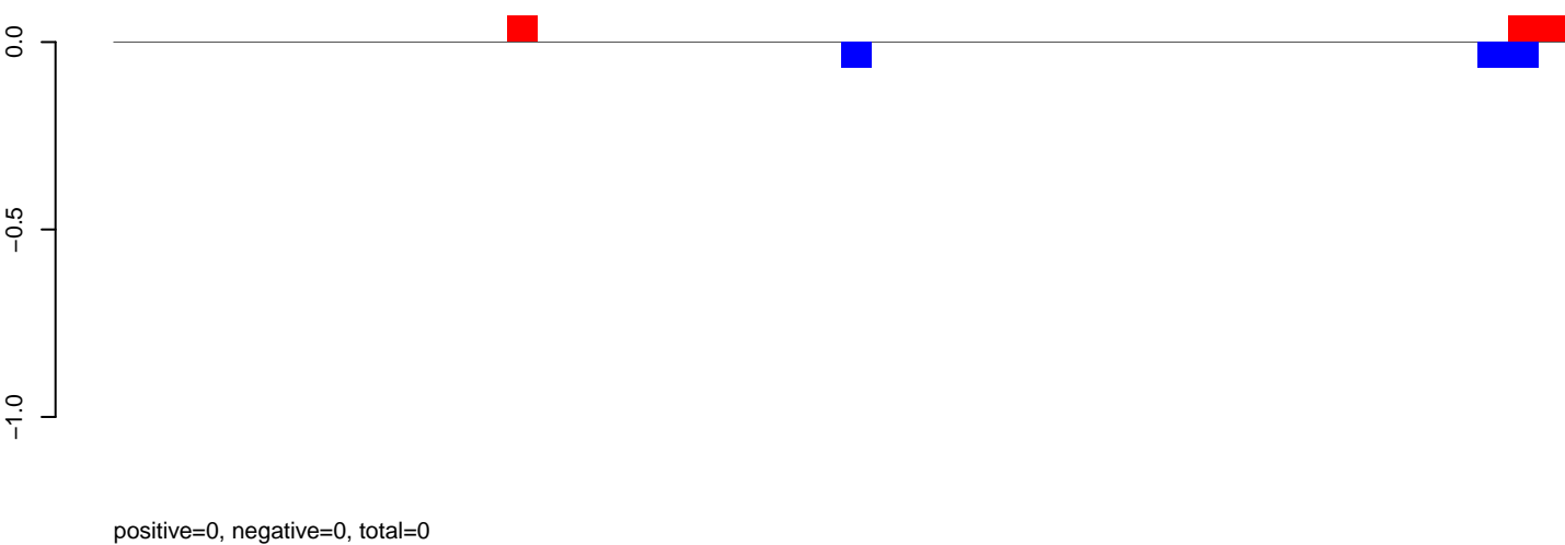
AeAeg_Aag2smallRNA_DENV2NGC_rep2.rep
