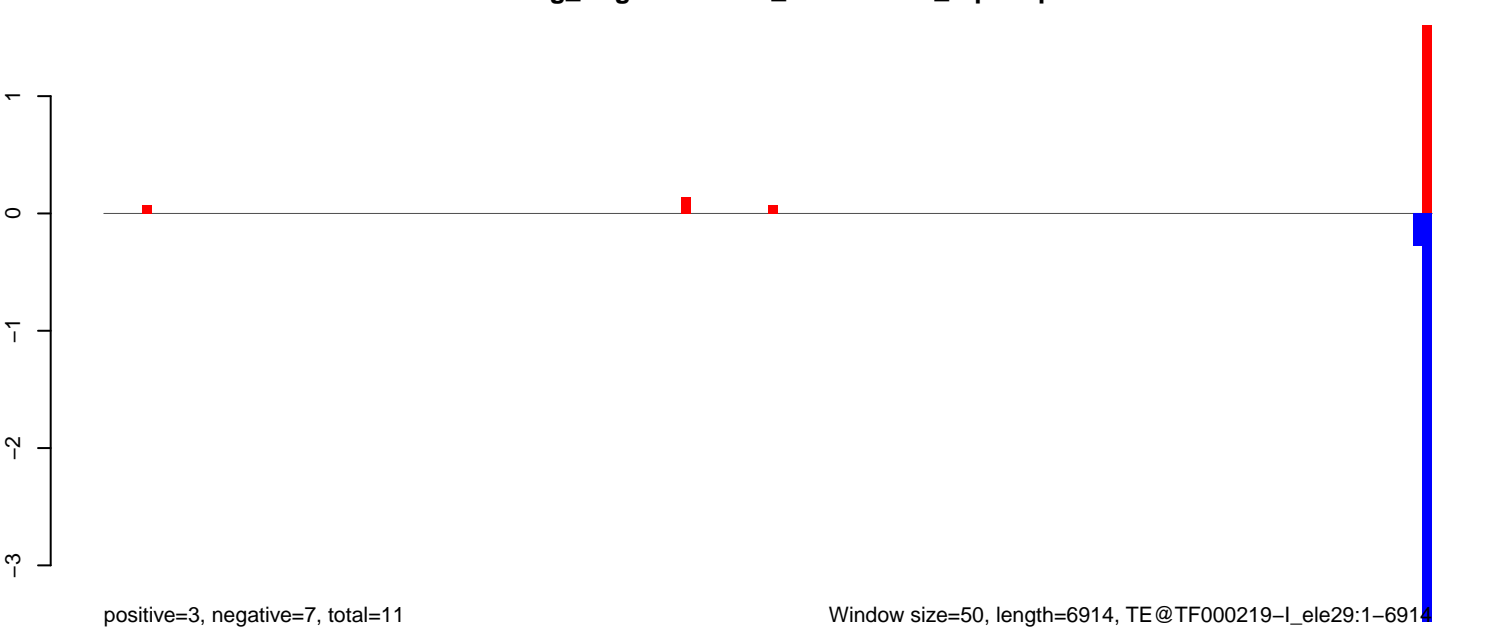
AeAeg_Aag2smallRNA_DENV2NGC_rep2.rep
