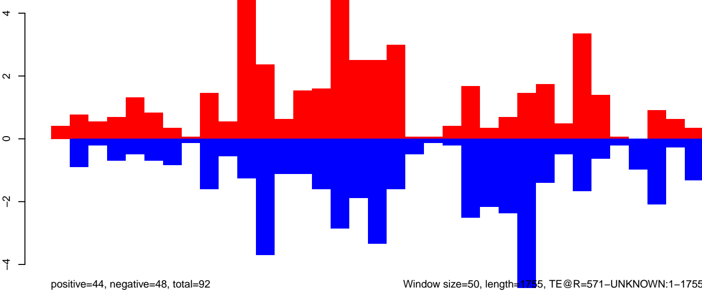
AeAeg_Aag2smallRNA_DENV2NGC_rep2.rep
