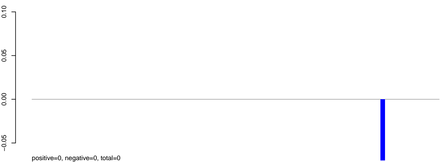
AeAeg_Aag2smallRNA_DENV2NGC_rep2.rep
