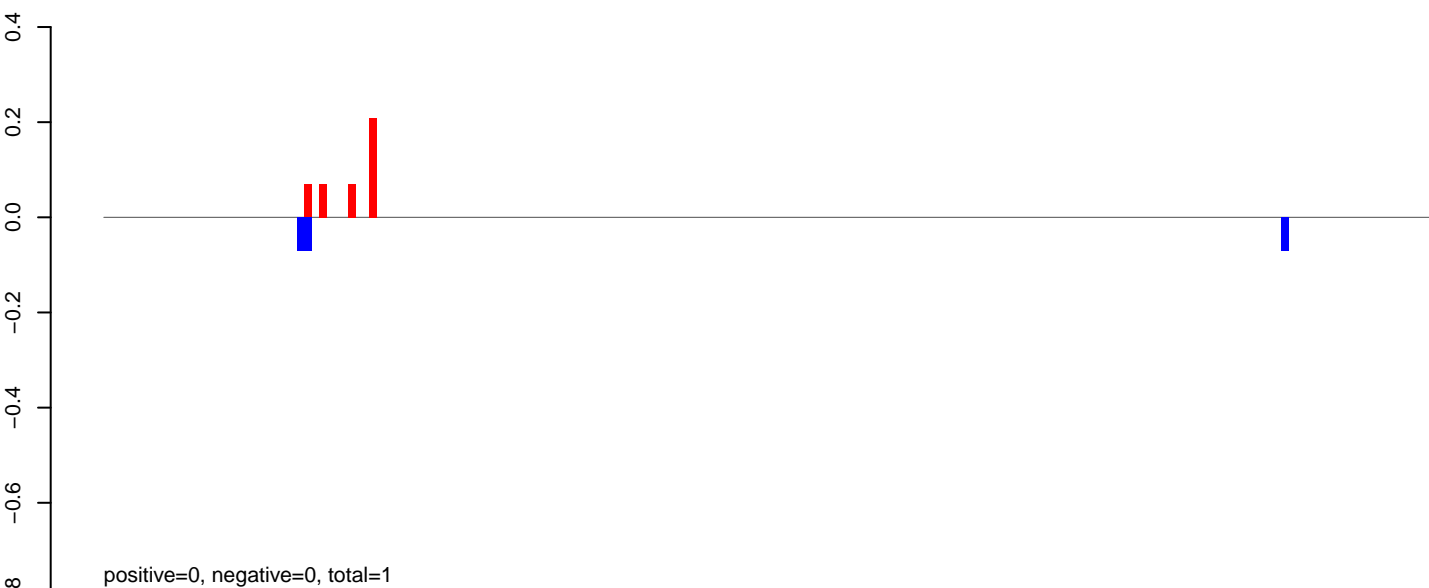
AeAeg_Aag2smallRNA_DENV2NGC_rep2.rep
