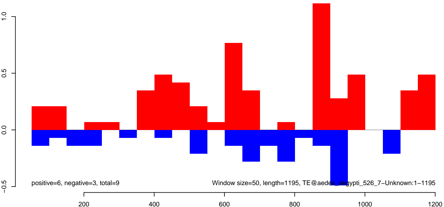
AeAeg_Aag2smallRNA_DENV2NGC_rep2.rep
