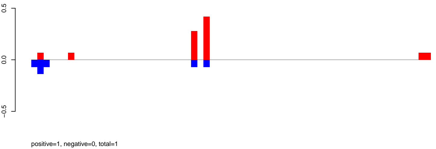
AeAeg_Aag2smallRNA_DENV2NGC_rep2.rep
