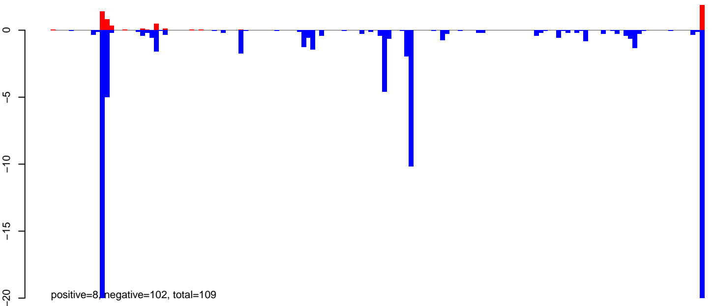
AeAeg_Aag2smallRNA_DENV2NGC_rep2.rep
