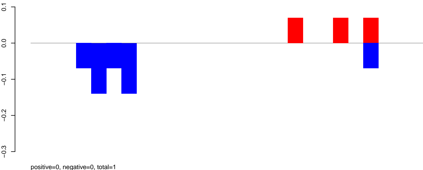
AeAeg_Aag2smallRNA_DENV2NGC_rep2.rep
