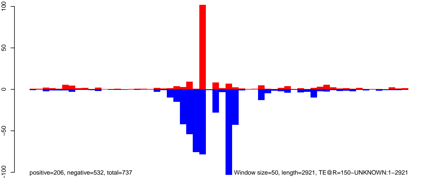
AeAeg_Aag2smallRNA_DENV2NGC_rep2.rep
