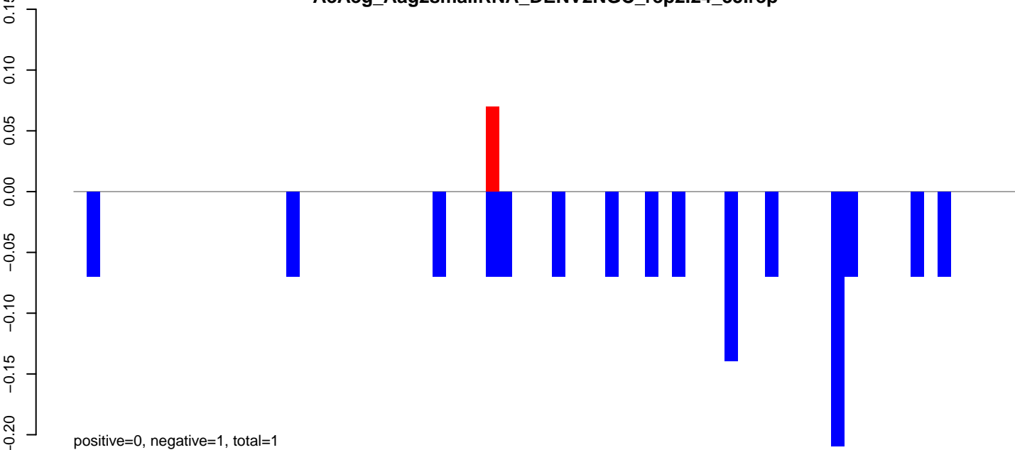
AeAeg_Aag2smallRNA_DENV2NGC_rep2.rep
