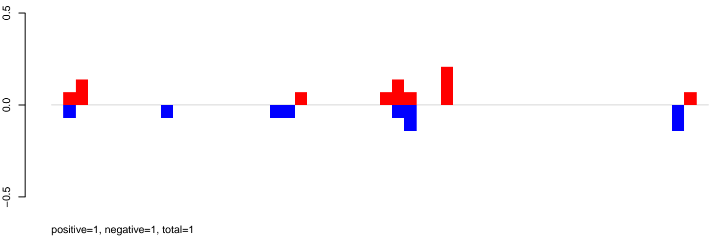
AeAeg_Aag2smallRNA_DENV2NGC_rep2.rep
