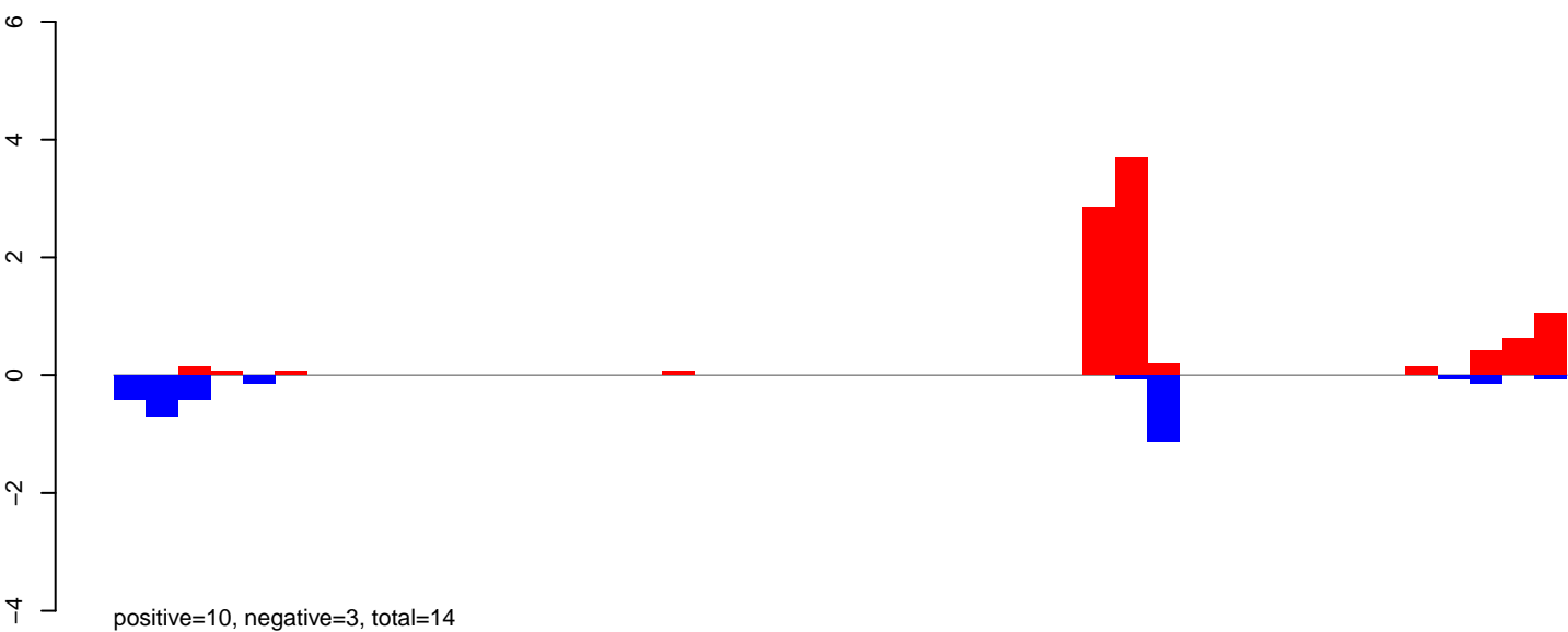
AeAeg_Aag2smallRNA_DENV2NGC_rep2.rep
