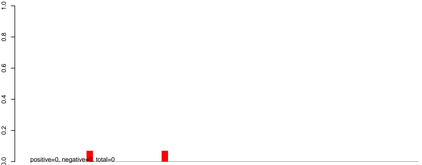
AeAeg_Aag2smallRNA_DENV2NGC_rep2.rep
