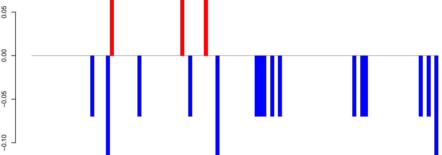
AeAeg_Aag2smallRNA_DENV2NGC_rep2.rep
