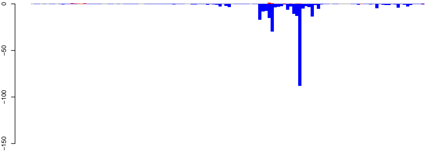
AeAeg_Aag2smallRNA_DENV2NGC_rep2.18_23.rep
