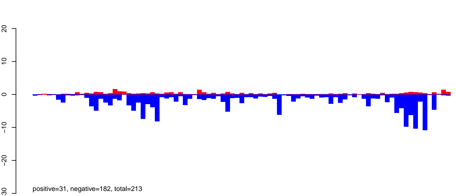
AeAeg_Aag2smallRNA_DENV2NGC_rep2.rep
