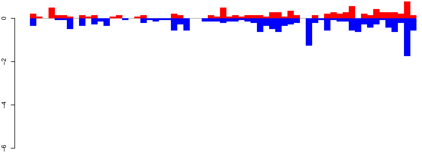
AeAeg_Aag2smallRNA_DENV2NGC_rep2.18_23.rep
