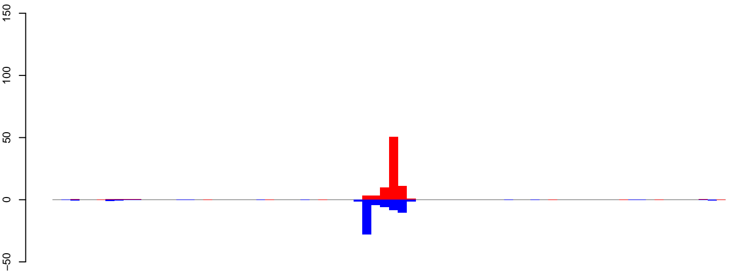
AeAeg_Aag2smallRNA_DENV2NGC_rep2.18_23.rep
