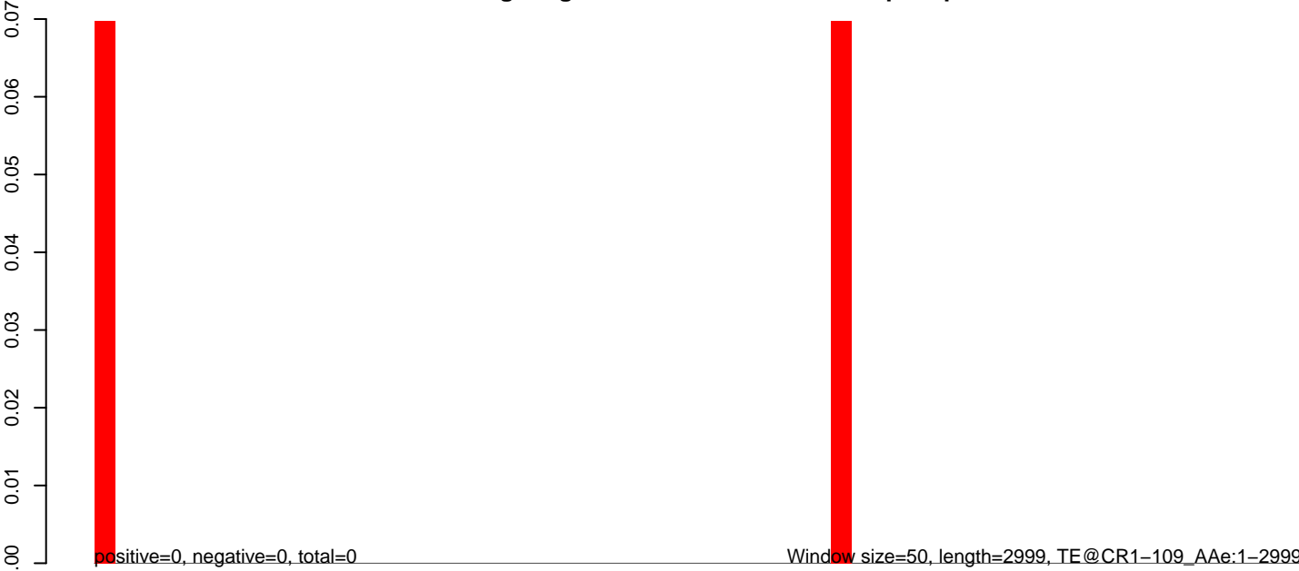
AeAeg_Aag2smallRNA_DENV2NGC_rep2.rep
