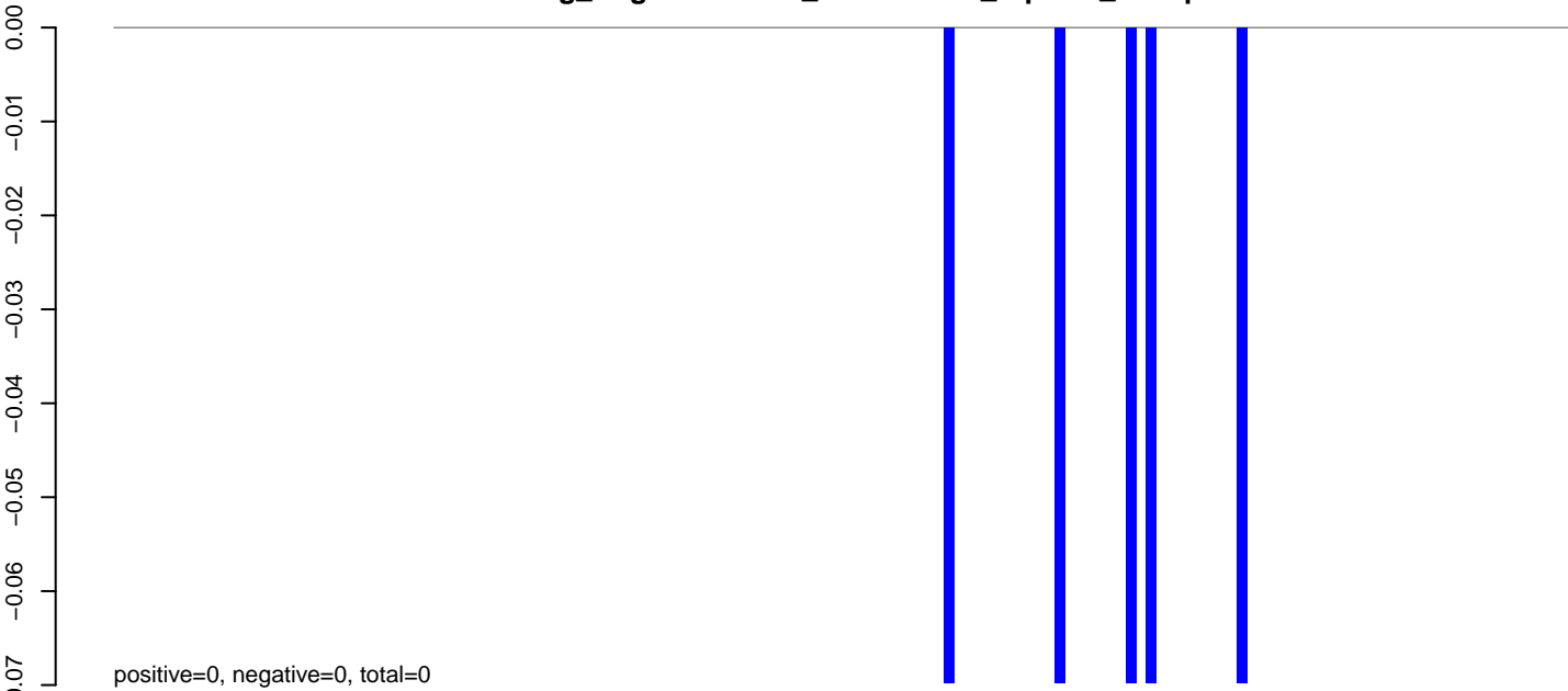
AeAeg_Aag2smallRNA_DENV2NGC_rep2.rep
