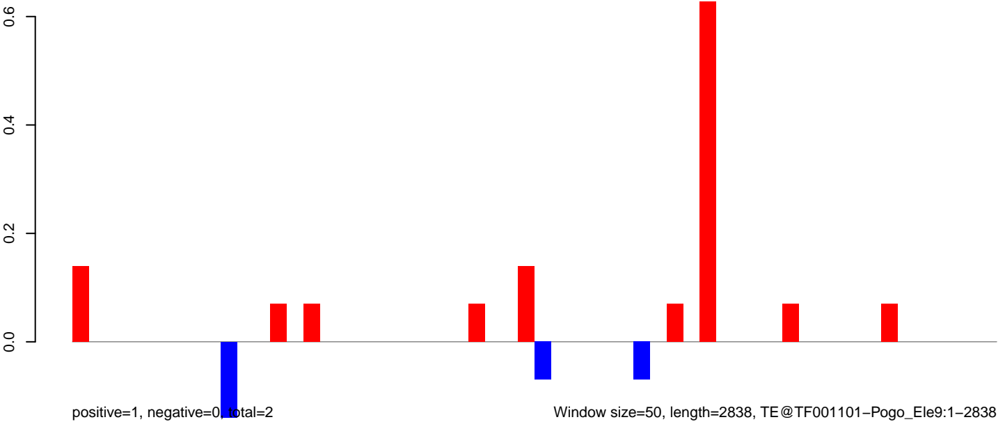
AeAeg_Aag2smallRNA_DENV2NGC_rep2.rep
