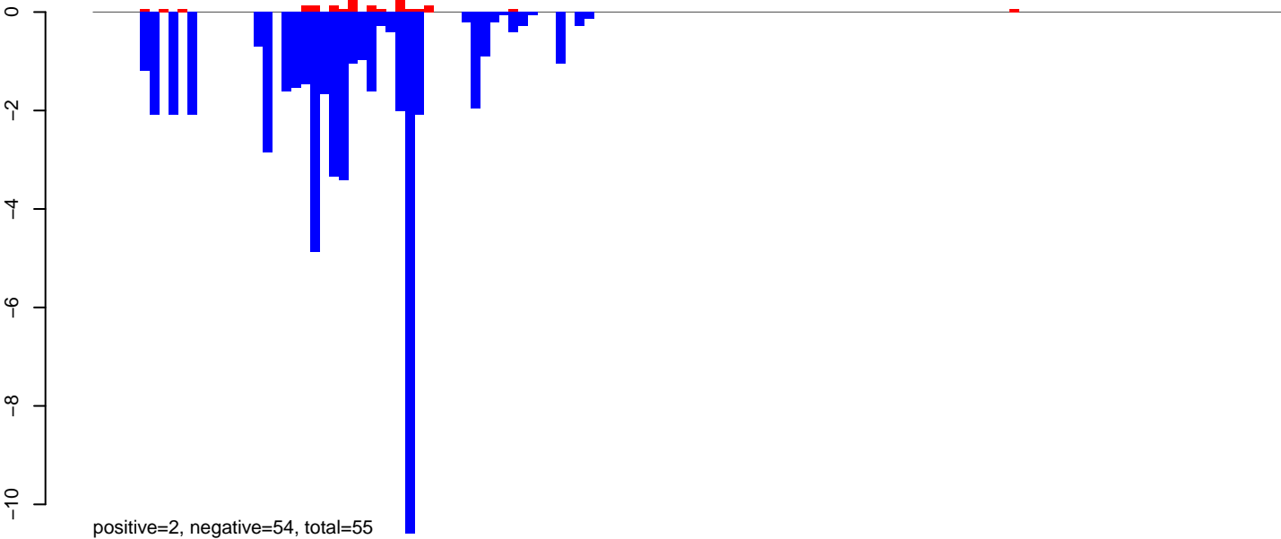
AeAeg_Aag2smallRNA_DENV2NGC_rep2.rep
