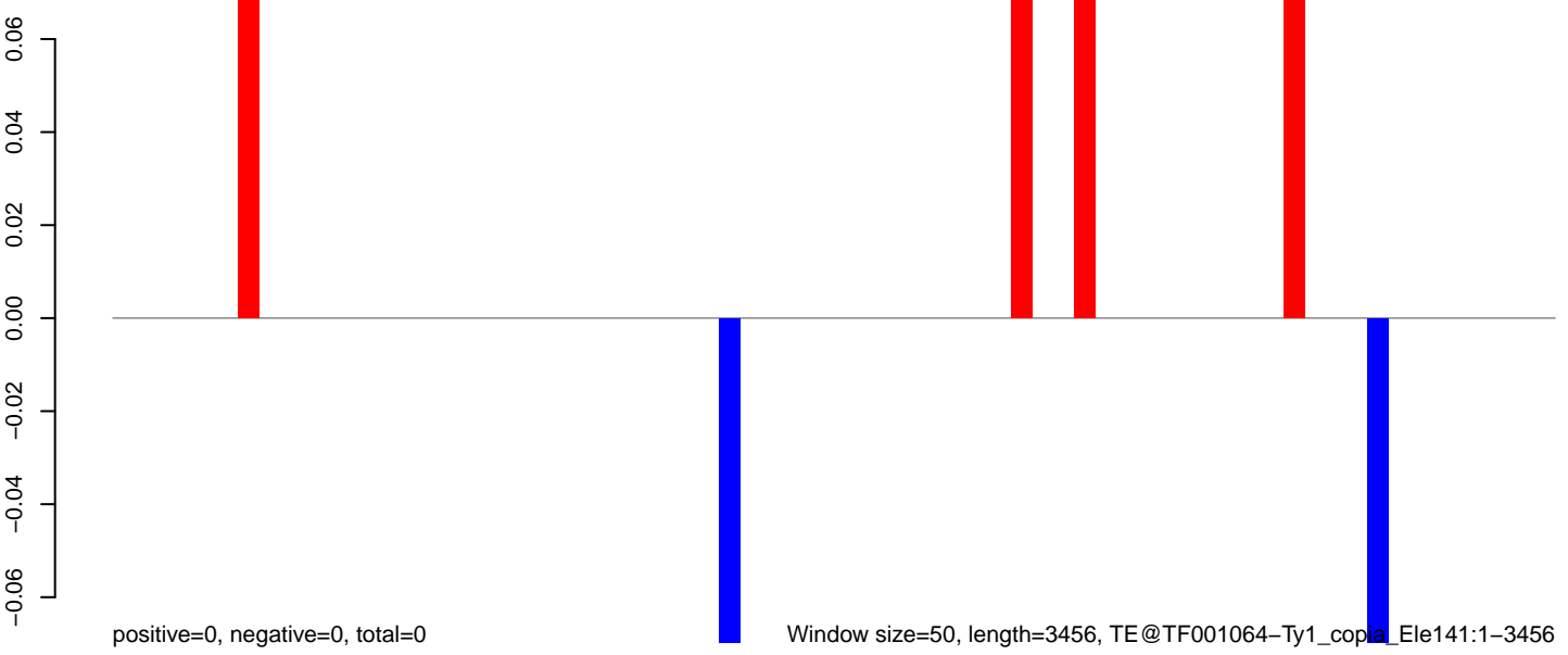
AeAeg_Aag2smallRNA_DENV2NGC_rep2.rep
