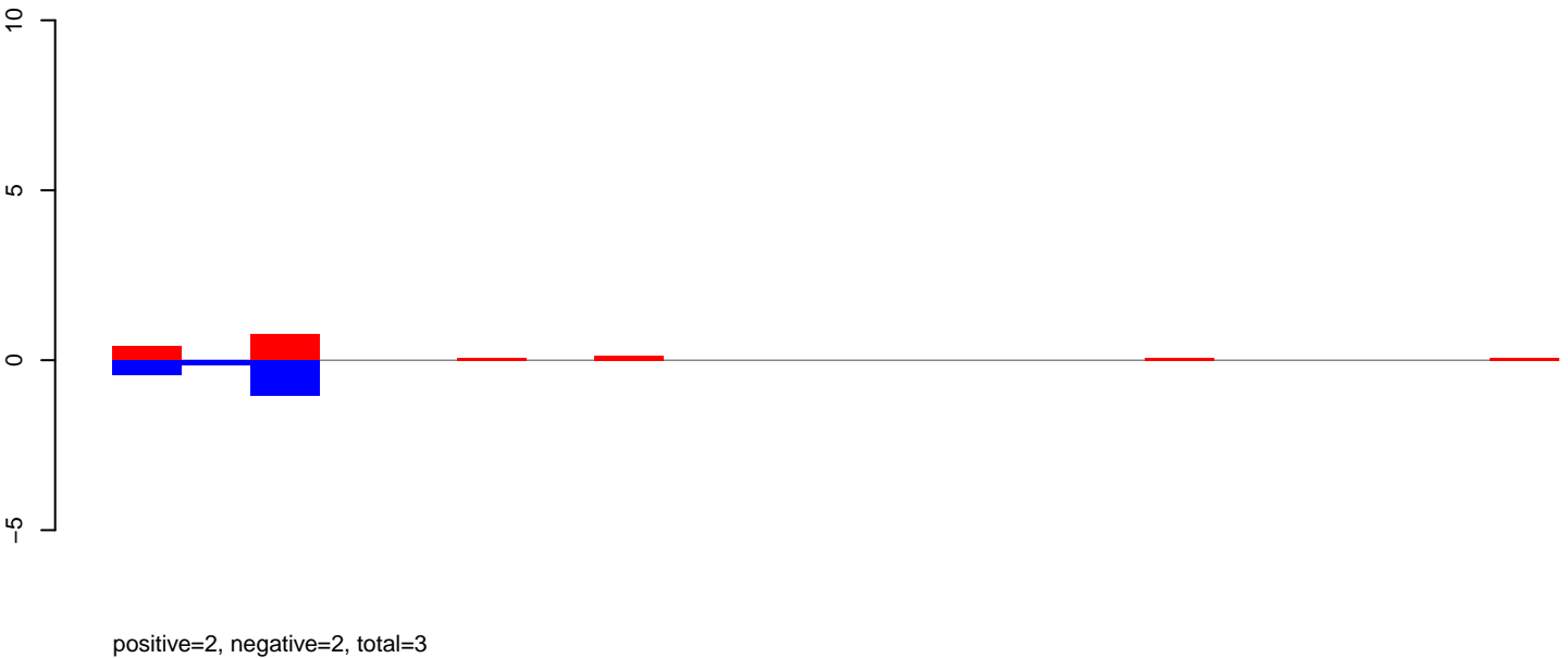
AeAeg_Aag2smallRNA_DENV2NGC_rep2.rep
