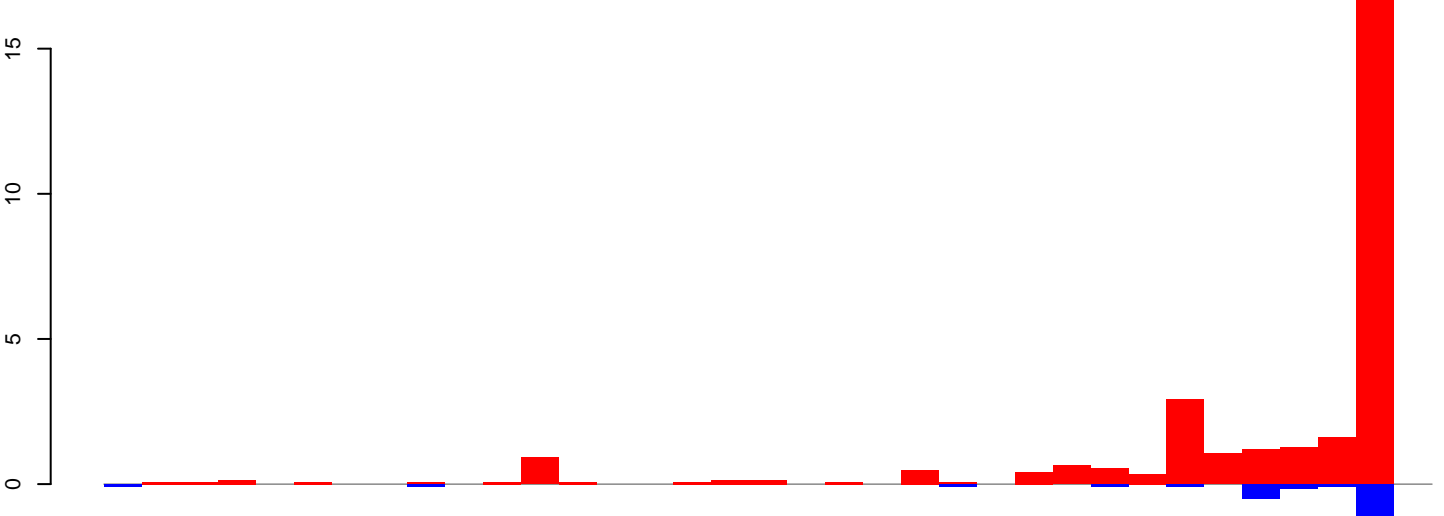
AeAeg_Aag2smallRNA_DENV2NGC_rep2.rep
