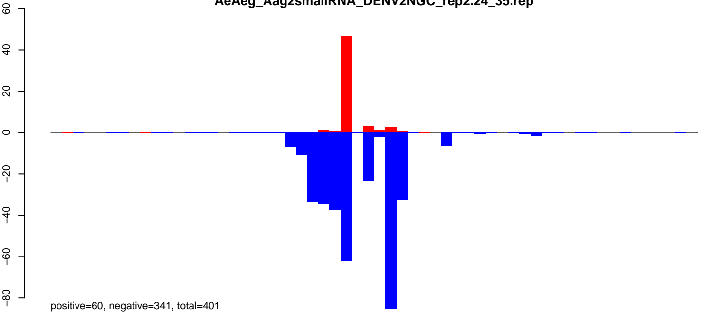
AeAeg_Aag2smallRNA_DENV2NGC_rep2.rep
