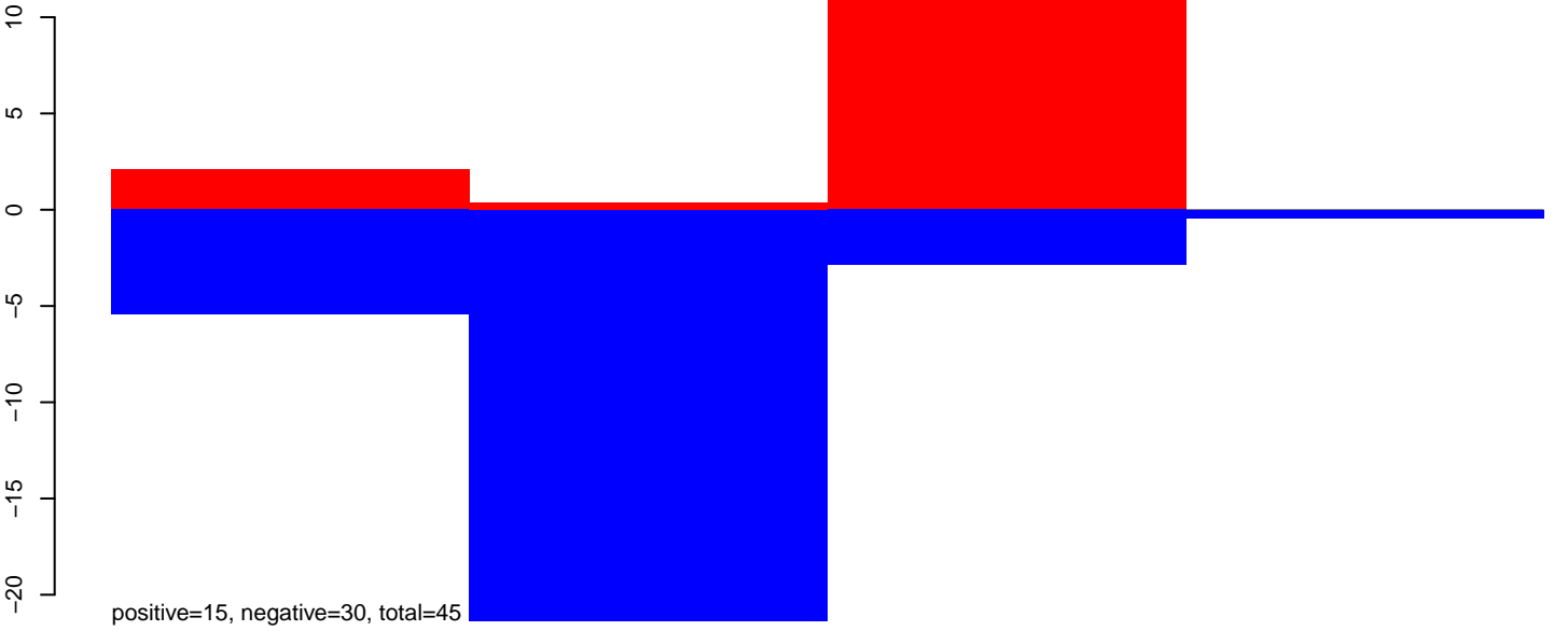
AeAeg_Aag2smallRNA_DENV2NGC_rep2.rep
