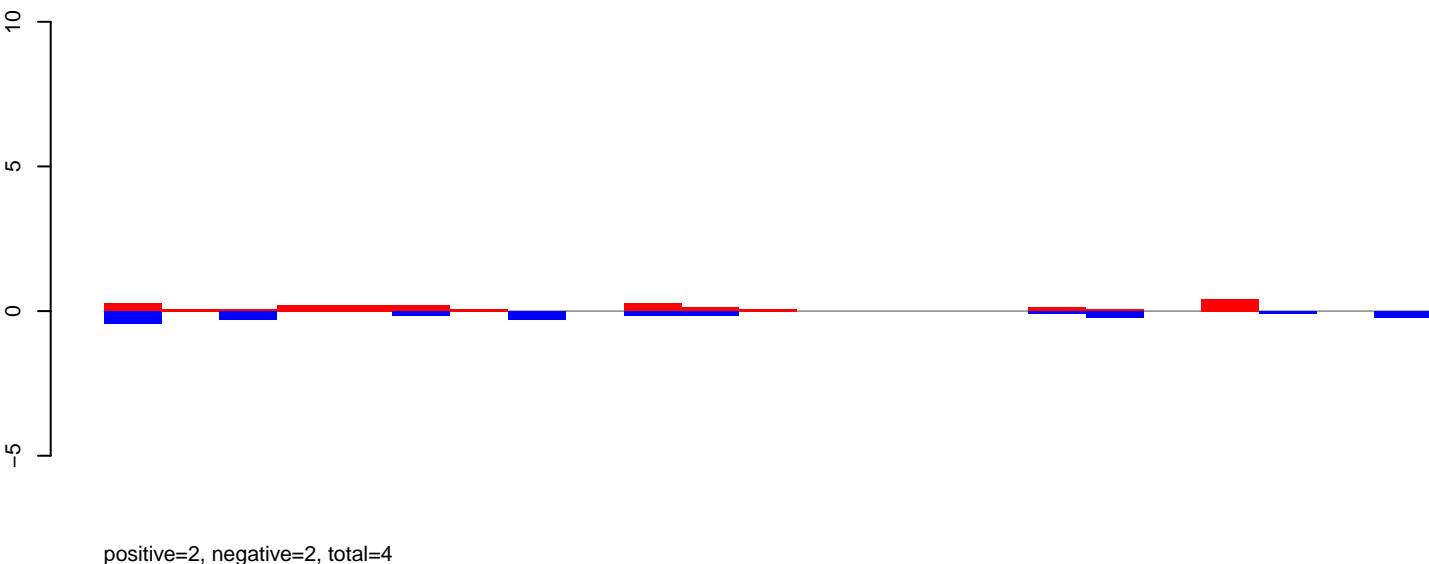
AeAeg_Aag2smallRNA_DENV2NGC_rep2.rep
