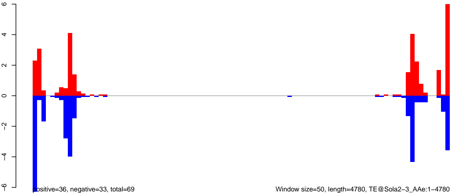
AeAeg_Aag2smallRNA_DENV2NGC_rep2.rep
