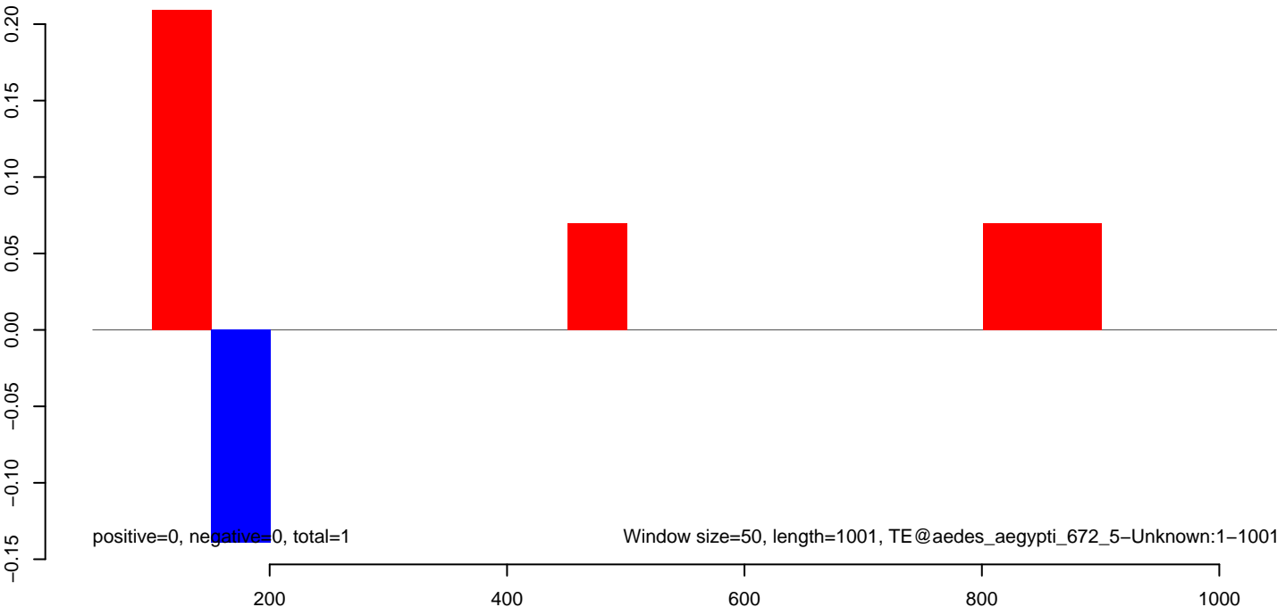
AeAeg_Aag2smallRNA_DENV2NGC_rep2.rep
