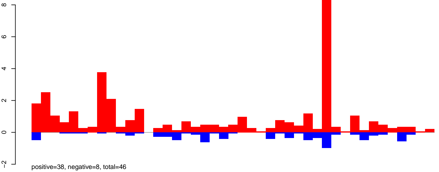
AeAeg_Aag2smallRNA_DENV2NGC_rep2.rep
