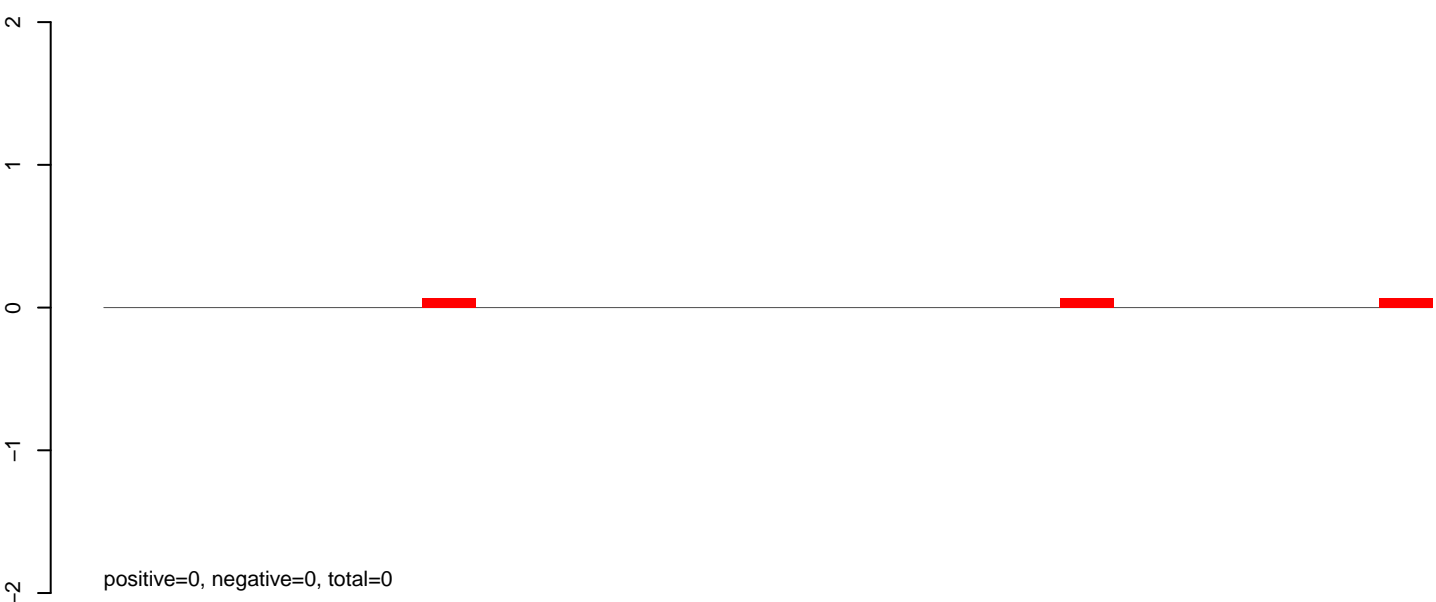
AeAeg_Aag2smallRNA_DENV2NGC_rep2.rep
