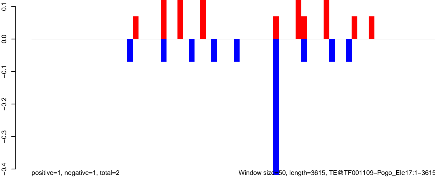
AeAeg_Aag2smallRNA_DENV2NGC_rep2.rep
