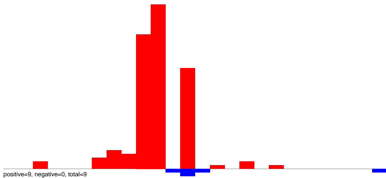
AeAeg_Aag2smallRNA_DENV2NGC_rep2.rep
