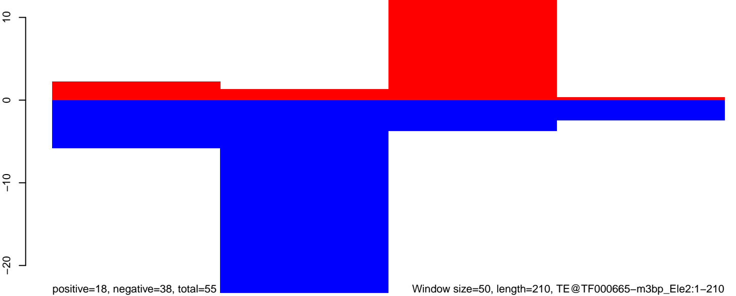
AeAeg_Aag2smallRNA_DENV2NGC_rep2.rep
