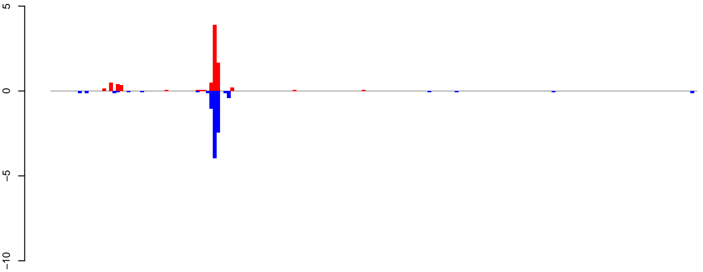
AeAeg_Aag2smallRNA_DENV2NGC_rep2.18_23.rep
