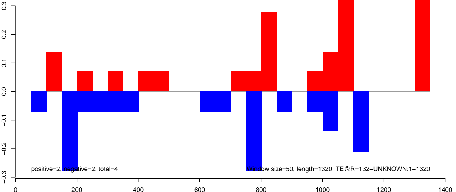
AeAeg_Aag2smallRNA_DENV2NGC_rep2.rep
