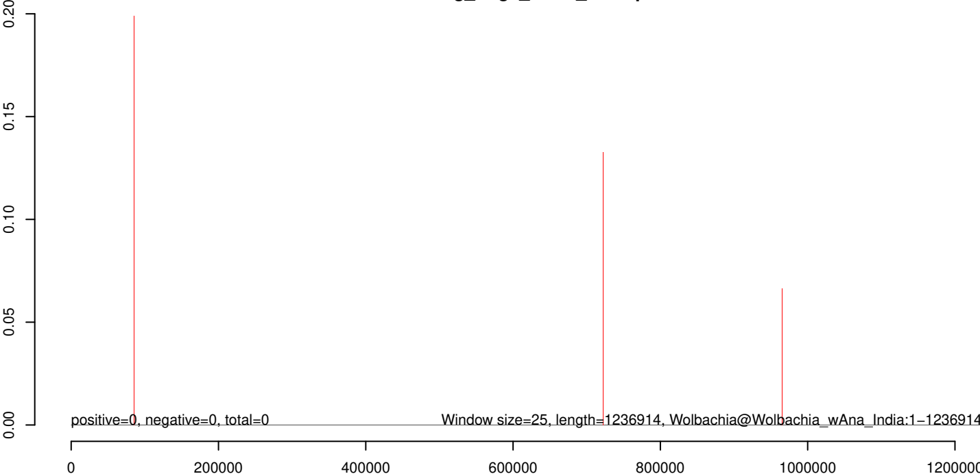
AeAeg_Aag2_BTV2_AK.rep
