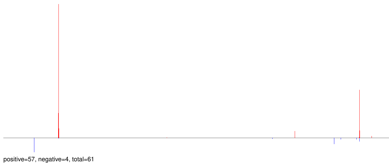
AeAeg_Whole_ZIKV_BM_RNA_GP.rep
