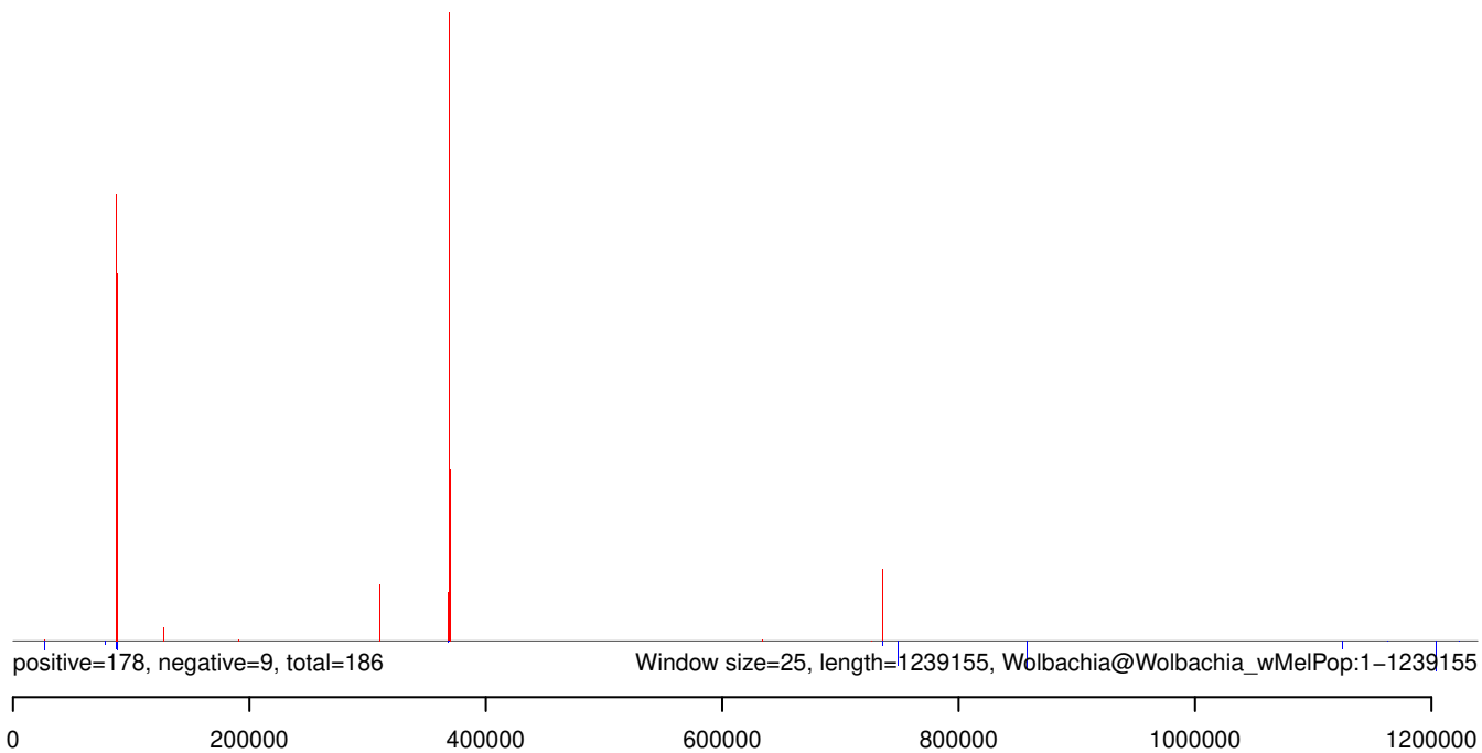
AeAeg_Whole_ZIKV_BM_RNA_GP.rep
