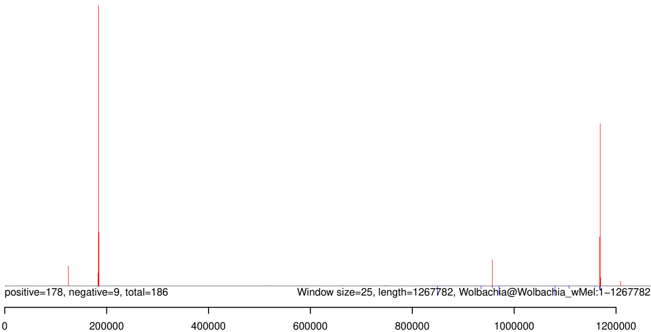
AeAeg_Whole_ZIKV_BM_RNA_GP.rep
