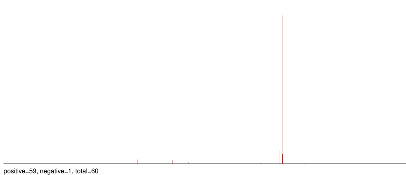
AeAeg_Whole_ZIKV_BM_RNA_GP.rep
