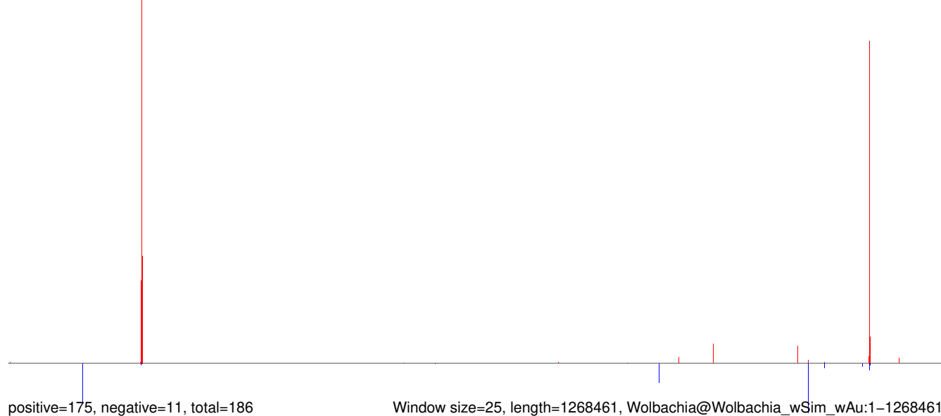
AeAeg_Whole_ZIKV_BM_RNA_GP.rep
