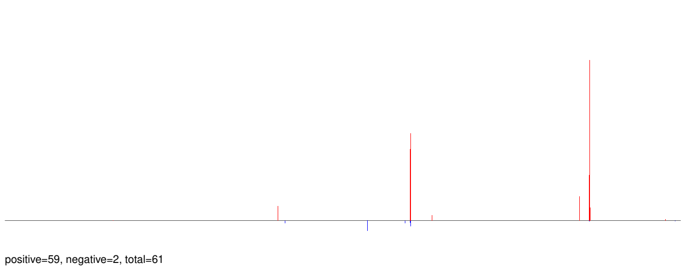
AeAeg_Whole_ZIKV_BM_RNA_GP.rep
