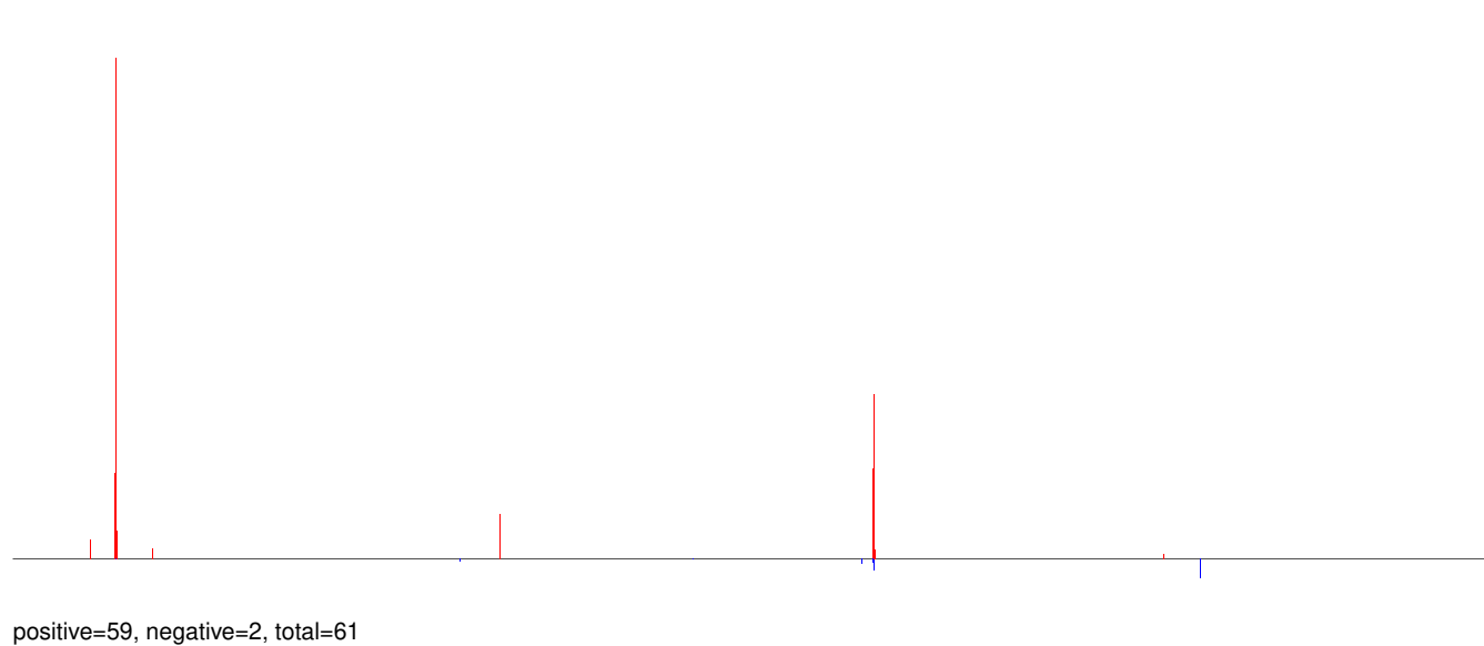
AeAeg_Whole_ZIKV_BM_RNA_GP.rep
