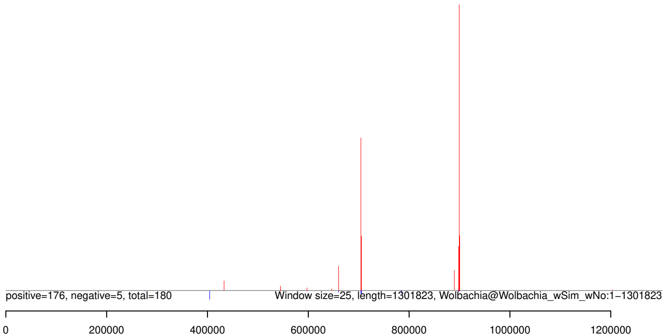
AeAeg_Whole_ZIKV_BM_RNA_GP.rep
