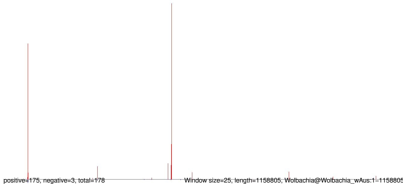
AeAeg_Whole_ZIKV_BM_RNA_GP.rep
