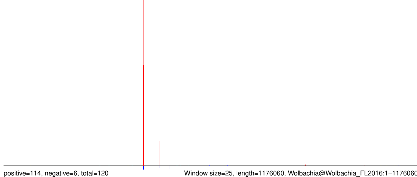
AeAeg_Whole_ZIKV_BM_RNA_GP.rep
