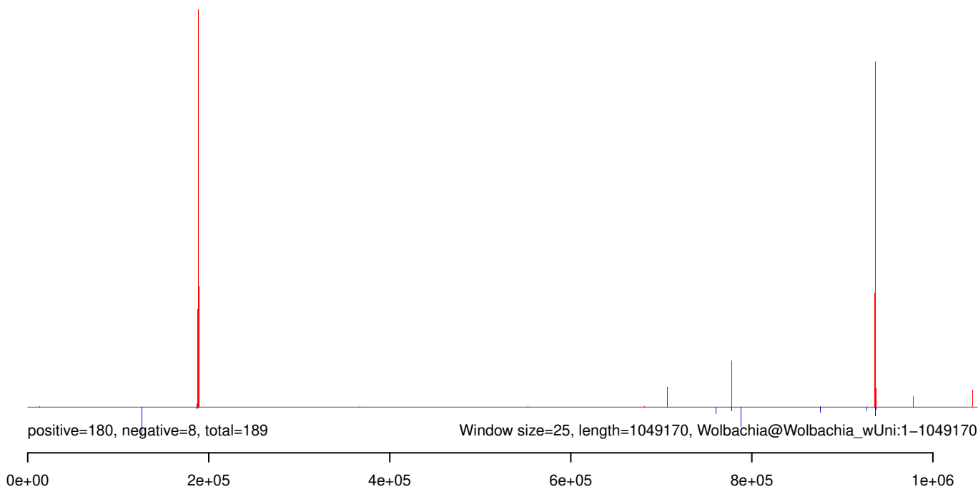
AeAeg_Whole_ZIKV_BM_RNA_GP.rep
