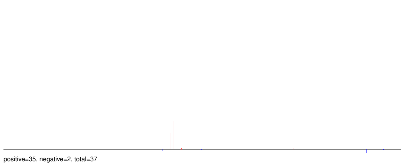
AeAeg_Whole_ZIKV_BM_RNA_GP.rep
