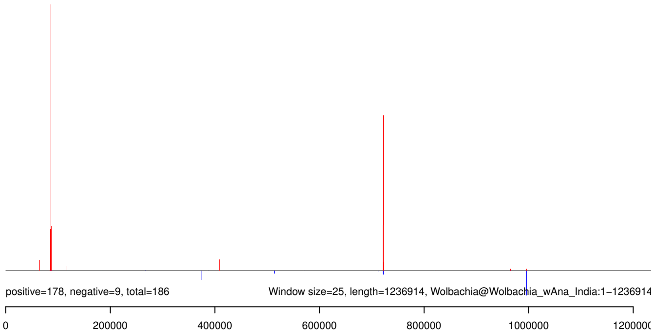
AeAeg_Whole_ZIKV_BM_RNA_GP.rep
