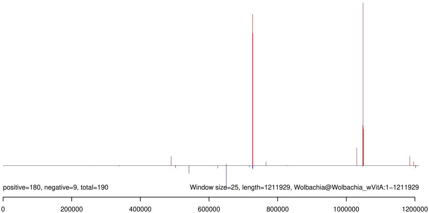
AeAeg_Whole_ZIKV_BM_RNA_GP.rep
