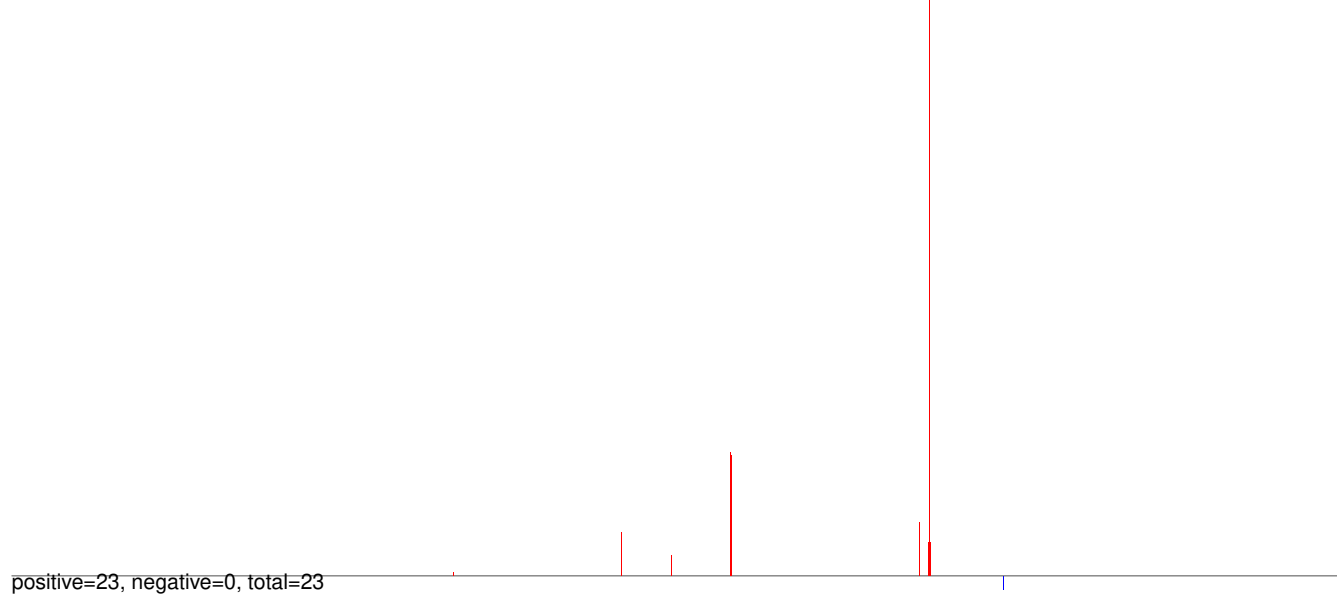
AeAeg_Whole_ZIKVdr_In3_GP.rep
