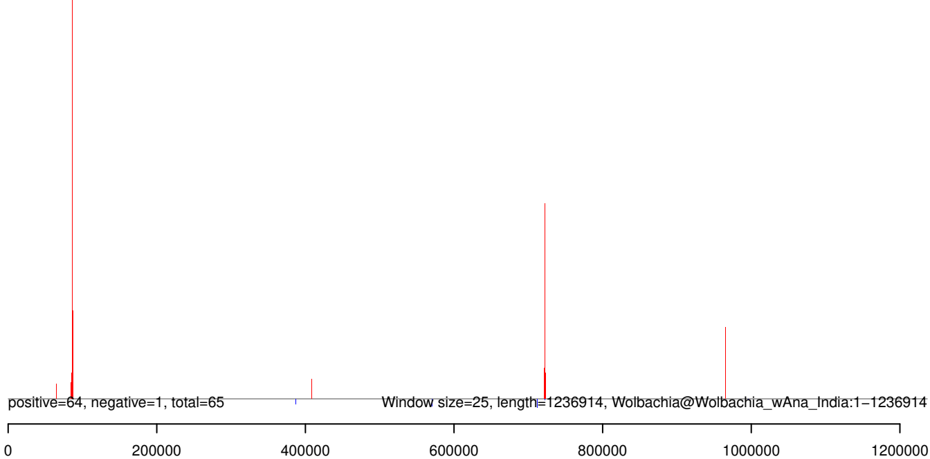
AeAeg_Whole_ZIKVdr_In3_GP.rep
