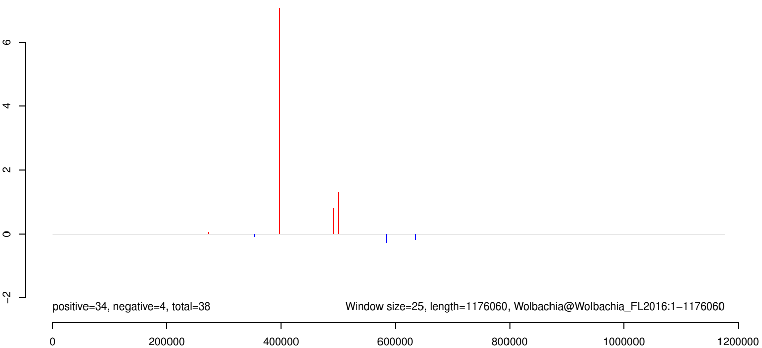
AeAeg_Whole_ZIKVdr_In3_GP.rep
