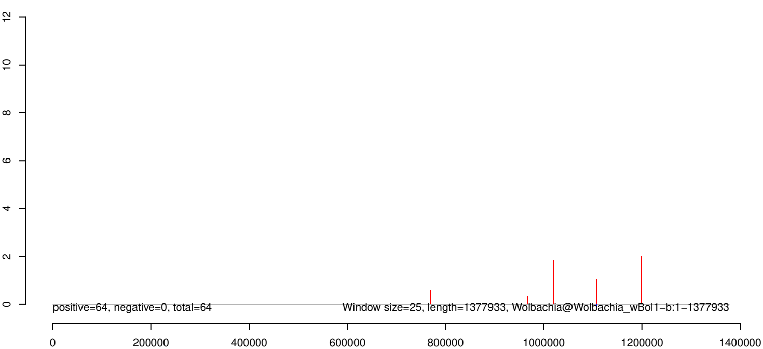
AeAeg_Whole_ZIKVdr_In3_GP.rep
