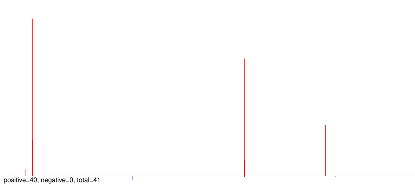
AeAeg_Whole_ZIKVdr_In3_GP.24_35.rep
