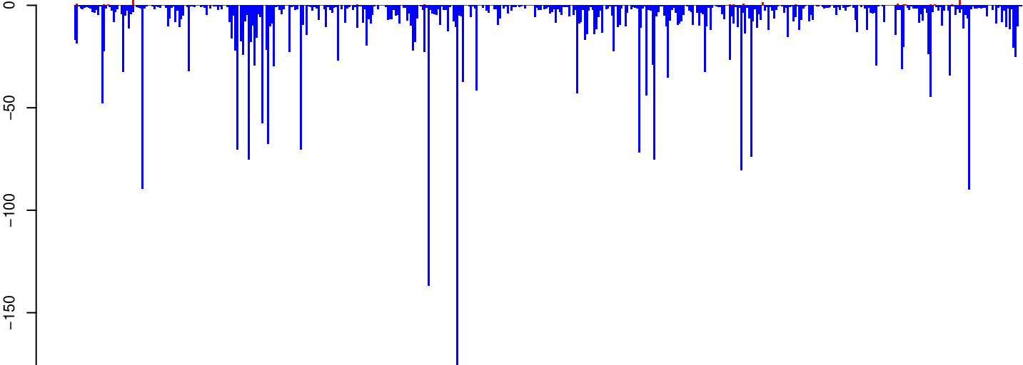
AeAeg_Aag2SINV_Ago3.IP.rep
