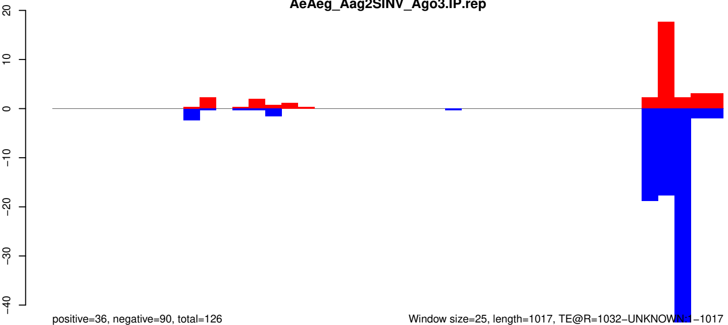
AeAeg_Aag2SINV_Ago3.IP.rep
