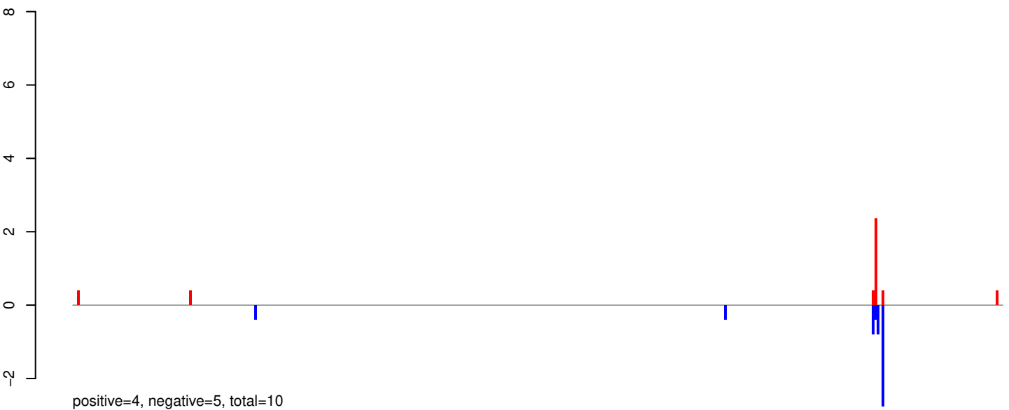
AeAeg_Aag2SINV_Ago3.IP.rep
