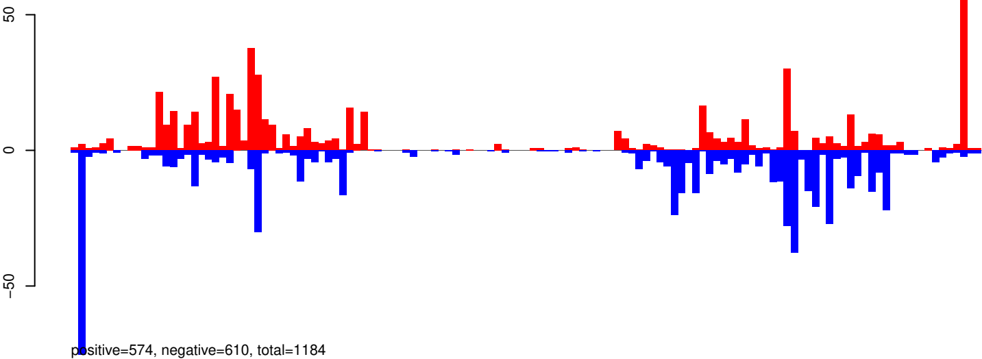
AeAeg_Aag2SINV_Ago3.IP.24_35.rep
