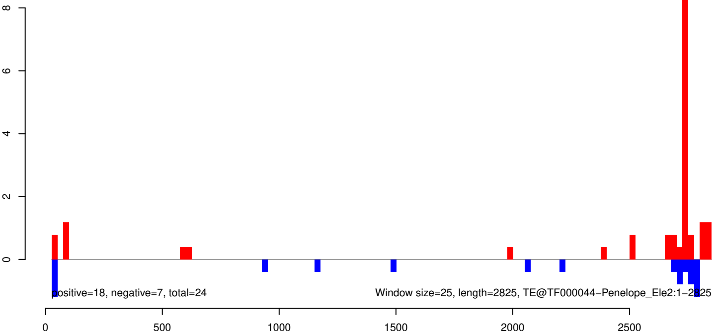
AeAeg_Aag2SINV_Ago3.IP.rep
