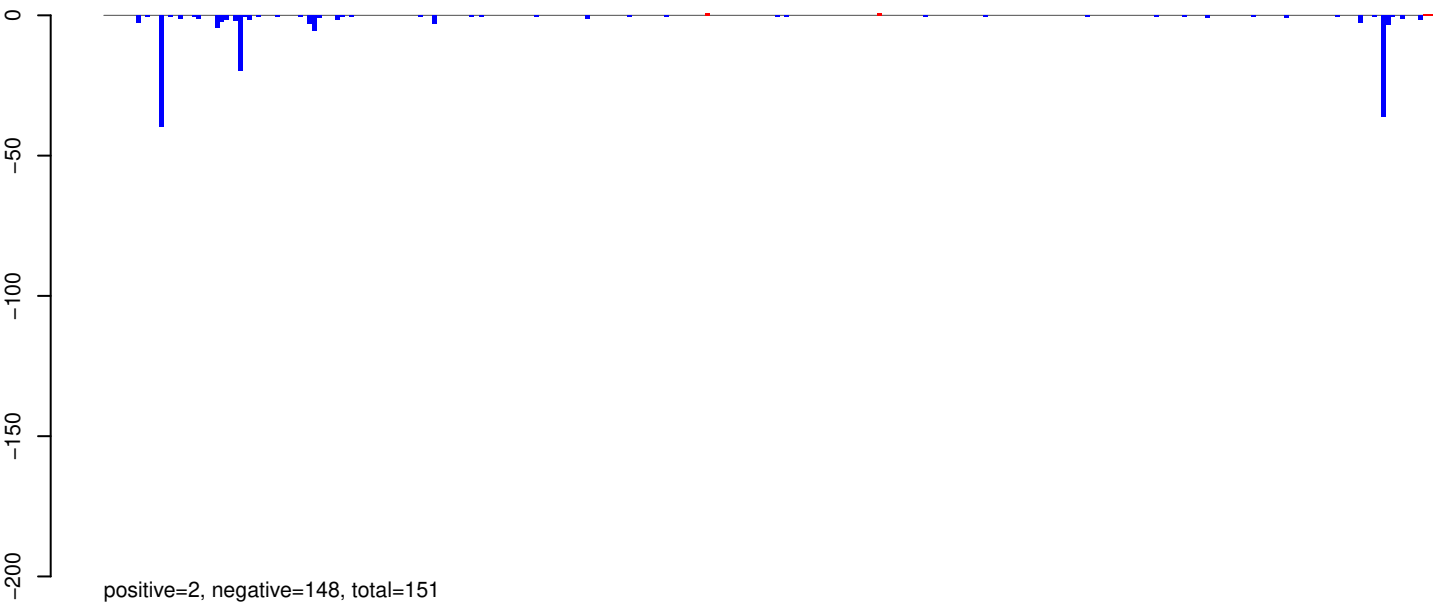
AeAeg_Aag2SINV_Ago3.IP.24_35.rep
