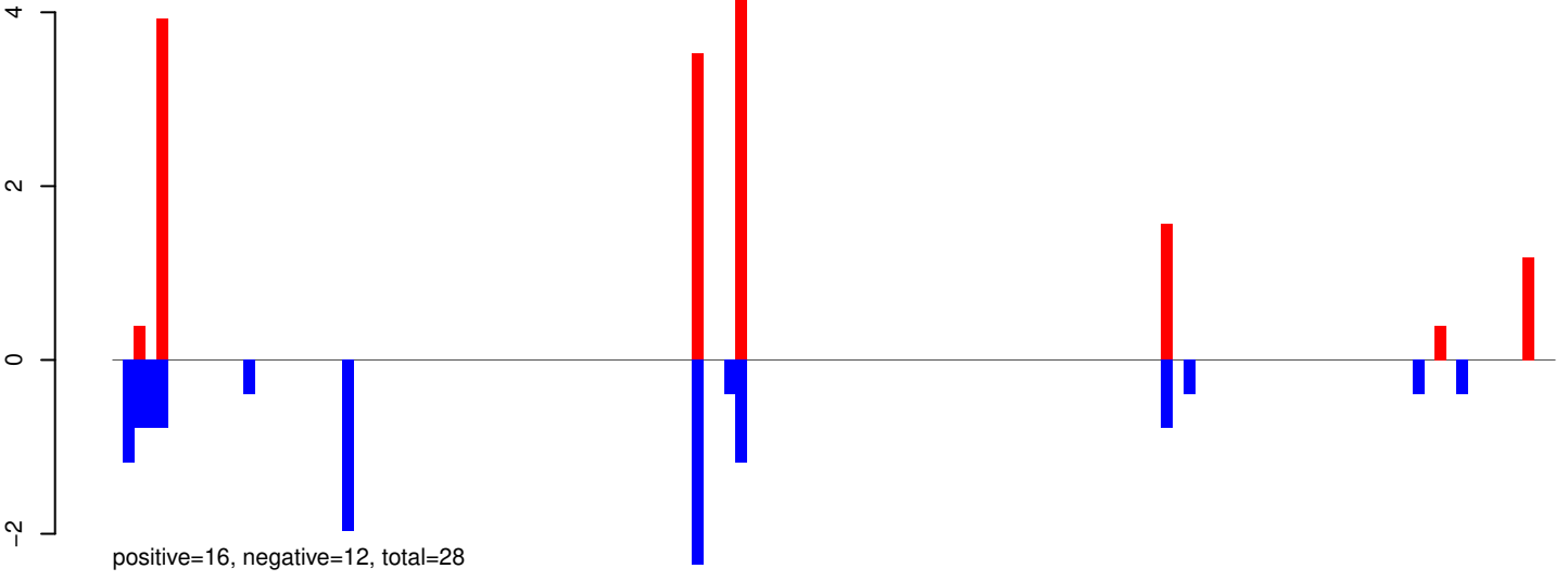
AeAeg_Aag2SINV_Ago3.IP.24_35.rep
