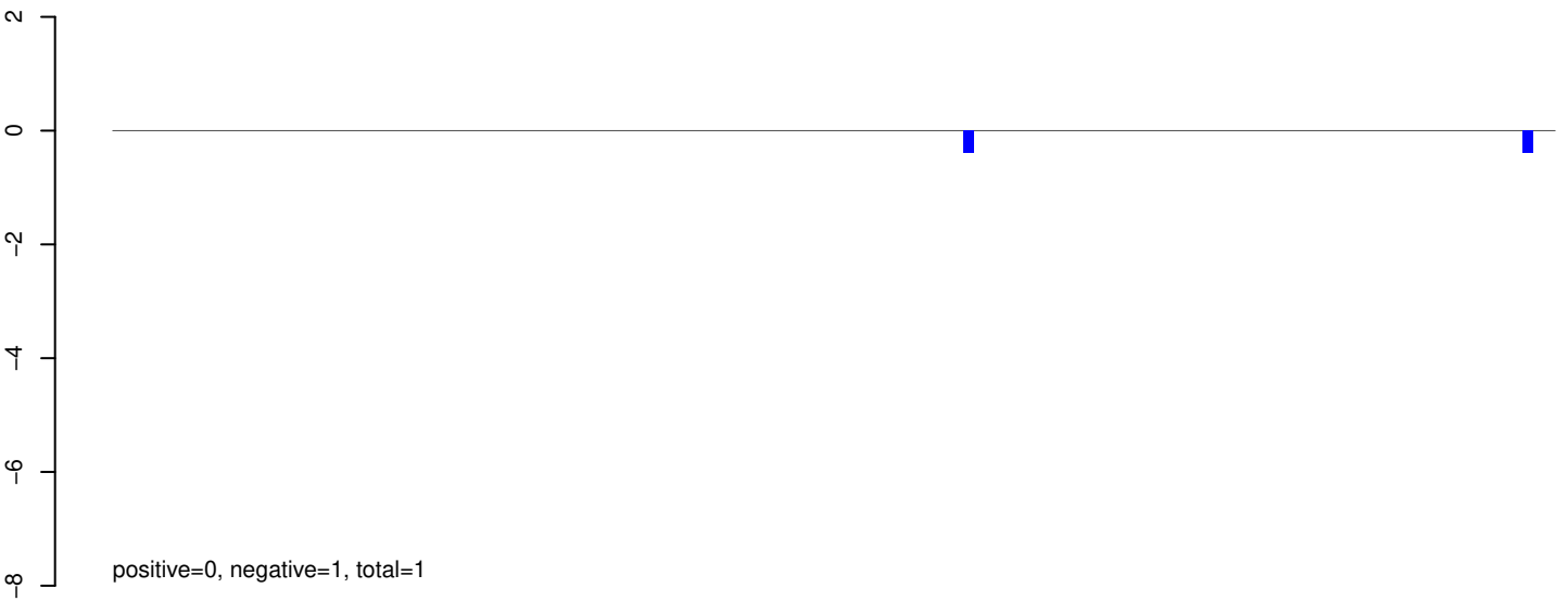
AeAeg_Aag2SINV_Ago3.IP.rep
