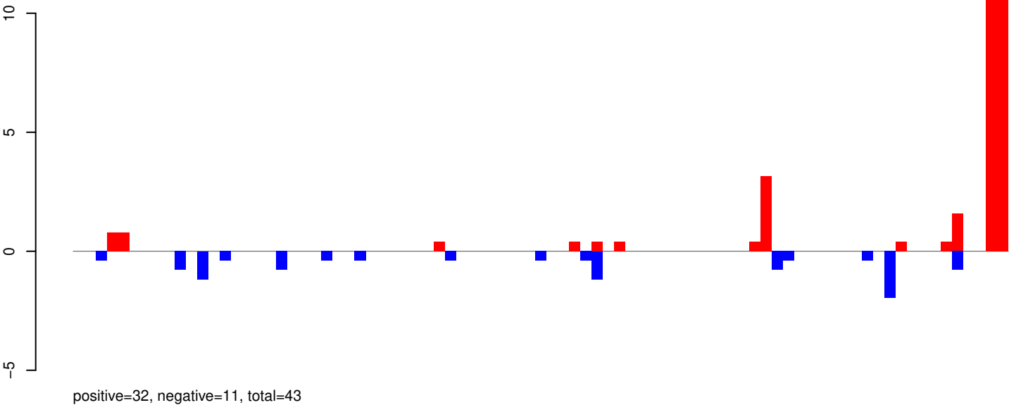
AeAeg_Aag2SINV_Ago3.IP.24_35.rep
