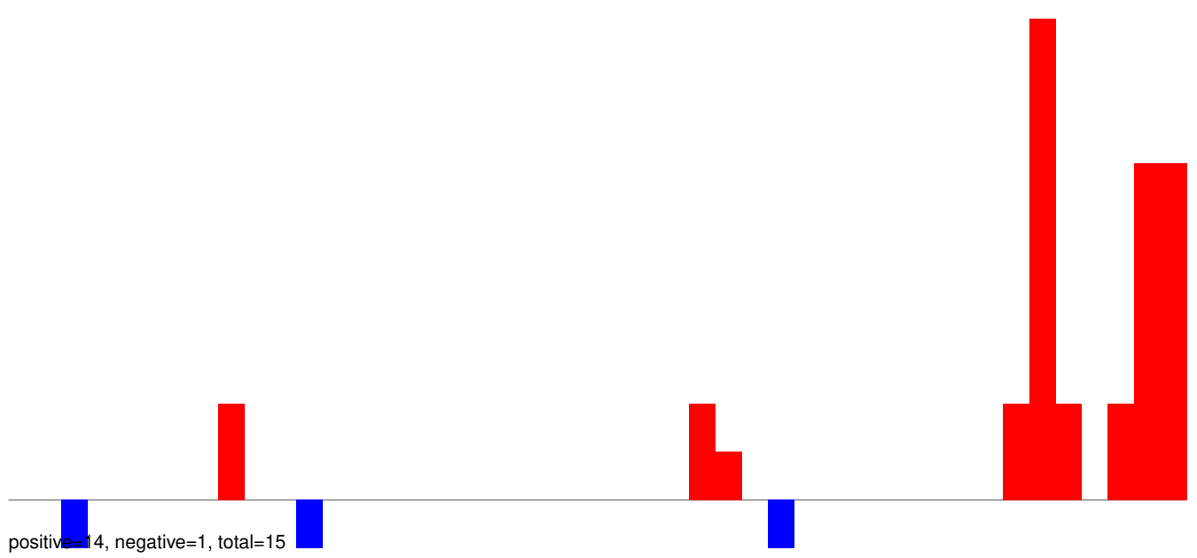
AeAeg_Aag2SINV_Ago3.IP.24_35.rep
