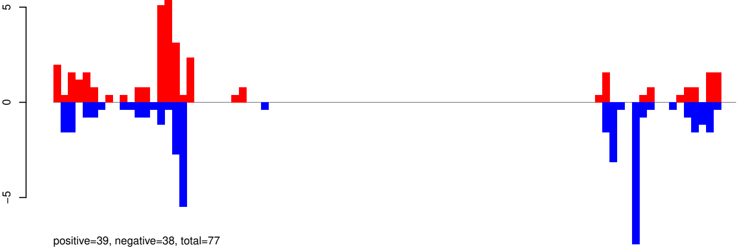
AeAeg_Aag2SINV_Ago3.IP.24_35.rep
