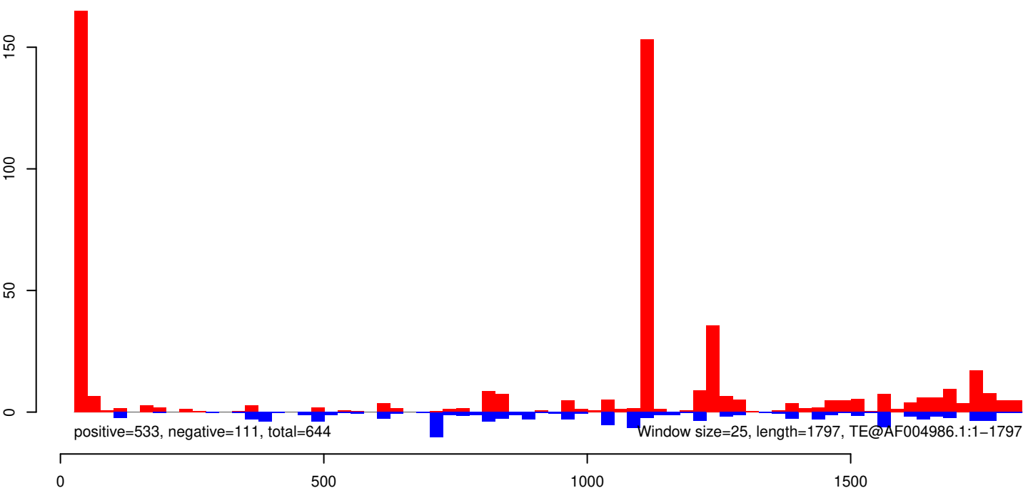
AeAeg_Aag2SINV_Ago3.IP.rep
