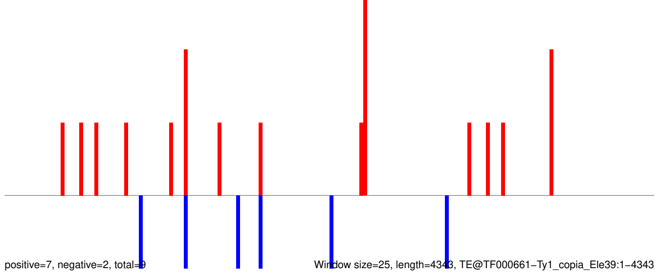
AeAeg_Aag2SINV_Ago3.IP.rep
