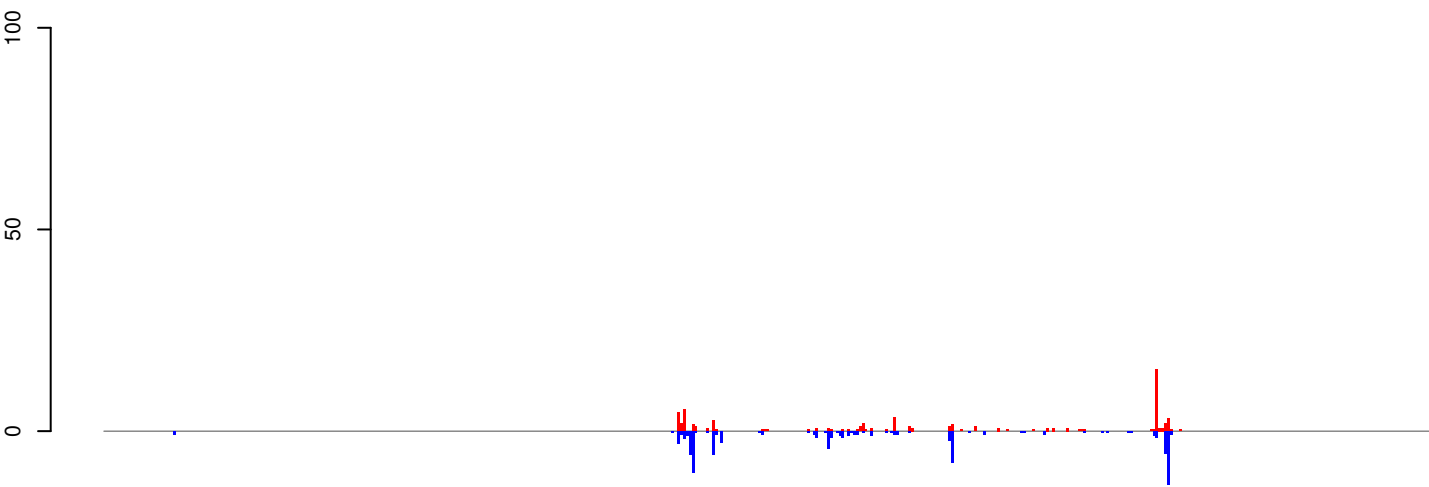
AeAeg_Aag2SINV_Ago3.IP.18_23.rep
