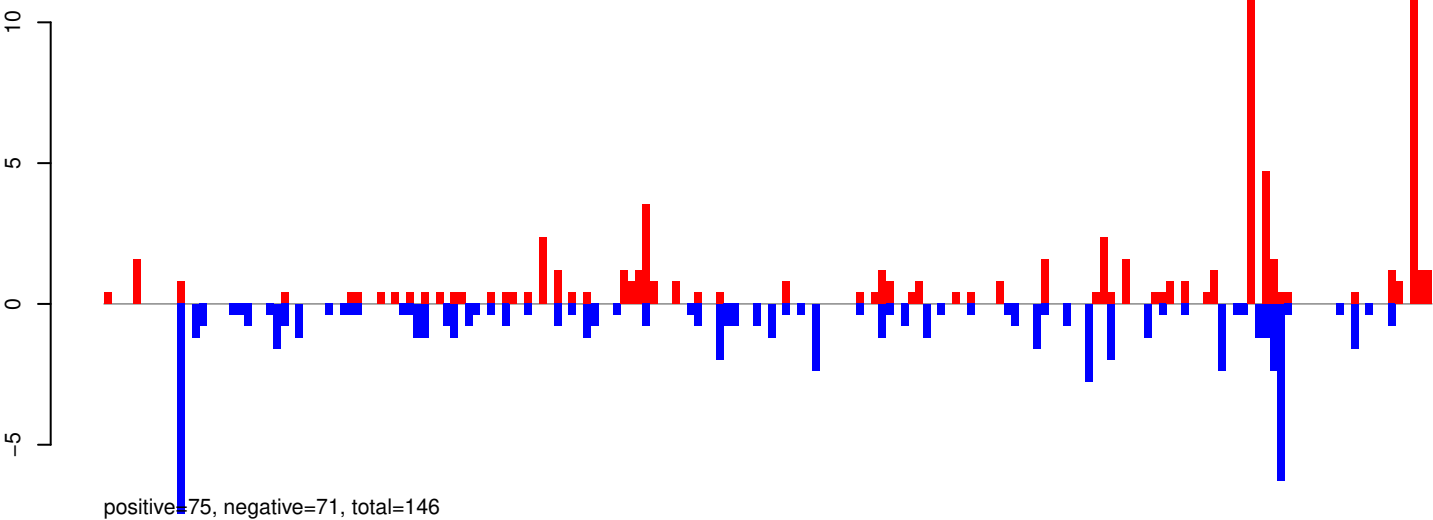
AeAeg_Aag2SINV_Ago3.IP.24_35.rep
