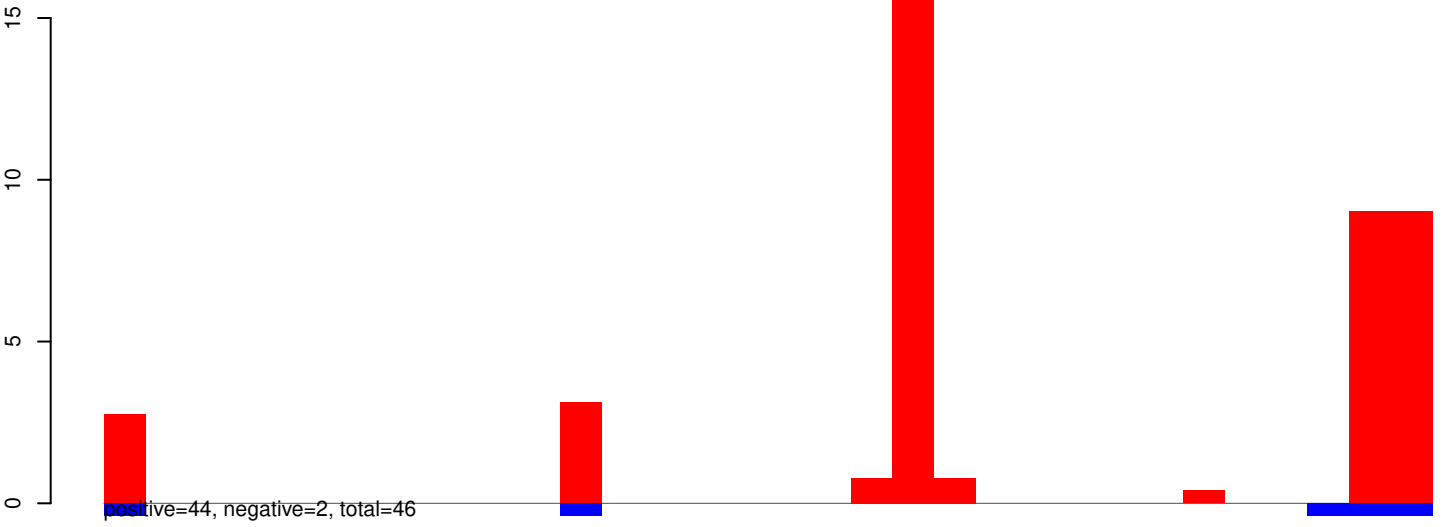
AeAeg_Aag2SINV_Ago3.IP.24_35.rep
