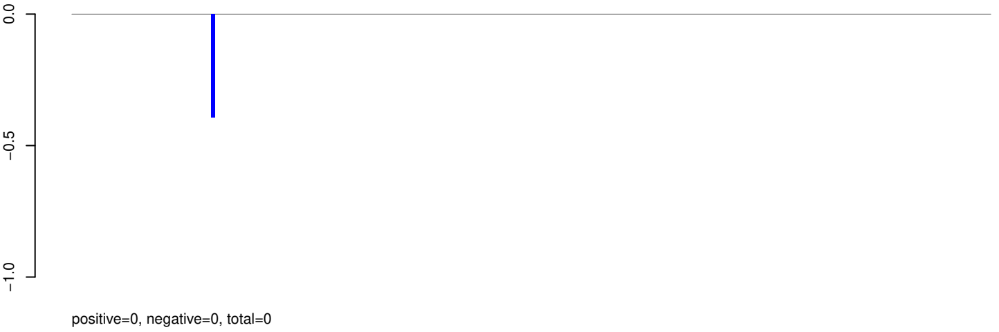
AeAeg_Aag2SINV_Ago3.IP.rep
