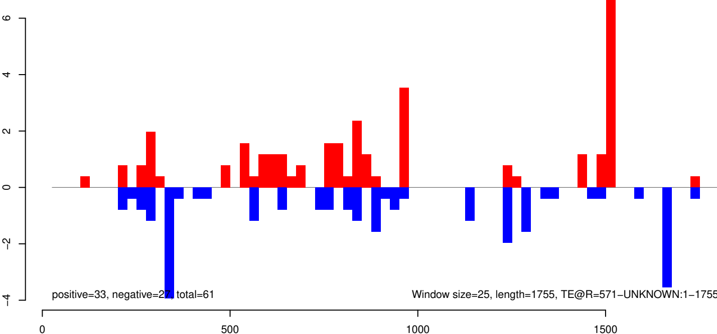
AeAeg_Aag2SINV_Ago3.IP.rep
