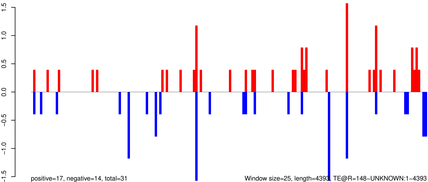
AeAeg_Aag2SINV_Ago3.IP.rep
