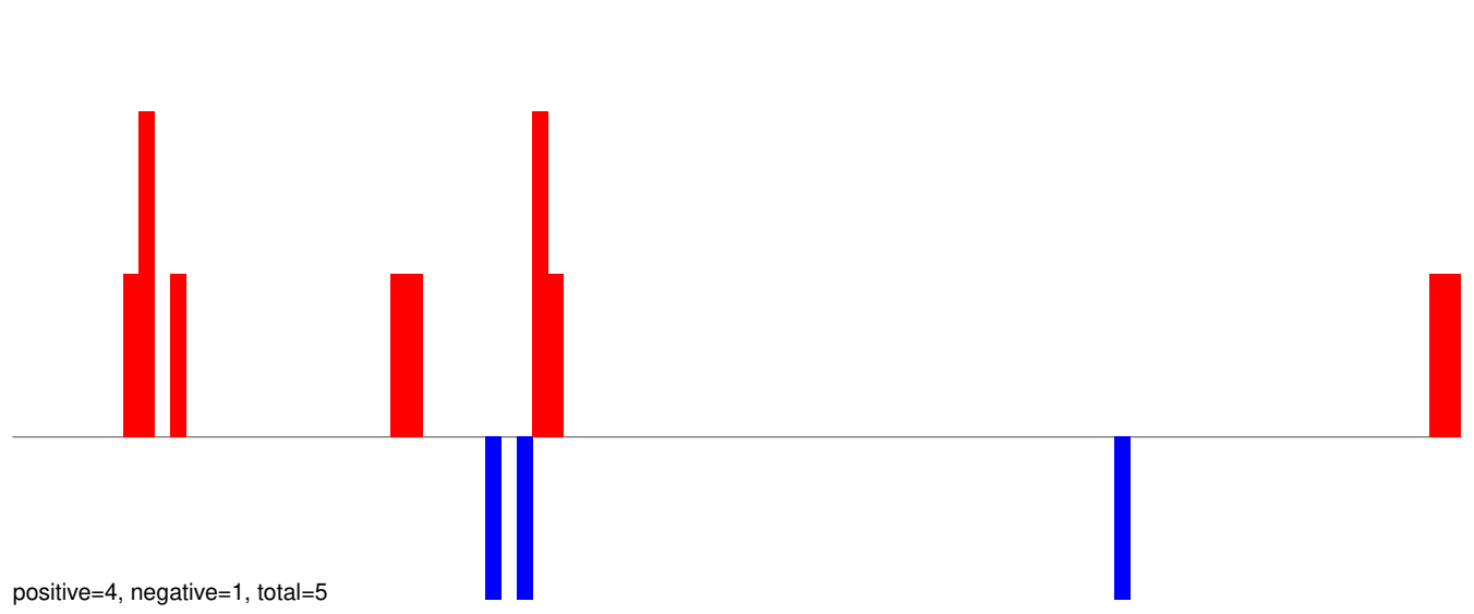
AeAeg_Aag2SINV_Ago3.IP.24_35.rep
