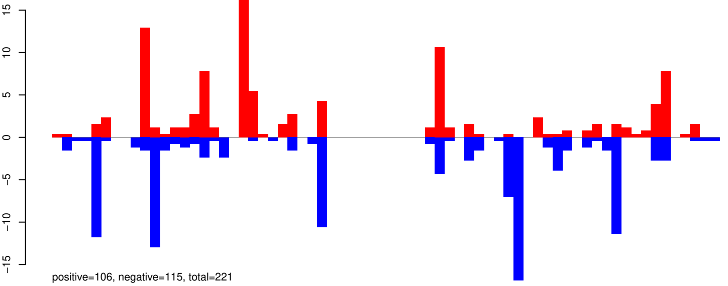
AeAeg_Aag2SINV_Ago3.IP.24_35.rep
