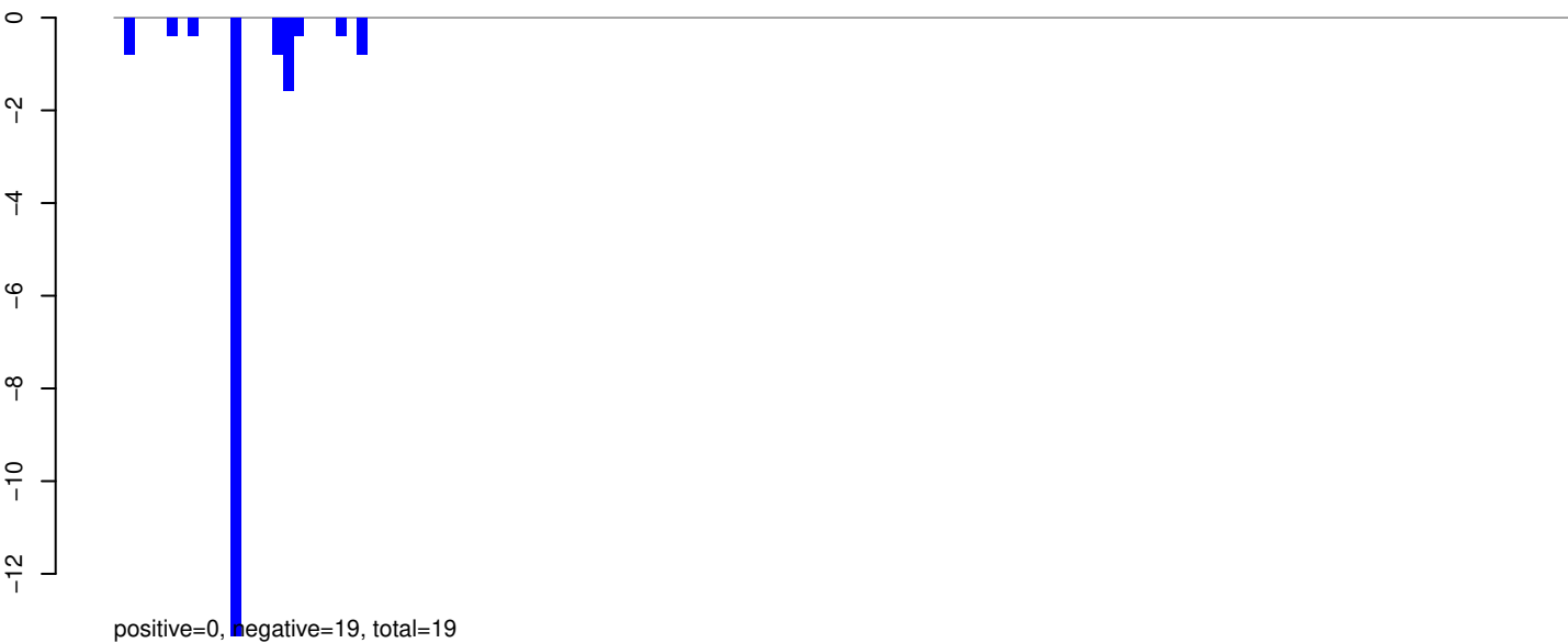
AeAeg_Aag2SINV_Ago3.IP.24_35.rep
