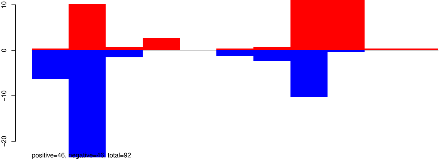
AeAeg_Aag2SINV_Ago3.IP.24_35.rep
