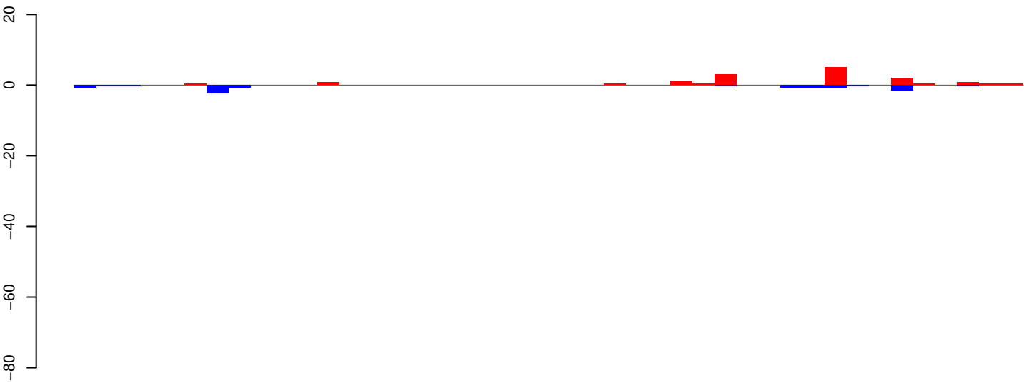
AeAeg_Aag2SINV_Ago3.IP.18_23.rep
