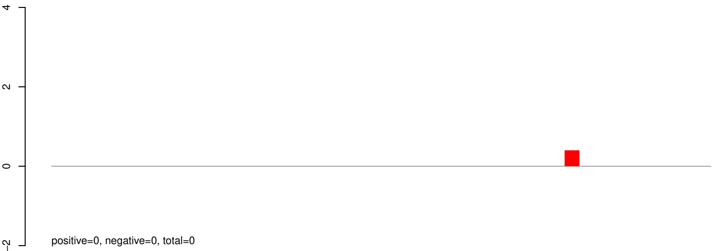
AeAeg_Aag2SINV_Ago3.IP.rep
