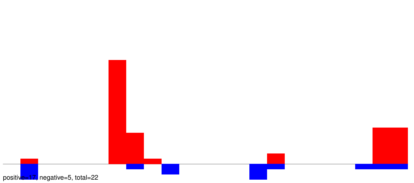
AeAeg_Aag2SINV_Ago3.IP.24_35.rep
