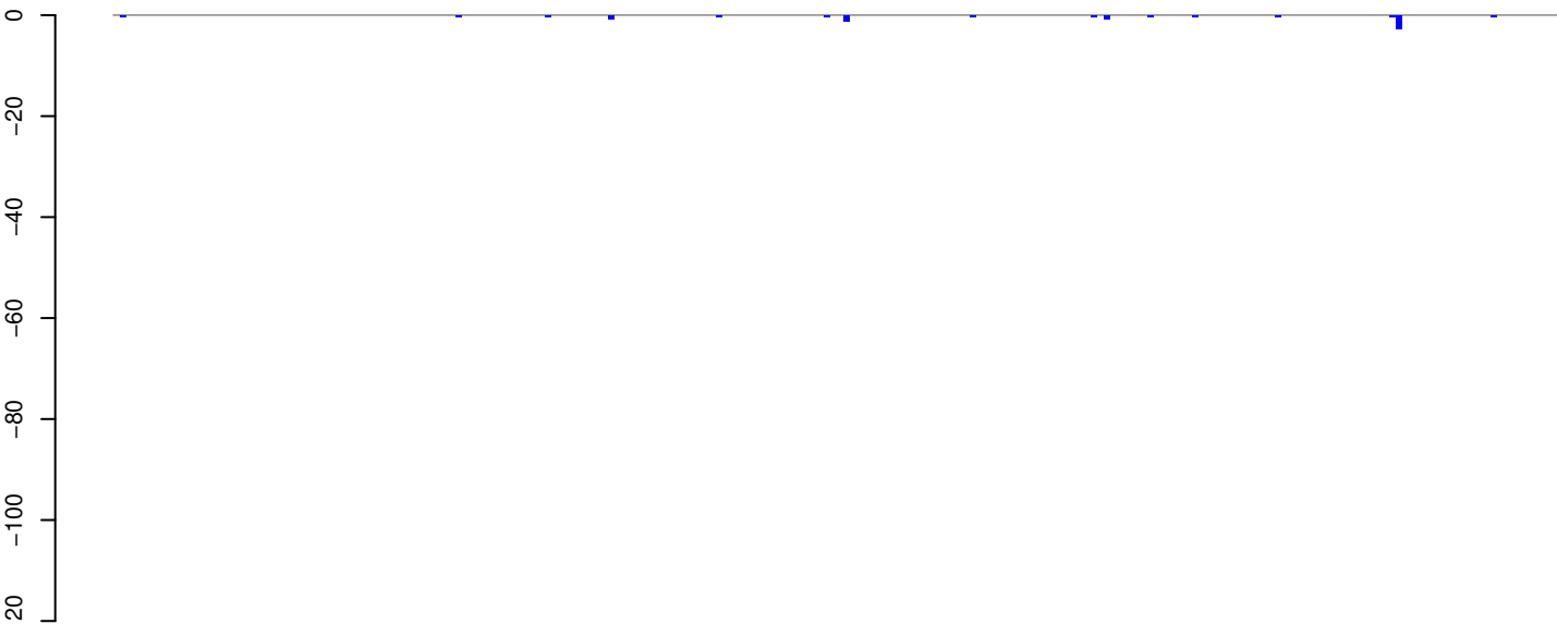
AeAeg_Aag2SINV_Ago3.IP.18_23.rep
