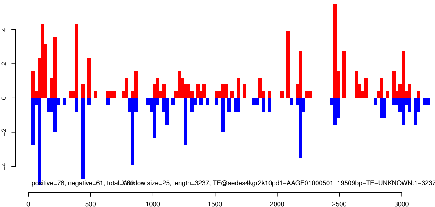
AeAeg_Aag2SINV_Ago3.IP.rep
