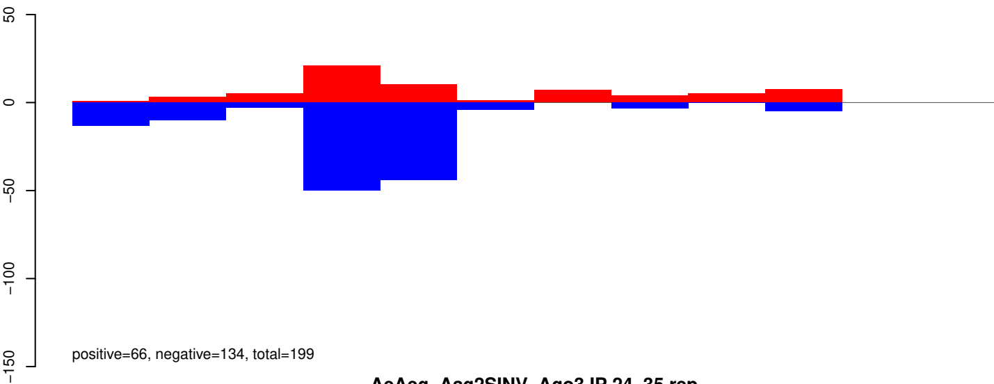
AeAeg_Aag2SINV_Ago3.IP.24_35.rep
