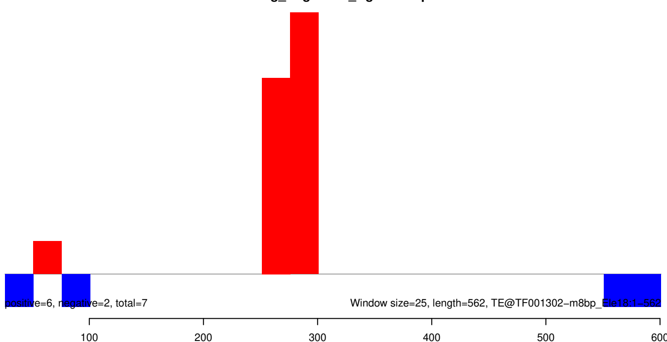
AeAeg_Aag2SINV_Ago3.IP.rep
