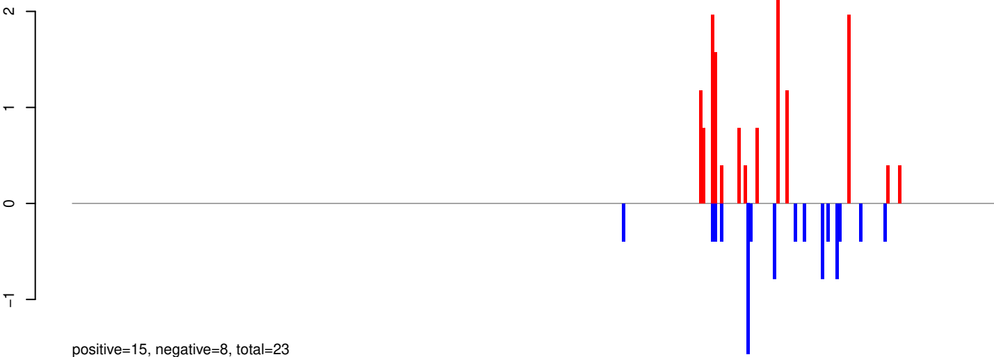
AeAeg_Aag2SINV_Ago3.IP.24_35.rep
