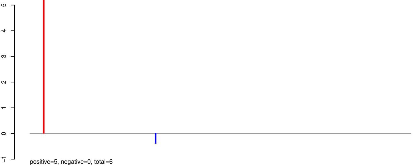
AeAeg_Aag2SINV_Ago3.IP.rep
