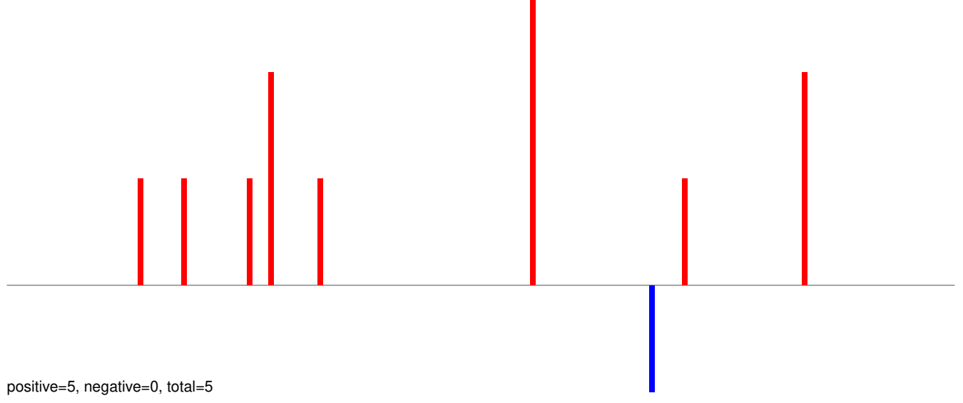
AeAeg_Aag2SINV_Ago3.IP.rep
