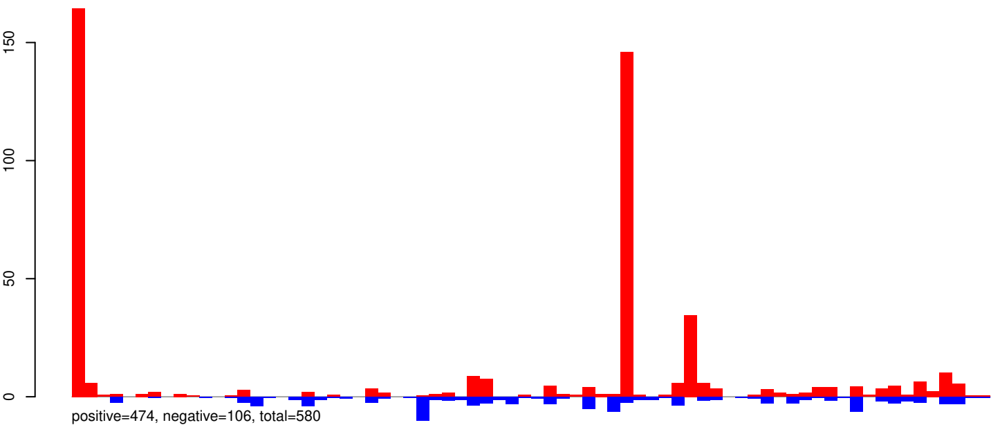
AeAeg_Aag2SINV_Ago3.IP.24_35.rep
