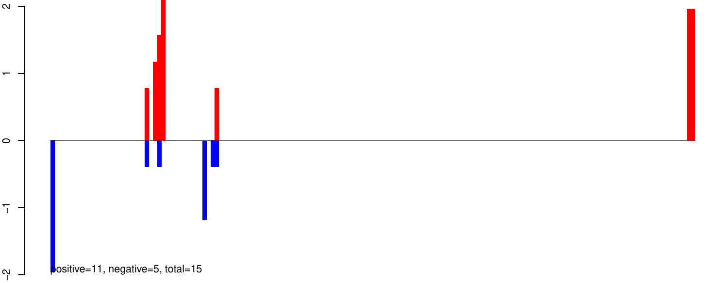
AeAeg_Aag2SINV_Ago3.IP.24_35.rep
