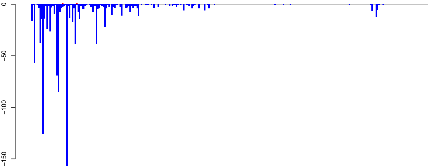
AeAeg_Aag2SINV_Ago3.IP.24_35.rep
