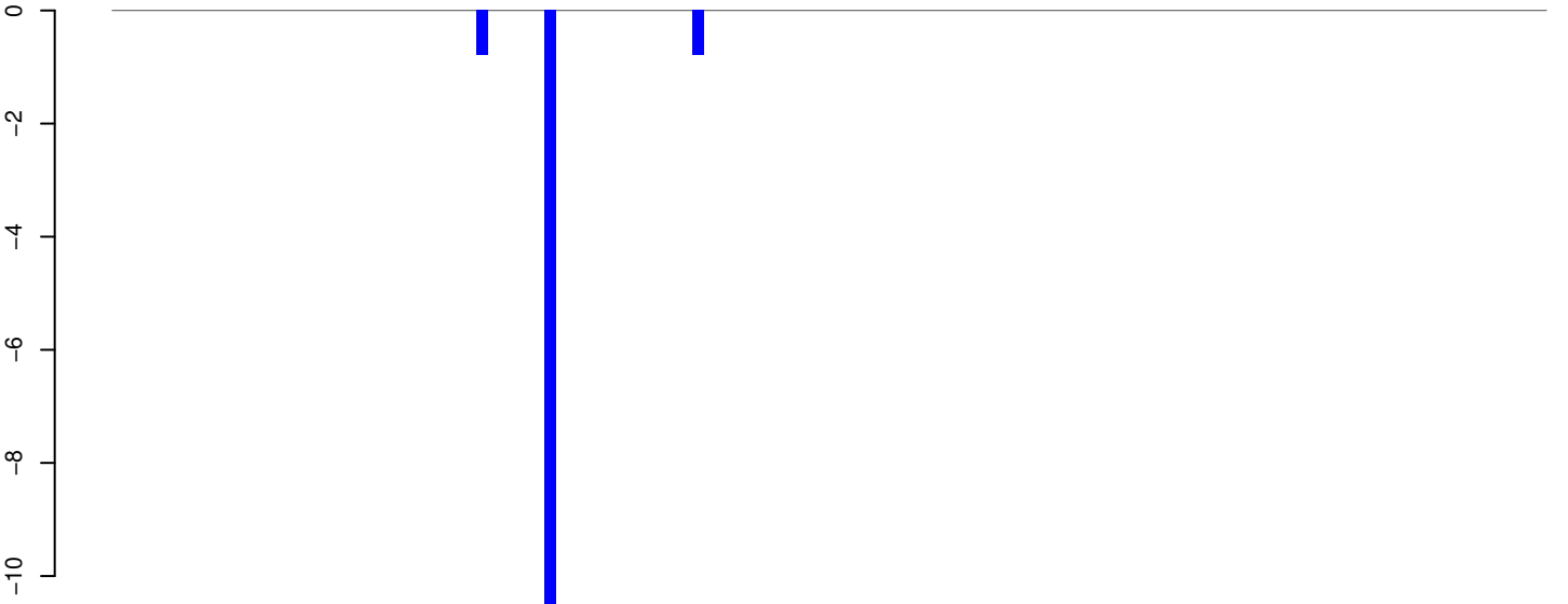
AeAeg_Aag2SINV_Ago3.IP.rep
