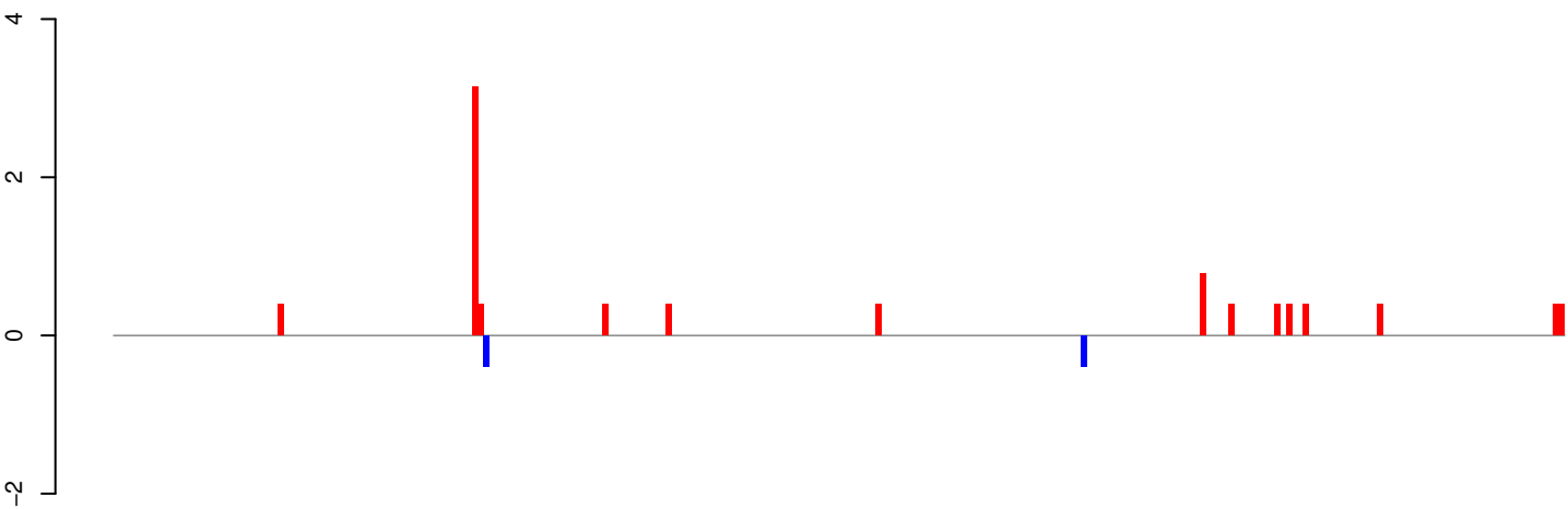
AeAeg_Aag2SINV_Ago3.IP.18_23.rep
