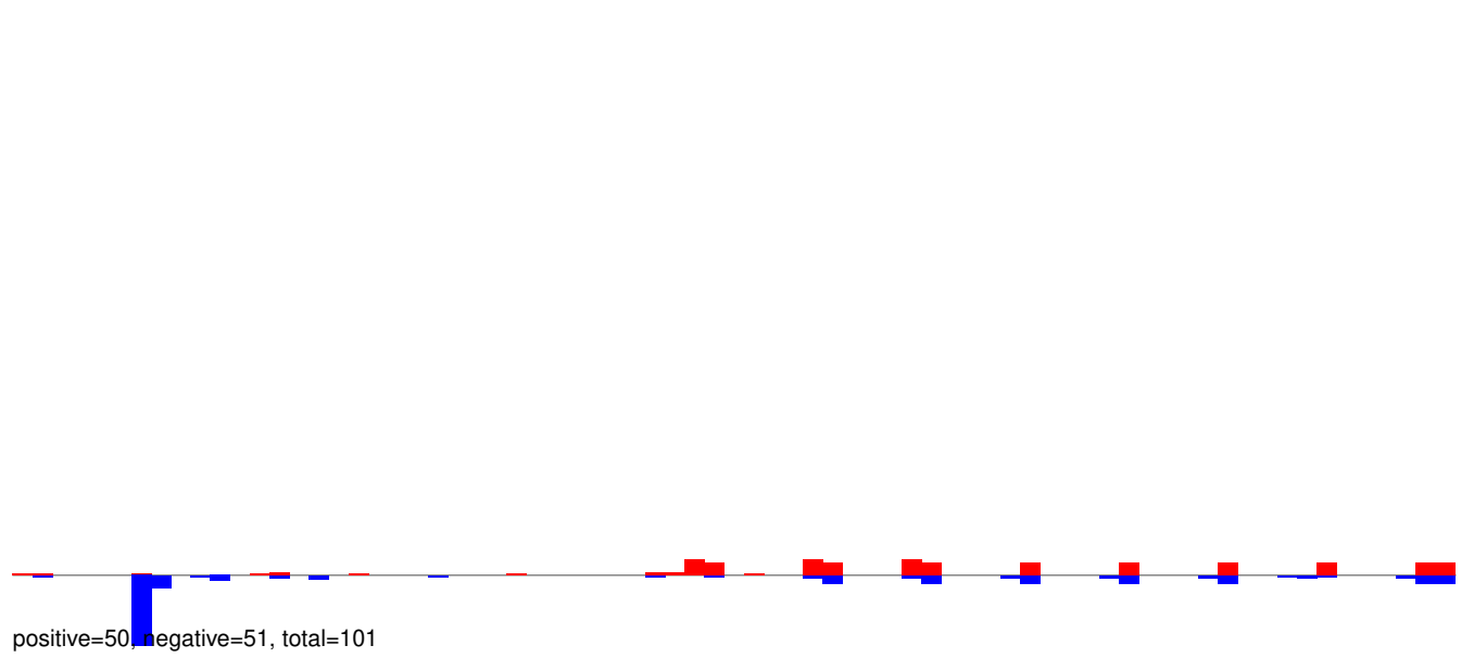
AeAeg_Aag2SINV_Ago3.IP.24_35.rep
