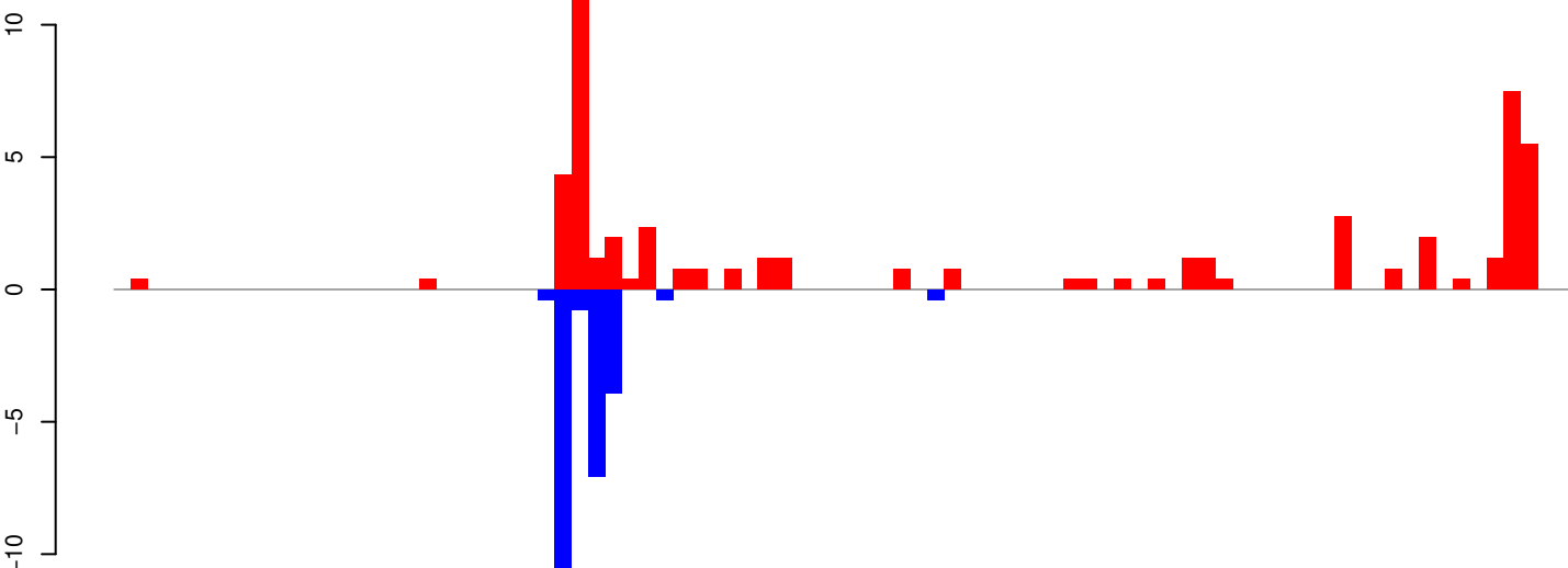
AeAeg_Aag2SINV_Ago3.IP.24_35.rep
