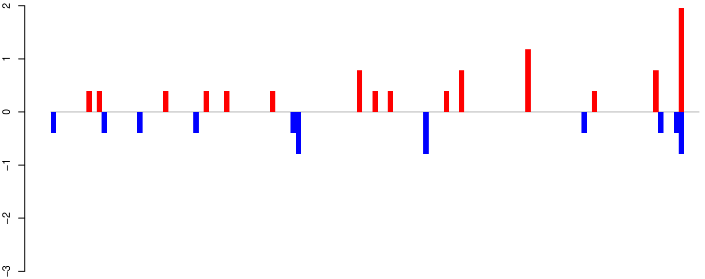
AeAeg_Aag2SINV_Ago3.IP.18_23.rep
