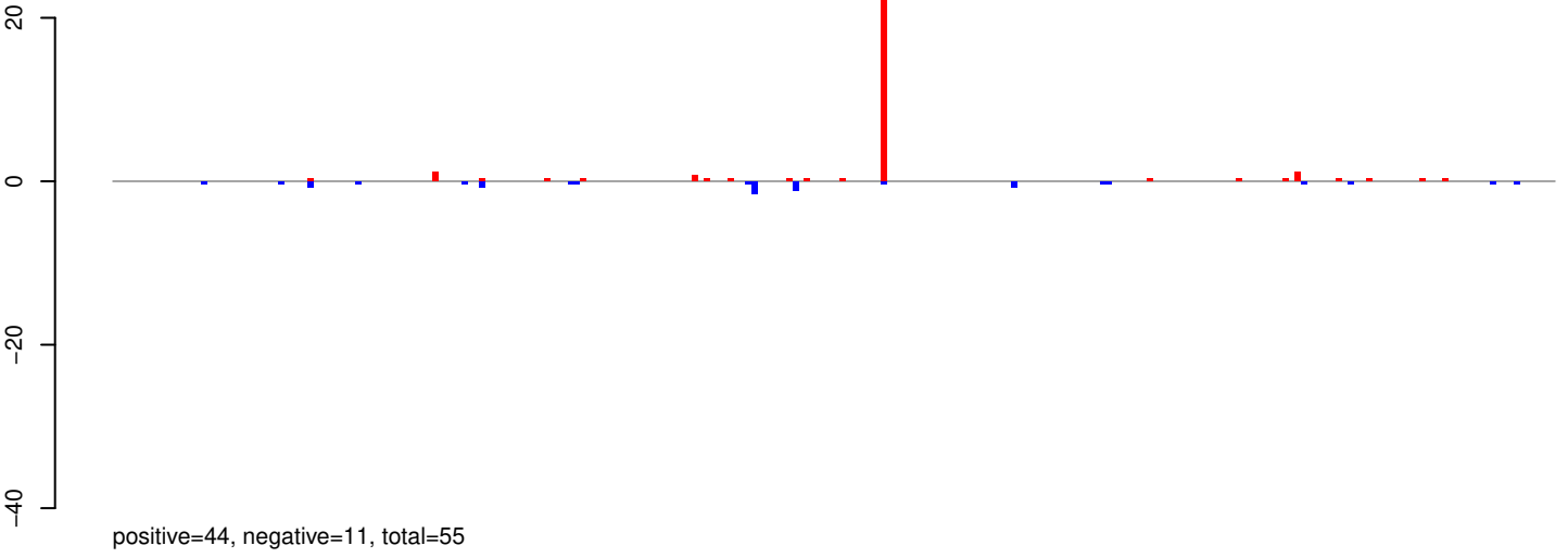
AeAeg_Aag2SINV_Ago3.IP.24_35.rep
