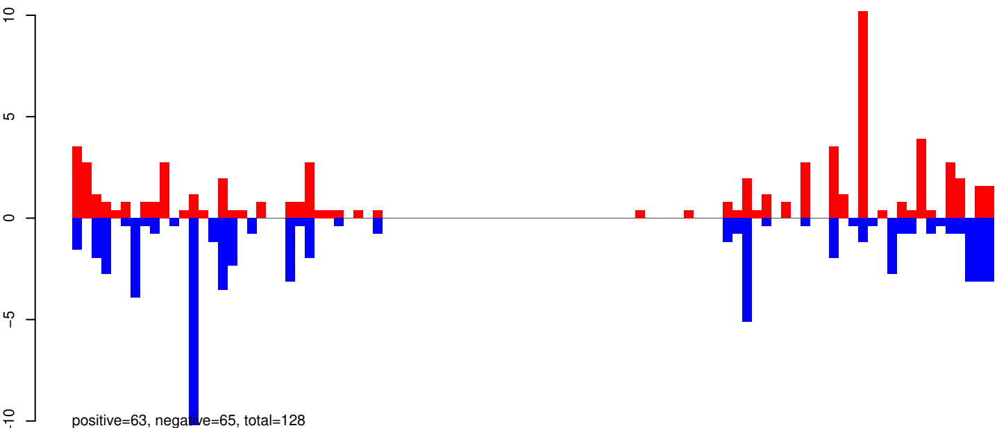
AeAeg_Aag2SINV_Ago3.IP.24_35.rep
