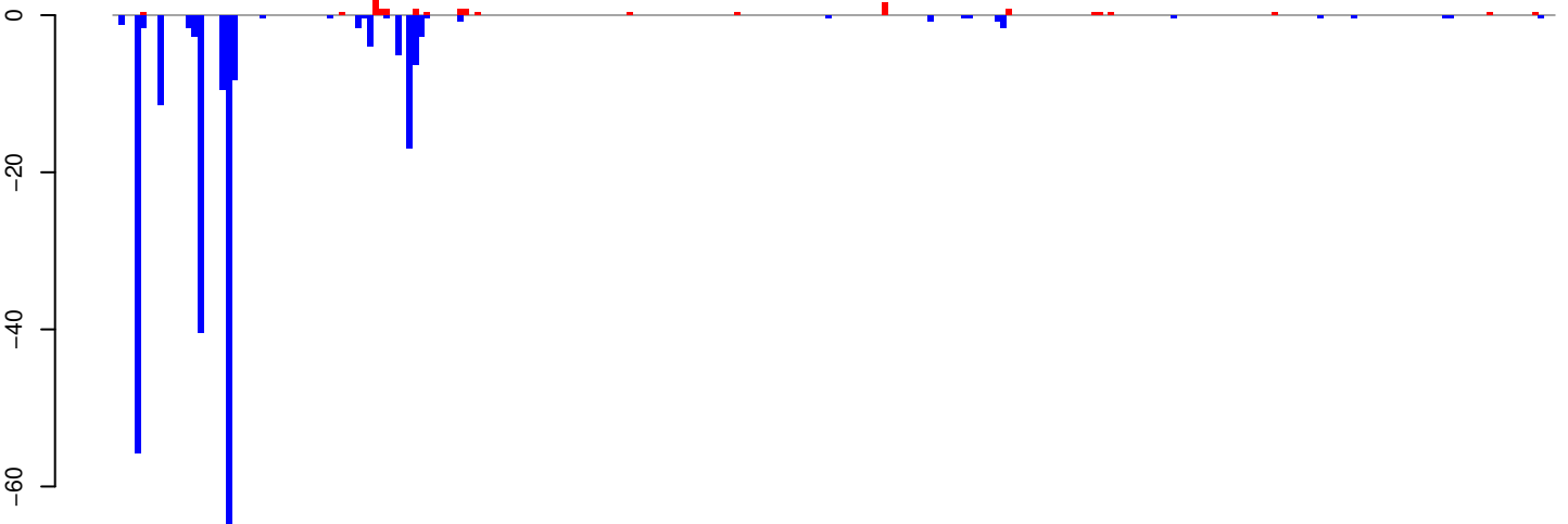
AeAeg_Aag2SINV_Ago3.IP.rep
