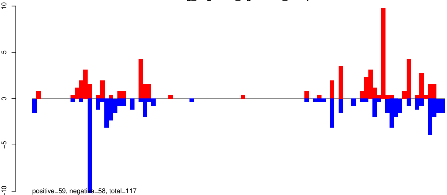
AeAeg_Aag2SINV_Ago3.IP.24_35.rep
