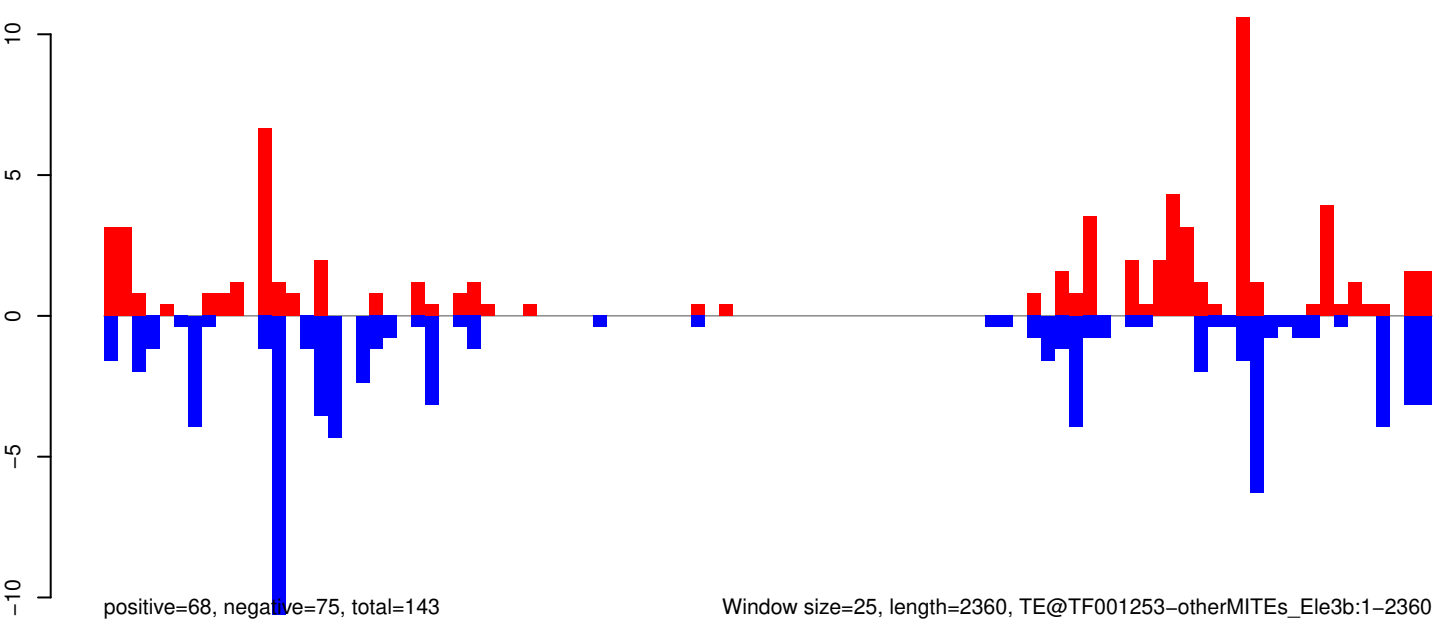
AeAeg_Aag2SINV_Ago3.IP.rep
