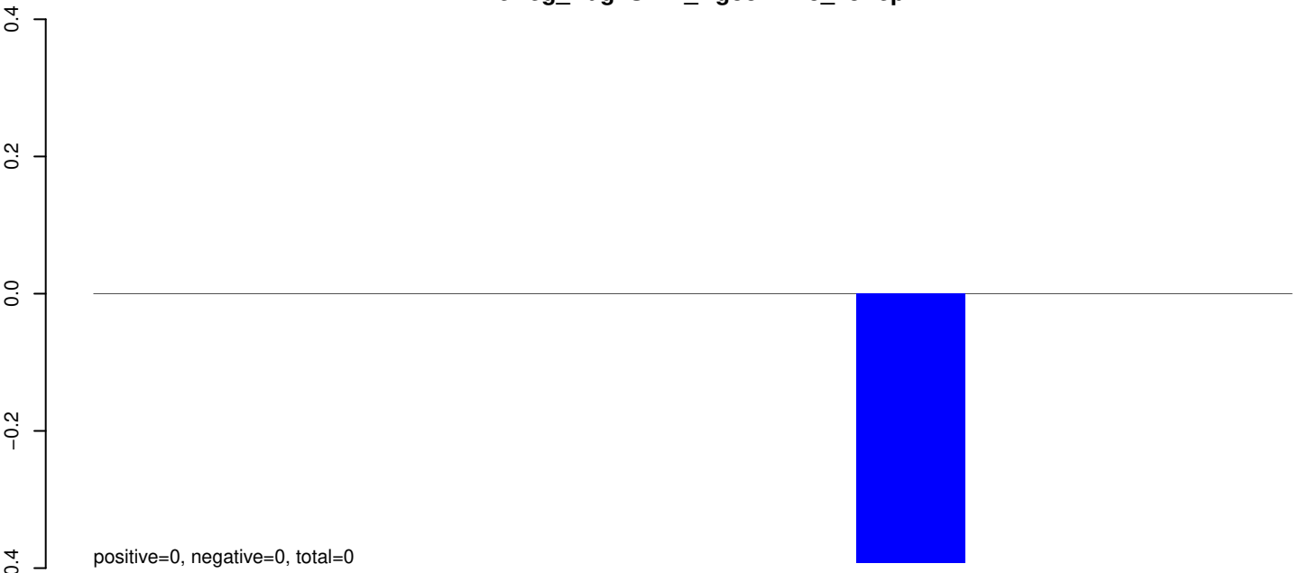
AeAeg_Aag2SINV_Ago3.IP.24_35.rep
