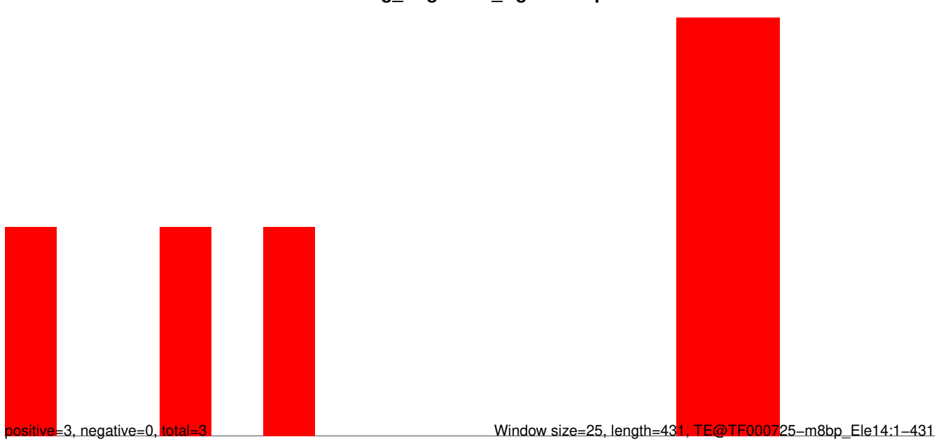
AeAeg_Aag2SINV_Ago3.IP.rep
