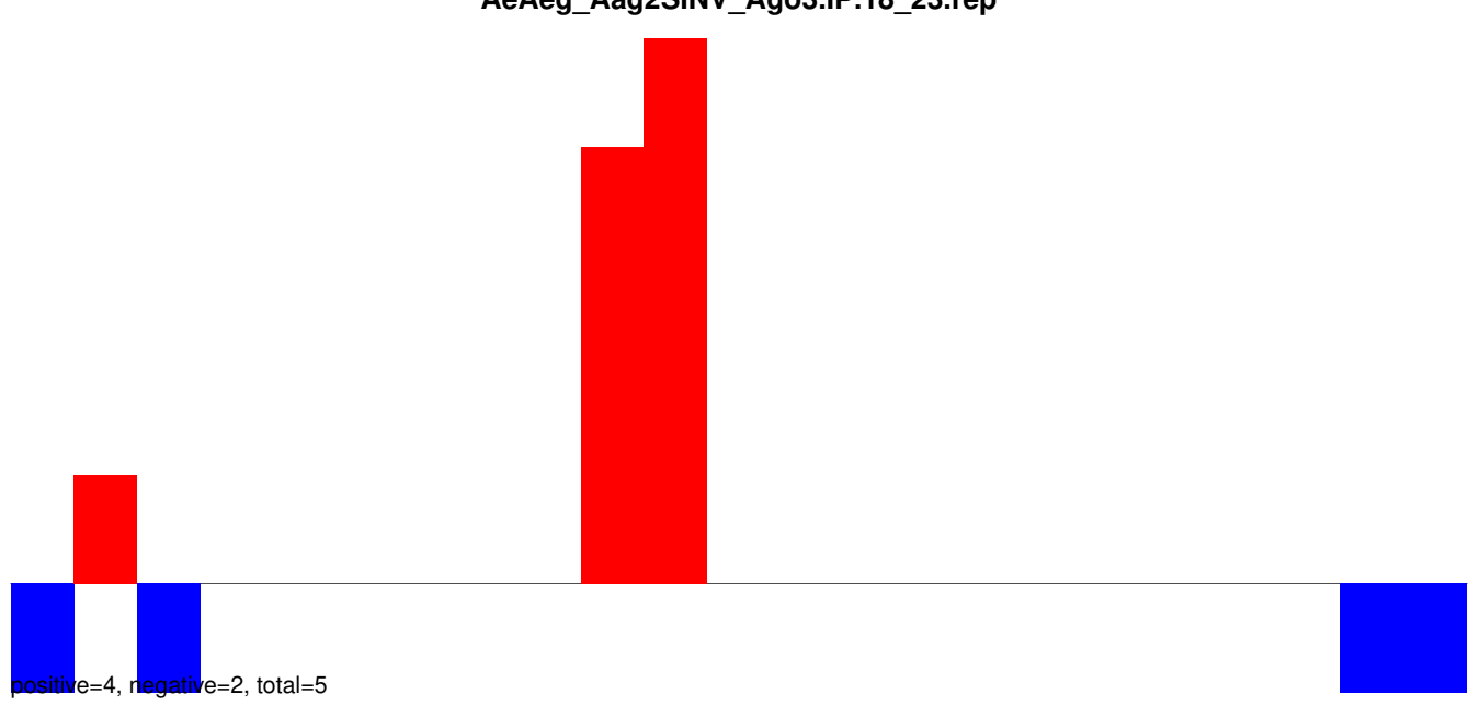
AeAeg_Aag2SINV_Ago3.IP.24_35.rep
