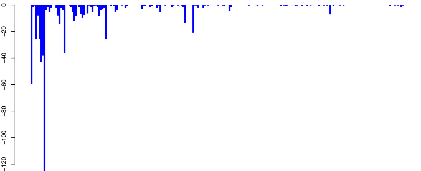
AeAeg_Aag2SINV_Ago3.IP.24_35.rep
