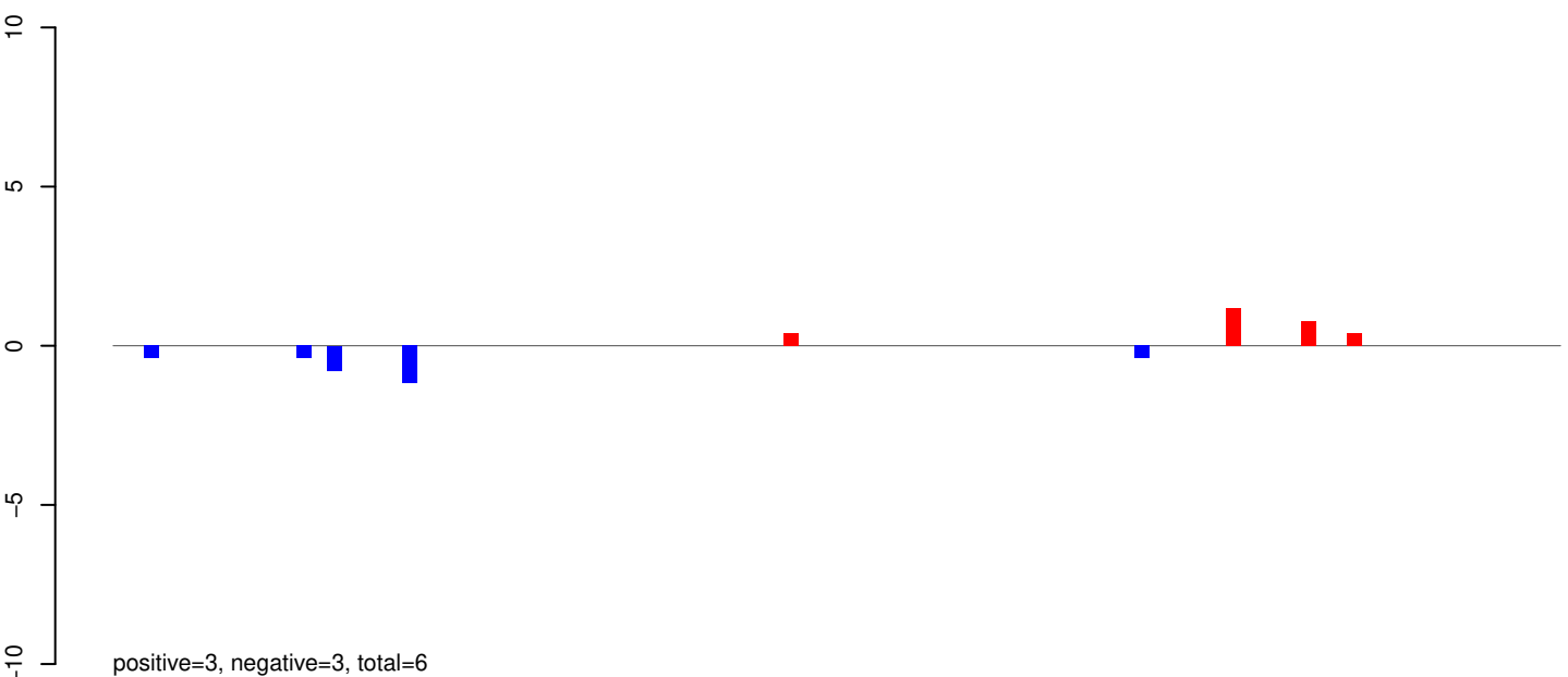
AeAeg_Aag2SINV_Ago3.IP.rep
