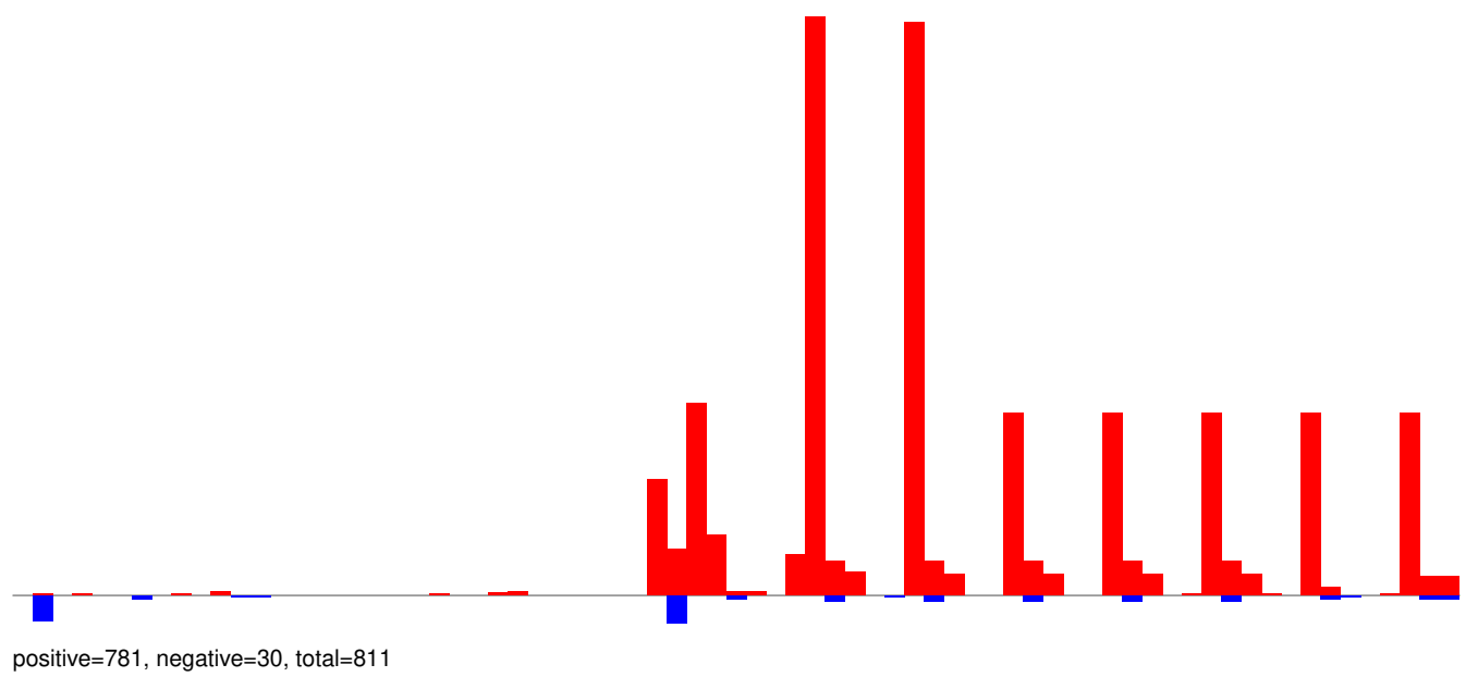
AeAeg_Aag2SINV_Ago3.IP.rep
