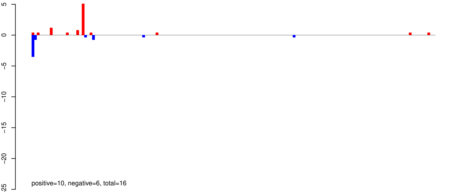
AeAeg_Aag2SINV_Ago3.IP.24_35.rep
