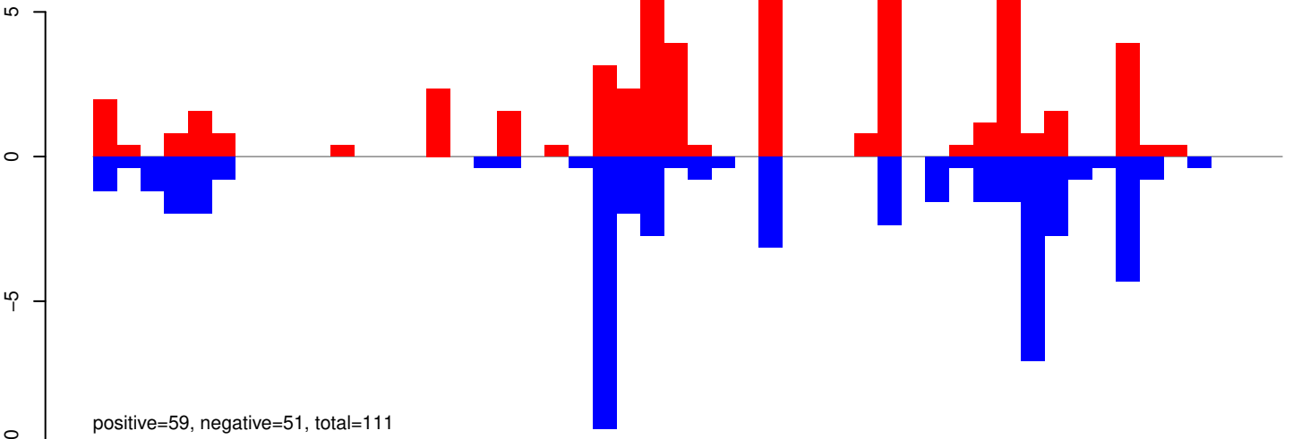
AeAeg_Aag2SINV_Ago3.IP.24_35.rep
