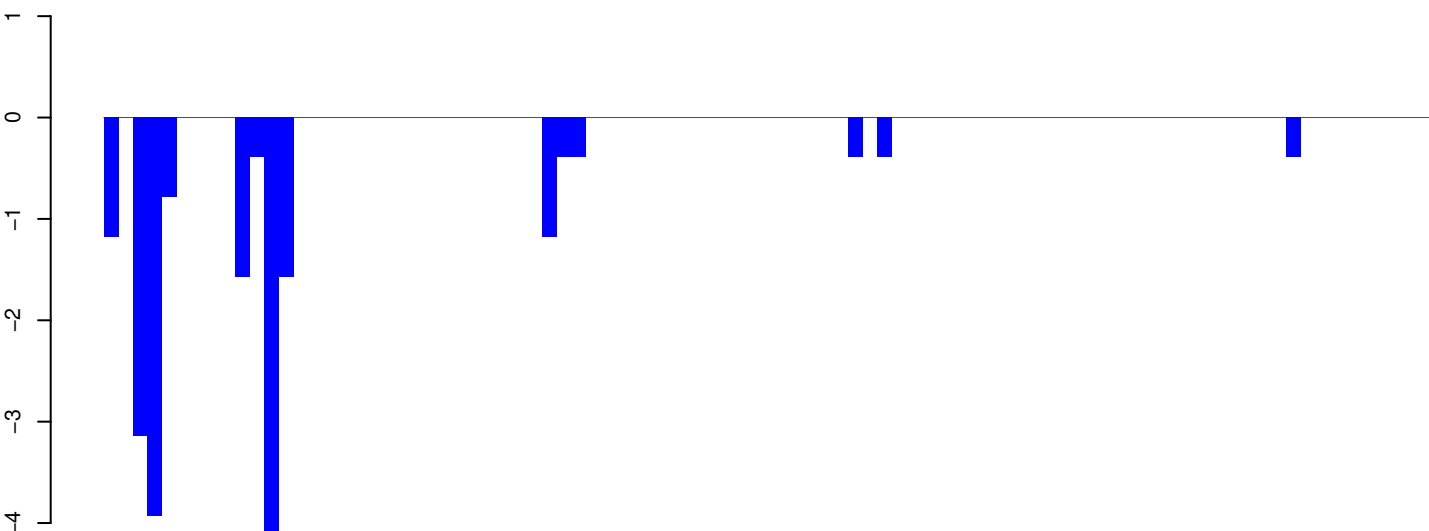
AeAeg_Aag2SINV_Ago3.IP.24_35.rep
