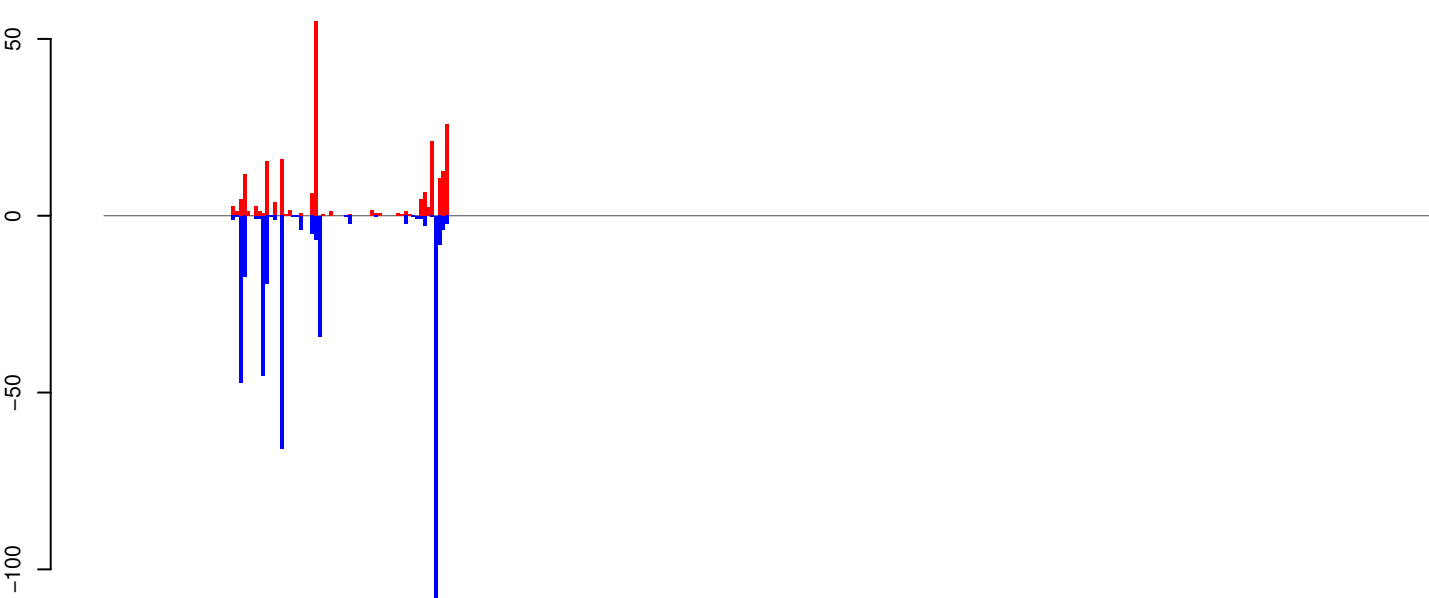
AeAeg_Aag2SINV_Ago3.IP.rep
