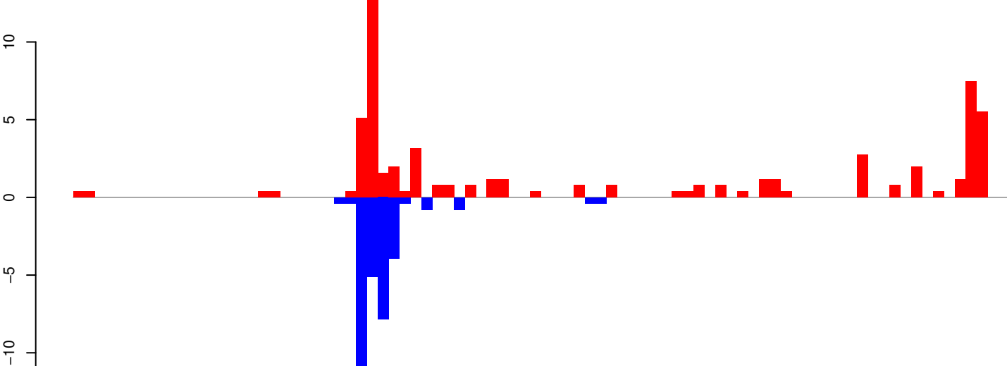
AeAeg_Aag2SINV_Ago3.IP.rep
