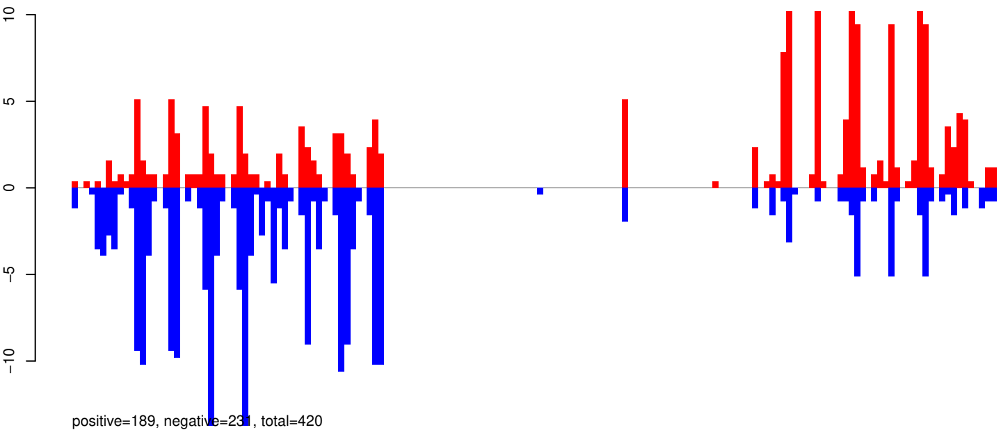
AeAeg_Aag2SINV_Ago3.IP.24_35.rep
