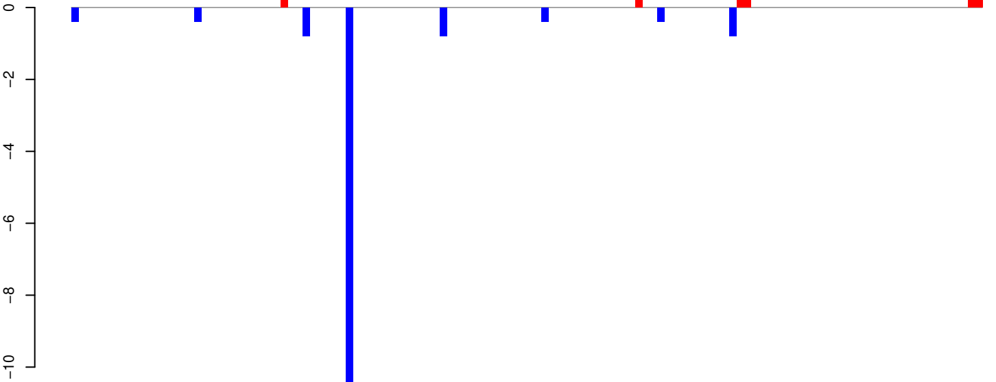
AeAeg_Aag2SINV_Ago3.IP.rep
