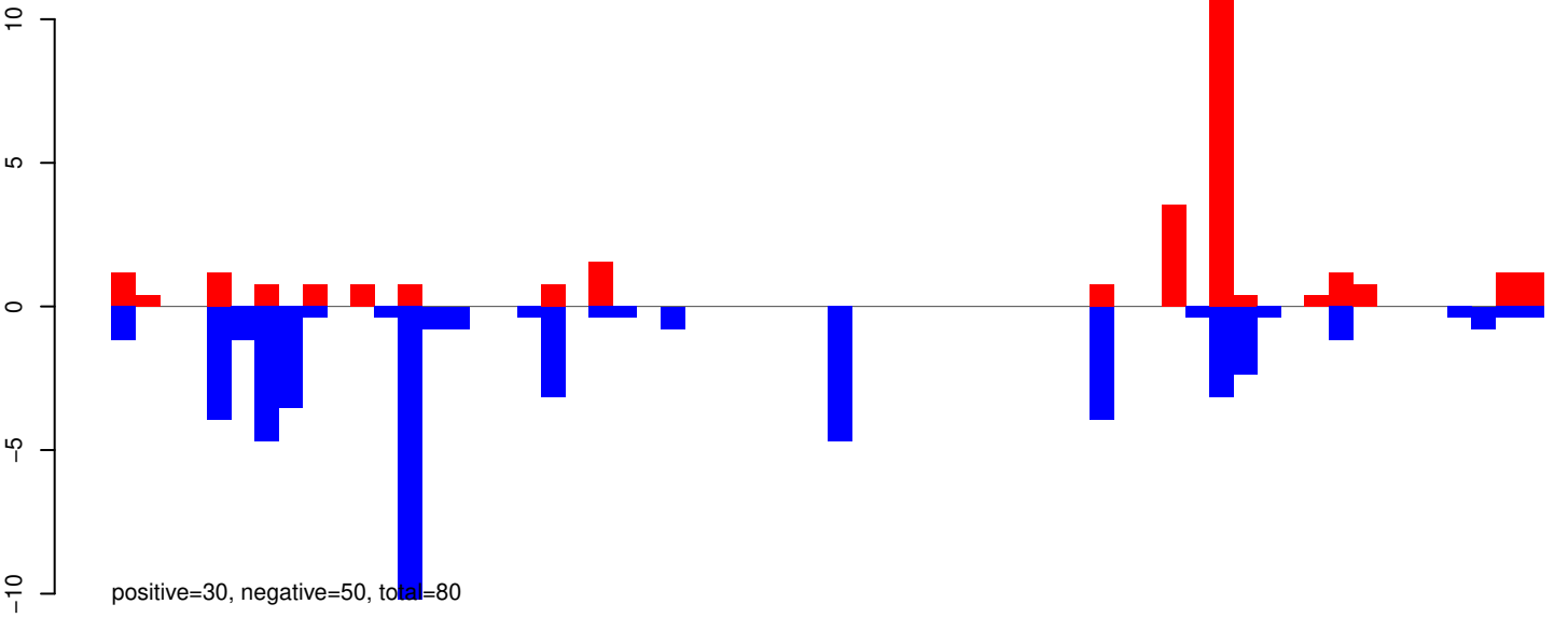
AeAeg_Aag2SINV_Ago3.IP.24_35.rep
