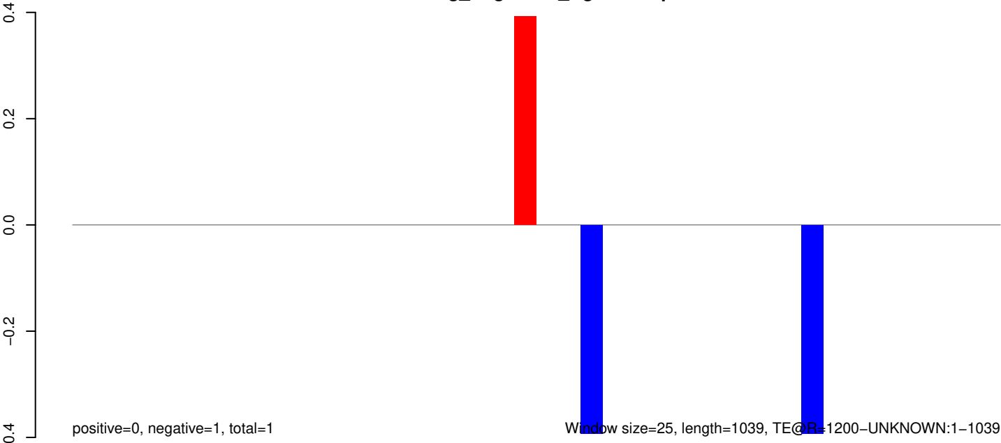
AeAeg_Aag2SINV_Ago3.IP.rep
