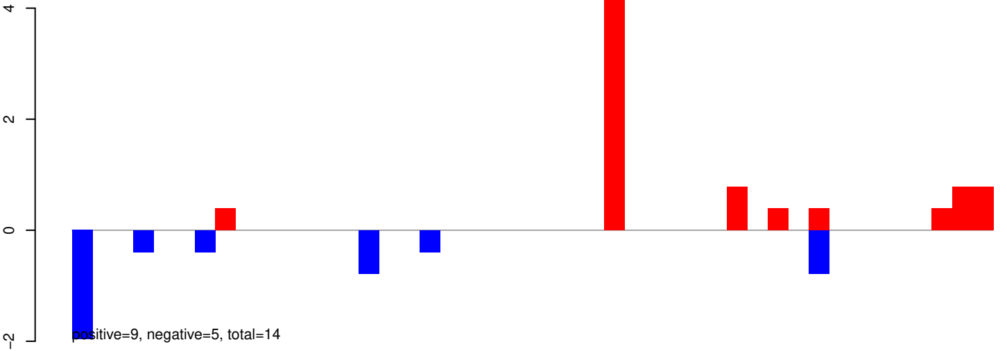
AeAeg_Aag2SINV_Ago3.IP.24_35.rep
