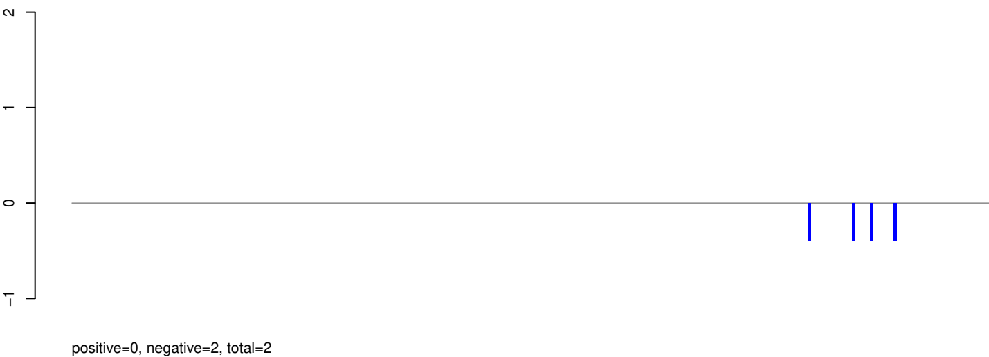
AeAeg_Aag2SINV_Ago3.IP.rep
