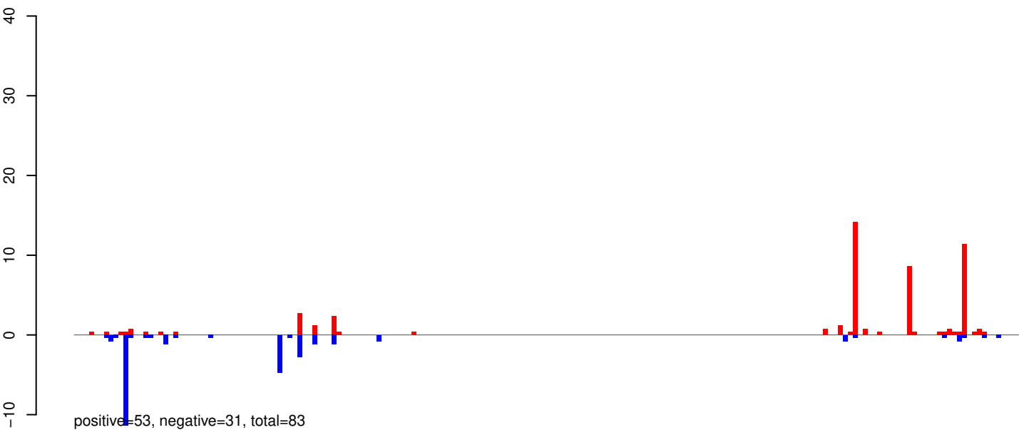
AeAeg_Aag2SINV_Ago3.IP.24_35.rep
