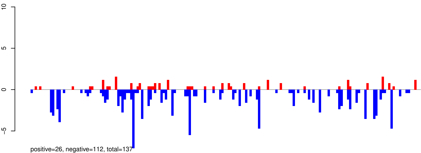
AeAeg_Aag2SINV_Ago3.IP.rep
