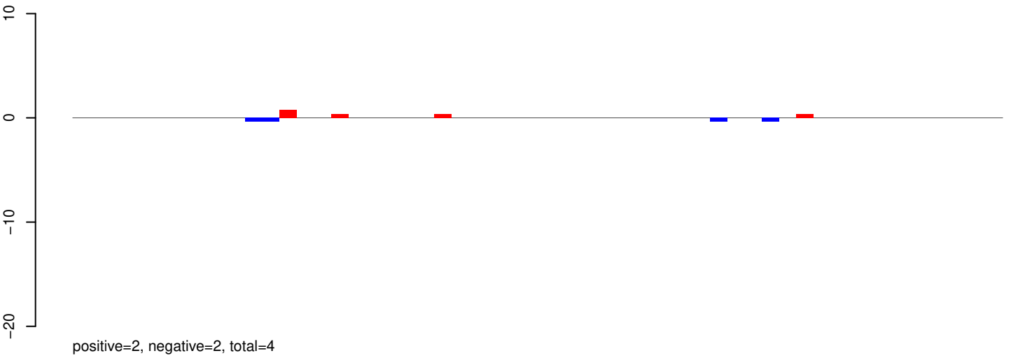
AeAeg_Aag2SINV_Ago3.IP.rep
