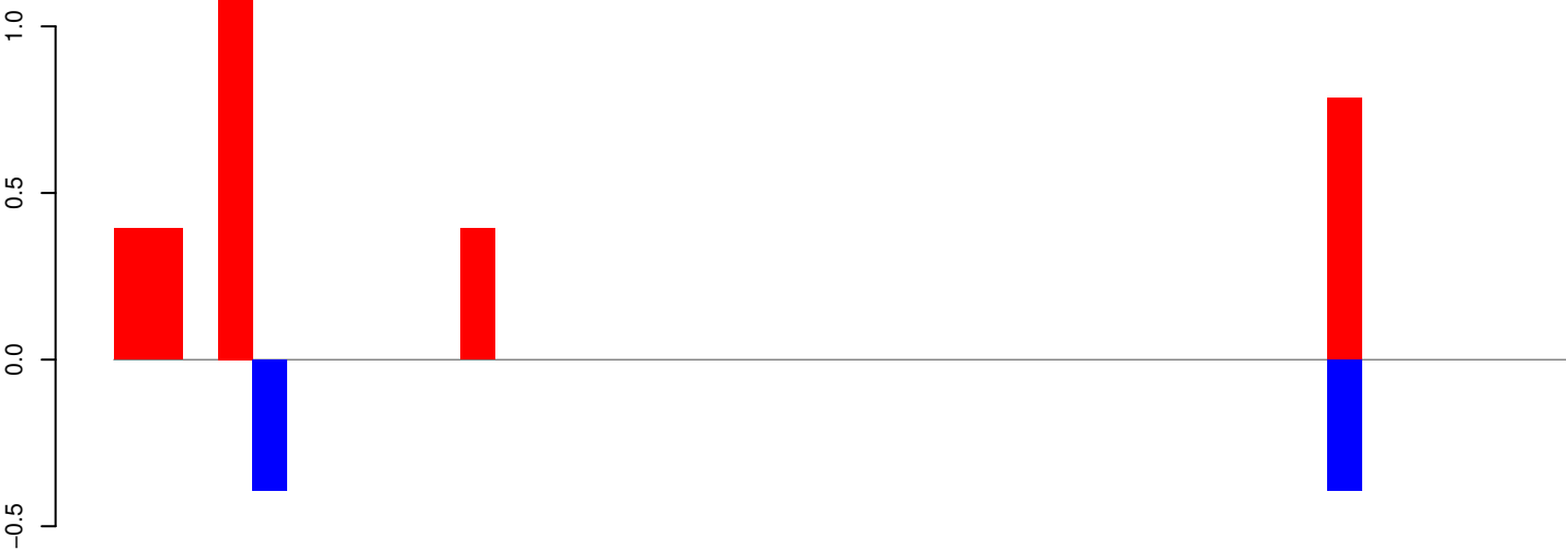
AeAeg_Aag2SINV_Ago3.IP.18_23.rep
