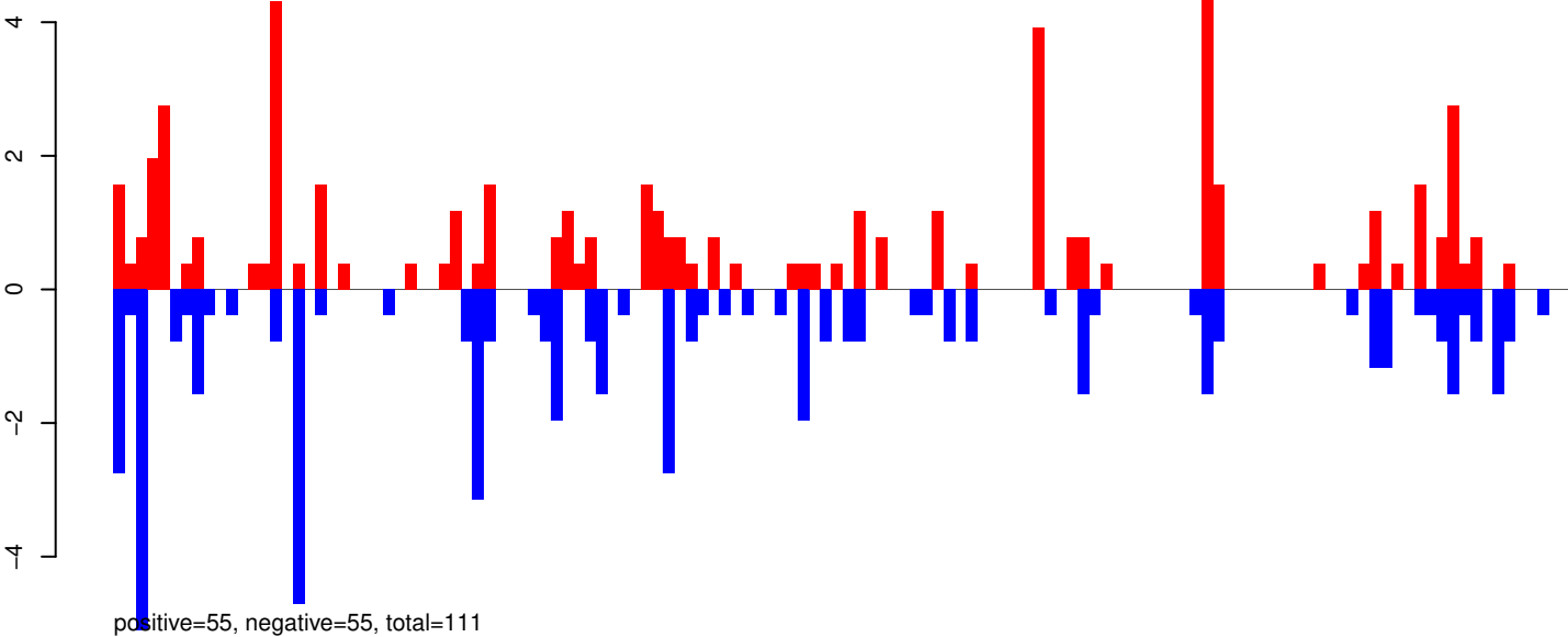
AeAeg_Aag2SINV_Ago3.IP.24_35.rep
