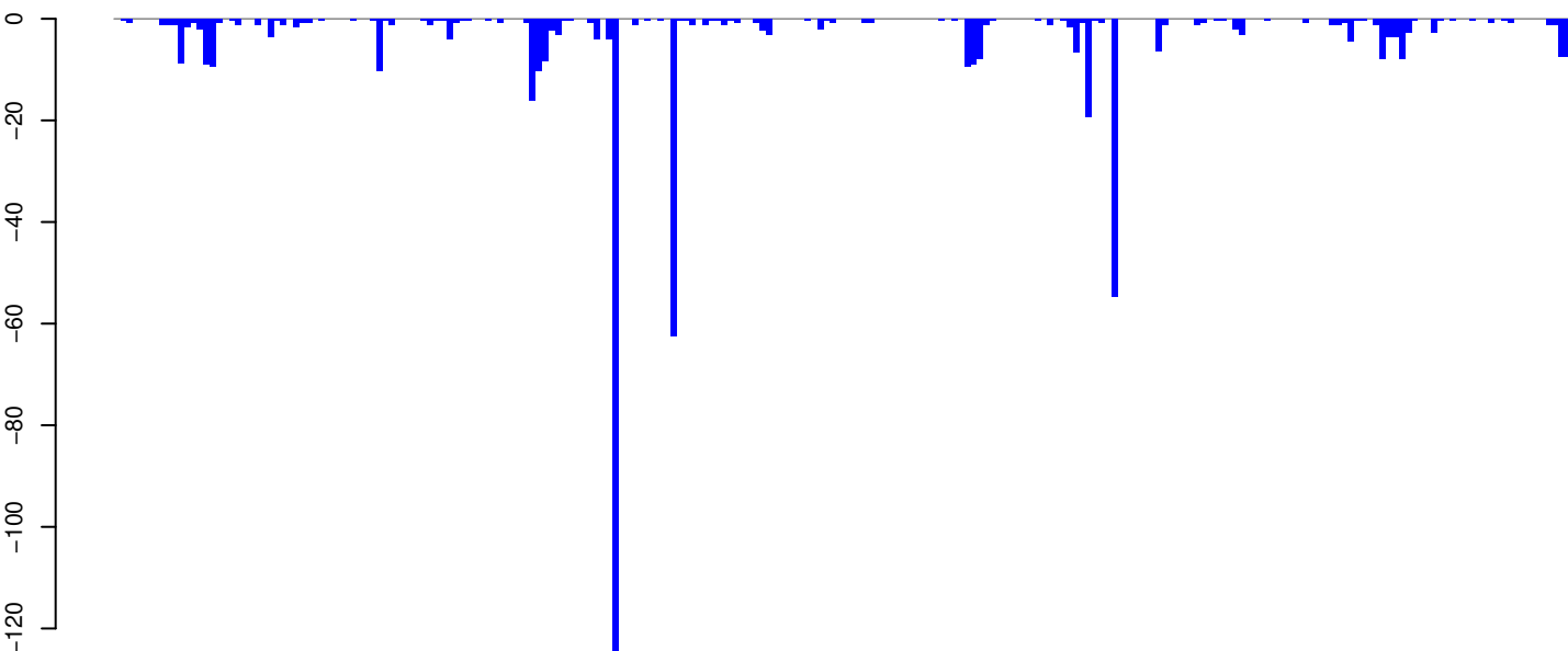
AeAeg_Aag2SINV_Ago3.IP.24_35.rep
