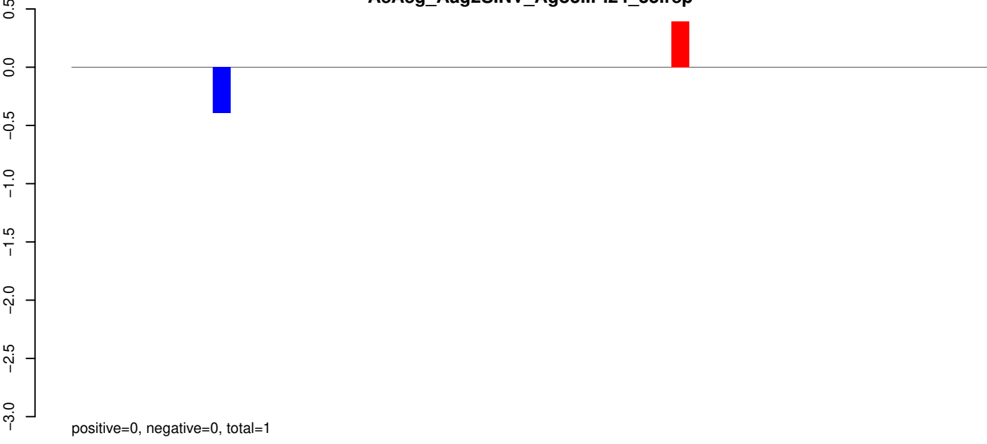
AeAeg_Aag2SINV_Ago3.IP.rep
