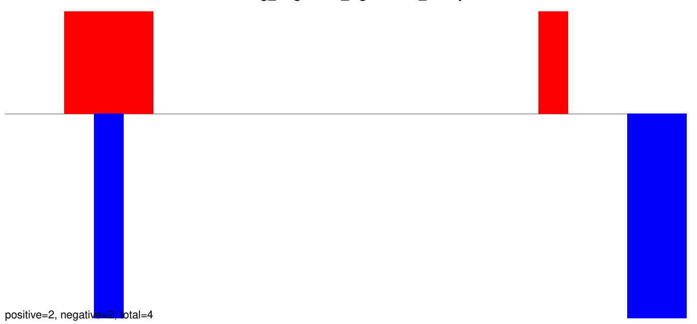
AeAeg_Aag2SINV_Ago3.IP.24_35.rep
