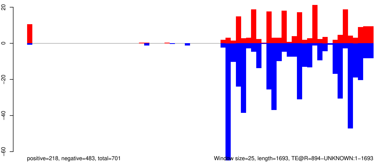
AeAeg_Aag2SINV_Ago3.IP.rep
