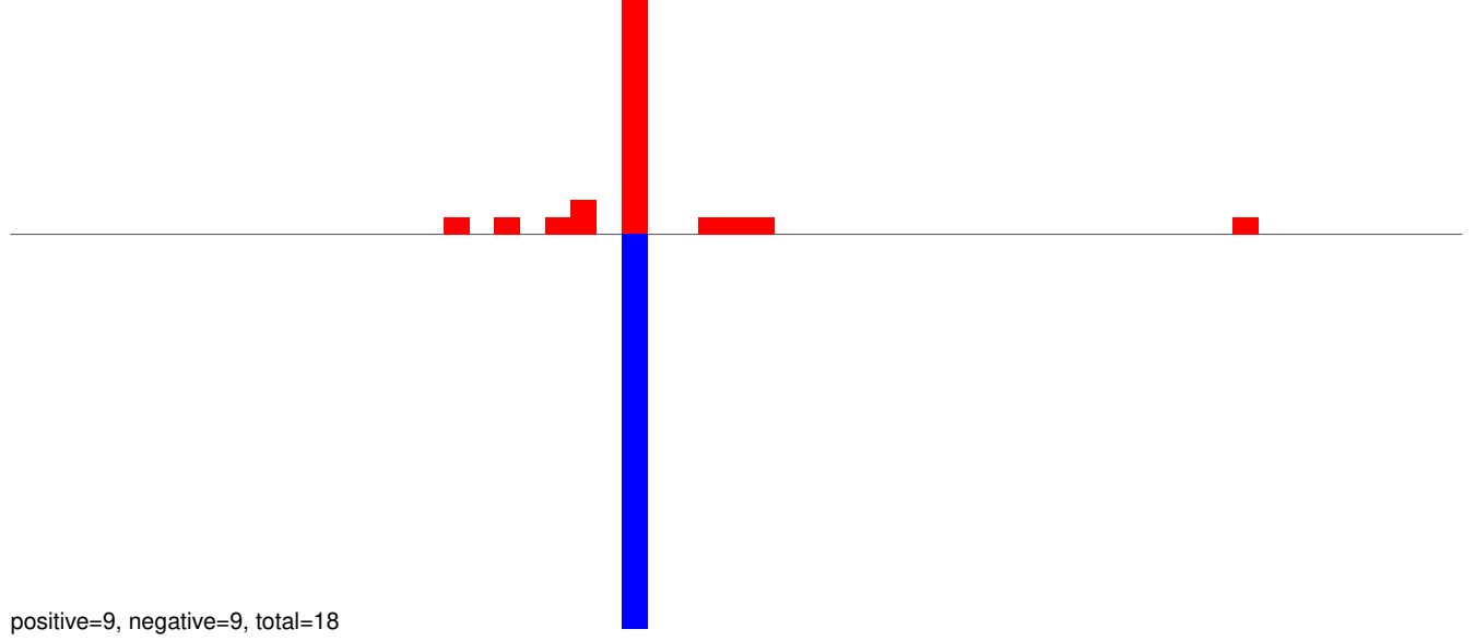
AeAeg_Aag2SINV_Ago3.IP.24_35.rep
