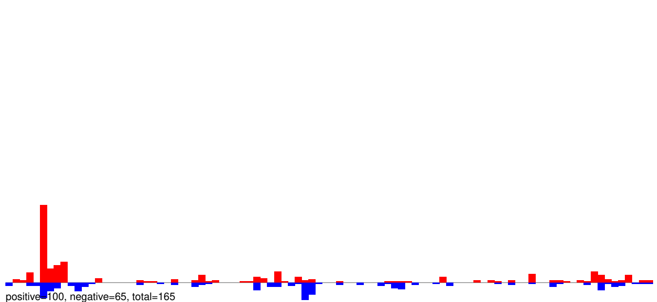
AeAeg_Aag2SINV_Ago3.IP.24_35.rep
