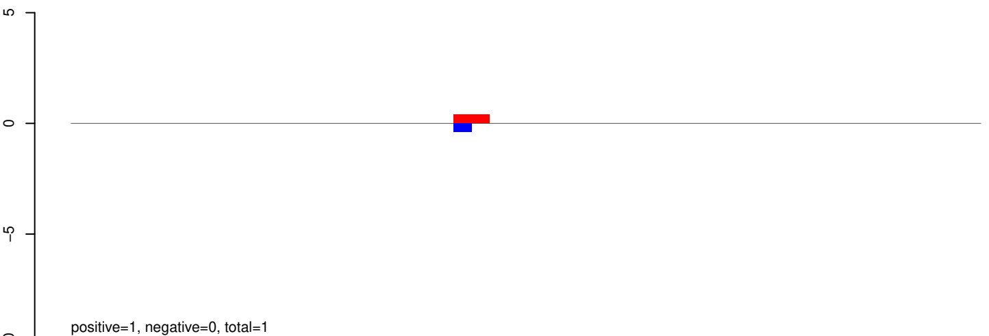
AeAeg_Aag2SINV_Ago3.IP.rep
