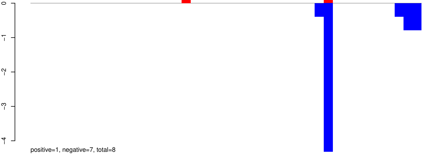
AeAeg_Aag2SINV_Ago3.IP.24_35.rep
