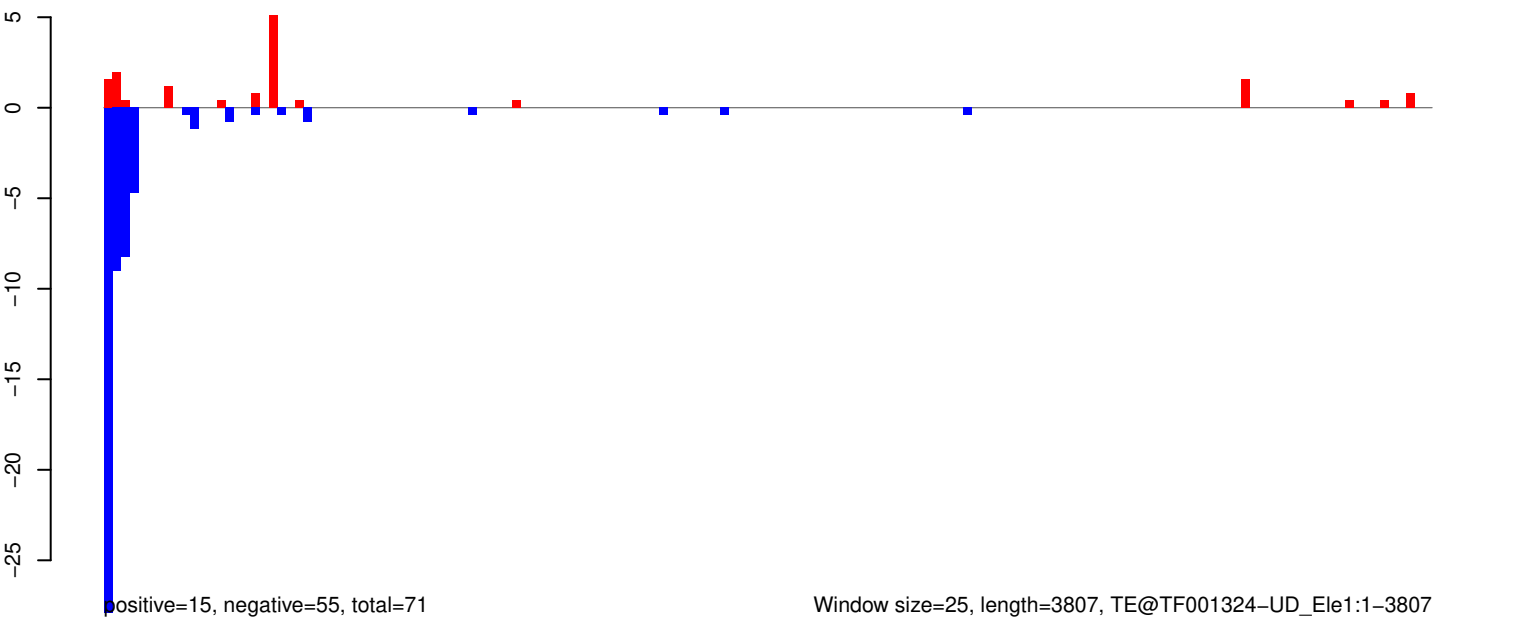
AeAeg_Aag2SINV_Ago3.IP.rep
