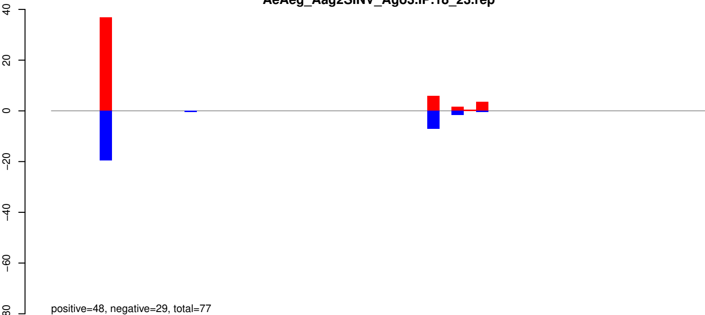
AeAeg_Aag2SINV_Ago3.IP.24_35.rep
