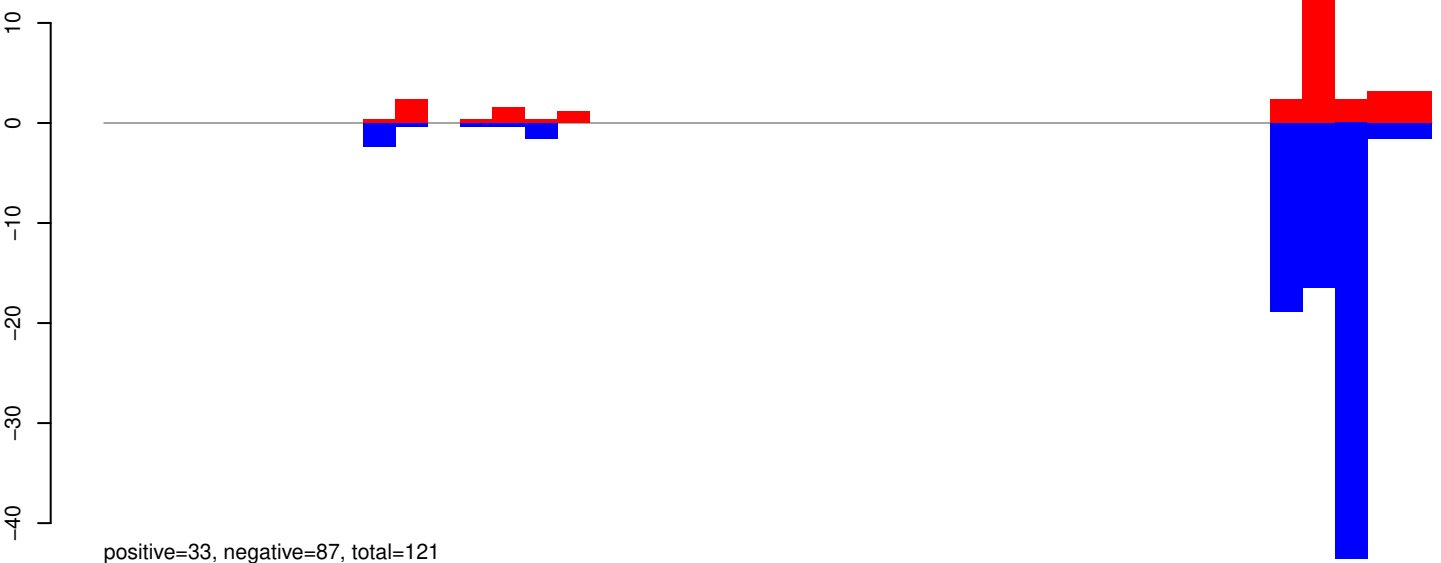
AeAeg_Aag2SINV_Ago3.IP.24_35.rep
