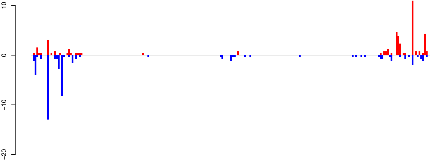
AeAeg_Aag2SINV_Ago3.IP.18_23.rep
