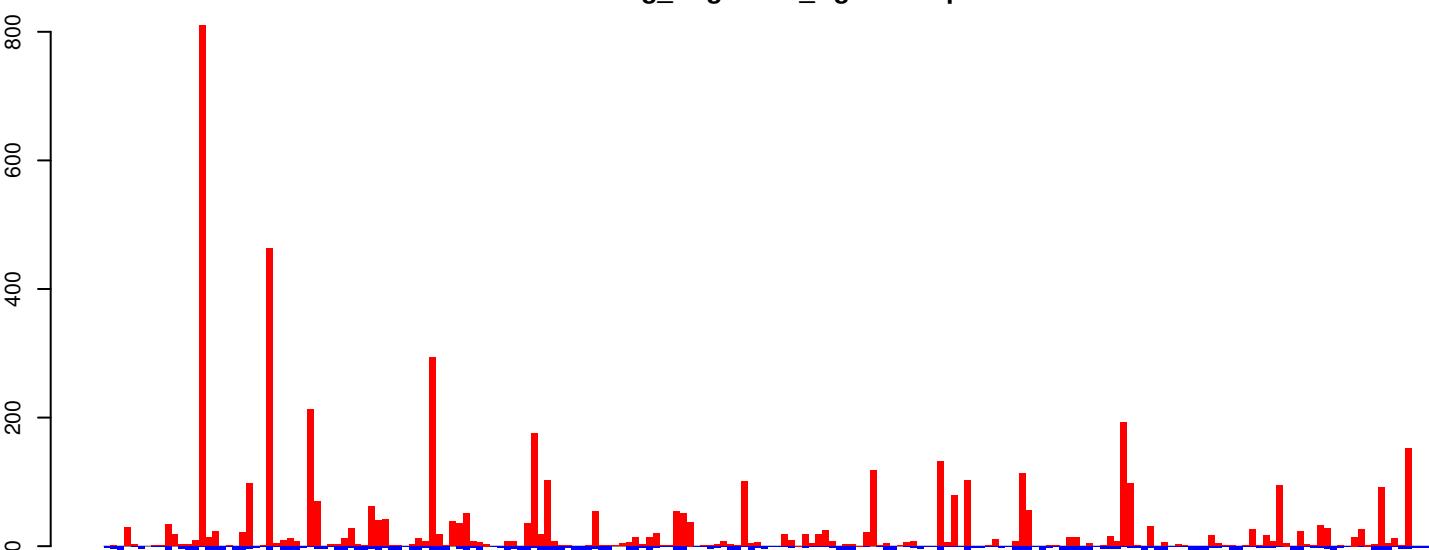
AeAeg_Aag2SINV_Ago3.IP.rep
