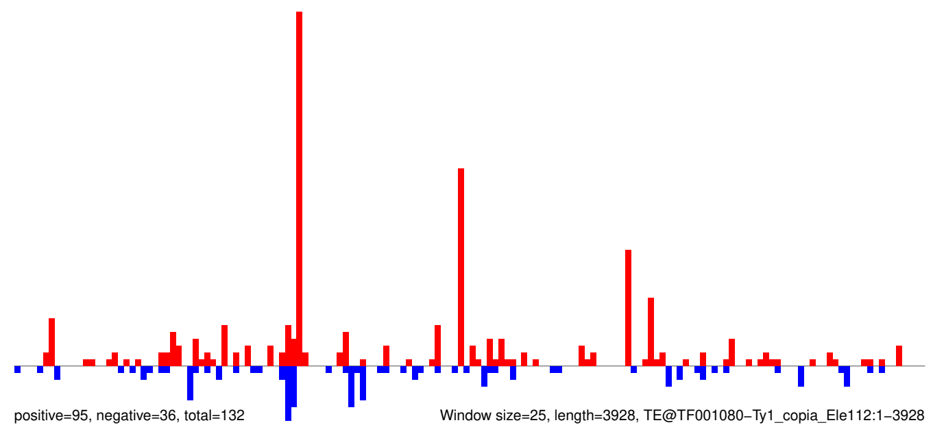
AeAeg_Aag2SINV_Ago3.IP.rep
