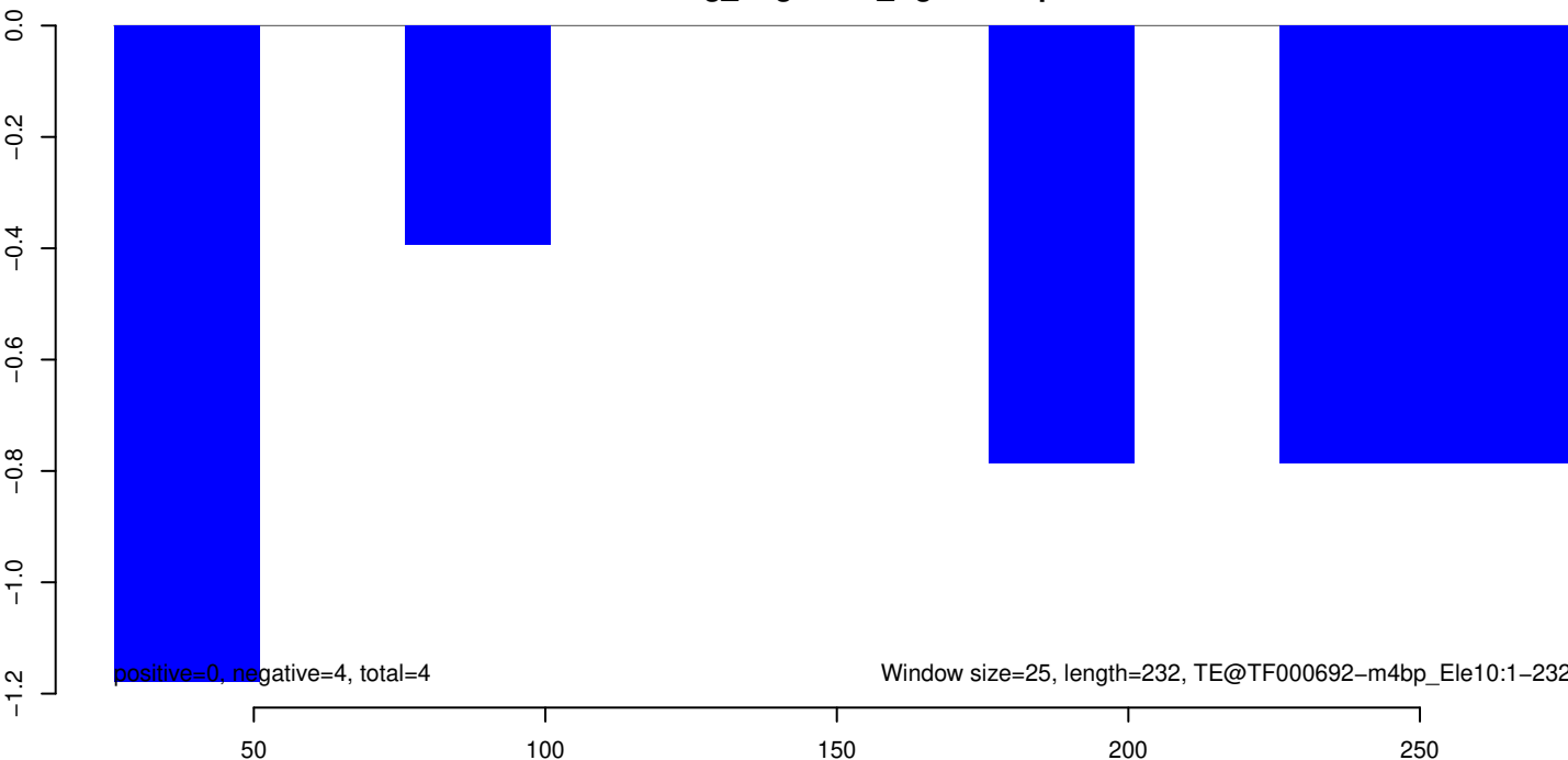
AeAeg_Aag2SINV_Ago3.IP.rep
