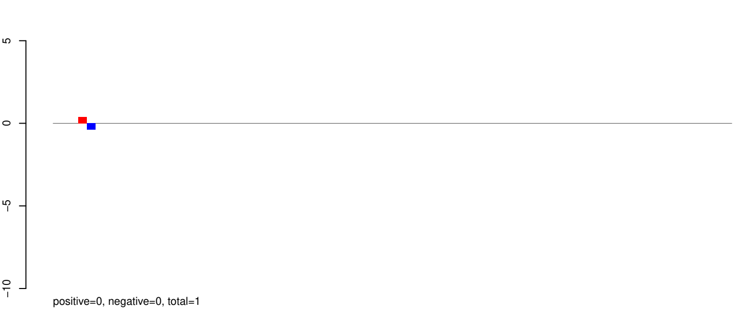
AeAeg_Aag2SINV_Ago3.IP.rep
