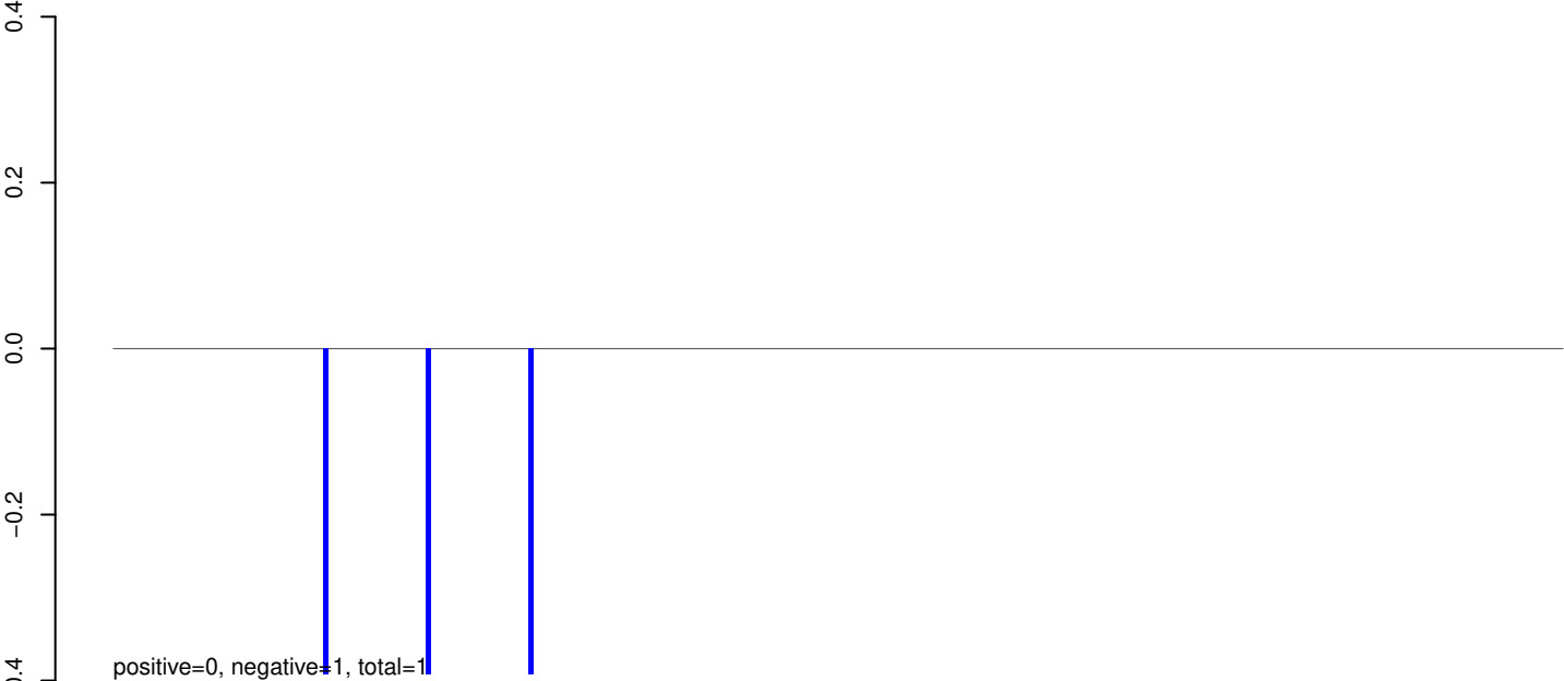
AeAeg_Aag2SINV_Ago3.IP.24_35.rep
