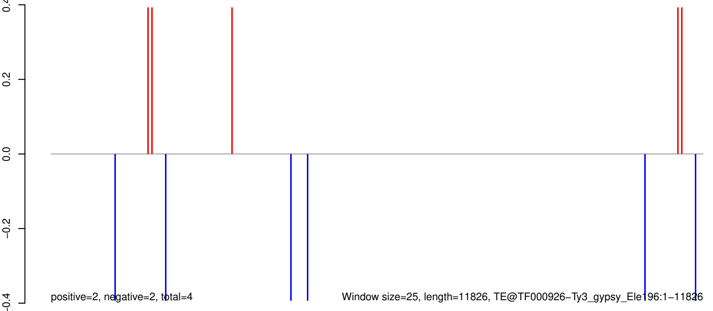
AeAeg_Aag2SINV_Ago3.IP.rep
