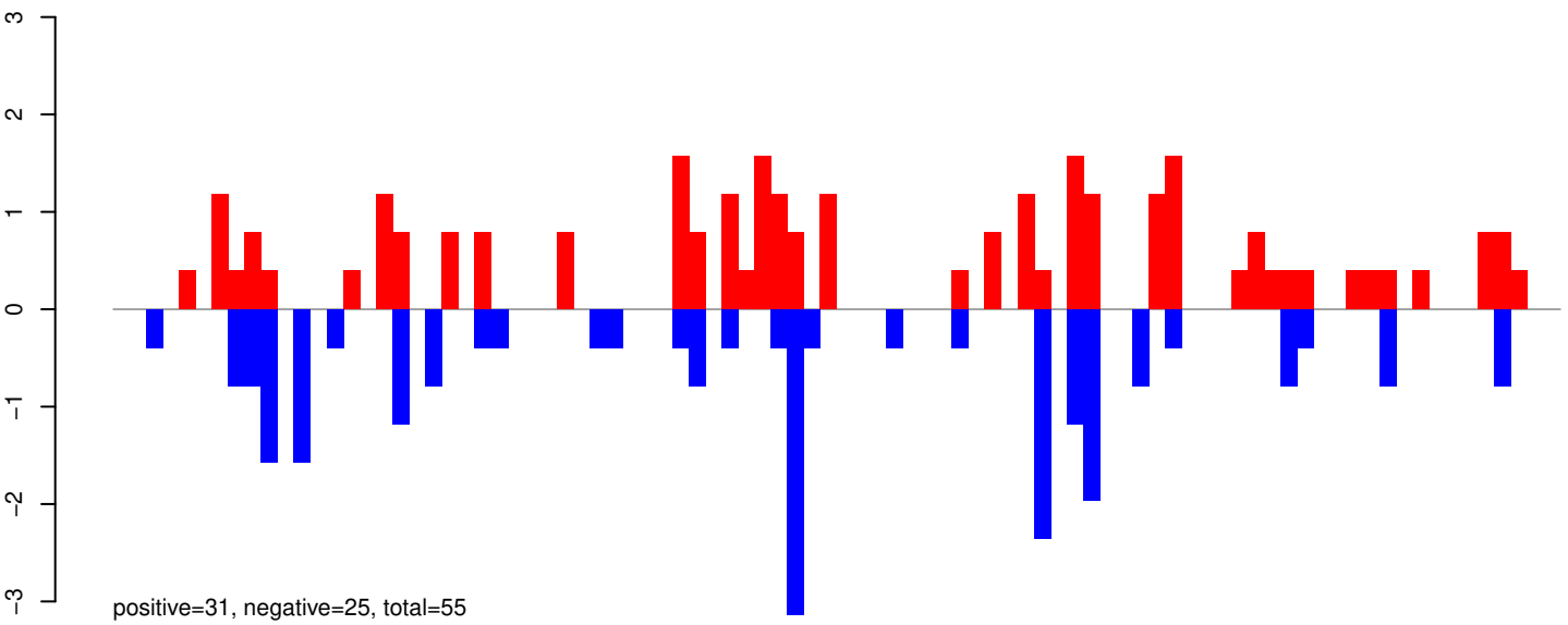
AeAeg_Aag2SINV_Ago3.IP.24_35.rep
