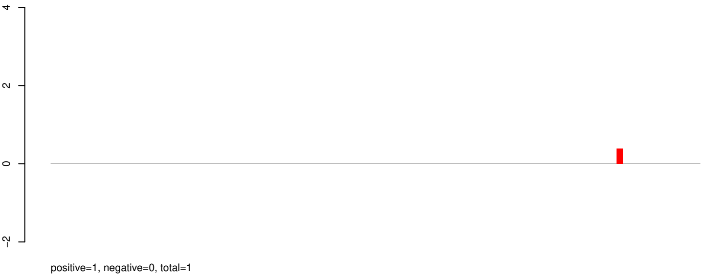
AeAeg_Aag2SINV_Ago3.IP.rep
