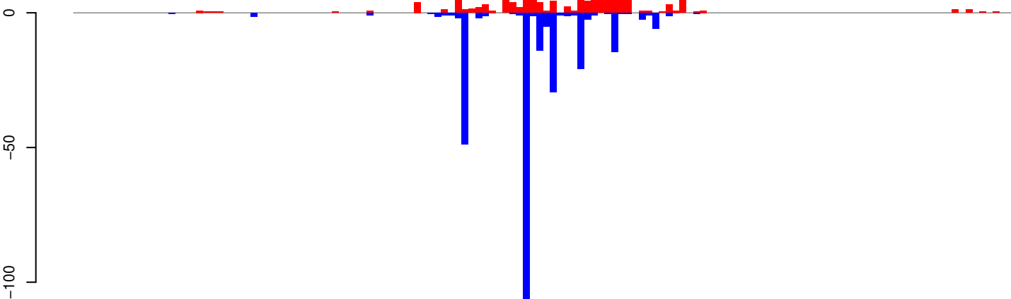
AeAeg_Aag2SINV_Ago3.IP.rep
