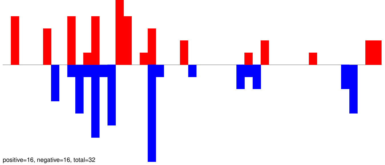
AeAeg_Aag2SINV_Ago3.IP.24_35.rep
