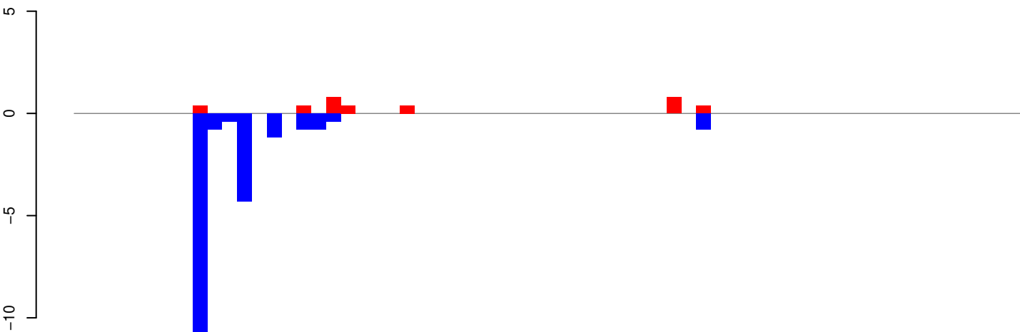
AeAeg_Aag2SINV_Ago3.IP.rep
