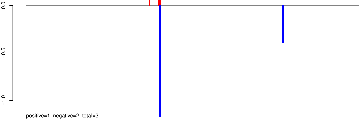
AeAeg_Aag2SINV_Ago3.IP.24_35.rep
