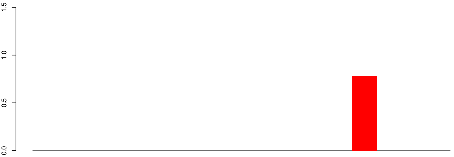
AeAeg_Aag2SINV_Ago3.IP.18_23.rep
