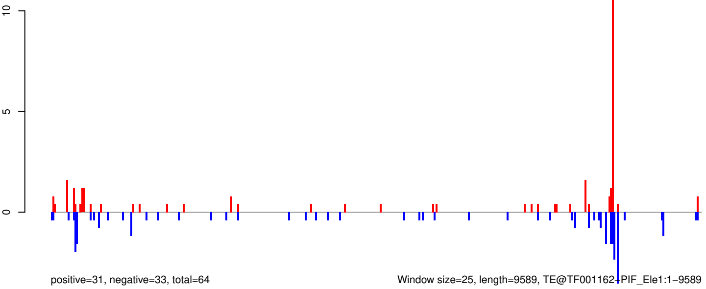
AeAeg_Aag2SINV_Ago3.IP.rep
