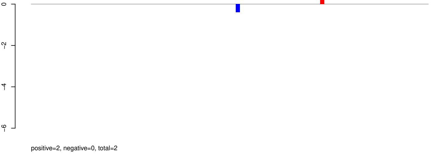
AeAeg_Aag2SINV_Ago3.IP.rep
