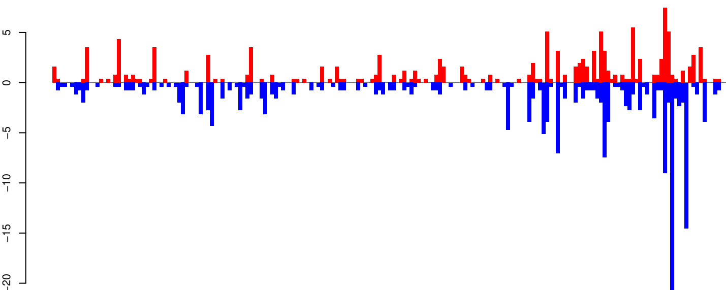
AeAeg_Aag2SINV_Ago3.IP.rep
