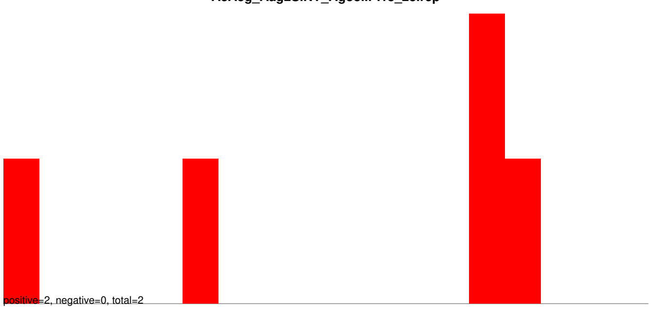
AeAeg_Aag2SINV_Ago3.IP.24_35.rep
