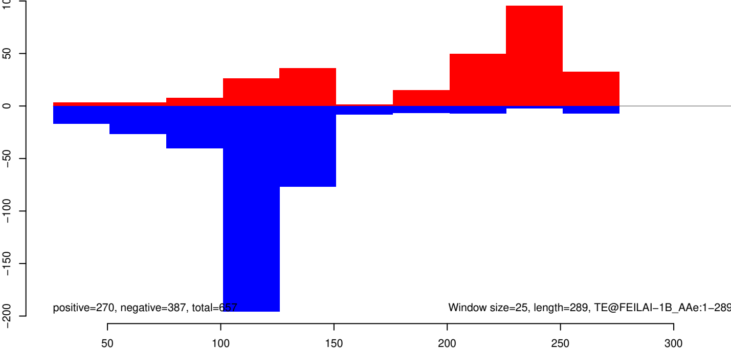
AeAeg_Aag2SINV_Ago3.IP.rep
