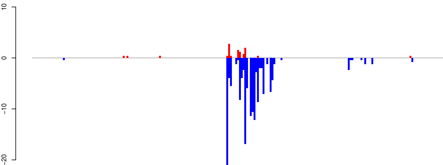
AeAeg_Aag2SINV_Ago3.IP.24_35.rep
