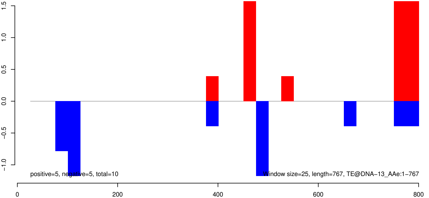
AeAeg_Aag2SINV_Ago3.IP.rep
