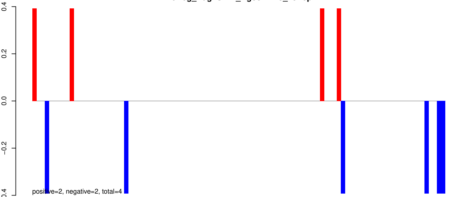
AeAeg_Aag2SINV_Ago3.IP.24_35.rep
