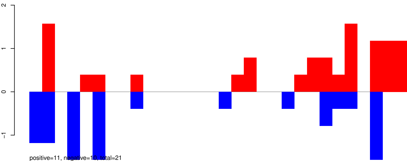
AeAeg_Aag2SINV_Ago3.IP.24_35.rep
