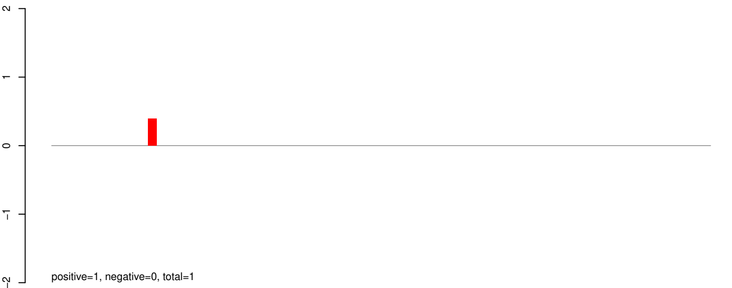
AeAeg_Aag2SINV_Ago3.IP.rep
