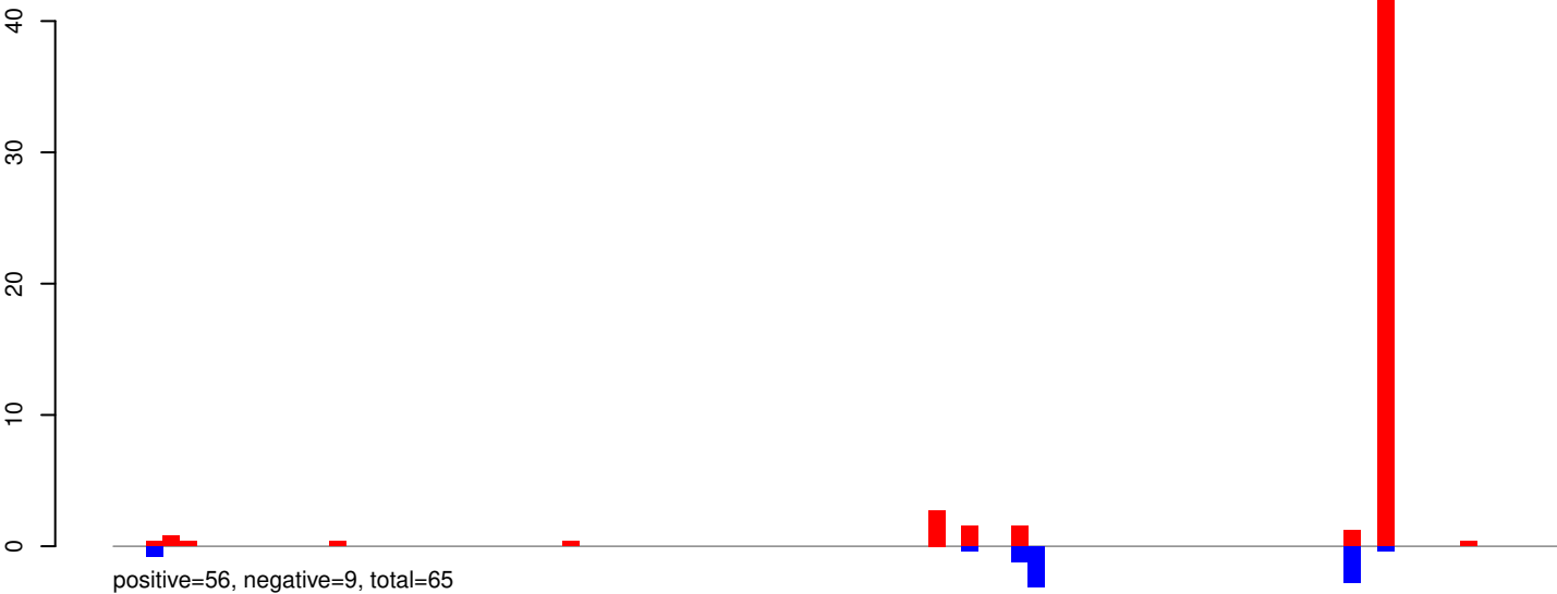
AeAeg_Aag2SINV_Ago3.IP.24_35.rep
