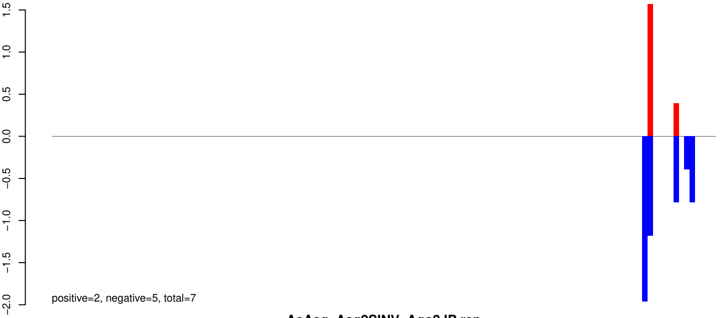
AeAeg_Aag2SINV_Ago3.IP.rep
