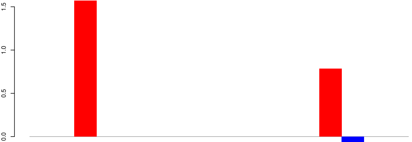
AeAeg_Aag2SINV_Ago3.IP.rep
