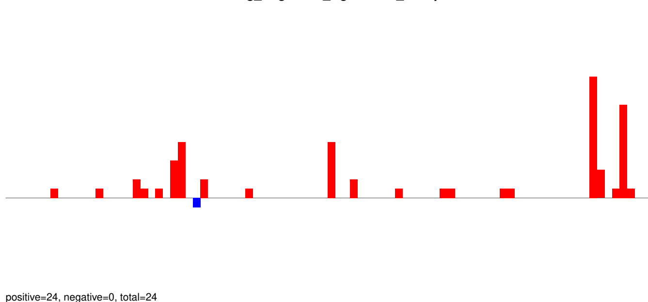
AeAeg_Aag2SINV_Ago3.IP.rep
