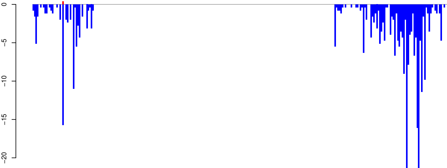
AeAeg_Aag2SINV_Ago3.IP.rep
