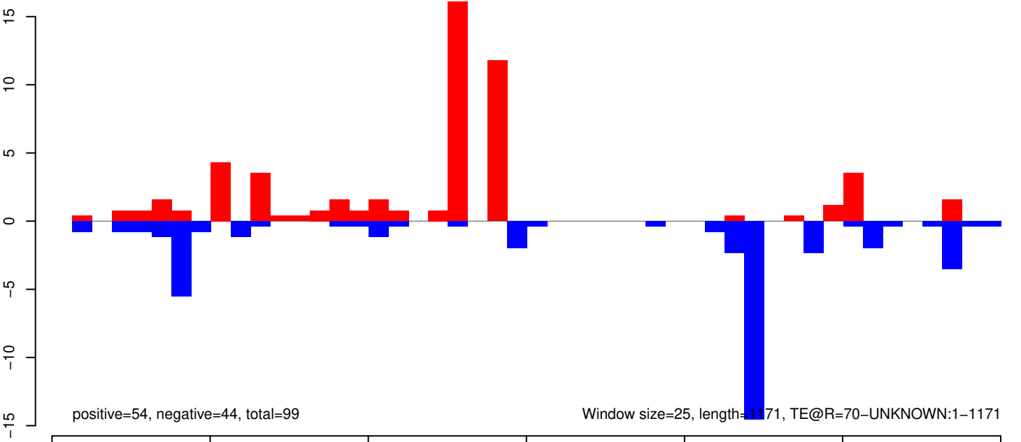
AeAeg_Aag2SINV_Ago3.IP.rep
