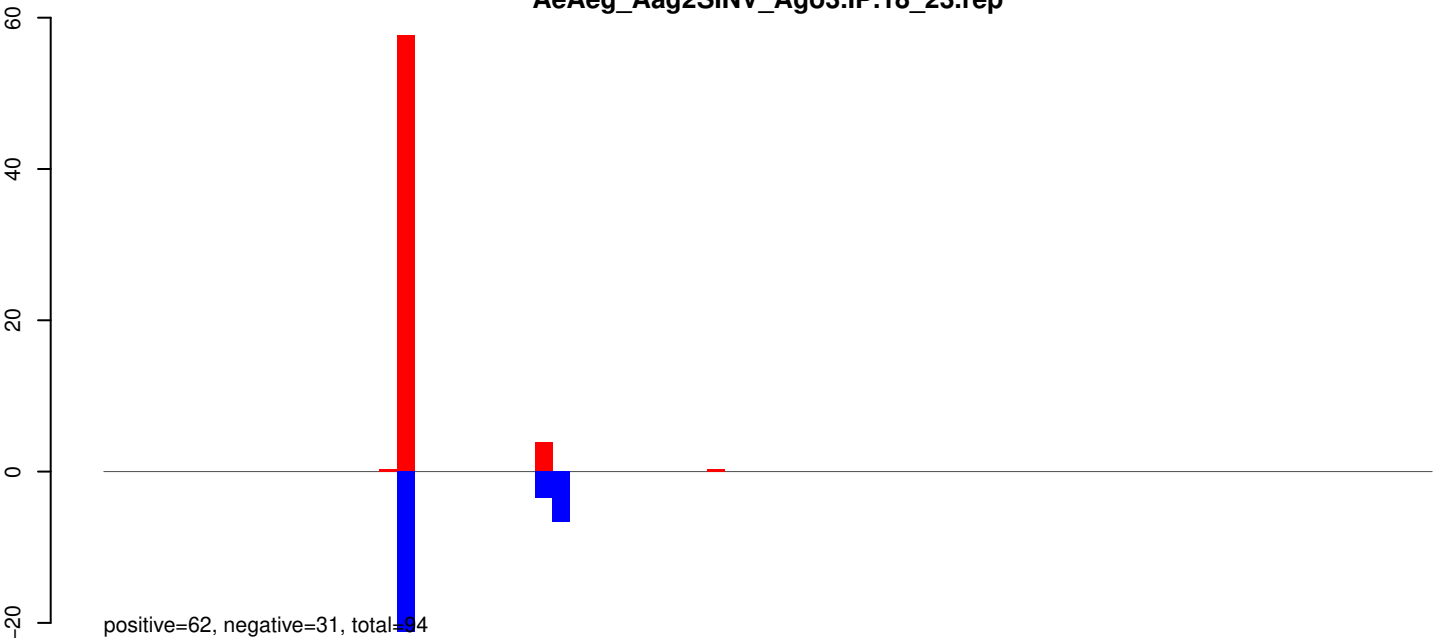
AeAeg_Aag2SINV_Ago3.IP.24_35.rep
