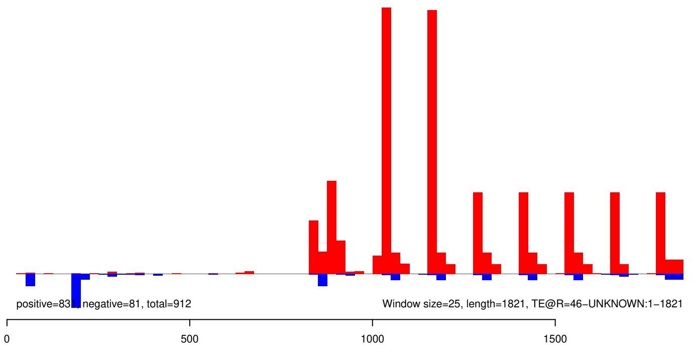
AeAeg_Aag2SINV_Ago3.IP.rep
