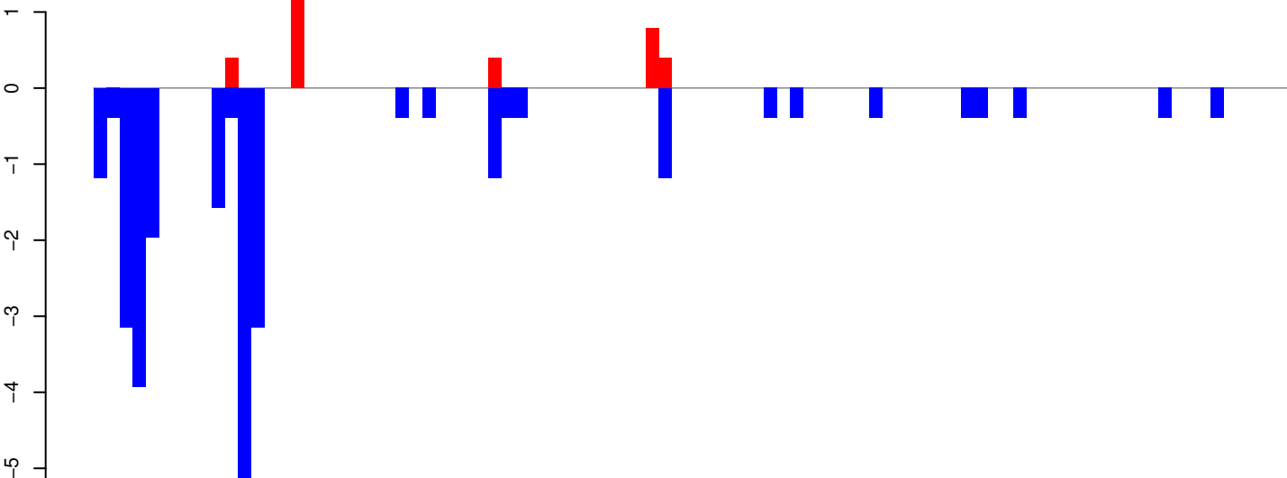
AeAeg_Aag2SINV_Ago3.IP.rep
