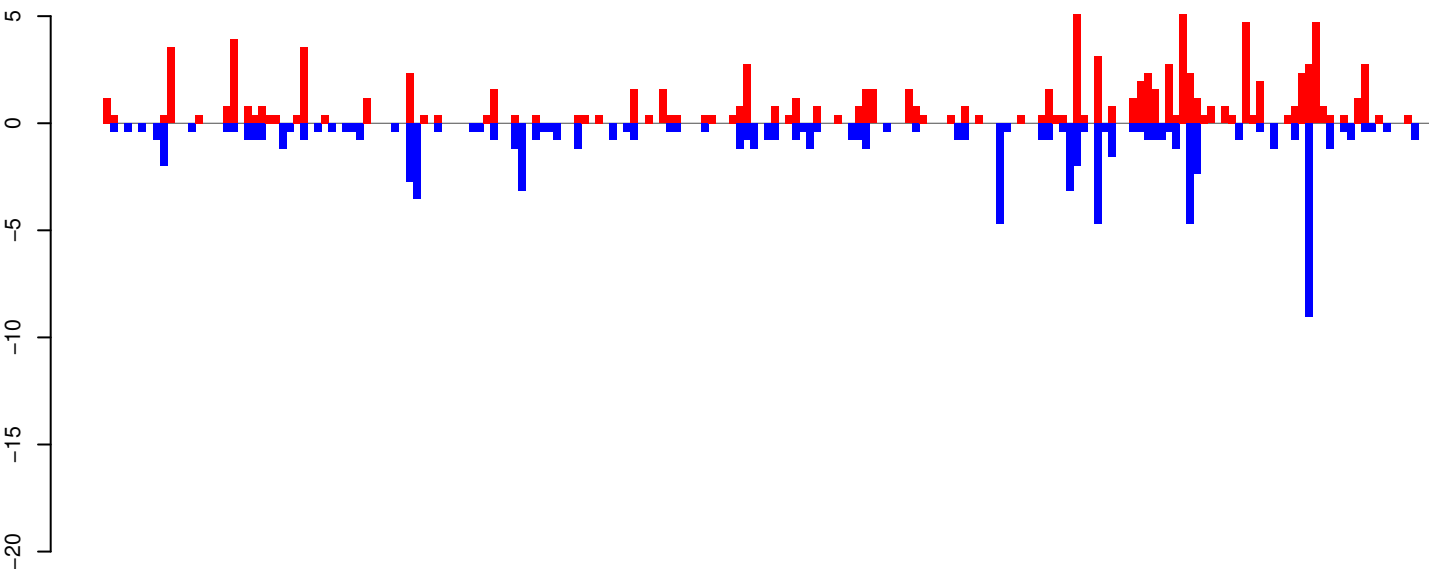
AeAeg_Aag2SINV_Ago3.IP.18_23.rep
