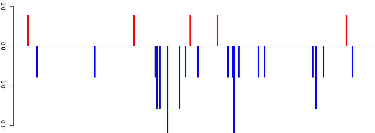
AeAeg_Aag2SINV_Ago3.IP.rep
