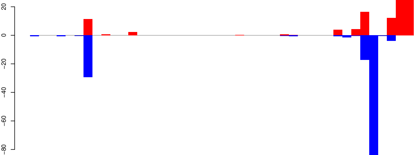
AeAeg_Aag2SINV_Ago3.IP.24_35.rep
