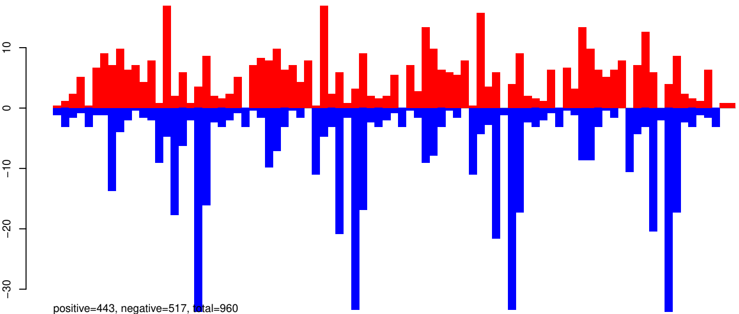
AeAeg_Aag2SINV_Ago3.IP.24_35.rep
