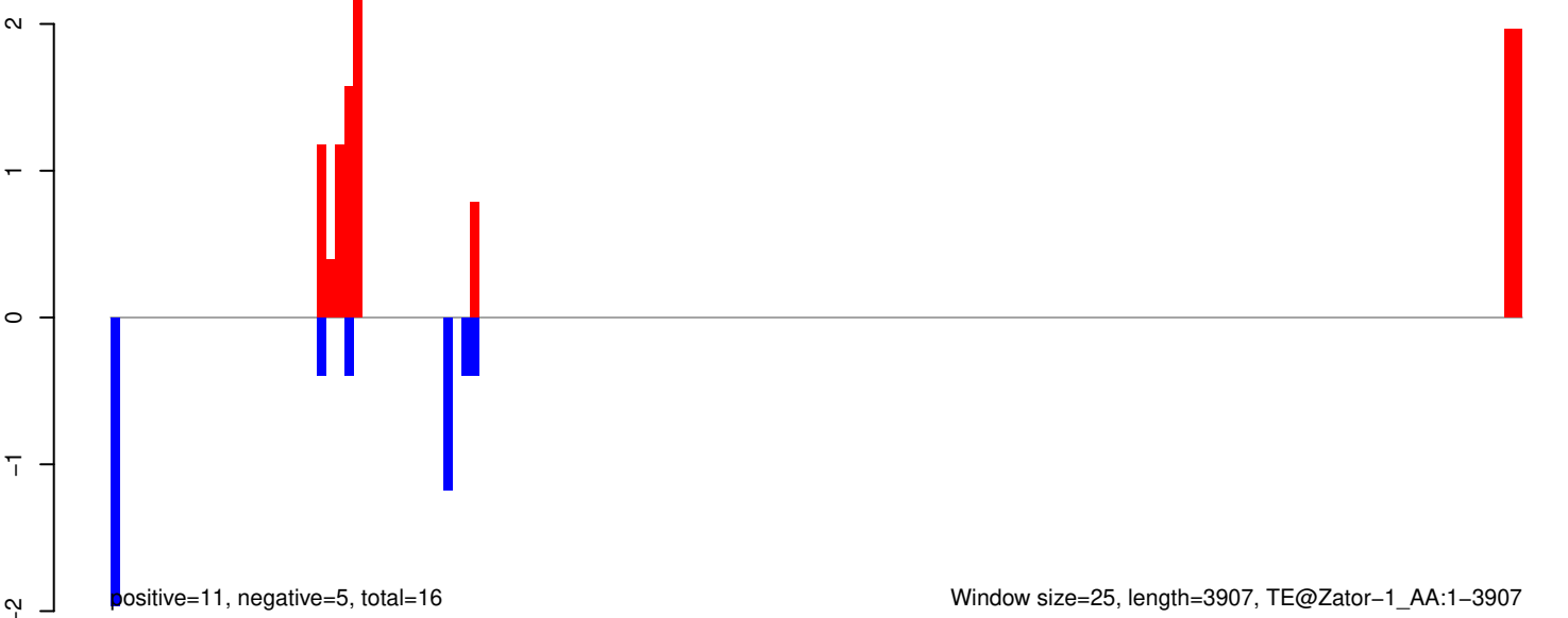
AeAeg_Aag2SINV_Ago3.IP.rep
