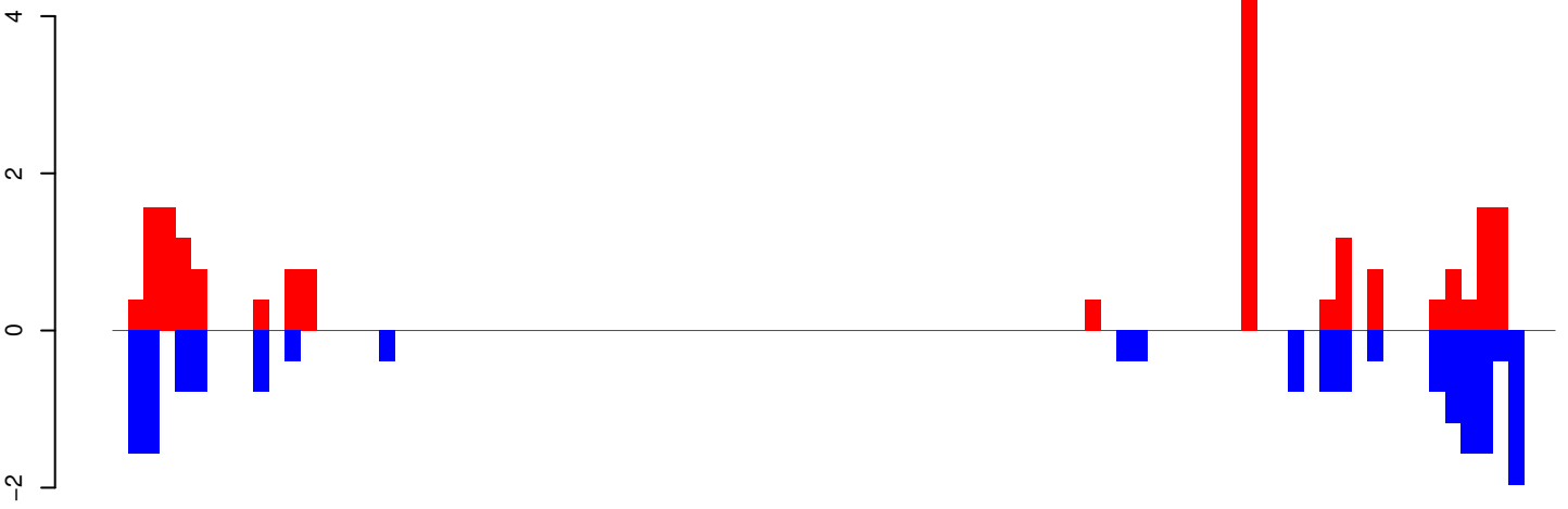
AeAeg_Aag2SINV_Ago3.IP.24_35.rep
