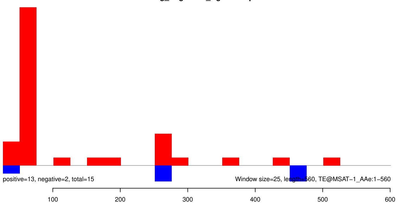
AeAeg_Aag2SINV_Ago3.IP.rep
