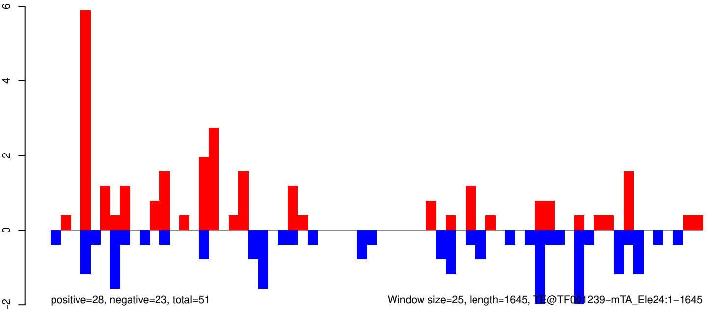
AeAeg_Aag2SINV_Ago3.IP.rep
