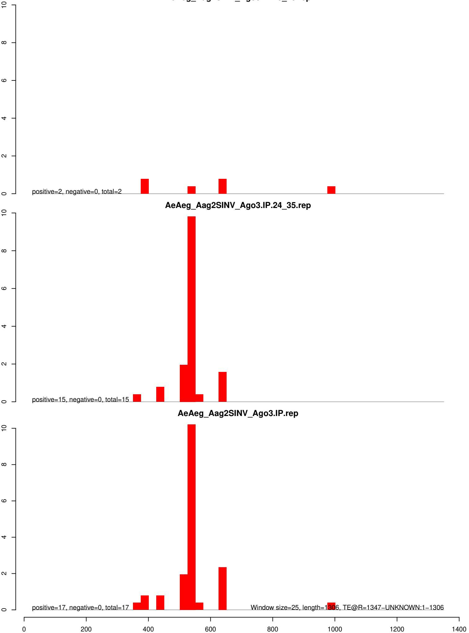
AeAeg_Aag2SINV_Ago3.IP.18_23.rep
