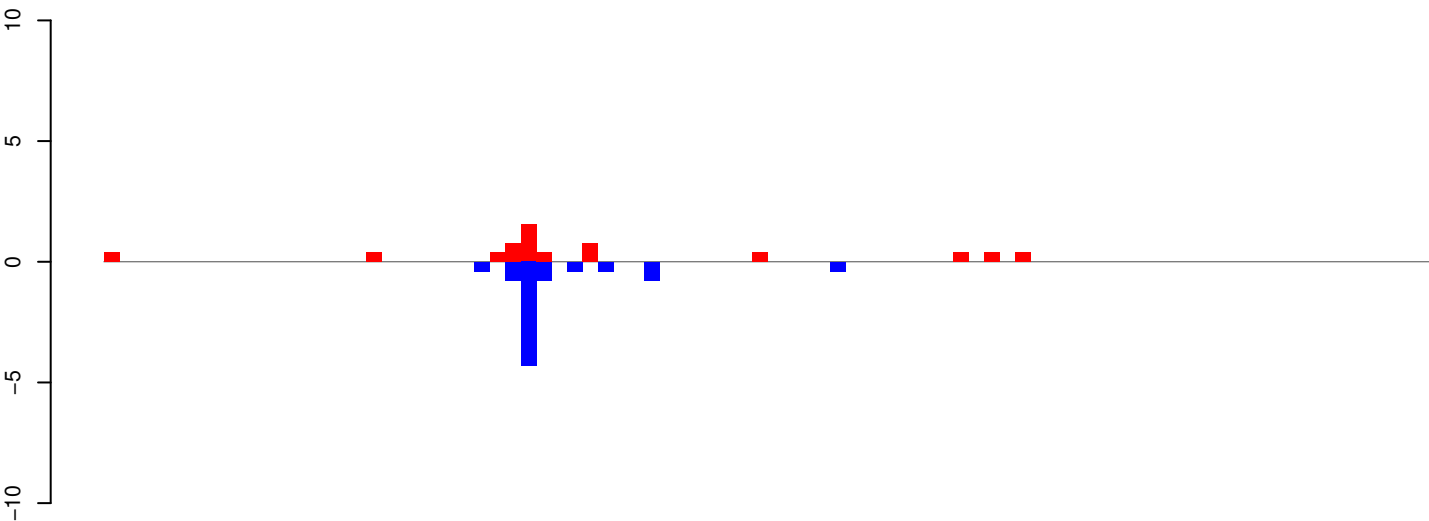
AeAeg_Aag2SINV_Ago3.IP.18_23.rep
