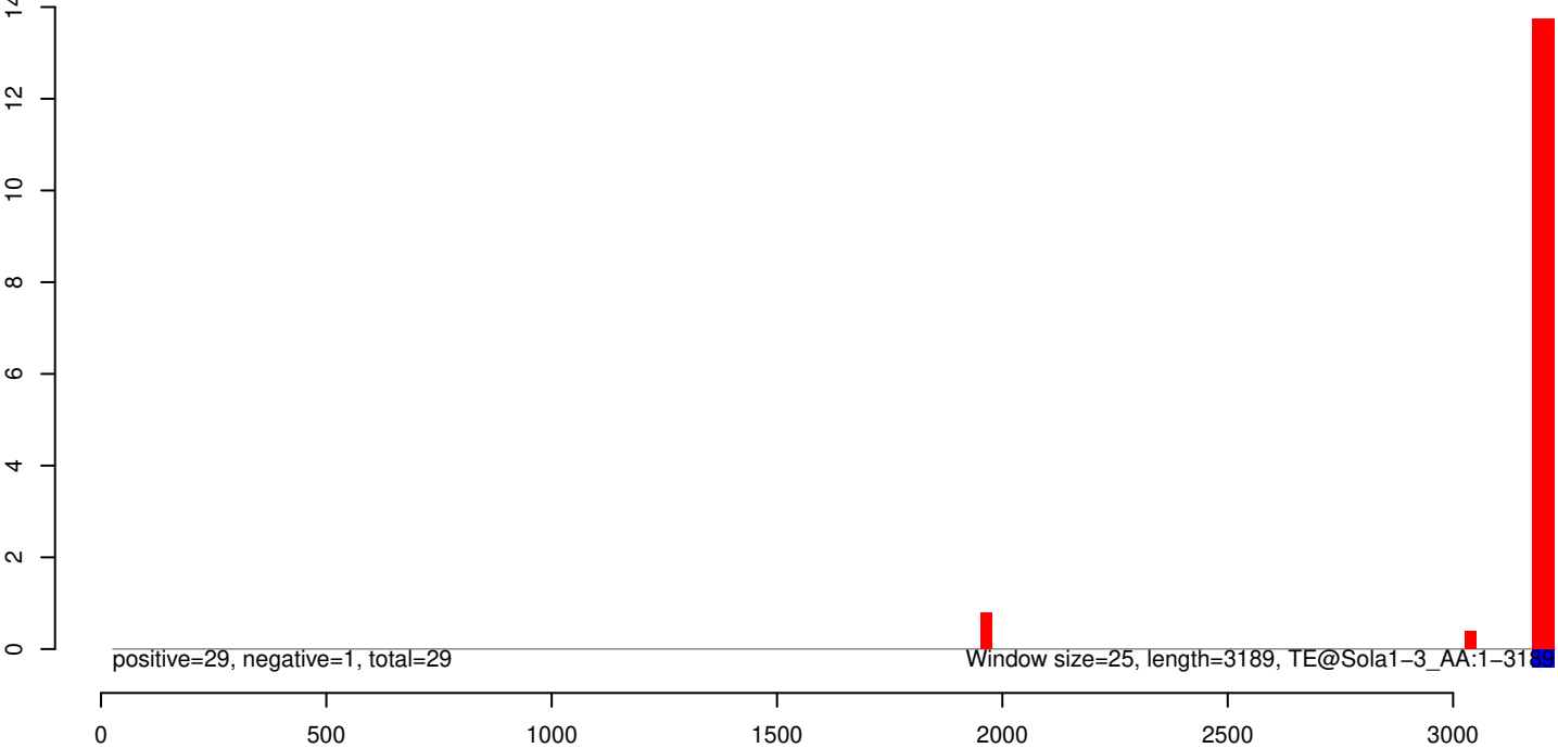
AeAeg_Aag2SINV_Ago3.IP.rep
