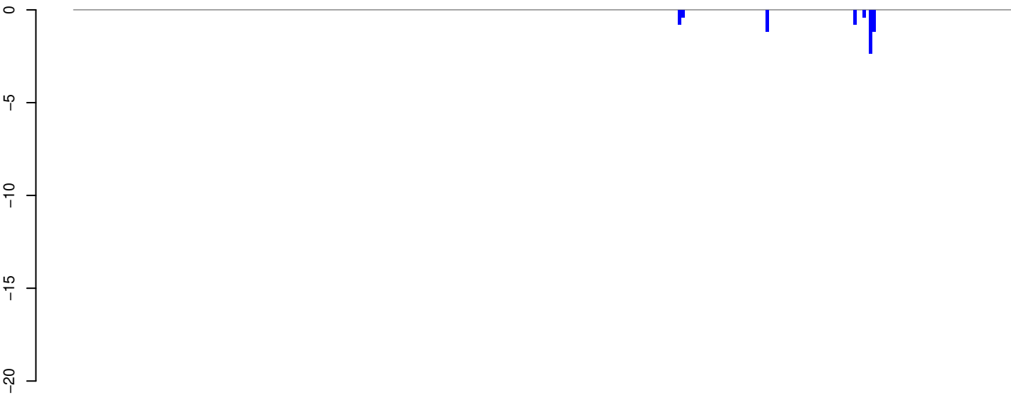
AeAeg_Aag2SINV_Ago3.IP.18_23.rep
