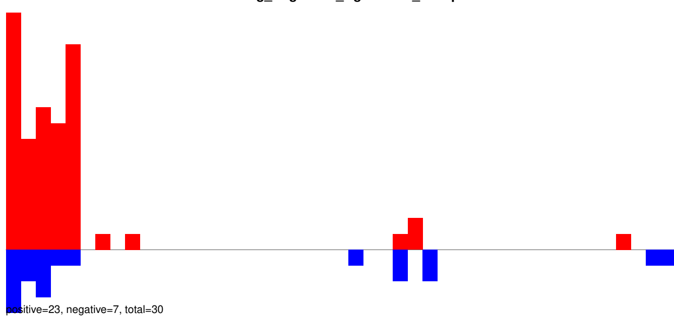
AeAeg_Aag2SINV_Ago3.IP.24_35.rep
