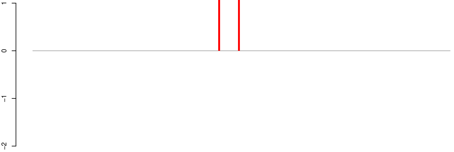
AeAeg_Aag2SINV_Ago3.IP.18_23.rep
