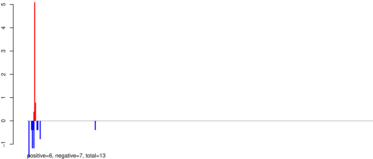
AeAeg_Aag2SINV_Ago3.IP.24_35.rep
