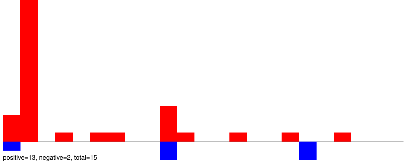
AeAeg_Aag2SINV_Ago3.IP.24_35.rep
