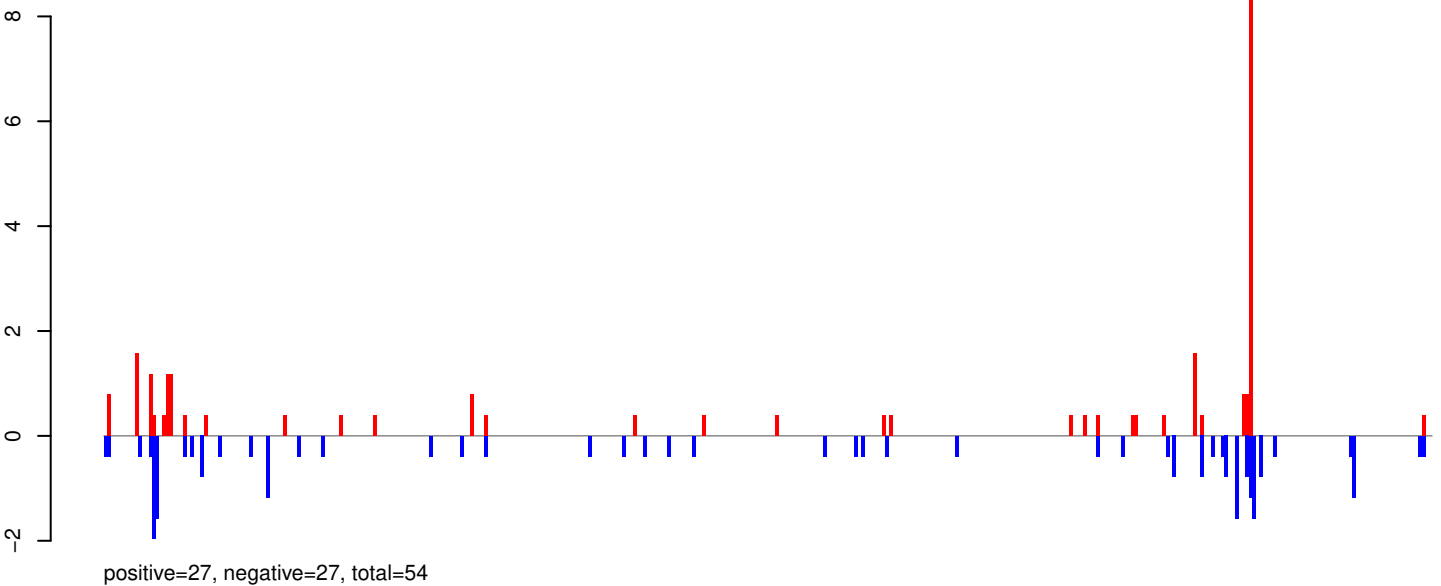
AeAeg_Aag2SINV_Ago3.IP.24_35.rep
