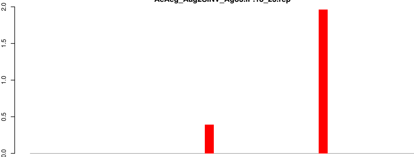
AeAeg_Aag2SINV_Ago3.IP.18_23.rep
