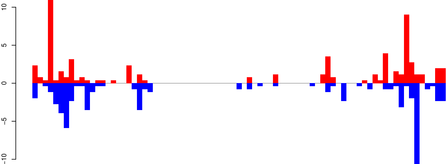
AeAeg_Aag2SINV_Ago3.IP.24_35.rep
