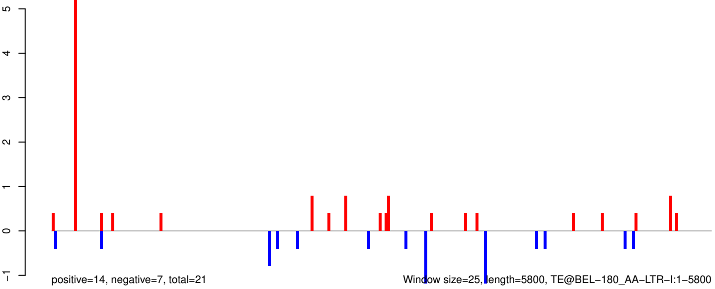
AeAeg_Aag2SINV_Ago3.IP.rep
