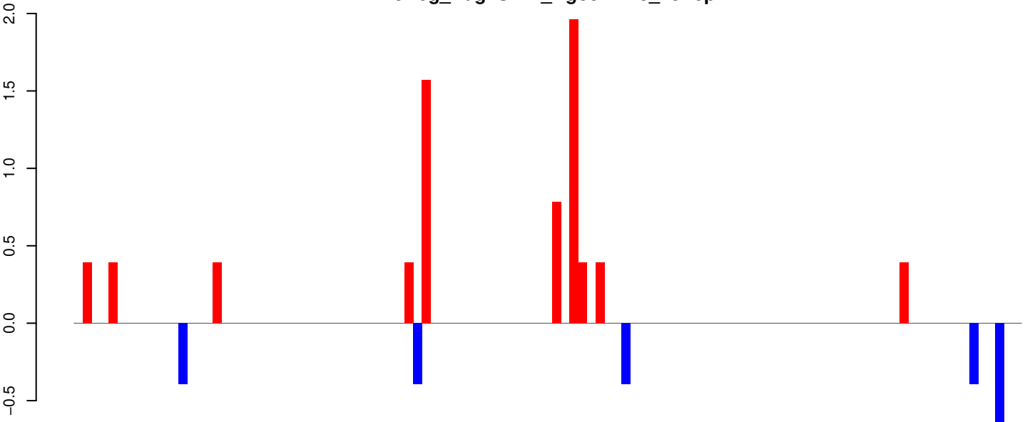
AeAeg_Aag2SINV_Ago3.IP.18_23.rep
