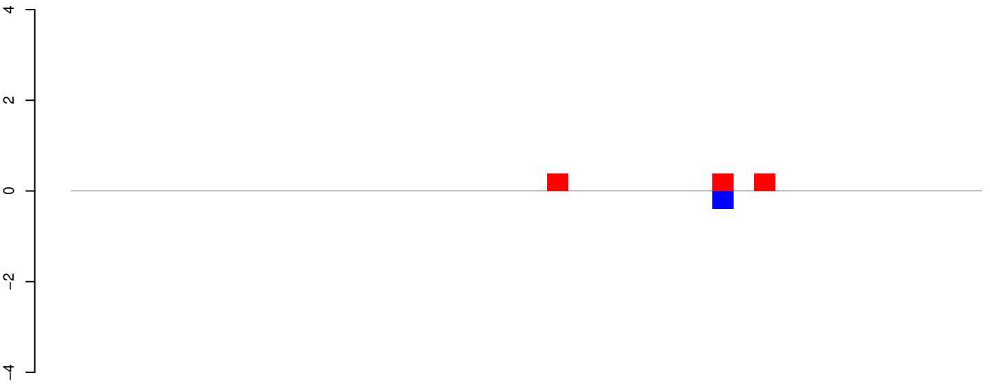
AeAeg_Aag2SINV_Ago3.IP.18_23.rep
