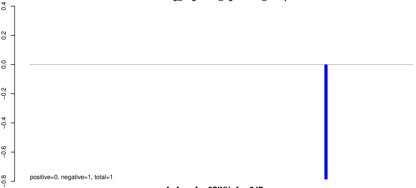
AeAeg_Aag2SINV_Ago3.IP.rep
