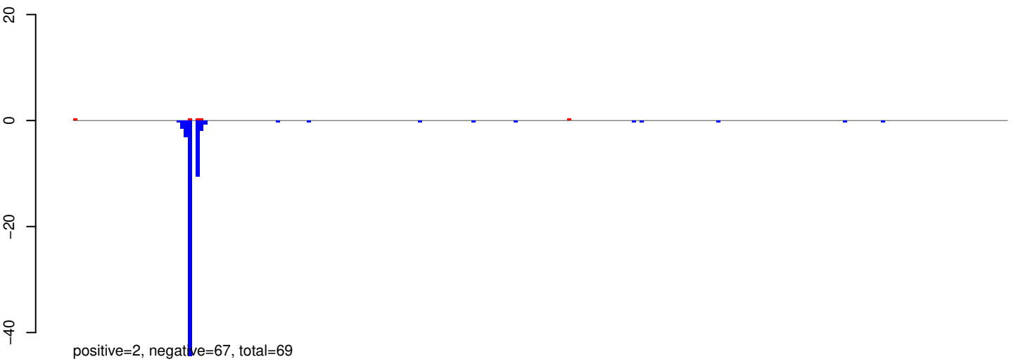
AeAeg_Aag2SINV_Ago3.IP.rep
