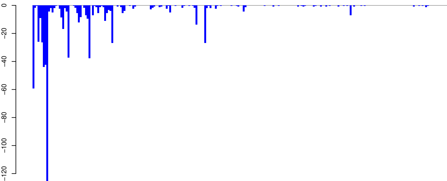
AeAeg_Aag2SINV_Ago3.IP.rep
