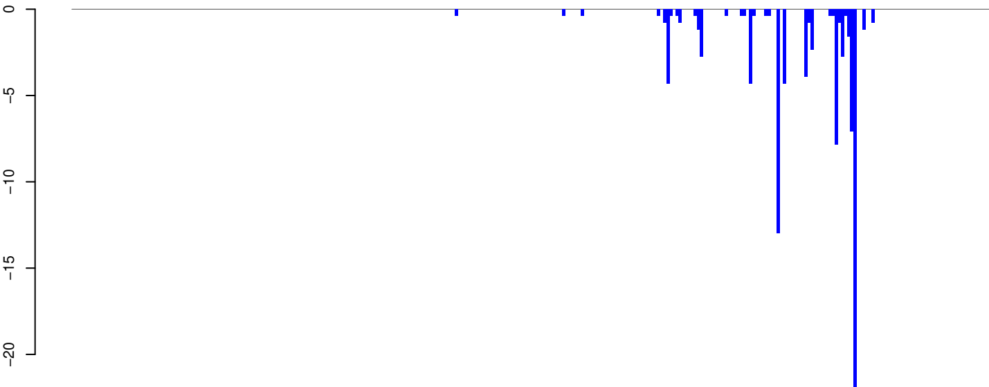
AeAeg_Aag2SINV_Ago3.IP.rep
