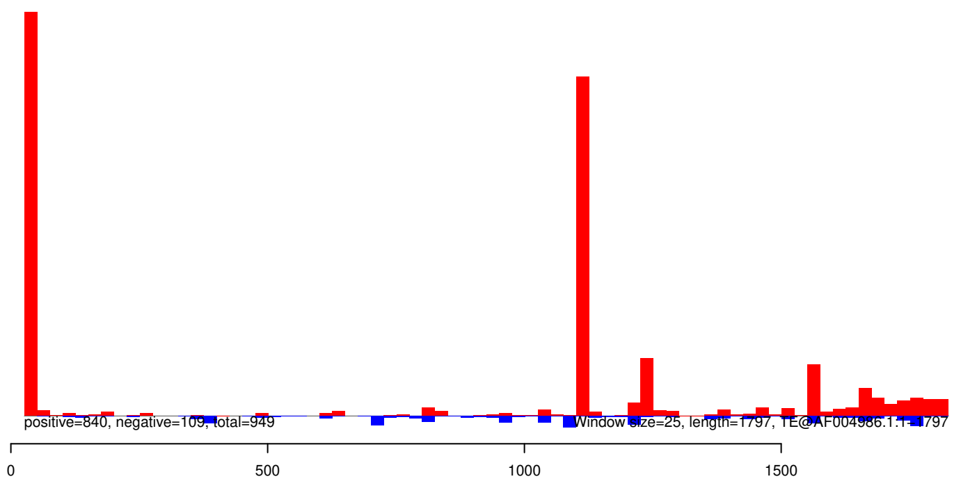
AeAeg_Aag2SINV_Piwi4.IP.rep
