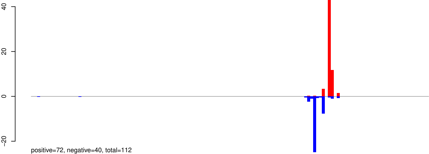
AeAeg_Aag2SINV_Piwi4.IP.rep
