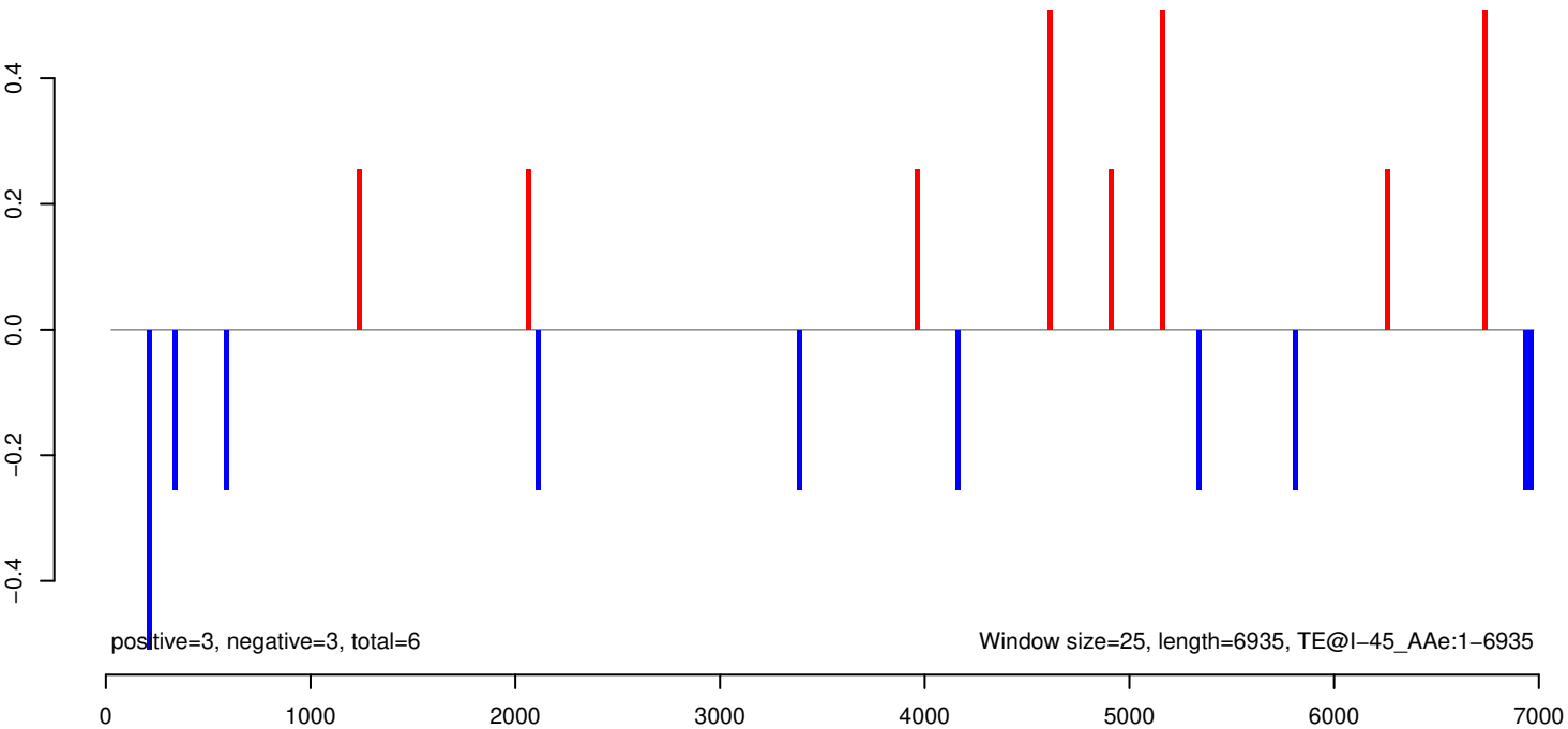
AeAeg_Aag2SINV_Piwi4.IP.rep
