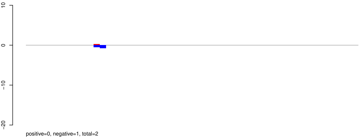
AeAeg_Aag2SINV_Piwi4.IP.rep
