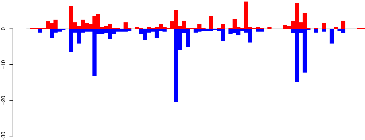
AeAeg_Aag2SINV_Piwi4.IP.18_23.rep
