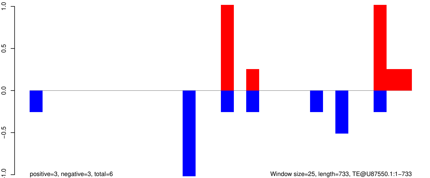
AeAeg_Aag2SINV_Piwi4.IP.rep
