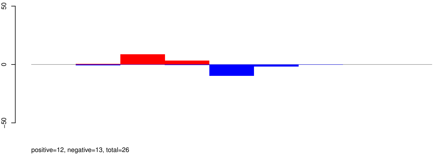
AeAeg_Aag2SINV_Piwi4.IP.rep
