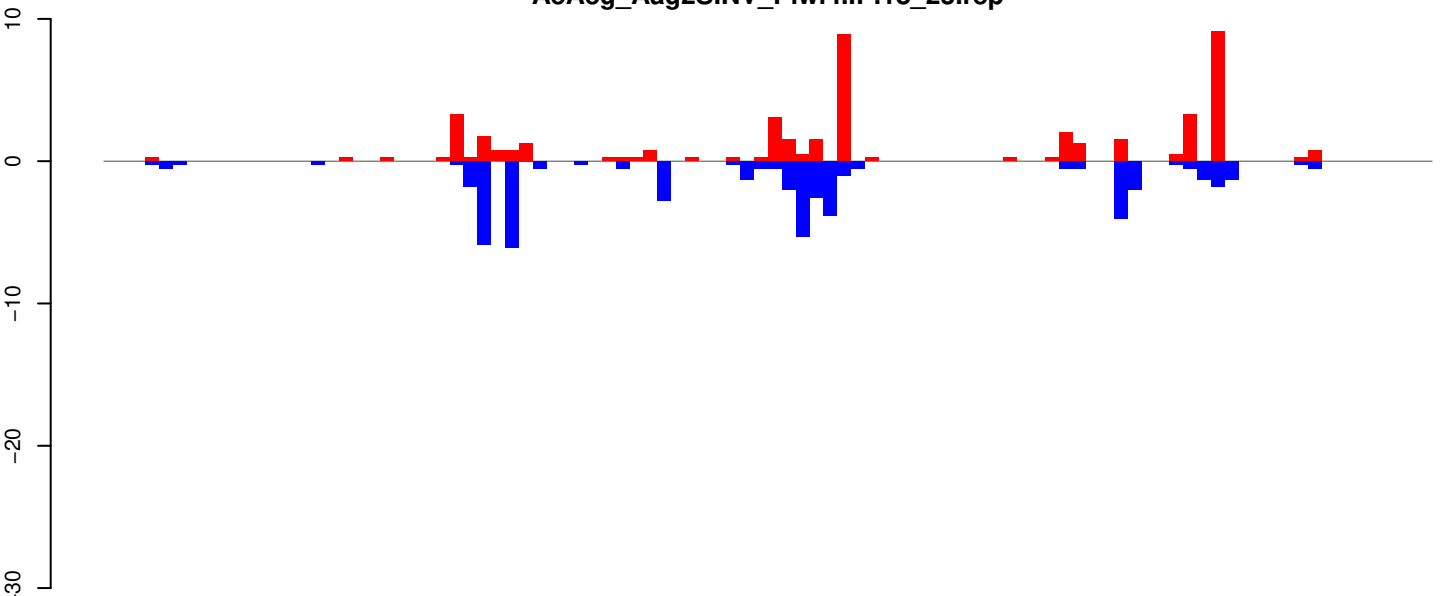
AeAeg_Aag2SINV_Piwi4.IP.18_23.rep
