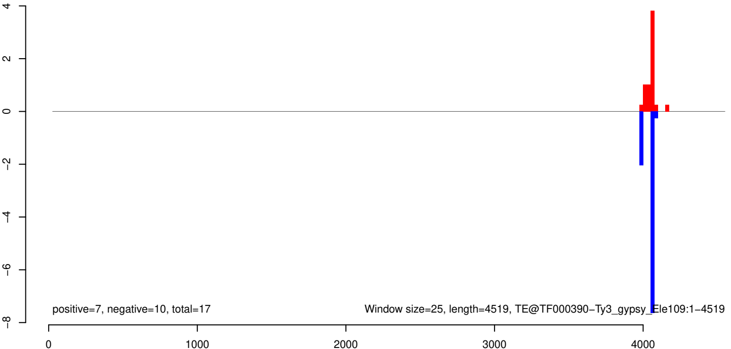
AeAeg_Aag2SINV_Piwi4.IP.rep
