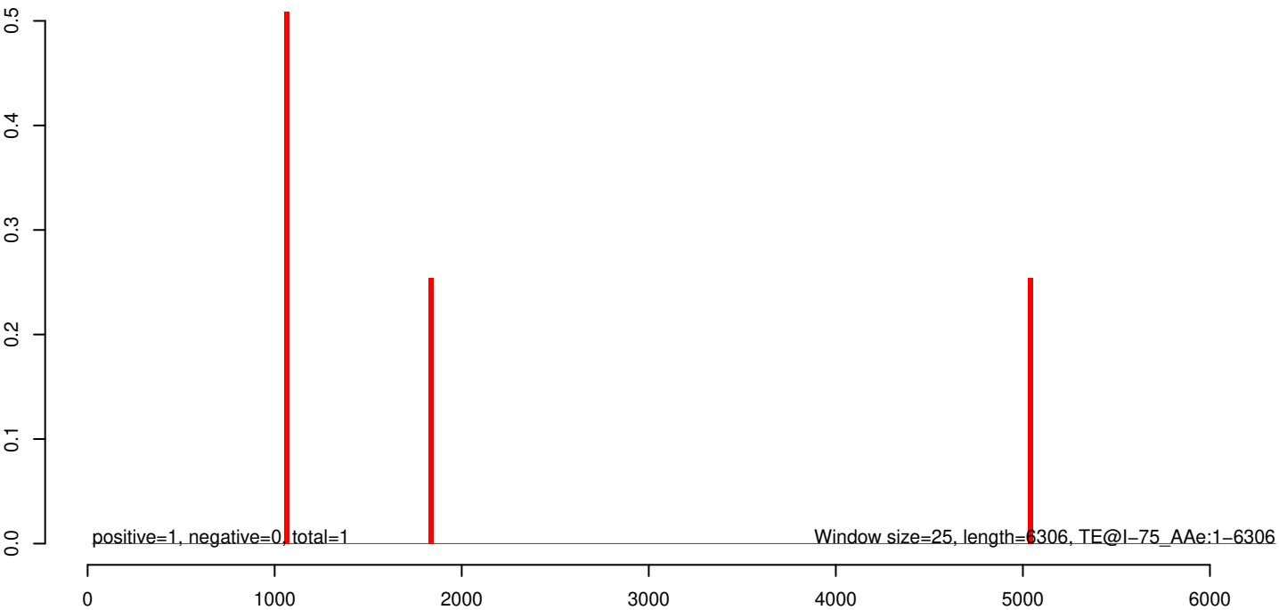
AeAeg_Aag2SINV_Piwi4.IP.rep
