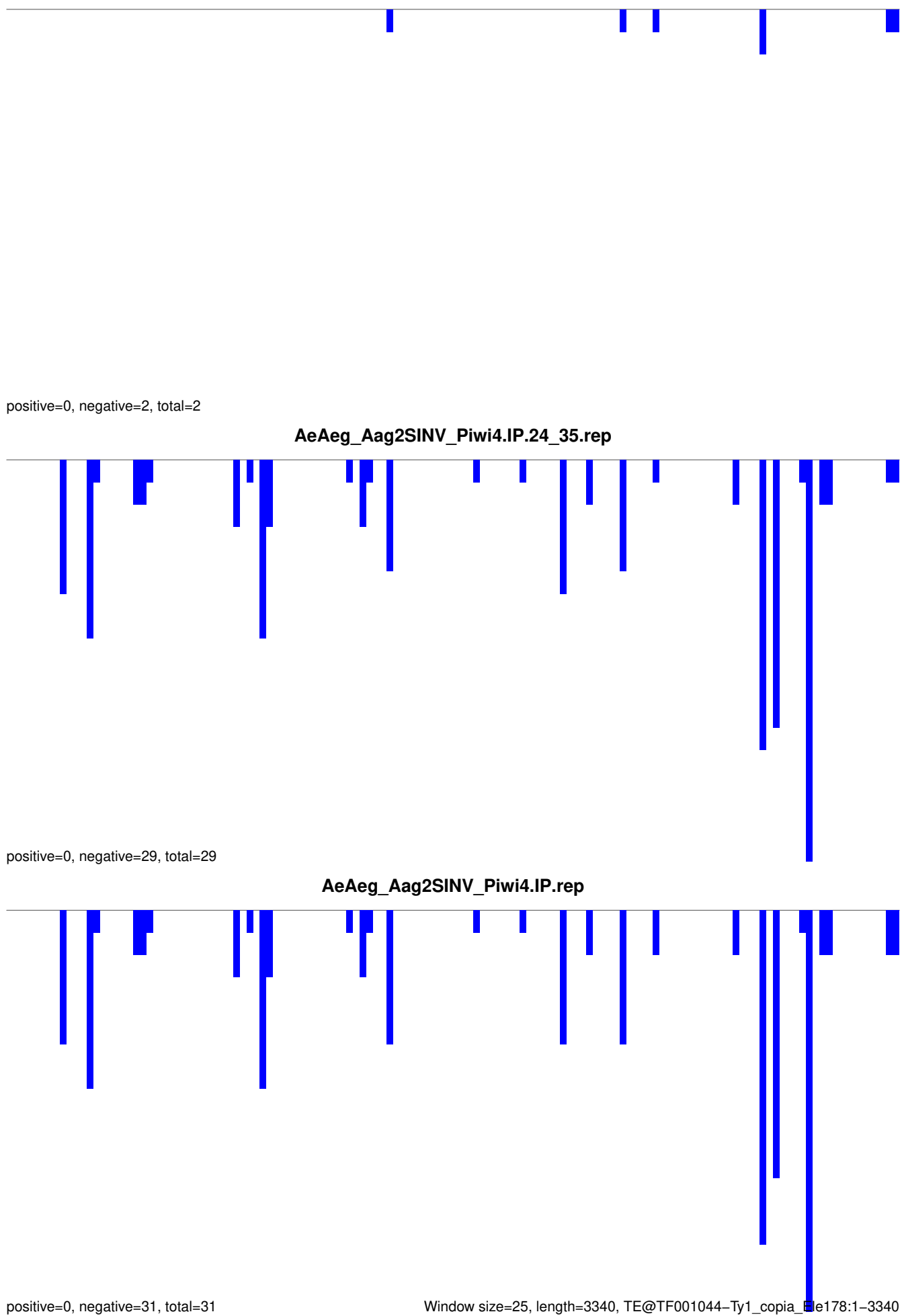
AeAeg_Aag2SINV_Piwi4.IP.18_23.rep
