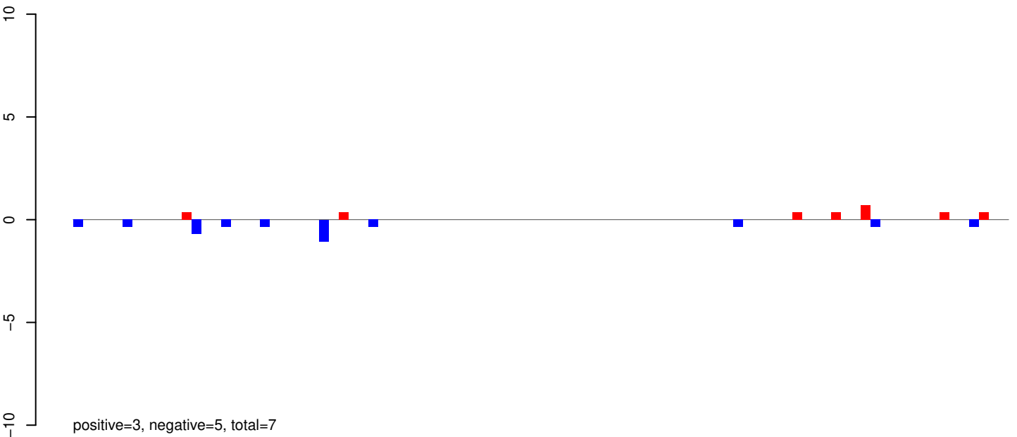
AeAeg_Aag2SINV_Piwi6.IP.rep
