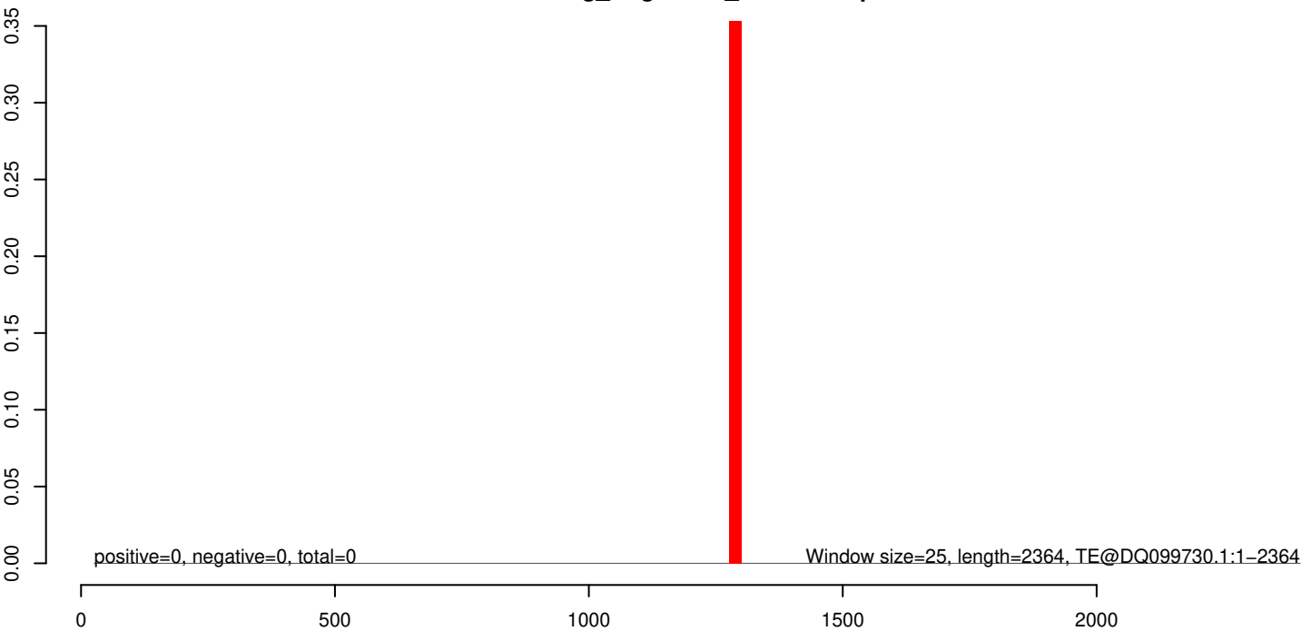
AeAeg_Aag2SINV_Piwi6.IP.rep
