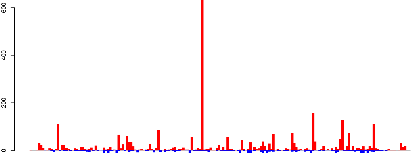
AeAeg_Aag2SINV_Piwi6.IP.rep
