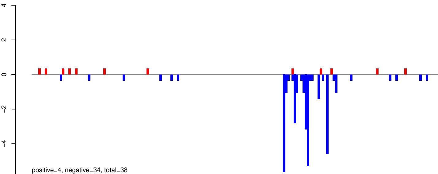
AeAeg_Aag2SINV_Piwi6.IP.rep
