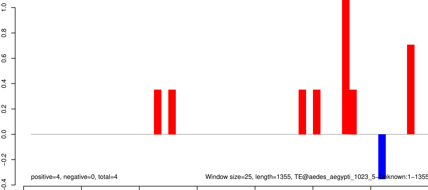
AeAeg_Aag2SINV_Piwi6.IP.rep
