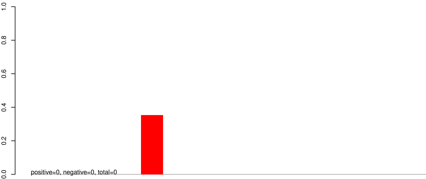
AeAeg_Aag2SINV_Piwi6.IP.rep
