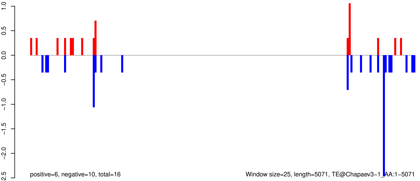
AeAeg_Aag2SINV_Piwi6.IP.rep
