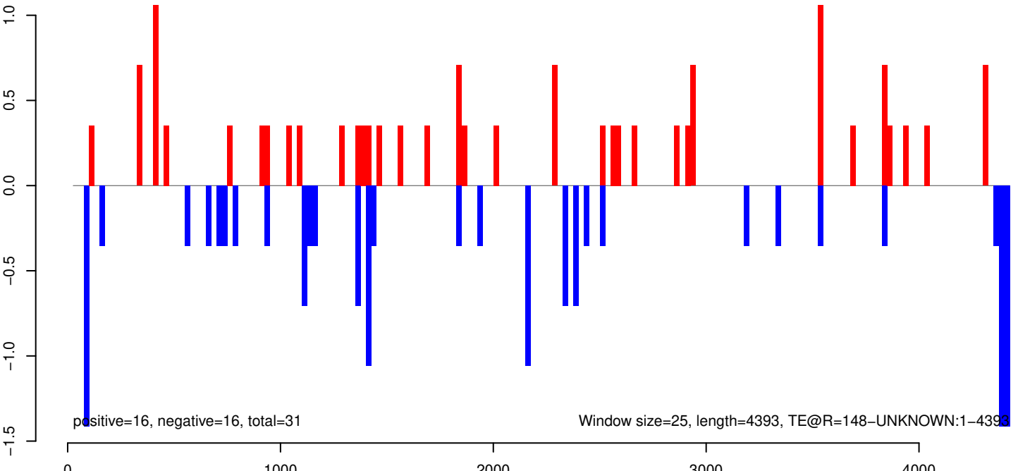
AeAeg_Aag2SINV_Piwi6.IP.rep
