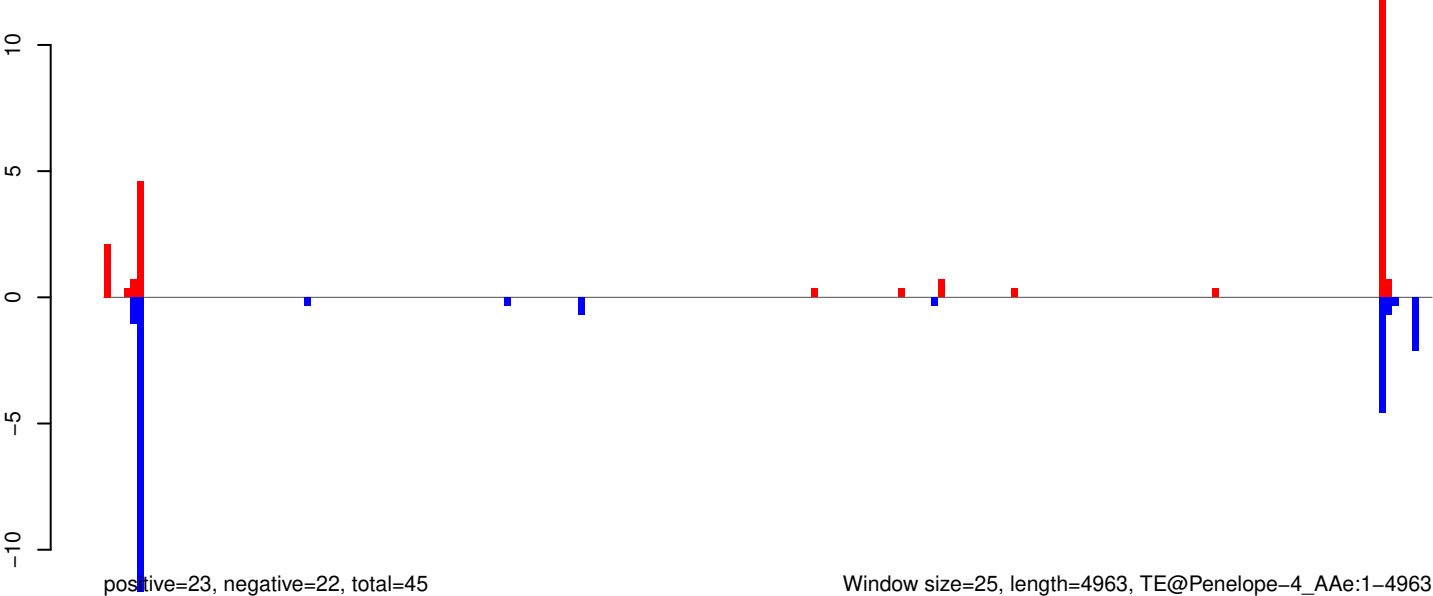
AeAeg_Aag2SINV_Piwi6.IP.rep
