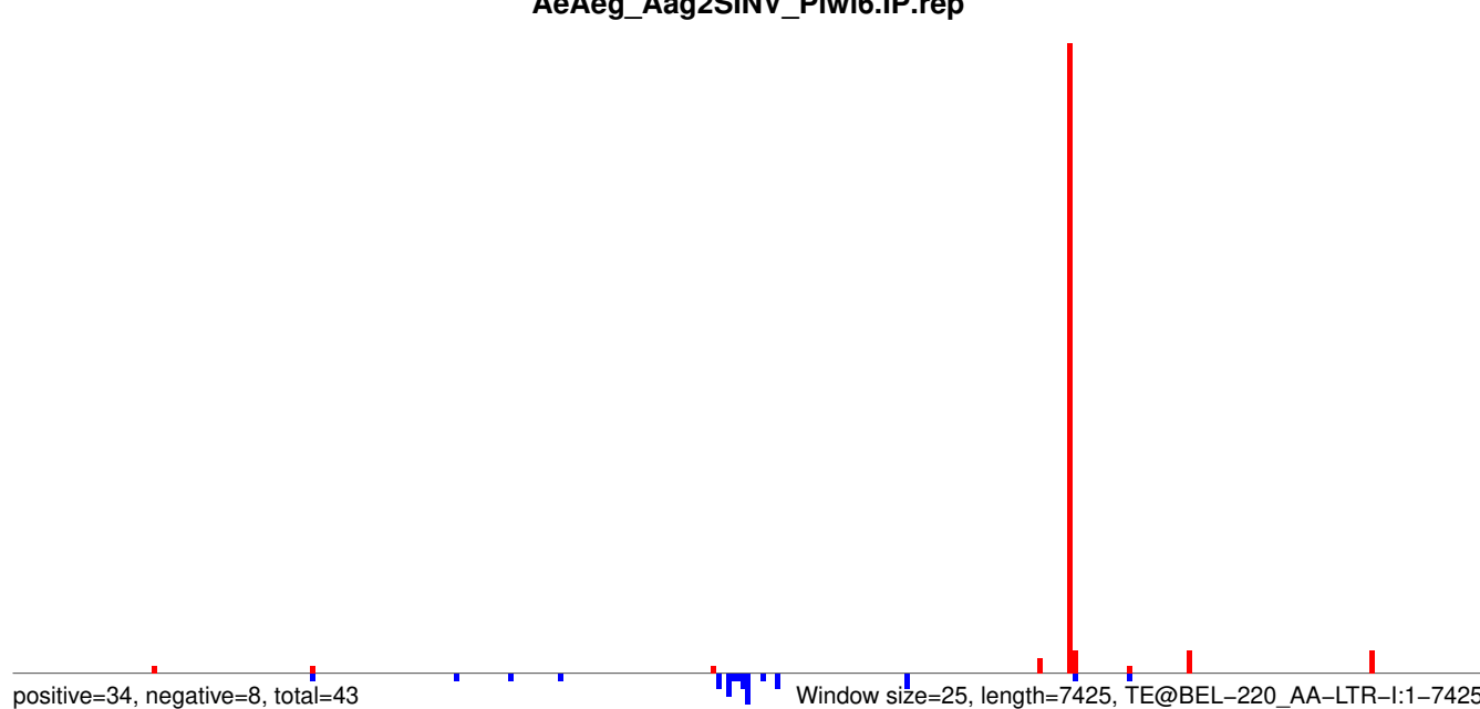
AeAeg_Aag2SINV_Piwi6.IP.rep
