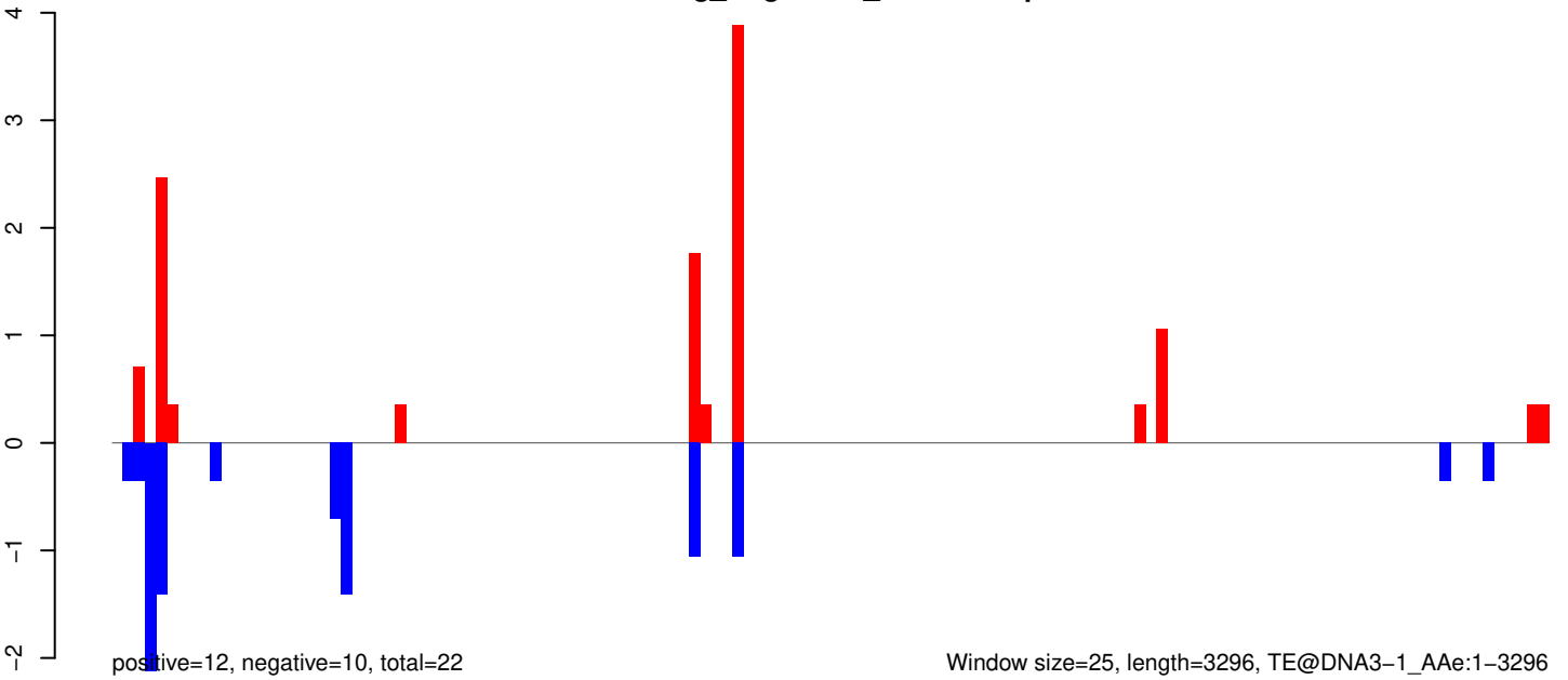
AeAeg_Aag2SINV_Piwi6.IP.rep
