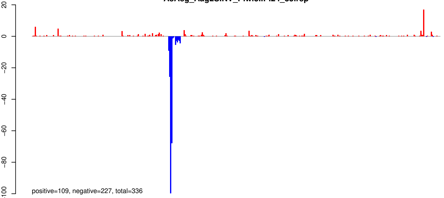
AeAeg_Aag2SINV_Piwi5.IP.rep
