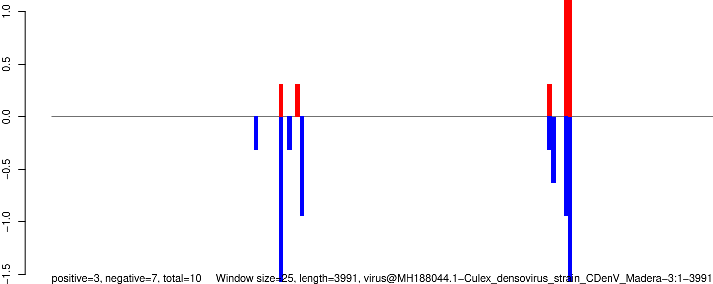
AeAeg_Aag2SINV_Piwi5.IP.rep
