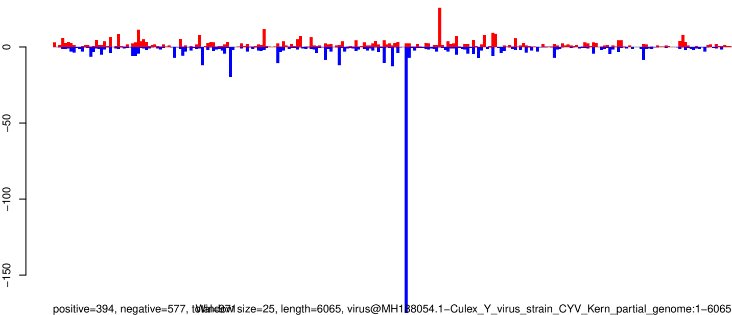
AeAeg_Aag2SINV_Piwi5.IP.rep
