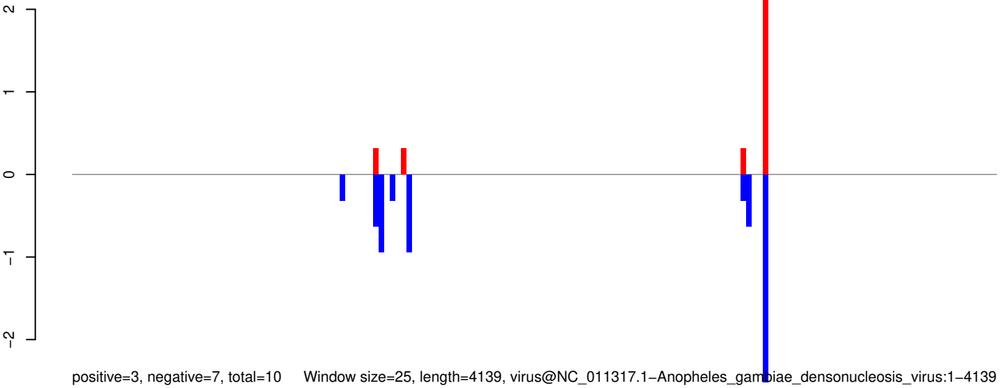
AeAeg_Aag2SINV_Piwi5.IP.rep
