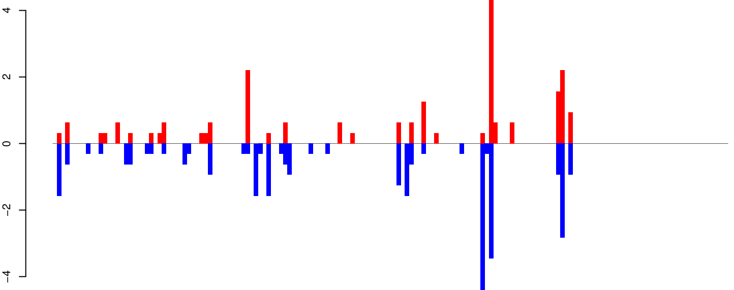
AeAeg_Aag2SINV_Piwi5.IP.rep
