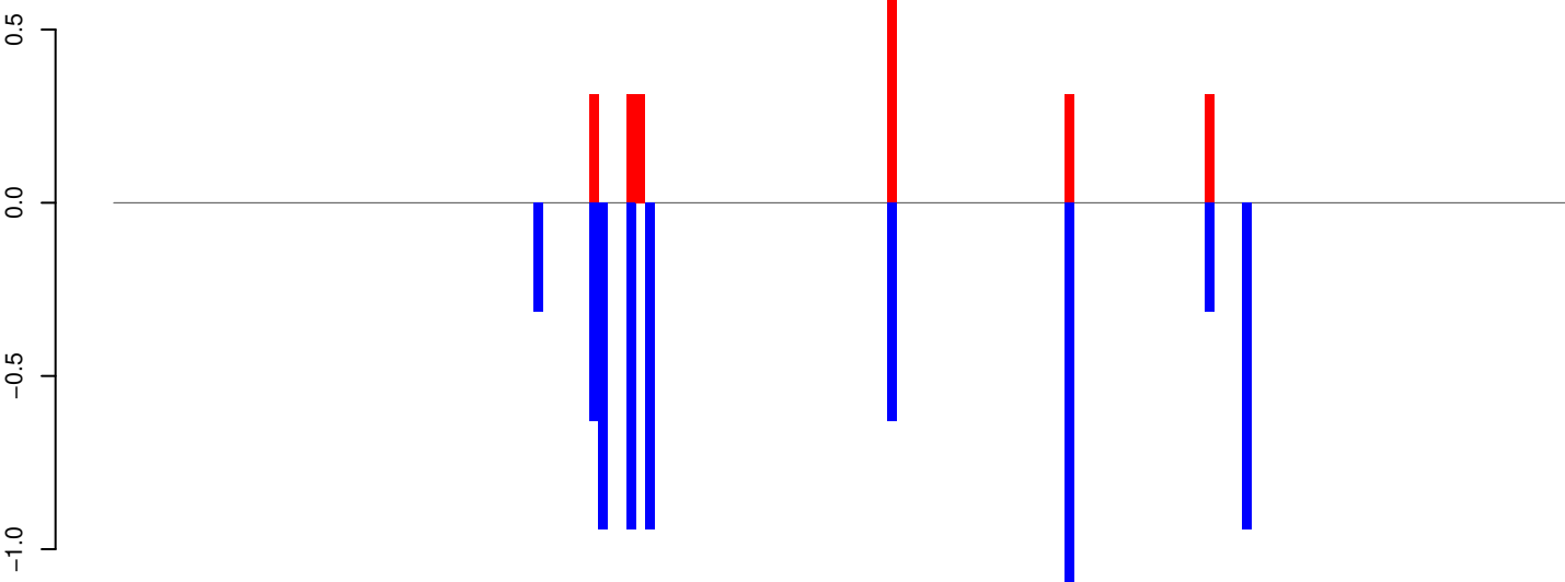
AeAeg_Aag2SINV_Piwi5.IP.rep
