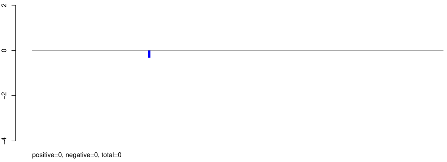
AeAeg_Aag2SINV_Piwi5.IP.rep
