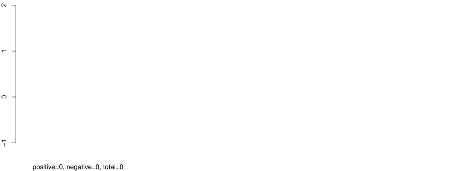
AeAeg_Aag2SINV_Piwi5.IP.rep
