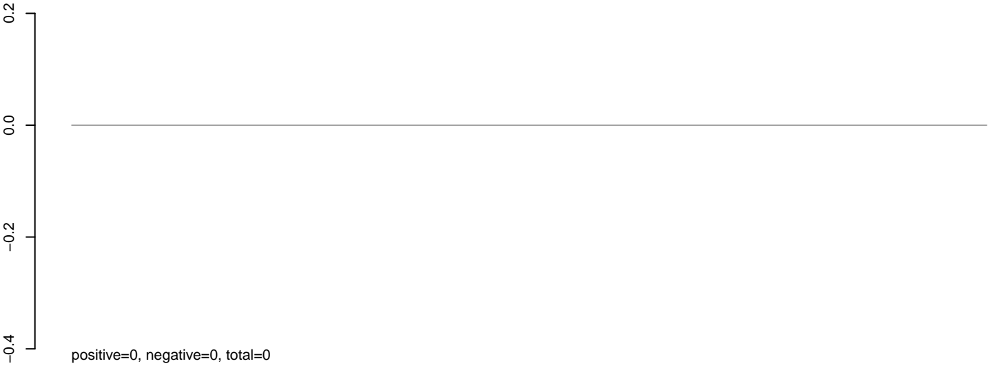
AeAlbo_Larv_OA.rep
