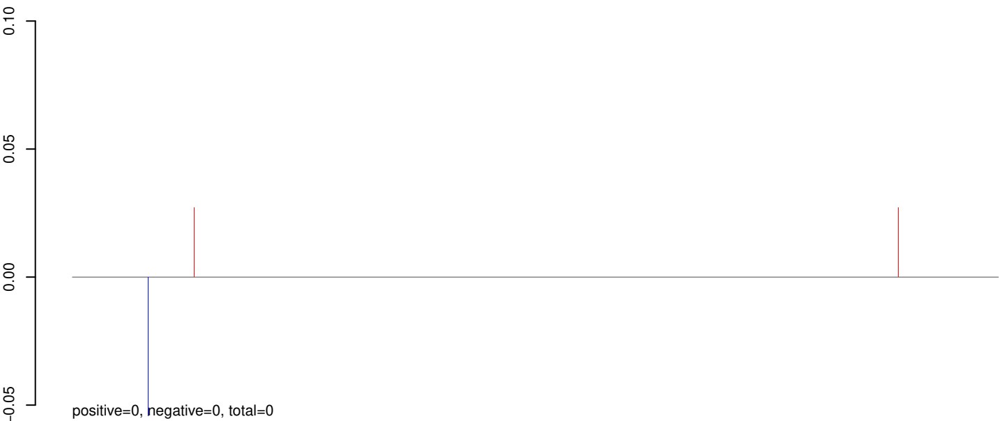
AeAlbo_BUNV_U4.4_rep1_ES.rep
