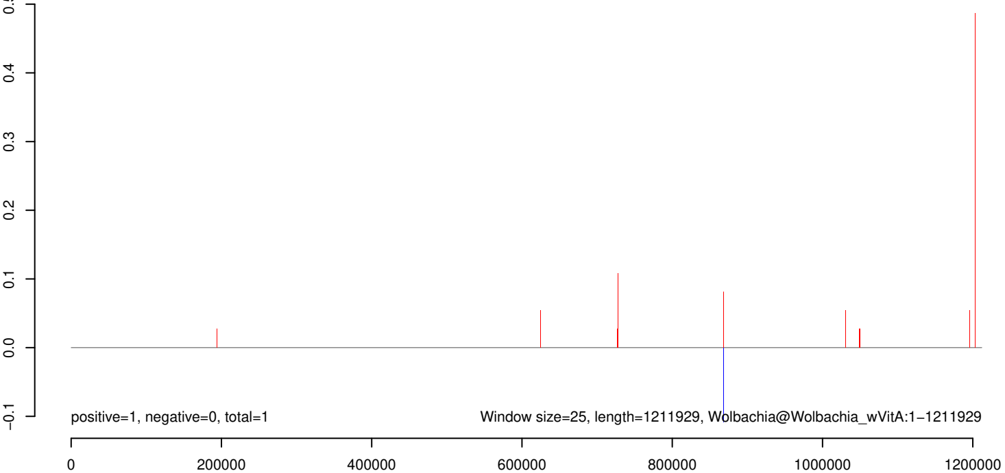
AeAlbo_BUNV_U4.4_rep1_ES.rep
