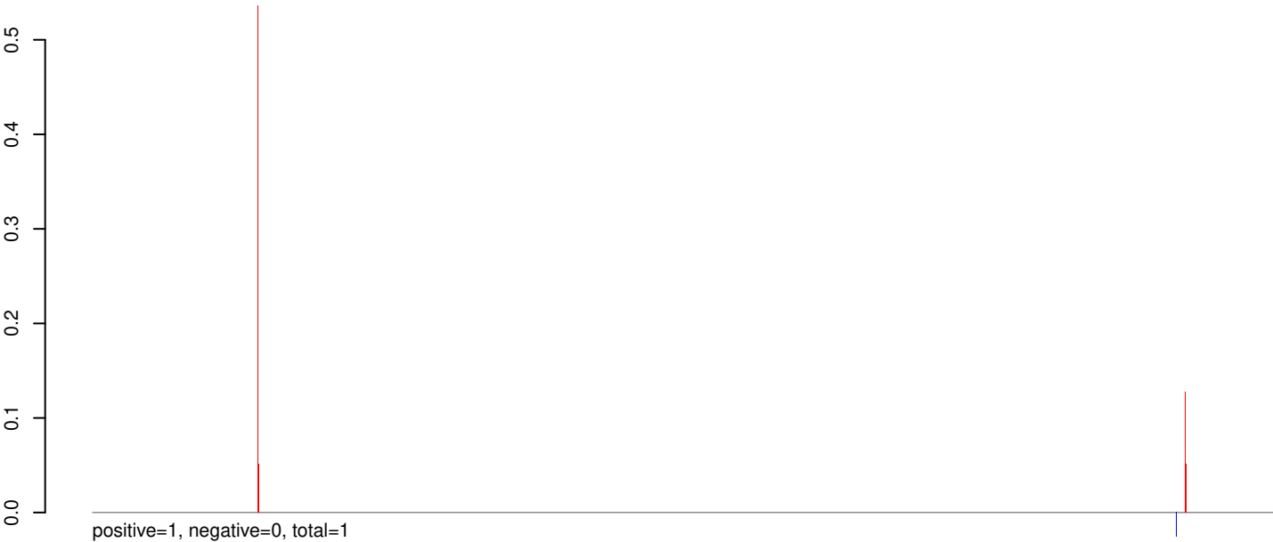
AeAlbo_BUNV_U4.4_rep2_ES.24_35.rep
