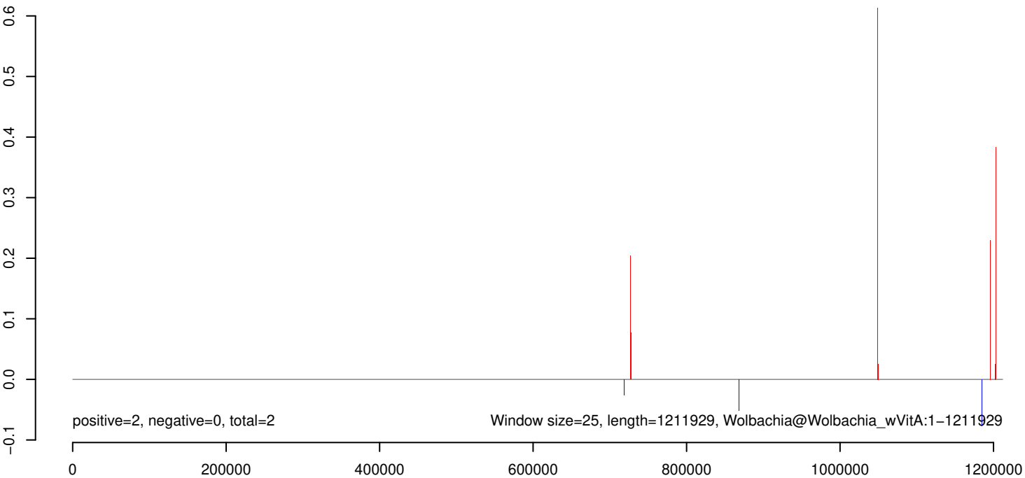
AeAlbo_BUNV_U4.4_rep2_ES.rep
