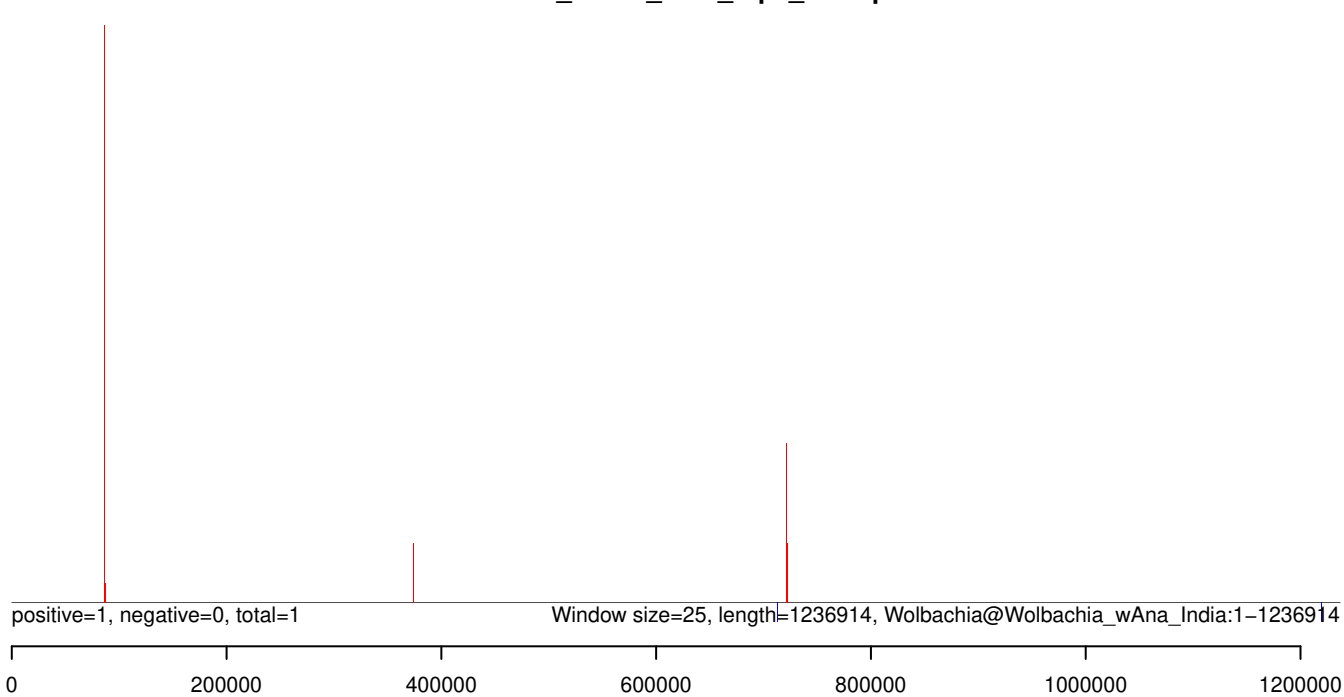
AeAlbo_BUNV_U4.4_rep2_ES.rep
