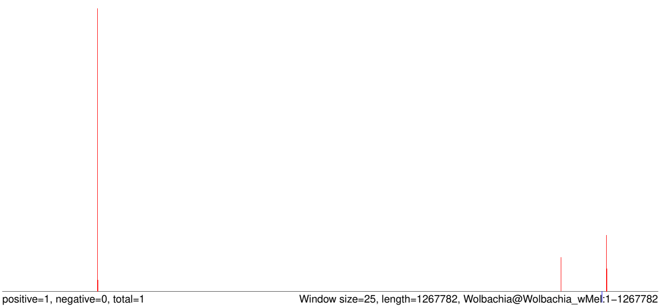
AeAlbo_BUNV_U4.4_rep2_ES.rep
