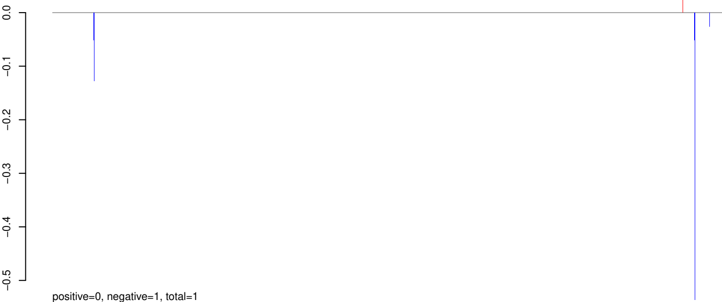
AeAlbo_BUNV_U4.4_rep2_ES.24_35.rep
