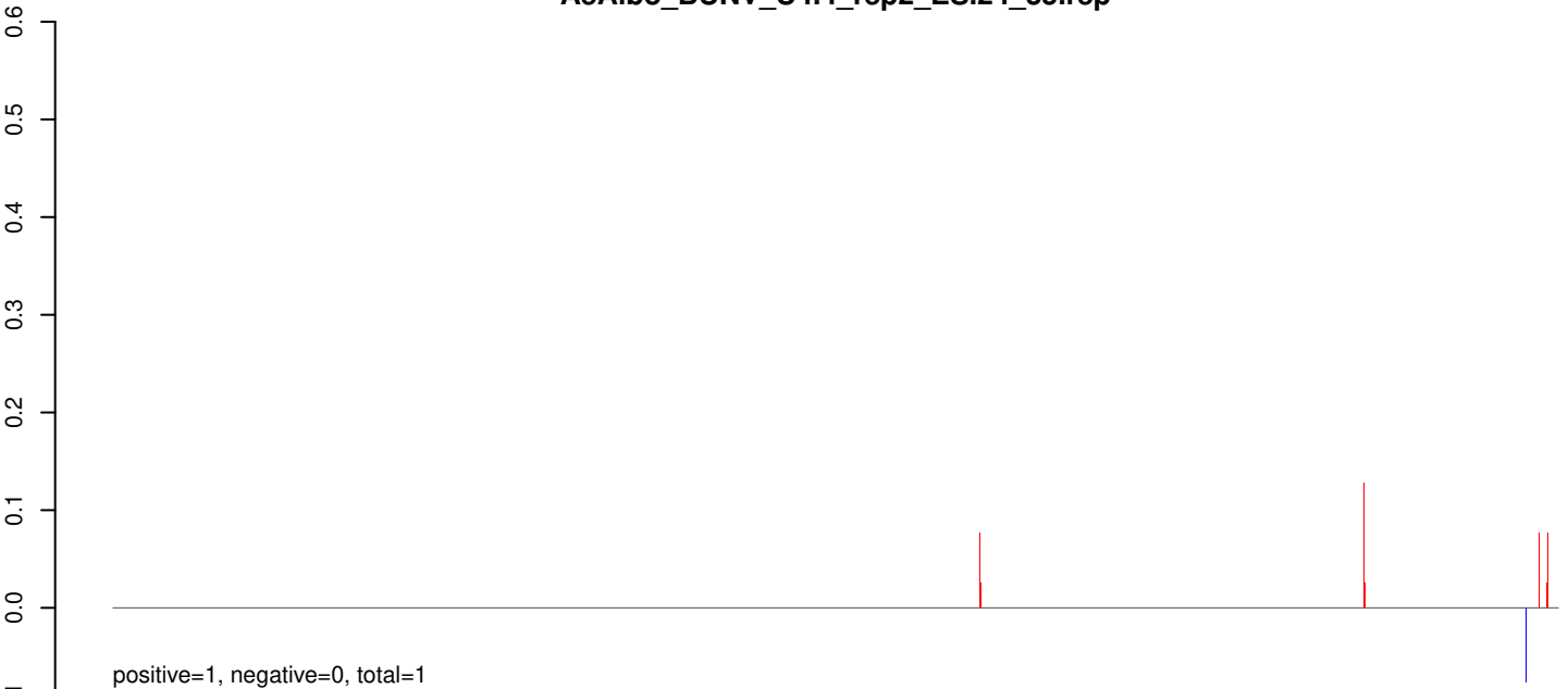
AeAlbo_BUNV_U4.4_rep2_ES.rep
