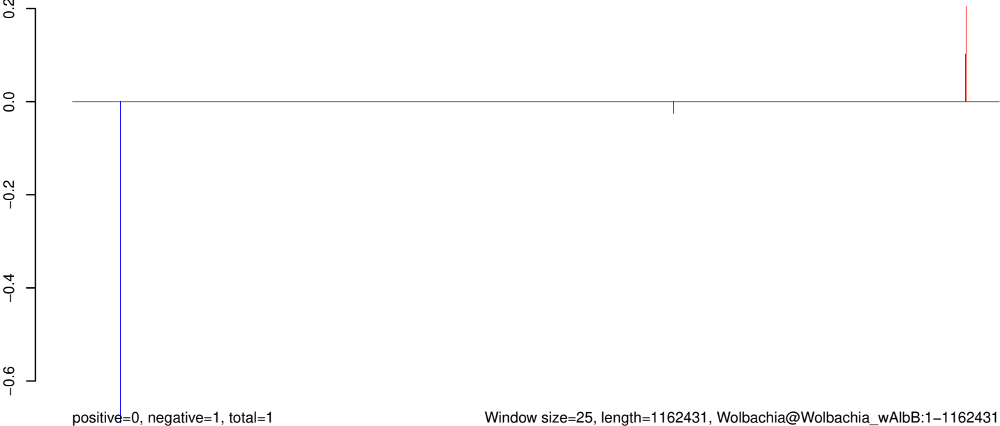
AeAlbo_BUNV_U4.4_rep2_ES.rep
