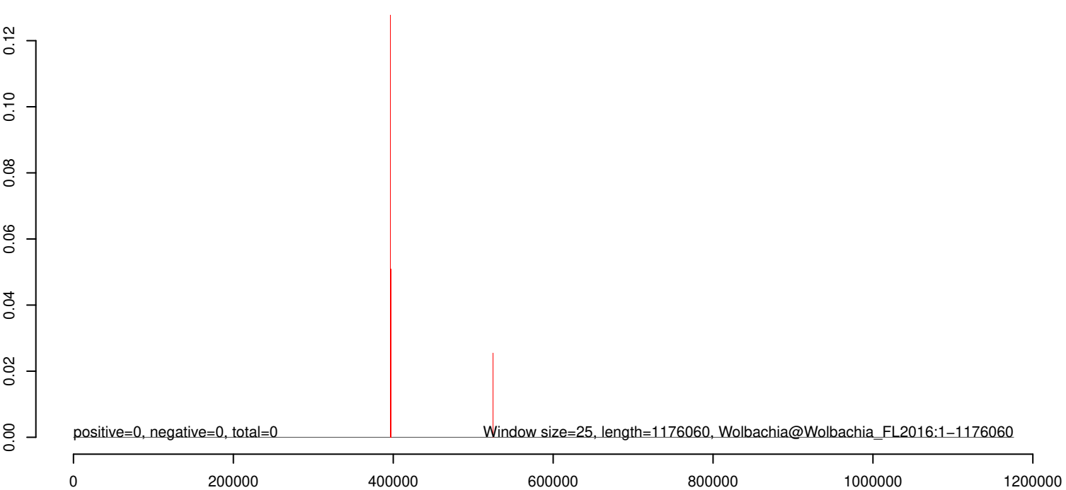
AeAlbo_BUNV_U4.4_rep2_ES.rep
