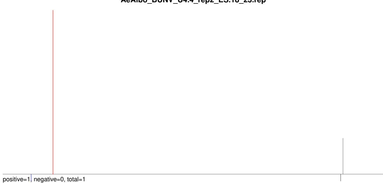
AeAlbo_BUNV_U4.4_rep2_ES.24_35.rep
