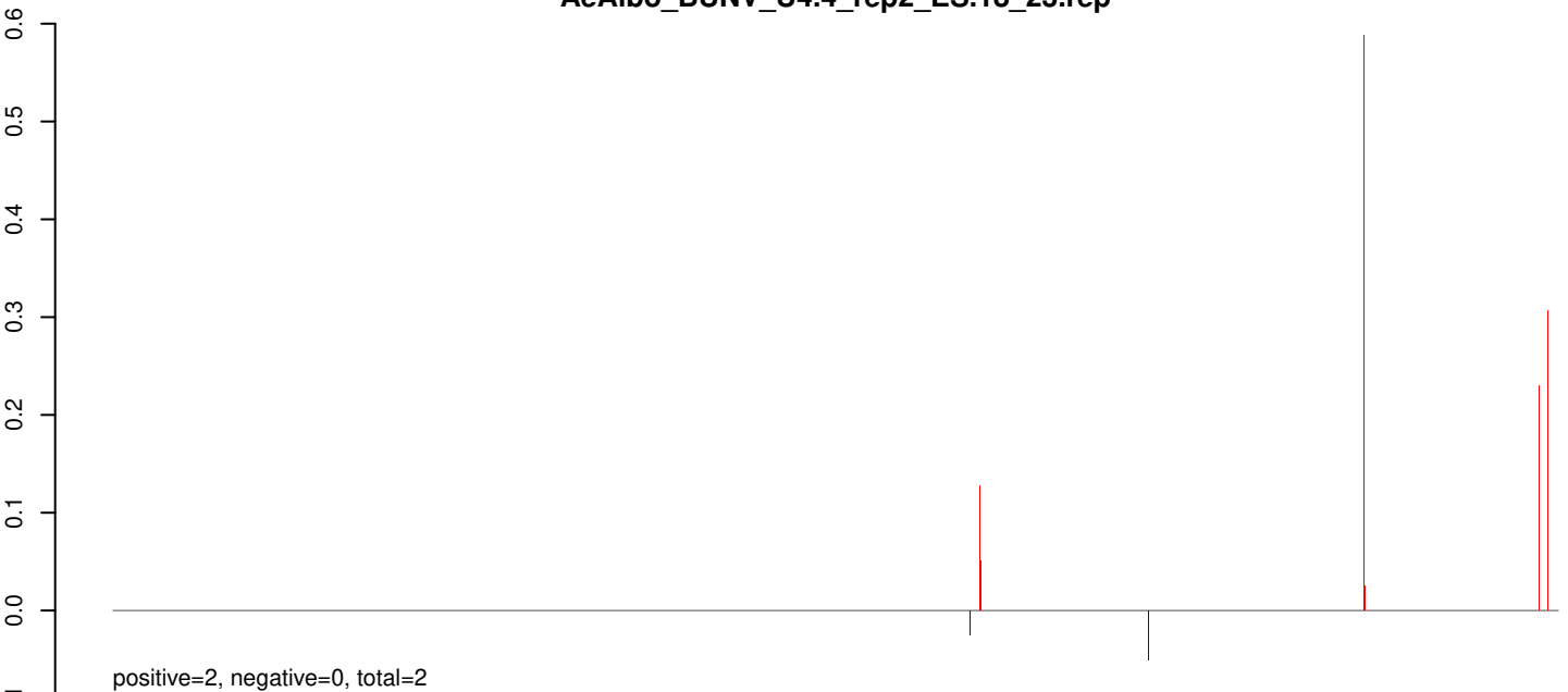
AeAlbo_BUNV_U4.4_rep2_ES.24_35.rep
