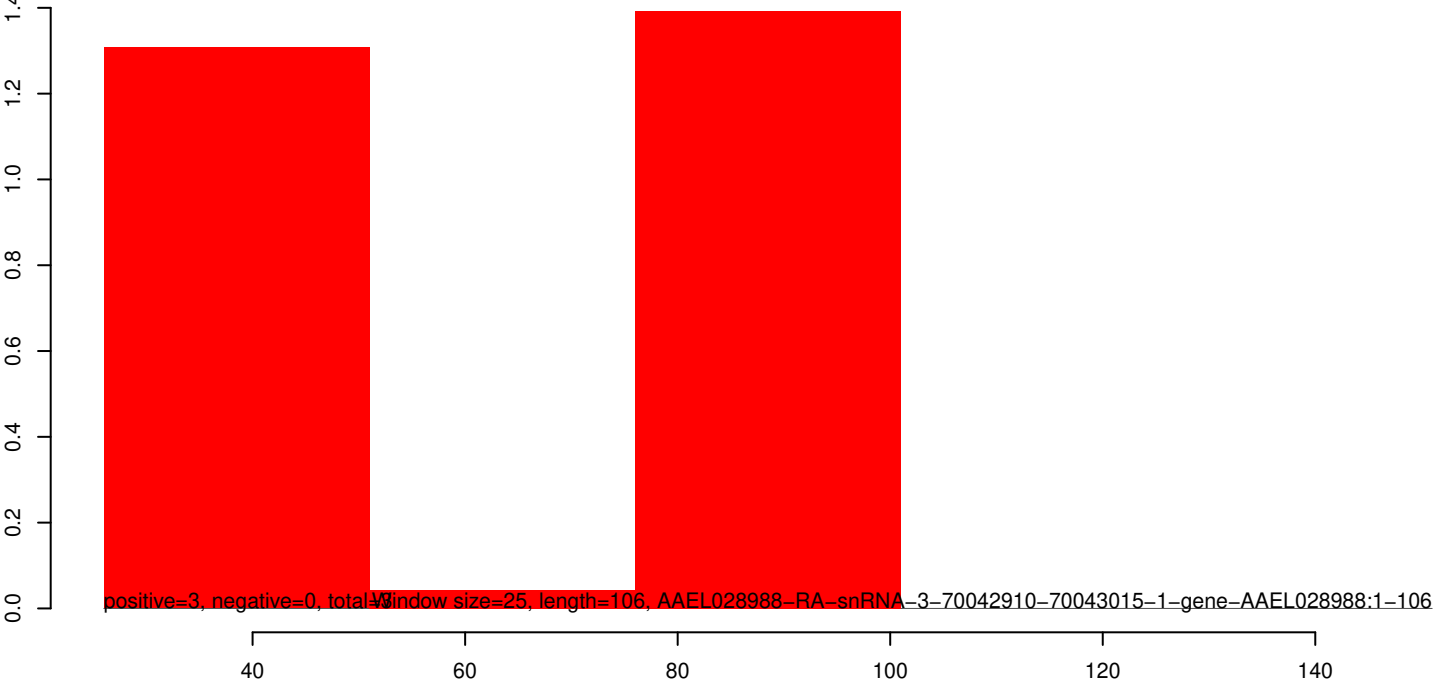
AeAlbo_VietMcar_AEFV_MERV_SHTV_YS.rep
