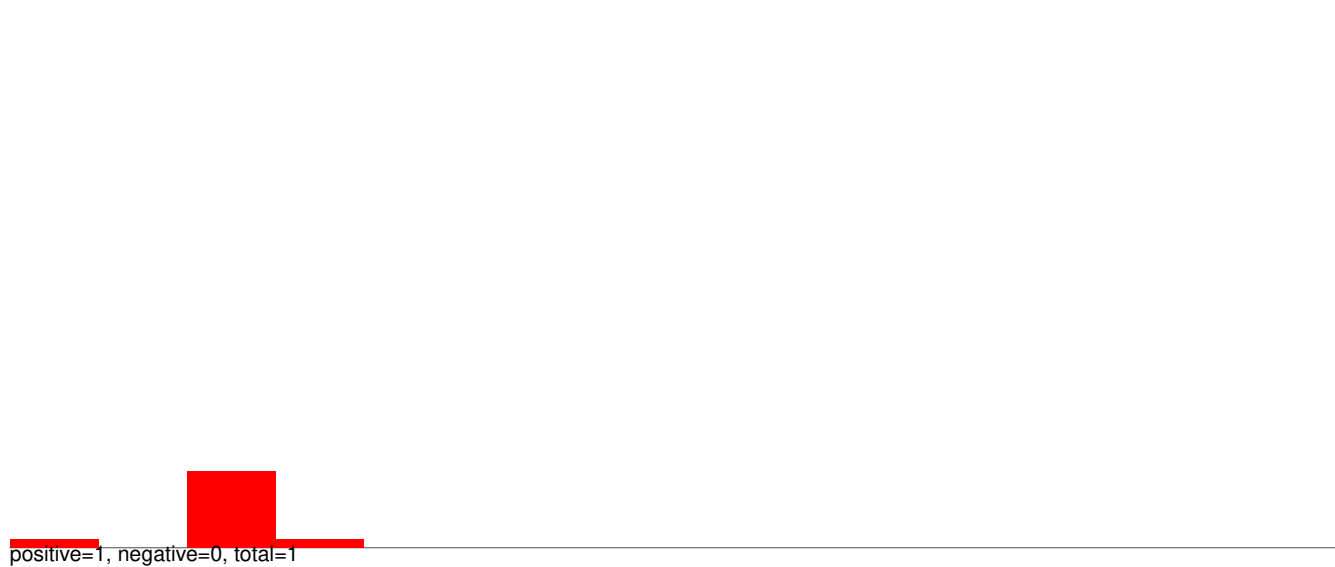
AeAlbo_VietMcar_AEFV_MERV_SHTV_YS.rep
