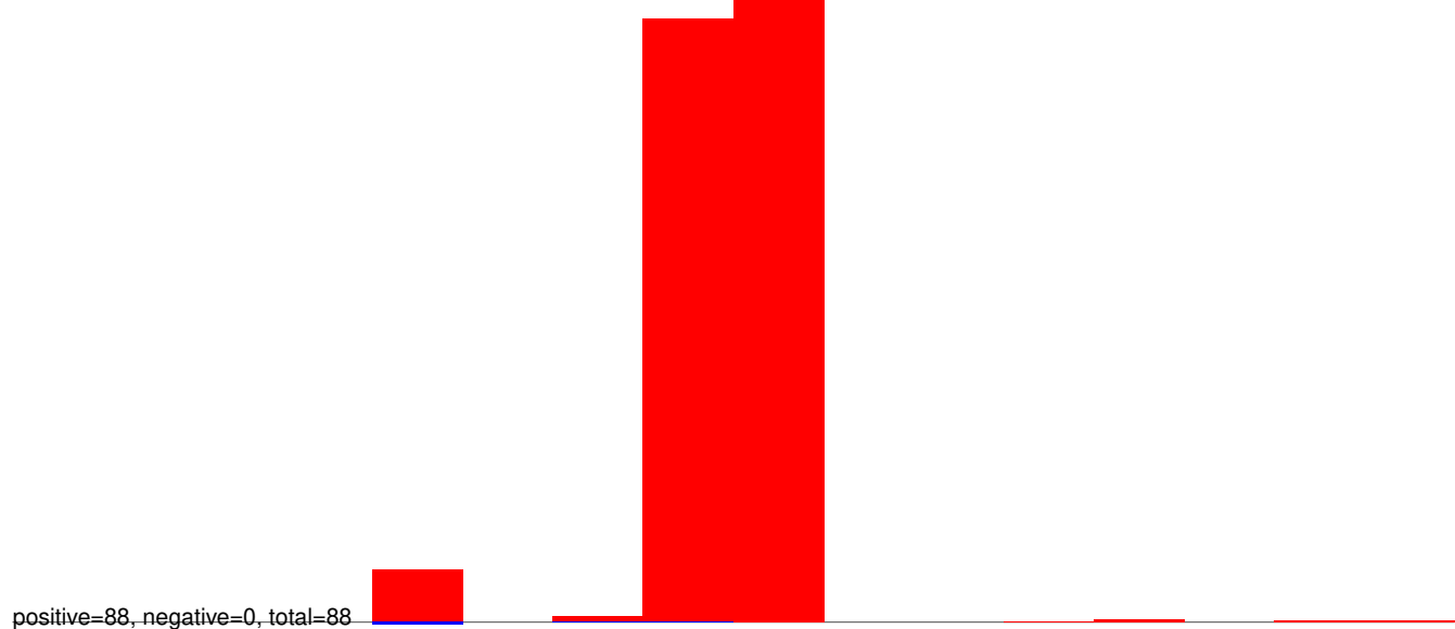
AeAlbo_VietMcar_AEFV_MERV_SHTV_YS.24_35.rep
