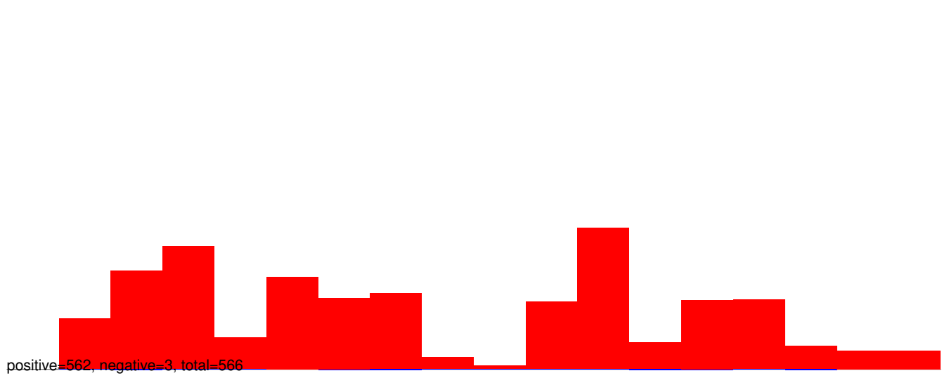
AeAlbo_VietMcar_AEFV_MERV_SHTV_YS.24_35.rep
