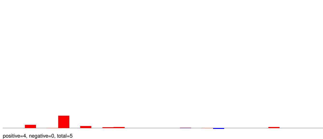
AeAlbo_VietMcar_AEFV_MERV_SHTV_YS.rep
