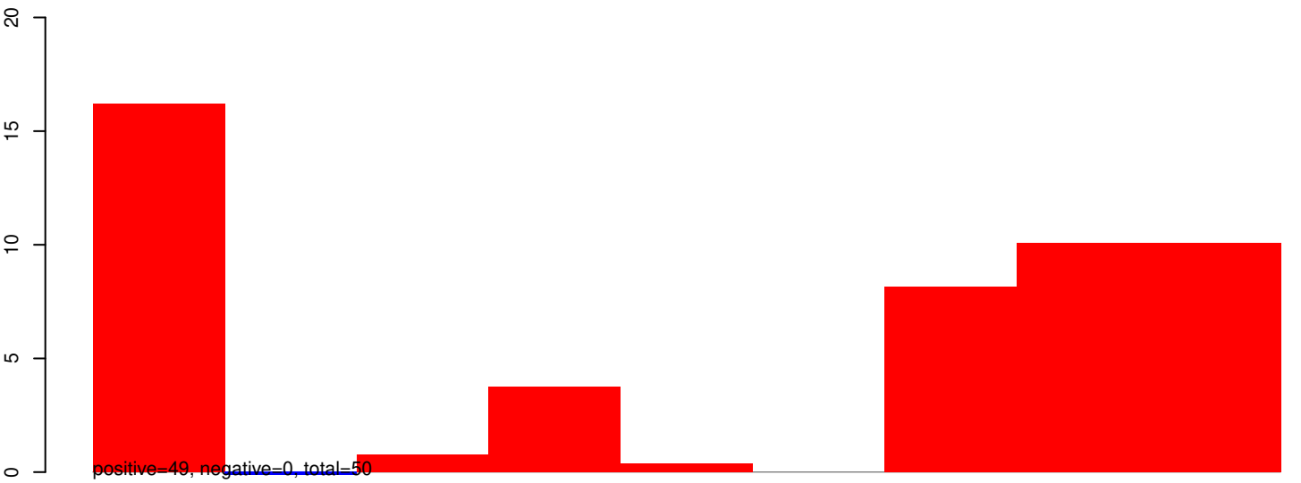
AeAlbo_VietMcar_AEFV_MERV_SHTV_YS.24_35.rep
