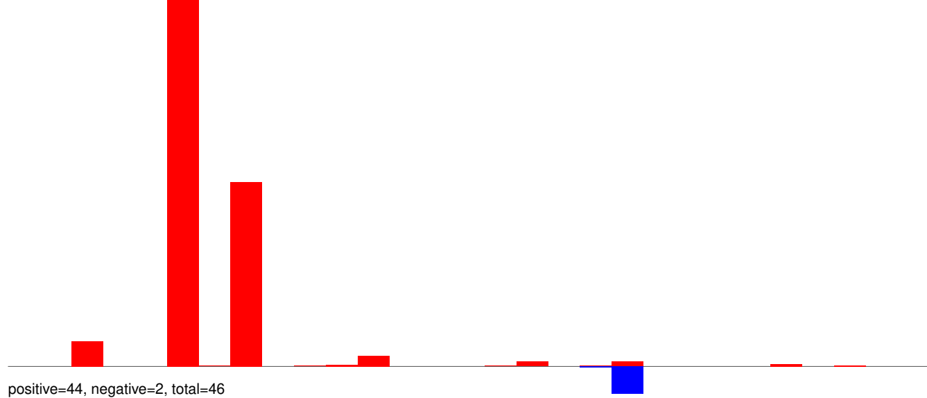
AeAlbo_VietMcar_AEFV_MERV_SHTV_YS.24_35.rep
