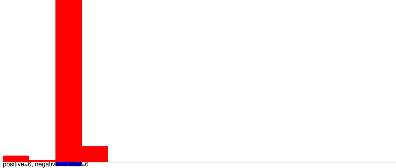
AeAlbo_VietMcar_AEFV_MERV_SHTV_YS.24_35.rep
