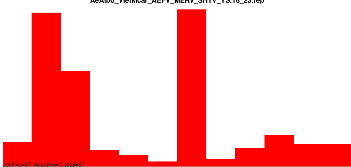
AeAlbo_VietMcar_AEFV_MERV_SHTV_YS.24_35.rep
