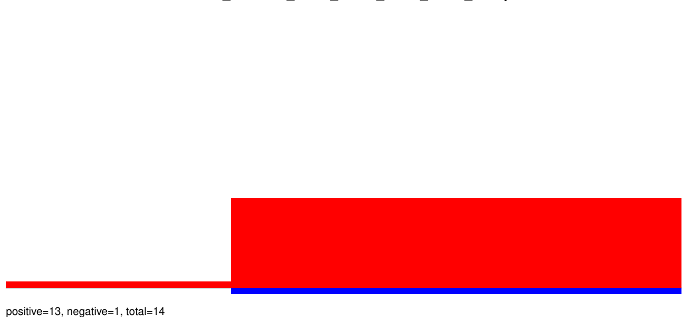
AeAlbo_VietMcar_AEFV_MERV_SHTV_YS.24_35.rep
