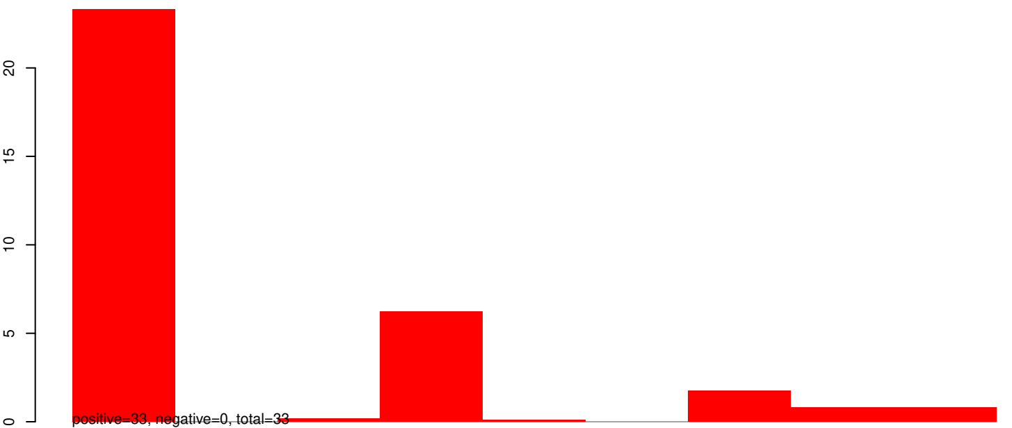
AeAlbo_VietMcar_AEFV_MERV_SHTV_YS.rep
