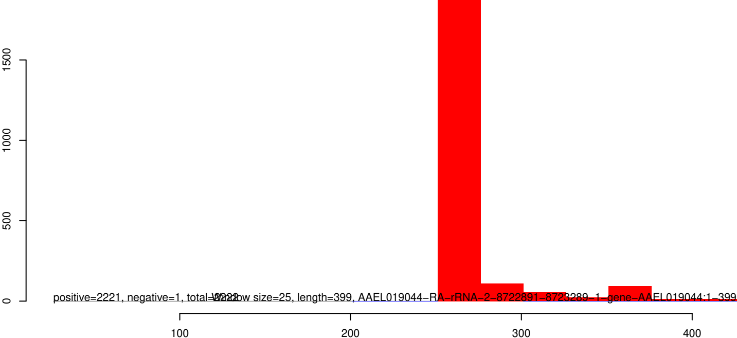
AeAlbo_VietMcar_AEFV_MERV_SHTV_YS.rep
