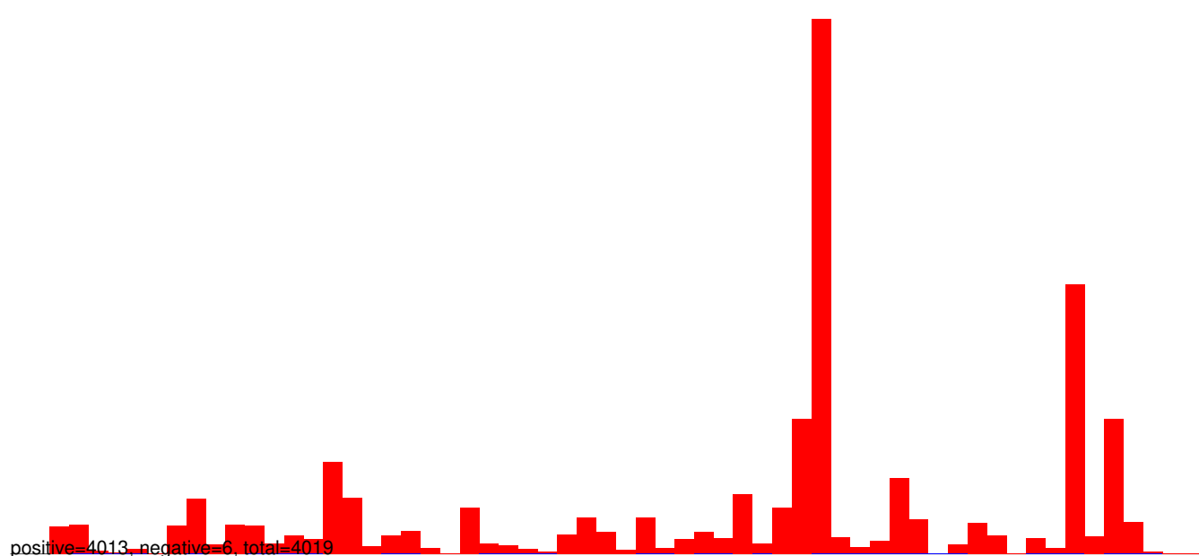
AeAlbo_VietMcar_AEFV_MERV_SHTV_YS.24_35.rep
