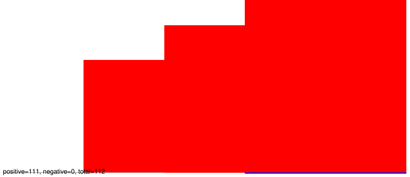
AeAlbo_VietMcar_AEFV_MERV_SHTV_YS.24_35.rep
