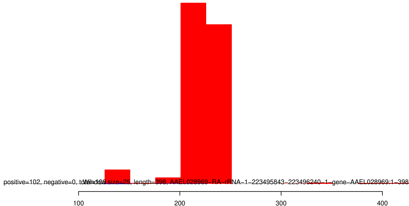
AeAlbo_VietMcar_AEFV_MERV_SHTV_YS.rep
