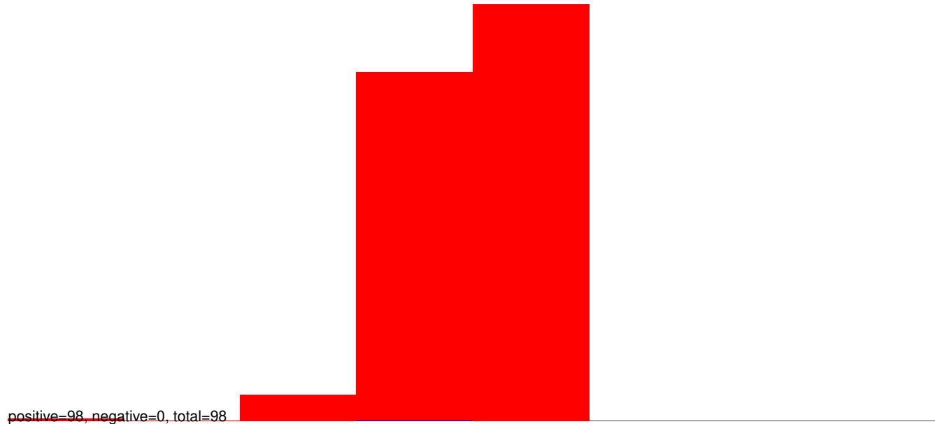
AeAlbo_VietMcar_AEFV_MERV_SHTV_YS.24_35.rep
