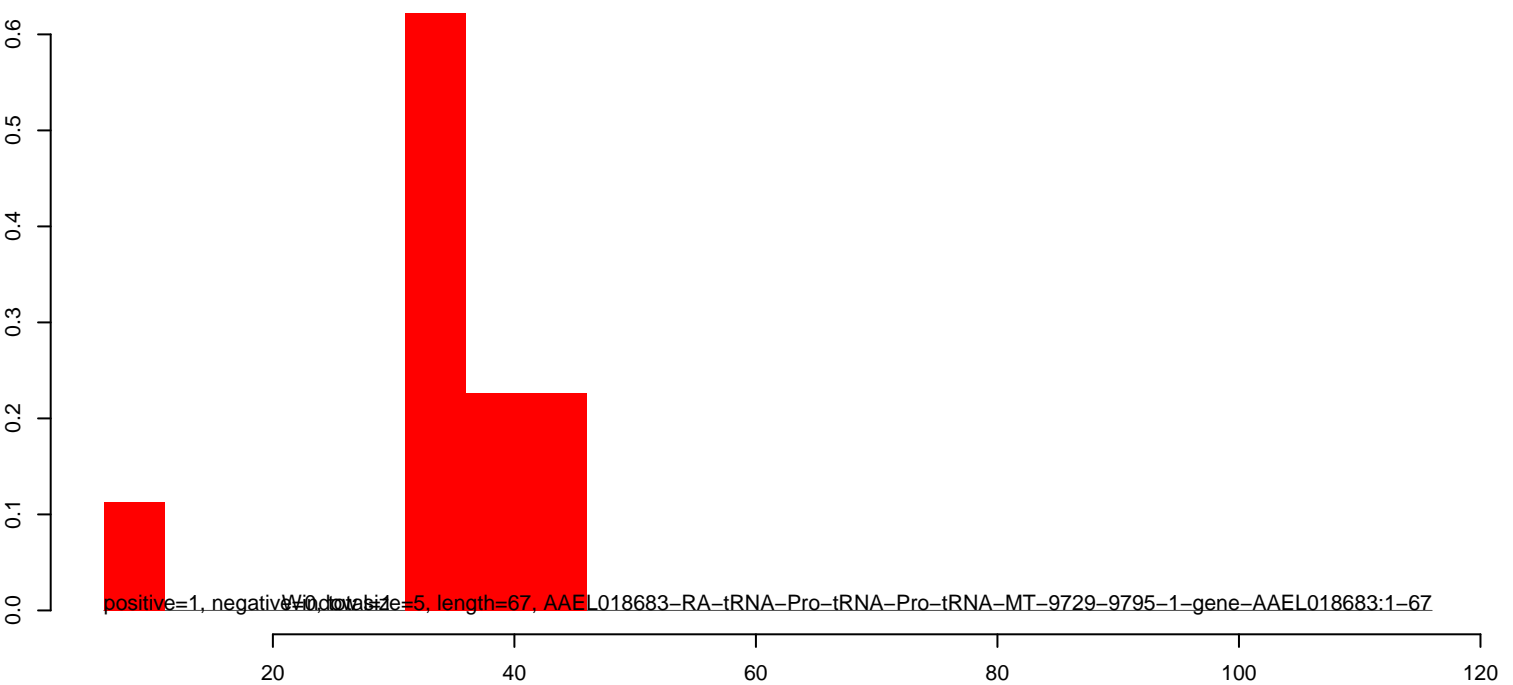
AeAlbo_C636HT_DENV2_Acute.rep
