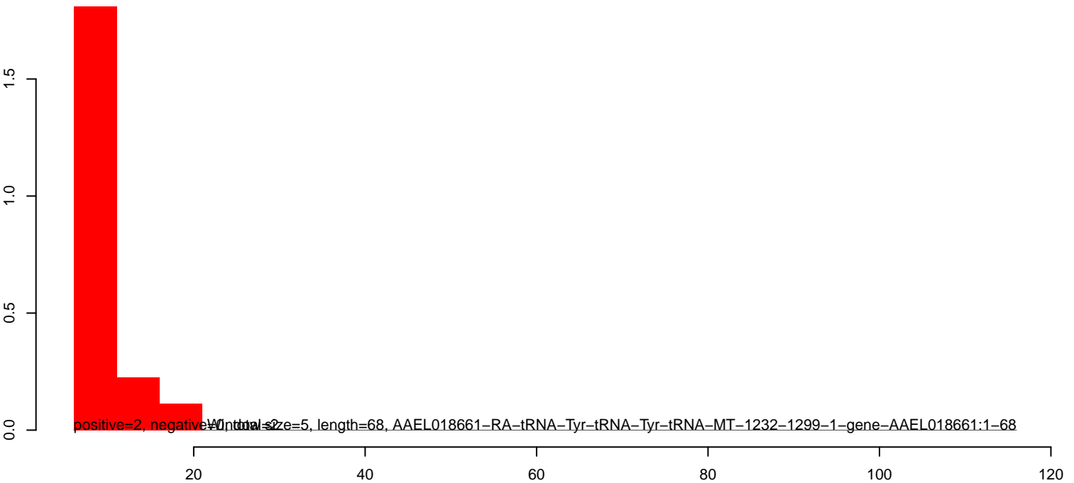
AeAlbo_C636HT_DENV2_Acute.rep
