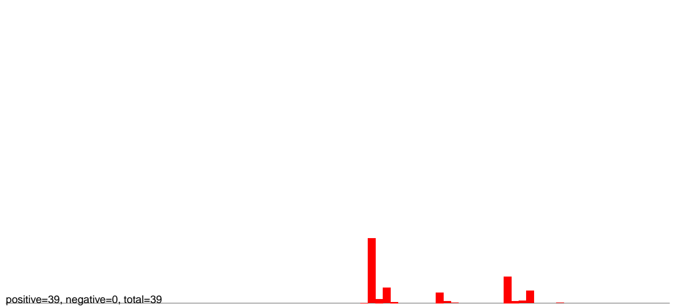
AeAlbo_C636HT_DENV2_Acute.rep
