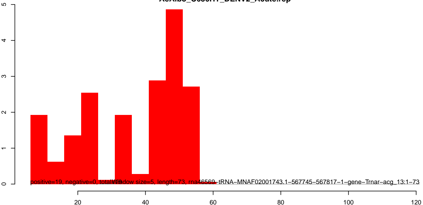
AeAlbo_C636HT_DENV2_Acute.rep
