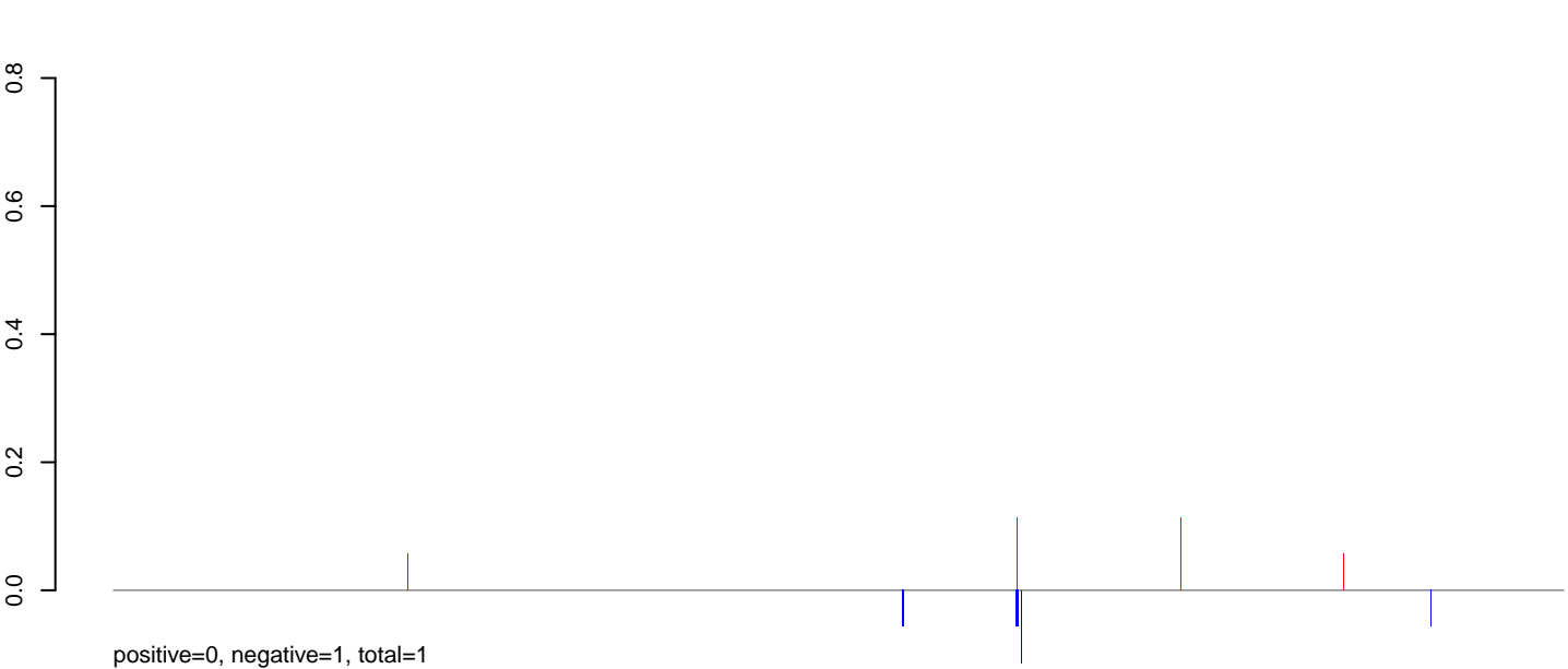
AeAlbo_C636HT_DENV2_Acute.rep
