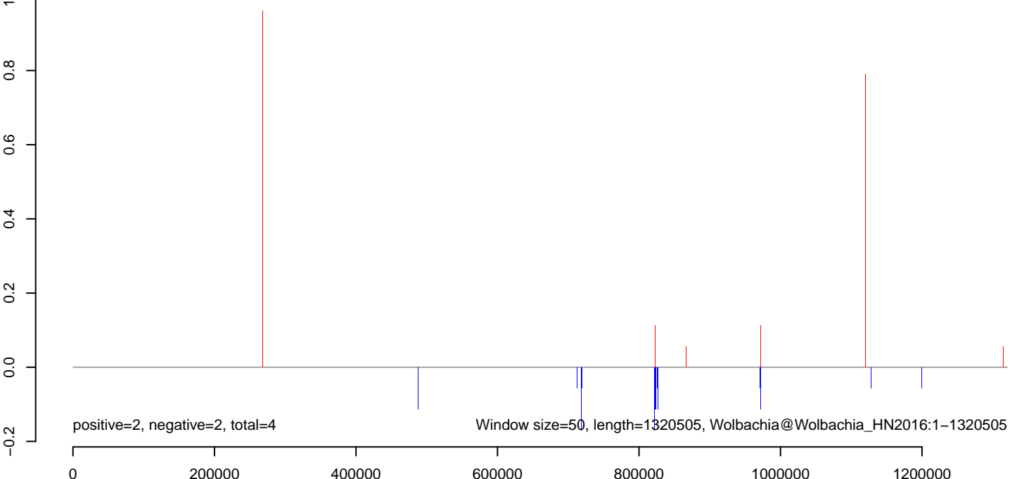
AeAlbo_C636HT_DENV2_Acute.rep
