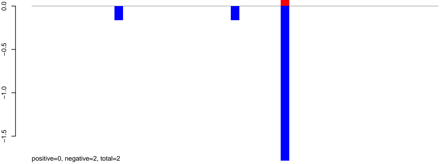
AeAlbo_C636_6dpi_SINV1.24_35.rep
