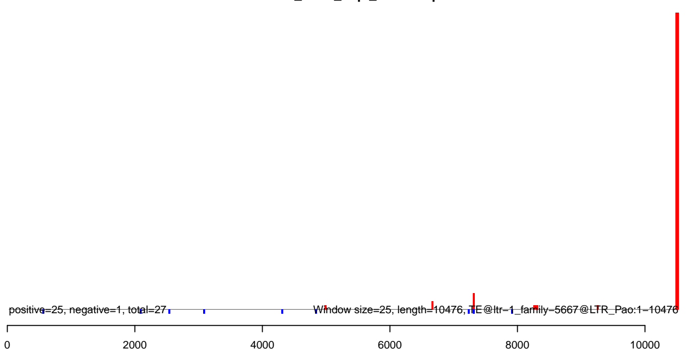
AeAlbo_C636_6dpi_SINV1.rep
