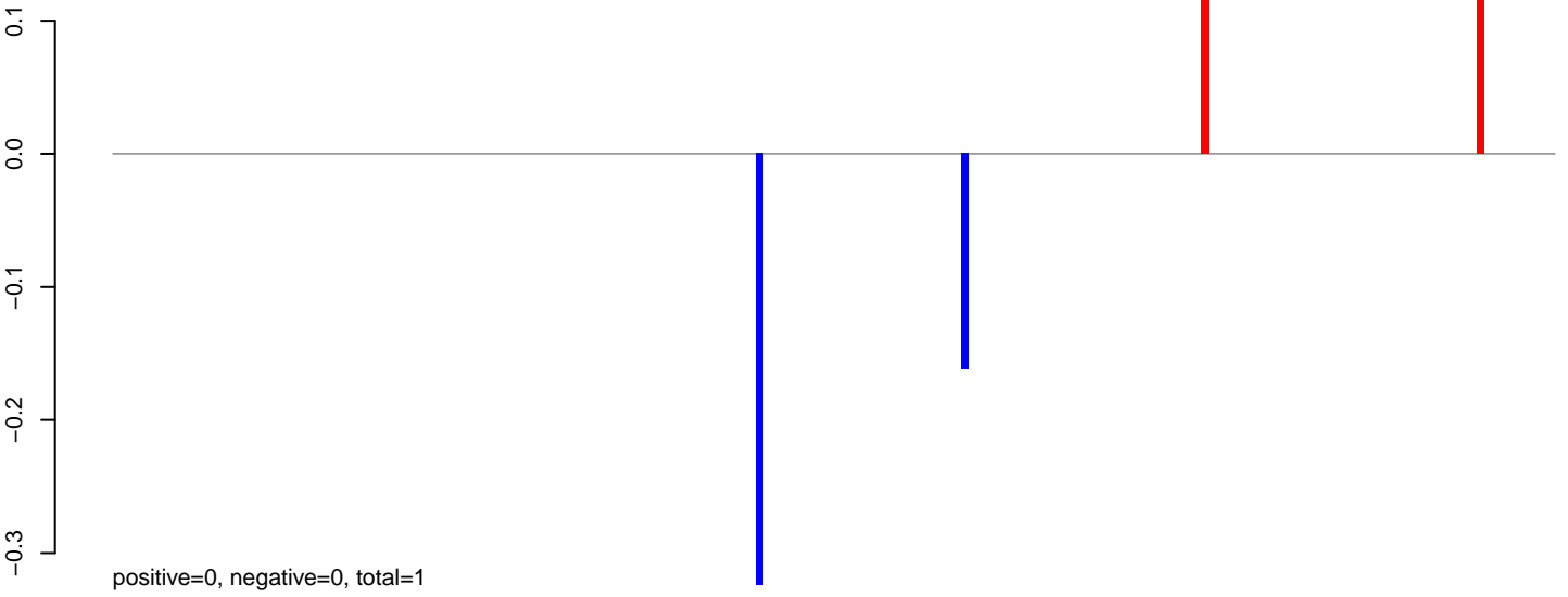
AeAlbo_C636_6dpi_SINV1.24_35.rep
