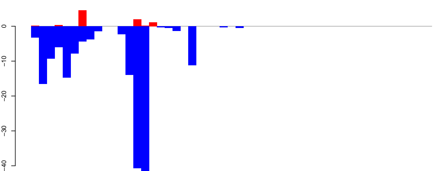
AeAlbo_C636_6dpi_SINV1.24_35.rep
