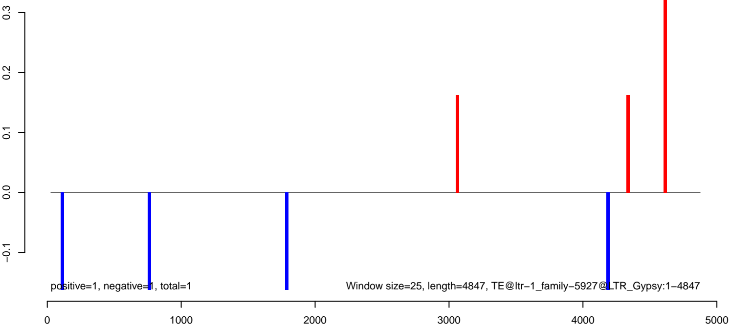
AeAlbo_C636_6dpi_SINV1.rep
