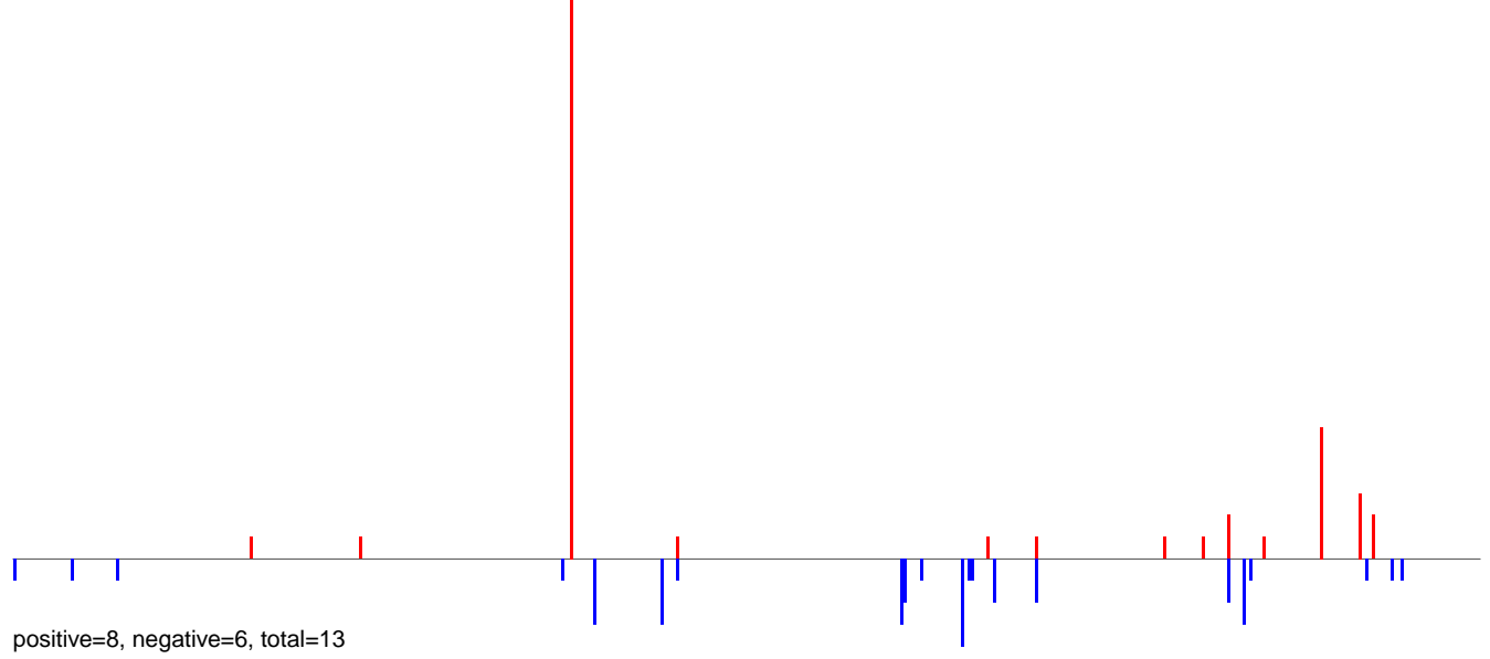
AeAlbo_C636_6dpi_SINV1.24_35.rep
