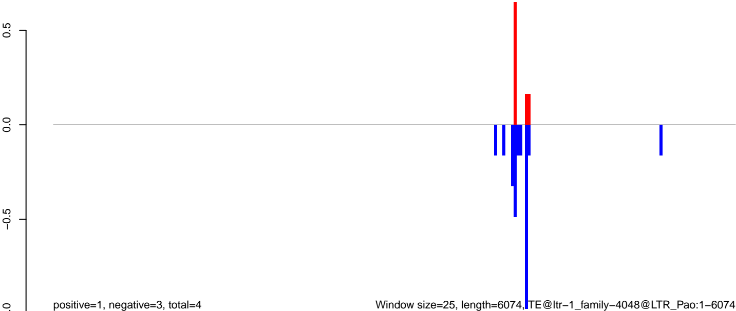
AeAlbo_C636_6dpi_SINV1.rep
