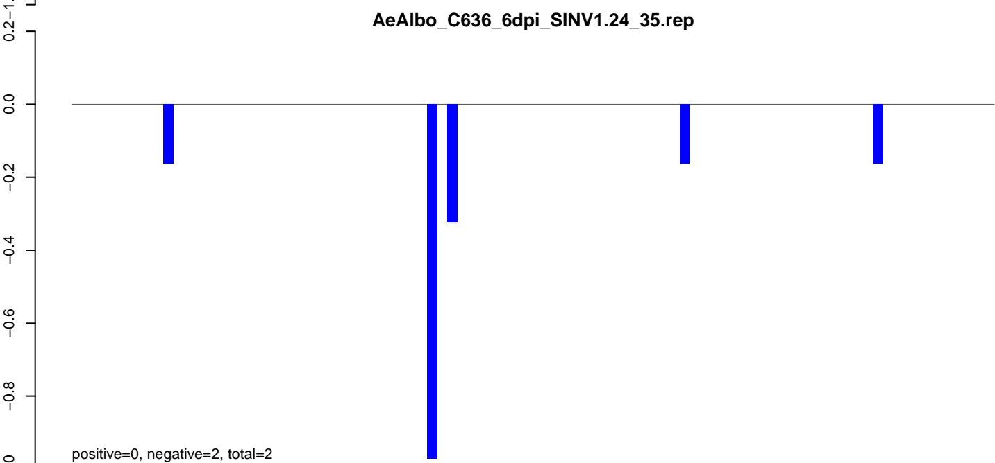
AeAlbo_C636_6dpi_SINV1.rep
