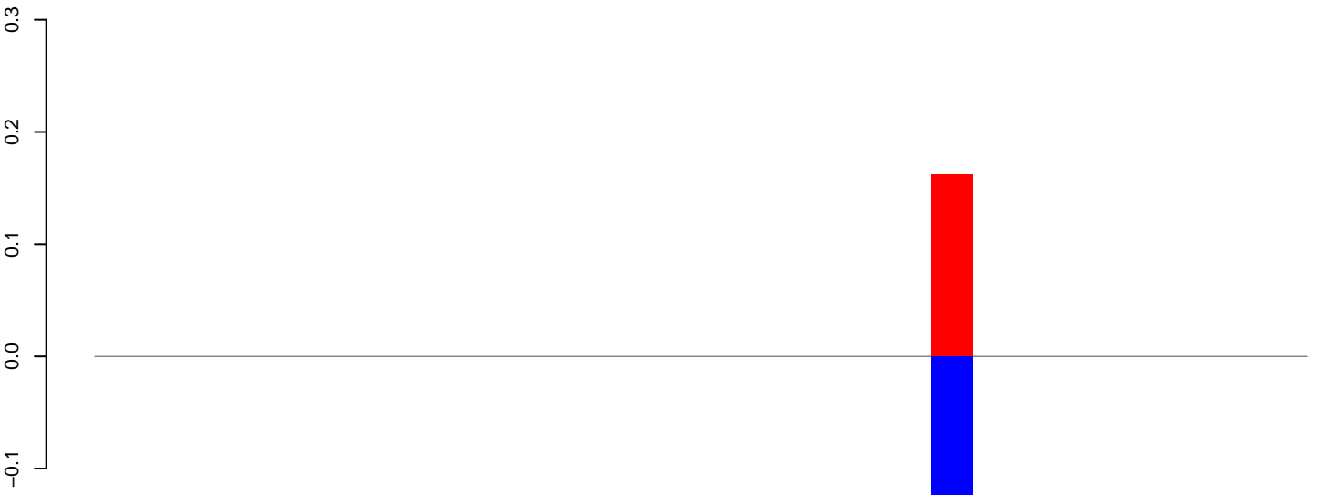
AeAlbo_C636_6dpi_SINV1.24_35.rep
