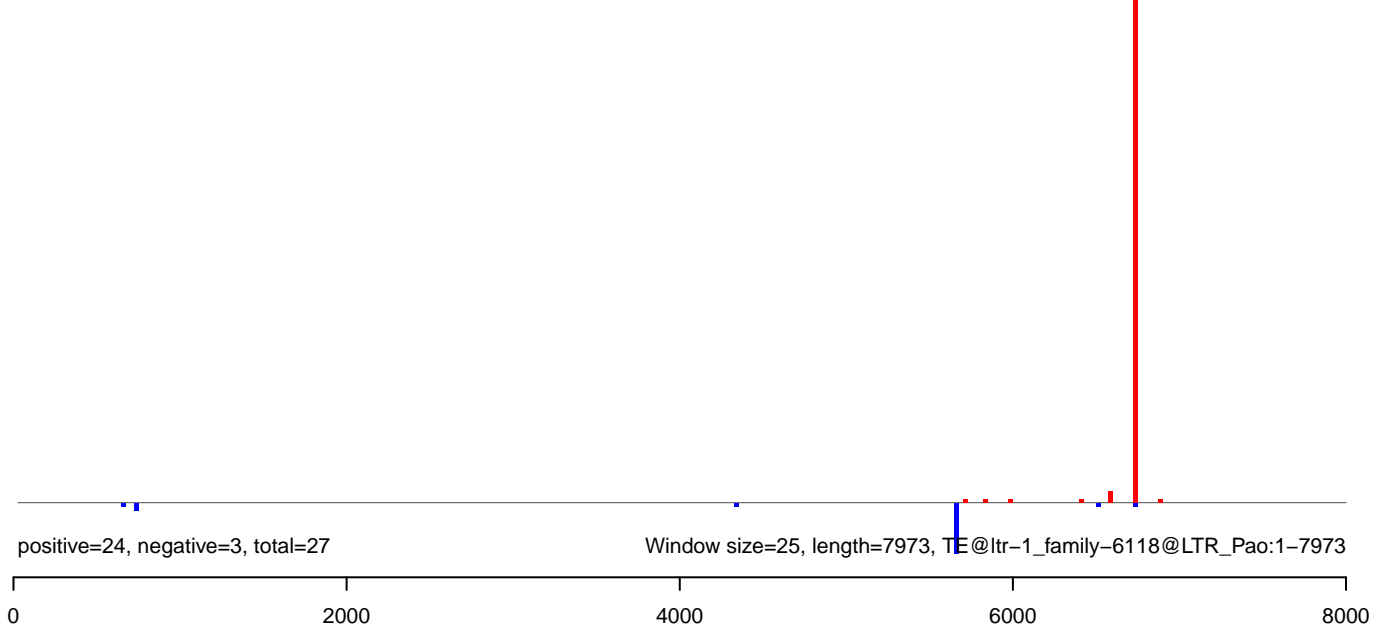
AeAlbo_C636_6dpi_SINV1.rep
