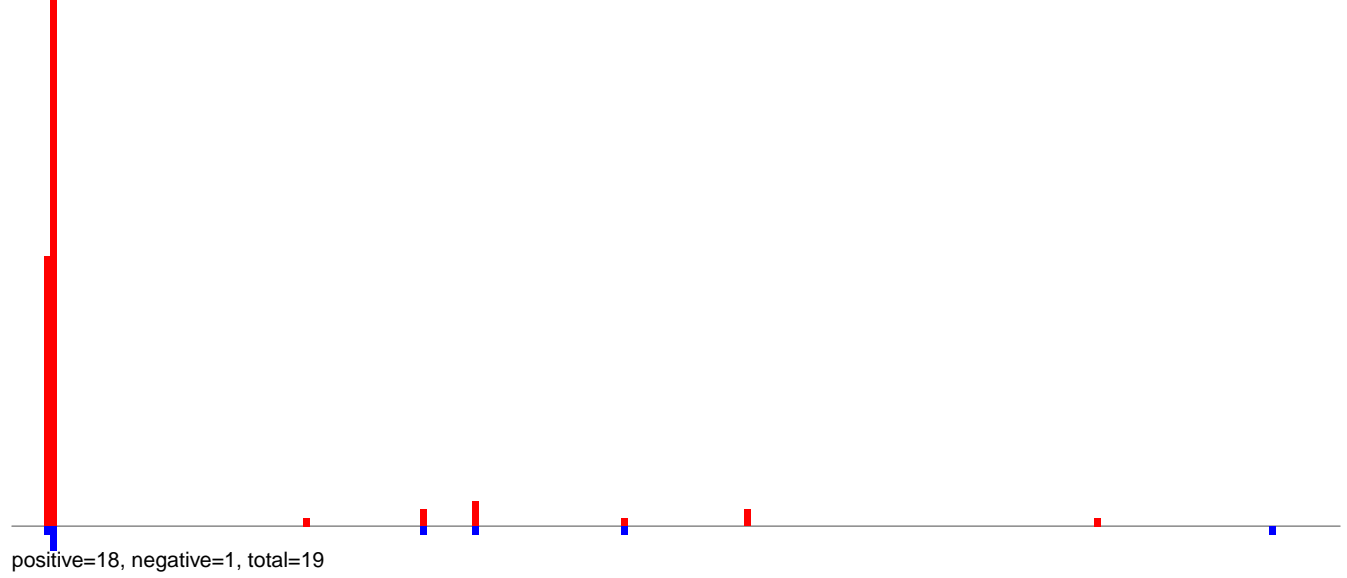
AeAlbo_C636_6dpi_SINV1.24_35.rep
