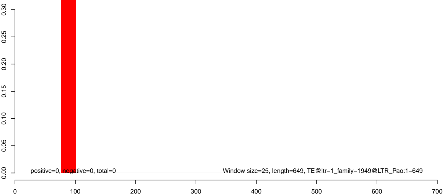
AeAlbo_C636_6dpi_SINV1.rep
