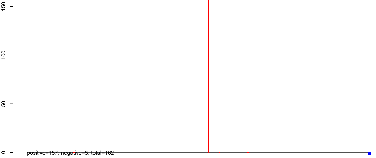
AeAlbo_C636_6dpi_SINV1.24_35.rep
