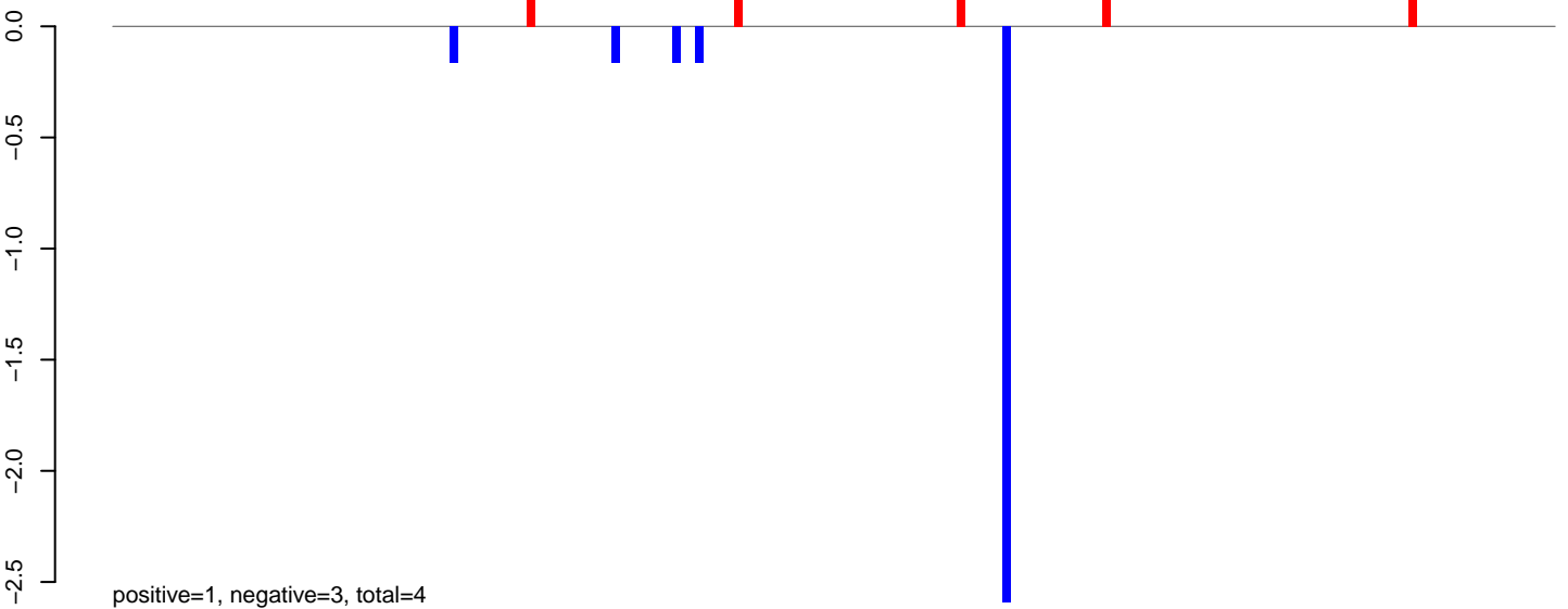
AeAlbo_C636_6dpi_SINV1.24_35.rep
