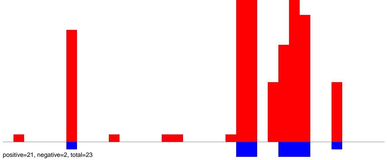
AeAlbo_C636_6dpi_SINV1.24_35.rep
