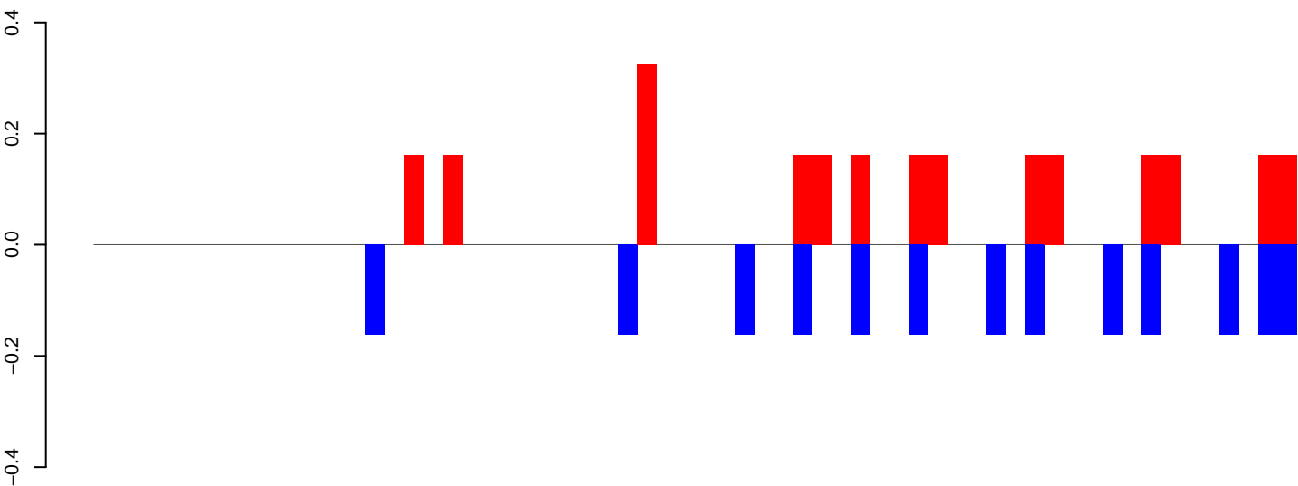
AeAlbo_C636_6dpi_SINV1.24_35.rep
