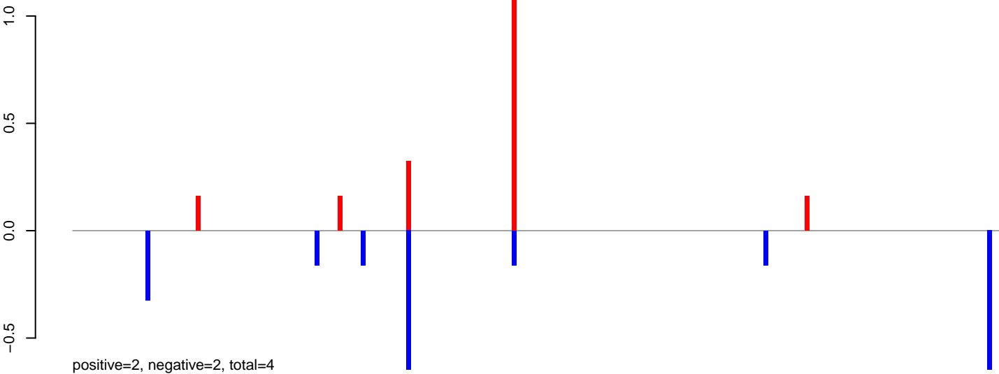
AeAlbo_C636_6dpi_SINV1.24_35.rep
