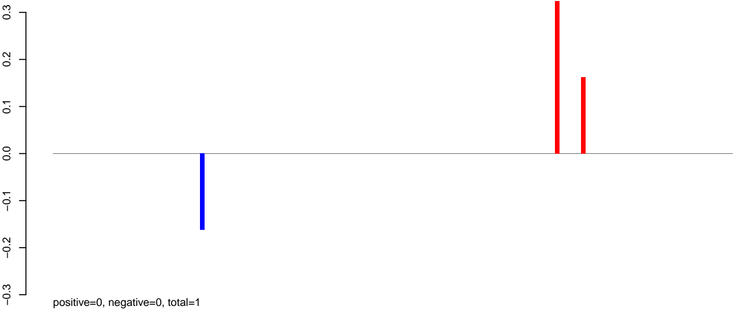
AeAlbo_C636_6dpi_SINV1.rep
