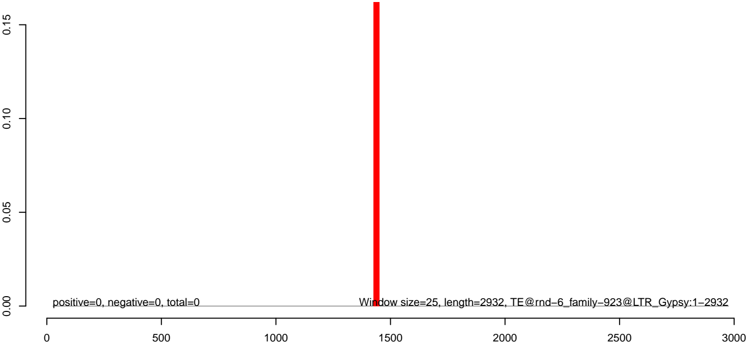
AeAlbo_C636_6dpi_SINV1.rep
