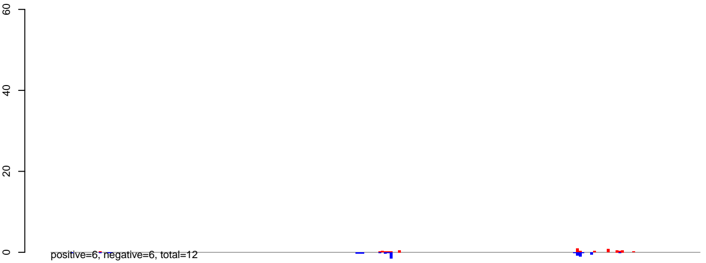
AeAlbo_C636_6dpi_SINV1.rep
