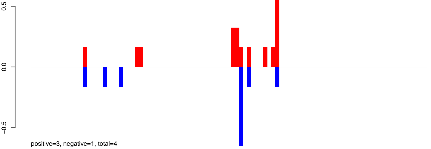
AeAlbo_C636_6dpi_SINV1.24_35.rep
