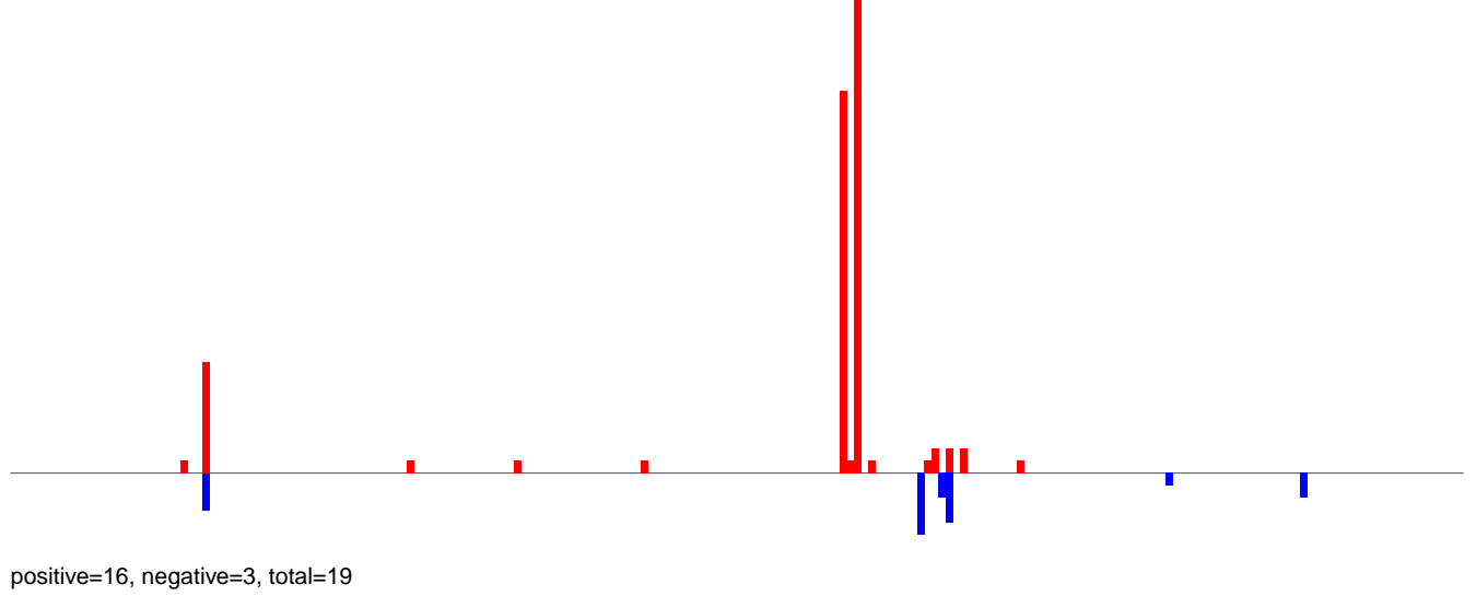
AeAlbo_C636_6dpi_SINV1.24_35.rep
