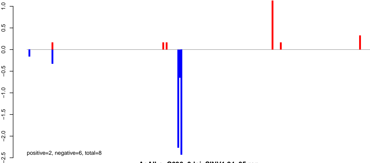
AeAlbo_C636_6dpi_SINV1.24_35.rep
