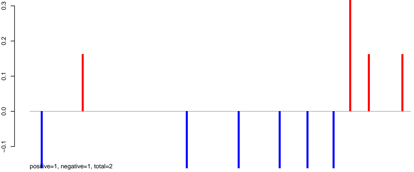
AeAlbo_C636_6dpi_SINV1.24_35.rep
