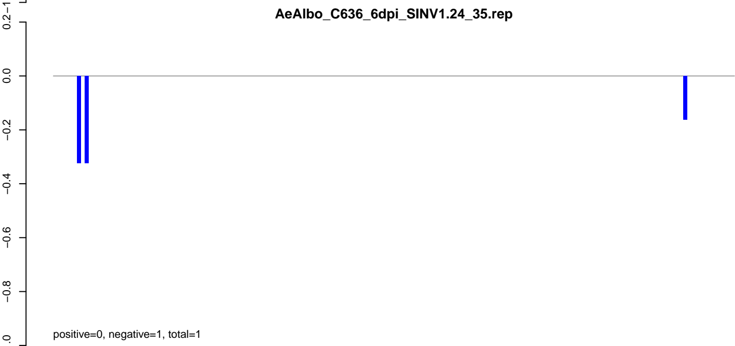
AeAlbo_C636_6dpi_SINV1.rep
