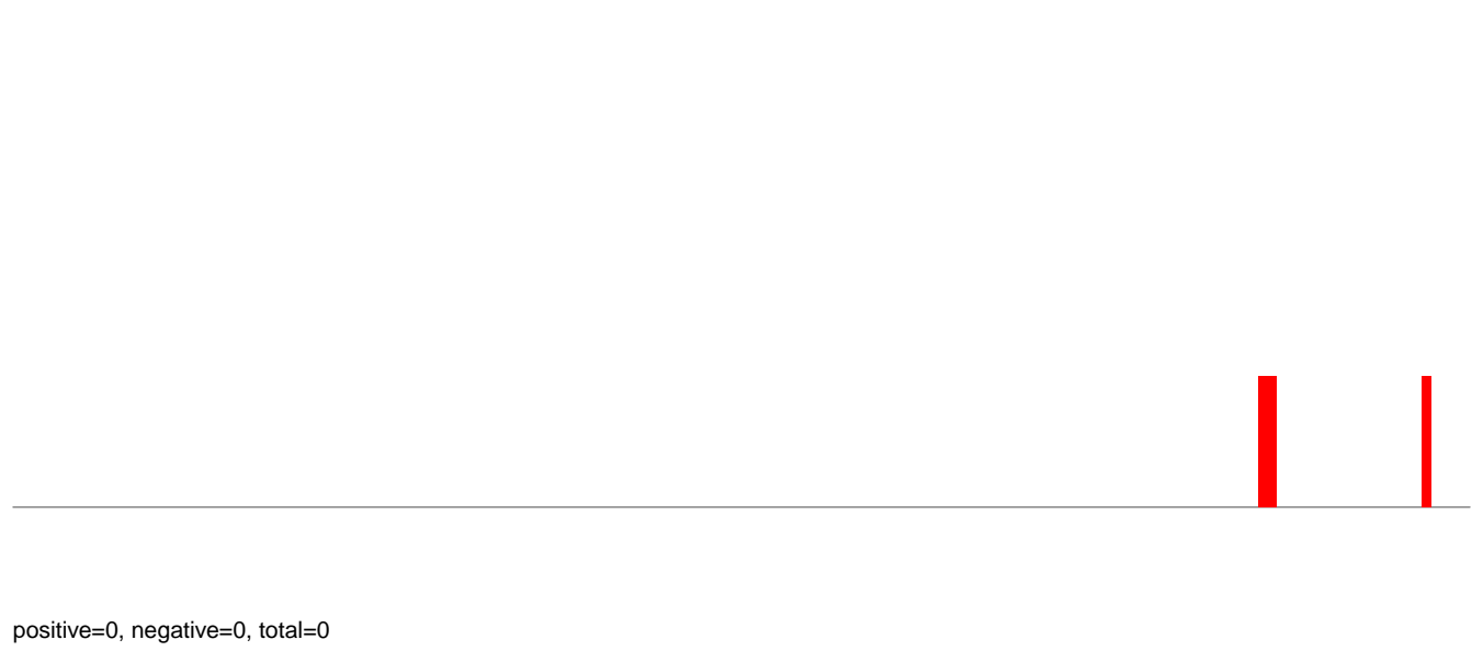
AeAlbo_C636_6dpi_SINV1.rep
