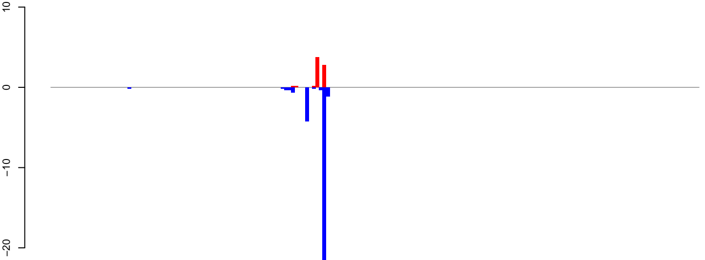
AeAlbo_C636_6dpi_SINV1.24_35.rep
