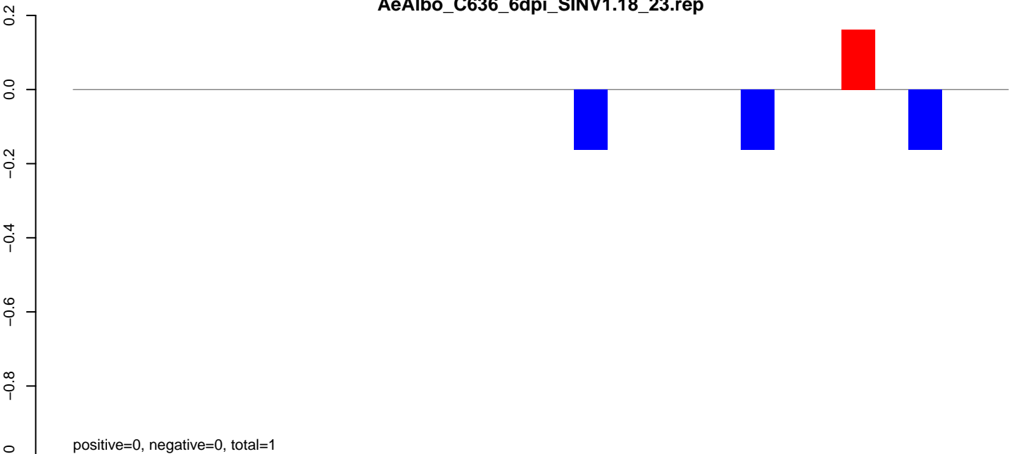
AeAlbo_C636_6dpi_SINV1.24_35.rep
