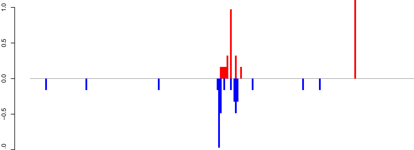
AeAlbo_C636_6dpi_SINV1.24_35.rep
