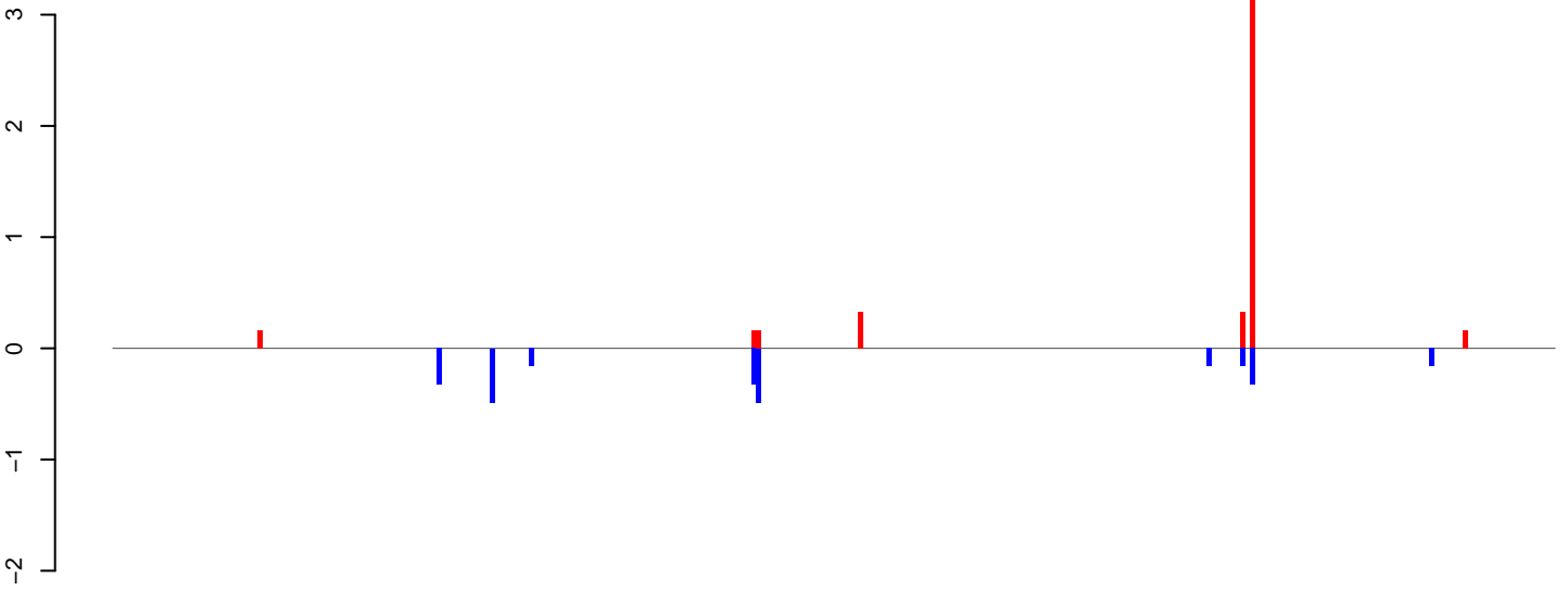
AeAlbo_C636_6dpi_SINV1.18_23.rep
