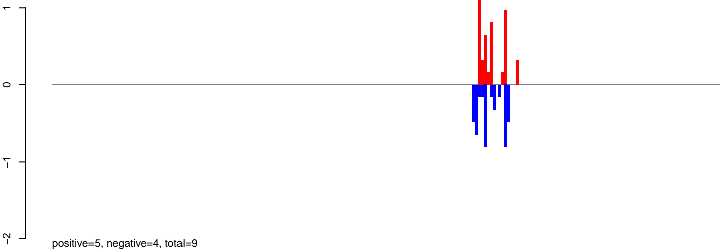
AeAlbo_C636_6dpi_SINV1.rep
