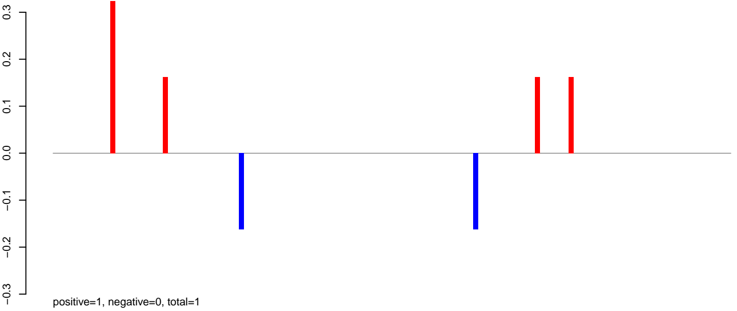
AeAlbo_C636_6dpi_SINV1.24_35.rep
