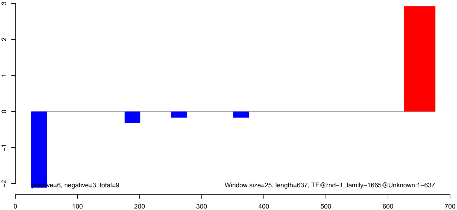
AeAlbo_C636_6dpi_SINV1.rep
