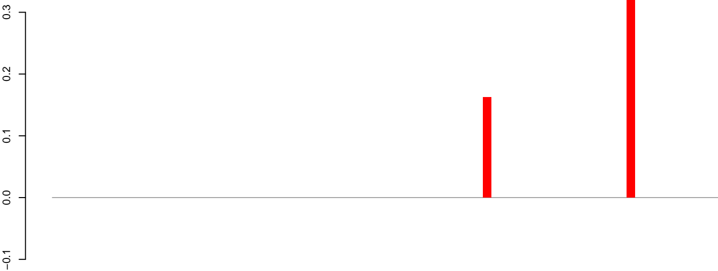
AeAlbo_C636_6dpi_SINV1.18_23.rep
