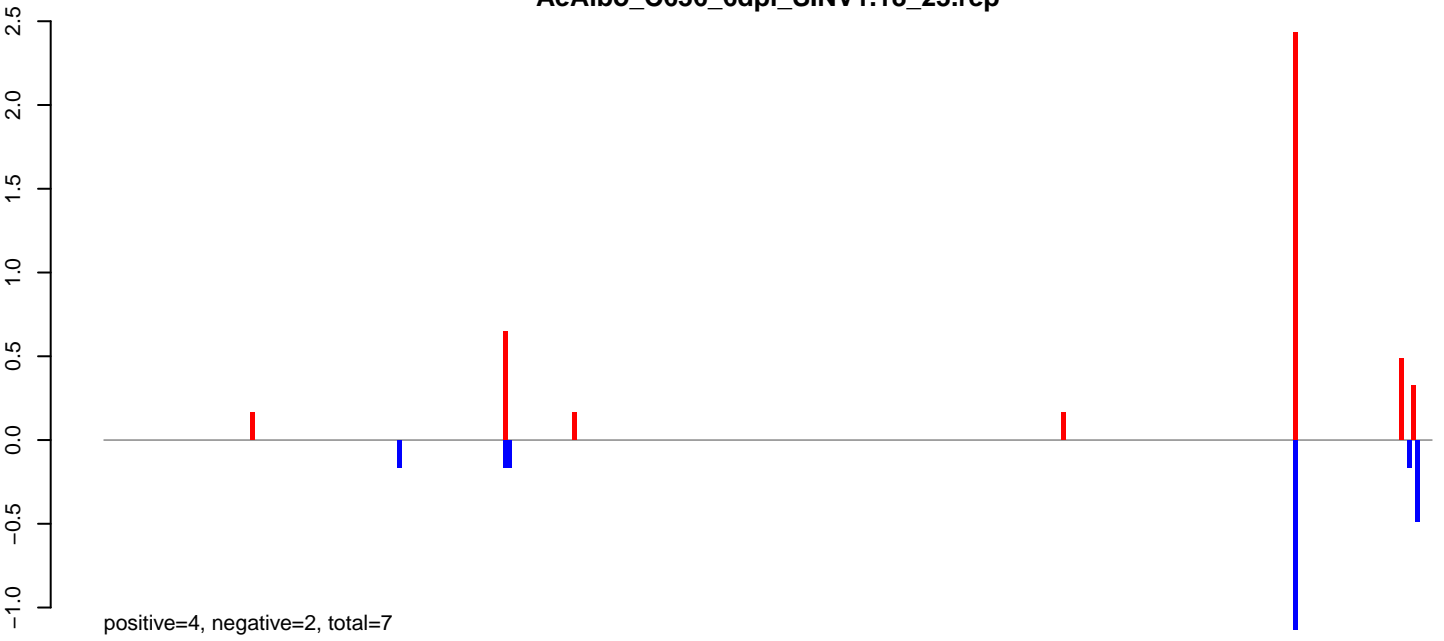
AeAlbo_C636_6dpi_SINV1.24_35.rep
