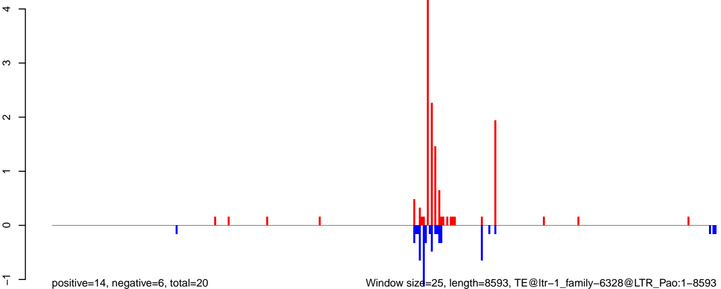
AeAlbo_C636_6dpi_SINV1.rep
