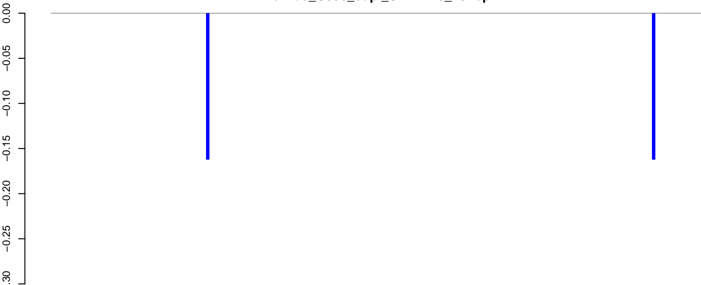
AeAlbo_C636_6dpi_SINV1.18_23.rep
