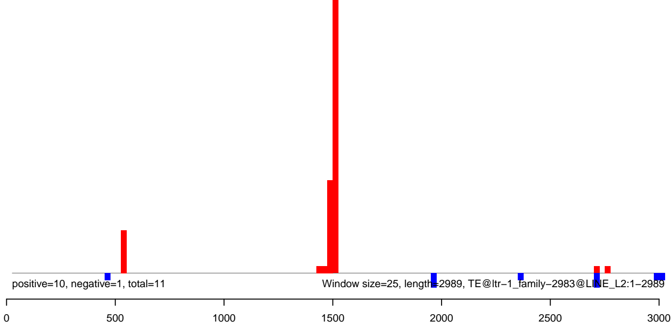
AeAlbo_C636_6dpi_SINV1.rep
