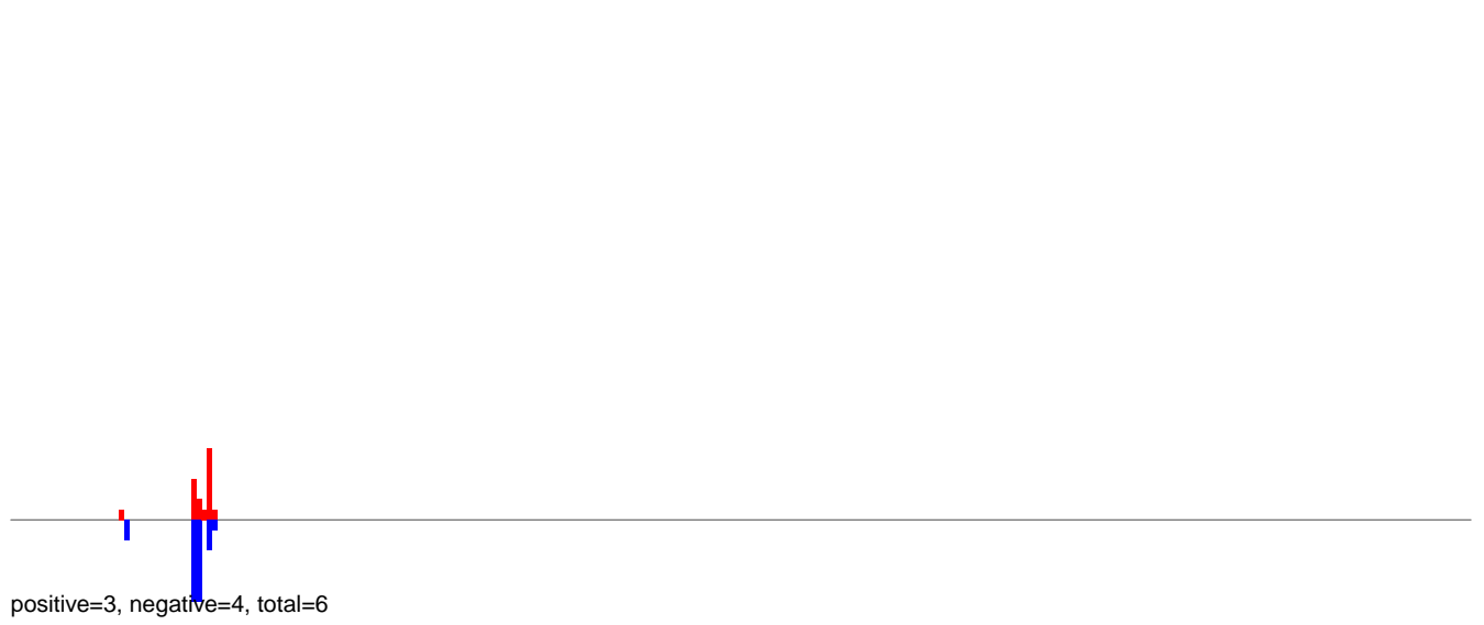
AeAlbo_C636_6dpi_SINV1.rep
