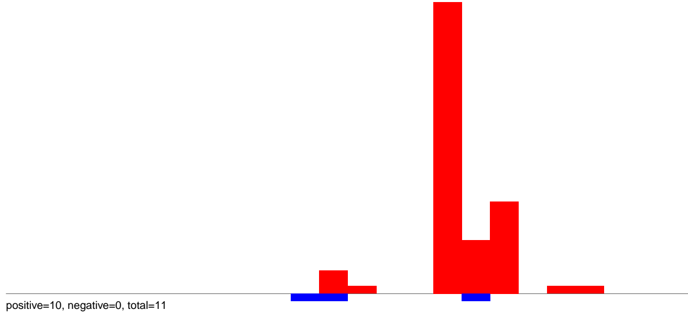
AeAlbo_C636_6dpi_SINV1.rep
