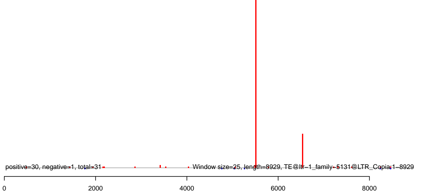
AeAlbo_C636_6dpi_SINV1.rep
