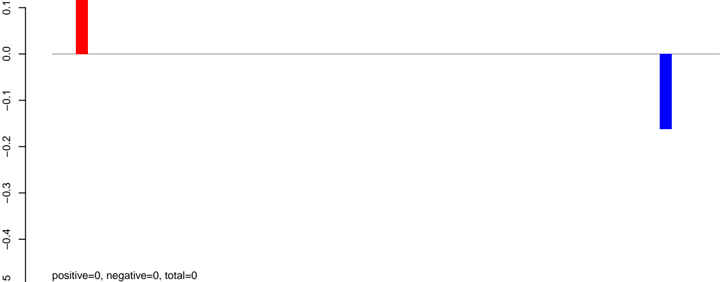
AeAlbo_C636_6dpi_SINV1.rep
