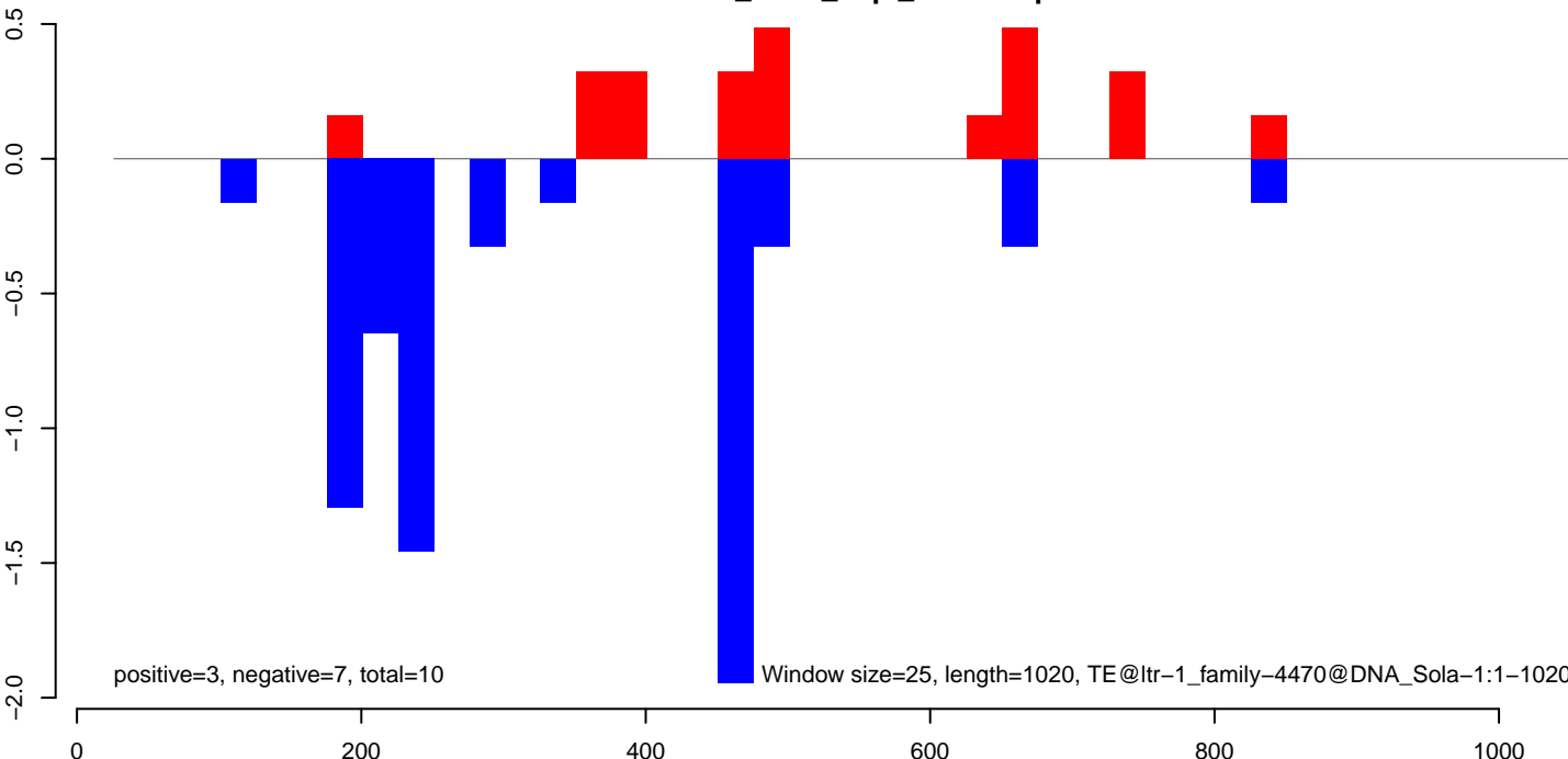
AeAlbo_C636_6dpi_SINV1.rep
