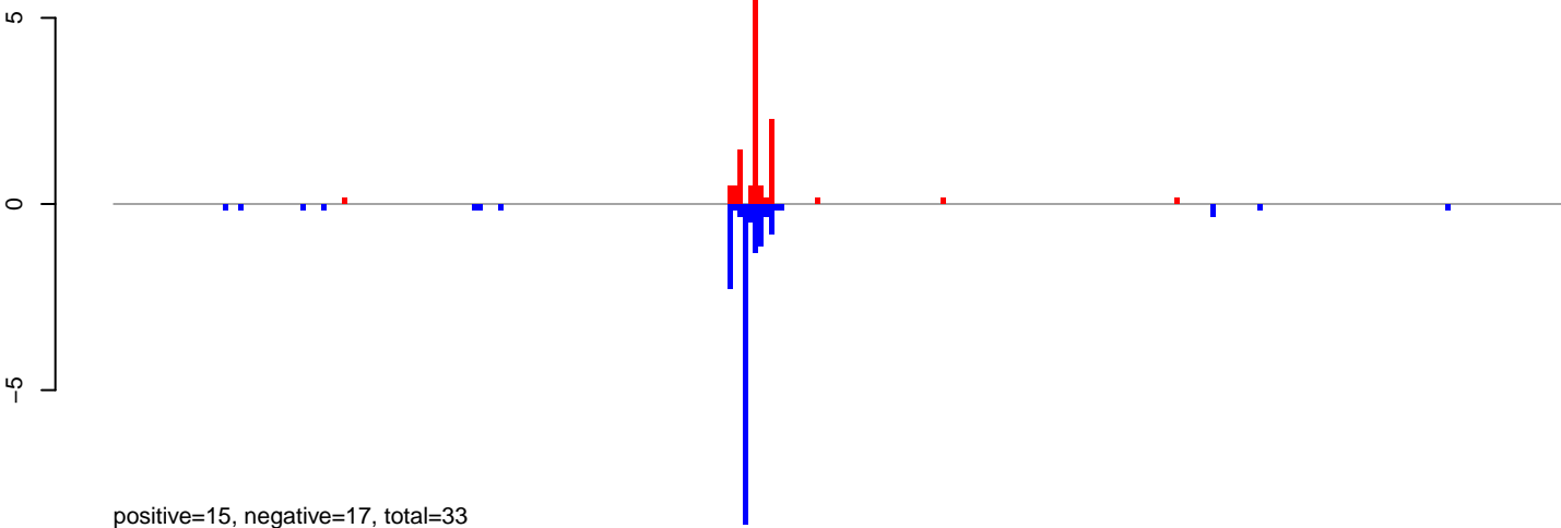
AeAlbo_C636_6dpi_SINV1.24_35.rep
