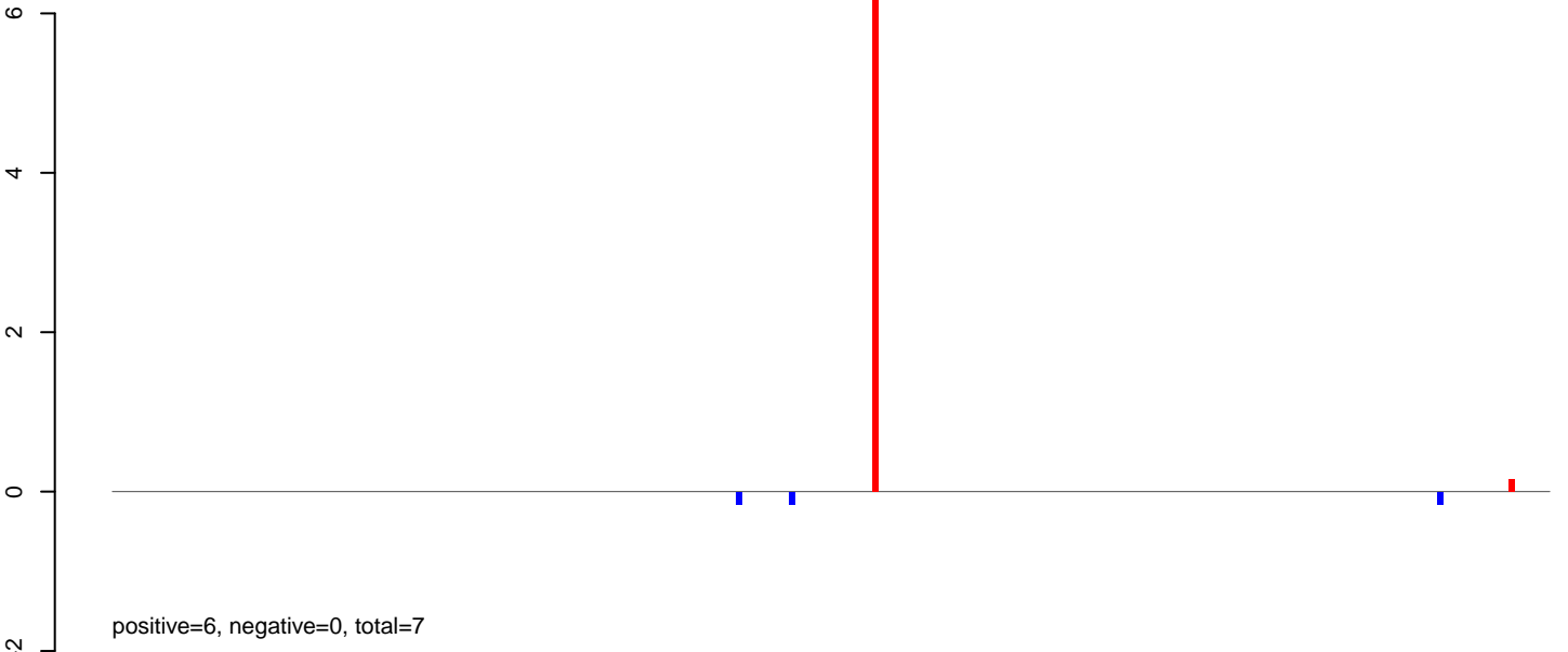
AeAlbo_C636_6dpi_SINV1.24_35.rep
