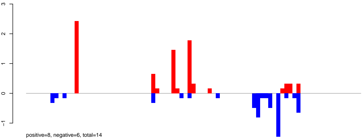
AeAlbo_C636_6dpi_SINV1.24_35.rep
