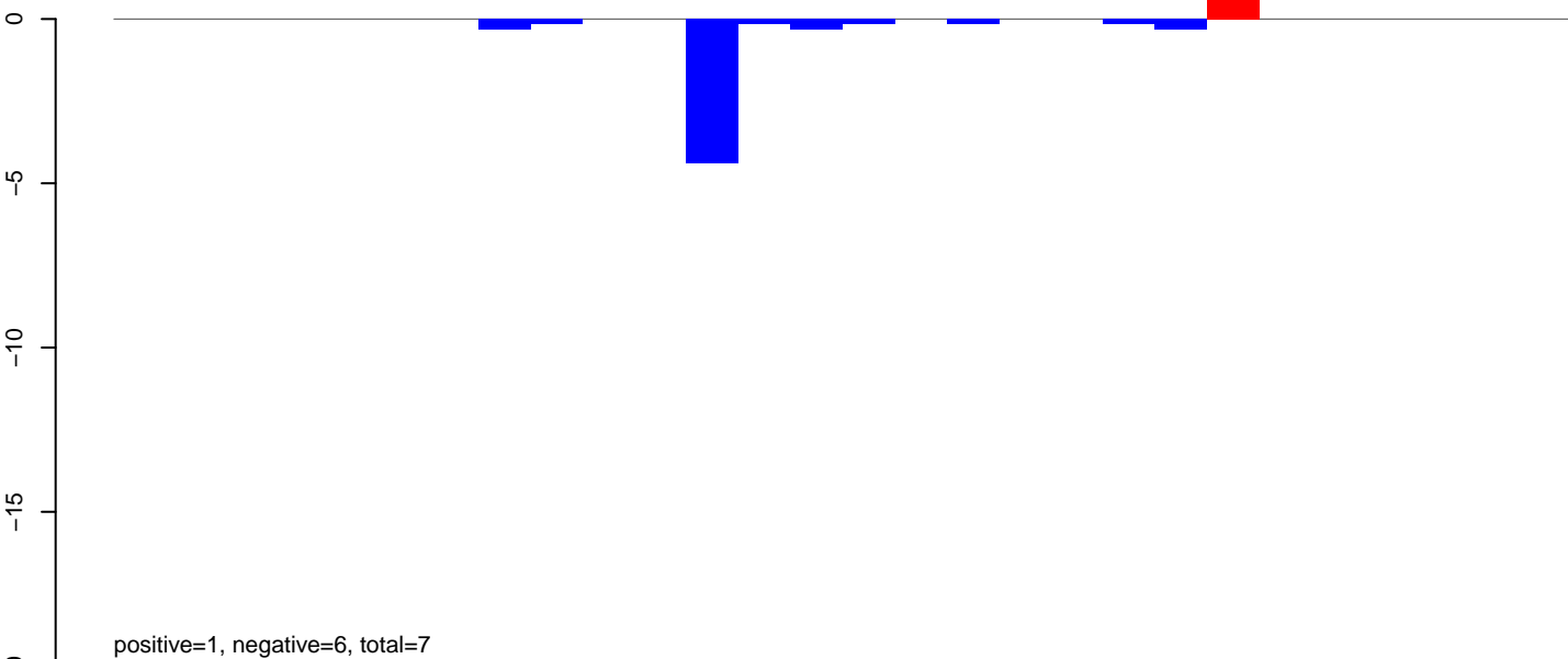
AeAlbo_C636_6dpi_SINV1.24_35.rep
