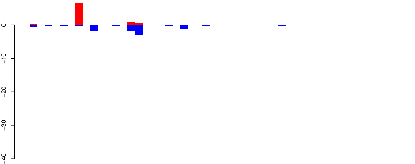
AeAlbo_C636_6dpi_SINV1.18_23.rep
