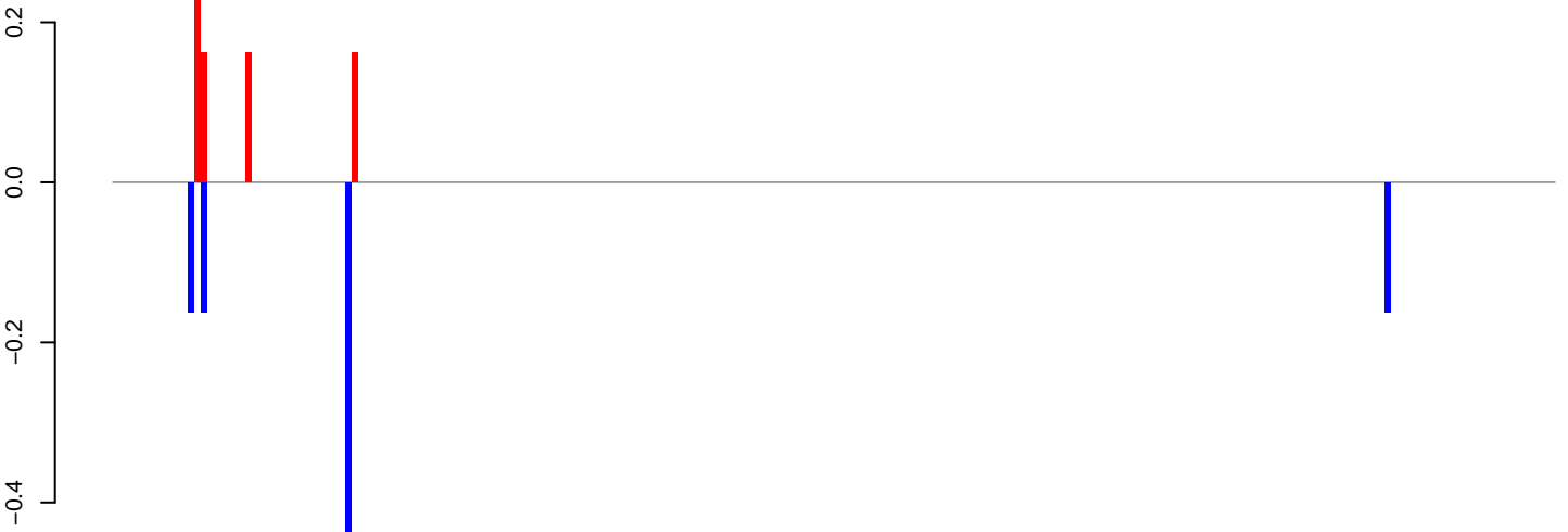
AeAlbo_C636_6dpi_SINV1.rep
