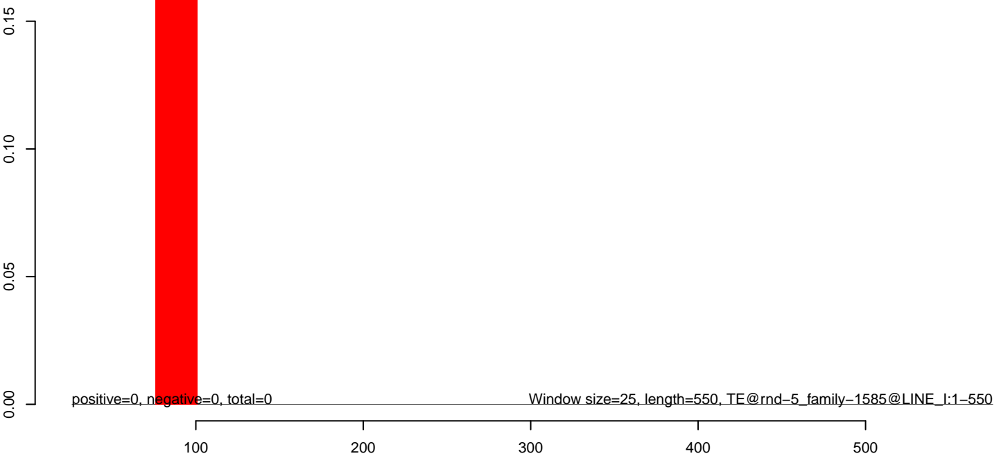
AeAlbo_C636_6dpi_SINV1.rep
