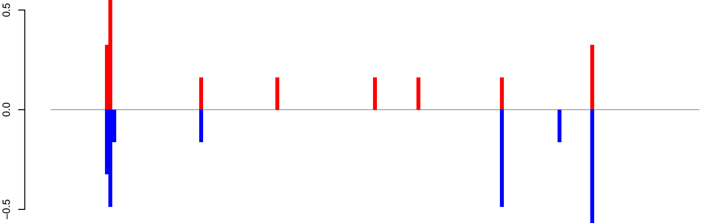
AeAlbo_C636_6dpi_SINV1.18_23.rep
