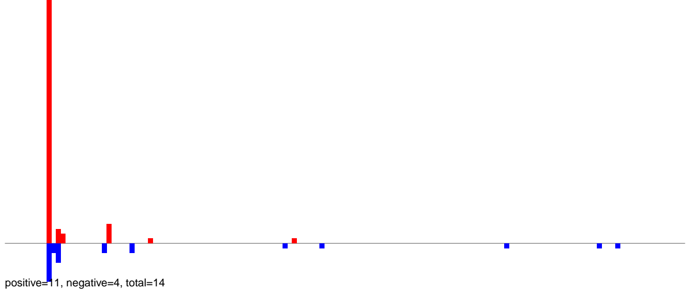
AeAlbo_C636_6dpi_SINV1.24_35.rep
