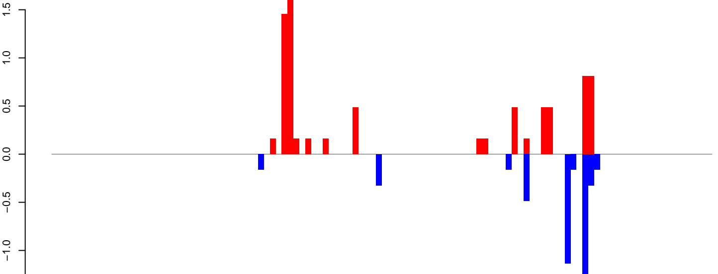
AeAlbo_C636_6dpi_SINV1.rep
