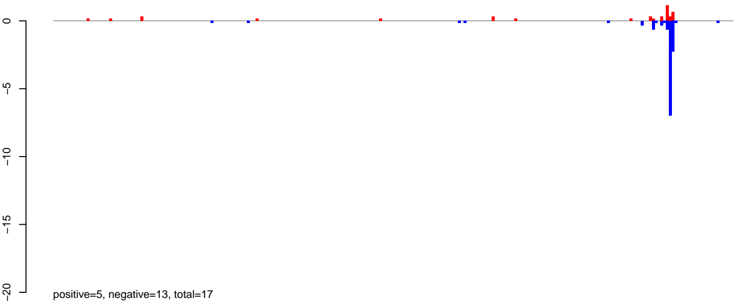
AeAlbo_C636_6dpi_SINV1.24_35.rep
