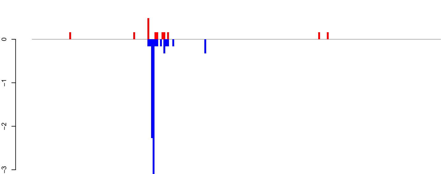
AeAlbo_C636_6dpi_SINV1.24_35.rep
