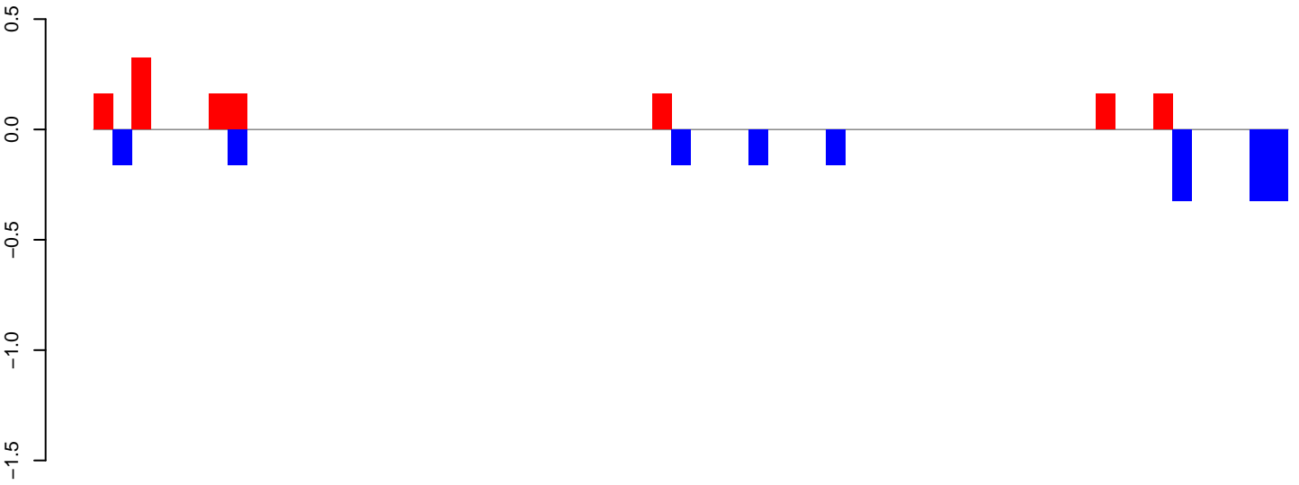
AeAlbo_C636_6dpi_SINV1.18_23.rep
