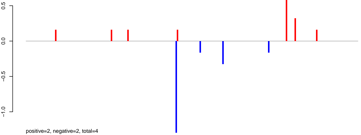
AeAlbo_C636_6dpi_SINV1.24_35.rep
