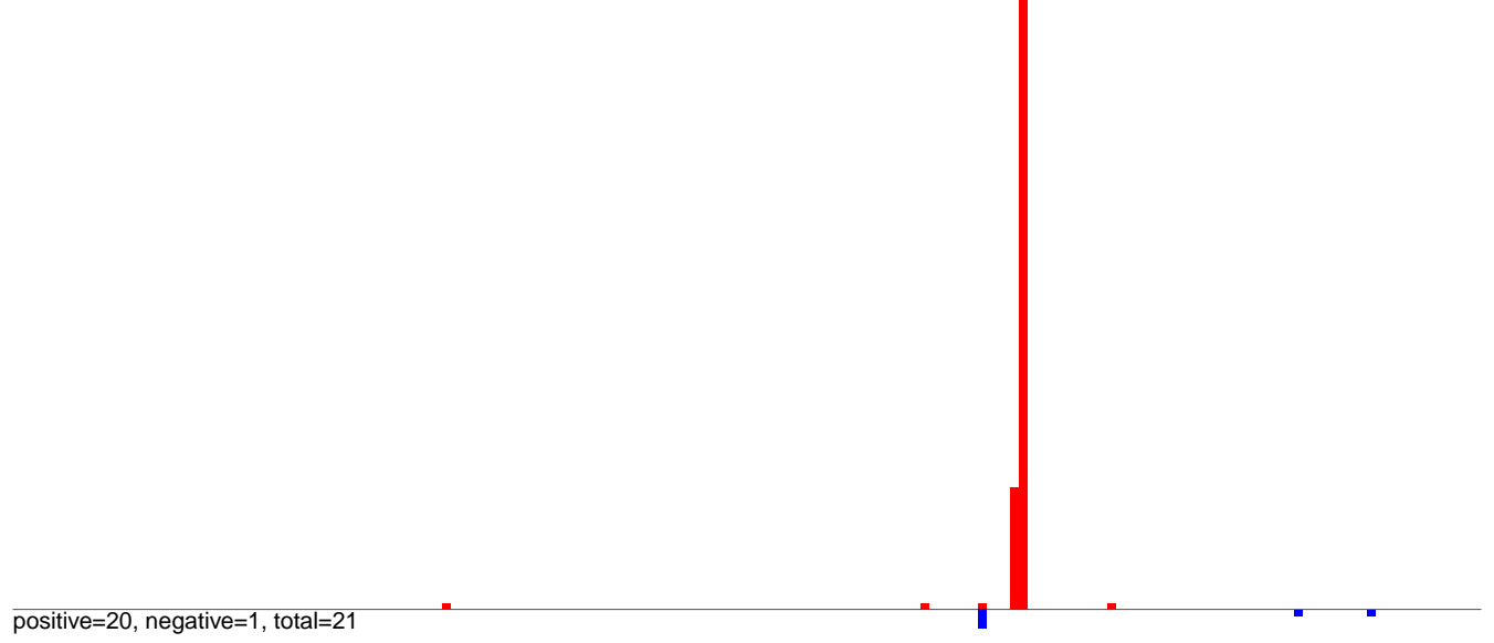
AeAlbo_C636_6dpi_SINV1.24_35.rep
