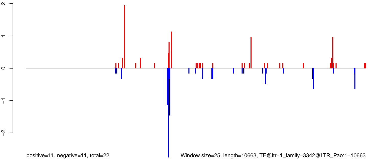
AeAlbo_C636_6dpi_SINV1.rep
