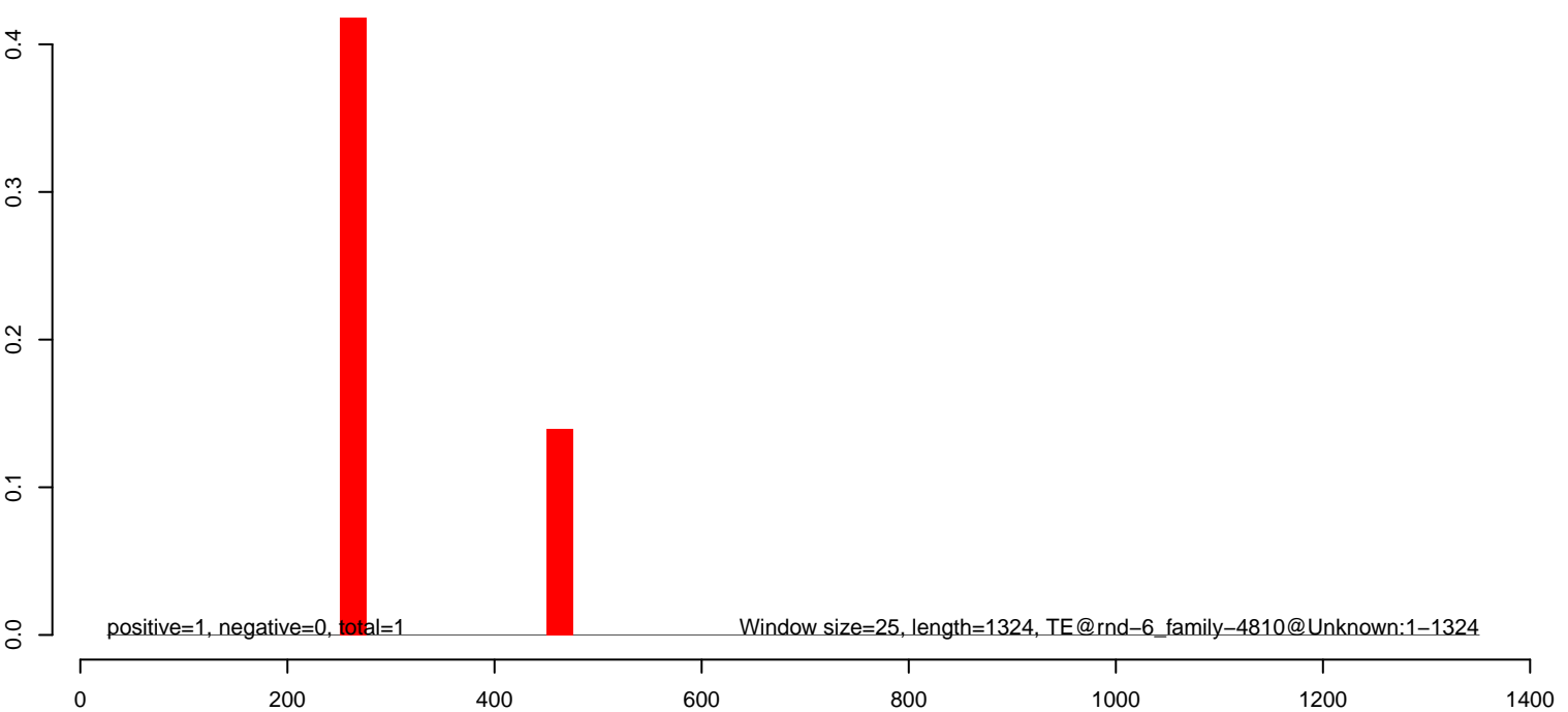
AeAlbo_C636_6dpi_SINV2.rep
