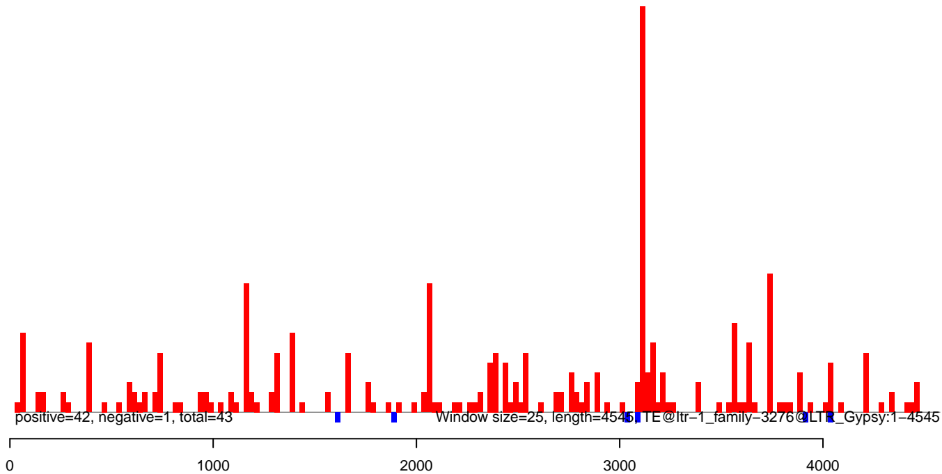
AeAlbo_C636_6dpi_SINV2.rep
