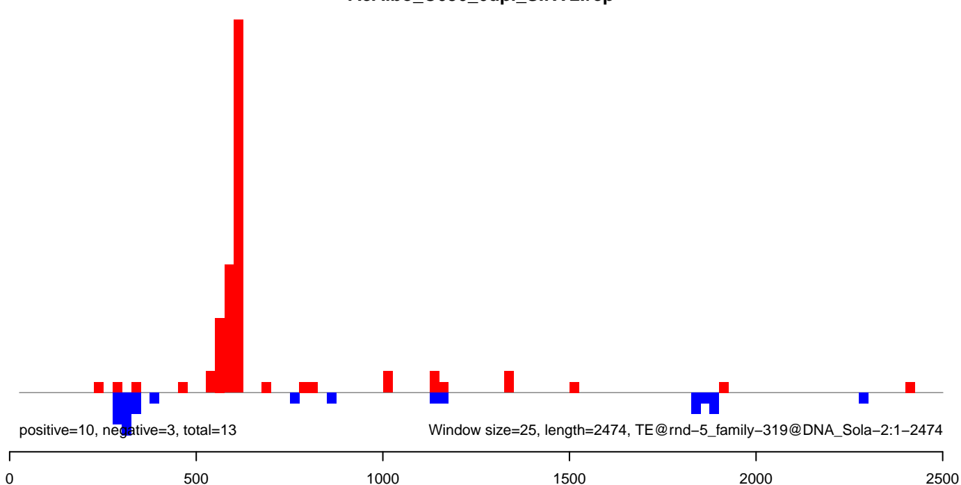
AeAlbo_C636_6dpi_SINV2.rep
