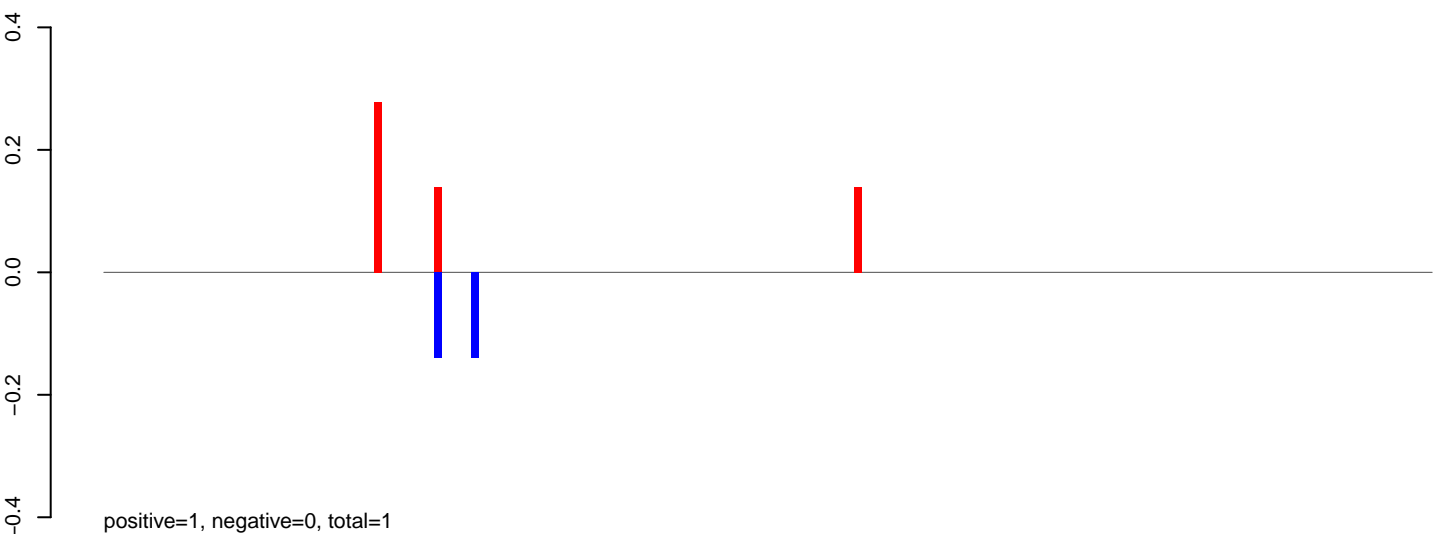
AeAlbo_C636_6dpi_SINV2.rep
