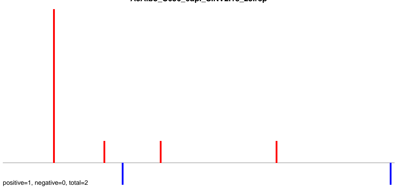
AeAlbo_C636_6dpi_SINV2.24_35.rep
