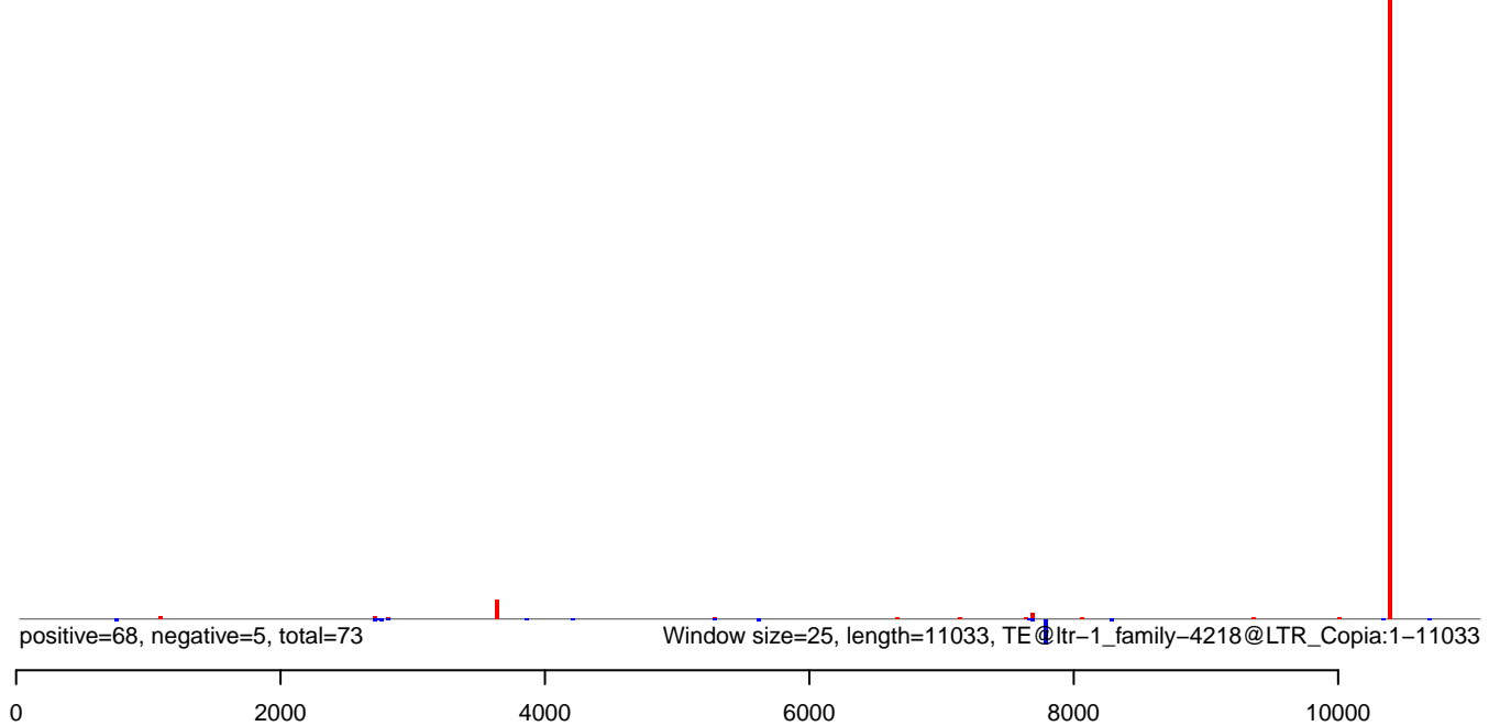
AeAlbo_C636_6dpi_SINV2.rep
