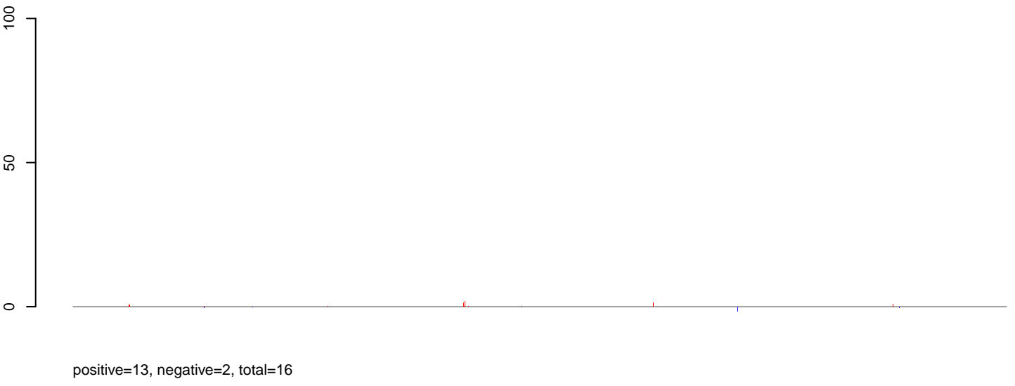
AeAlbo_C636_6dpi_SINV3.rep
