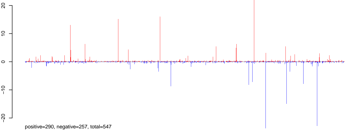
AeAlbo_C636_6dpi_SINV3.24_35.rep
