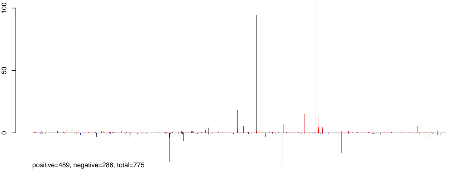
AeAlbo_C636_6dpi_SINV3.24_35.rep
