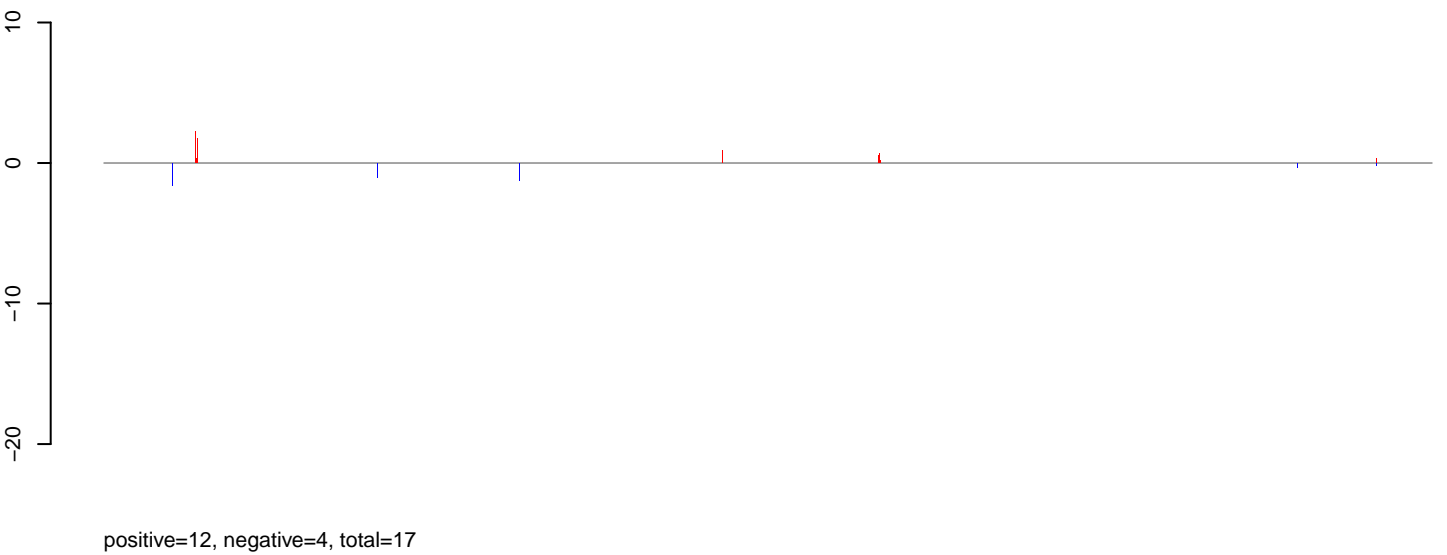
AeAlbo_C636_6dpi_SINV3.rep
