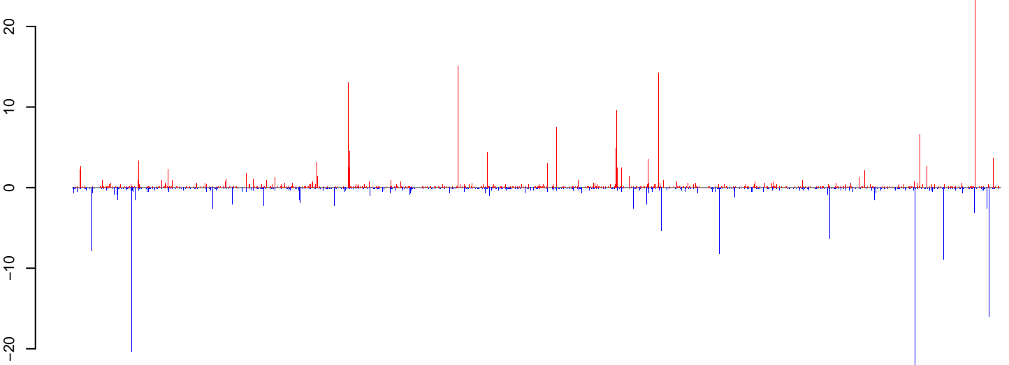
AeAlbo_C636_6dpi_SINV3.rep
