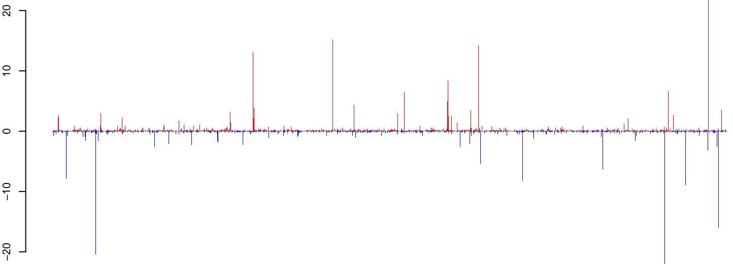
AeAlbo_C636_6dpi_SINV3.18_23.rep
