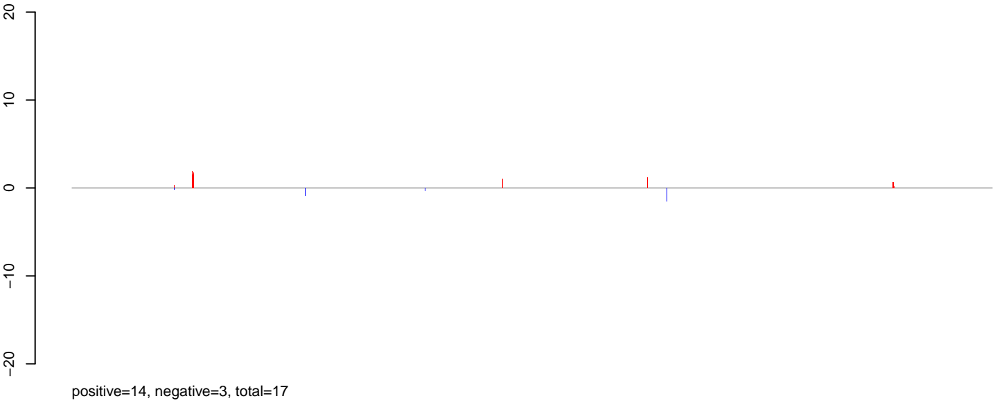
AeAlbo_C636_6dpi_SINV3.rep
