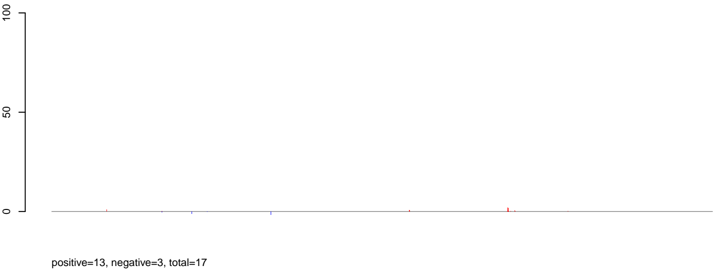
AeAlbo_C636_6dpi_SINV3.rep
