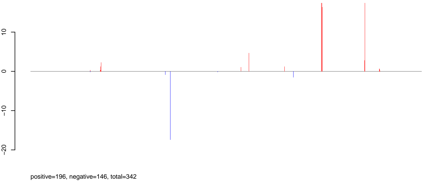
AeAlbo_C636_6dpi_SINV3.rep
