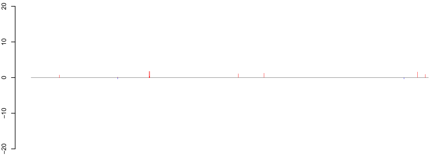
AeAlbo_C636_6dpi_SINV3.24_35.rep
