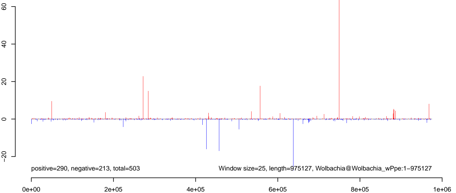
AeAlbo_C636_6dpi_SINV3.rep
