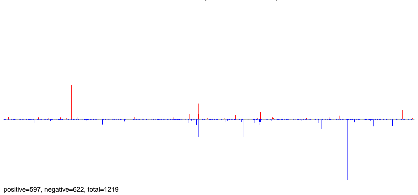
AeAlbo_C636_6dpi_SINV3.24_35.rep
