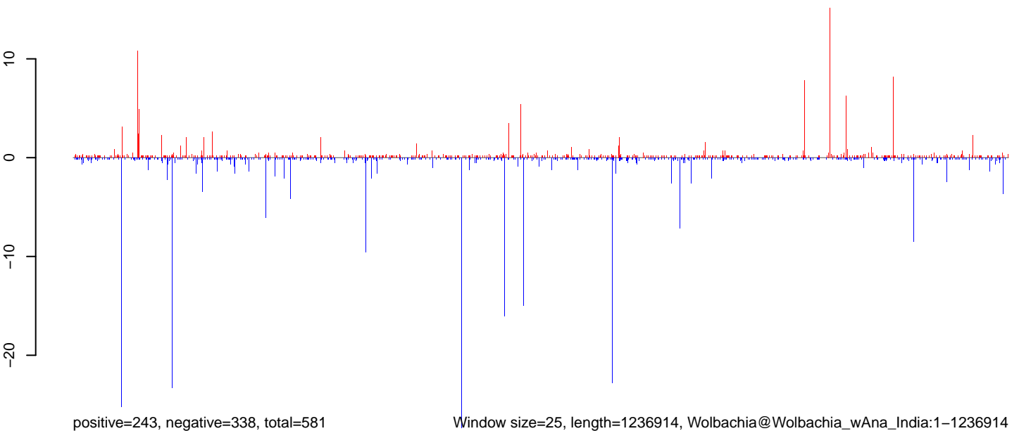
AeAlbo_C636_6dpi_SINV3.rep
