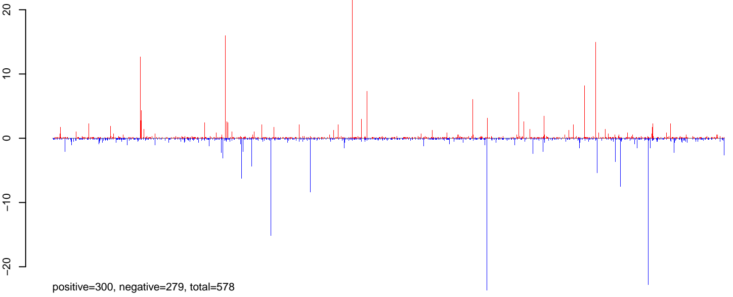
AeAlbo_C636_6dpi_SINV3.24_35.rep
