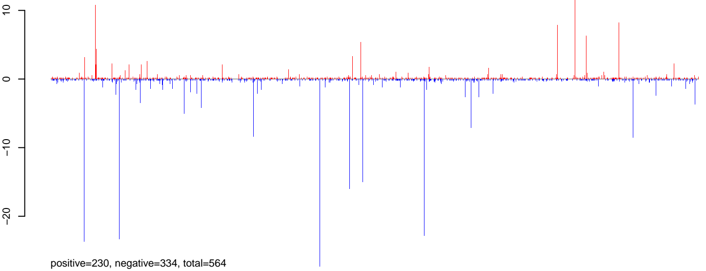
AeAlbo_C636_6dpi_SINV3.24_35.rep
