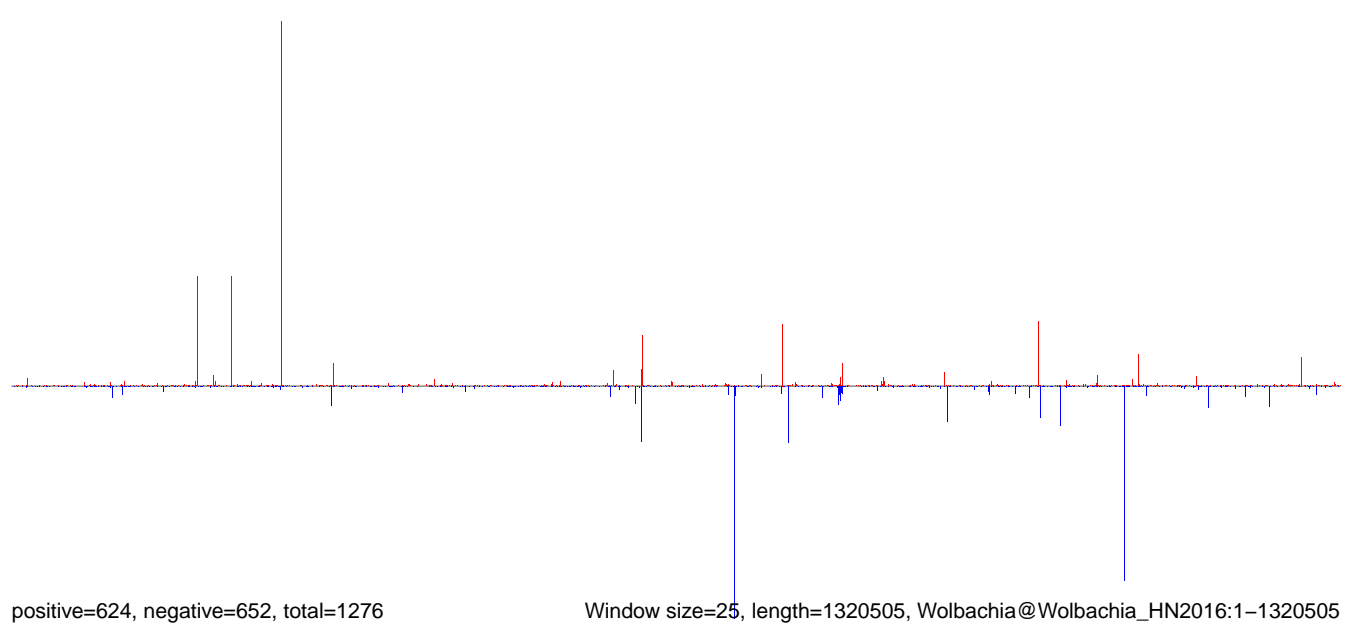
AeAlbo_C636_6dpi_SINV3.rep
