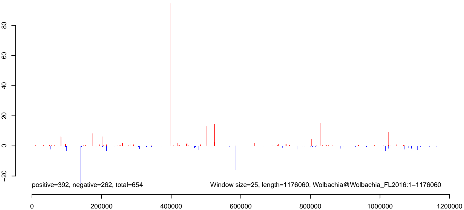
AeAlbo_C636_6dpi_SINV3.rep
