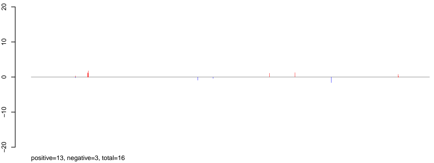
AeAlbo_C636_6dpi_SINV3.rep
