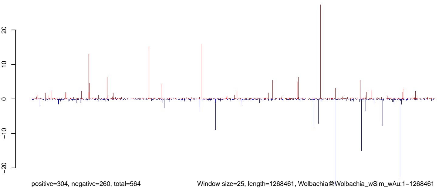
AeAlbo_C636_6dpi_SINV3.rep
