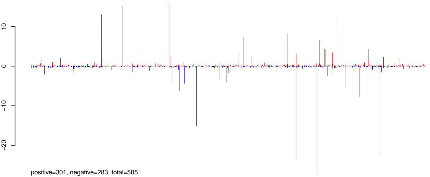
AeAlbo_C636_6dpi_SINV3.24_35.rep
