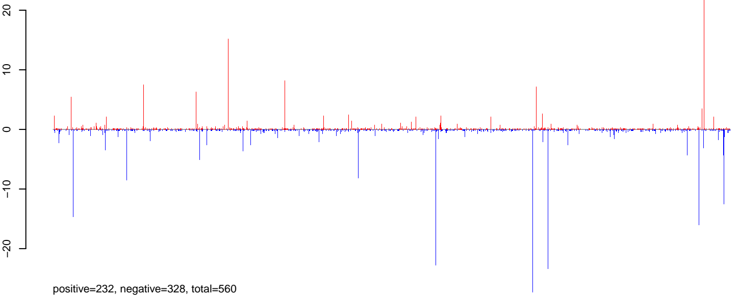
AeAlbo_C636_6dpi_SINV3.24_35.rep
