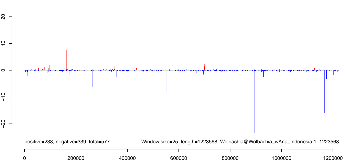
AeAlbo_C636_6dpi_SINV3.rep
