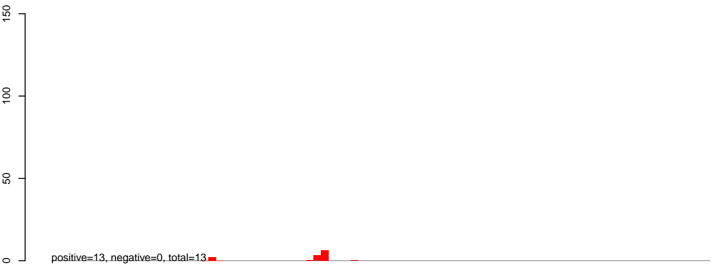
AeAlbo_FemaleMidgut_Denv2_JG.rep
