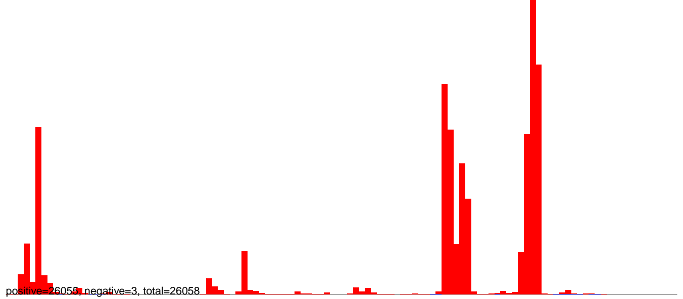
AeAlbo_FemaleMidgut_Denv2_JG.24_35.rep
