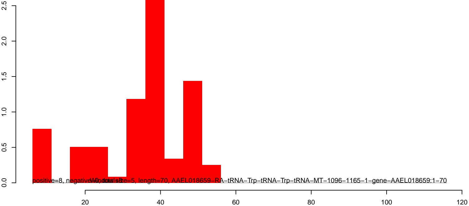
AeAlbo_FemaleMidgut_Denv2_JG.rep
