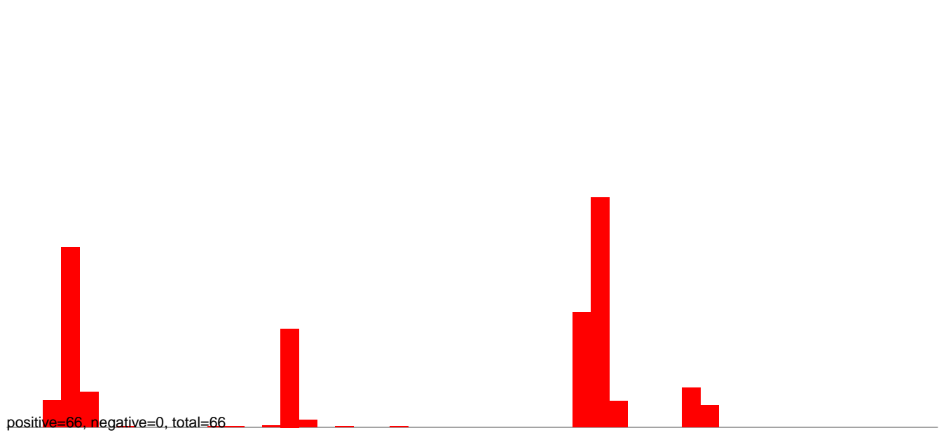
AeAlbo_FemaleMidgut_Denv2_JG.24_35.rep
