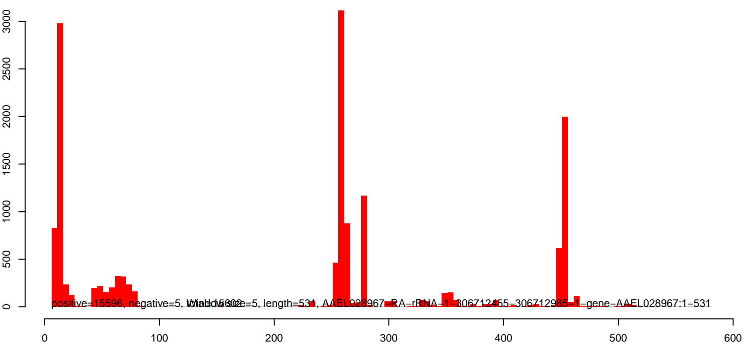
AeAlbo_FemaleMidgut_Denv2_JG.rep
