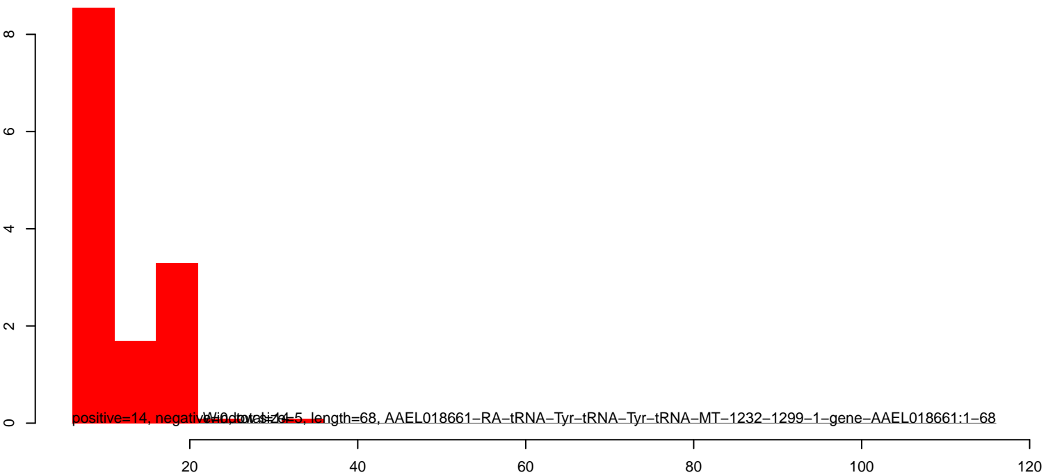
AeAlbo_FemaleMidgut_Denv2_JG.rep
