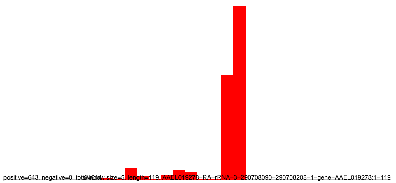
AeAlbo_FemaleMidgut_Denv2_JG.rep
