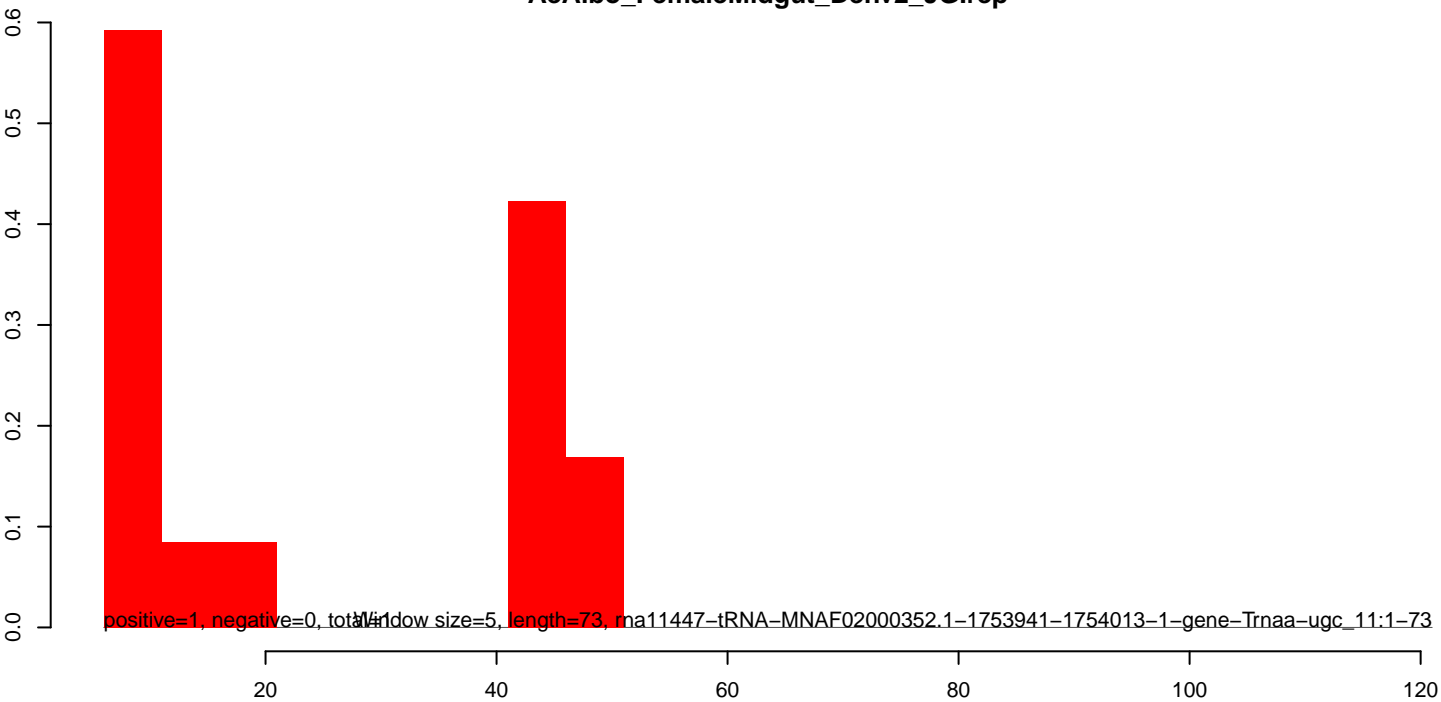
AeAlbo_FemaleMidgut_Denv2_JG.rep
