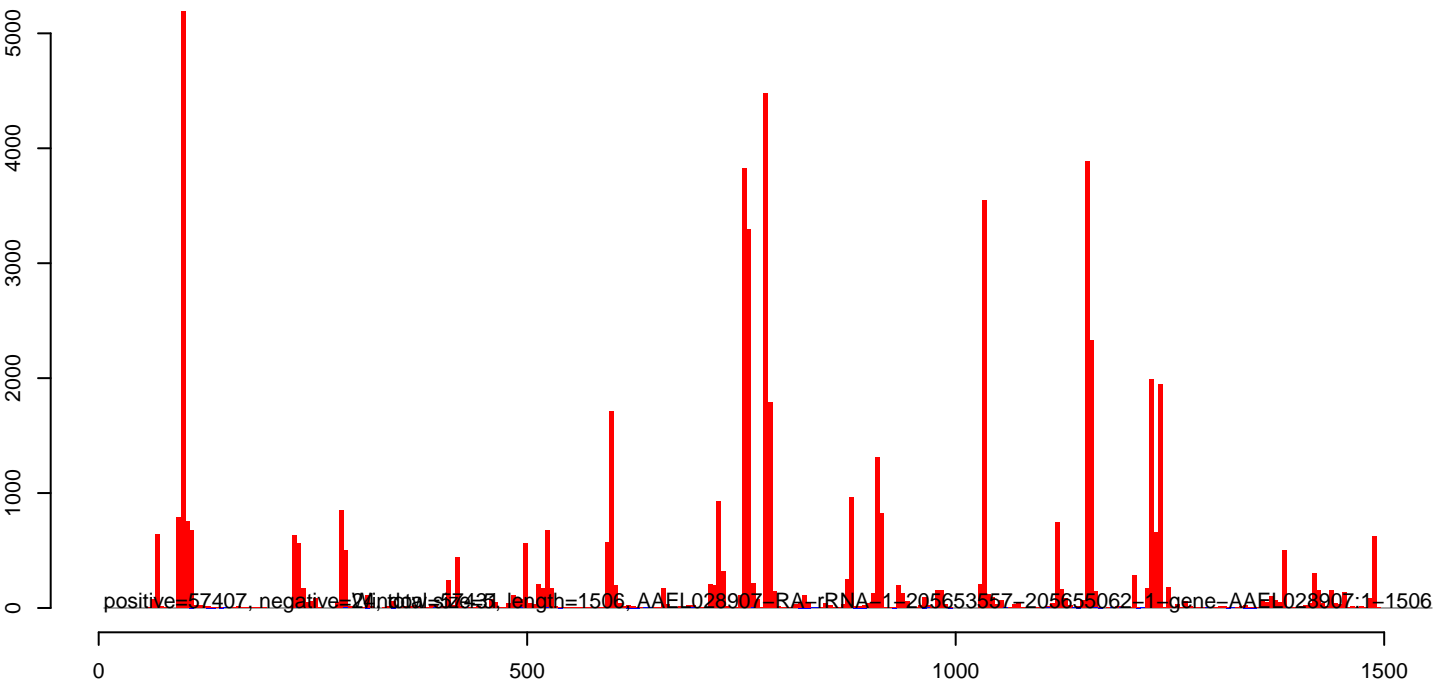
AeAlbo_FemaleMidgut_Denv2_JG.rep
