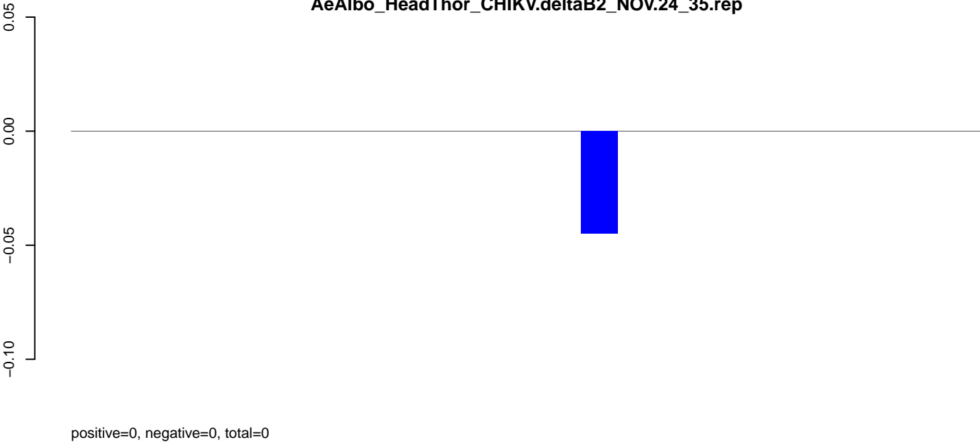
AeAlbo_HeadThor_CHIKV.deltaB2_NOV.rep
