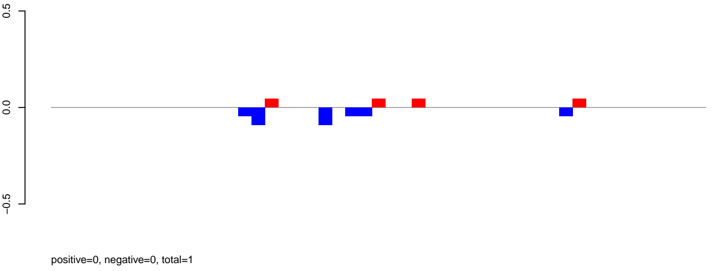
AeAlbo_HeadThor_CHIKV.deltaB2_NOV.rep
