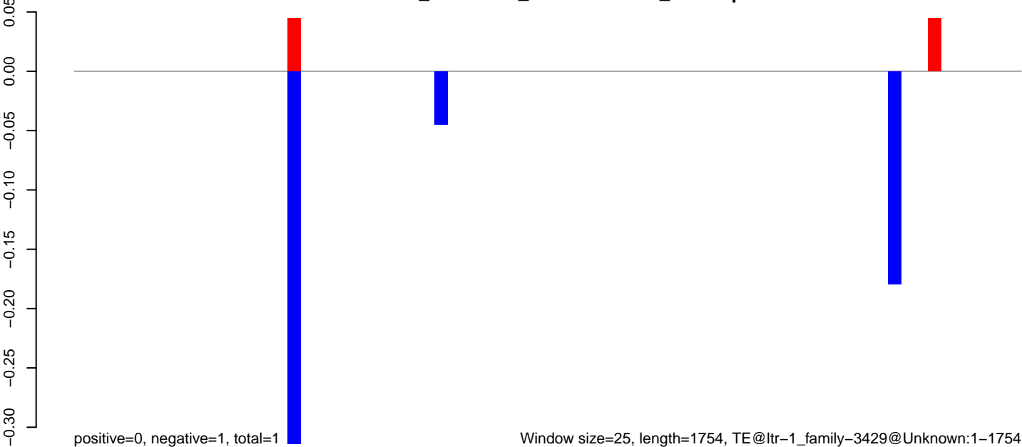
AeAlbo_HeadThor_CHIKV.deltaB2_NOV.rep
