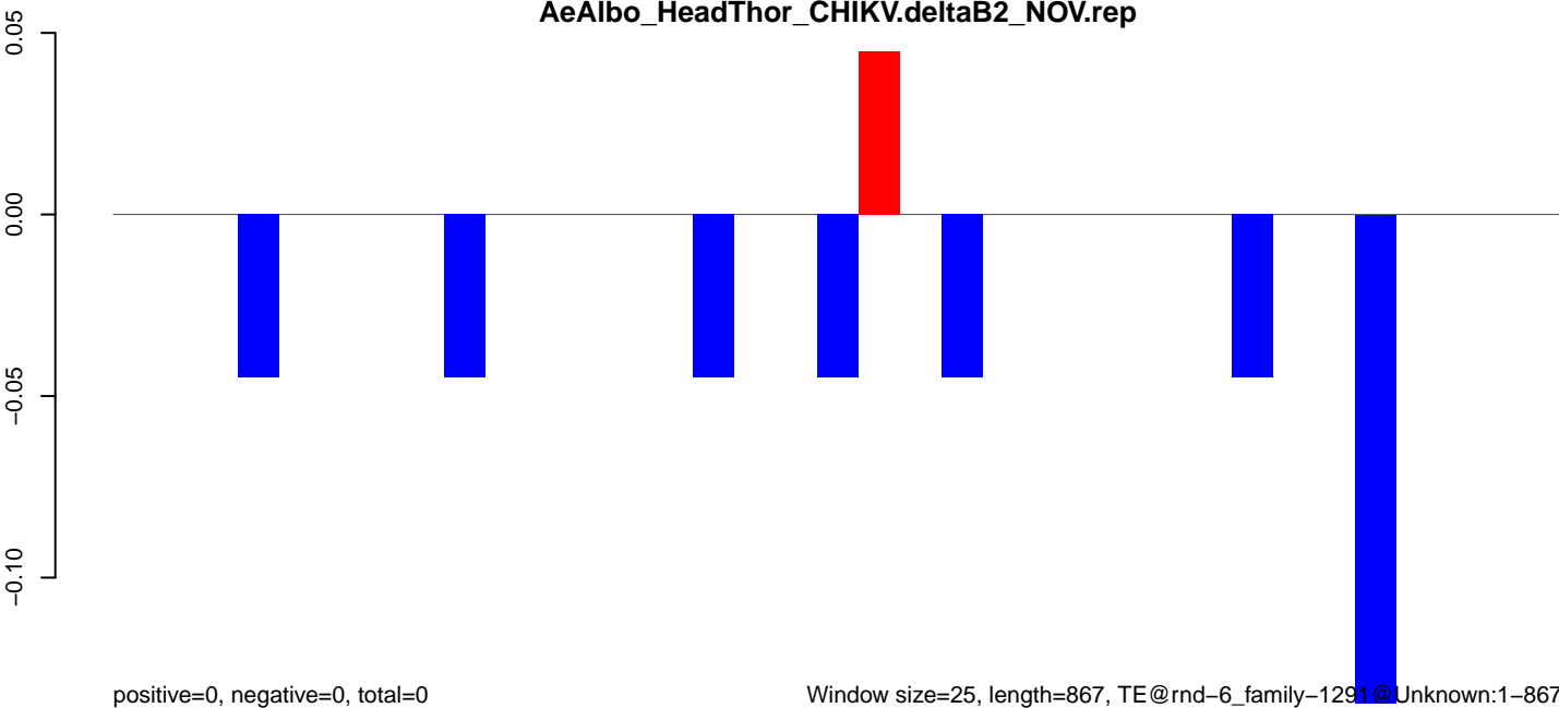
AeAlbo_HeadThor_CHIKV.deltaB2_NOV.rep
