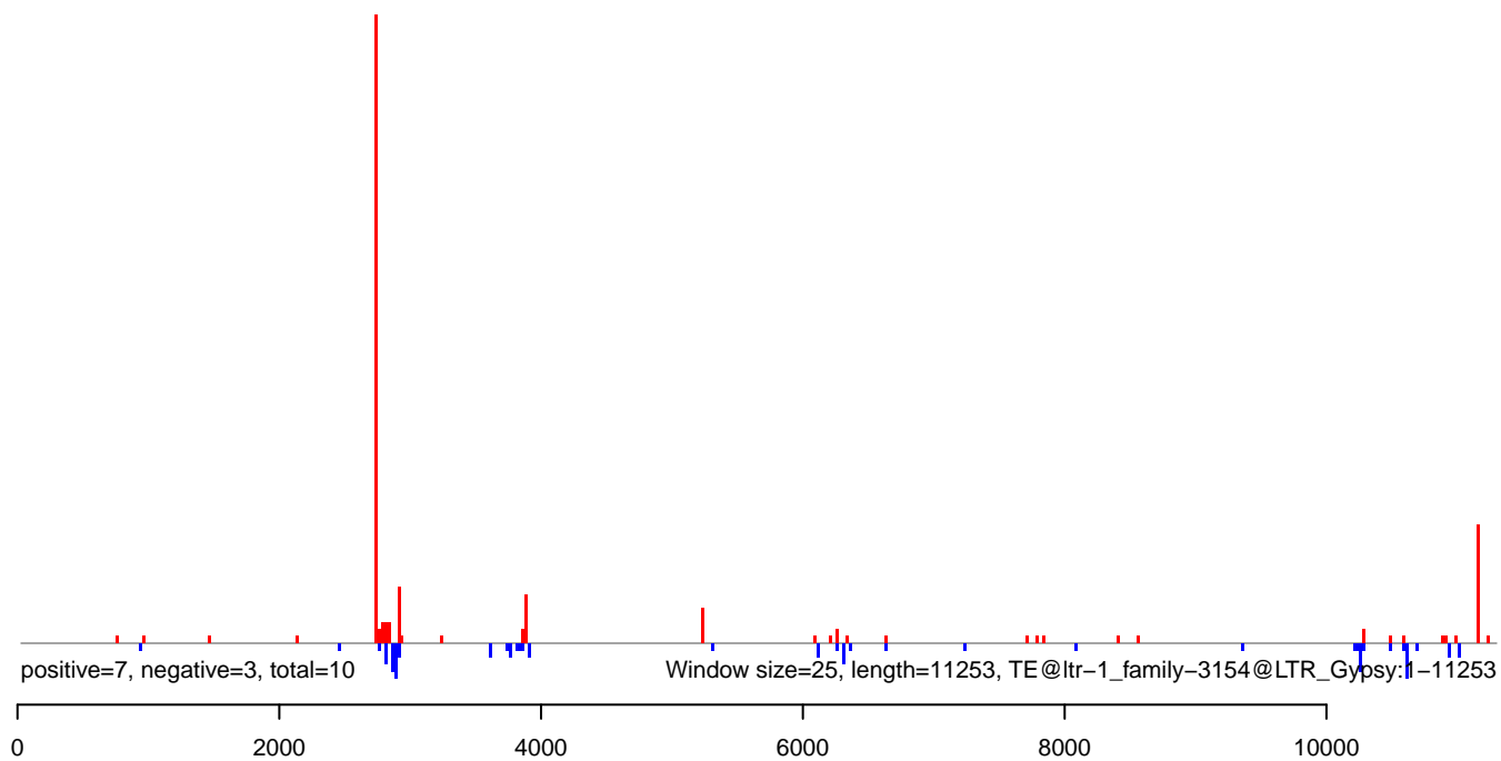
AeAlbo_HeadThor_CHIKV.deltaB2_NOV.rep
