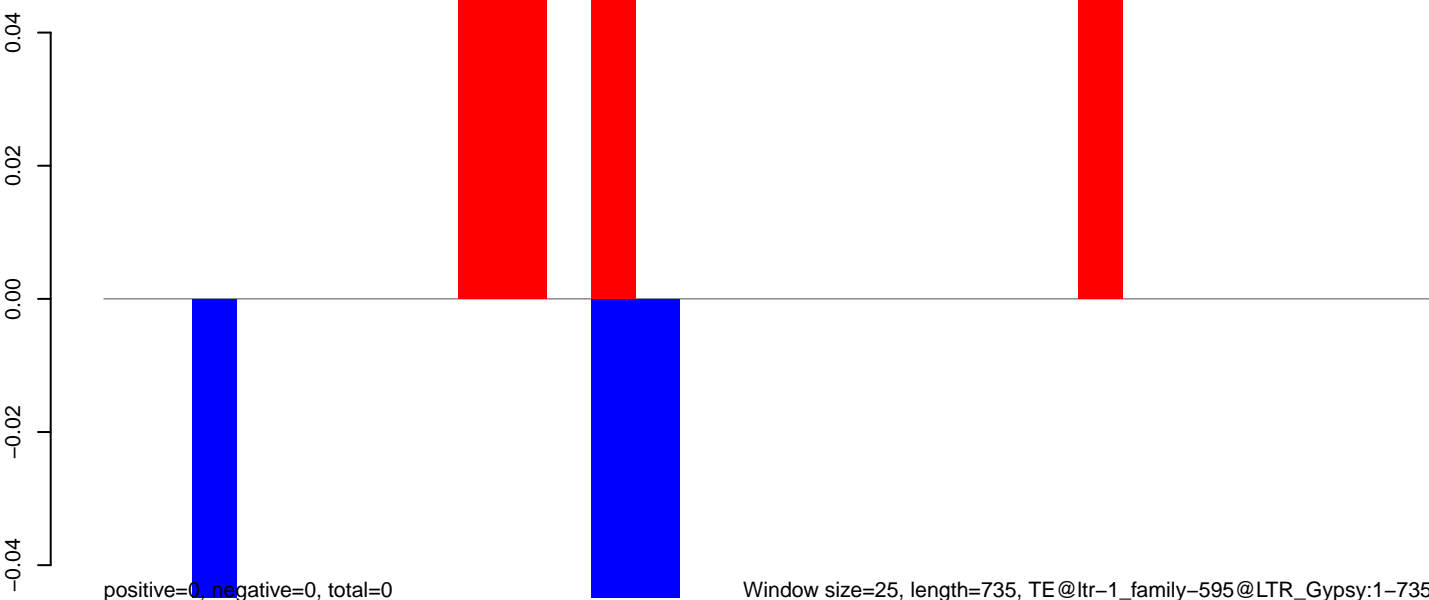
AeAlbo_HeadThor_CHIKV.deltaB2_NOV.rep
