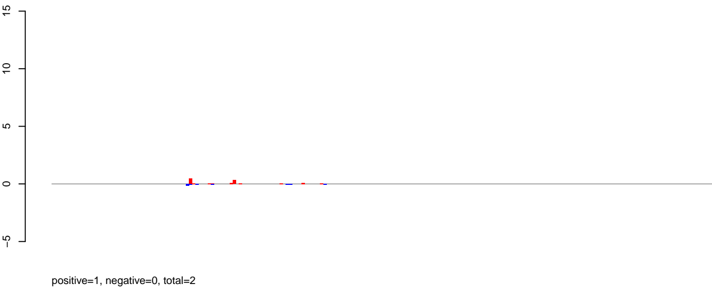
AeAlbo_HeadThor_CHIKV.deltaB2_NOV.rep
