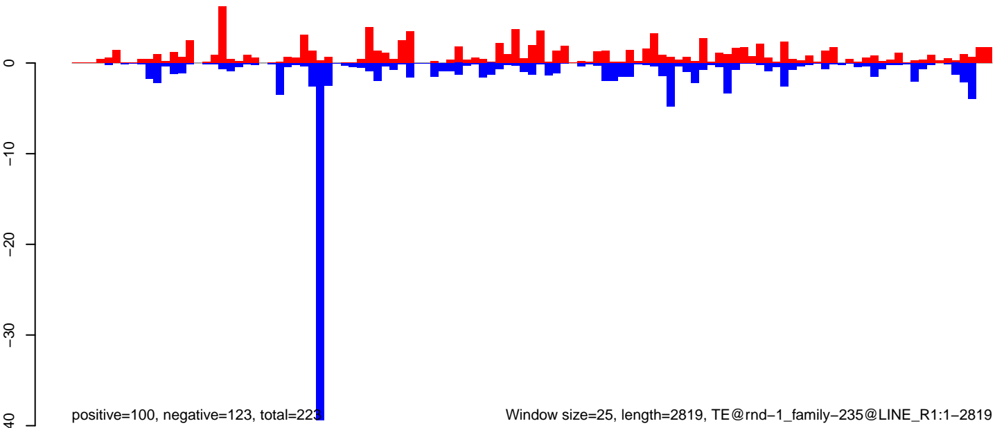
AeAlbo_HeadThor_CHIKV.deltaB2_NOV.rep
