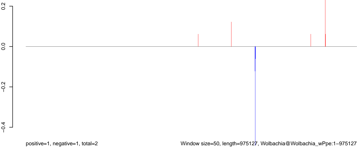
AeAlbo_C636_B2_FHV_r54q.rep
