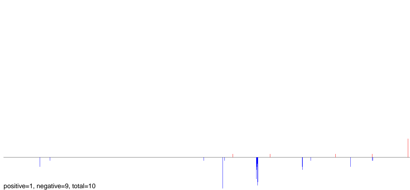
AeAlbo_C636_B2_FHV_r54q.rep
