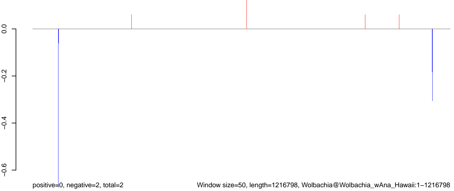
AeAlbo_C636_B2_FHV_r54q.rep
