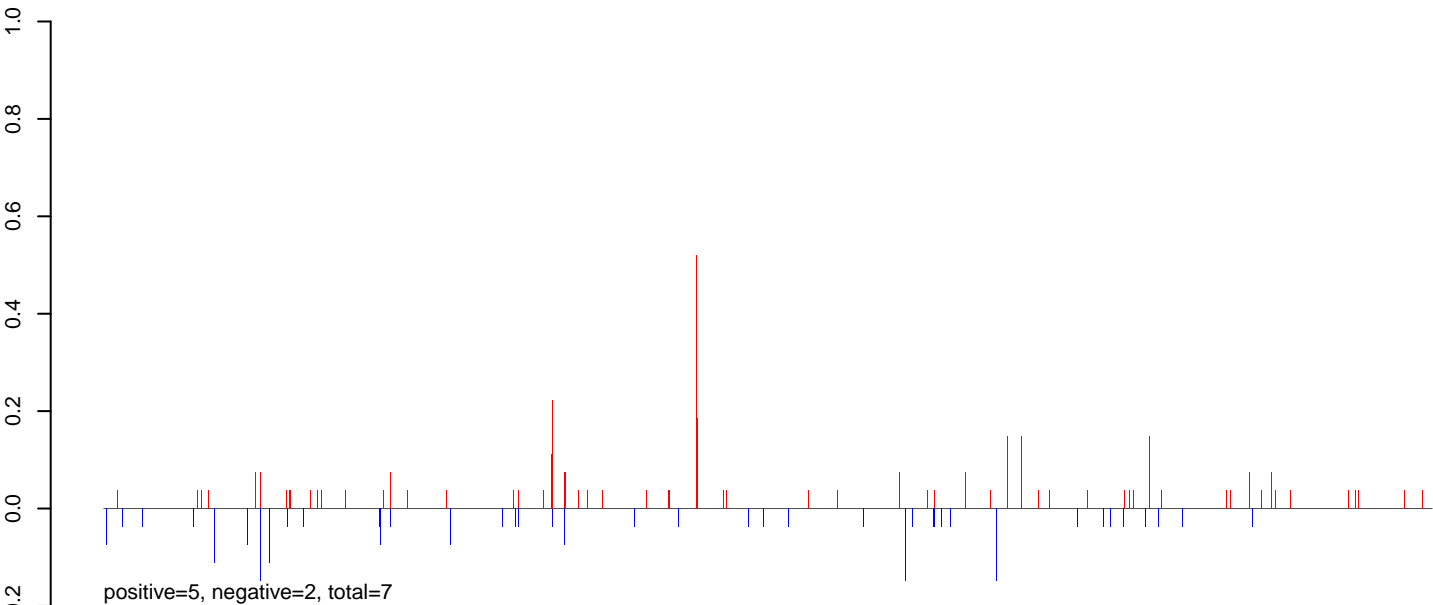
AeAlbo_HeadThor_CHIKV.B2_FHV.24_35.rep
