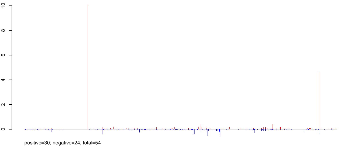
AeAlbo_HeadThor_CHIKV.B2_FHV.24_35.rep
