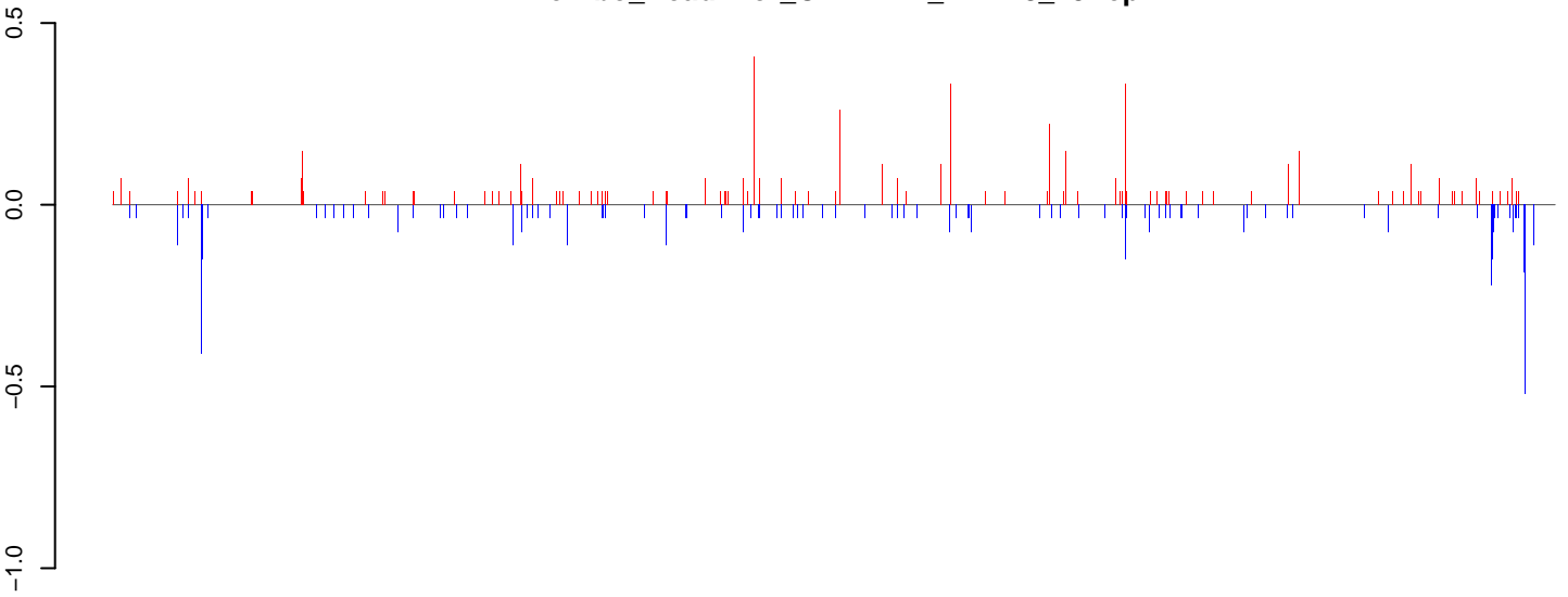
AeAlbo_HeadThor_CHIKV.B2_FHV.18_23.rep
