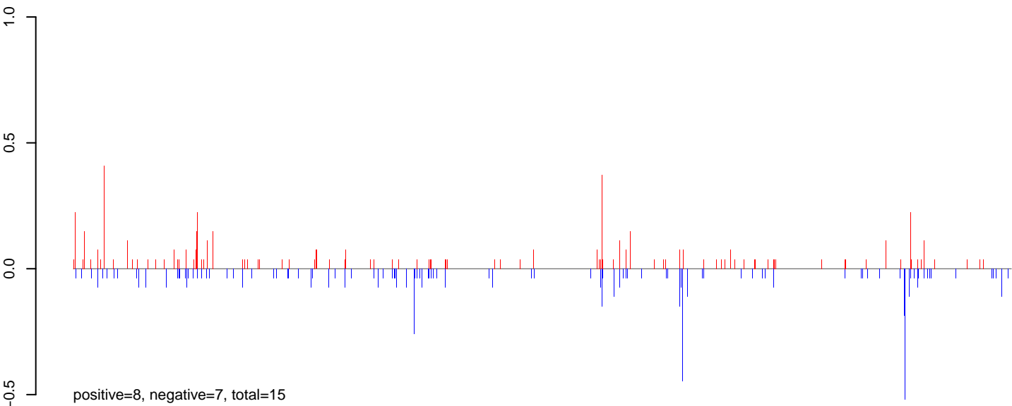
AeAlbo_HeadThor_CHIKV.B2_FHV.24_35.rep
