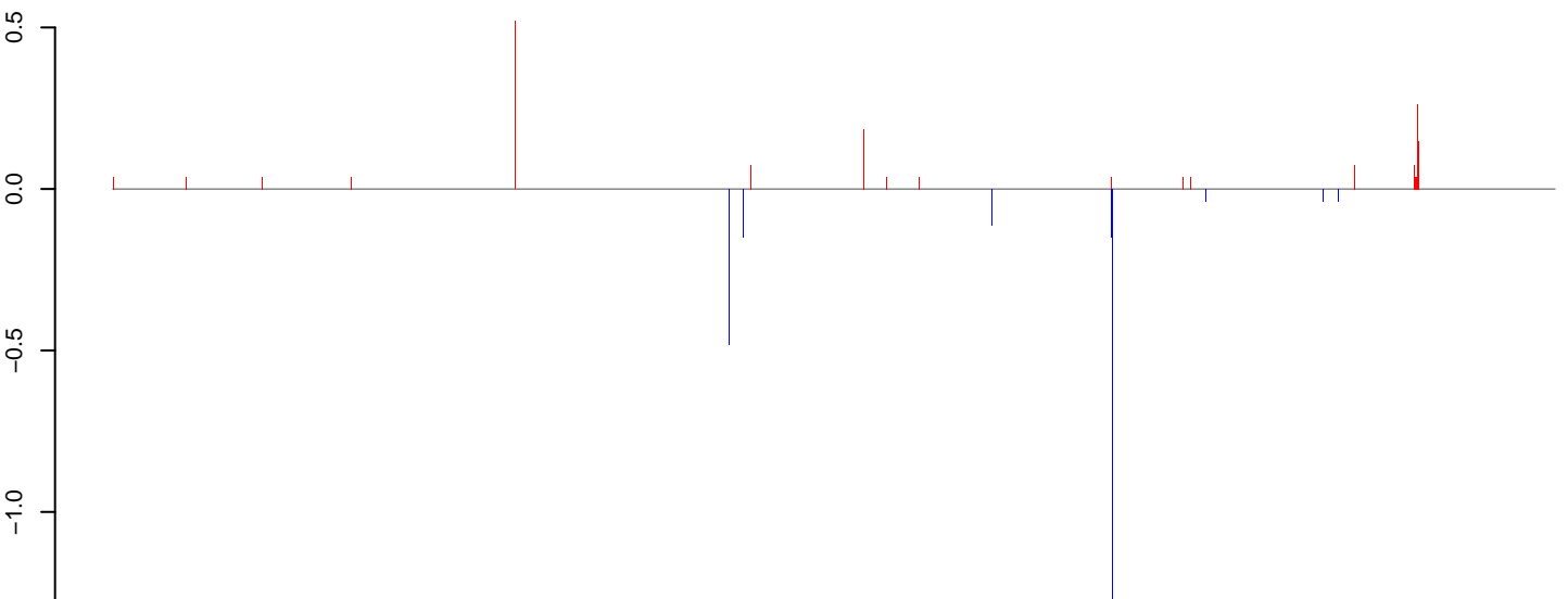
AeAlbo_HeadThor_CHIKV.B2_FHV.rep
