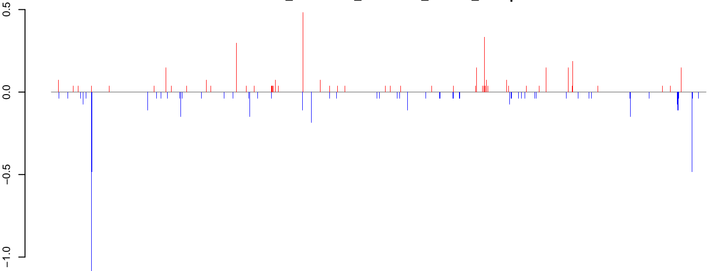
AeAlbo_HeadThor_CHIKV.B2_FHV.24_35.rep
