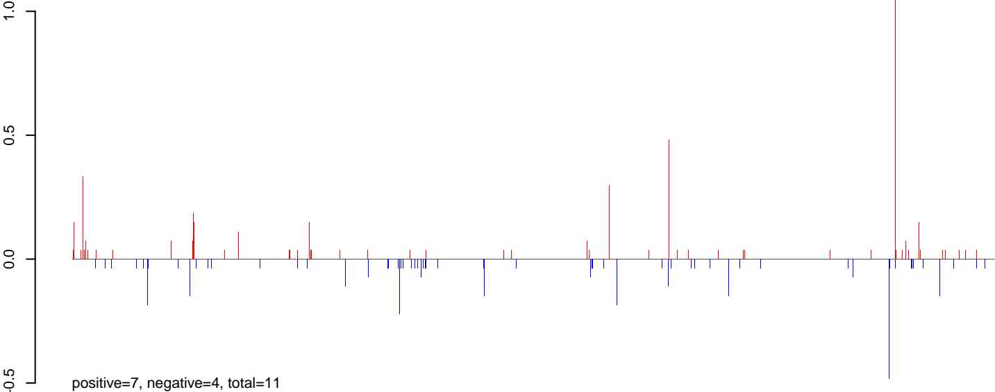
AeAlbo_HeadThor_CHIKV.B2_FHV.rep
