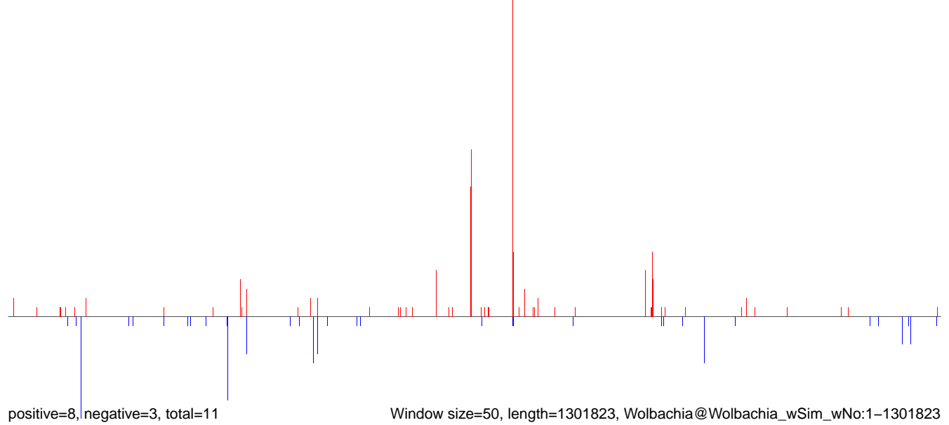
AeAlbo_HeadThor_CHIKV.B2_FHV.rep
