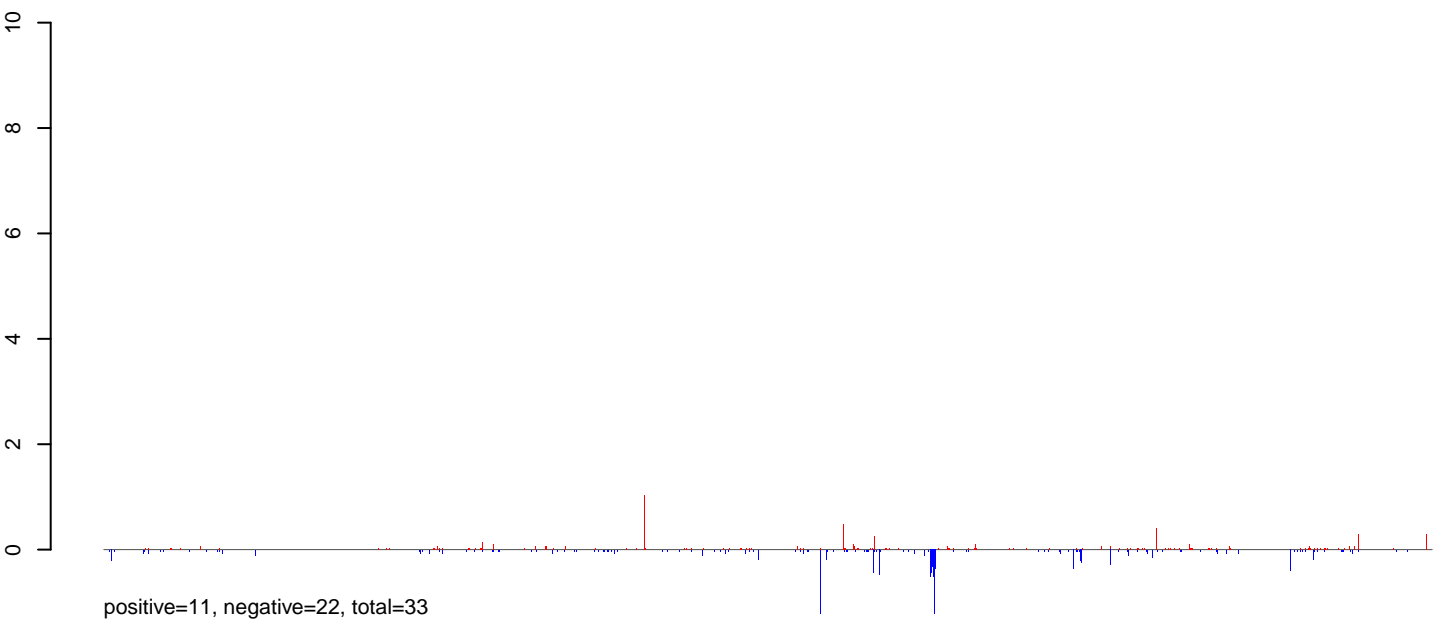
AeAlbo_HeadThor_CHIKV.B2_FHV.rep
