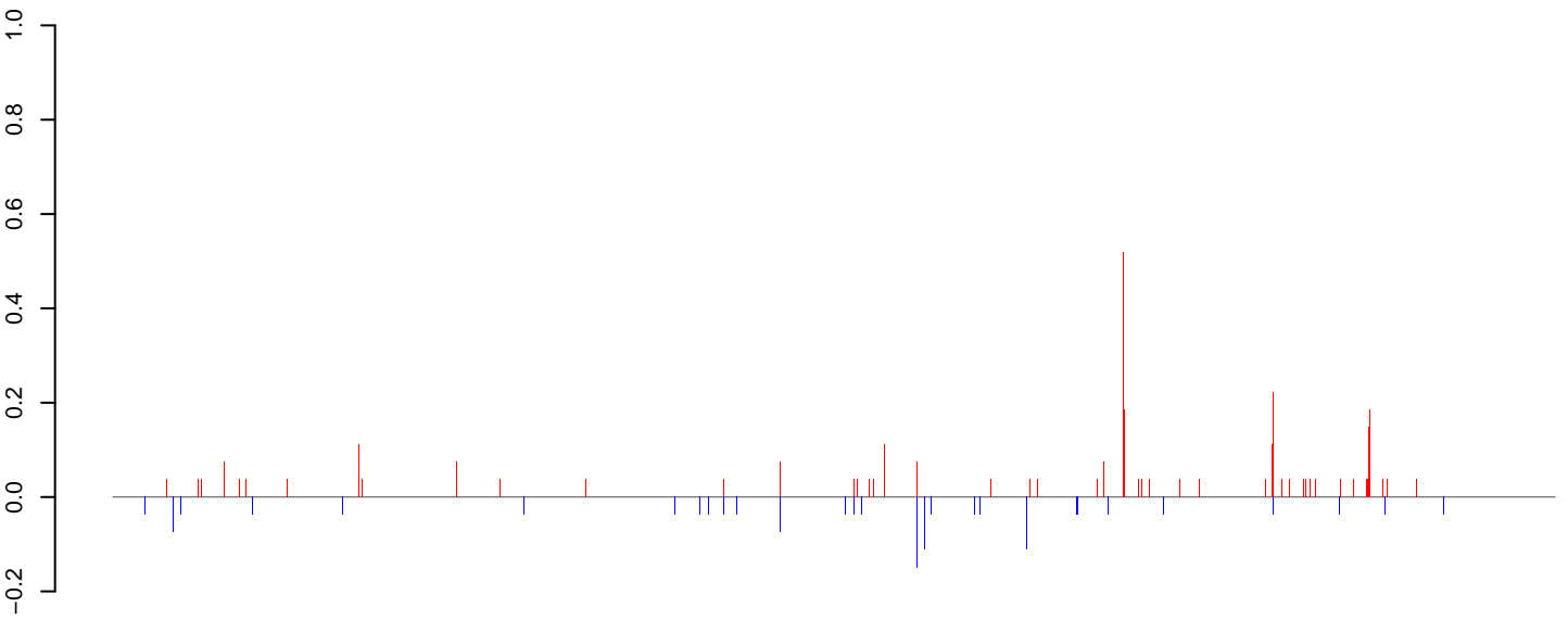
AeAlbo_HeadThor_CHIKV.B2_FHV.18_23.rep
