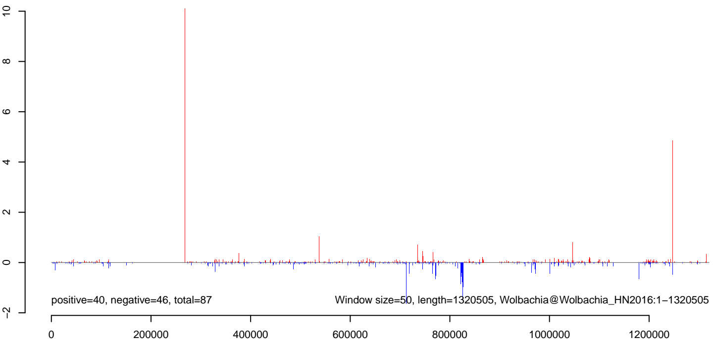
AeAlbo_HeadThor_CHIKV.B2_FHV.rep
