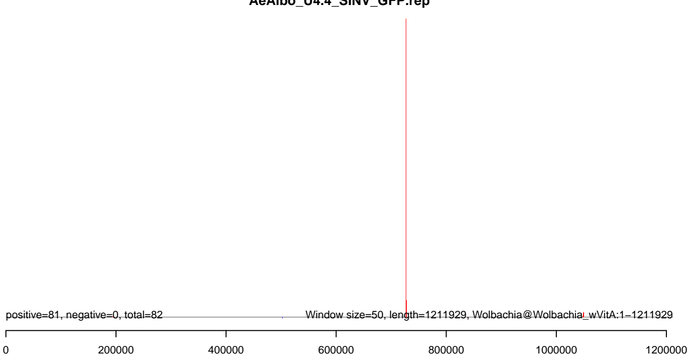
AeAlbo_U4.4_SINV_GFP.rep
