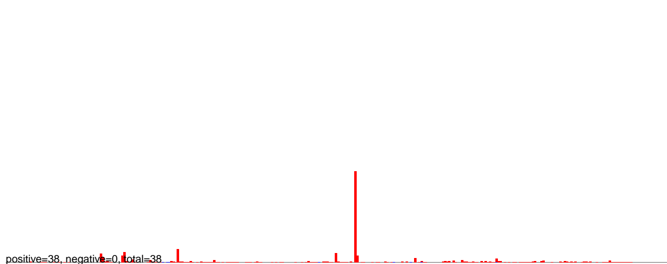
AeAlbo_C636_CHIKV_3dpi.rep
