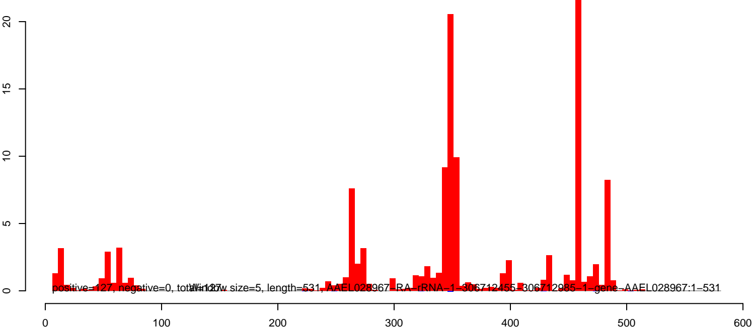
AeAlbo_C636_CHIKV_3dpi.rep
