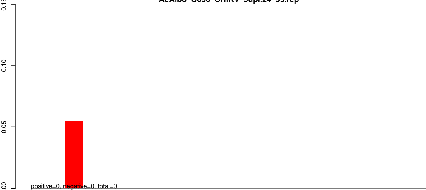
AeAlbo_C636_CHIKV_3dpi.rep
