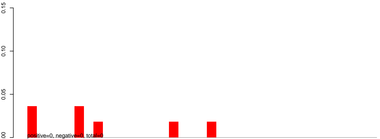
AeAlbo_C636_CHIKV_3dpi.rep
