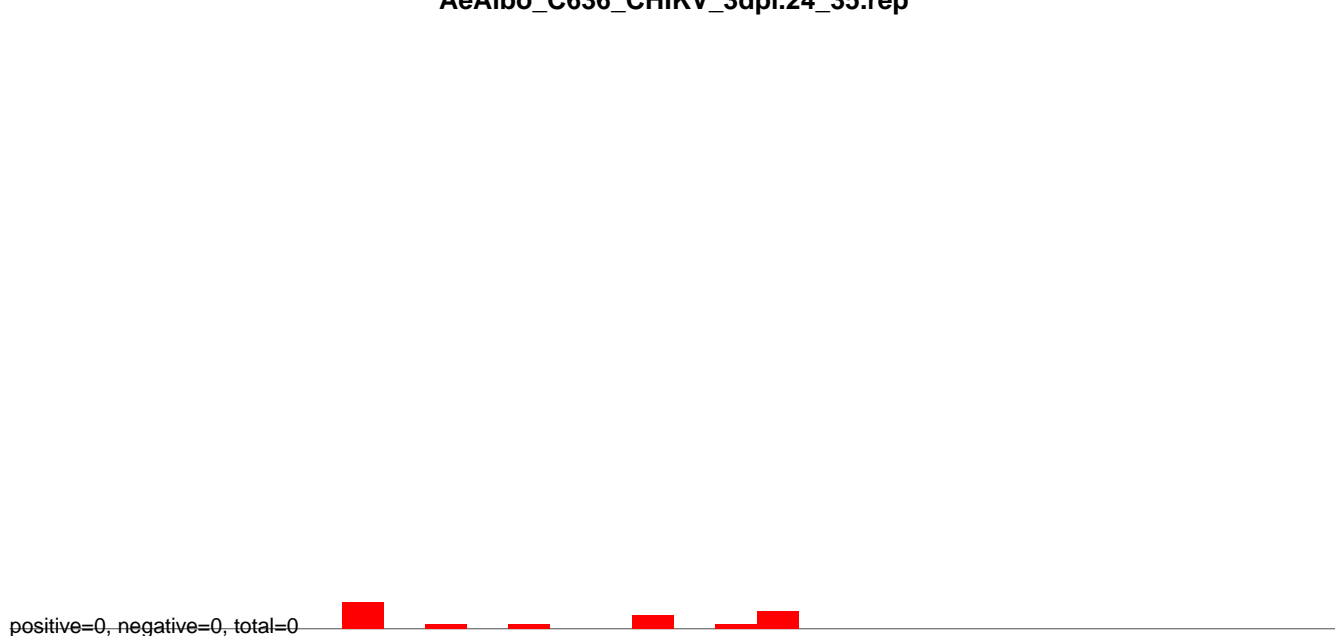
AeAlbo_C636_CHIKV_3dpi.rep
