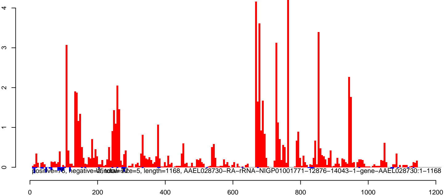
AeAlbo_C636_CHIKV_3dpi.rep
