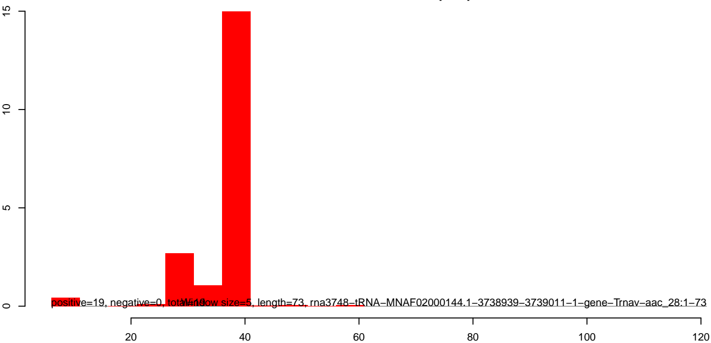
AeAlbo_C636_CHIKV_3dpi.rep
