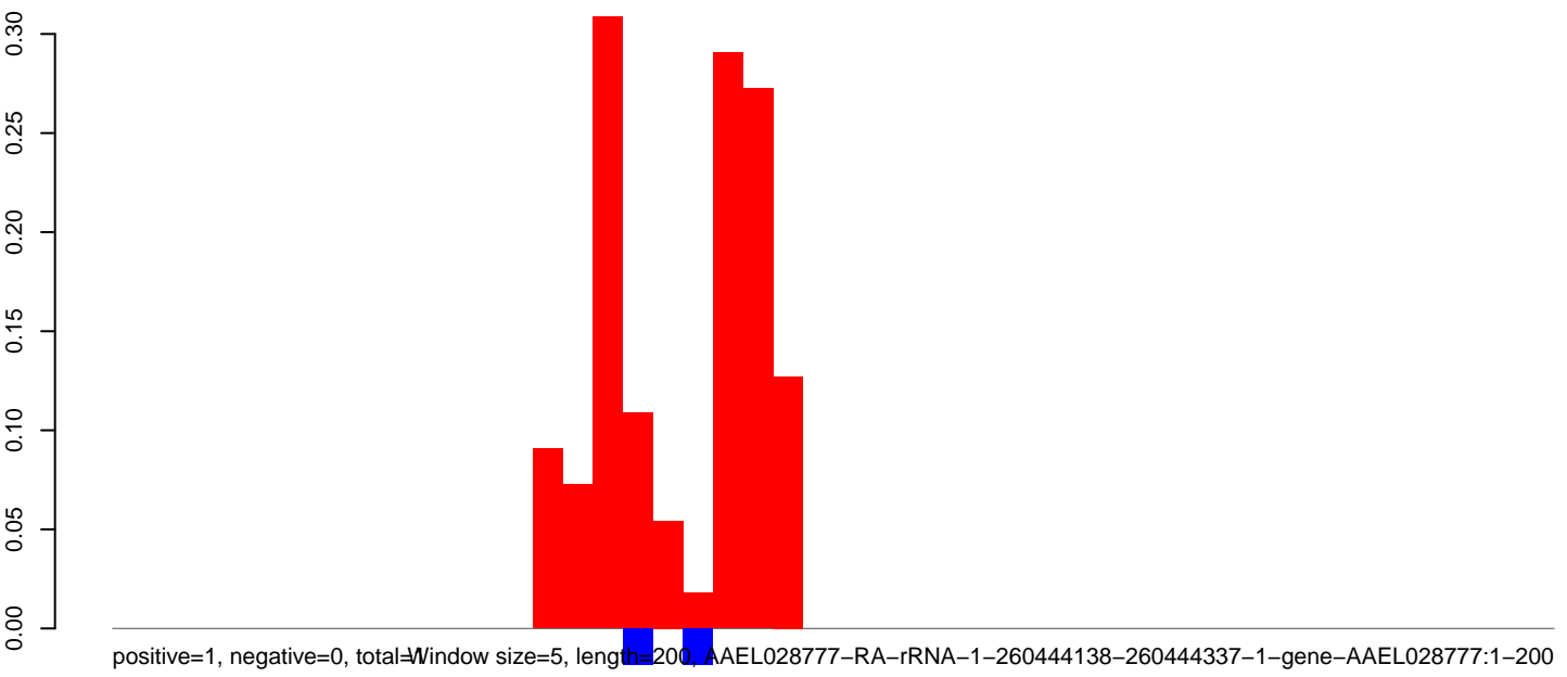
AeAlbo_C636_CHIKV_3dpi.rep
