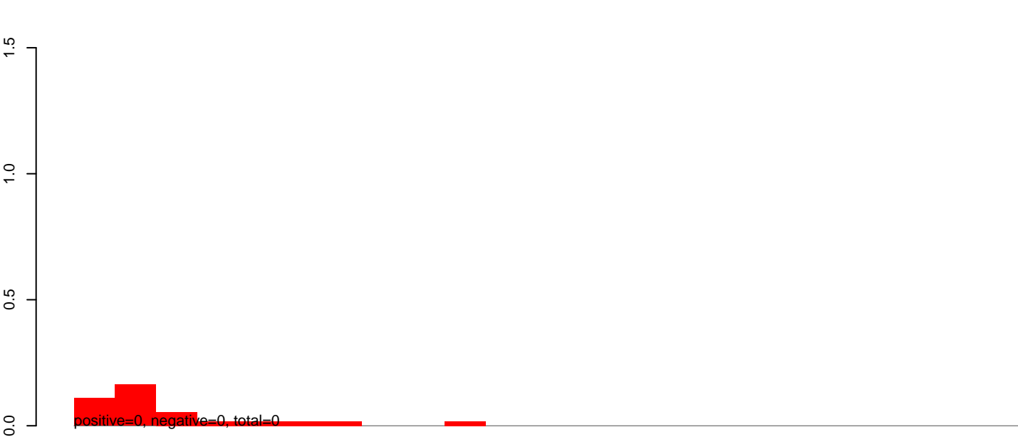
AeAlbo_C636_CHIKV_3dpi.rep
