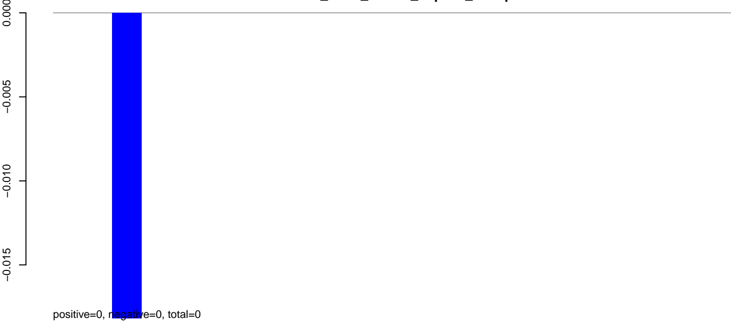
AeAlbo_C636_CHIKV_3dpi.rep
