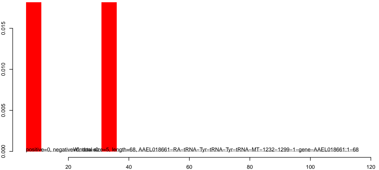
AeAlbo_C636_CHIKV_3dpi.rep
