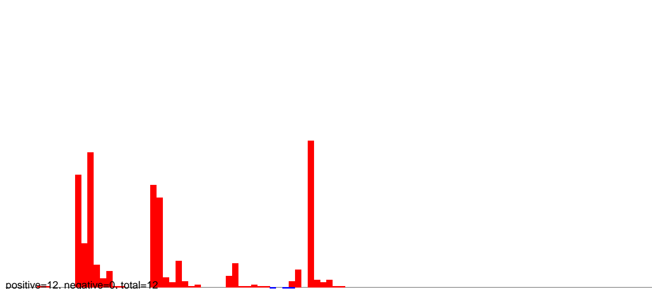
AeAlbo_C636_CHIKV_3dpi.rep
