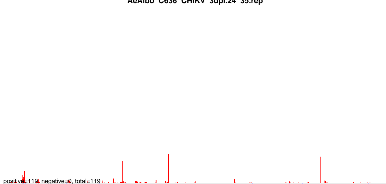
AeAlbo_C636_CHIKV_3dpi.rep
