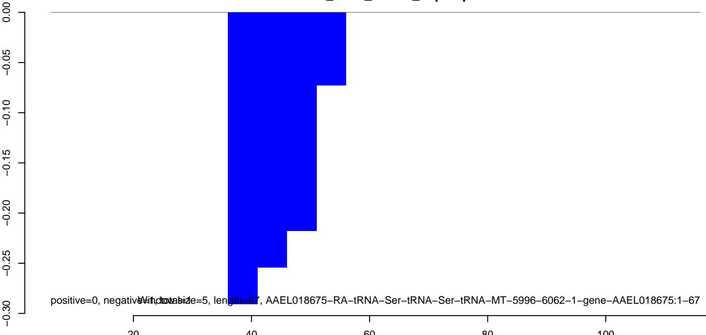
AeAlbo_C636_CHIKV_3dpi.rep
