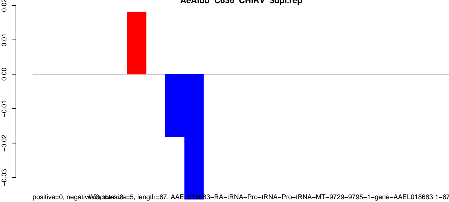
AeAlbo_C636_CHIKV_3dpi.rep
