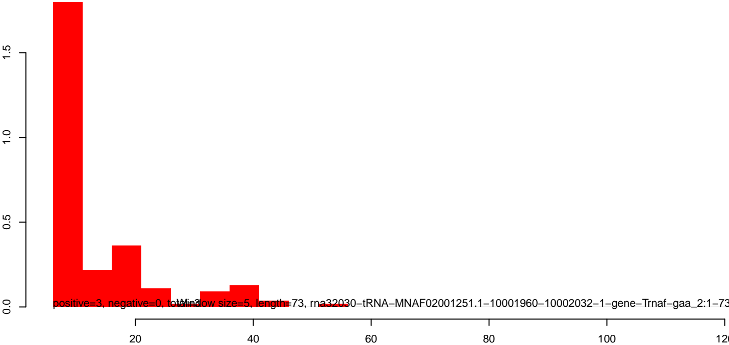
AeAlbo_C636_CHIKV_3dpi.rep
