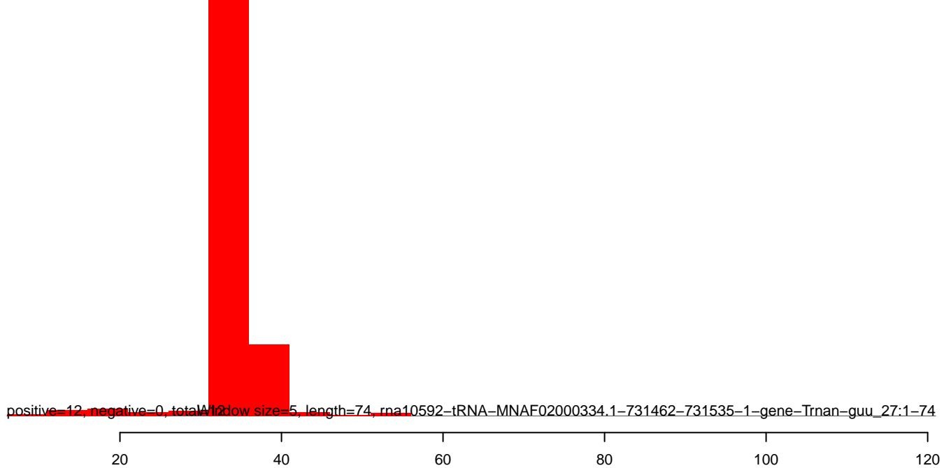
AeAlbo_C636_CHIKV_3dpi.rep
