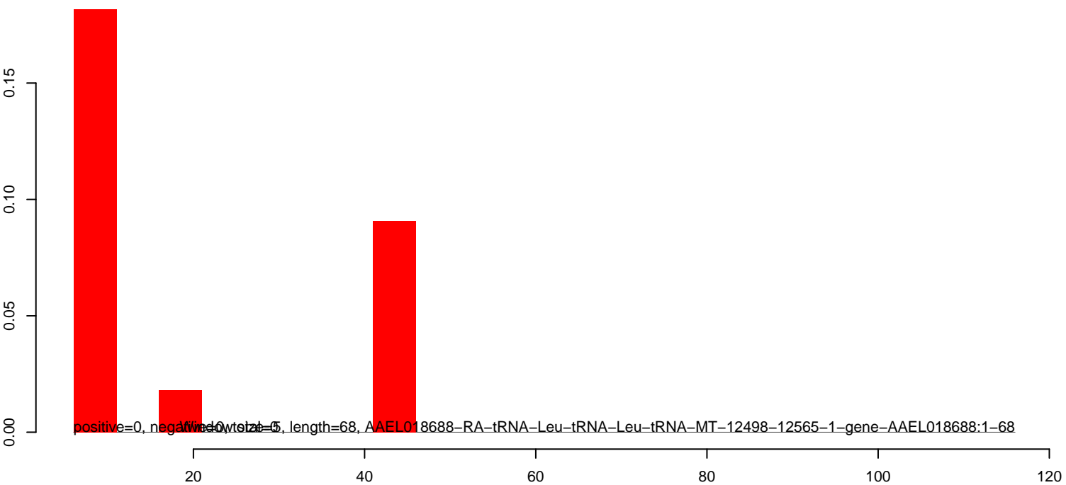
AeAlbo_C636_CHIKV_3dpi.rep
