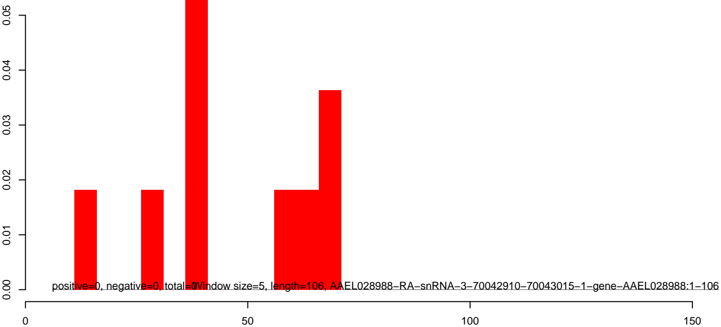
AeAlbo_C636_CHIKV_3dpi.rep
