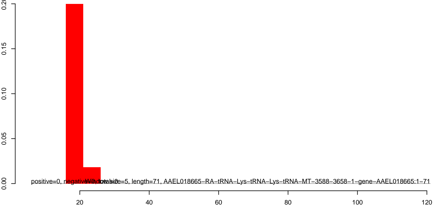
AeAlbo_C636_CHIKV_3dpi.rep
