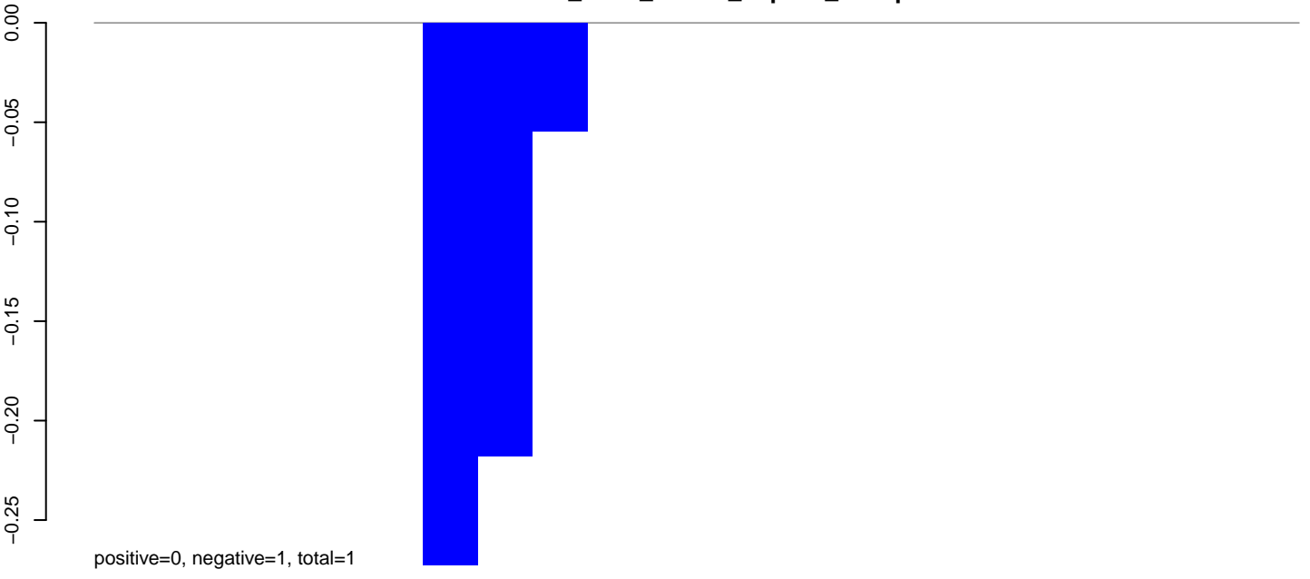
AeAlbo_C636_CHIKV_3dpi.rep
