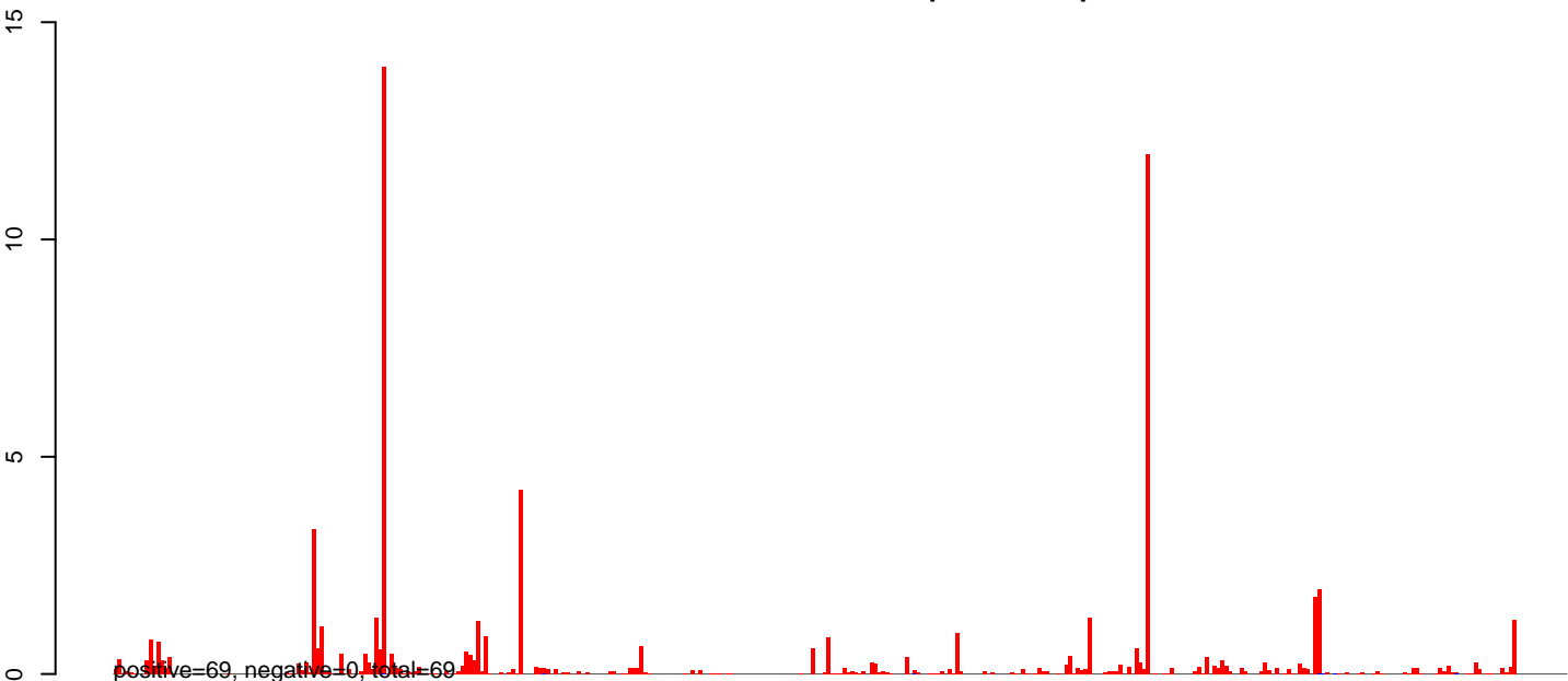
AeAlbo_C636_CHIKV_3dpi.rep
