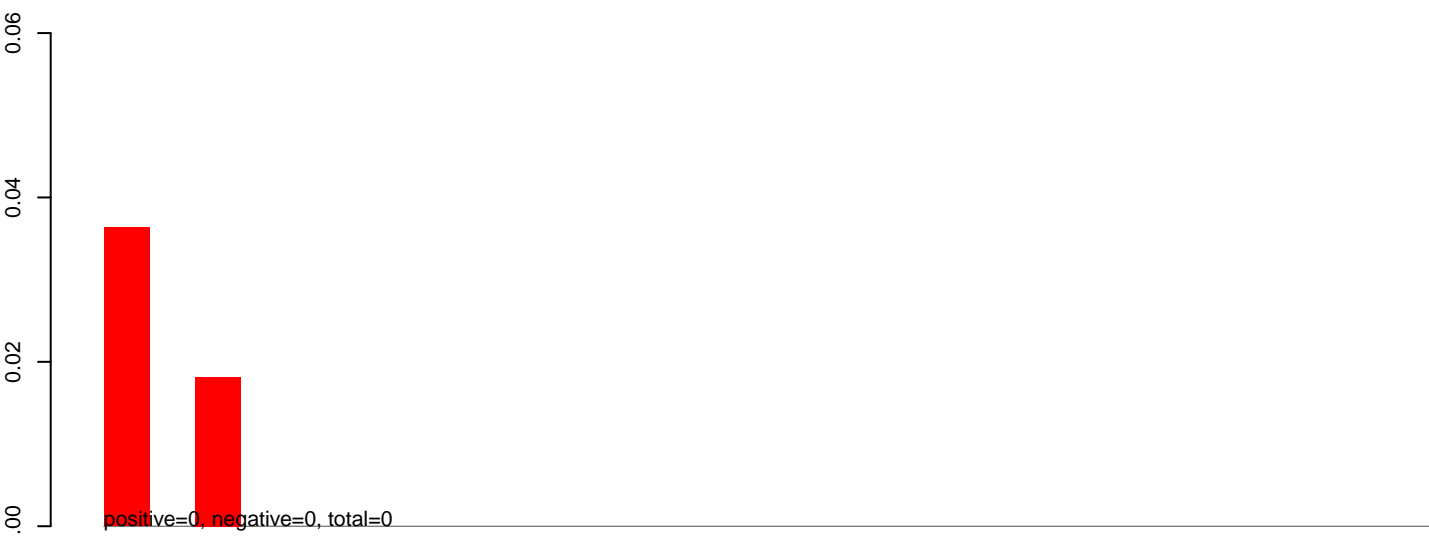
AeAlbo_C636_CHIKV_3dpi.rep
