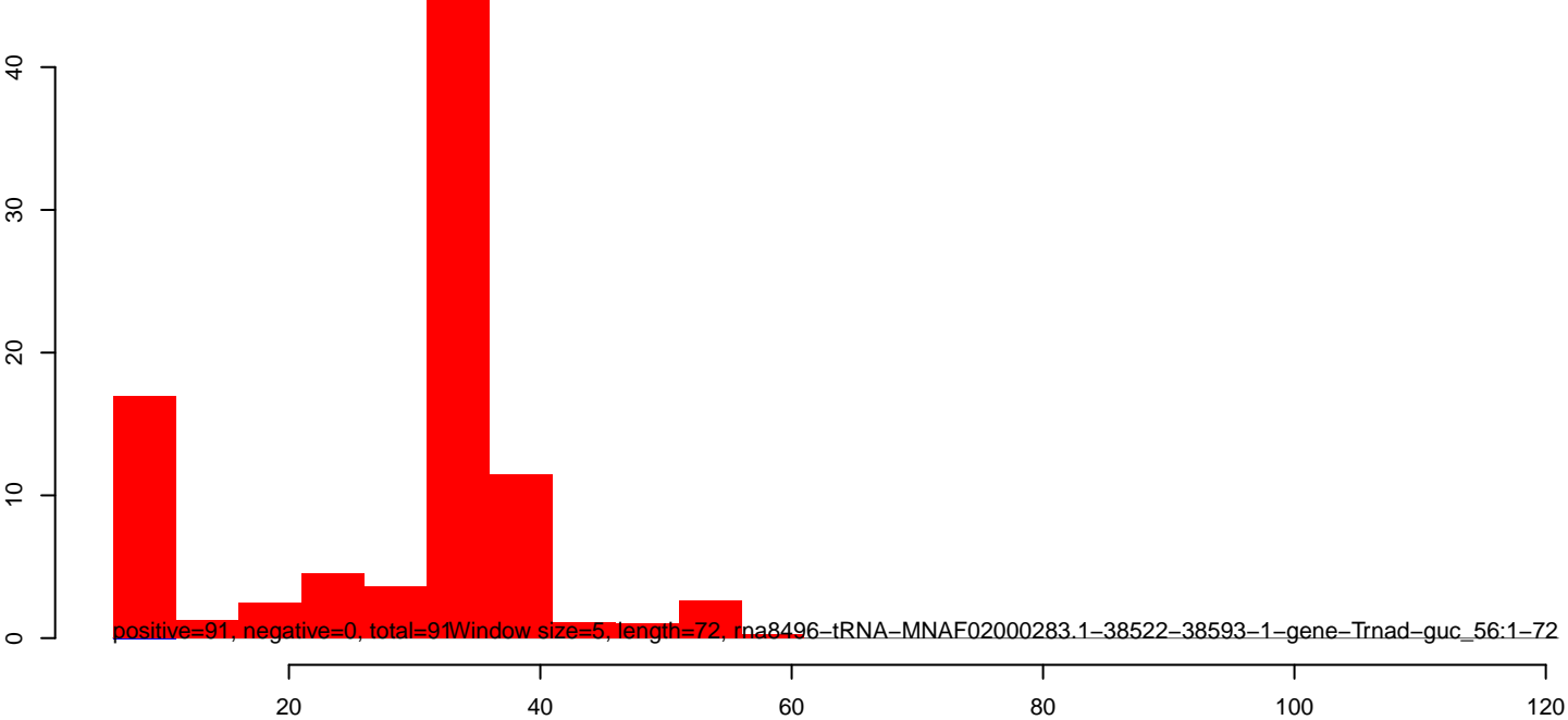
AeAlbo_C636_CHIKV_3dpi.rep
