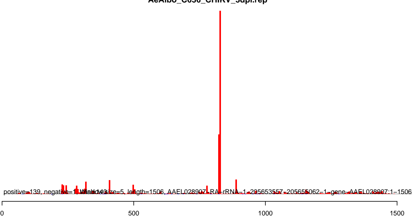
AeAlbo_C636_CHIKV_3dpi.rep
