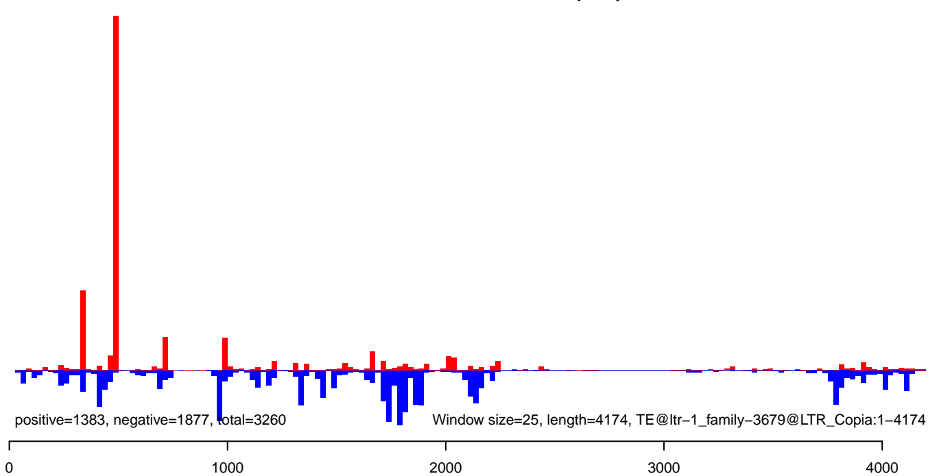
AeAlbo_C636_CHIKV_AZT_3dpi.rep
