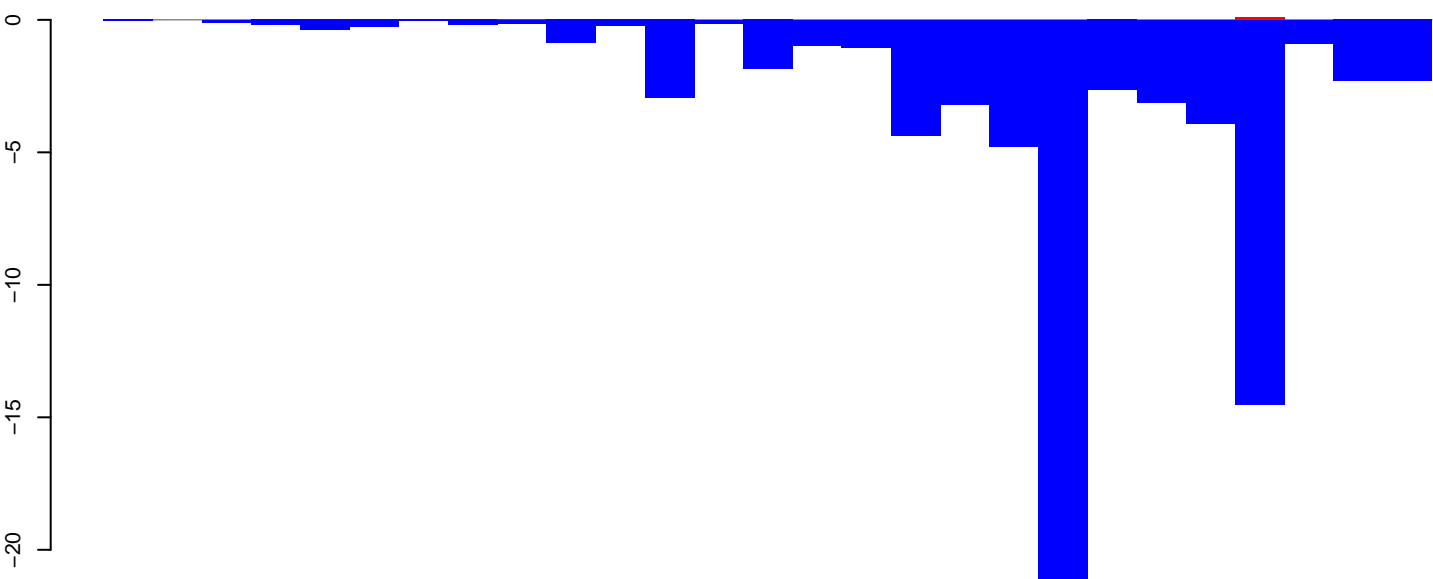
AeAlbo_C636_CHIKV_AZT_3dpi.rep
