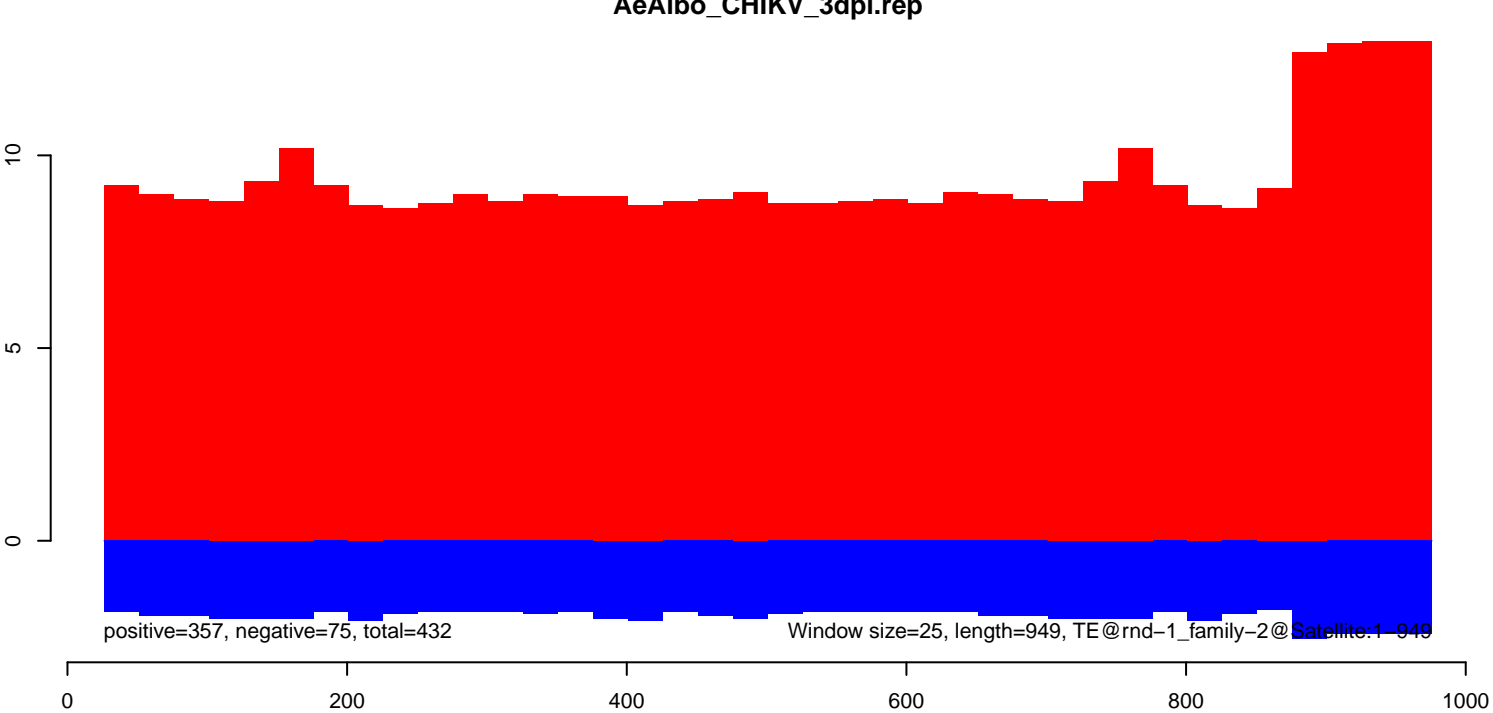
AeAlbo_CHIKV_3dpi.rep
