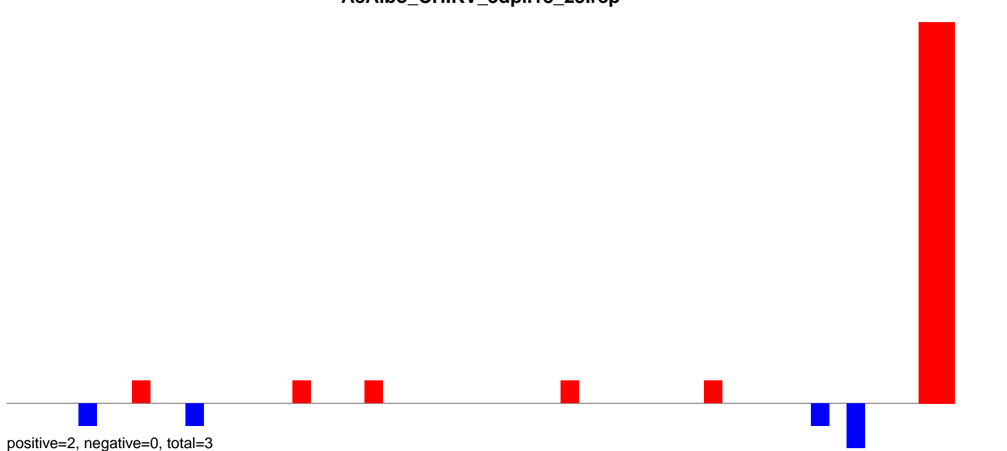
AeAlbo_CHIKV_3dpi.24_35.rep
