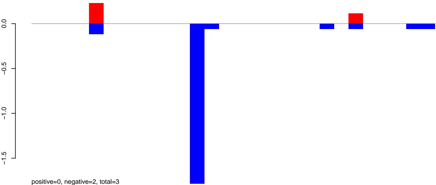
AeAlbo_CHIKV_3dpi.24_35.rep
