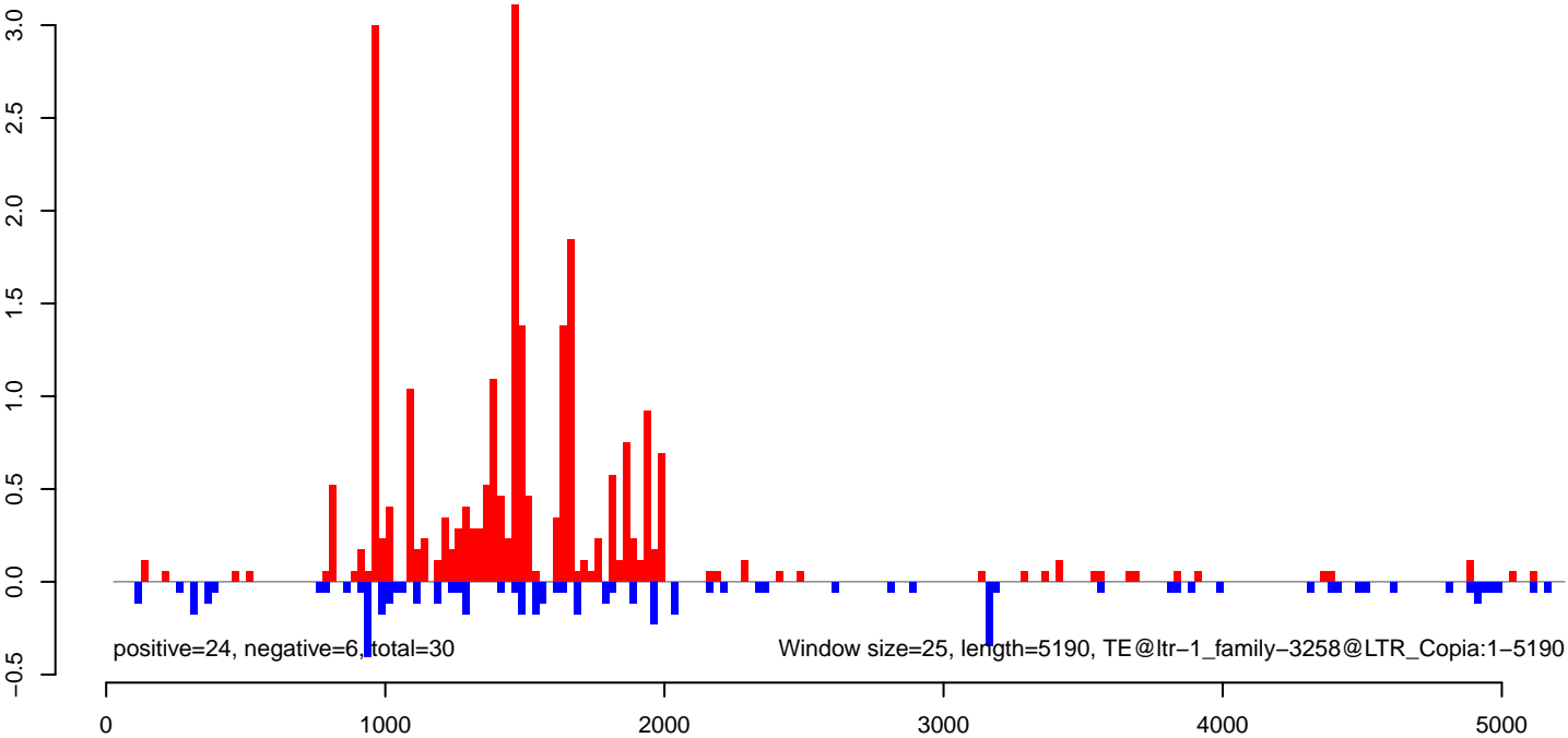
AeAlbo_CHIKV_3dpi.rep
