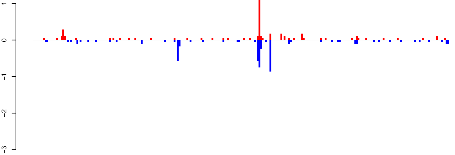
AeAlbo_CHIKV_3dpi.24_35.rep
