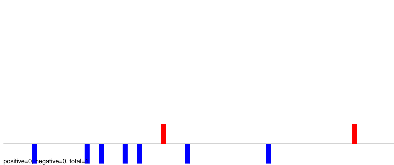
AeAlbo_CHIKV_3dpi.rep
