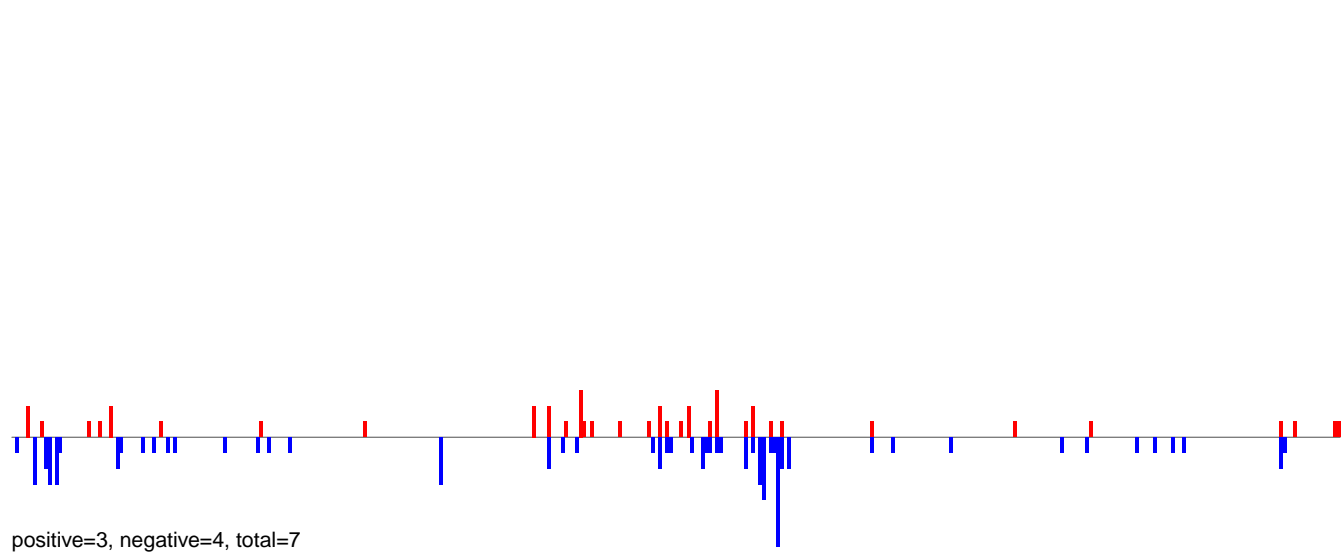
AeAlbo_CHIKV_3dpi.rep
