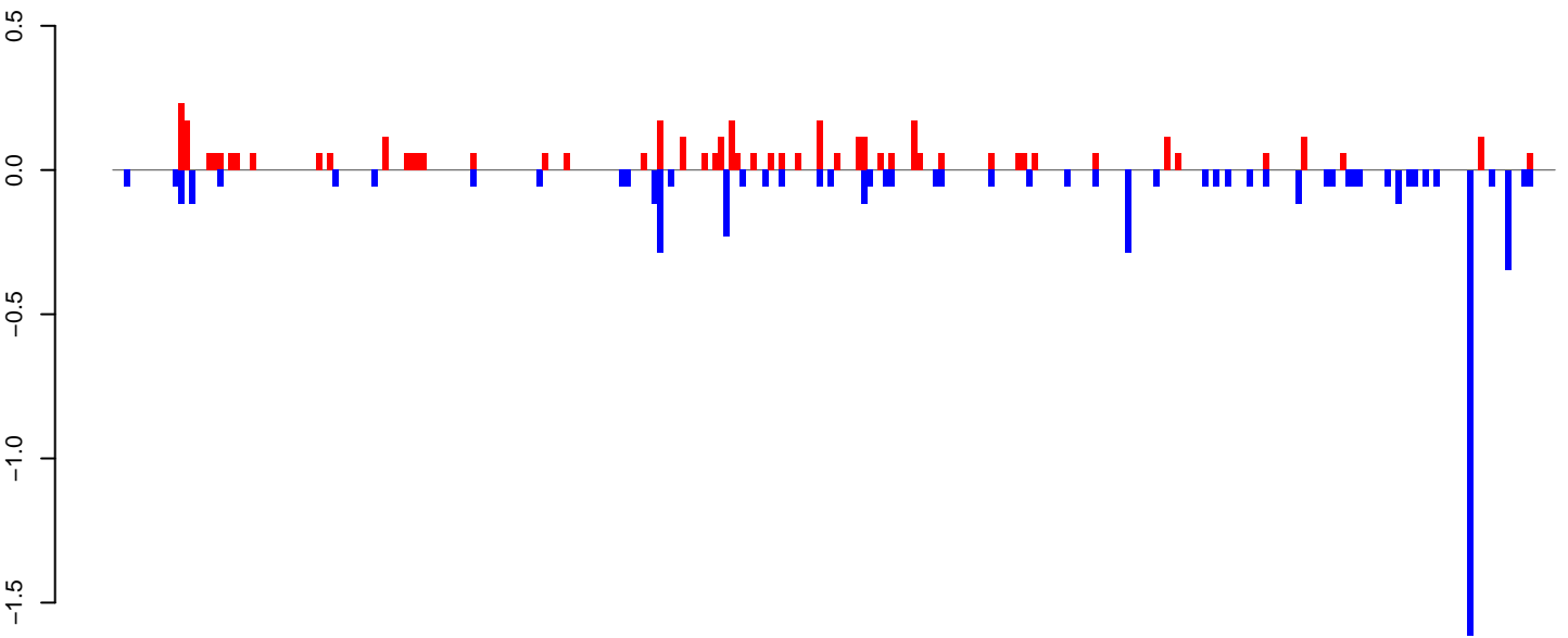
AeAlbo_CHIKV_3dpi.18_23.rep
