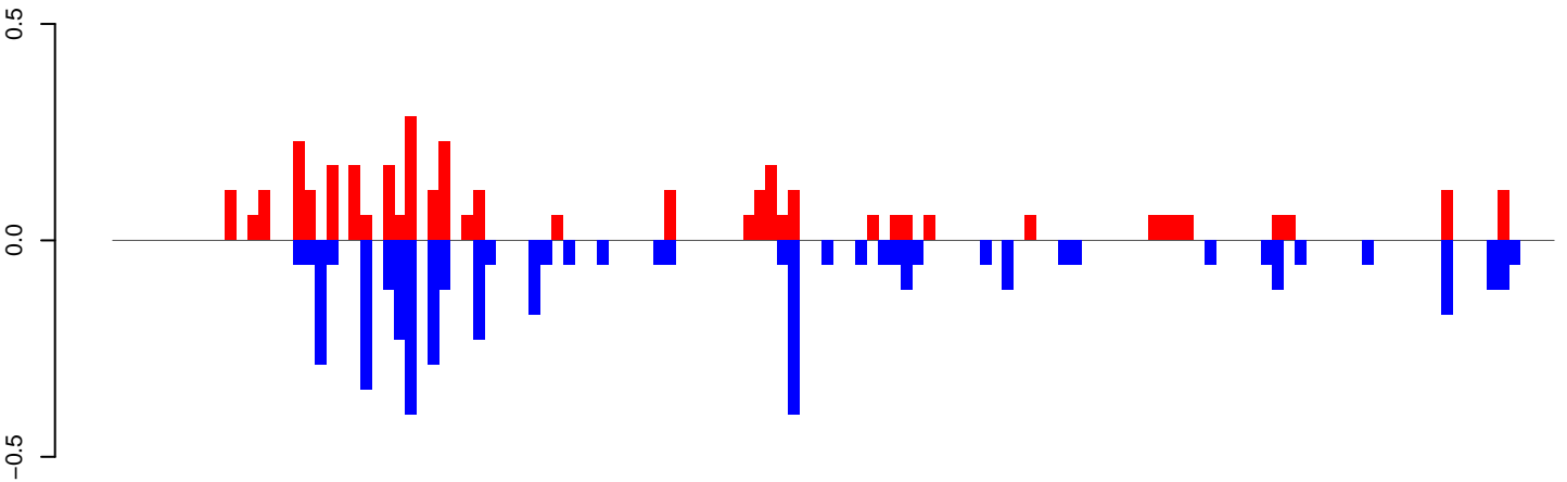
AeAlbo_CHIKV_3dpi.24_35.rep
