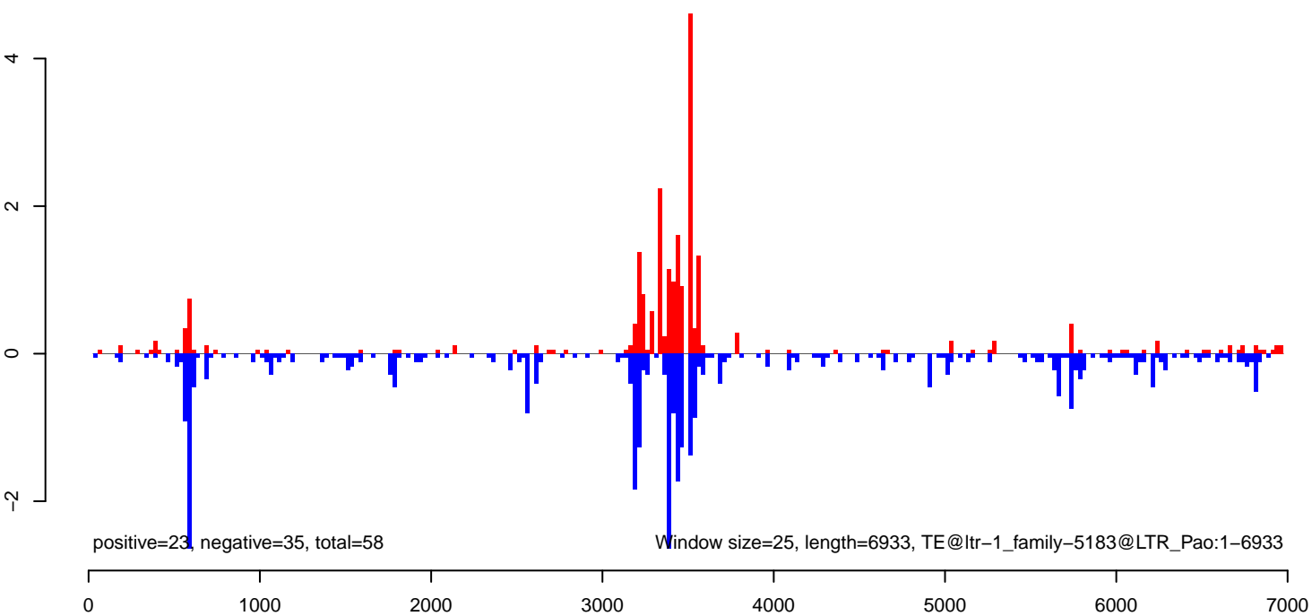
AeAlbo_CHIKV_3dpi.rep
