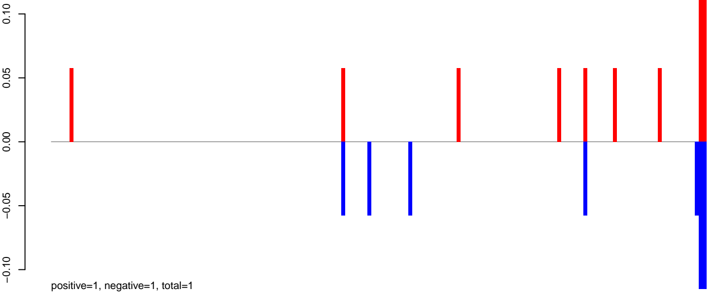
AeAlbo_CHIKV_3dpi.24_35.rep
