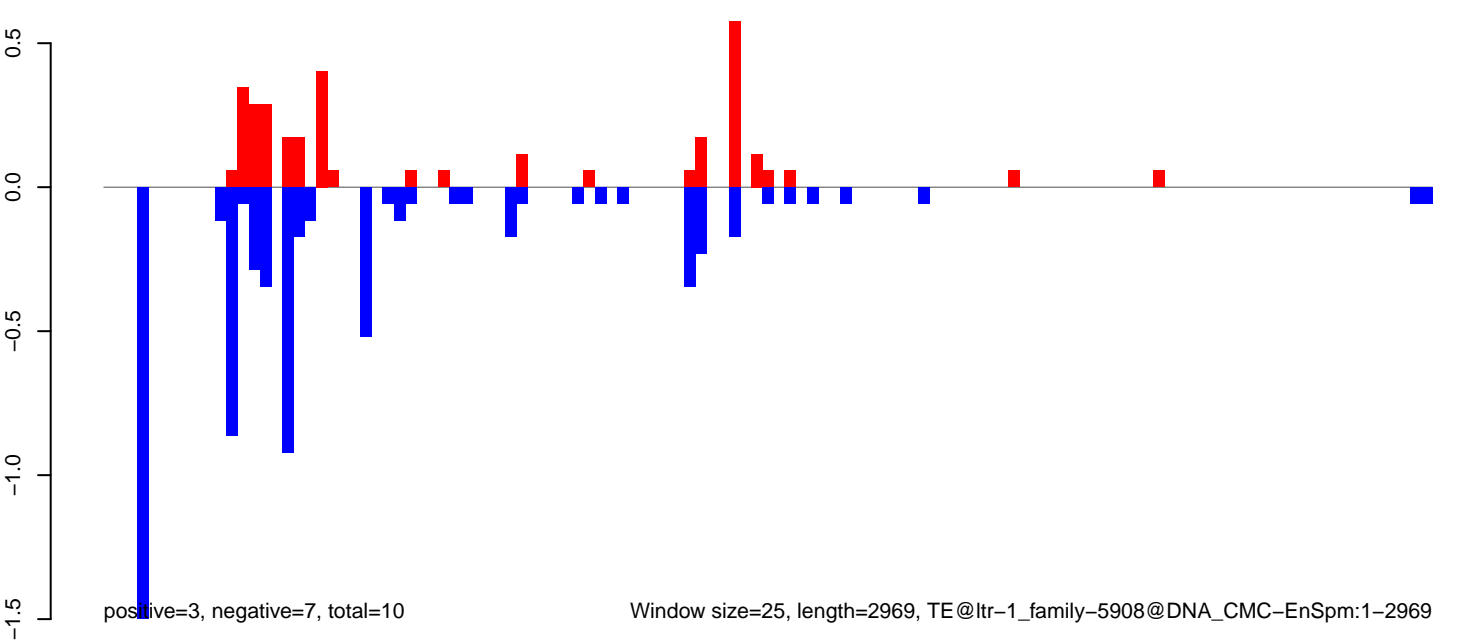
AeAlbo_CHIKV_3dpi.rep
