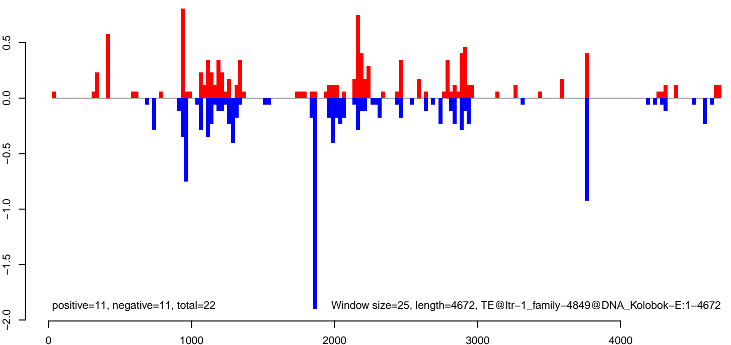
AeAlbo_CHIKV_3dpi.rep
