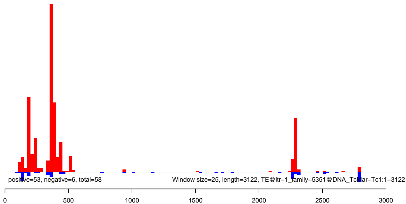
AeAlbo_CHIKV_3dpi.rep
