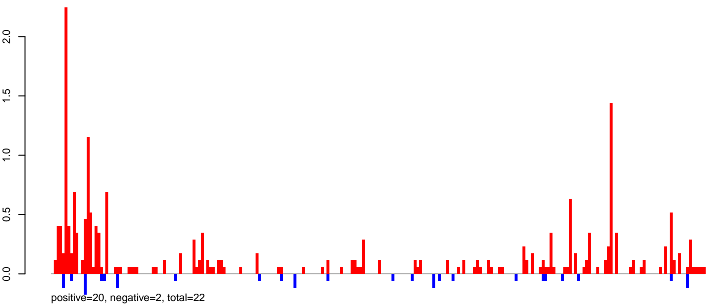
AeAlbo_CHIKV_3dpi.rep
