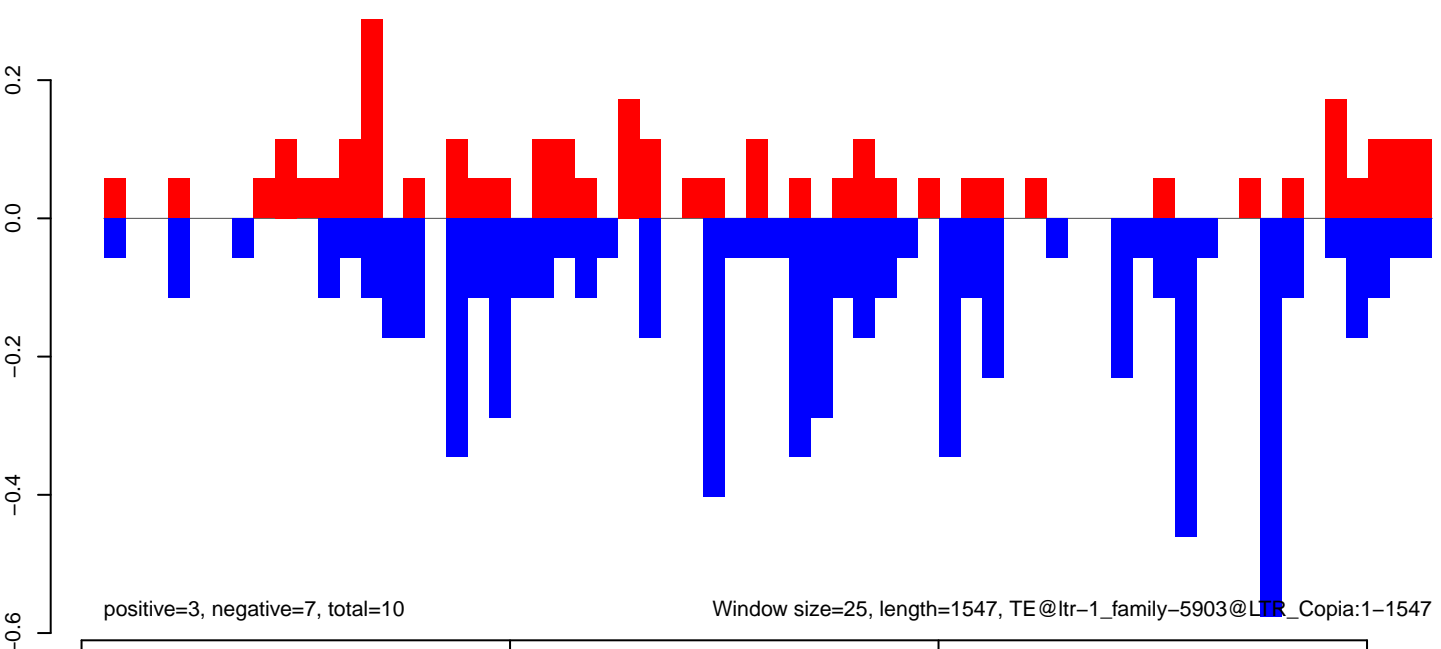
AeAlbo_CHIKV_3dpi.rep
