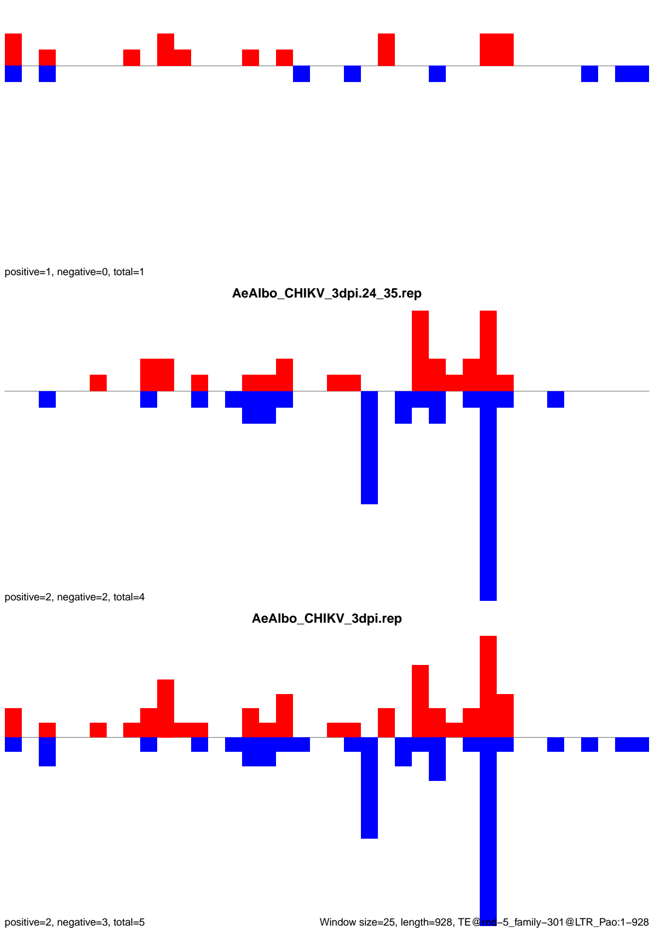
AeAlbo_CHIKV_3dpi.18_23.rep
