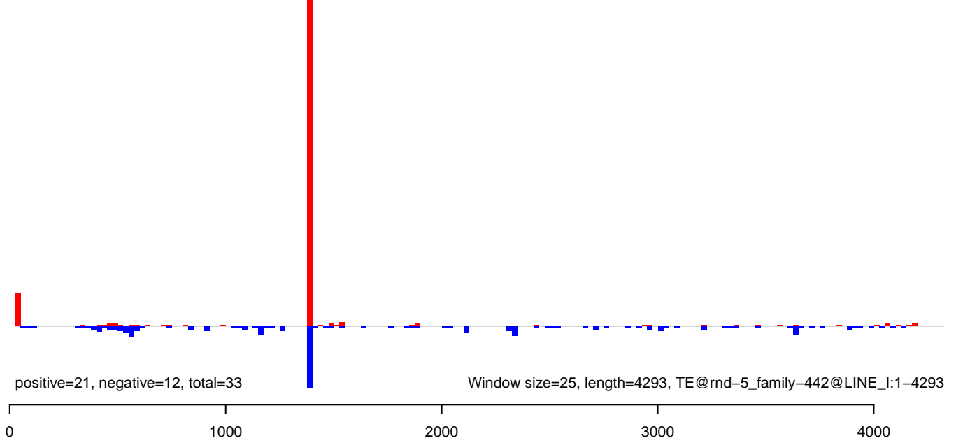
AeAlbo_CHIKV_3dpi.rep
