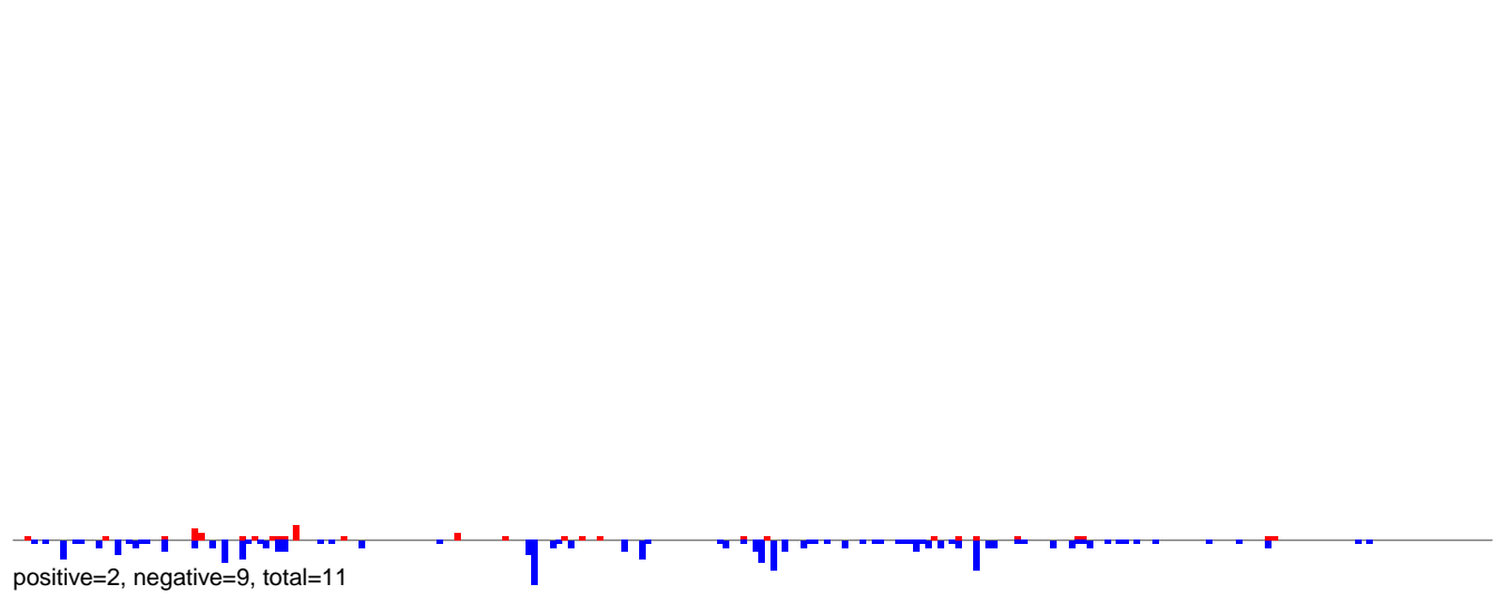
AeAlbo_CHIKV_3dpi.rep
