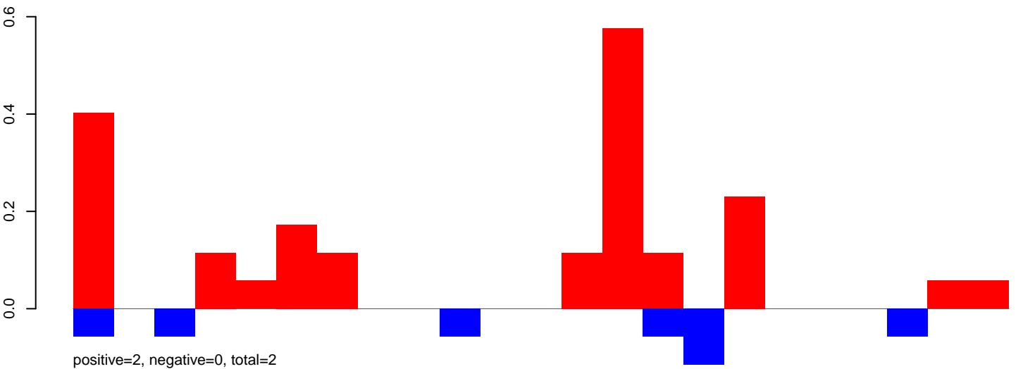
AeAlbo_CHIKV_3dpi.24_35.rep
