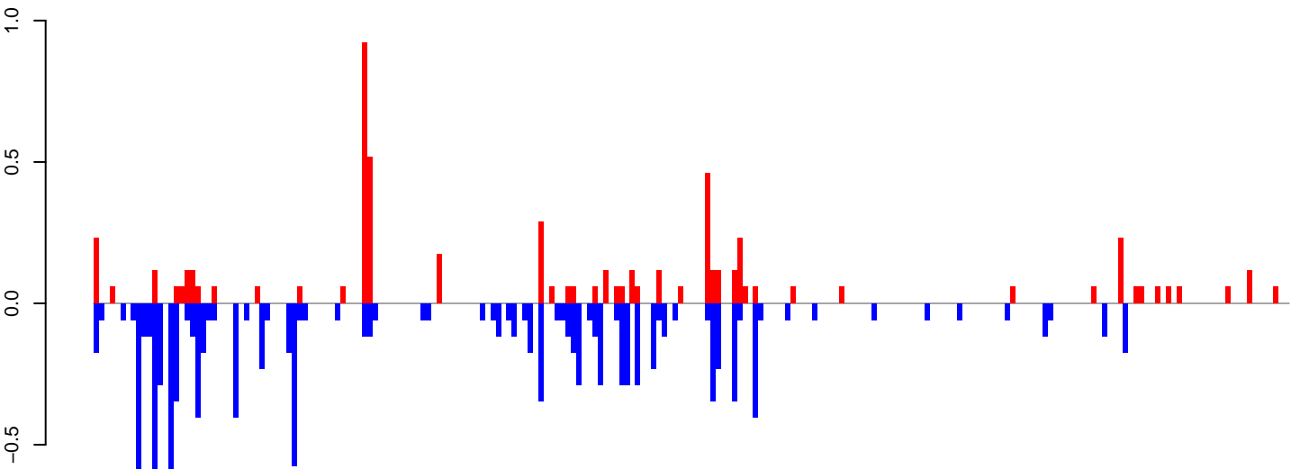
AeAlbo_CHIKV_3dpi.24_35.rep
