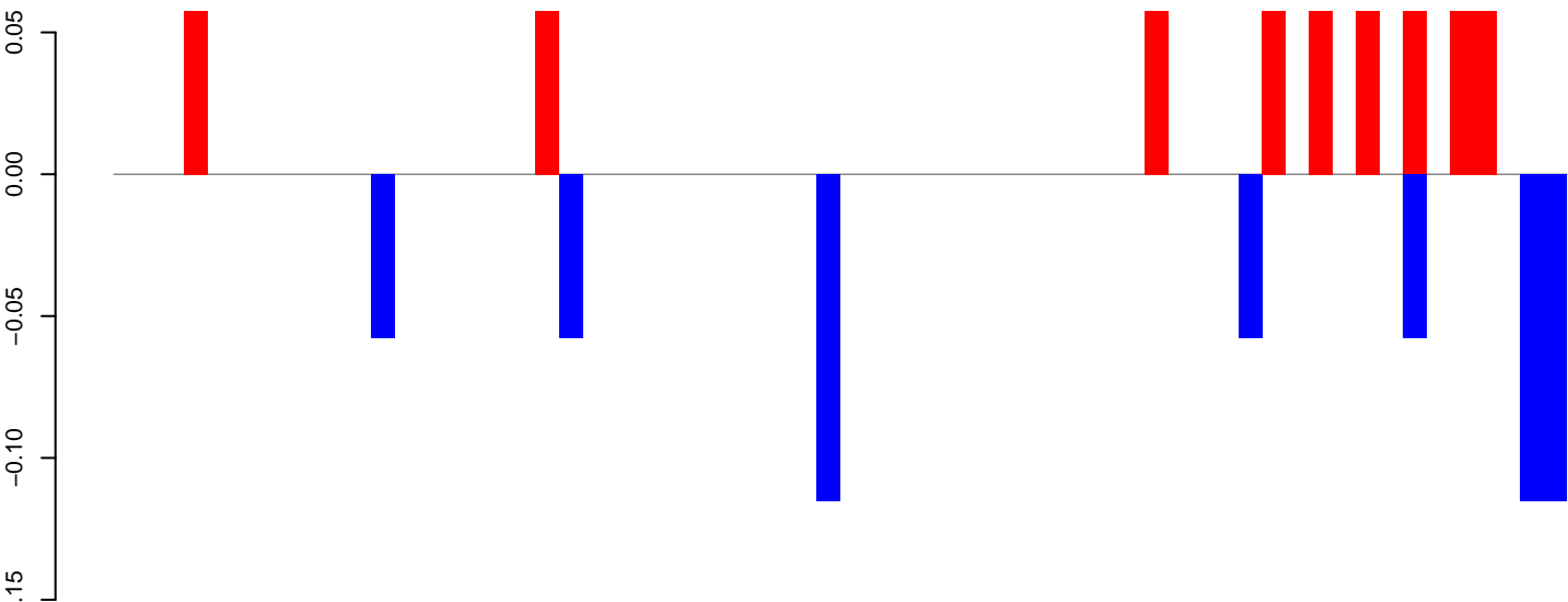
AeAlbo_CHIKV_3dpi.18_23.rep
