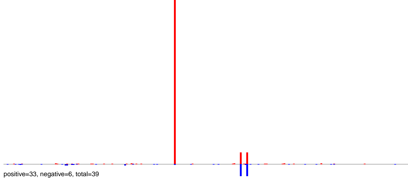
AeAlbo_CHIKV_3dpi.24_35.rep
