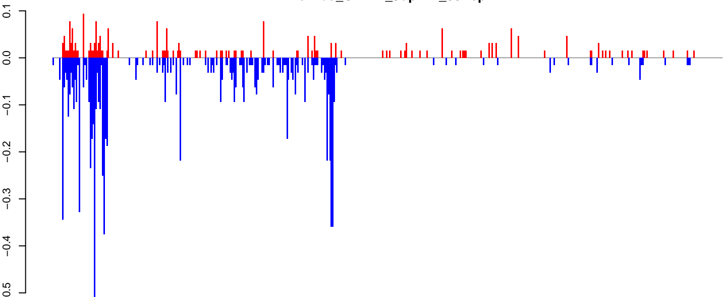
AeAlbo_CHIKV_9dpi.24_35.rep
