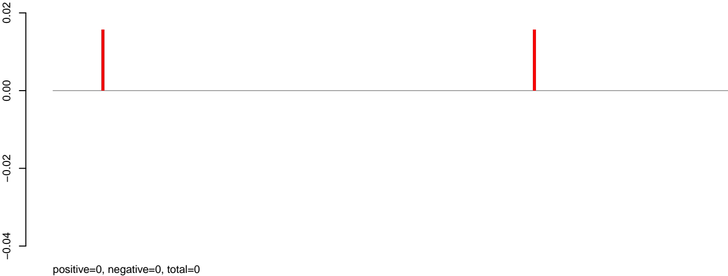
AeAlbo_CHIKV_9dpi.rep
