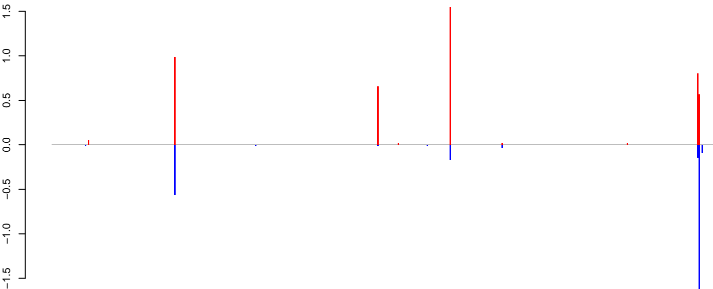
AeAlbo_CHIKV_9dpi.18_23.rep
