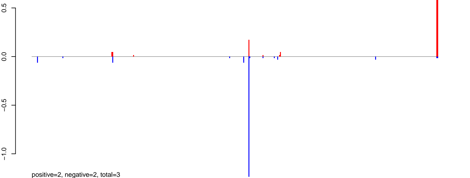
AeAlbo_CHIKV_9dpi.24_35.rep
