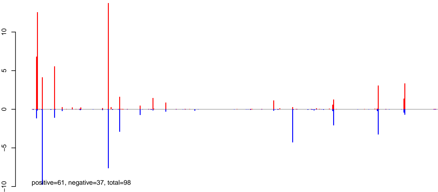
AeAlbo_CHIKV_9dpi.24_35.rep
