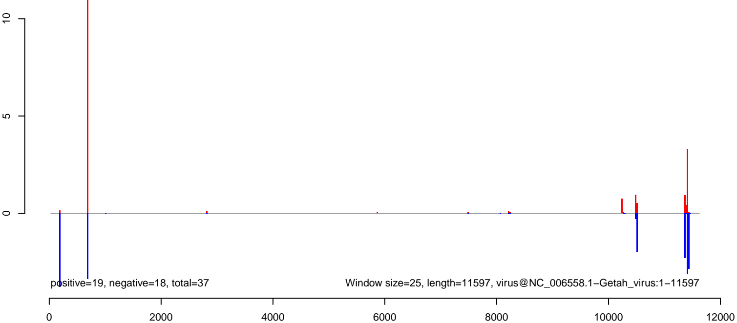
AeAlbo_CHIKV_9dpi.rep
