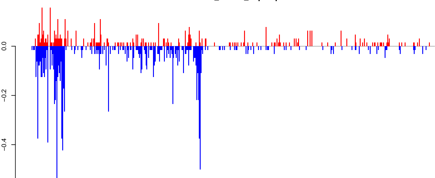
AeAlbo_CHIKV_9dpi.rep
