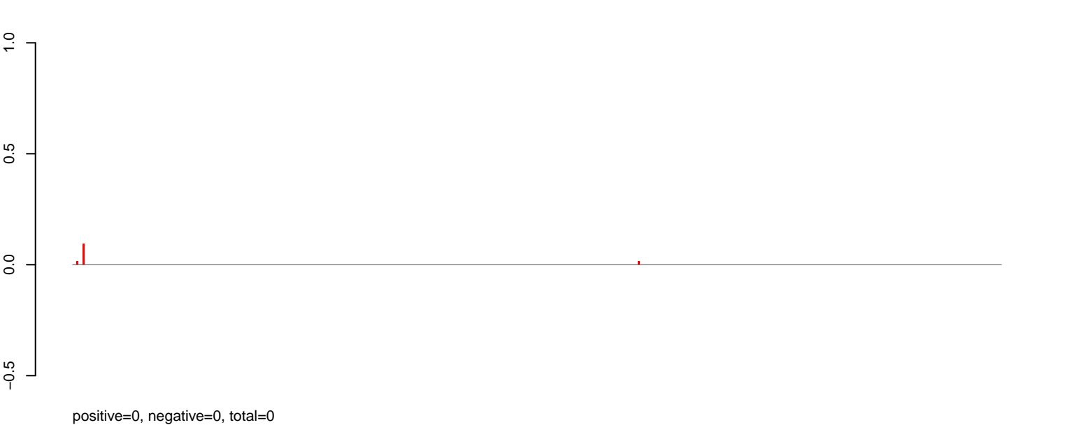
AeAlbo_CHIKV_9dpi.rep
