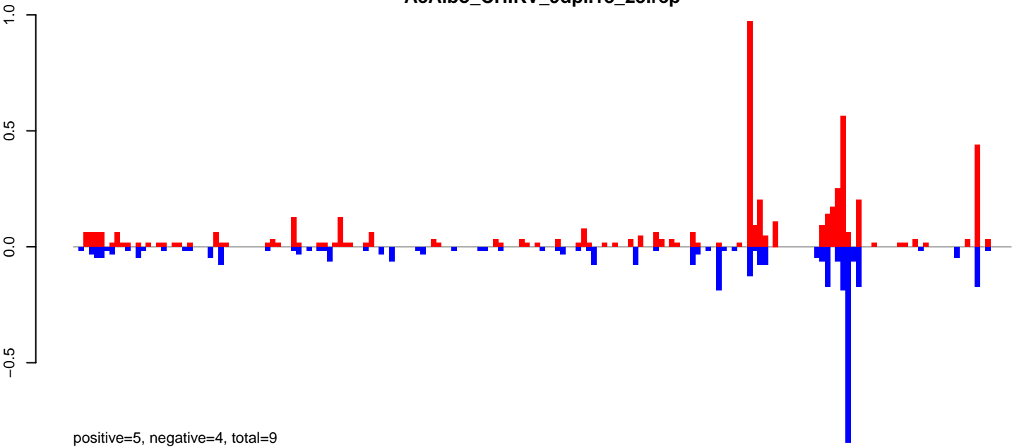
AeAlbo_CHIKV_9dpi.24_35.rep
