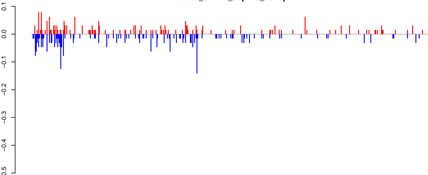
AeAlbo_CHIKV_9dpi.18_23.rep
