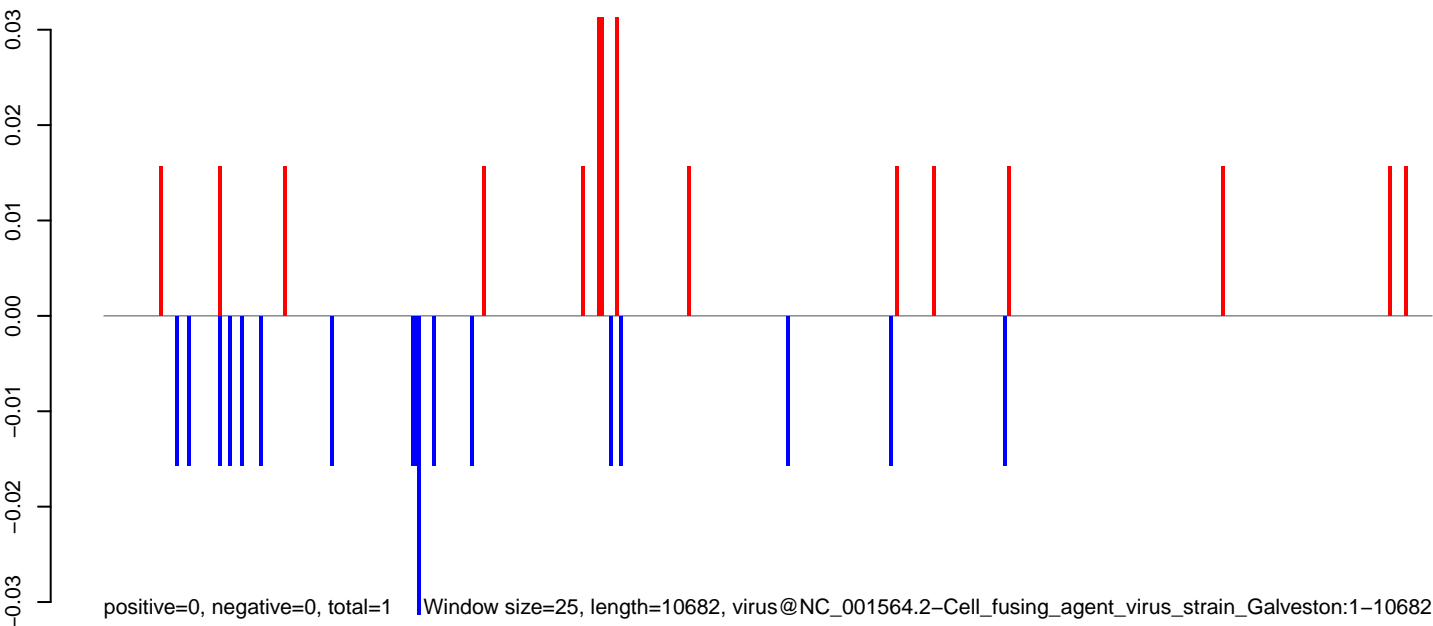
AeAlbo_CHIKV_9dpi.rep
