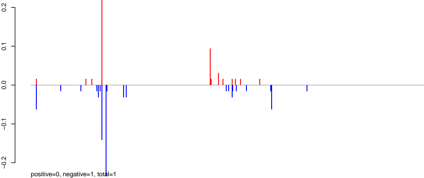
AeAlbo_CHIKV_9dpi.24_35.rep
