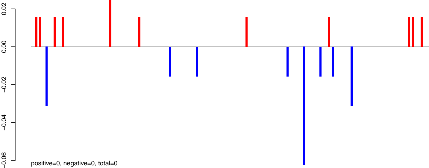
AeAlbo_CHIKV_9dpi.24_35.rep
