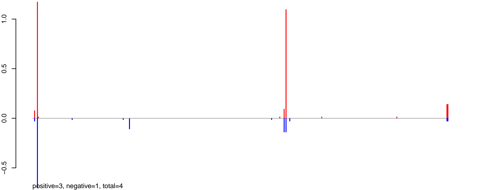
AeAlbo_CHIKV_9dpi.24_35.rep
