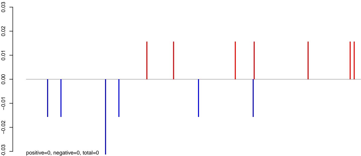
AeAlbo_CHIKV_9dpi.24_35.rep
