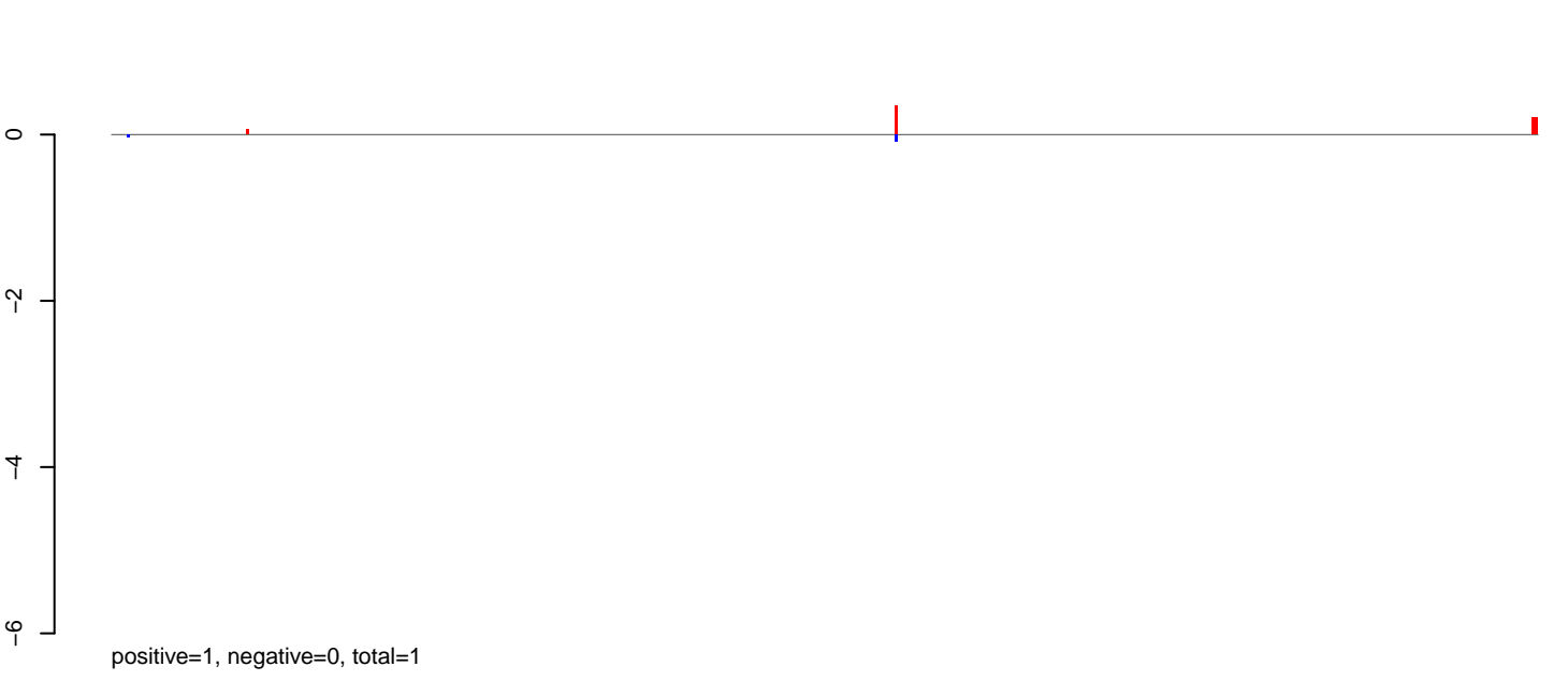
AeAlbo_CHIKV_9dpi.rep
