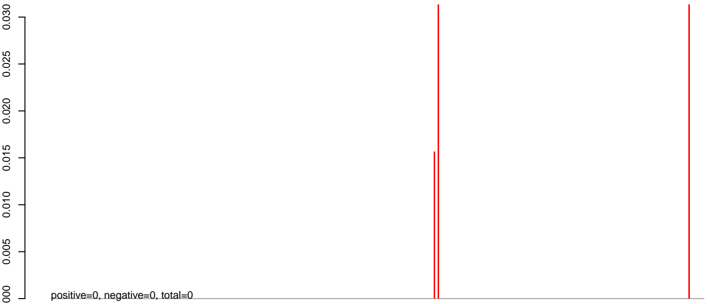
AeAlbo_CHIKV_9dpi.24_35.rep
