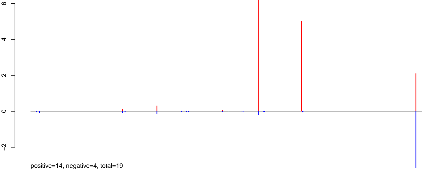
AeAlbo_CHIKV_9dpi.24_35.rep
