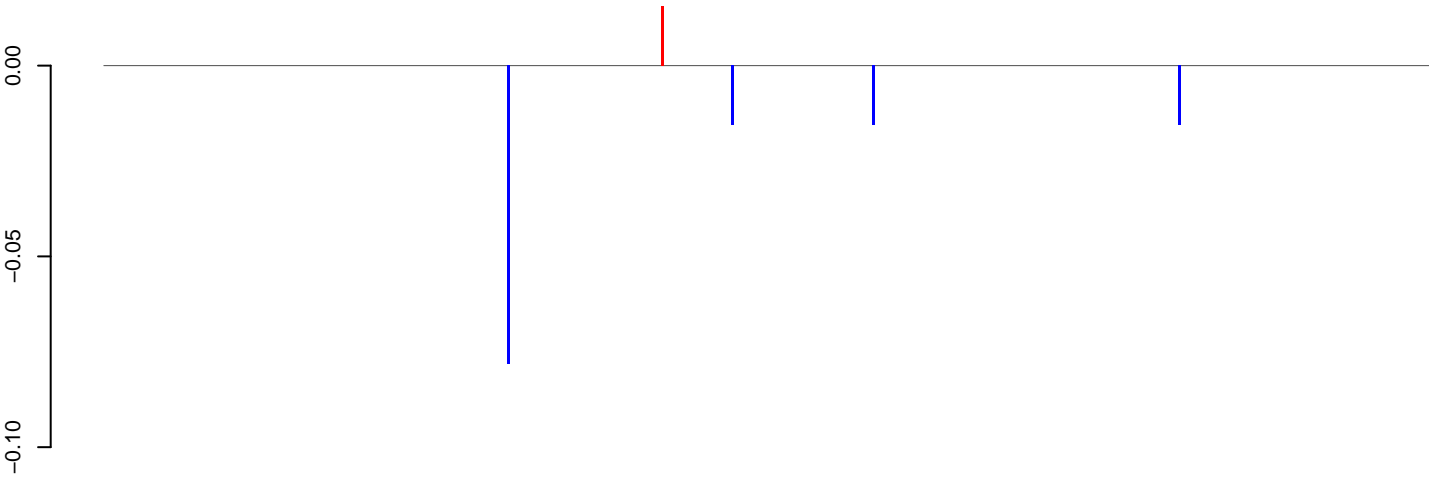
AeAlbo_CHIKV_9dpi.18_23.rep
