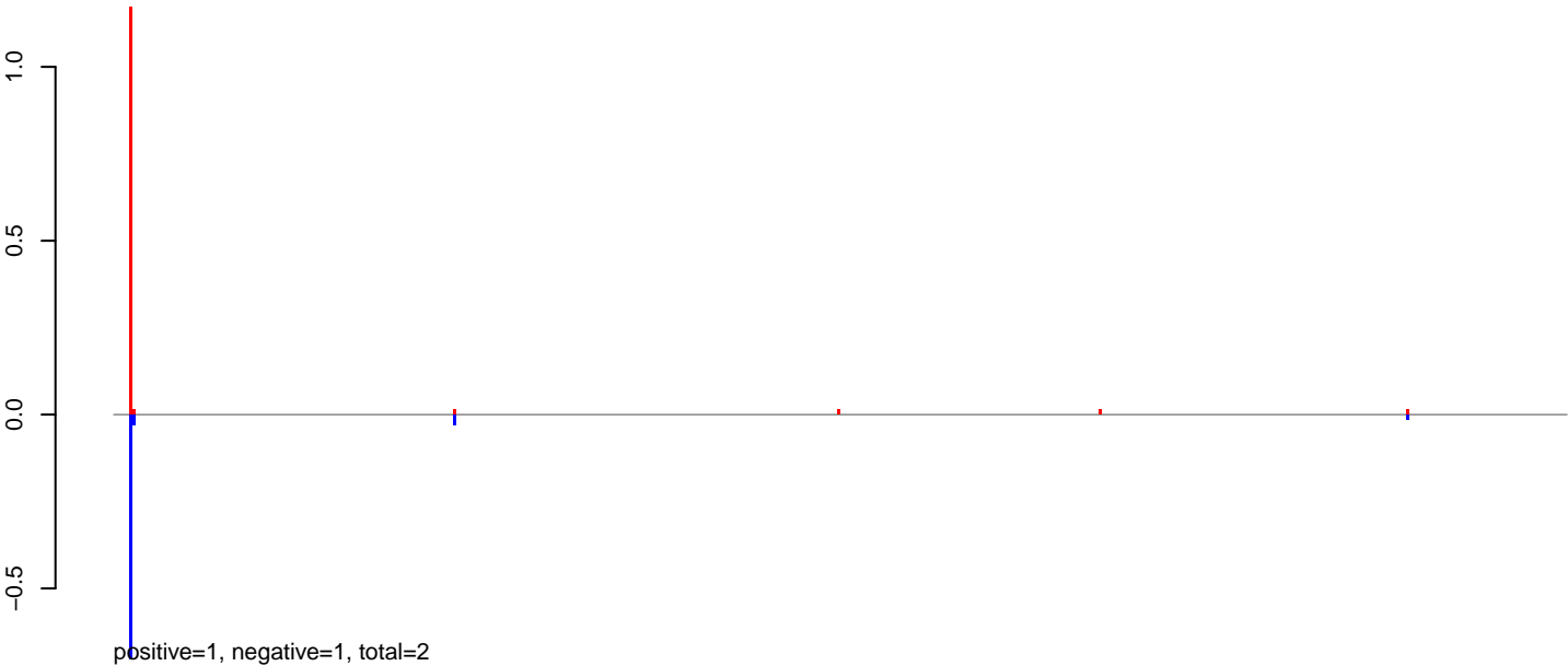
AeAlbo_CHIKV_9dpi.24_35.rep
