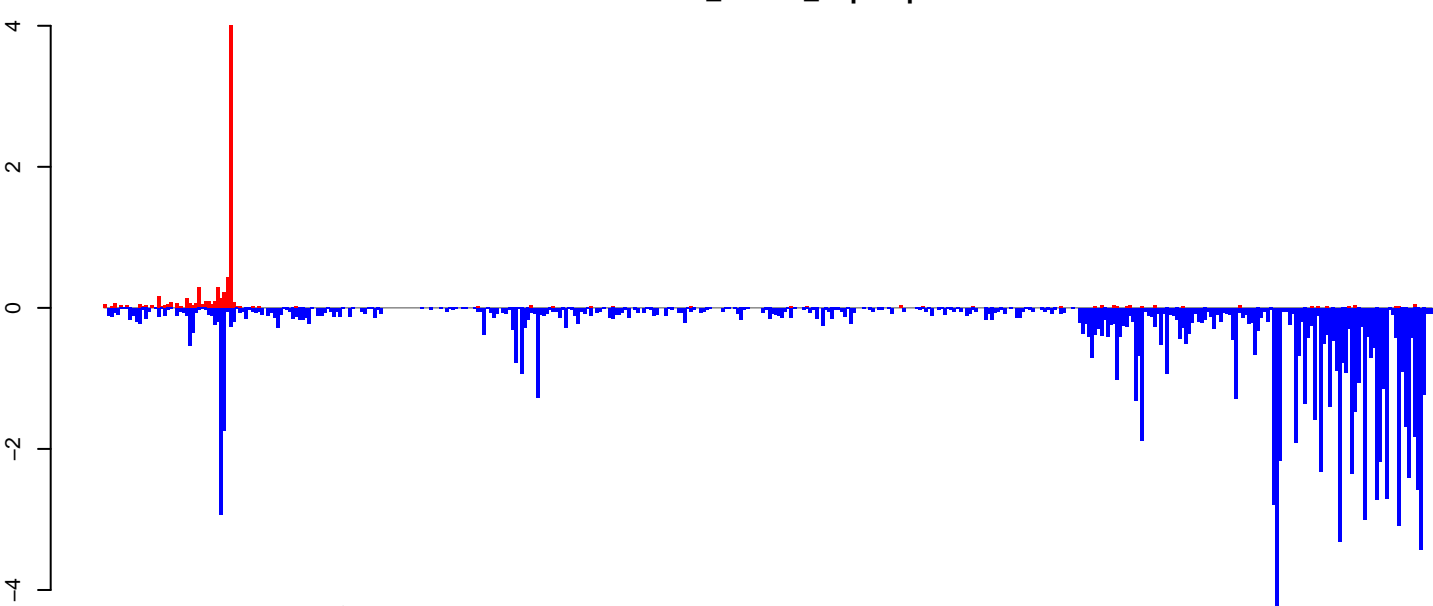
AeAlbo_CHIKV_9dpi.rep
