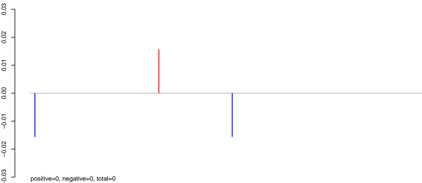
AeAlbo_CHIKV_9dpi.rep
