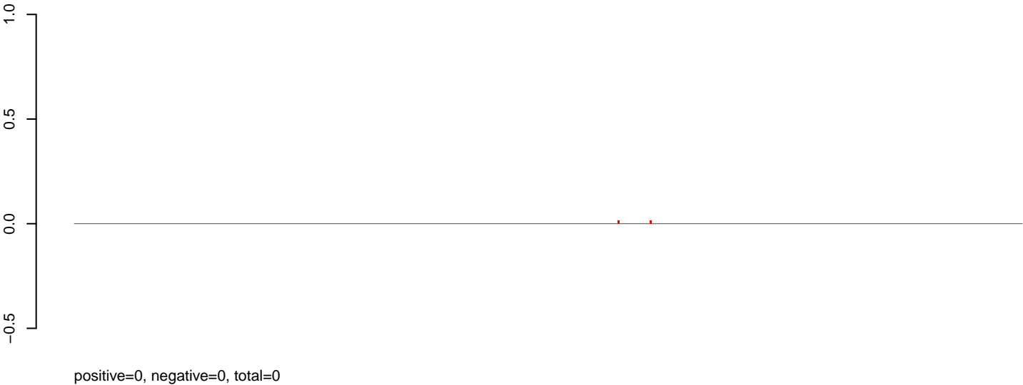
AeAlbo_CHIKV_9dpi.rep
