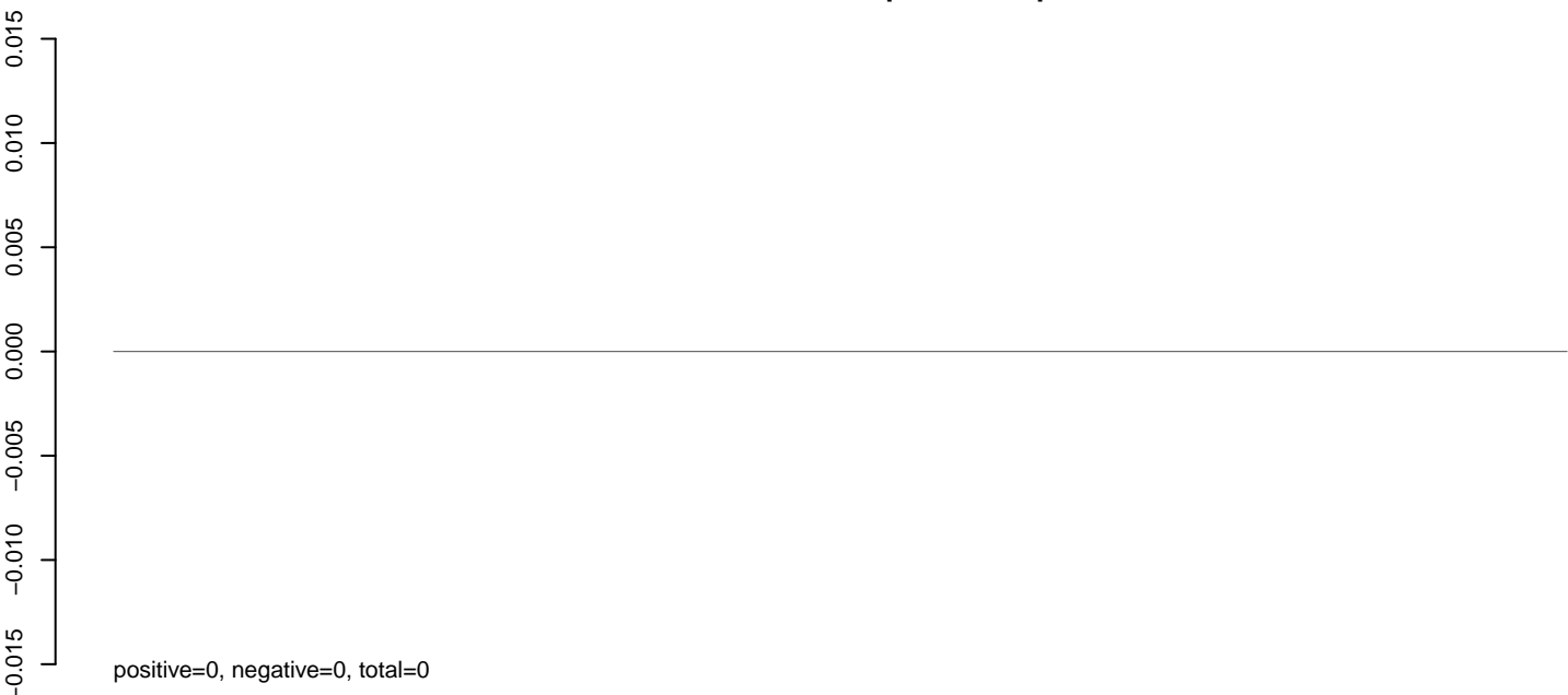
AeAlbo_CHIKV_9dpi.rep
