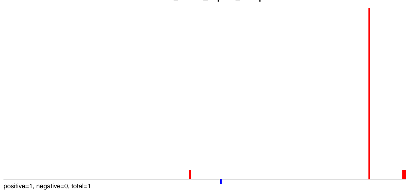
AeAlbo_CHIKV_9dpi.24_35.rep
