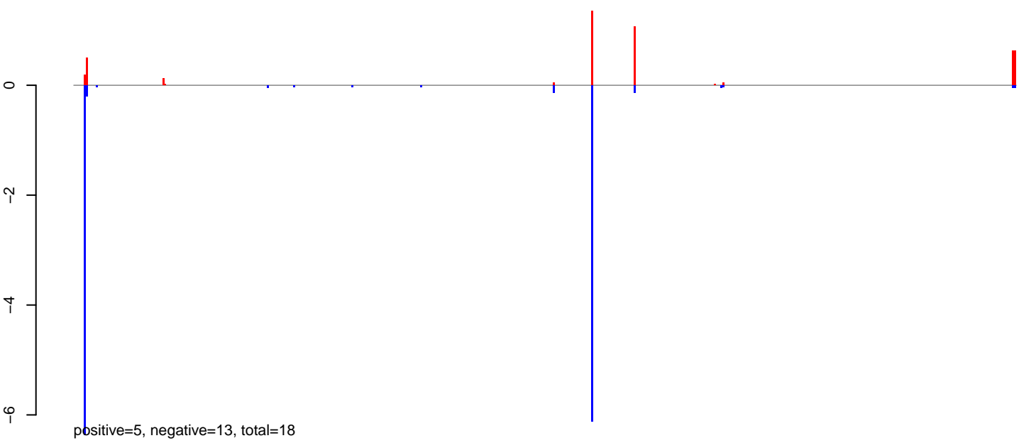
AeAlbo_CHIKV_9dpi.24_35.rep
