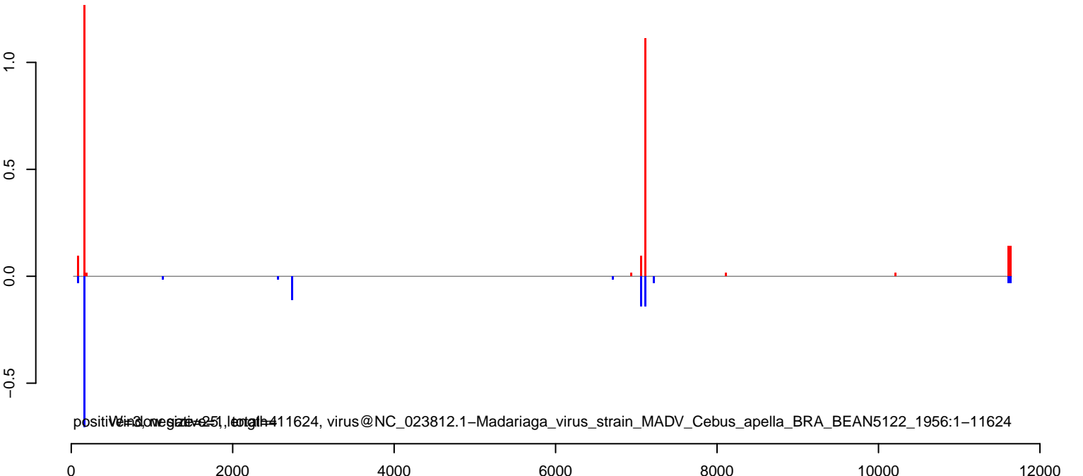
AeAlbo_CHIKV_9dpi.rep
