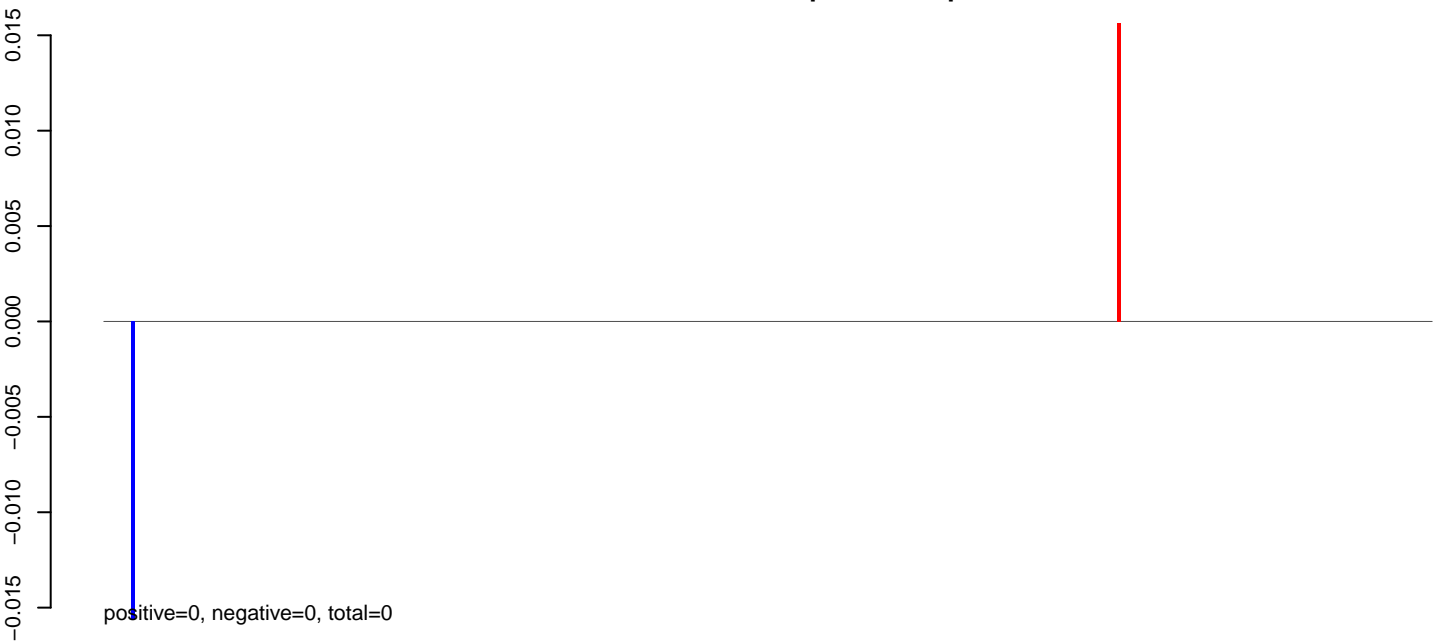
AeAlbo_CHIKV_9dpi.24_35.rep
