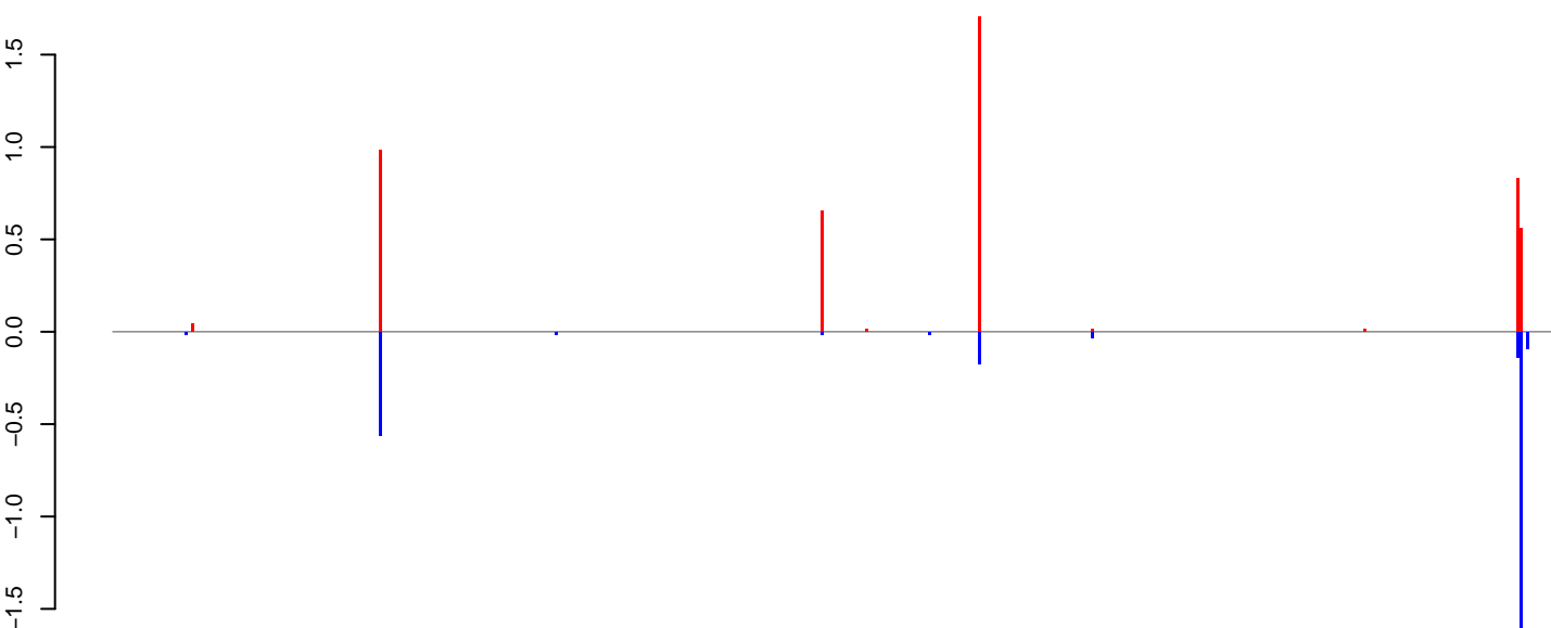
AeAlbo_CHIKV_9dpi.rep
