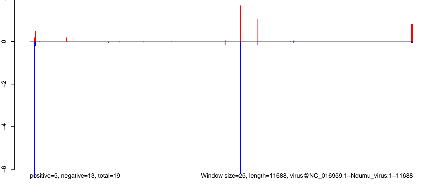
AeAlbo_CHIKV_9dpi.rep
