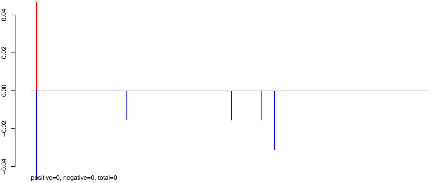
AeAlbo_CHIKV_9dpi.24_35.rep
