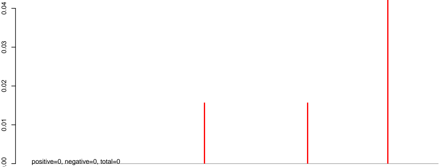
AeAlbo_CHIKV_9dpi.24_35.rep
