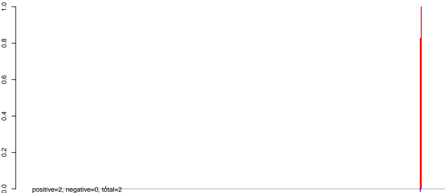
AeAlbo_CHIKV_9dpi.24_35.rep
