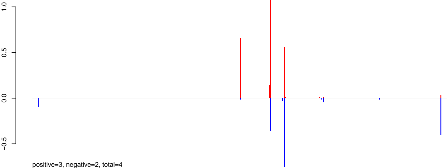
AeAlbo_CHIKV_9dpi.24_35.rep
