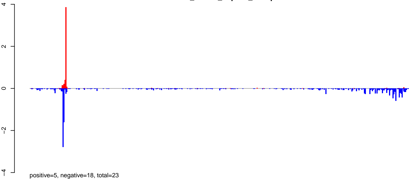
AeAlbo_CHIKV_9dpi.24_35.rep
