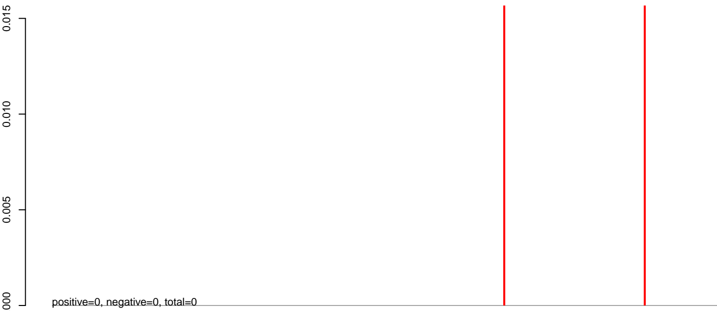
AeAlbo_CHIKV_9dpi.24_35.rep
