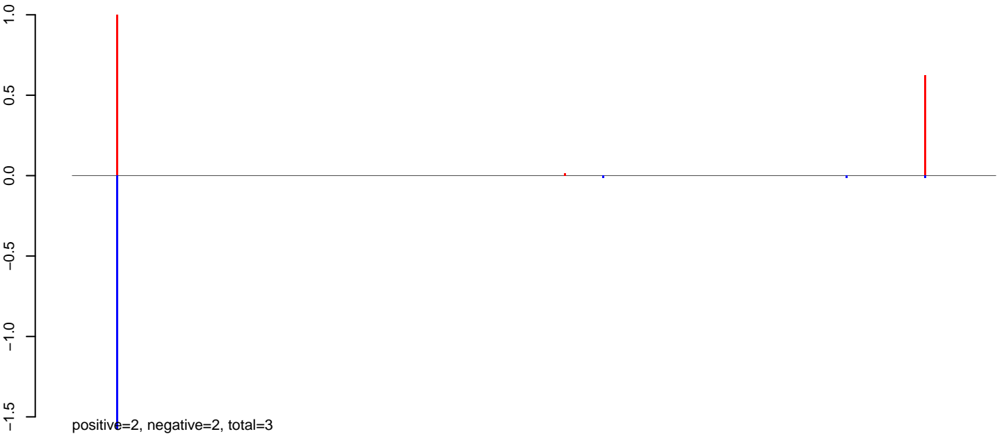
AeAlbo_CHIKV_9dpi.24_35.rep
