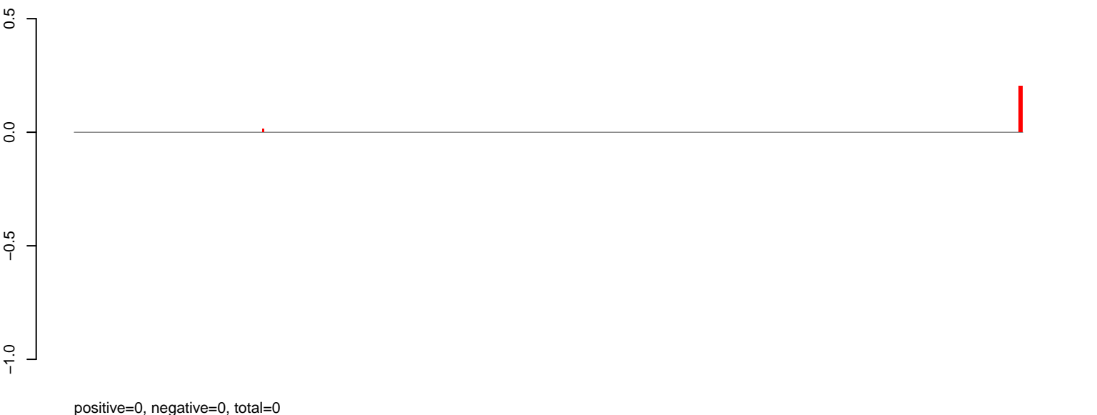
AeAlbo_CHIKV_9dpi.rep
