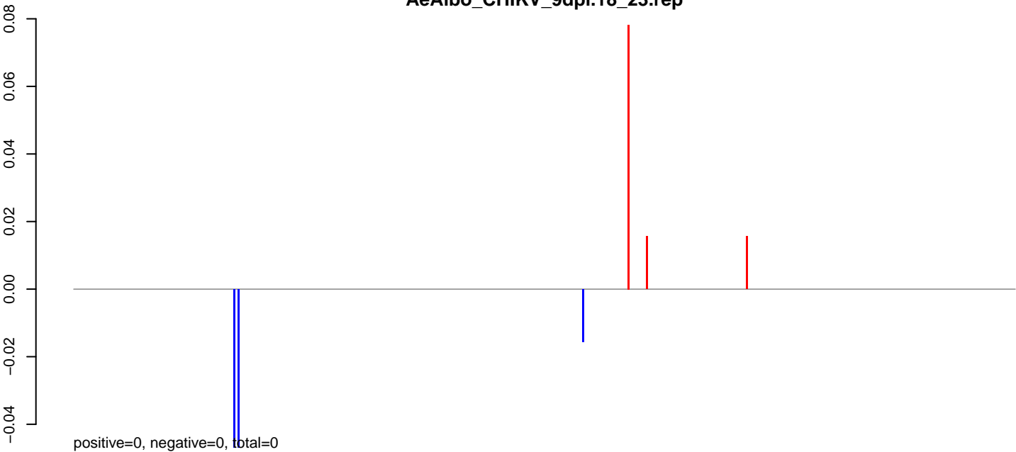
AeAlbo_CHIKV_9dpi.24_35.rep
