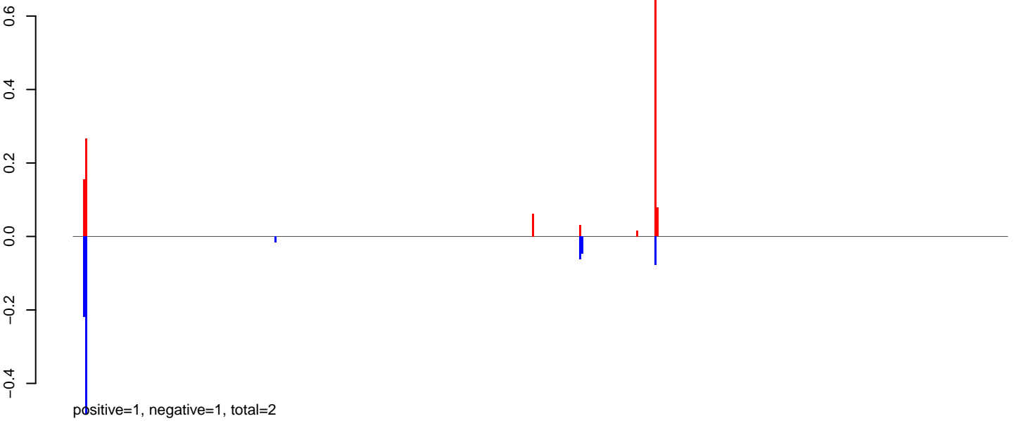
AeAlbo_CHIKV_9dpi.24_35.rep
