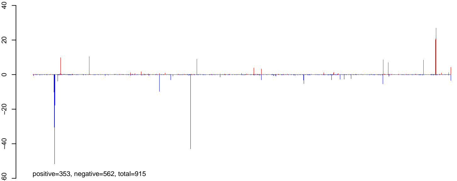
AeAlbo_CHIKV_AZT_3dpi.rep
