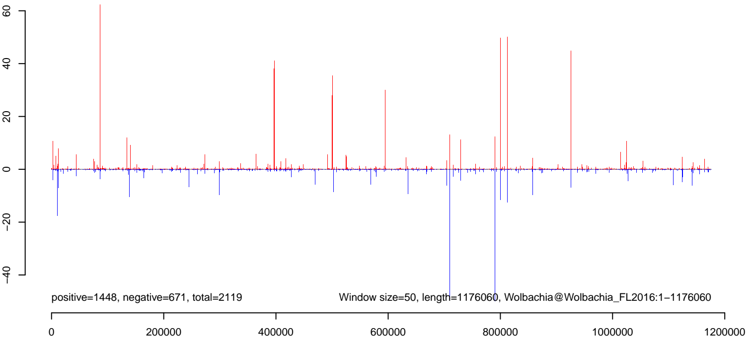
AeAlbo_CHIKV_AZT_3dpi.rep
