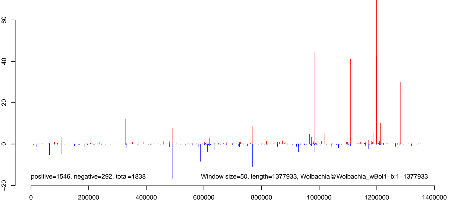
AeAlbo_CHIKV_AZT_3dpi.rep
