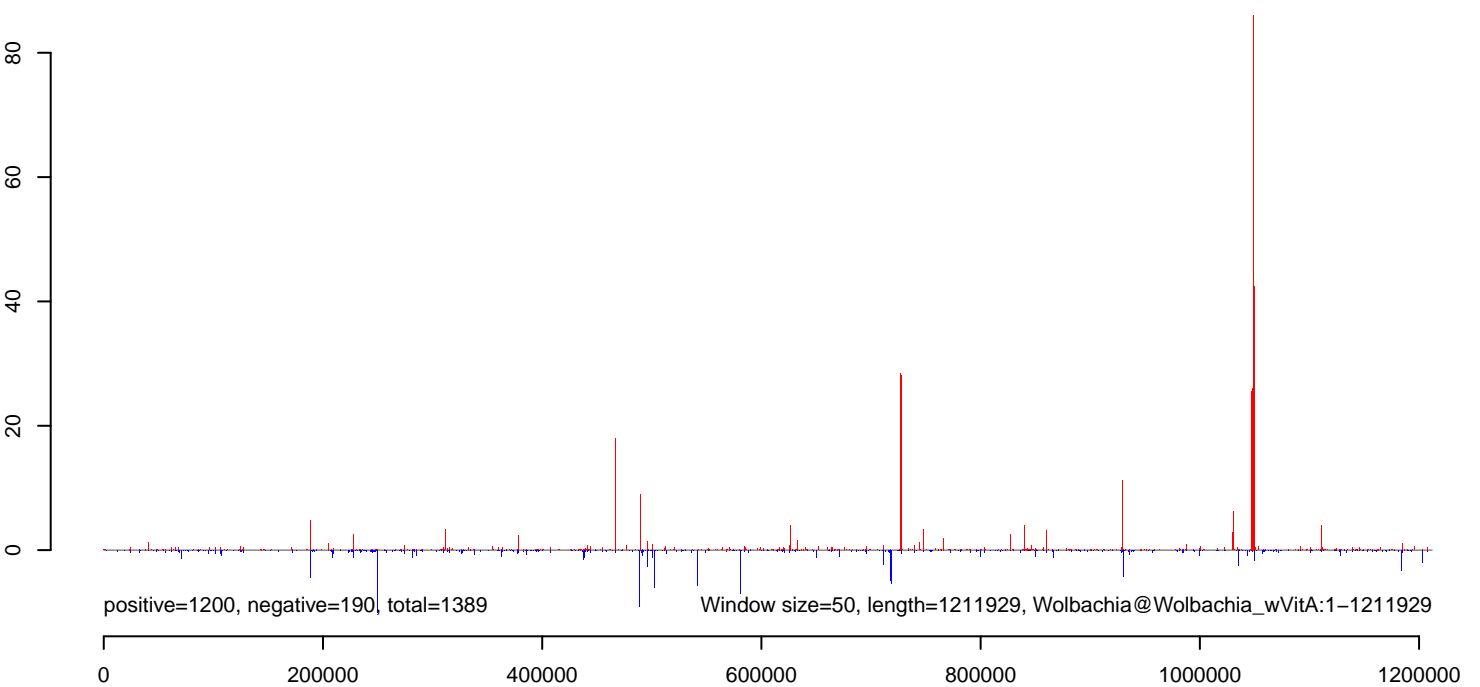
AeAlbo_CHIKV_AZT_3dpi.rep
