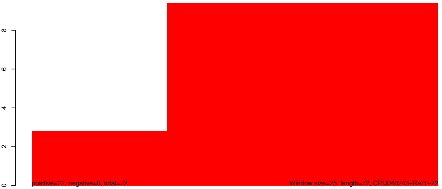
CuQuin_SG_14dpi2.rep
