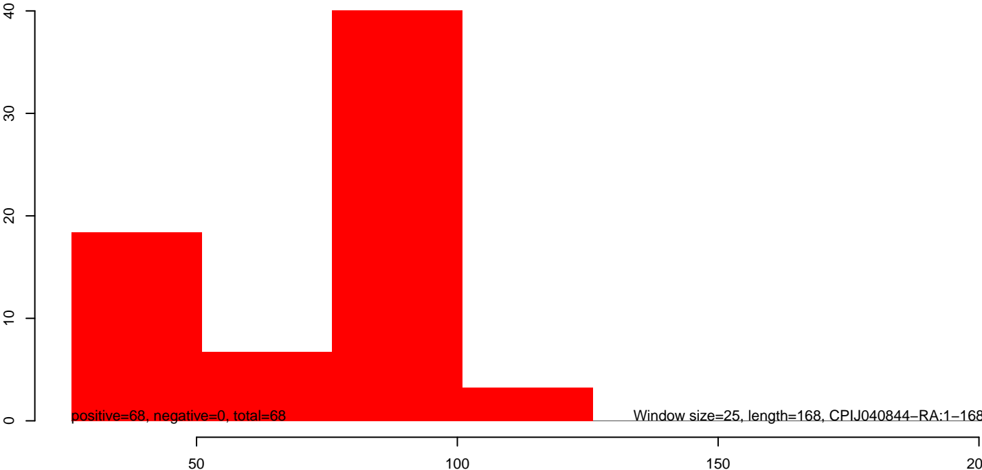
CuQuin_SG_14dpi2.rep
