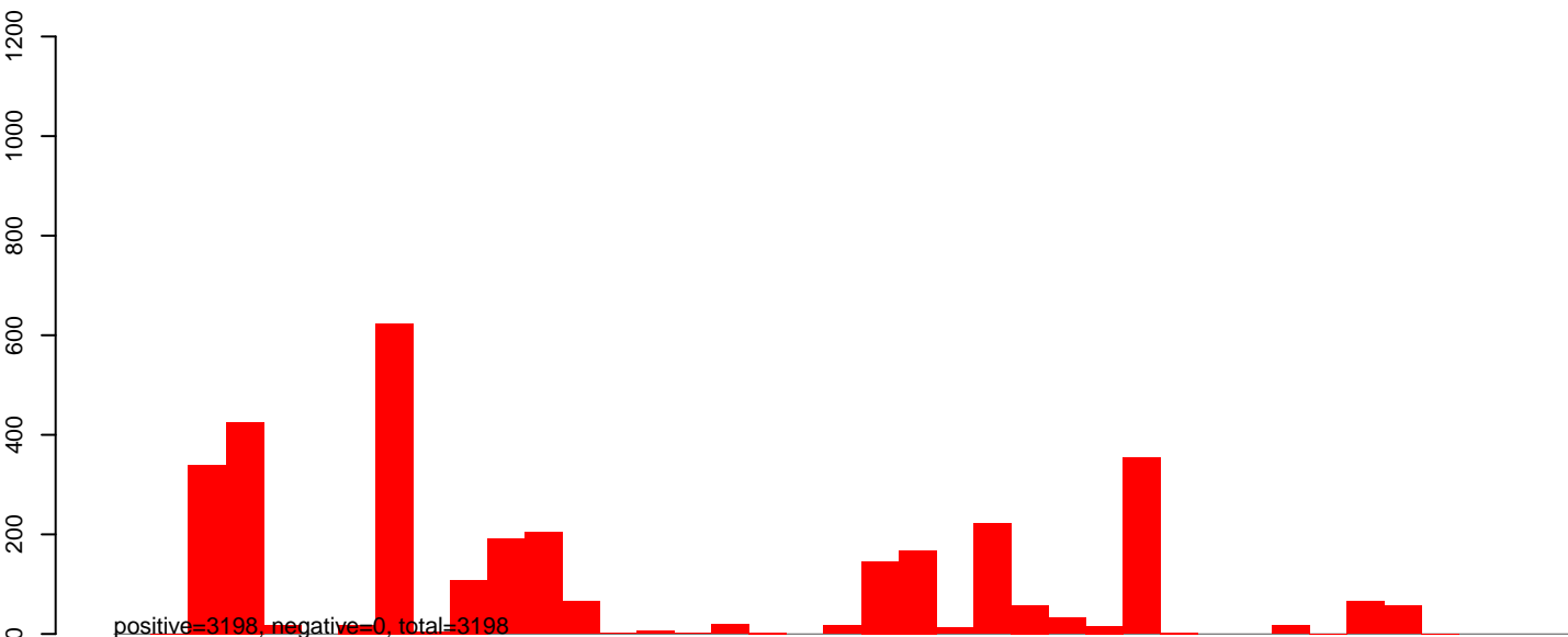
CuQuin_SG_14dpi2.rep
