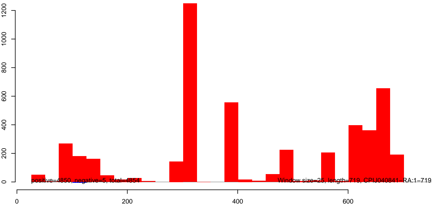
CuQuin_SG_14dpi2.rep
