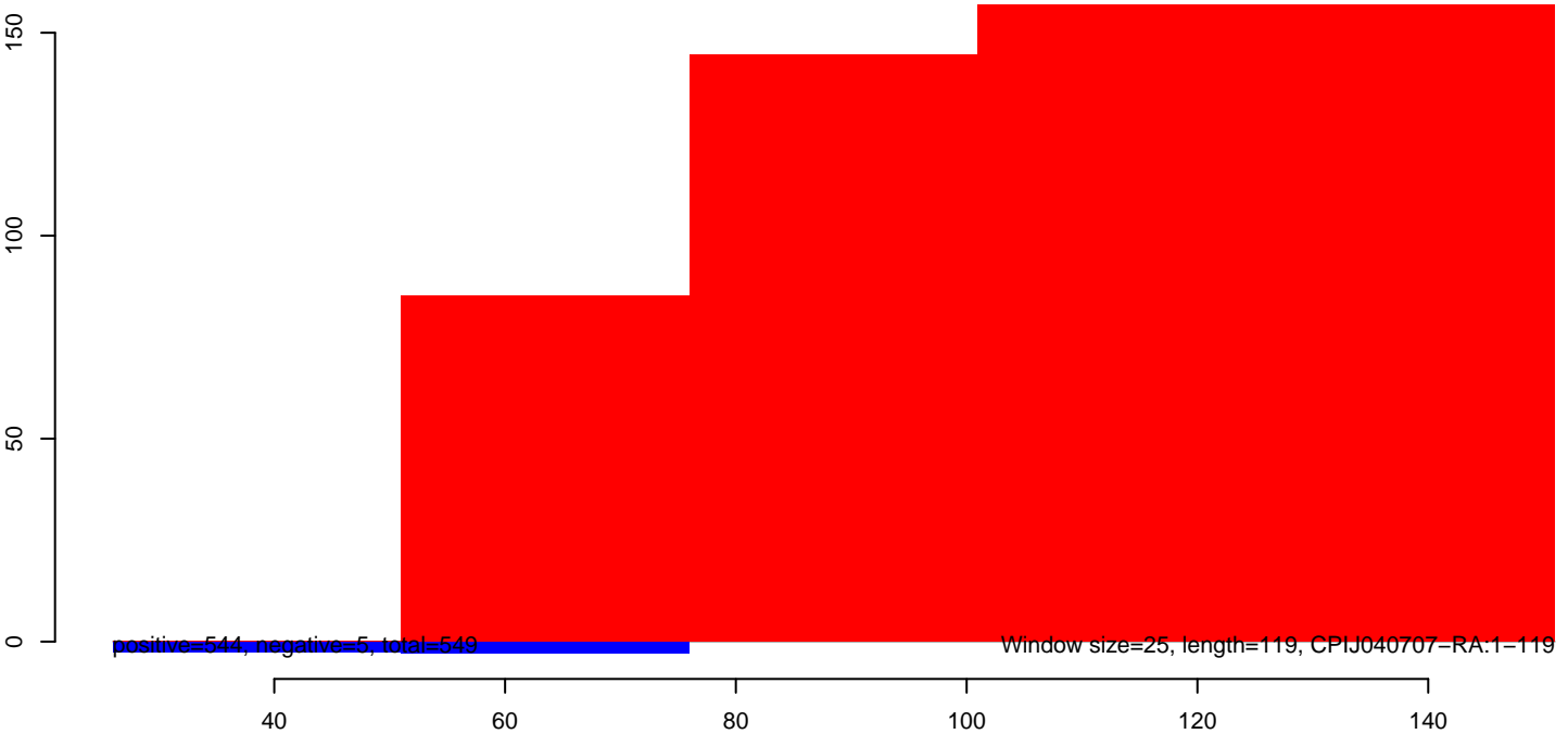
CuQuin_SG_14dpi2.rep
