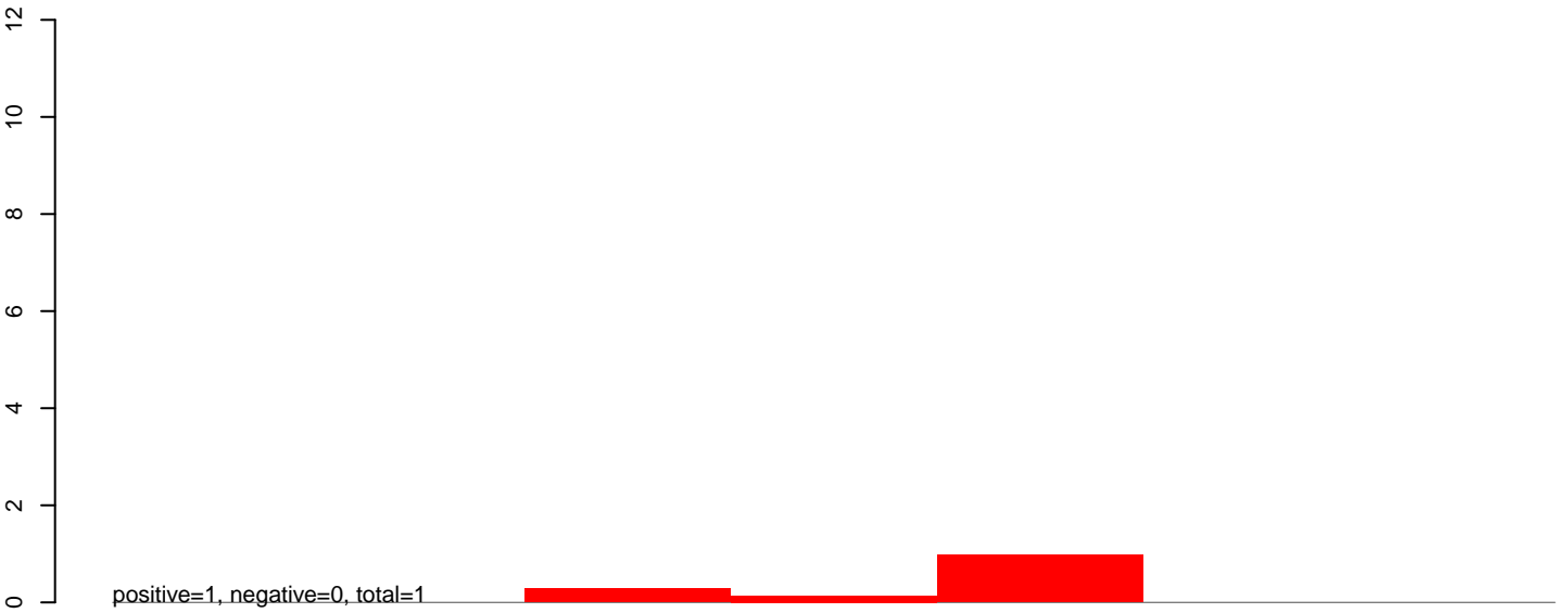
CuQuin_SG_14dpi2.rep
