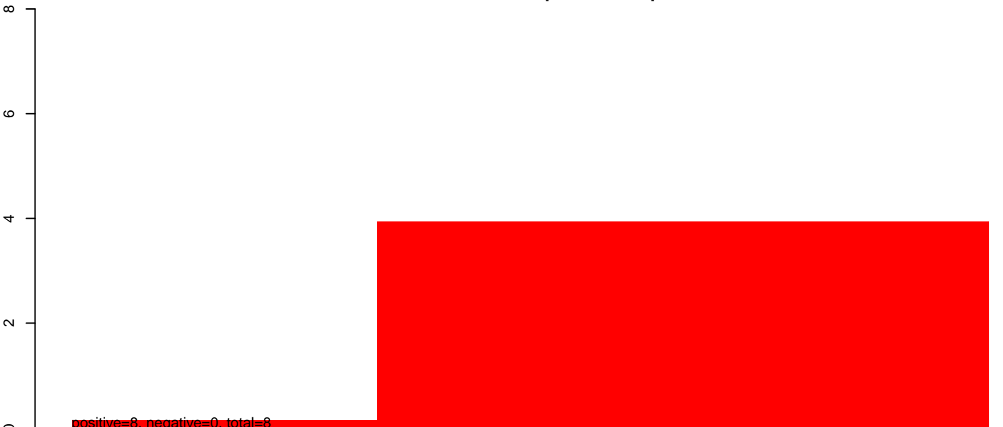
CuQuin_SG_14dpi2.rep
