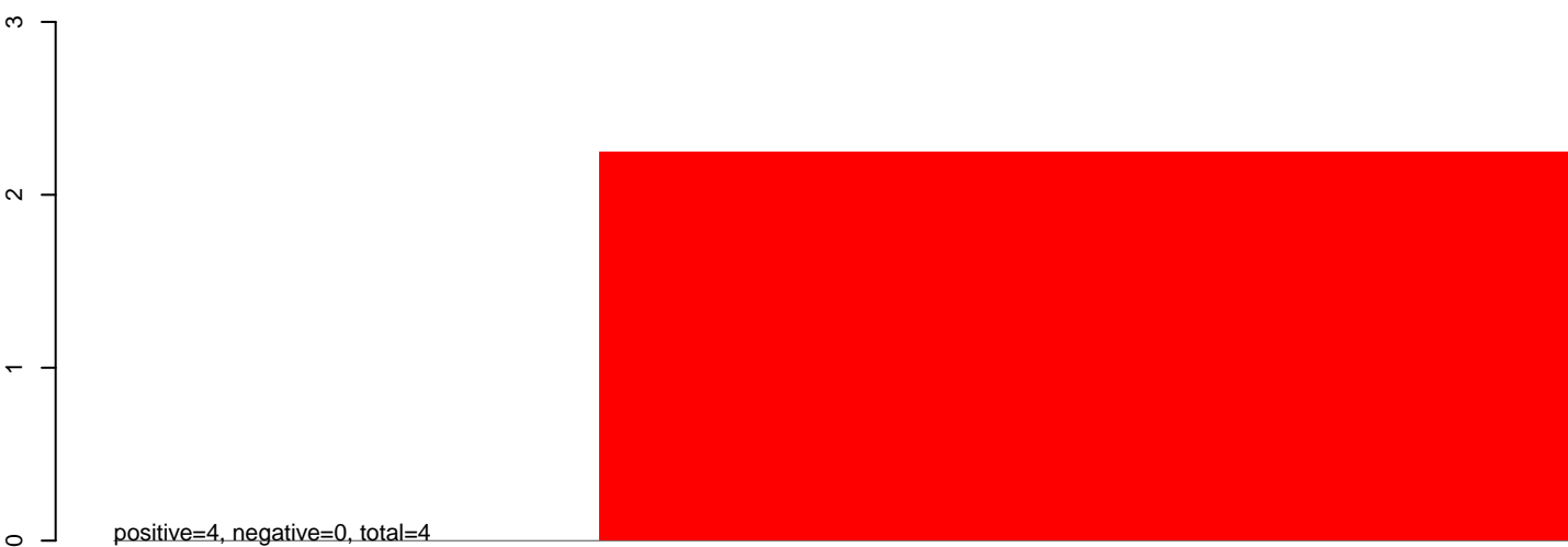
CuQuin_SG_14dpi2.rep
