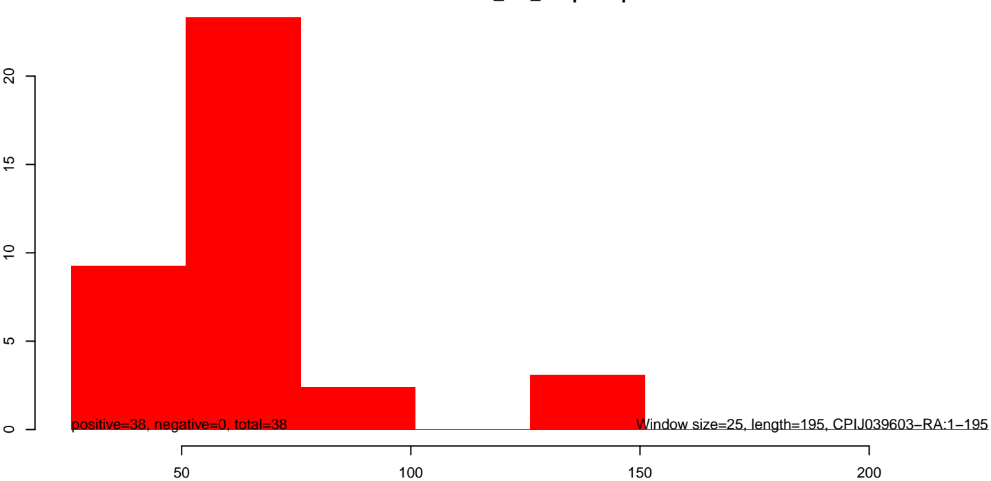
CuQuin_SG_14dpi2.rep
