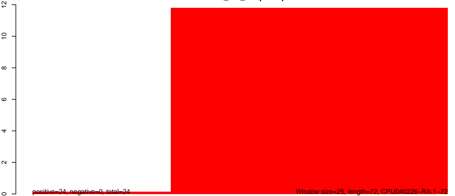
CuQuin_SG_14dpi2.rep
