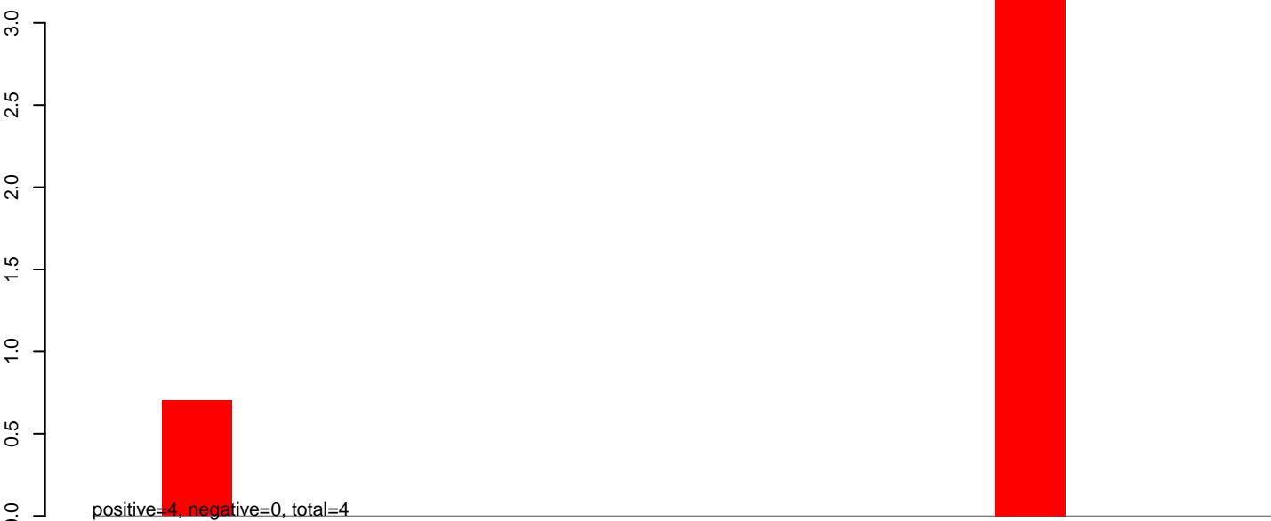
CuQuin_SG_14dpi2.rep
