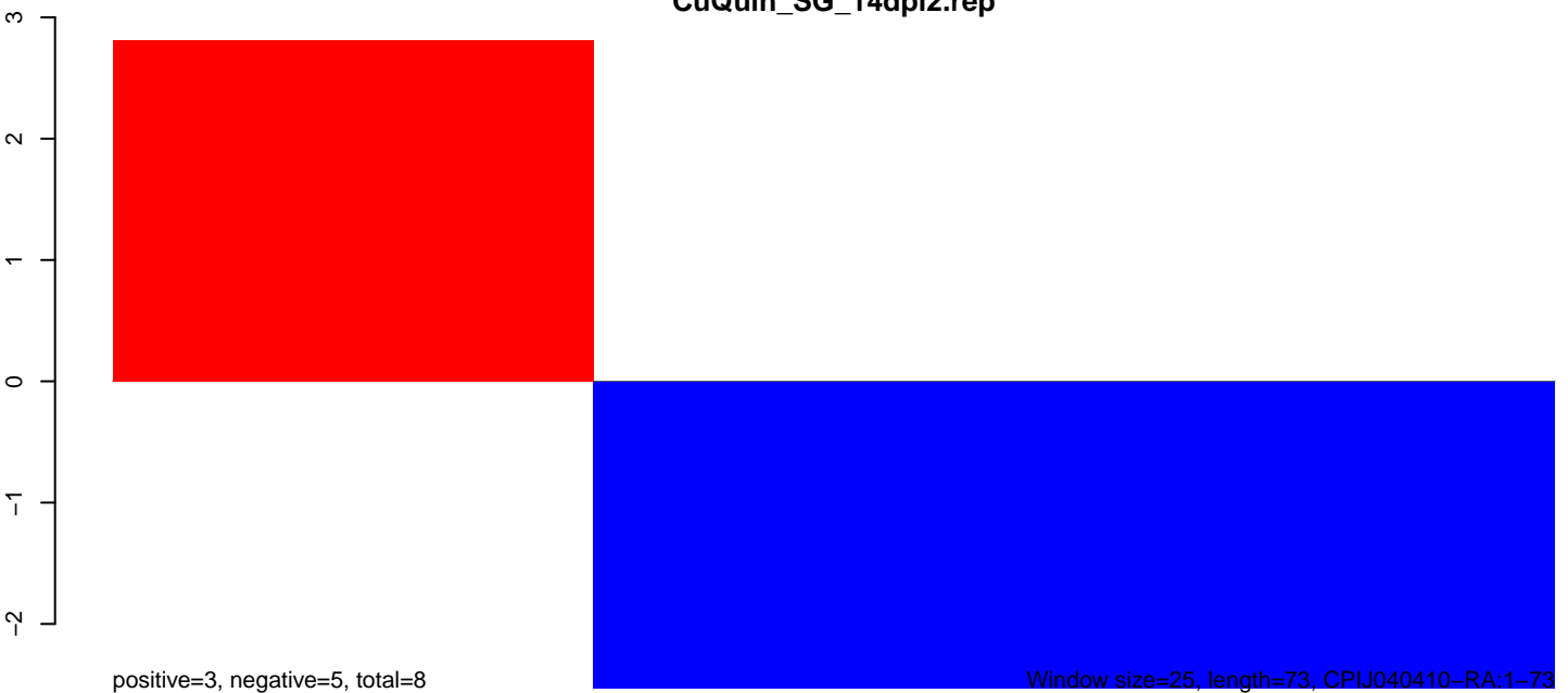
CuQuin_SG_14dpi2.rep
