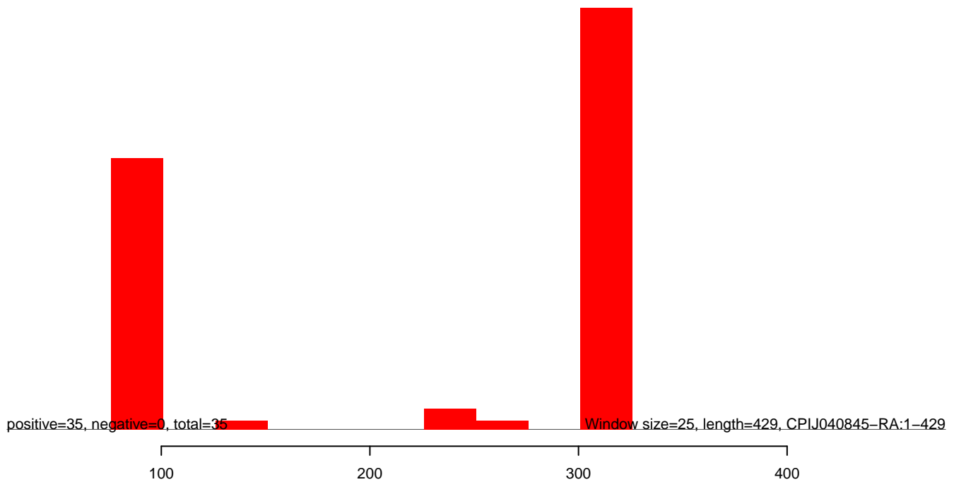
CuQuin_SG_14dpi2.rep
