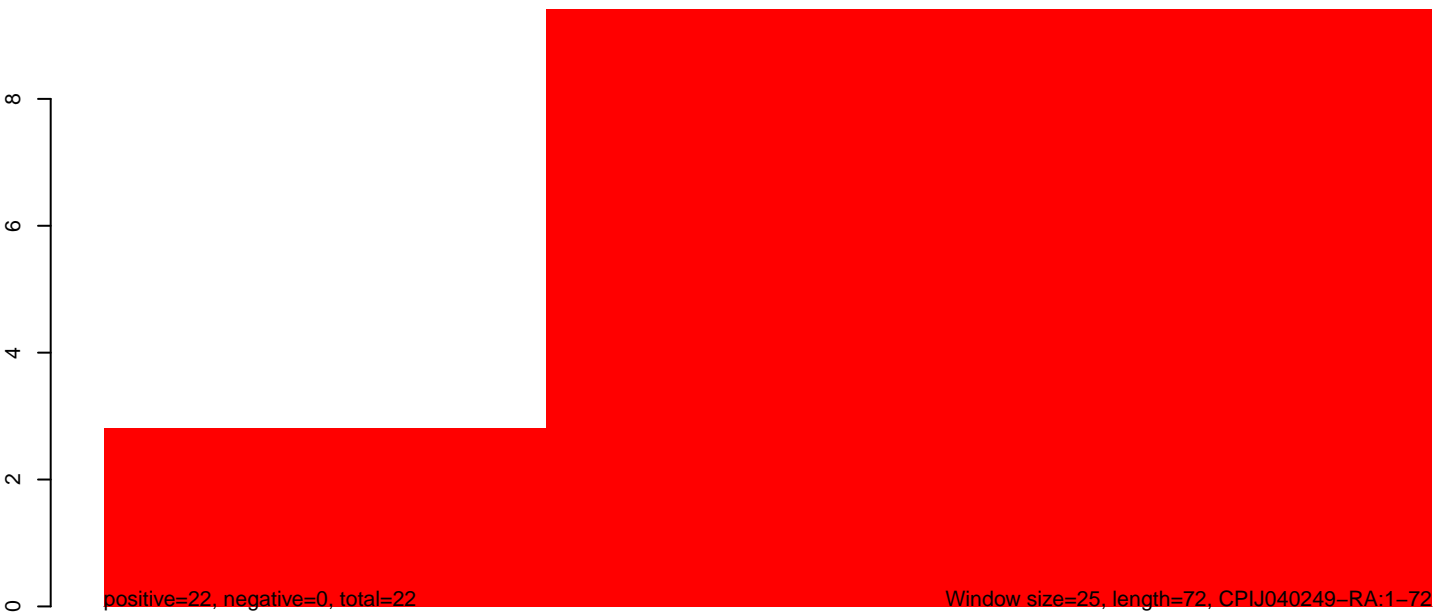
CuQuin_SG_14dpi2.rep
