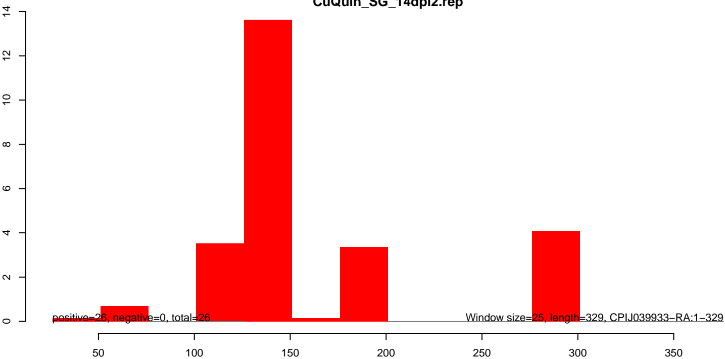
CuQuin_SG_14dpi2.rep
