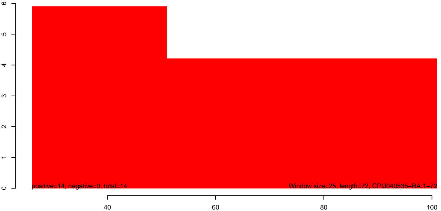
CuQuin_SG_14dpi2.rep
