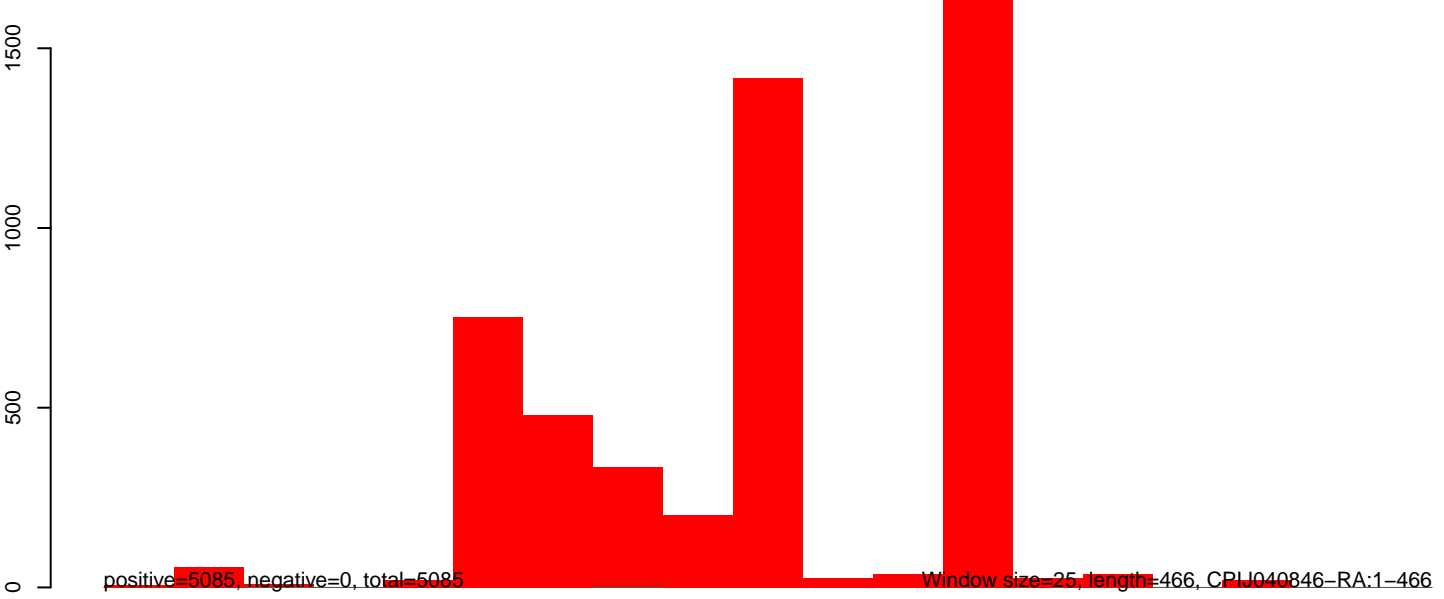
CuQuin_SG_14dpi2.rep
