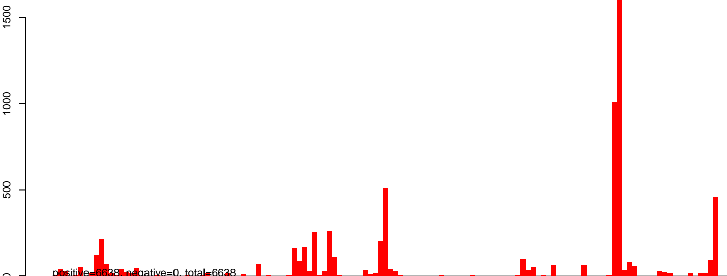
CuQuin_SG_14dpi2.rep
