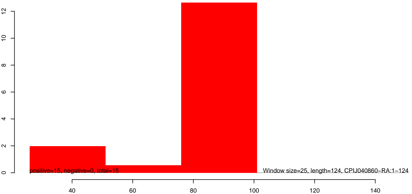
CuQuin_SG_14dpi2.rep
