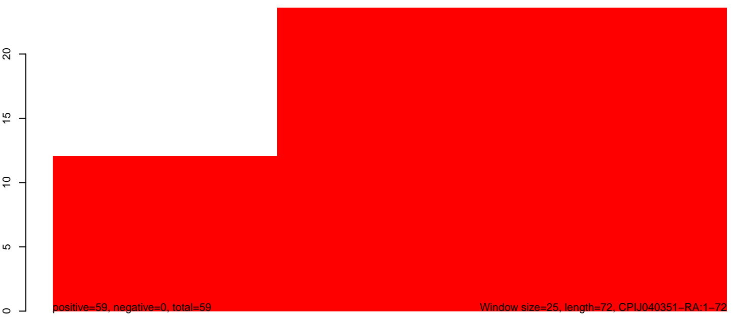
CuQuin_SG_14dpi2.rep
